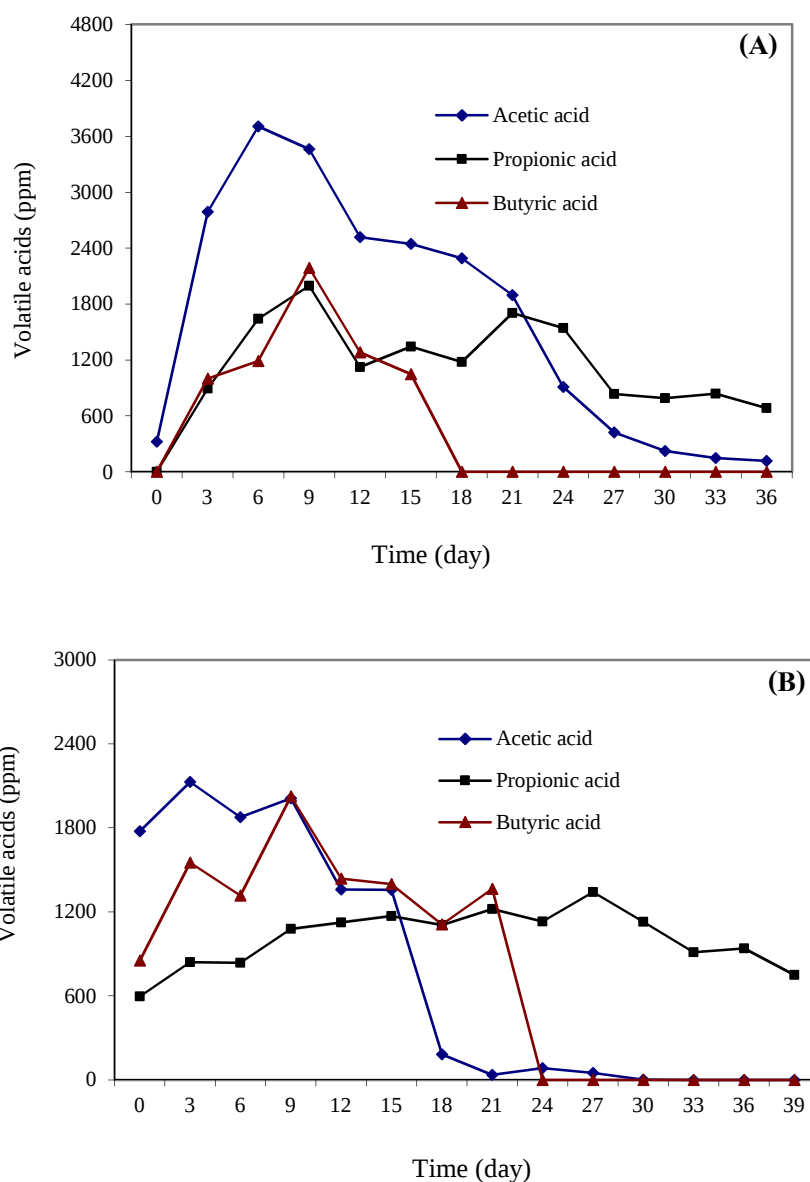
รูปที่ 3.21 Volatile fatty acids ที่สะสมระหว่างการผลิตก๊าซชีวภาพจากหัวมันสำปะหลังแห้งทั้งเปลือกพันธุ์ CMR 35-22-196 (หรือพันธุ์ระยอง 11) ที่มีความชื้น 17.34% ใช้ Total solids ปริมาณ 1.0% (น้ำหนักต่อปริมาตร) เติมนูเรีย 0.04% ใน Single-stage digester ที่มีปริมาตรหมัก 20 (A) และ 50 (B) ลิตร
