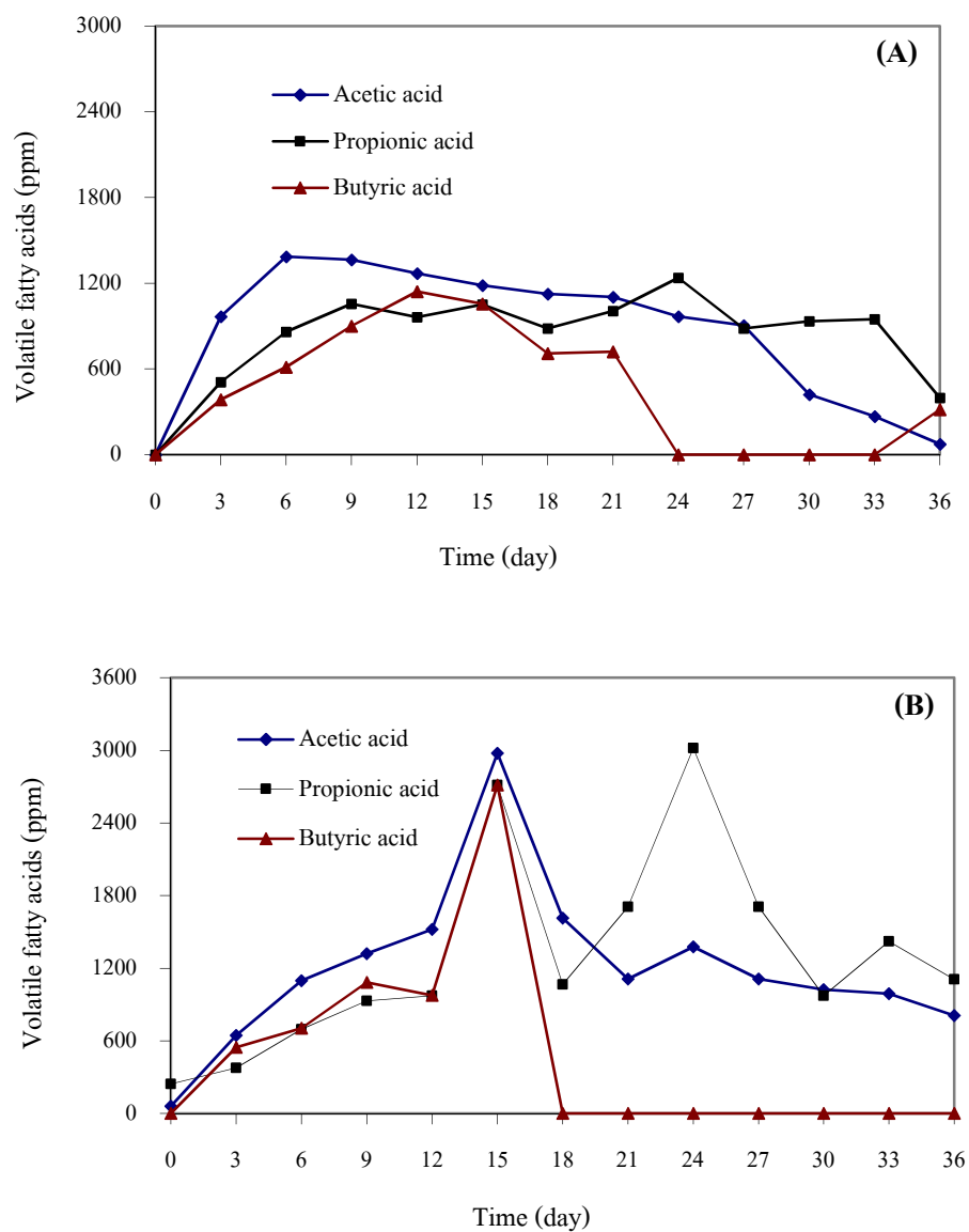
รูปที่ 3.27 Volatile fatty acids ที่สะสมระหว่างการผลิตก๊าซชีวภาพจากกากมันสำปะหลังแห้งที่มีความชื้น 15.19% ใช้ Total solids 1.0% (น้ำหนักต่อปริมาตร) เติมนูเรีย 0.04% ใน Single-stage digester ที่มีปริมาตรหมัก 20 (A) และ 50 (B) ลิตร
