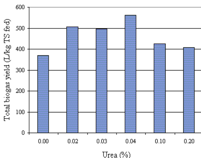
รูปที่ 3.15 ปริมาณก๊าซชีวภาพทั้งหมดที่ผลิตได้จากหัวมันสำปะหลังแห้งทั้งเปลือก (ความชื้น 17.34%) ที่ใช้ Total solids 1.0% (น้ำหนักต่อปริมาตร) และเติมยูเรียที่ความเข้มข้นต่างกันดังนี้ 0.00, 0.02, 0.03, 0.04, 0.10 และ 0.20% (น้ำหนักต่อปริมาตร) ใน Single-stage digester ปริมาตรหมัก 5 ลิตร
