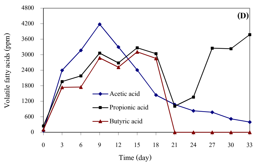
รูปที่ 3.17 (ต่อ) Volatile fatty acids ที่สะสมระหว่างการผลิตก๊าซชีวภาพจากกากมันสำปะหลังแห้งที่มีความชื้น 15.19% ใช้ Total solids ปริมาณ (% , น้ำหนักต่อปริมาตร) 0.5 (A), 1.0 (B), 1.5 (C) และ 2.0 (D) และเติมยูเรีย 0.04% ใน Single-stage digester ที่มีปริมาตรหมัก 10 ลิตร
