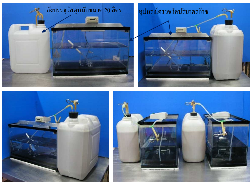
รูปที่ 3.9 ลักษณะของถังบรรจุวัสดุหมักปริมาตร 20 ลิตร ที่เตรียมเพื่อใช้ทดลองผลิตมีเทนจากกากมันสำปะหลัง และอุปกรณ์วัดปริมาตรก๊าซโดยการแทนที่น้ำ
