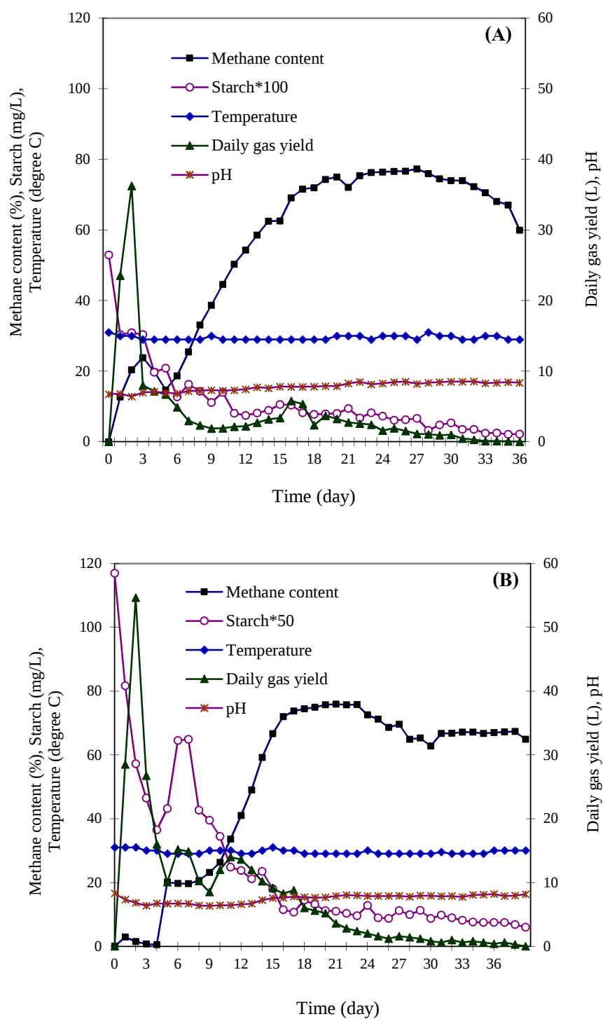
รูปที่ 3.19 การผลิตมีเทนในรูปก๊าซชีวภาพจากหัวมันสำปะหลังแห้งทั้งเปลือกพันธุ์ CMR 35-22-196 (หรือพันธุ์ระยะของ 11) ที่มีความชื้น 17.34% ใช้ Total solids ปริมาณ 1.0% (น้ำหนักต่อ ปริมาตร) เติมนูเรีย 0.04% ใน Single-stage digester ที่มีปริมาตรหมัก 20 (A) และ 50 (B) ลิตร
