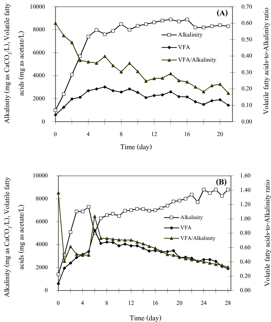
รูปที่ 3.18 Alkalinity และ Volatile fatty acids ที่เปลี่ยนแปลงระหว่างการผลิตก๊าซชีวภาพจากกากมันสำปะหลังแห้งที่มีความชื้น 15.19% ใช้ Total solids ปริมาณ (% , น้ำหนักต่อปริมาตร) 0.5 (A), 1.0 (B), 1.5 (C) และ 2.0 (D) และเติมยูเรีย 0.04% ใน Single-stage digester ที่มีปริมาตรหมัก 10 ลิตร
