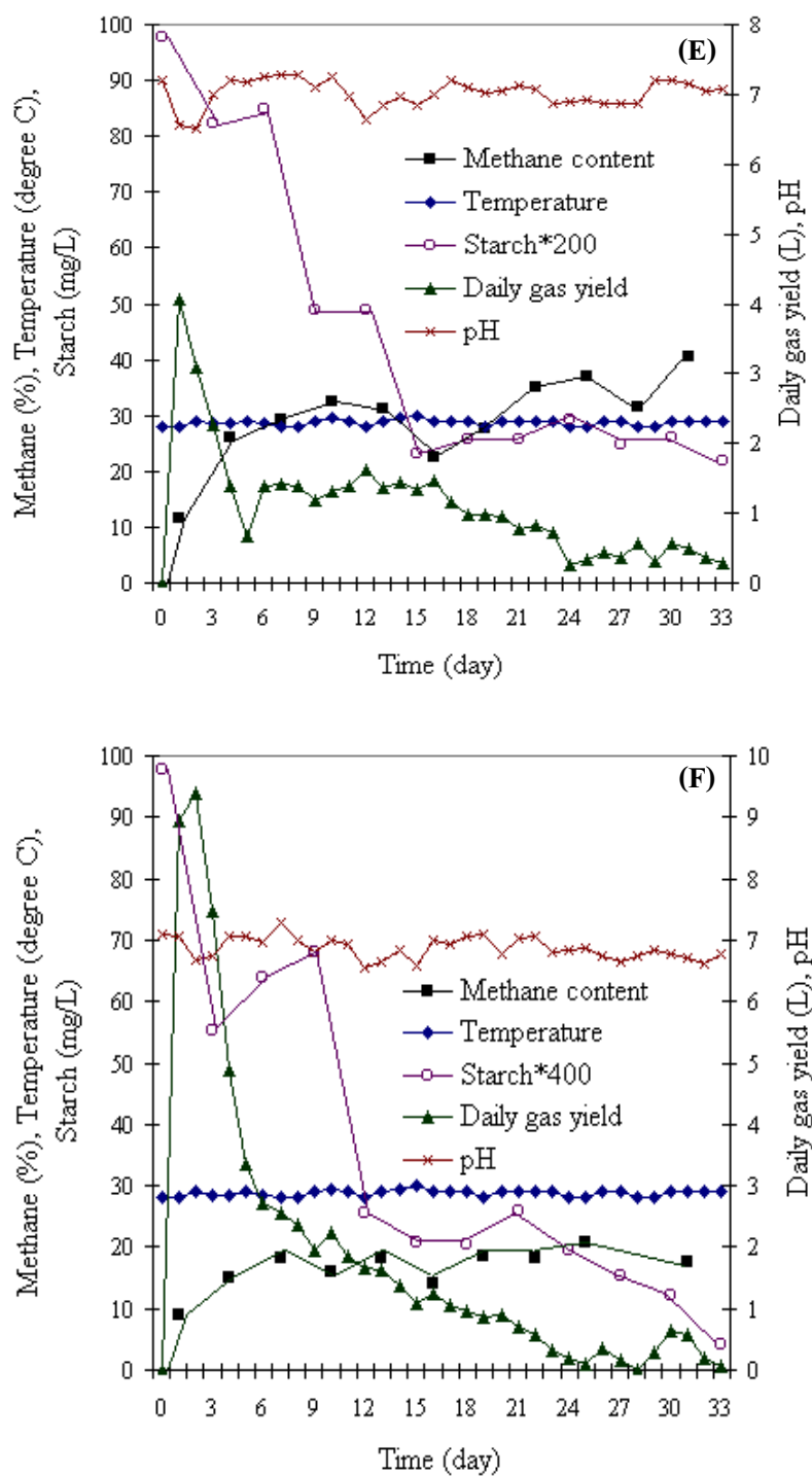
รูปที่ 3.12 (ต่อ) การผลิตมีเทนในรูปก๊าซชีวภาพจากหัวมันสำปะหลังแห้งทั้งเปลือก (ความชื้น 17.34%) ที่ใช้ Total solids ปริมาณ (% , น้ำหนักต่อปริมาตร) แตกต่างกันดังนี้ 0.25 (A), 0.5 (B), 1.0 (C), 2.0 (D), 4.0 (E), 8.0 (F) และ 16.0 (G) ใน Single-stage digester ปริมาตรหมัก 5 ลิตร
