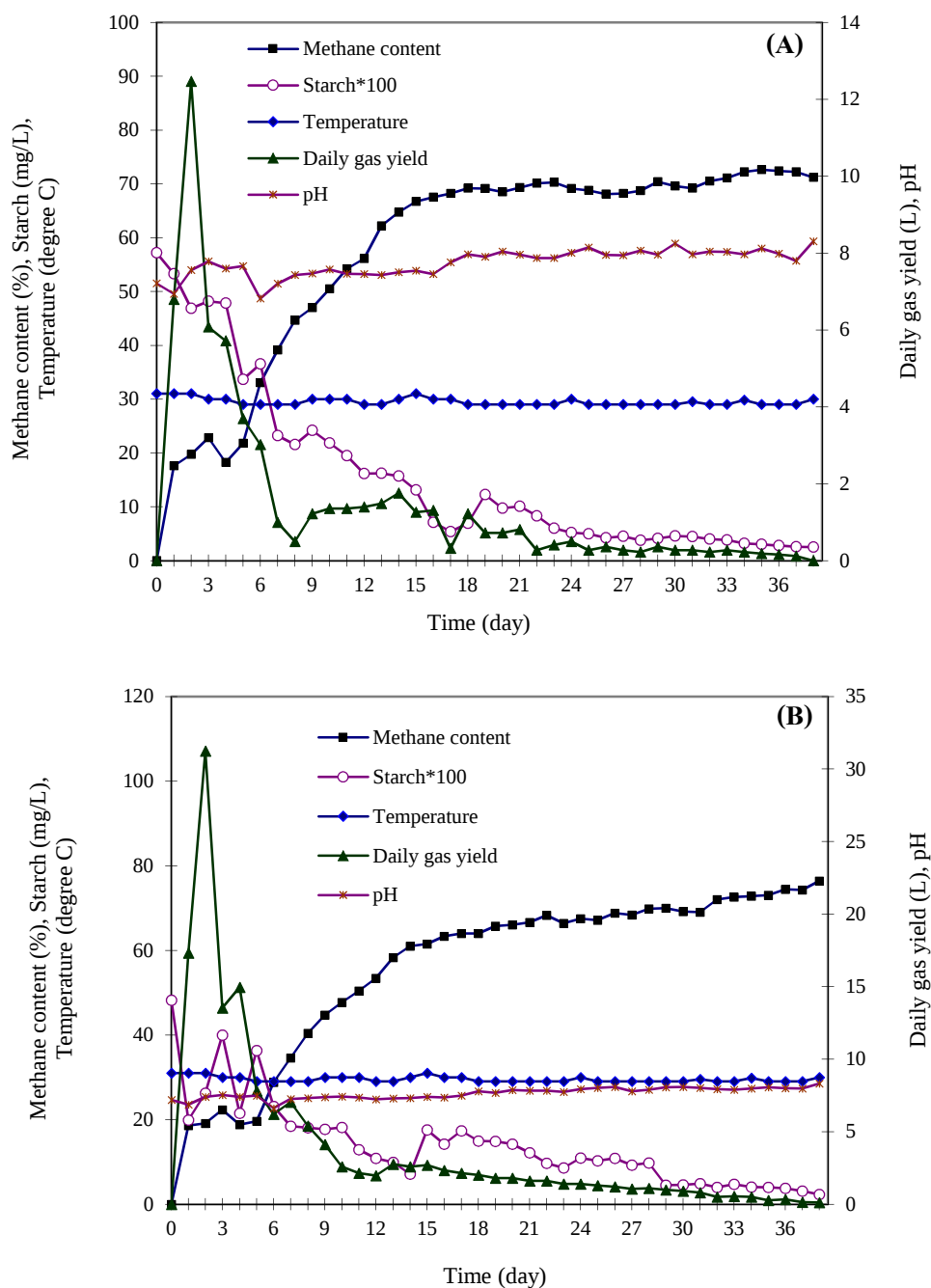
รูปที่ 3.26 การผลิตมีเทนในรูปแบบก๊าซชีวภาพจากกากมันสำปะหลังแห้งที่มีความชื้น 15.19% ใช้ Total solids 1.0% (น้ำหนักต่อปริมาตร) เติมนูเรีย 0.04% ใน Single-stage digester ที่มีปริมาตรหมัก 20 (A) และ 50 (B) ลิตร
