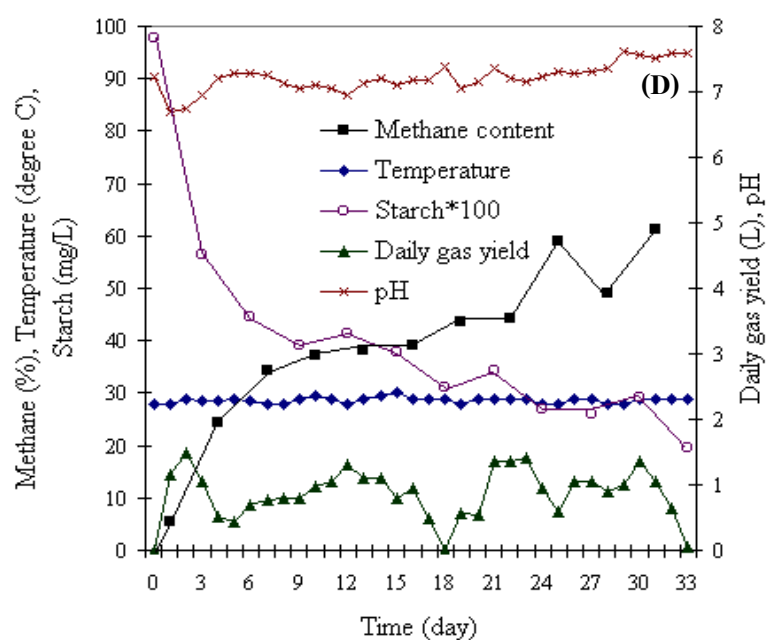
รูปที่ 3.12 (ต่อ) การผลิตมีเทนในรูปก๊าซชีวภาพจากหัวมันสำปะหลังแห้งทั้งเปลือก (ความชื้น 17.34%) ที่ใช้ Total solids ปริมาณ (% , น้ำหนักต่อปริมาตร) แตกต่างกันดังนี้ 0.25 (A), 0.5 (B), 1.0 (C), 2.0 (D), 4.0 (E), 8.0 (F) และ 16.0 (G) ใน Single-stage digester ปริมาตรหมัก 5 ลิตร
