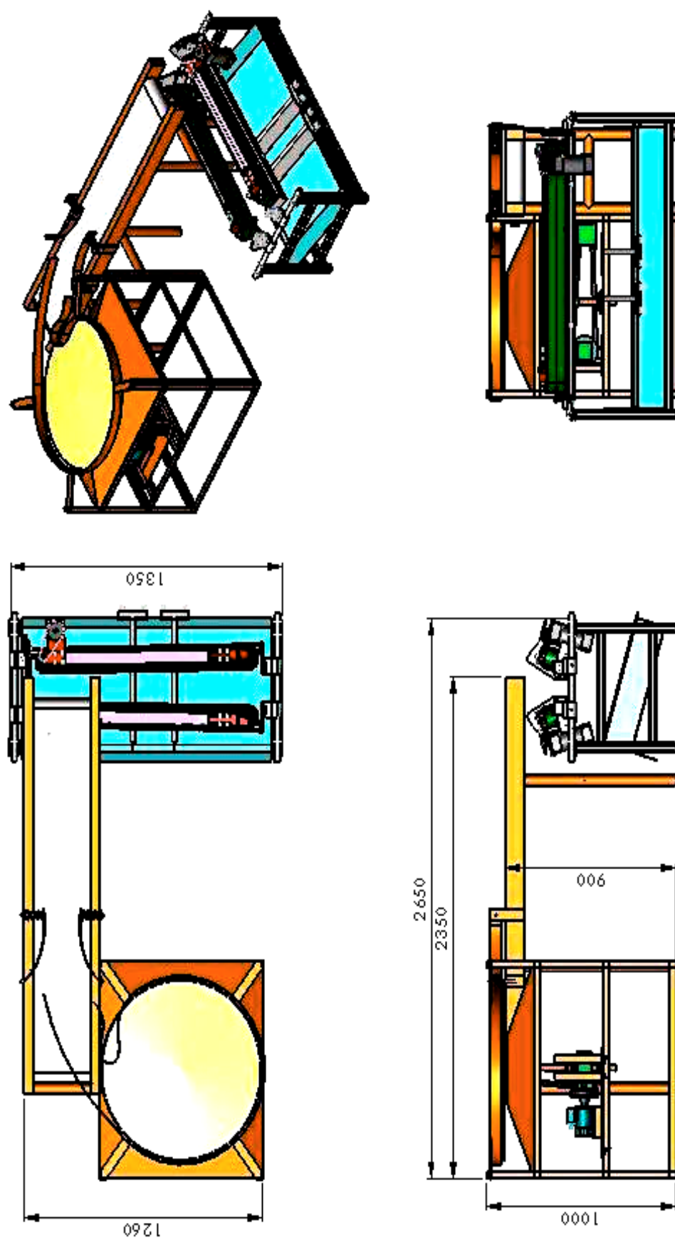
ภาพผนวกที่ 3 "โดยะแกรมภาพด้านต่าง ๆ ของเครื่องคัดขนาดและเครื่องป้อนผลส้มโอ
