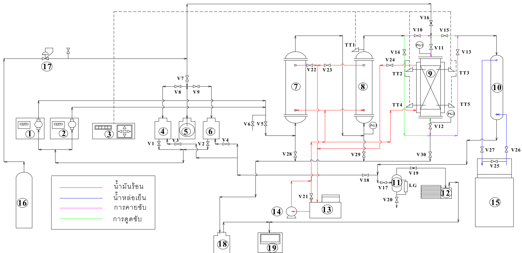
ภาพที่ 39 แผนภาพแสดงอุปกรณ์ของชุดทดสอบสารดูดซับในกระบวนการผลิตเอทานอลใรน้ำที่ใช้ในงานวิจัย
