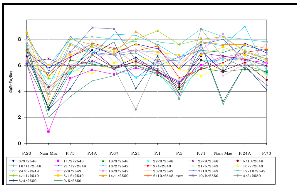
ภาพที่ 20 การเปลี่ยนแปลงค่า DO ของทุกจุดตรวจวัดจากต้นน้ำถึงท้ายน้ำสำหรับแต่ละเหตุการณ์
