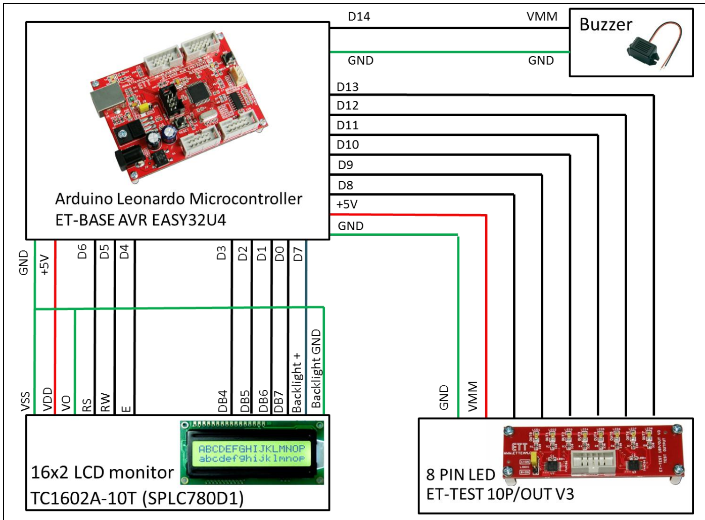
รูปที่ ๓.1 วงจรของ Pos-Monitor
