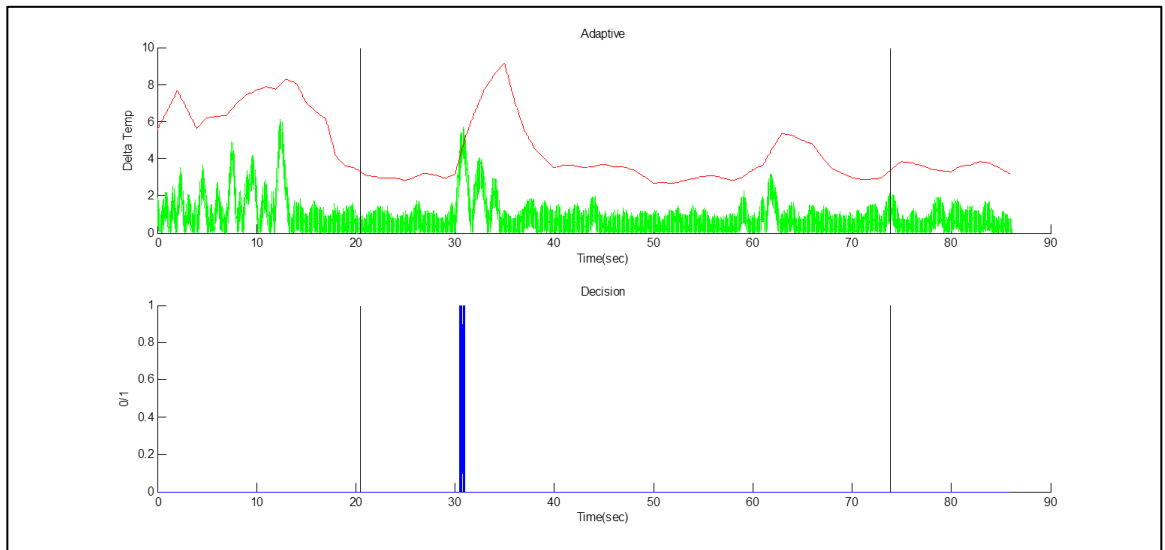
รูปที่ ก.6 ผลที่ได้จากระบบการเปลี่ยนเฟสแบบอัตโนมัติของ Incoloy 800H
