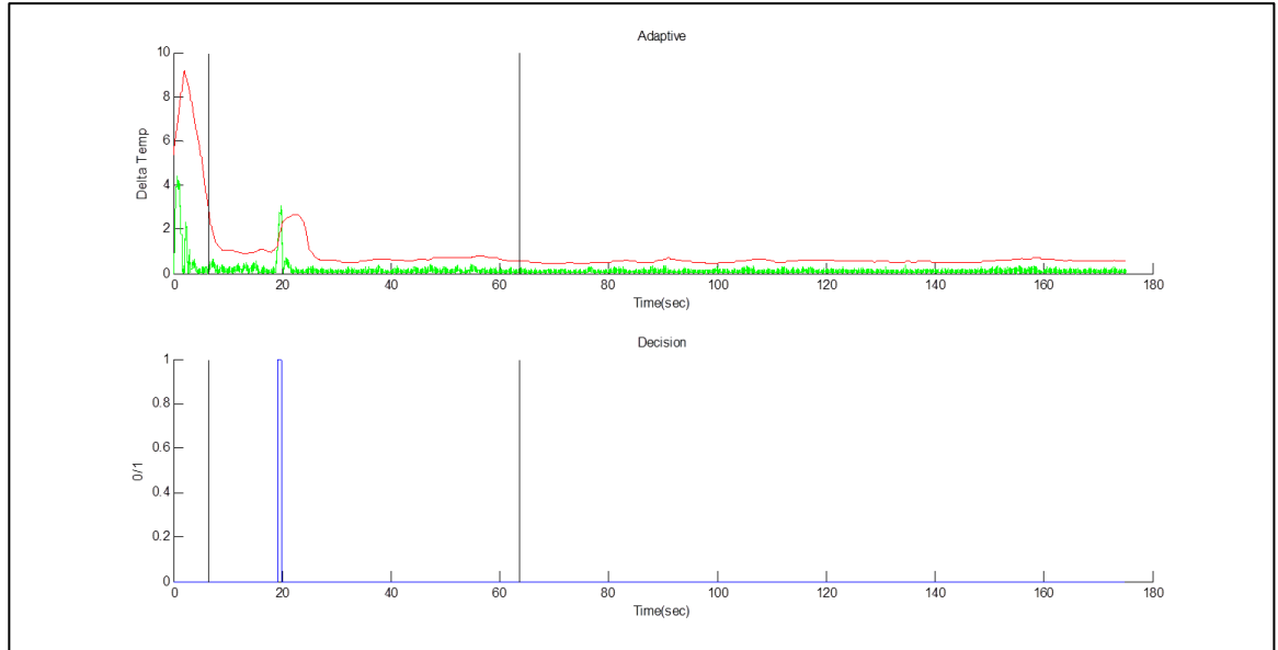
รูปที่ ก.1 ผลที่ได้จากระบบการเปลี่ยนเฟสแบบอัตโนมัติของสแตนเลส SUS321
