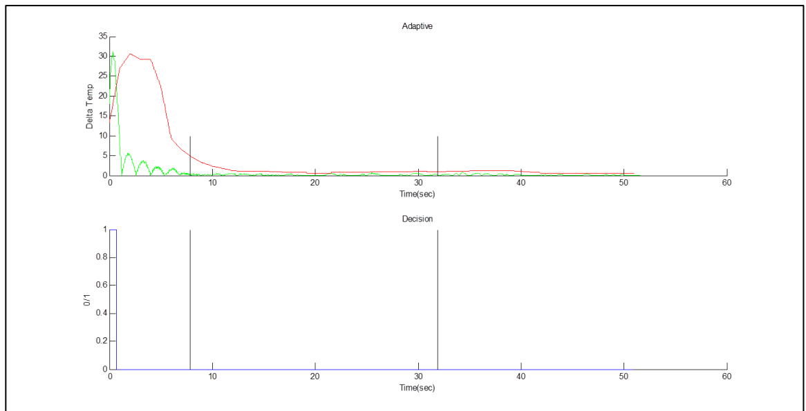
รูปที่ ก.2 ผลที่ได้จากระบบการเปลี่ยนเฟสแบบอัตโนมัติของสแตนเลส SUS321
