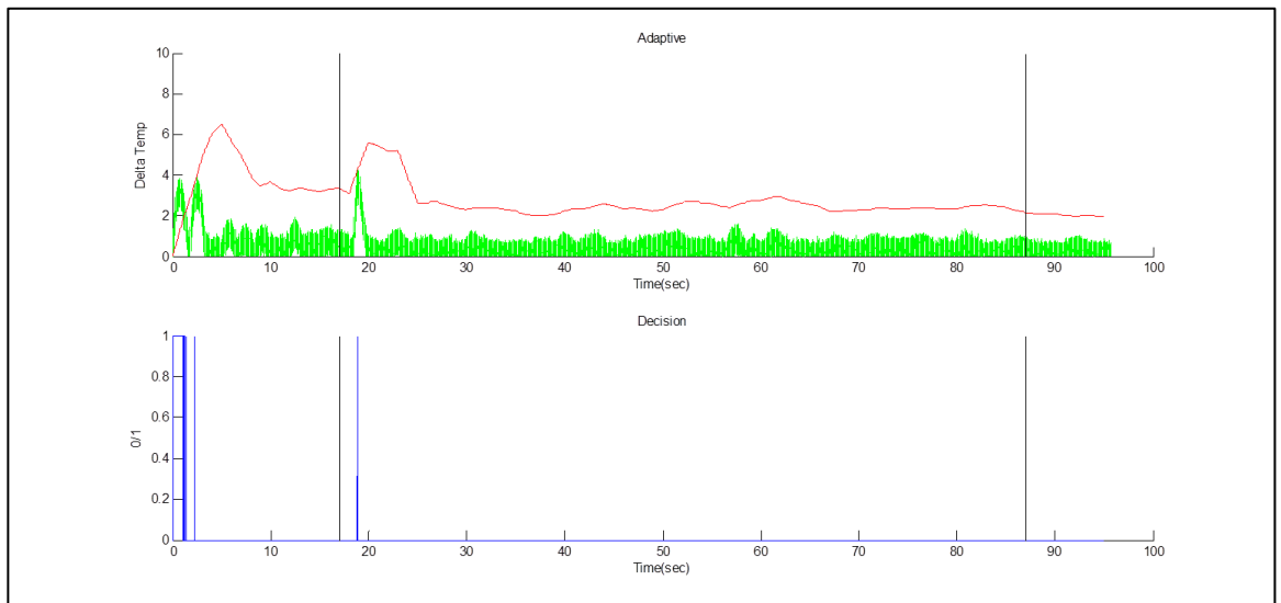
รูปที่ ก.4 ผลที่ได้จากระบบการเปลี่ยนเฟสแบบอัตโนมัติของ alloy617
