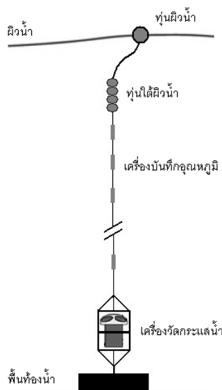
ภาพที่ 3 ลักษณะการติดตั้งเครื่องวัดกระแสไฟฟ้าและเครื่องบันทึกอุณหภูมิตื้นน้ำที่สถานีตรวจวัด
