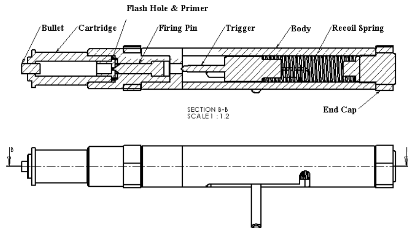
รูปที่ ก.1 ชุดปล่อยกระสุนปืน (launcher หรือ powder gun)
