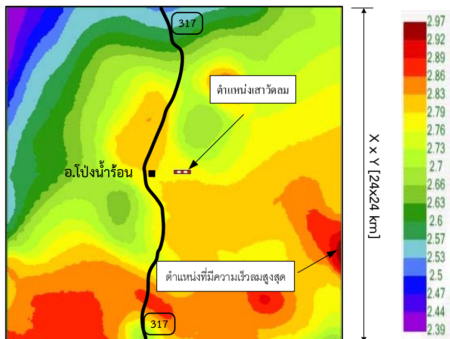
รูปที่ 211 แผนที่ศักยภาพพลังงานลมของพื้นที่ที่ติดตั้งเสาวัดลมที่ ต.ทับไทร อ.โป่งน้ำร้อน จ.จันทบุรี ที่ระดับความสูง 10 เมตร หน่วย ( W/m^2 )
