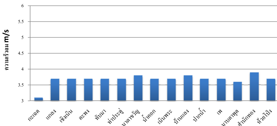
รูปที่ 32 กราฟแสดงค่าความเร็วลมเฉลี่ยของตำบลต่างๆ ในอำเภอเมือง
