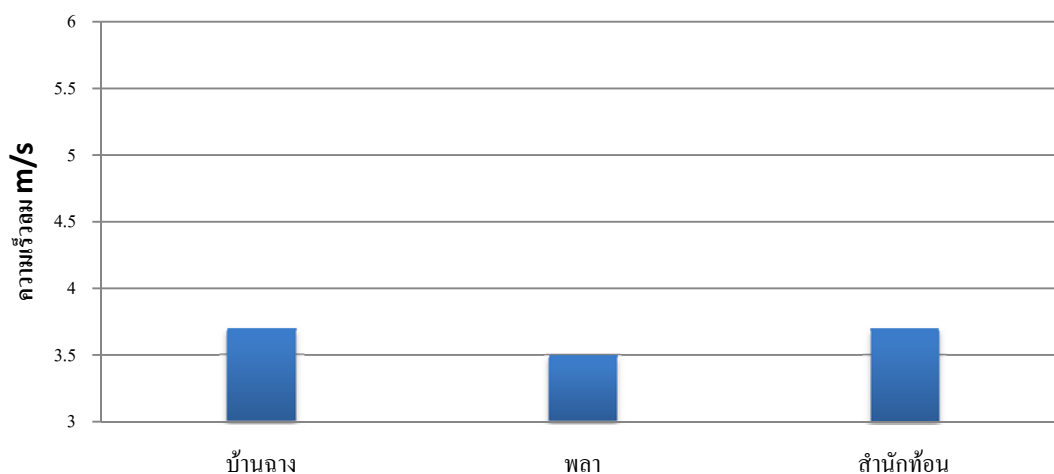
รูปที่ 30 กราฟแสดงค่าความเร็วลมเฉลี่ยของตำบลต่างๆ ในอำเภอบ้านฉาง
