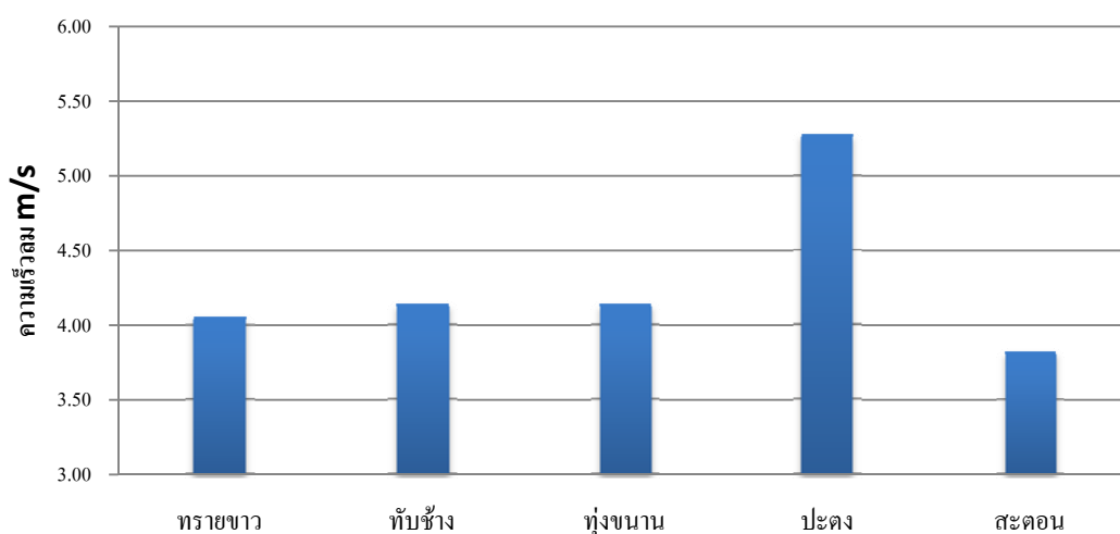
รูปที่ 47 กราฟแสดงค่าความเร็วลมเฉลี่ยของตำบลต่าง ๆ ในอำเภอสอยดาว
