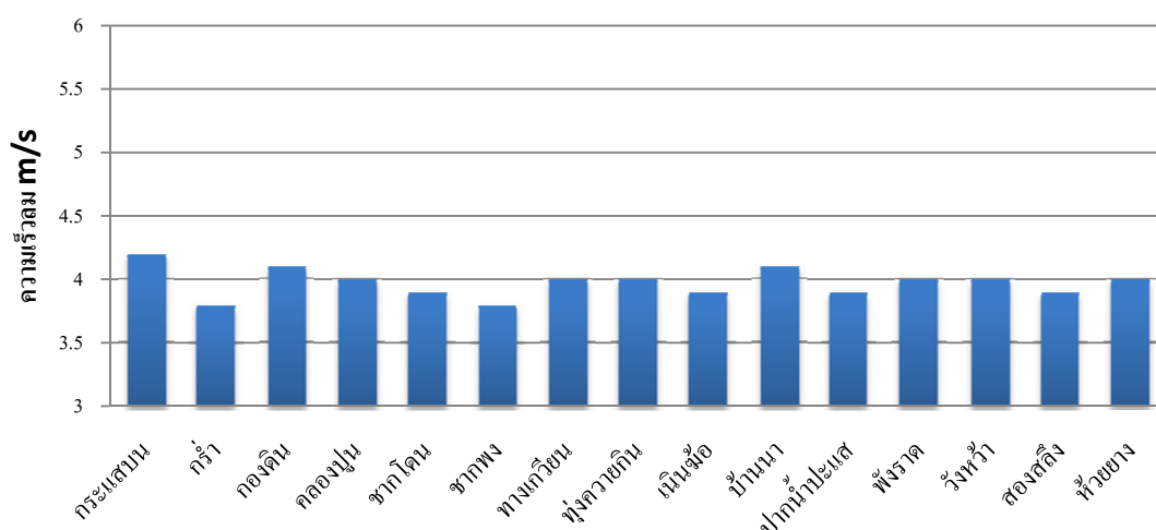
รูปที่ 26 กราฟแสดงค่าความเร็วลมเฉลี่ยของตำบลต่างๆ ในอำเภอแกลง
