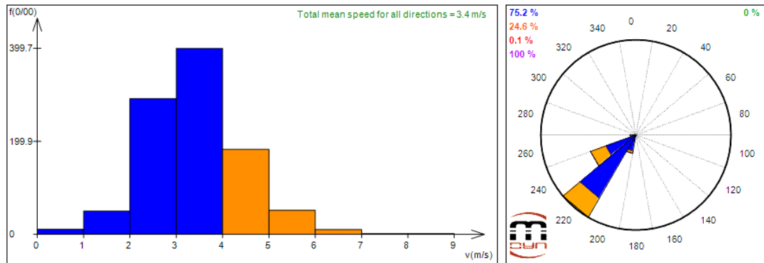
รูปที่ 168 กราฟการกระจายความเร็วลมสำหรับข้อมูลลมเฉลี่ยทุกๆ 10 นาที ของสถานีวัดลมที่ ต.ทับไทร อ. โป่งน้ำร้อน จ. จันทบุรี ที่ระดับความสูง 10 เมตร เดือน มิถุนายน 2555
