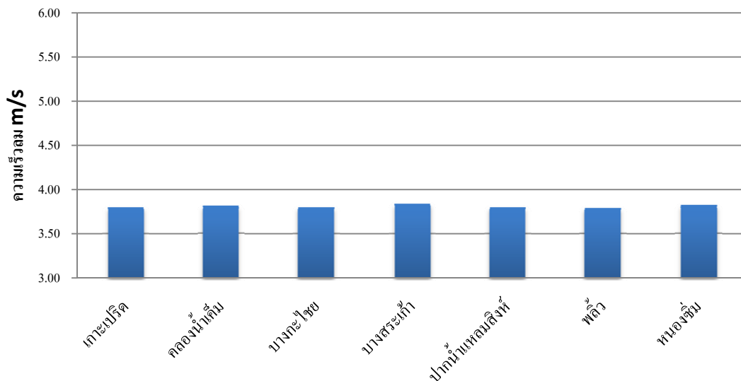
รูปที่ 48 กราฟแสดงค่าความเร็วลมเฉลี่ยของตำบลต่างๆ ในอำเภอสหัสขันธ์
