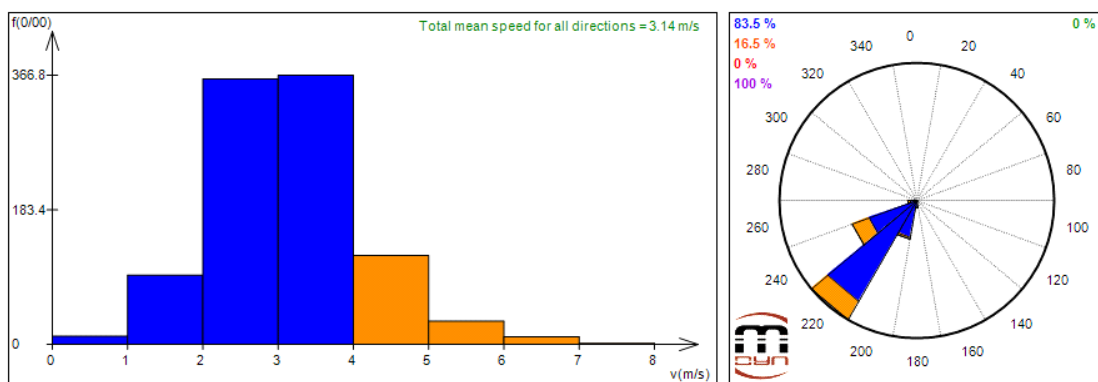
รูปที่ 172 กราฟการกระจายความเร็วลมสำหรับข้อมูลลมเฉลี่ยทุกๆ 10 นาที ของสถานีวัดลมที่ ต.ทับไทร อ. โป่งน้ำร้อน จ. จันทบุรี ที่ระดับความสูง 10 เมตร เดือน กรกฎาคม 2555
