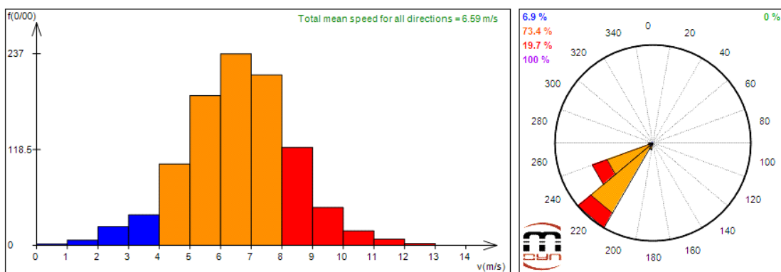
รูปที่ 173 กราฟการกระจายความเร็วลมสำหรับข้อมูลลมเฉลี่ยทุกๆ 10 นาที ของสถานีวัดลมที่ ต.ทับไทร อ. โป่งน้ำร้อน จ. จันทบุรี ที่ระดับความสูง 65 เมตร เดือน กรกฎาคม 2555
