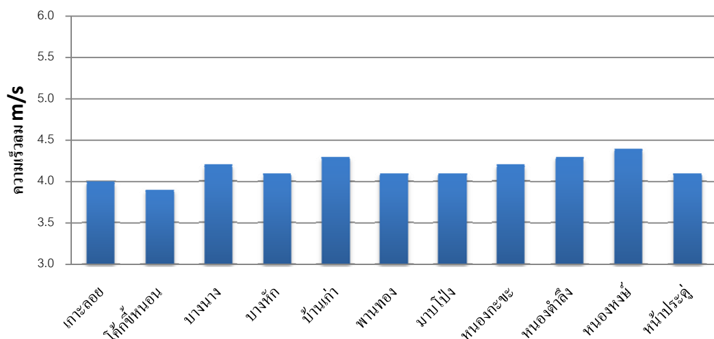
รูปที่ 14 กราฟแสดงค่าความเร็วลมเฉลี่ยของตำบลต่างๆ ในอำเภอนาทอง
