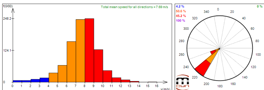
รูปที่ 170 กราฟการกระจายความเร็วลมสำหรับข้อมูลลมเฉลี่ยทุกๆ 10 นาที ของสถานีวัดลมที่ ต.ทับไทร อ. โป่งน้ำร้อน จ. จันทบุรี ที่ระดับความสูง 90 เมตร เดือน มิถุนายน 2555
