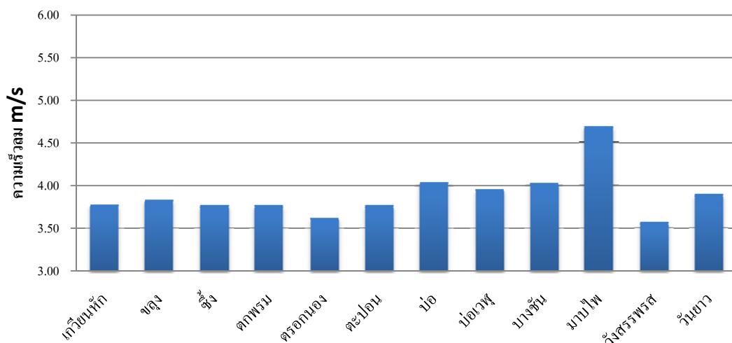
รูปที่ 41 กราฟแสดงค่าความเร็วลมเฉลี่ยของตำบลต่างๆ ในอำเภอขลุง
