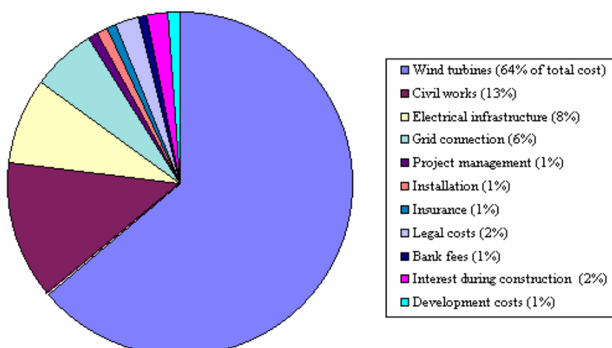
รูปที่ 223 การแจกแจงค่าใช้จ่ายของระบบกังหันลม (ที่มา: Wind Energy โดย M.Chandra Sekhar www.che.iitm.ac.in/~sjayanti/presentations/wind.ppt )
