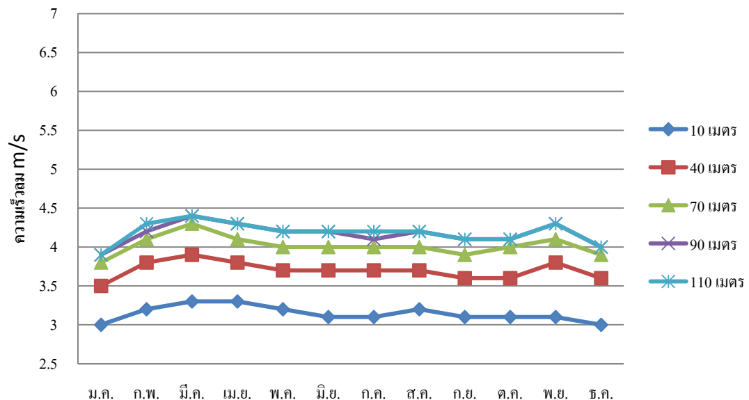
รูปที่ 23 แผนภาพแสดงศักยภาพความเร็วลมของตำบลชุมแสง อำเภอวังจันทร์ จังหวัดระยอง
