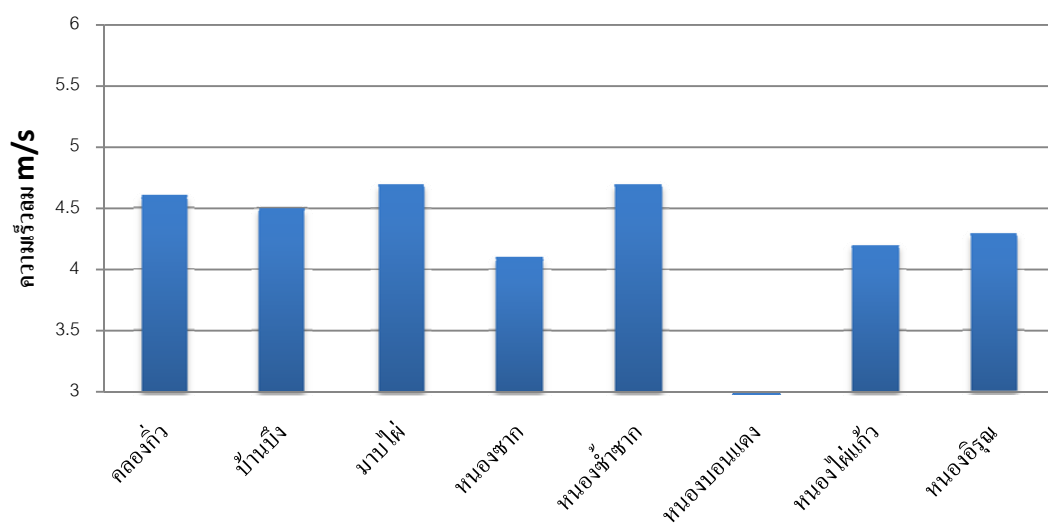
รูปที่ 12 กราฟแสดงค่าความเร็วลมเฉลี่ยของตำบลต่างๆ ในอำเภอบ้านบึง
