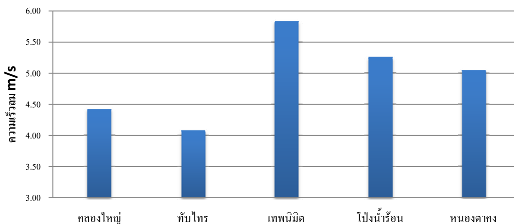
รูปที่ 44 กราฟแสดงค่าความเร็วลมเฉลี่ยของตำบลต่างๆ ในอำเภอโป่งน้ำร้อน
