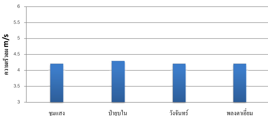
รูปที่ 33 กราฟแสดงค่าความเร็วลมเฉลี่ยของตำบลต่างๆ ในอำเภอวังจันทร์
