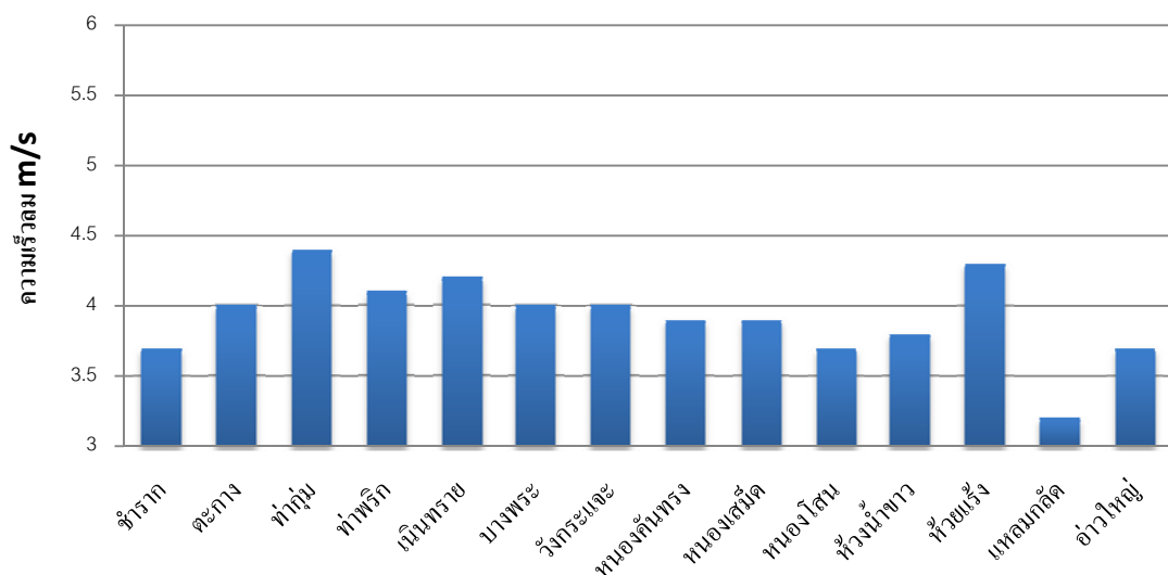
รูปที่ 59 กราฟแสดงค่าความเร็วลมเฉลี่ยของตำบลต่างๆ ในอำเภอเมืองตราด
