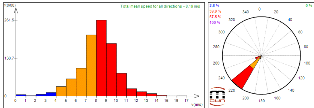
รูปที่ 171 กราฟการกระจายความเร็วลมสำหรับข้อมูลลมเฉลี่ยทุกๆ 10 นาที ของสถานีวัดลมที่ ต.ทับไทร อ. โป่งน้ำร้อน จ. จันทบุรี ที่ระดับความสูง 120 เมตร เดือน มิถุนายน 2555
