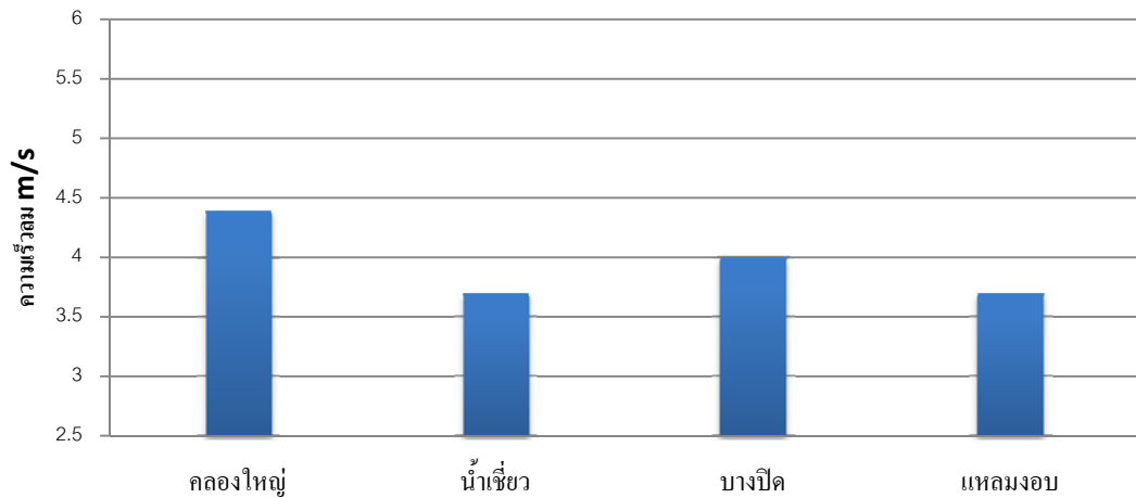
รูปที่ 60 กราฟแสดงค่าความเร็วลมเฉลี่ยของตำบลต่างๆ ในอำเภอสทิงพระ
