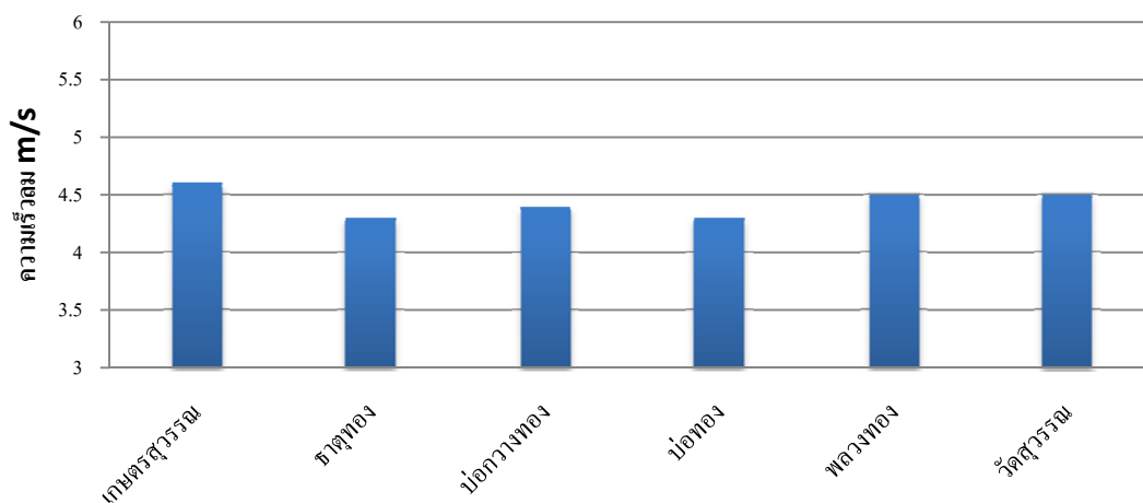
รูปที่ 10 กราฟแสดงค่าความเร็วลมเฉลี่ยของตำบลต่างๆ ในอำเภอบ่อทอง
