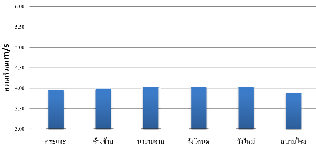
รูปที่ 43 กราฟแสดงค่าความเร็วลมเฉลี่ยของตำบลต่างๆ ในอำเภอนายายอาม
