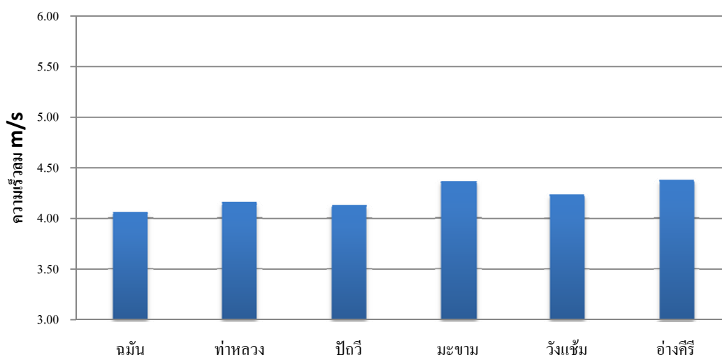
รูปที่ 45 กราฟแสดงค่าความเร็วลมเฉลี่ยของตำบลต่างๆ ในอำเภอมะขาม
