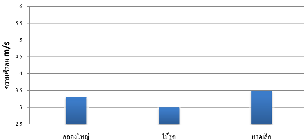
รูปที่ 57 กราฟแสดงค่าความเร็วลมเฉลี่ยของตำบลต่างๆ ในอำเภอคลองใหญ่
