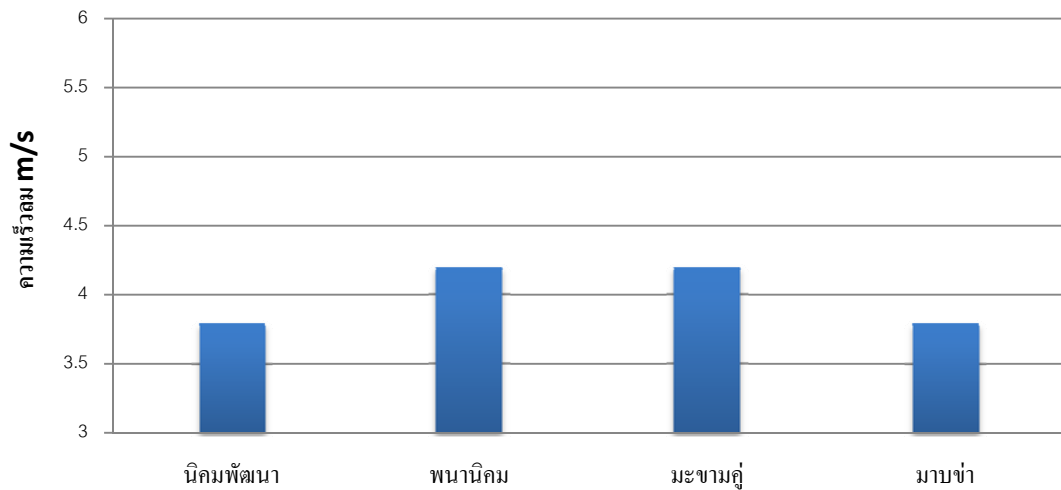
รูปที่ 28 กราฟแสดงค่าความเร็วลมเฉลี่ยของตำบลต่างๆ ในอำเภอนิคมพัฒนา
