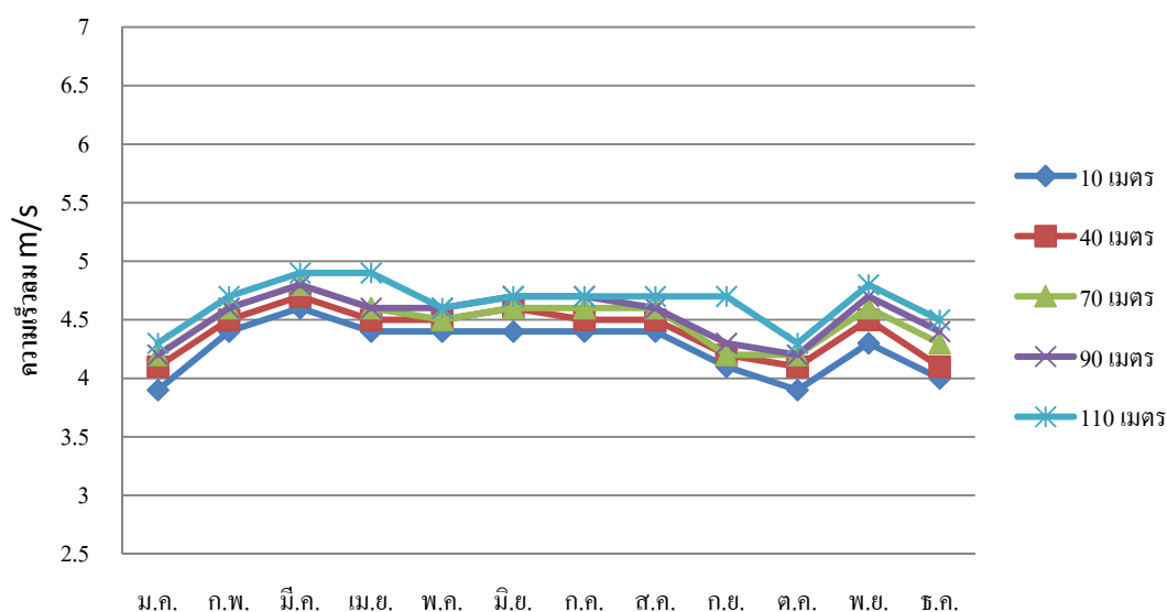
รูปที่ 6 แผนภาพแสดงศักยภาพความเร็วลมของตำบลหนองข้าซาก อำเภอบ้านบึง จังหวัดชลบุรี
