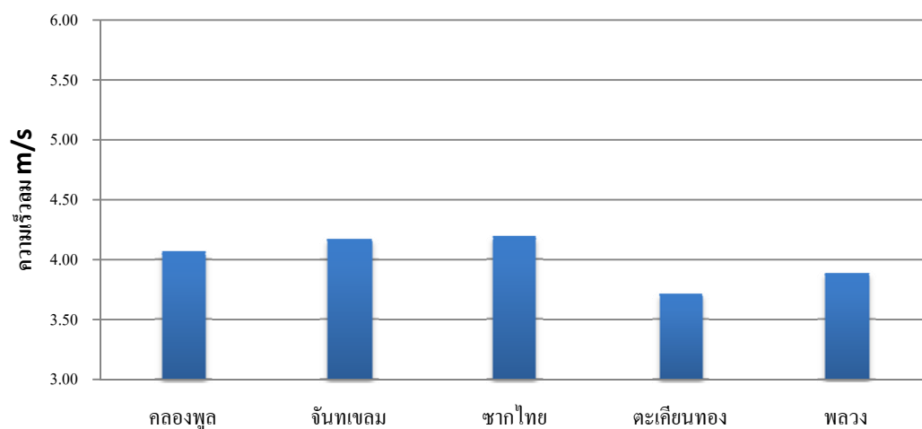
รูปที่ 49 กราฟแสดงค่าความเร็วลมเฉลี่ยของตำบลต่างๆ ในอำเภอลำลูกเกด
