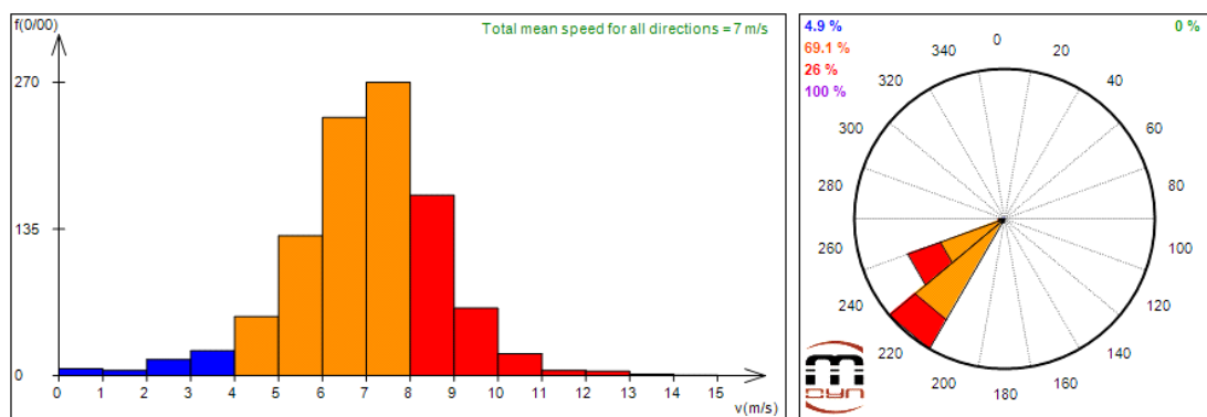
รูปที่ 169 กราฟการกระจายความเร็วลมสำหรับข้อมูลลมเฉลี่ยทุกๆ 10 นาที ของสถานีวัดลมที่ ต.ทับไทร อ. โป่งน้ำร้อน จ. จันทบุรี ที่ระดับความสูง 65 เมตร เดือน มิถุนายน 2555
