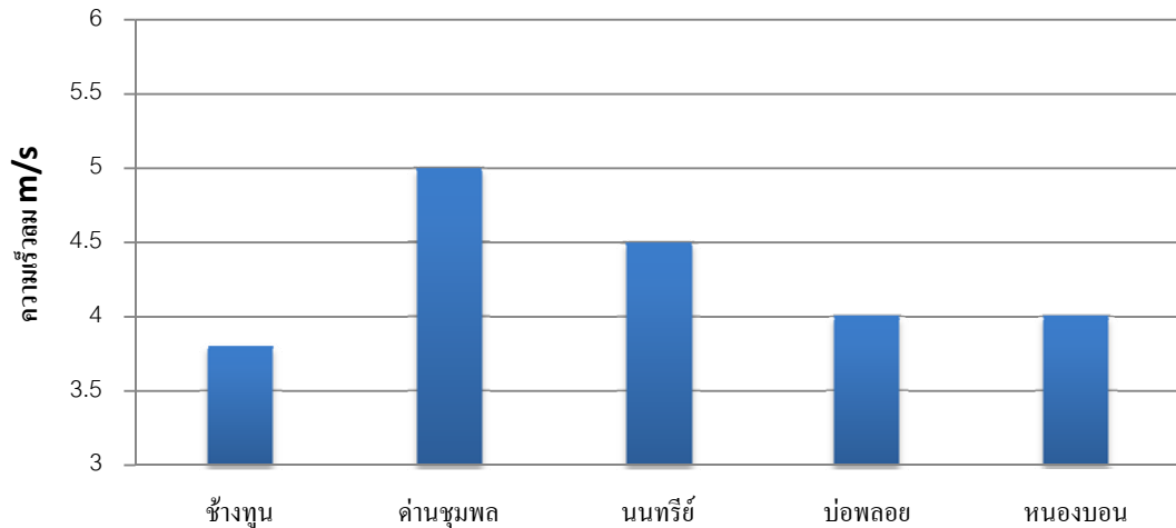
รูปที่ 58 กราฟแสดงค่าความเร็วลมเฉลี่ยของตำบลต่างๆ ในอำเภอบ่อไร่
