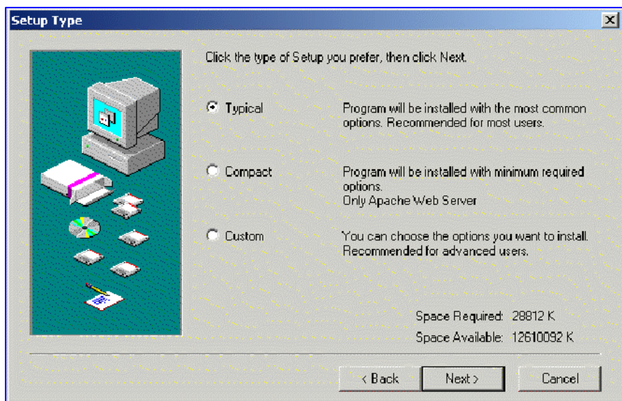
รูป ก.3 แสดงการเลือกรูปแบบการติดตั้งโปรแกรม
