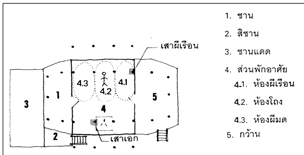
ภาพที่ 27 ผังเรือนไทดำแบบดั้งเดิมของชนชั้นผู้น้อย
