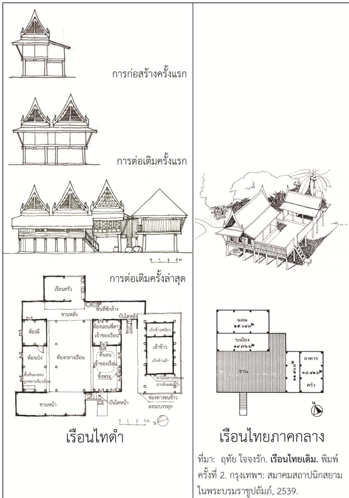
ภาพที่ 171 เปรียบเทียบเรือนไทยภาคกลางกับเรือนไทดำ
