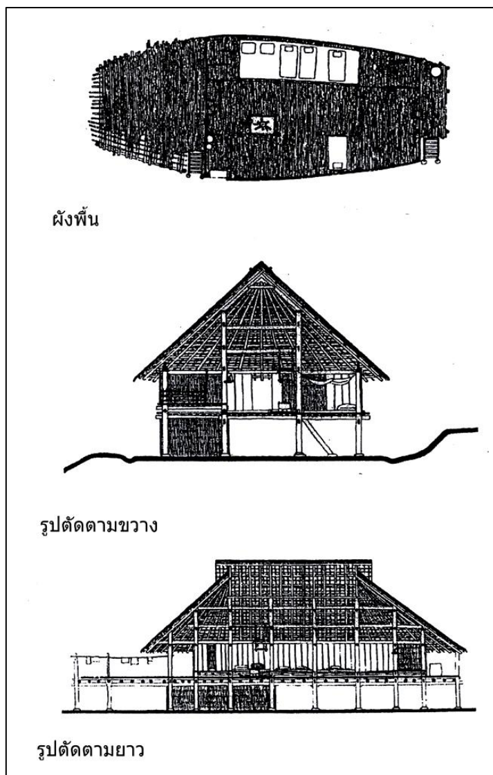
ภาพที่ 22 ผังพื้นและรูปตัดของเรือนไทดำแบบแผนเดิมแบบเรือนตูบกกลมสันหลังคาเต่า ที่มา: วีระ อินพันทั้ง และคณะ, รายงานการวิจัยฉบับสมบูรณ์ โครงการโลกของชาวไทดำ: ความสัมพันธ์ซึ่งกันระหว่างสภาพแวดล้อมที่อยู่อาศัยของชาวไทดำในไทยกับในเวียดนาม (กรุงเทพฯ: คณะสถาปัตยกรรมศาสตร์ มหาวิทยาลัยศิลปากร, 2549), 205.
