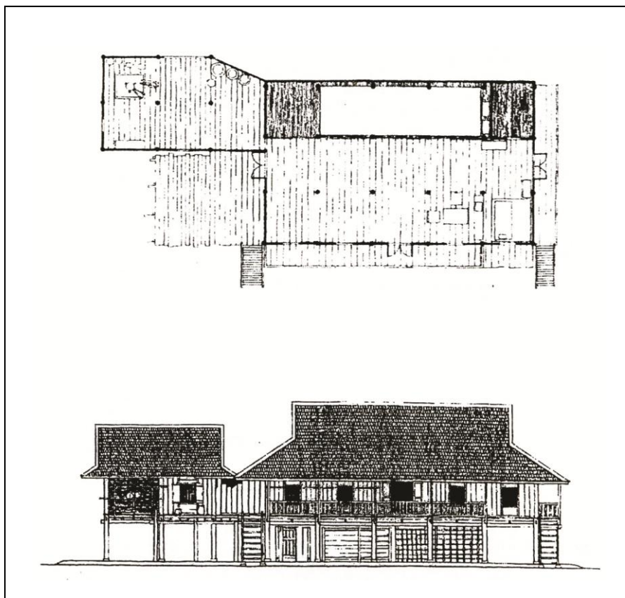
ภาพที่ 24 ผังพื้นและรูปด้านเรือนไทดำแบบพัฒนา
