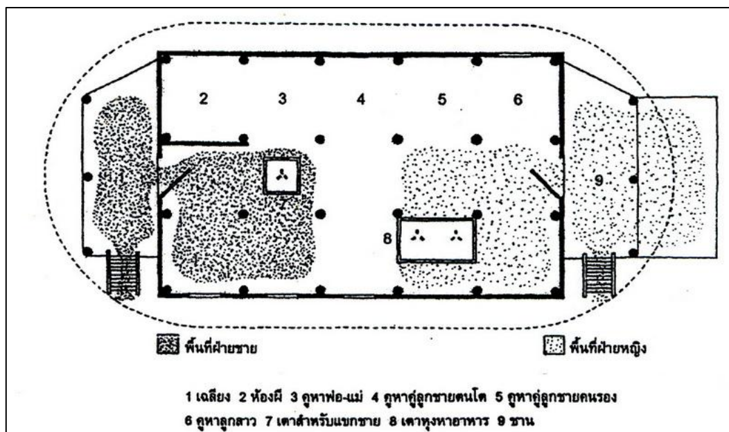
ภาพที่ 19 แผนผังแสดงการใช้พื้นที่ในเรือนไทดำ
