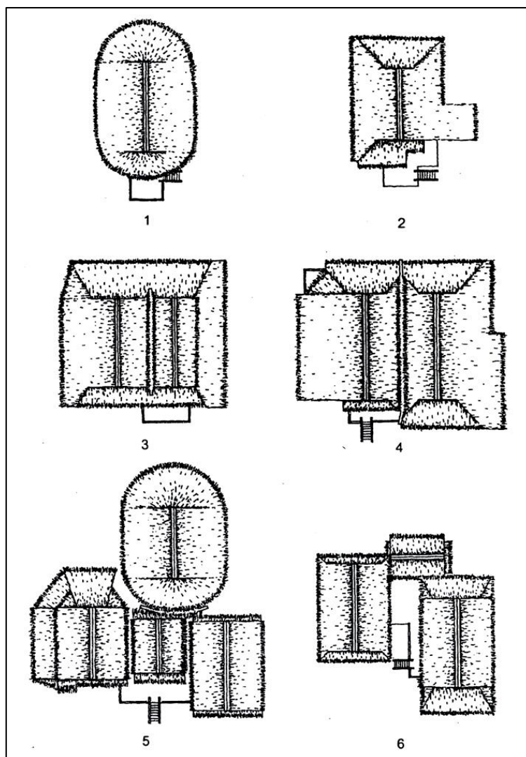
ภาพที่ 33 ผังหลังคาแสดงการขยายตัวของเรือนไทดำในแบบต่างๆ
