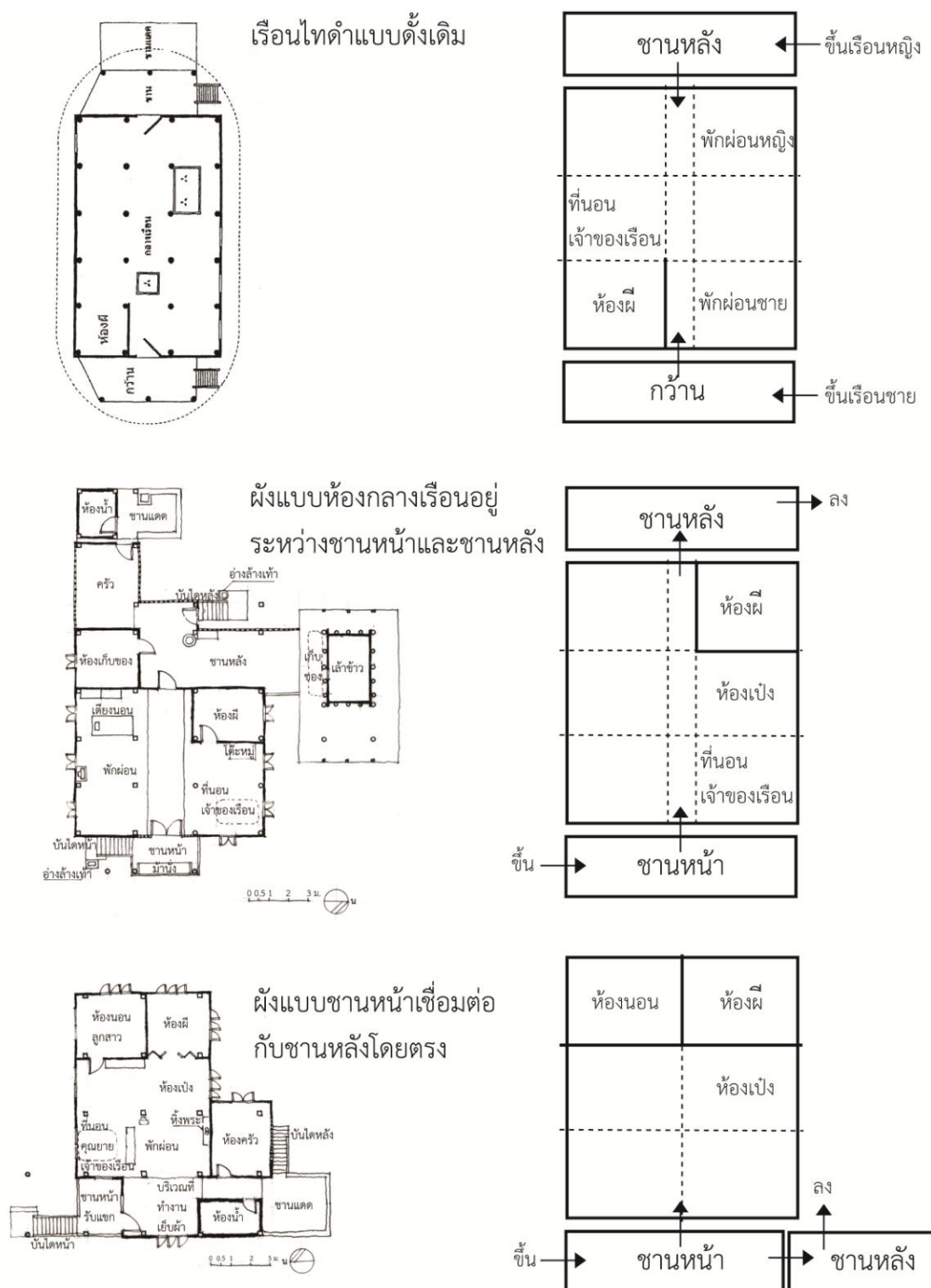
ภาพที่ 169 เปรียบเทียบการใช้พื้นที่ในระดับพื้นเรือนแบบห้องกลางเรือนอยู่ระหว่างชานหน้าและแบบชานหน้าเชื่อมต่อกับชานหลังโดยตรงกับผังเรือนไทดำแบบดั้งเดิม
