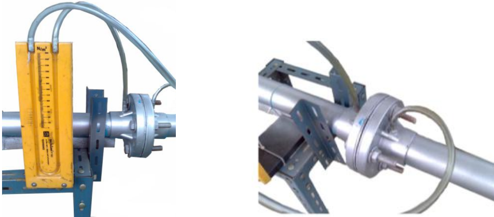
รูปที่ ก.5 ชุดควบคุมอัตราการป้อนอากาศ
