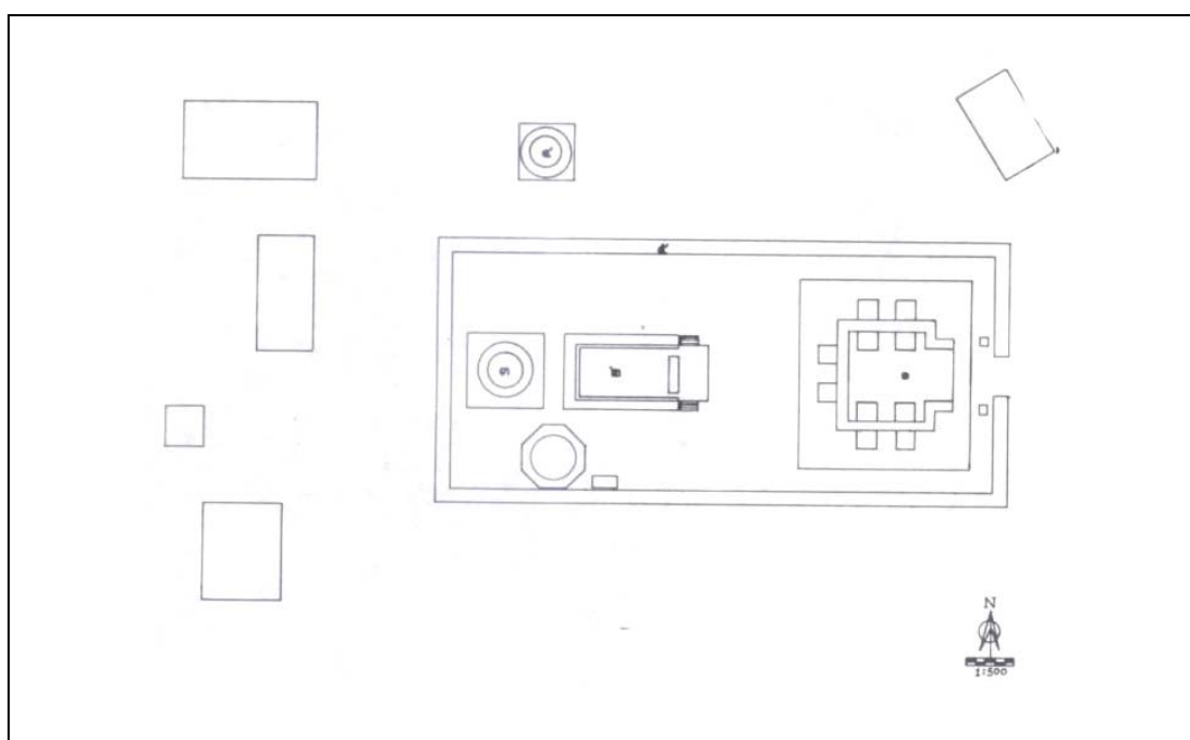
แผนผังที่ ๔ โบราณสถานวัดป่าเลไลยก์ที่พบจากการขุดแต่งทางโบราณคดี
