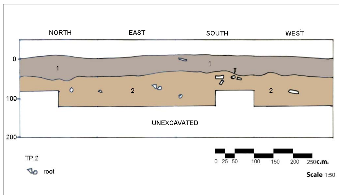
แผนผังที่ ๑๔ แผนผังชั้นดิน (Soil profile description) หลุมขุดค้น TP.2
