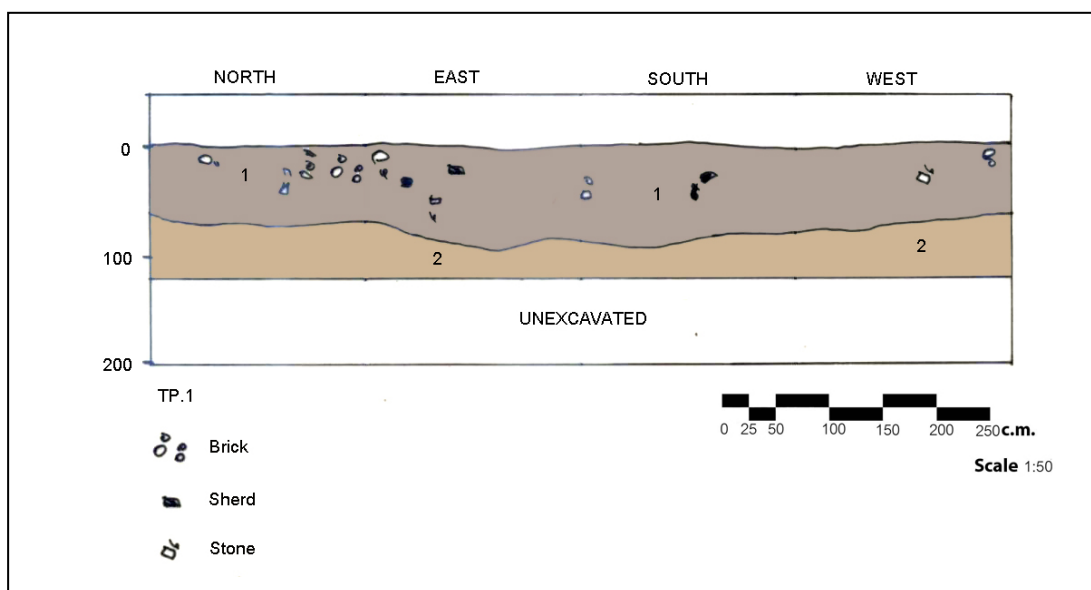
แผนผังที่ ๑๓ แผนผังชั้นดิน (Soil profile description) หลุมขุดค้น TP.1
