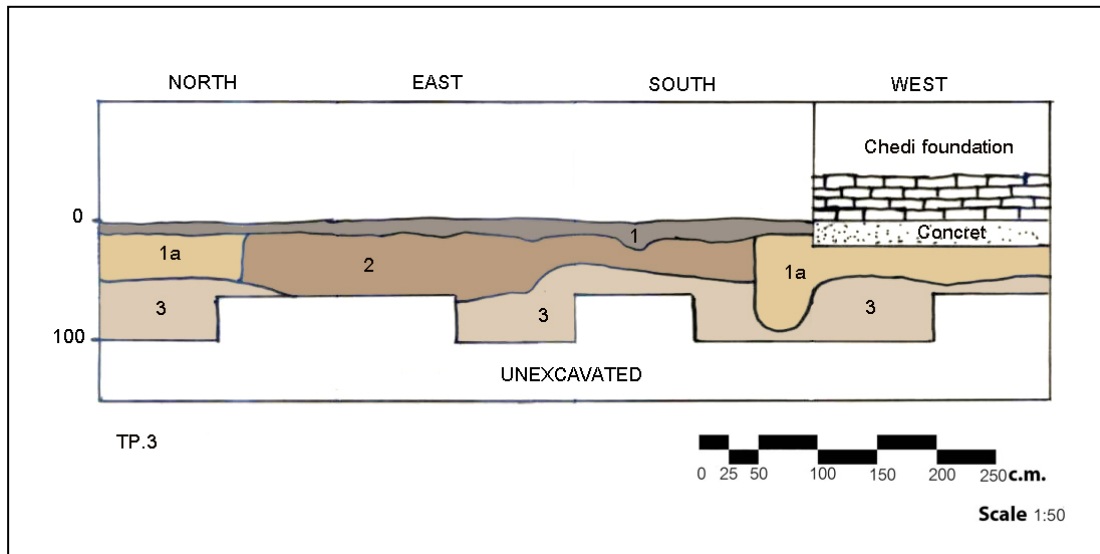
แผนผังที่ ๑๕ แผนผังชั้นดิน (Soil profile description) หลุมขุดค้น TP.3
