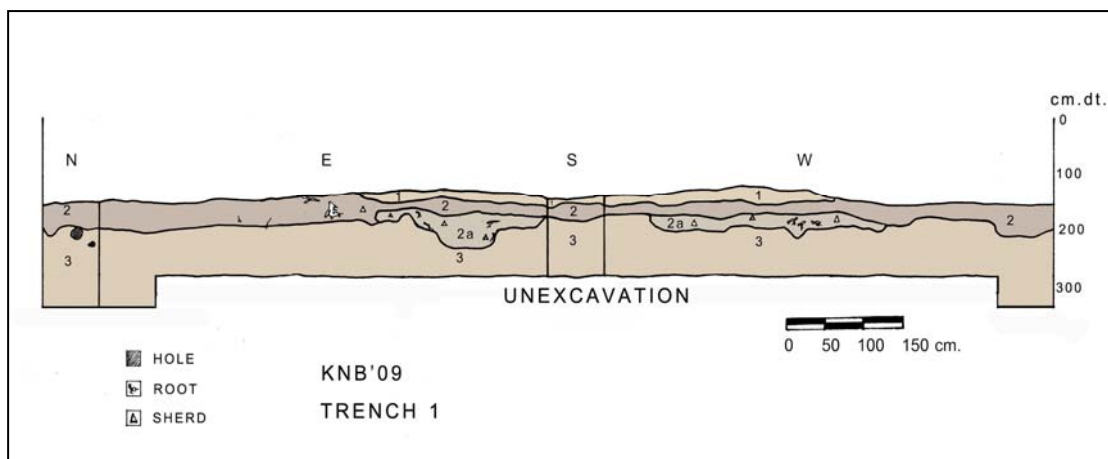
แผนผังที่ ๑๑ แผนผังชั้นดิน (Soil profile description) หลุมขุดค้น T.1
