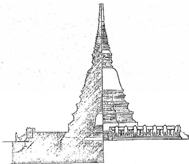
ภาพที่ 4 ภาพด้านตัดแสดงลักษณะเจดีย์สิงห์ล้อมที่สร้างครอบทับเจดีย์ทรงลังกาองค์เดิมไว้
