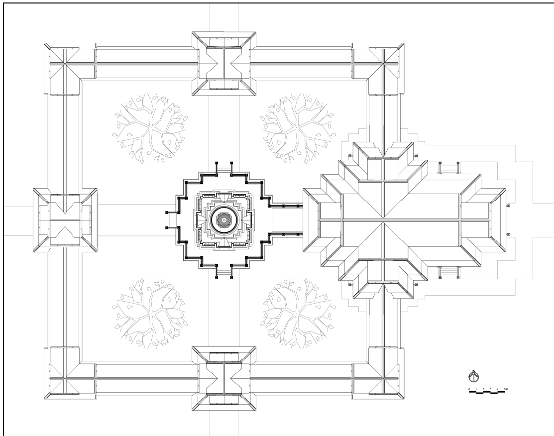
ภาพที่ 54 ผังบริเวณพระอุโบสถ – พระเจดีย์
