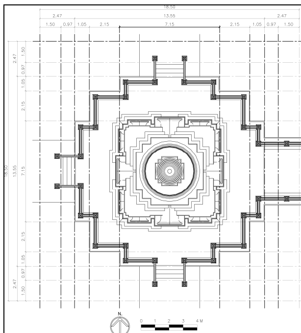
ภาพที่ 76 แบบสถาปัตยกรรมพระเจดีย์ : ผังหลังคา
