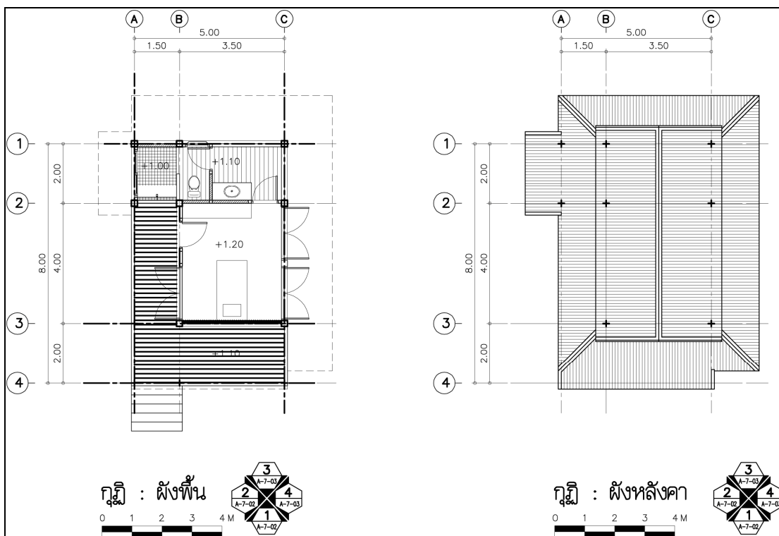
ภาพที่ 98 แบบสถาปัตยกรรมกุฏิพระ : ผัง
