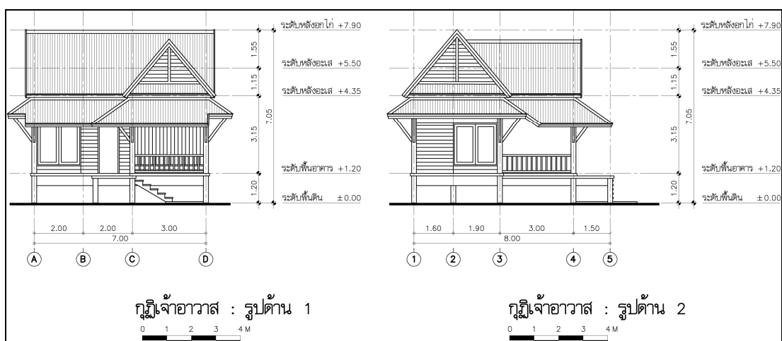
ภาพที่ 95 แบบสถาปัตยกรรมกุฏิเจ้าอาวาส : รูปด้าน
