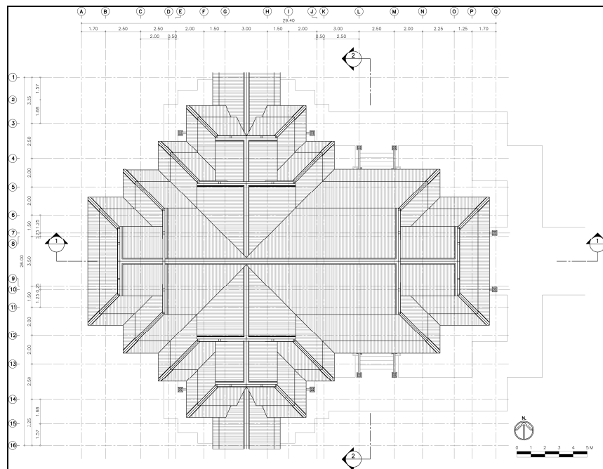
ภาพที่ 64 แบบสถาปัตยกรรม พระอุโบสถ : ผังหลังคา
