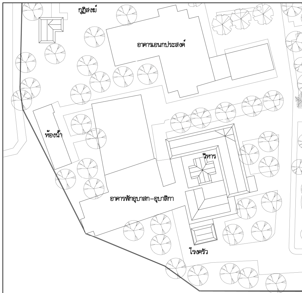
ภาพที่ 105 ผังบริเวณส่วนอาคารเดิม
