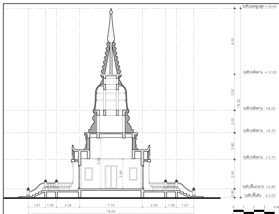
ภาพที่ 78 แบบสถาปัตยกรรมพระเจดีย์: รูปตัด
