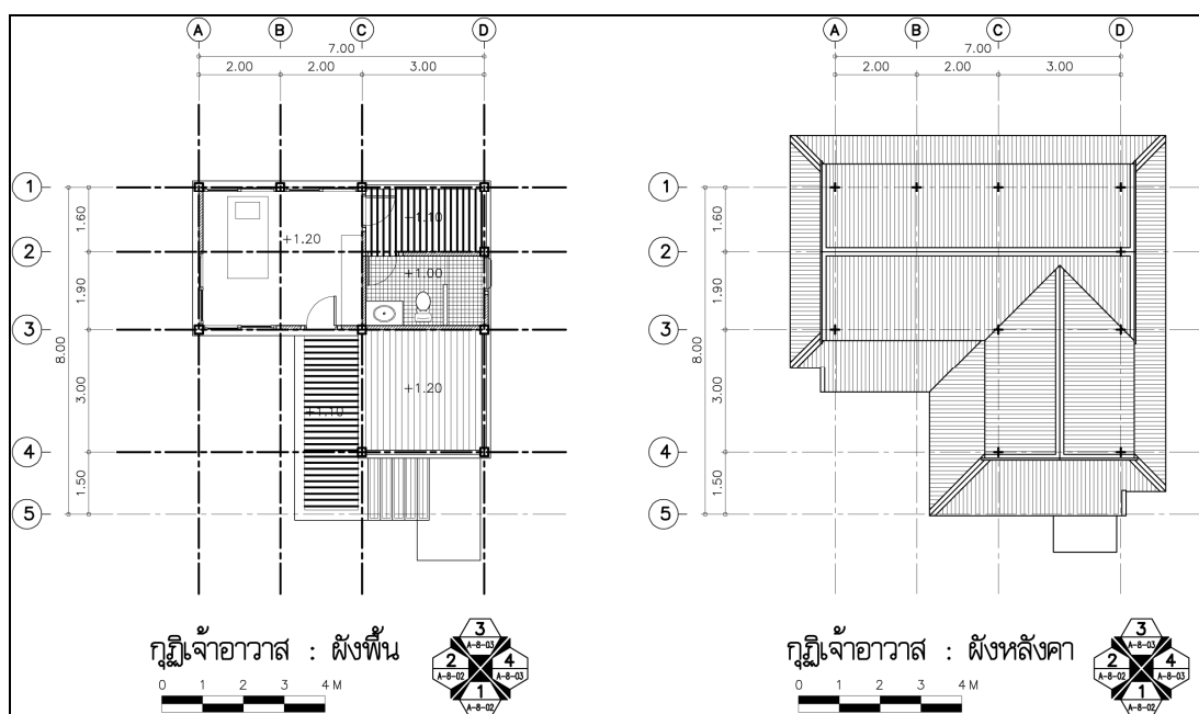
ภาพที่ 94 แบบสถาปัตยกรรมกุฏิเจ้าอาวาส : ผัง
