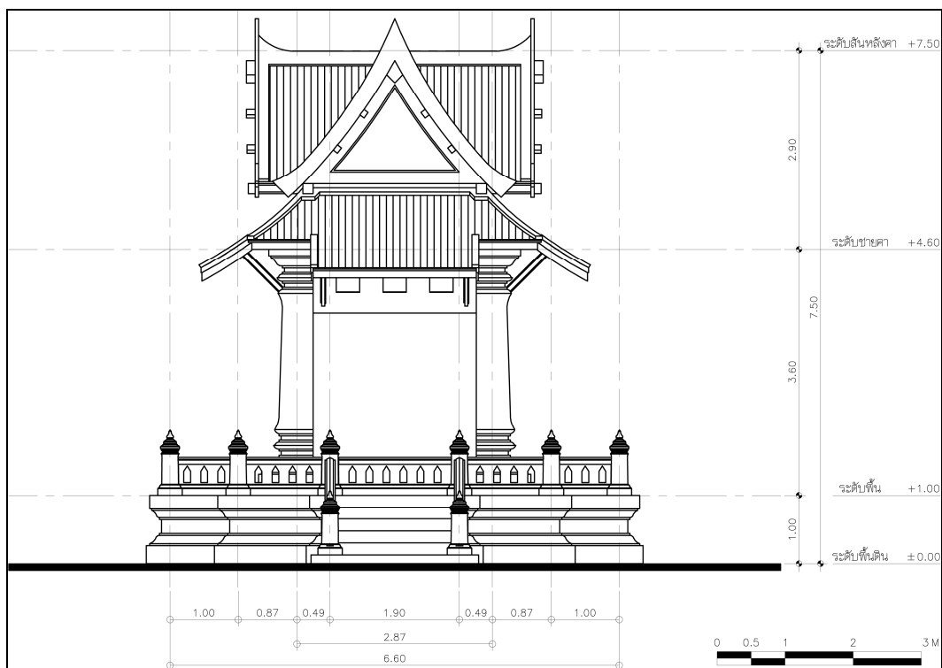
ภาพที่ 89 แบบสถาปัตยกรรมหอกลองและหอรอง : รูปด้าน ด้านหน้า
