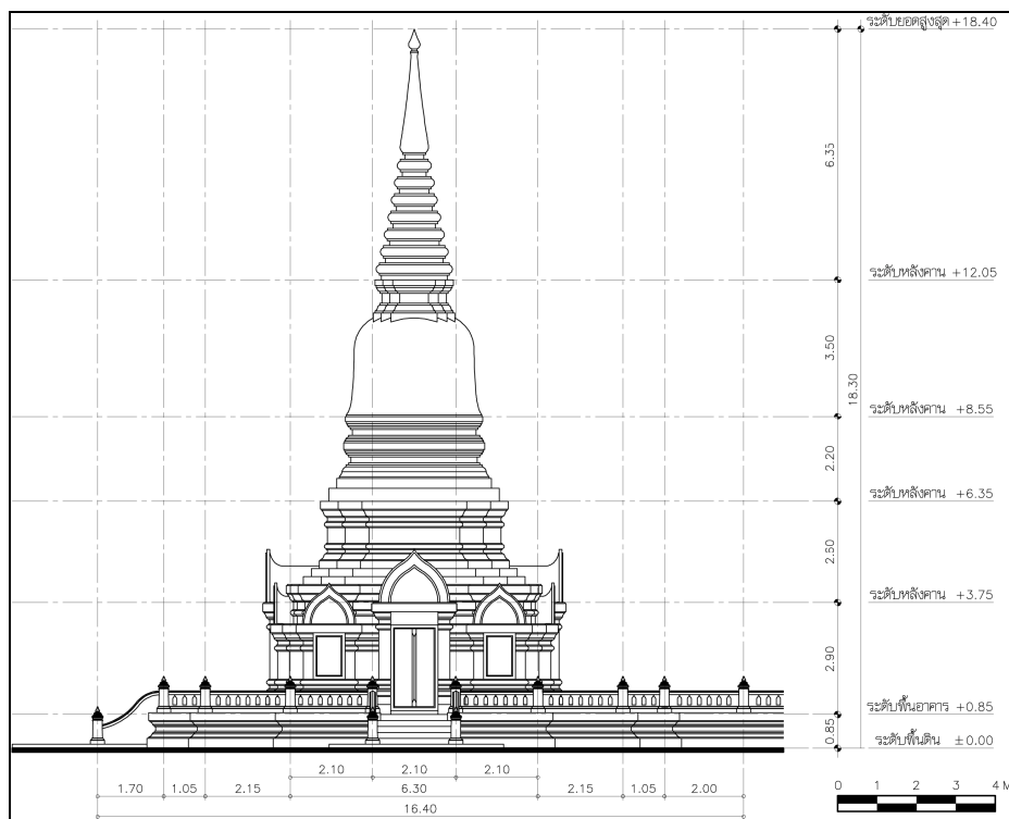
ภาพที่ 77 แบบสถาปัตยกรรมพระเจดีย์: รูปด้าน
