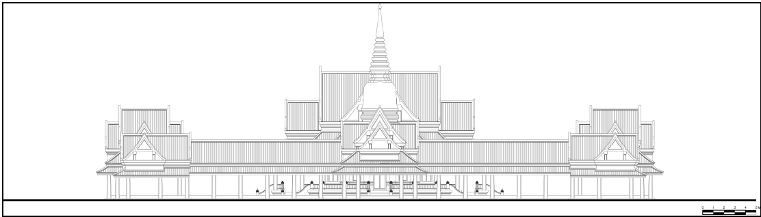
ภาพที่ 56 แบบสถาปัตยกรรม พระอุโบสถ – พระเจดีย์ : รูปด้านรวมด้านทิศตะวันตก
