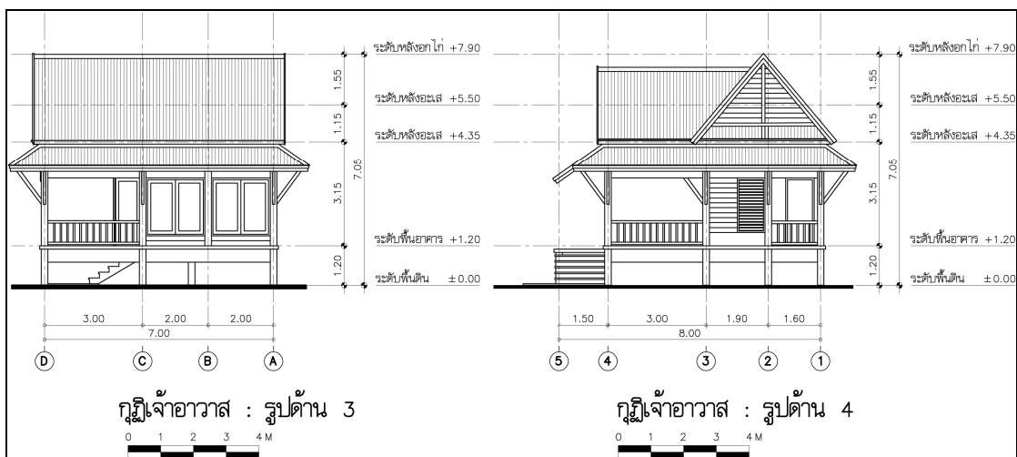
ภาพที่ 96 แบบสถาปัตยกรรมกุฎีเจ้าอาวาส : รูปด้าน
