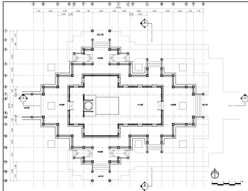
ภาพที่ 63 แบบสถาปัตยกรรม พระอุโบสถ : ผังพื้น
