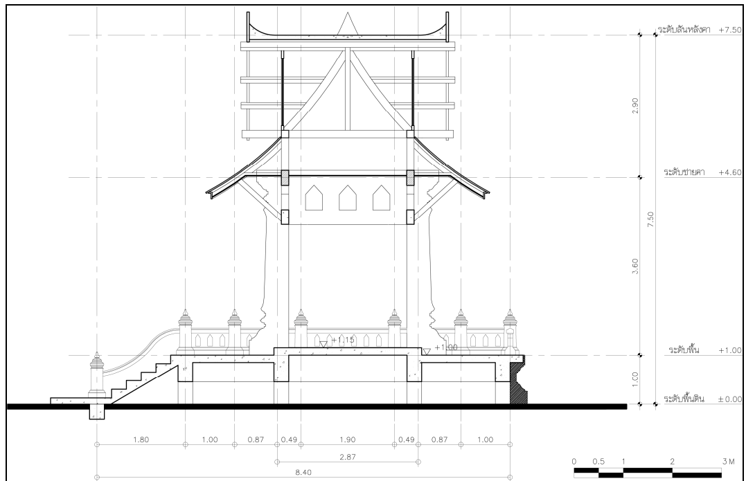
ภาพที่ 91 แบบสถาปัตยกรรมหอกลองและหอรระฆัง : รูปตัด
