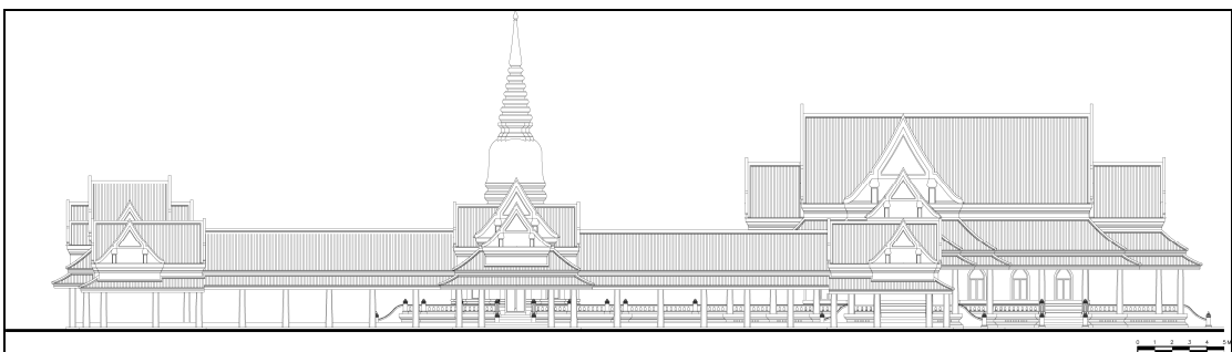
ภาพที่ 58 แบบสถาปัตยกรรม พระอุโบสถ – พระเจดีย์ : รูปด้านรวมด้านทิศใต้
