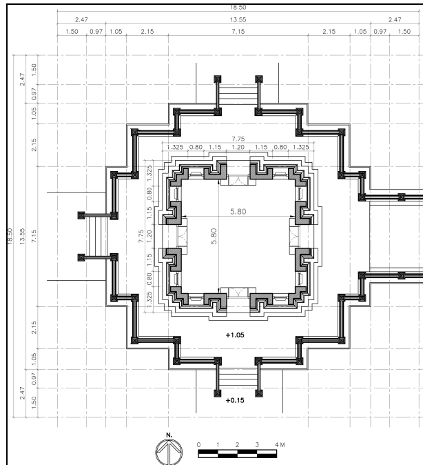
ภาพที่ 75 แบบสถาปัตยกรรมพระเจดีย์ : ผังพื้น
