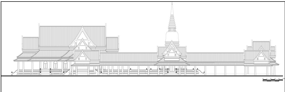
ภาพที่ 57 แบบสถาปัตยกรรม พระอุโบสถ – พระเจดีย์ : รูปด้านรวมด้านทิศเหนือ
