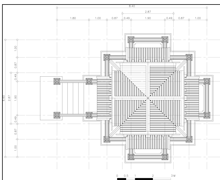
ภาพที่ 88 แบบสถาปัตยกรรมหอกลองและหอรระฆัง : ผังหลังคา
