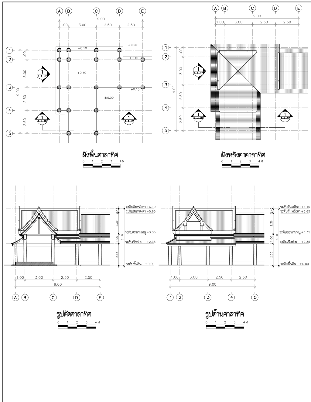
ภาพที่ 83 แบบสถาปัตยกรรมศาลาทิศ
