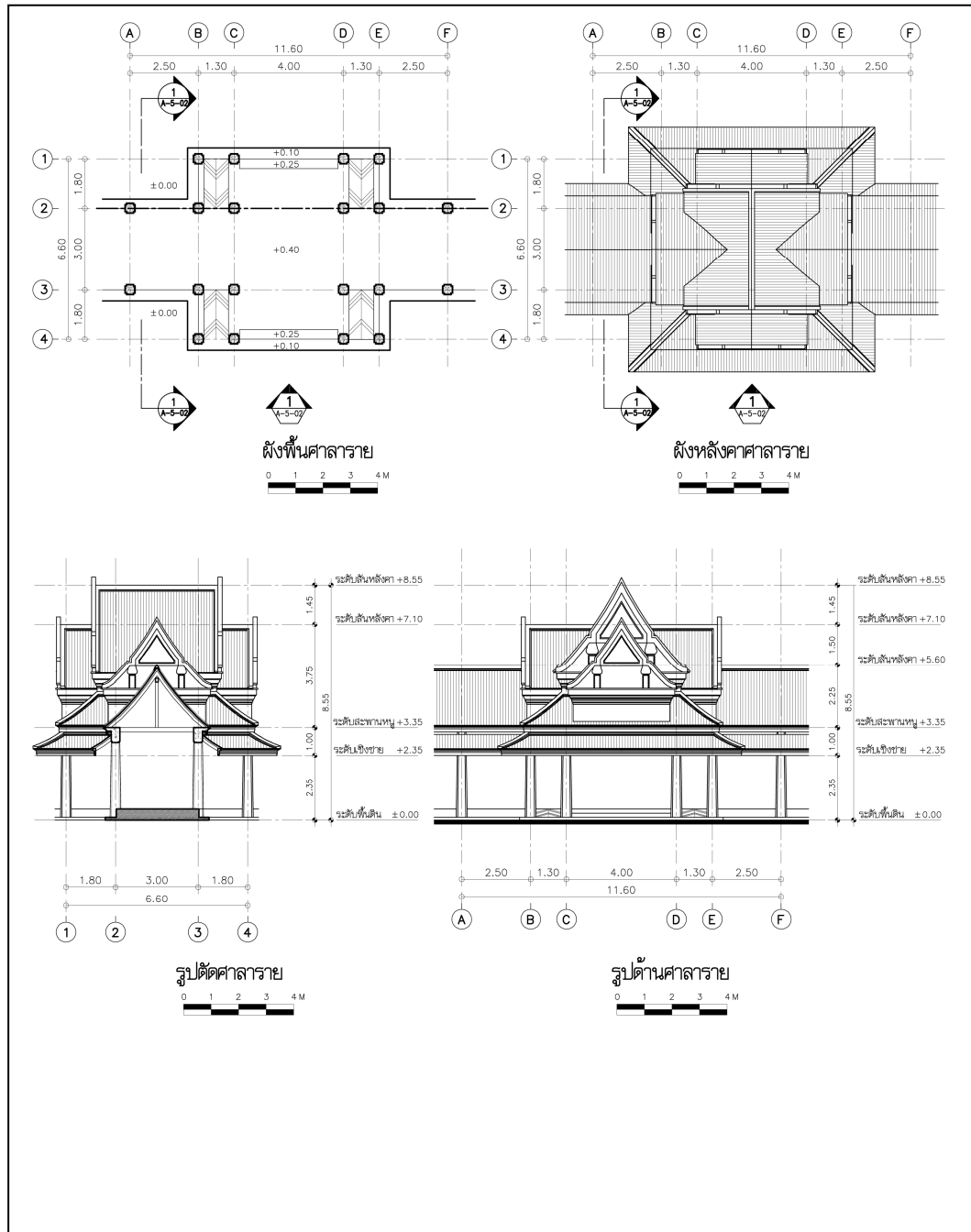
ภาพที่ 81 แบบสถาปัตยกรรมศาลาราย
