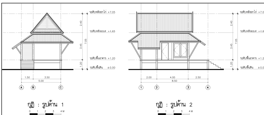
ภาพที่ 99 แบบสถาปัตยกรรมกุฏิพระ : รูปด้าน
