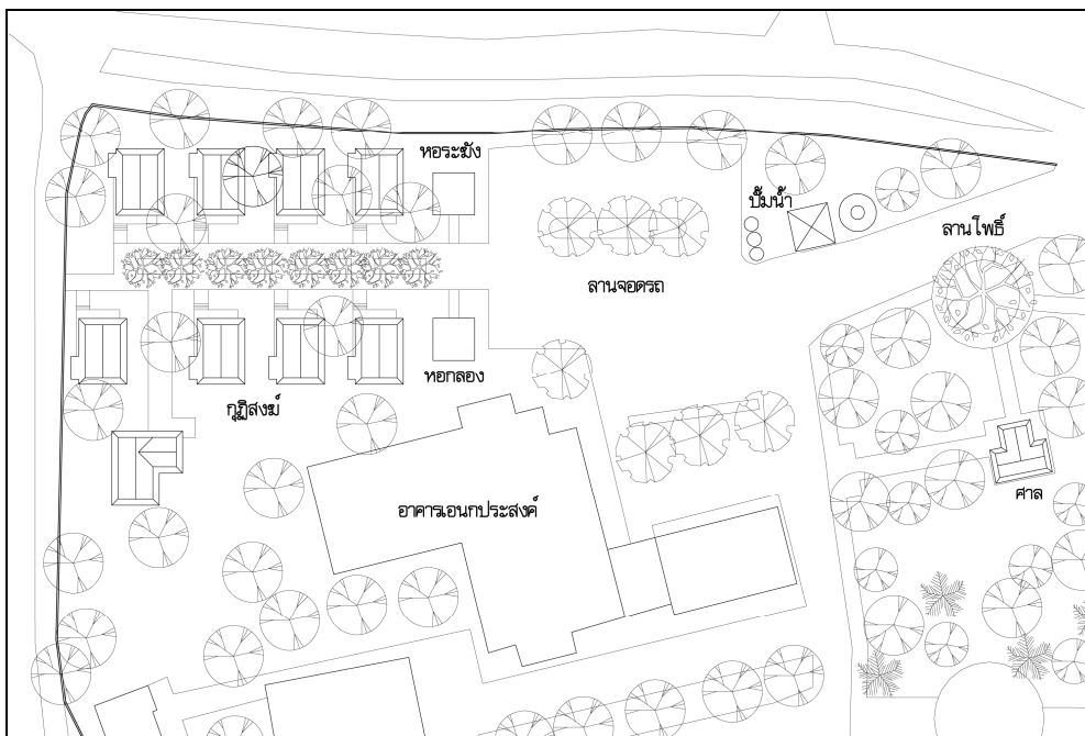
ภาพที่ 85 ผังบริเวณส่วนสังฆาวาส
