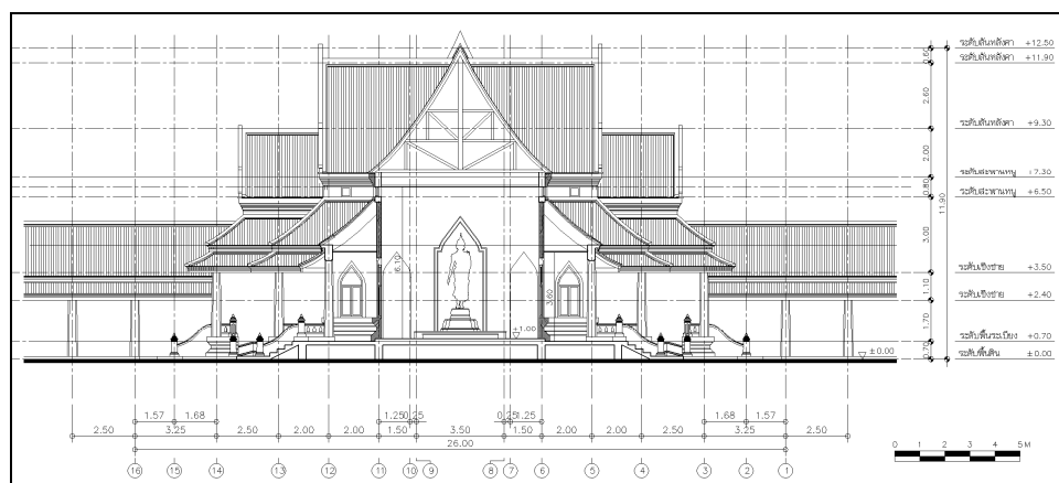
ภาพที่ 70 แบบสถาปัตยกรรมพระอุโบสถ : รูปตัด 2
