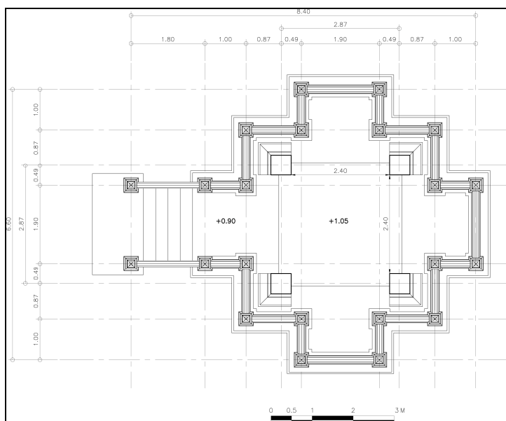
ภาพที่ 87 แบบสถาปัตยกรรมหอกลองและหอรระฆัง : ผังพื้น
