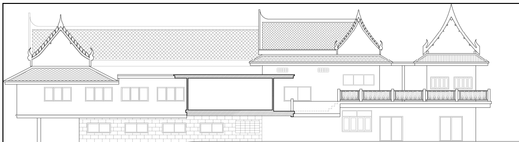
ภาพที่ 46 รูปตัดทางเชื่อมระหว่างอาคาร 6 และอาคาร 8 (แสดงรูปด้านทิศตะวันตกของอาคาร 8 ตามผังสำรวจ)
