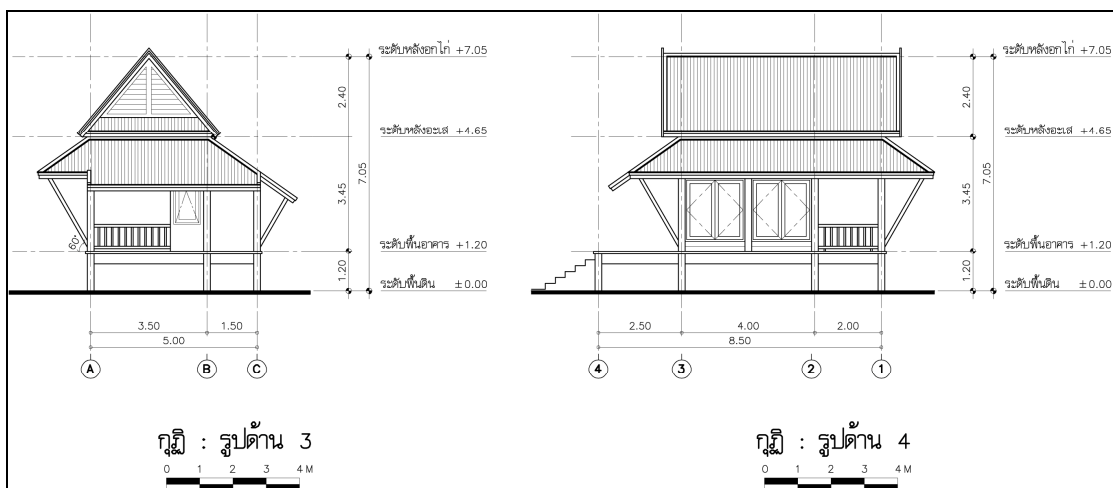
ภาพที่ 100 แบบสถาปัตยกรรมกุฏิพระ : รูปด้าน
