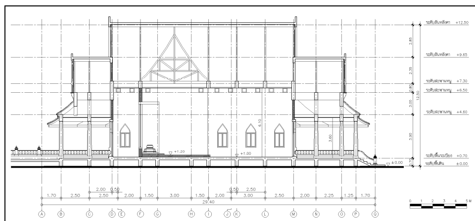
ภาพที่ 69 แบบสถาปัตยกรรมพระอุโบสถ : รูปตัด 1
