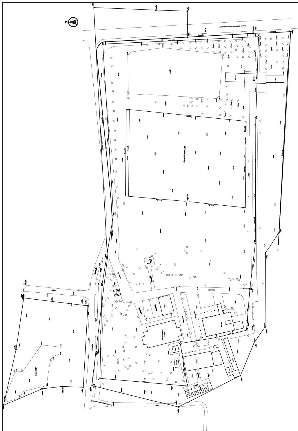
ภาพที่ 36 ผังวัดป่าไทรย่อยจากการสำรวจ รังวัด
