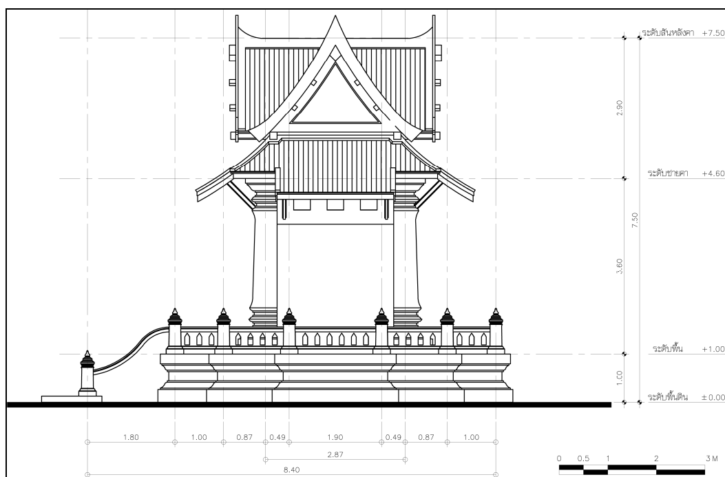
ภาพที่ 90 แบบสถาปัตยกรรมหอกลองและหอรอง : รูปด้าน ด้านข้าง
