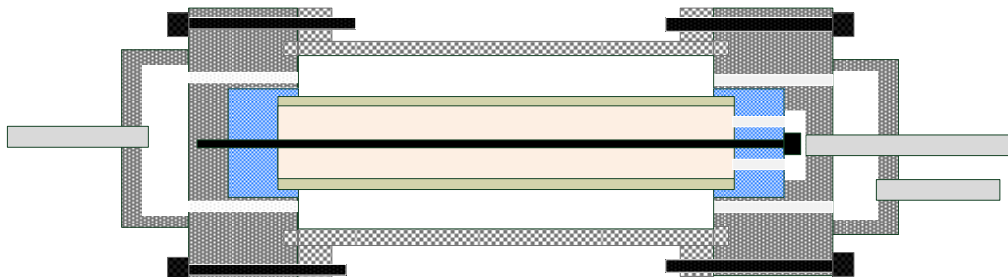
ภาพที่ ง-5 ภาพตัดขวางการประกอบเครื่องปฏิกรณ์เมมเบรน
