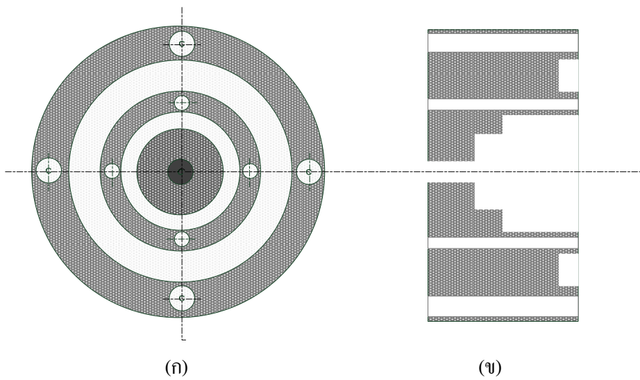
ภาพ ง-1 ภาพอุปกรณ์ด้านท้ายเข้า (ก) ภาพด้านหน้า (ข) ภาพตัดขวาง
