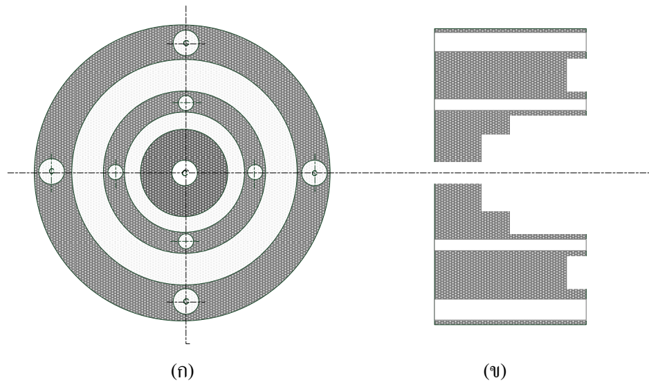
ภาพ ง-3 ภาพอุปกรณ์ด้านท้ายออก (ก) ภาพด้านหน้า (ข) ภาพตัดขวาง
