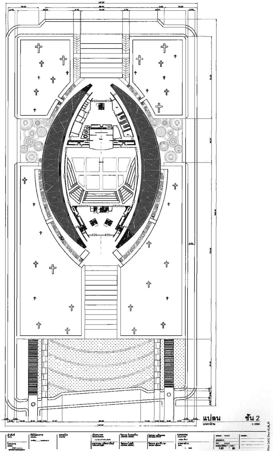
ภาพที่ 37 แปลนชั้น 2 แบบหน้าที่ 1.03
