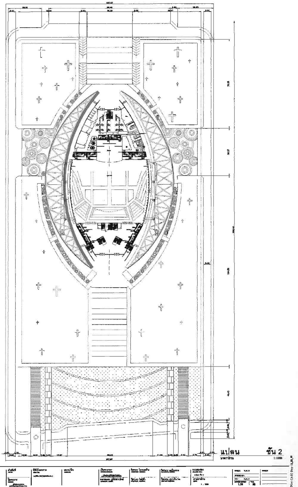
ภาพที่ 101 แปลนปรับอากาศ ชั้น 2 แบบหน้าที่ 1.24
