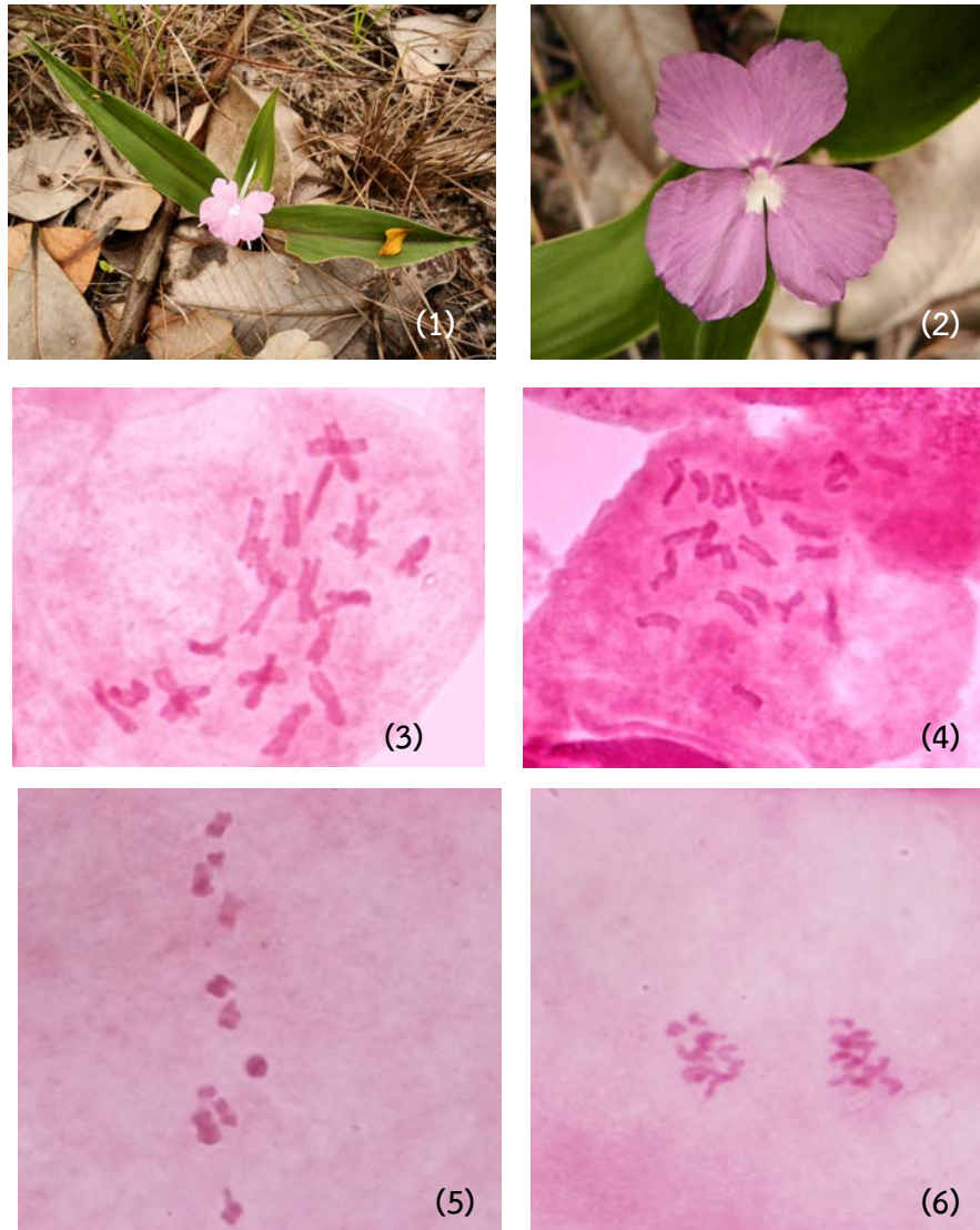
รูปที่ 5 เปราะราศี จังหวัดอุดรธาธานี (1) ลักษณะใบและดอก (2) ดอก (3) – (4) โครโมโซมจากเซลล์ปลายรากระยะเมทาเฟส 2n=22 : (3) จากอานโทซังเจียม (4) จากอานโทพิบูลมั่งสาหาร (5) – (6) โครโมโซมจากเซลล์กำเนิดเรณู อานโทซังเจียม : (5) ระยะเมทาเฟสแรกโครโมโซมจับคู่กัน 11 bivalents (6) ระยะแอนาเฟสแรก (11:11)
