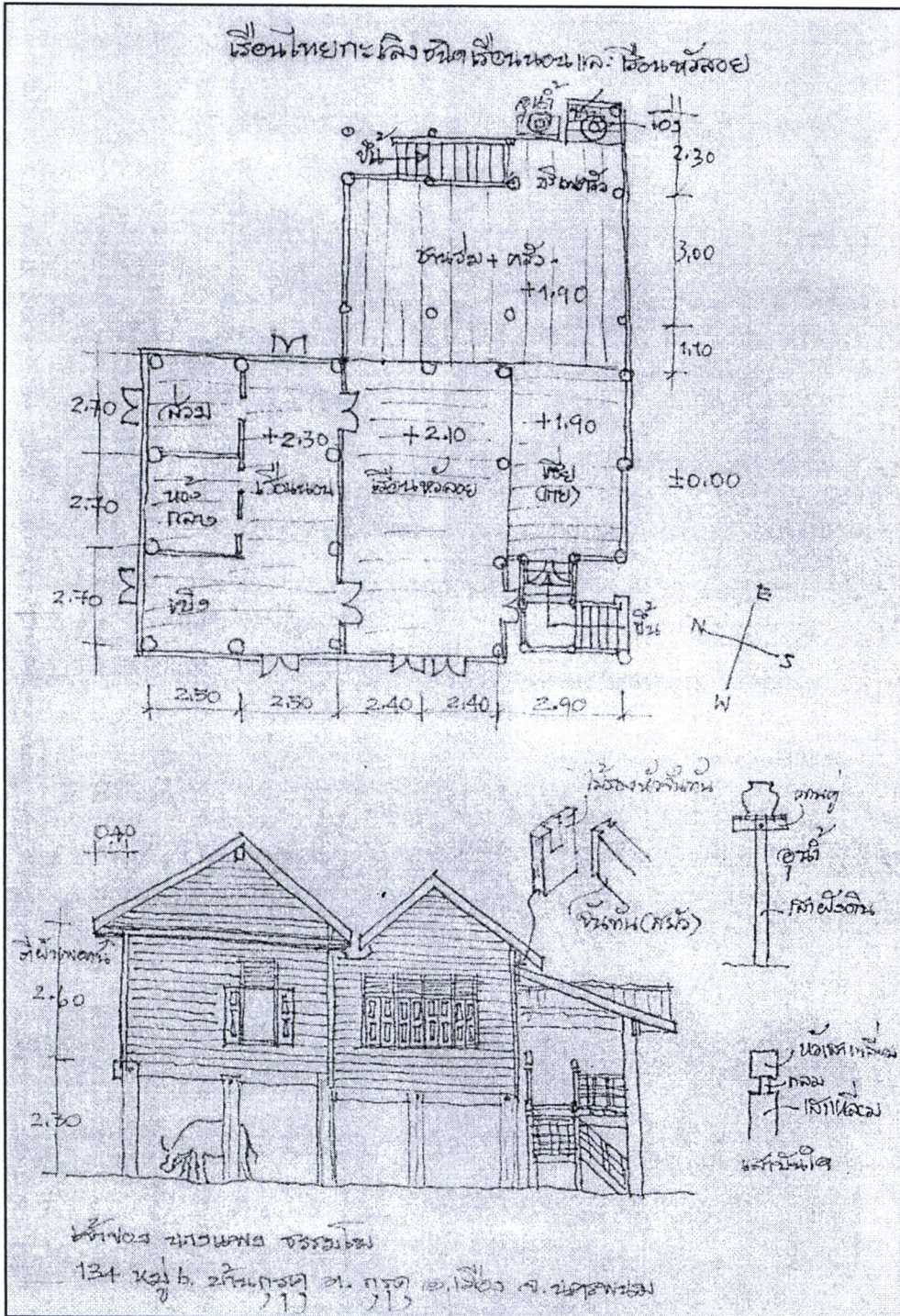
ภาพที่ 4.24 เรือนไทยกะเลิงชนิดเรือนนอนและเรือนหัวลอย (วิจิต คลังบุญครอง, 2550)
