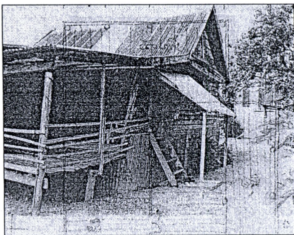
ภาพที่ 4.65 เรือนเกย (เชียบ) มีเทียบันได (วิจิต คลังบุญครอง, 2550)
