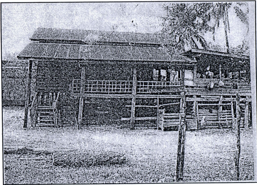
ภาพที่ 4.25 เรือนนอน เรือนหัวลอย (หอลอย) เข็ย (เกข) เรือนครัว (เรือนไฟ) ทรงเพิงหมาแหงน (วิจิต คลังบุญครอง, 2550)
