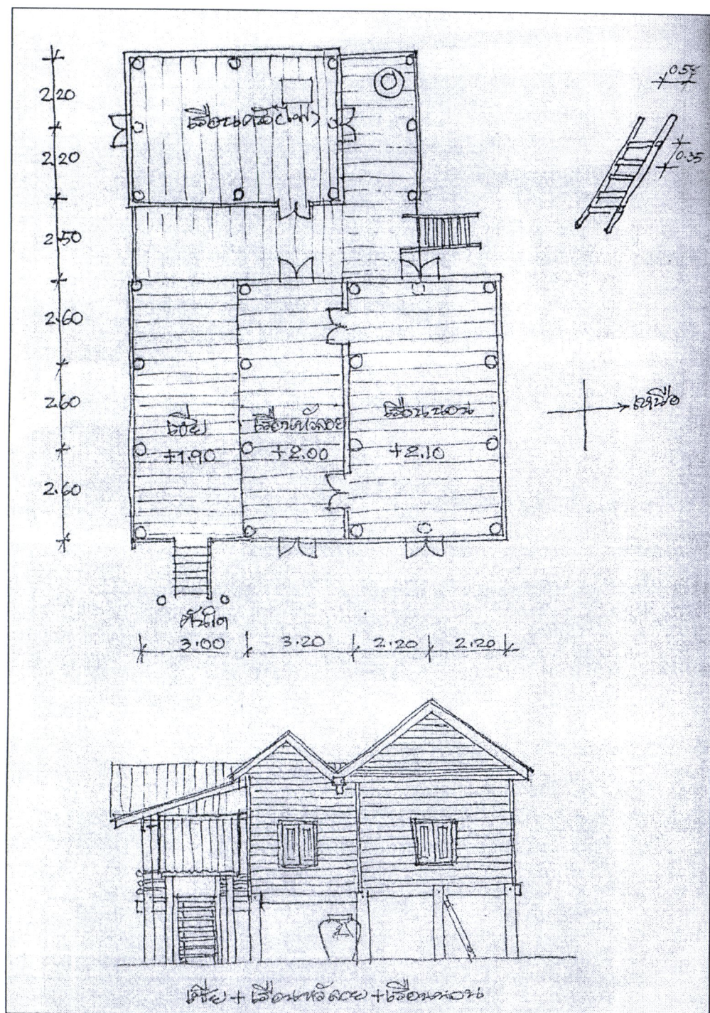
ภาพที่ 4.43 เรือนไทยอีสานเรือนหัวถอย (วิจิต คลังบุญครอง, 2550)
