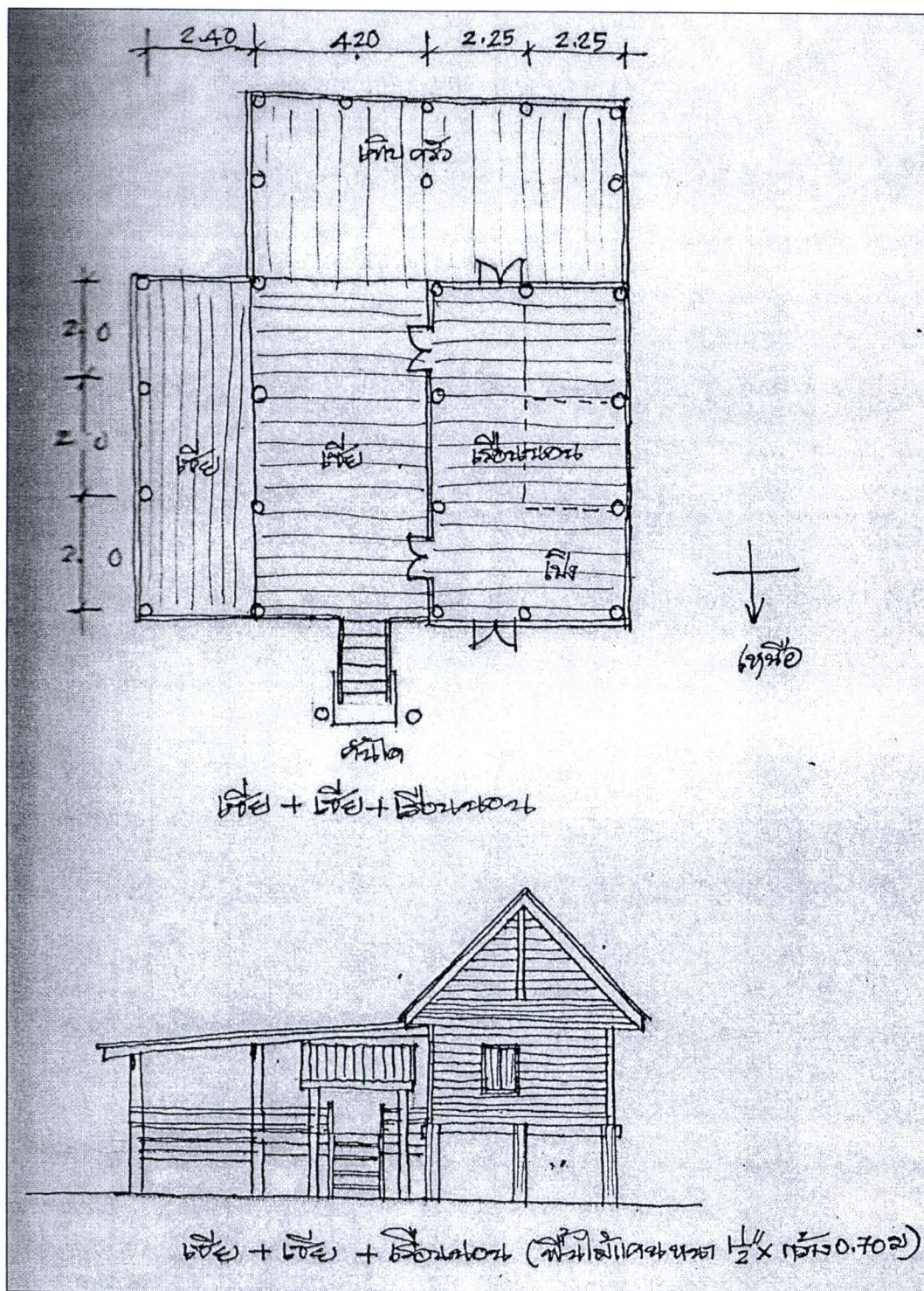
ภาพที่ 4.66 เรือนไทยอีสานชนิดเรือนเขี้ยว (วิจิตร กลังบุญครอง, 2550)
