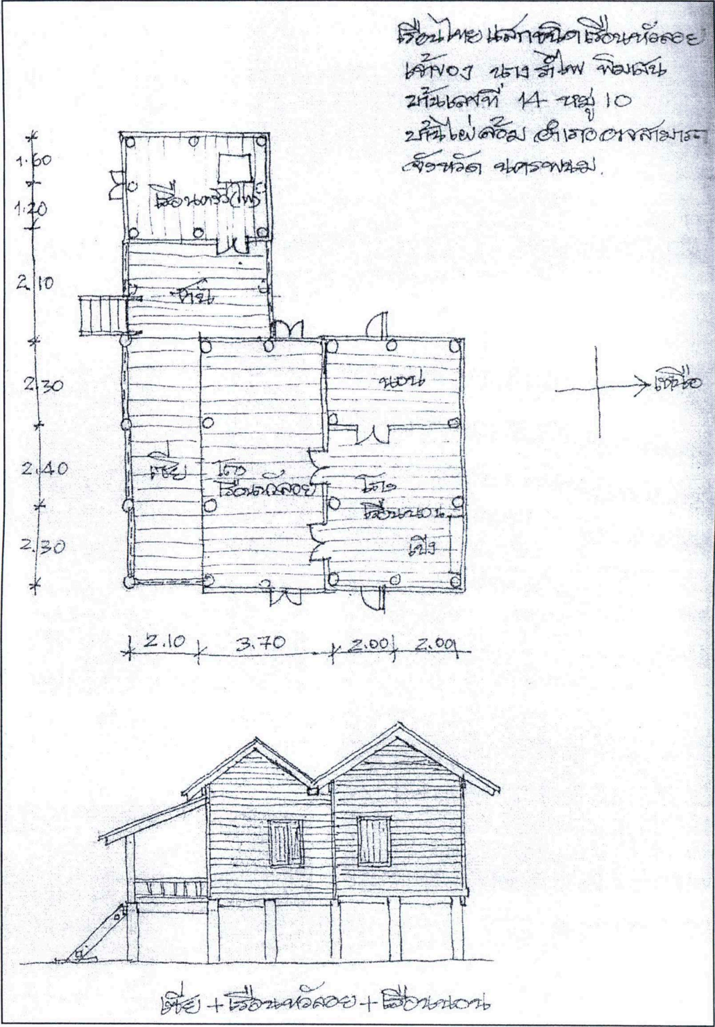
ภาพที่ 4.35 เรือนไทยแยกชนิดเรือนหัวลอย (วิจิต คลังบุญครอง, 2550)
