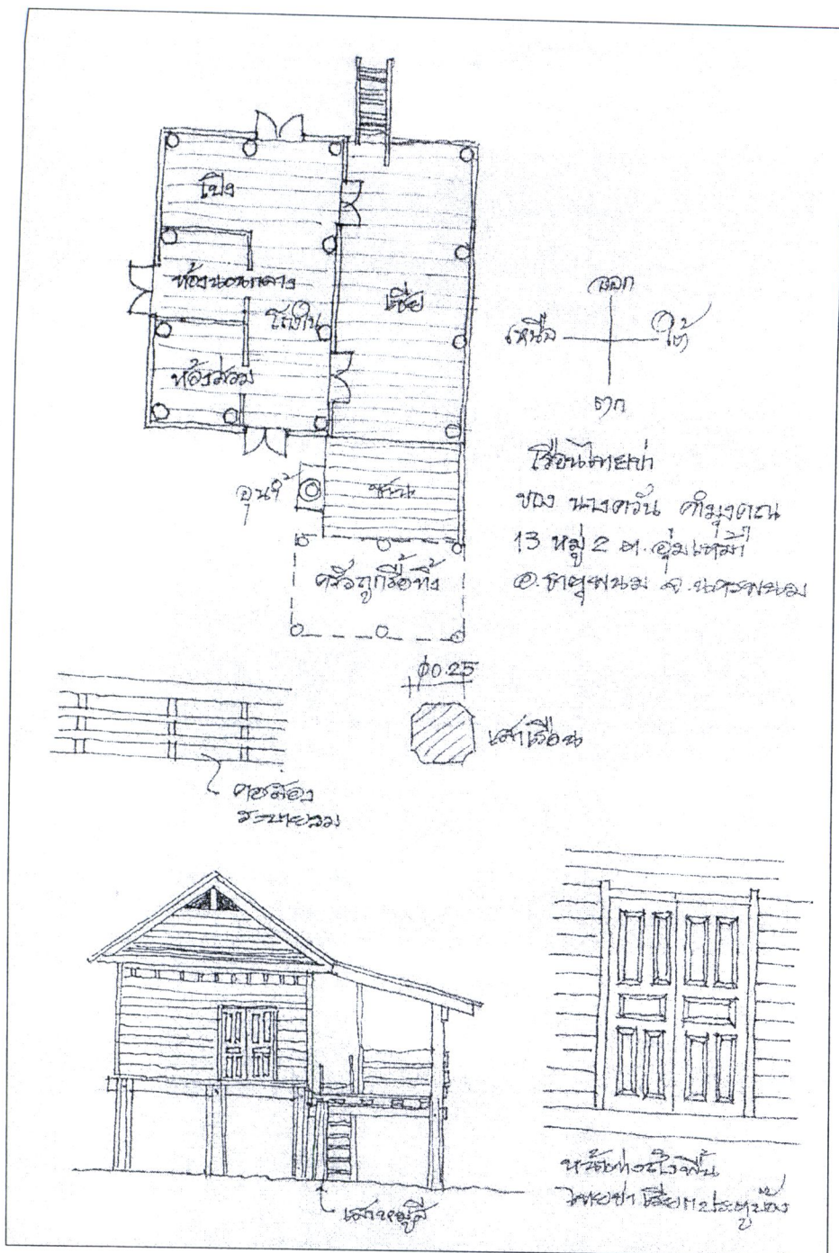
ภาพที่ 4.61 ลักษณะเรือนไทยช่างนาคเรือนเซีย (วิจิต คลังบุญครอง, 2550)
