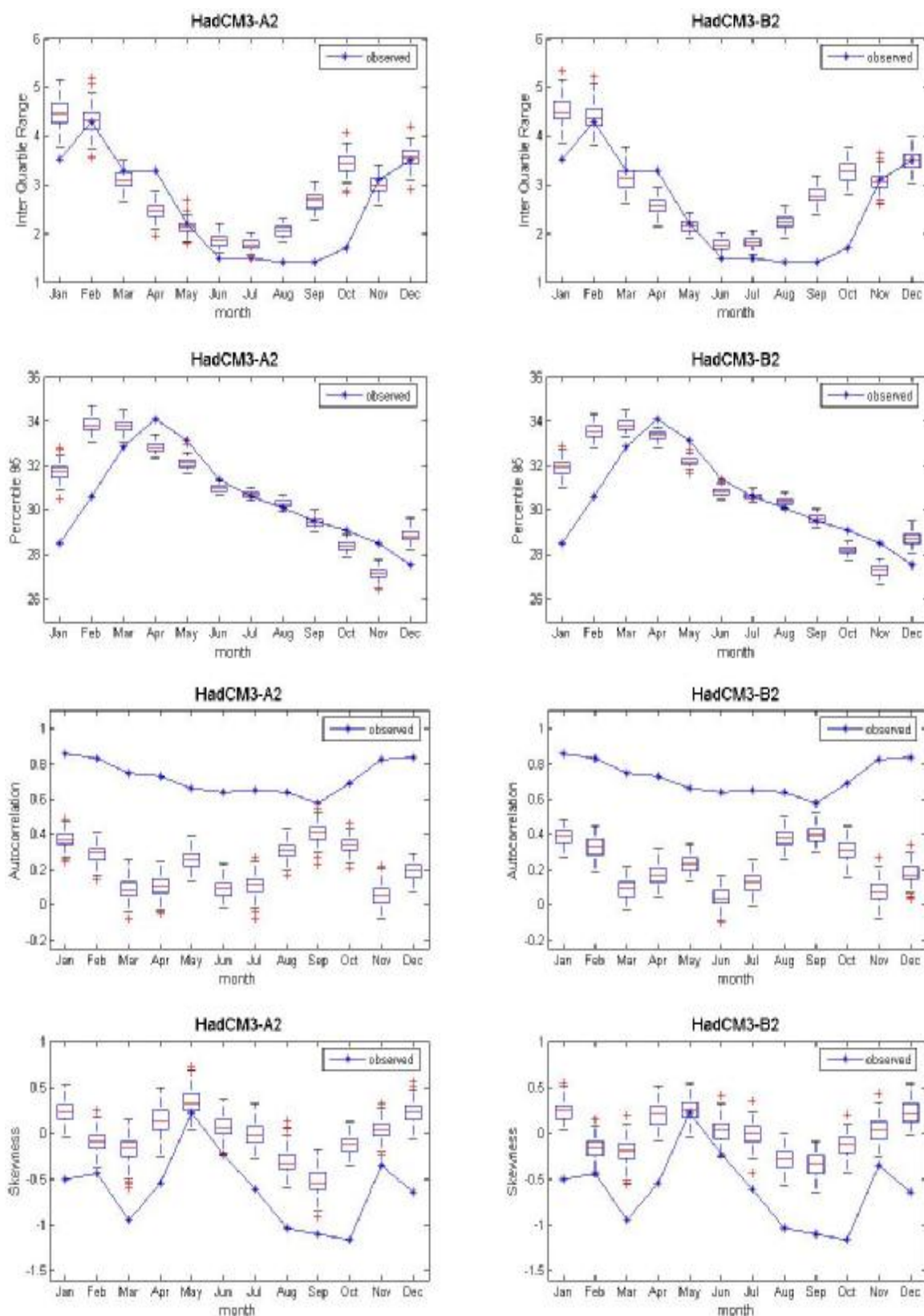
ภาพที่ ค.62 ค่าพิสัยระหว่างควอร์ไทล์ที่ 75 กับควอร์ไทล์ที่ 25 ค่าเปอร์เซ็นต์ไทล์ที่ 95 ค่าสัมประสิทธิ์สหสัมพันธ์ และค่าความเบ้ของข้อมูลอุณหภูมิเฉลี่ยรายวันอดีต และของข้อมูลสังเคราะห์จากภาพฉาย HadCM3A2 และ HadCM3B2 สำหรับสถานี 432401 (ปี ค.ศ.1991-2001)
