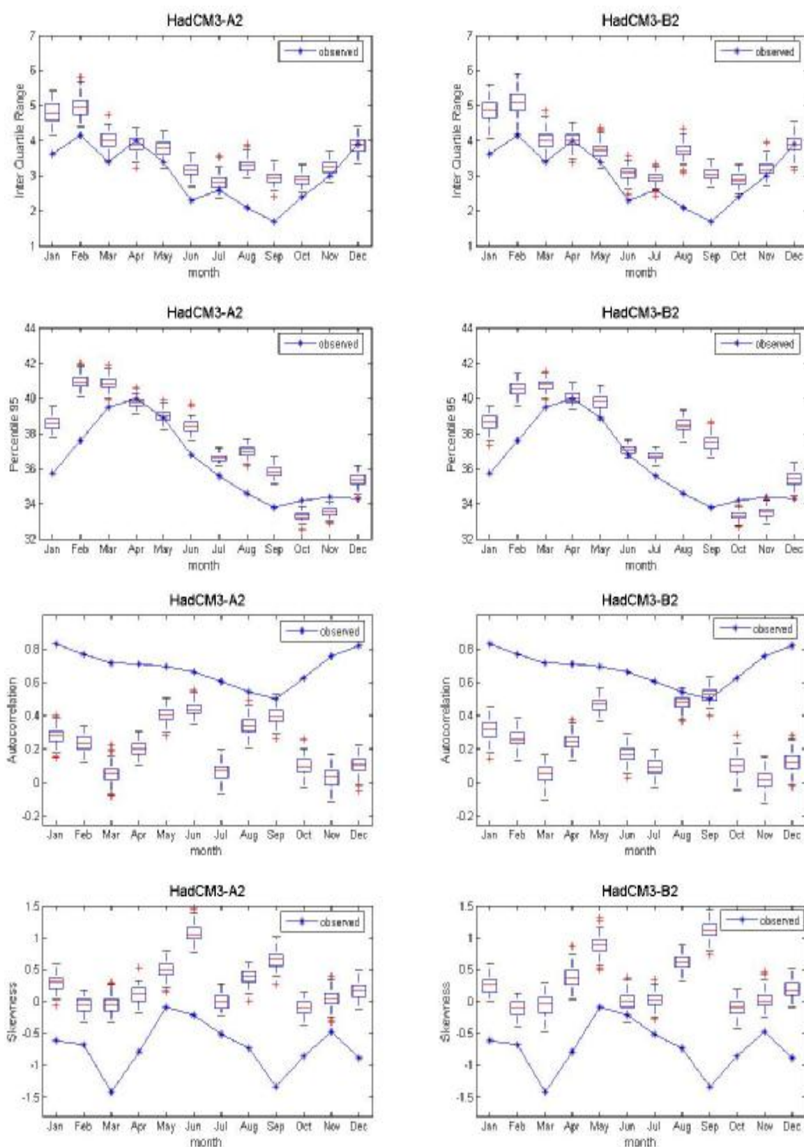
ภาพที่ ค.14 ค่าพิสัยระหว่างควอร์ไทล์ที่ 75 กับควอร์ไทล์ที่ 25 ค่าเปอร์เซ็นต์ไทล์ที่ 95 ค่าสัมประสิทธิ์สหสัมพันธ์ และค่าความเบ้ของข้อมูลอุณหภูมิสูงสุดรายวันอดีต และของข้อมูลสังเคราะห์จากภาพฉาย HadCM3A2 และ HadCM3B2 สำหรับสถานี 403201(ปี ค.ศ.1991-2001)
