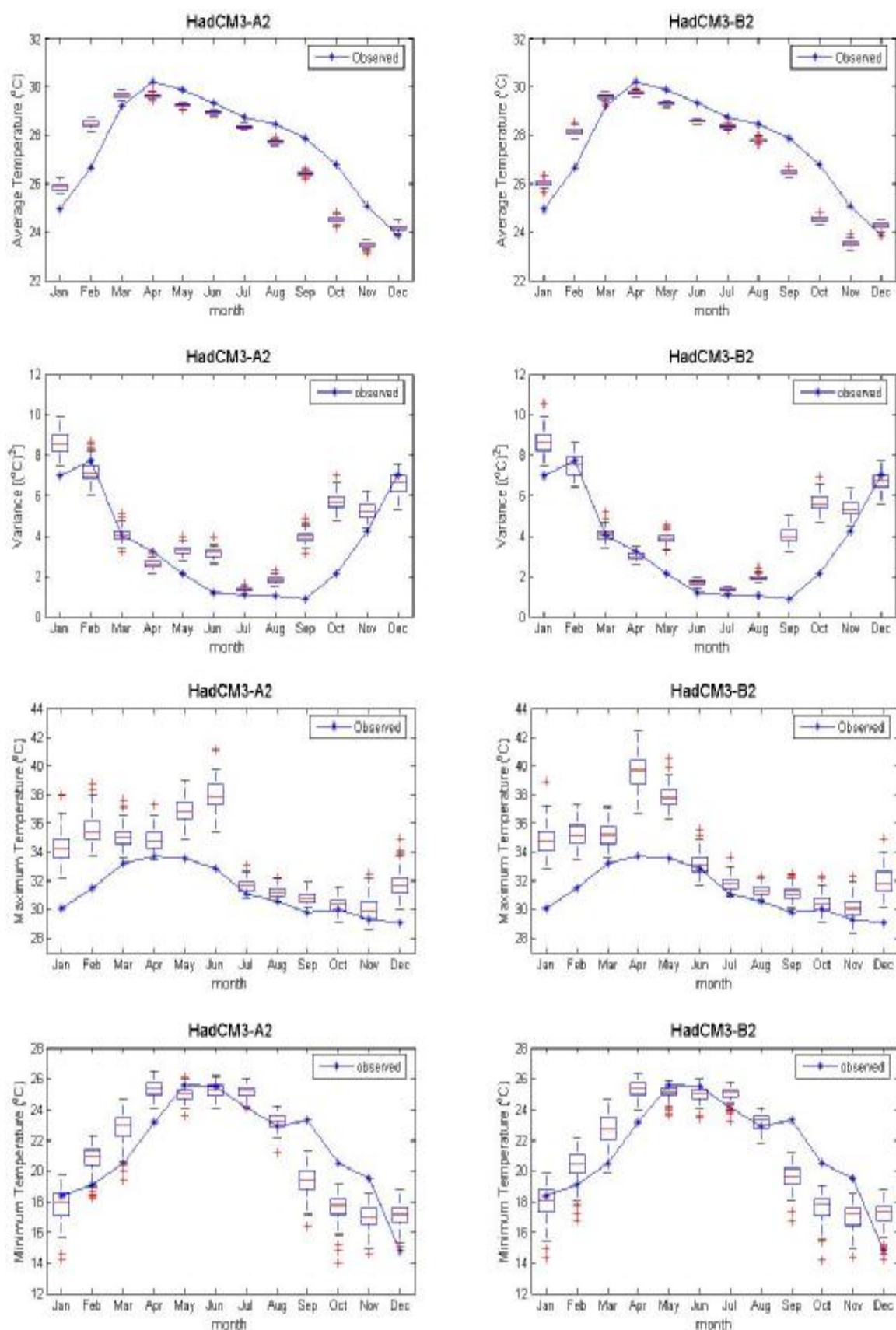
ภาพที่ ค.63 ค่าเฉลี่ย ค่าความแปรปรวน ค่าสูงสุด และค่าต่ำสุดของข้อมูลอุณหภูมิเฉลี่ยรายวันอดีต และของข้อมูลสังเคราะห์จากภาพฉาย HadCM3A2 และ HadCM3B2 สำหรับสถานี 436401 (ปี ค.ศ.1991-2001)
