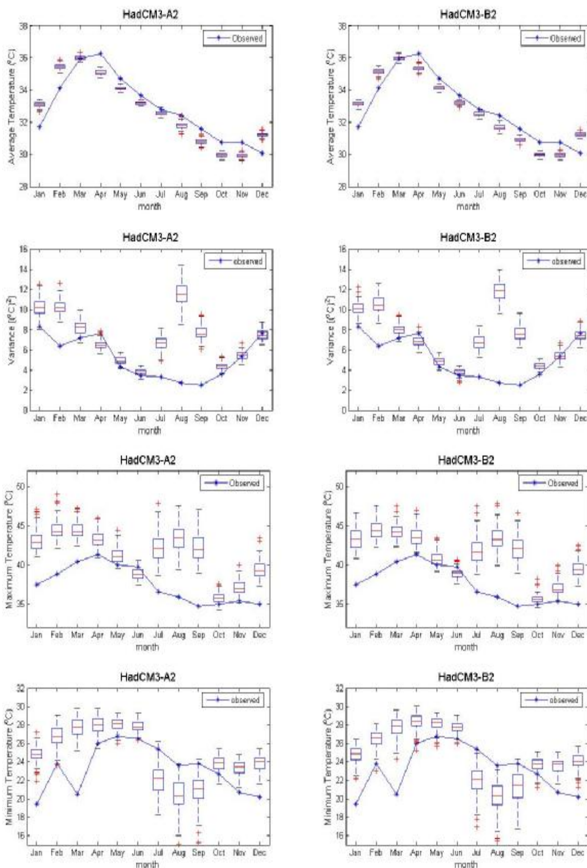
ภาพที่ ค.75 ค่าเฉลี่ย ค่าความแปรปรวน ค่าสูงสุด และค่าต่ำสุดของข้อมูลอุณหภูมิสูงสุดรายวันอดีต และของข้อมูลสังเคราะห์จากภาพฉาย HadCM3A2 และ HadCM3B2 สำหรับสถานี 432301 (ปี ค.ศ.1991-2001)
