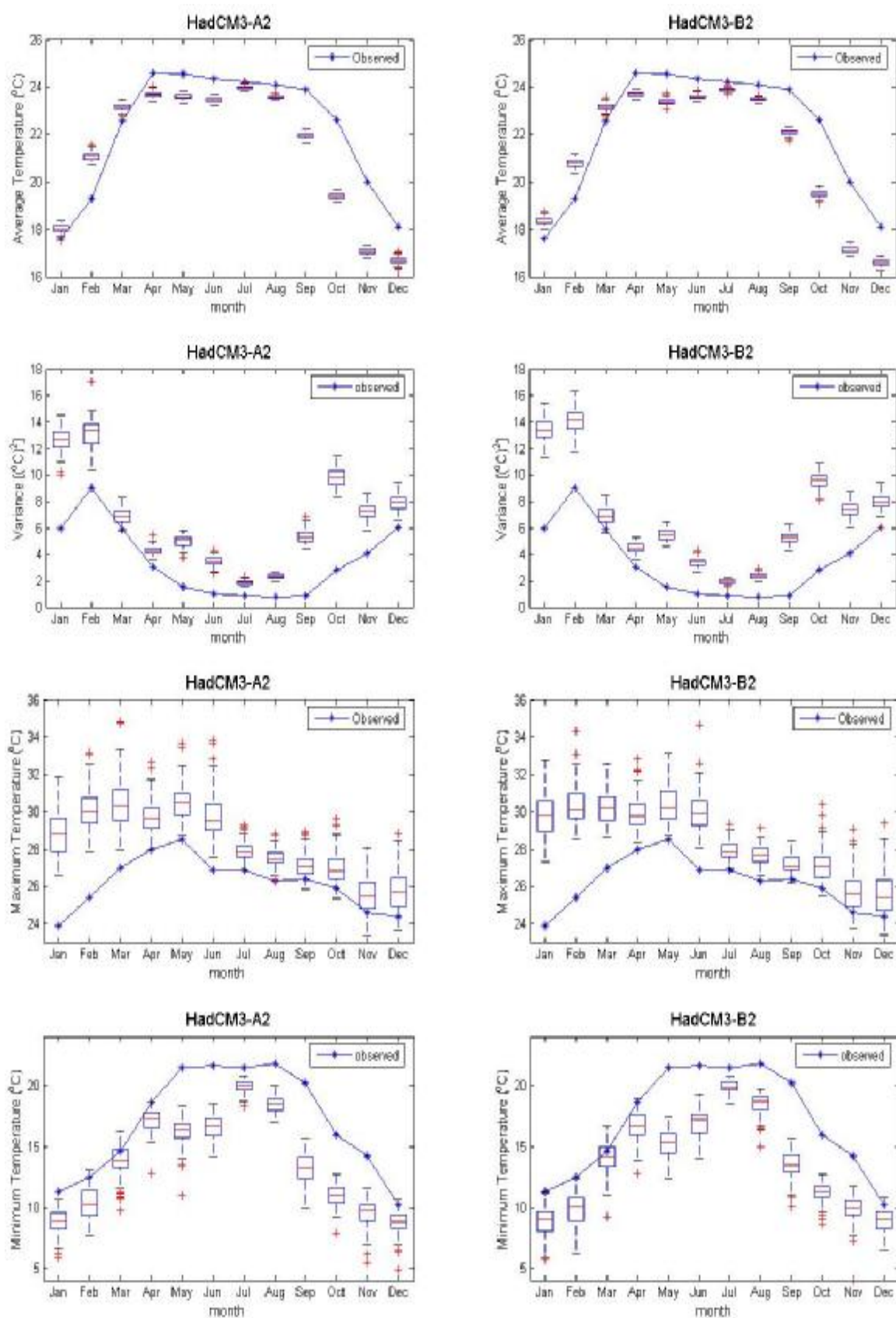
ภาพที่ ค.81 ค่าเฉลี่ย ค่าความแปรปรวน ค่าสูงสุด และค่าต่ำสุดของข้อมูลอุณหภูมิรายวันอดีต และของข้อมูลสังเคราะห์จากภาพฉาย HadCM3A2 และ HadCM3B2 สำหรับสถานี 407301 (ปี ค.ศ.1991-2001)
