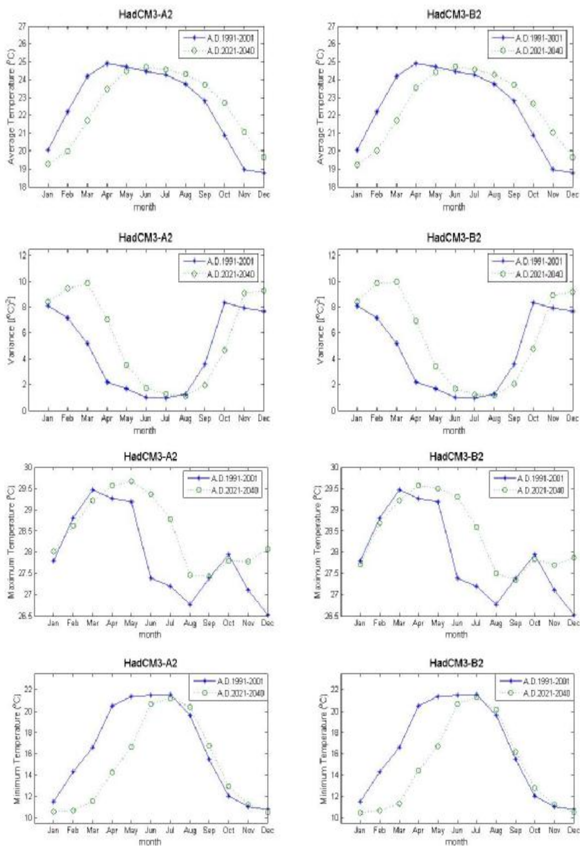
ภาพที่ ค.45 ค่าเฉลี่ย ค่าความแปรปรวน ค่าสูงสุด และค่าต่ำสุดของข้อมูลอุณหภูมิรายวันสังเคราะห์จากภาพฉาย HadCM3A2 และ HadCM3B2 สำหรับช่วงปี ค.ศ.1991-2001 และช่วงปี ค.ศ.2021-2040 (สถานี 403201)
