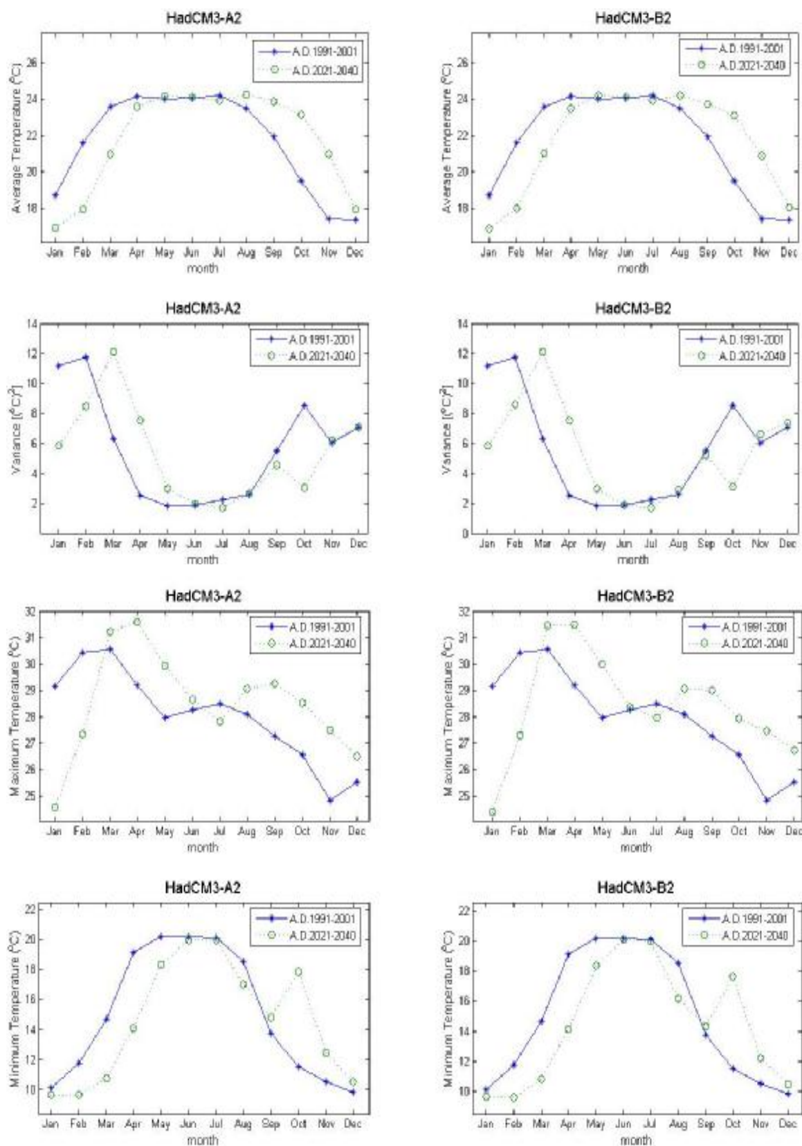
ภาพที่ ค.131 ค่าเฉลี่ย ค่าความแปรปรวน ค่าสูงสุด และค่าต่ำสุดของข้อมูลอุณหภูมิรายวันสังเคราะห์จาก ภาพฉาย HadCM3A2 และ HadCM3B2 สำหรับช่วงปี ค.ศ.1991-2001 และช่วงปี ค.ศ.2021-2040 (สถานี 407501)
