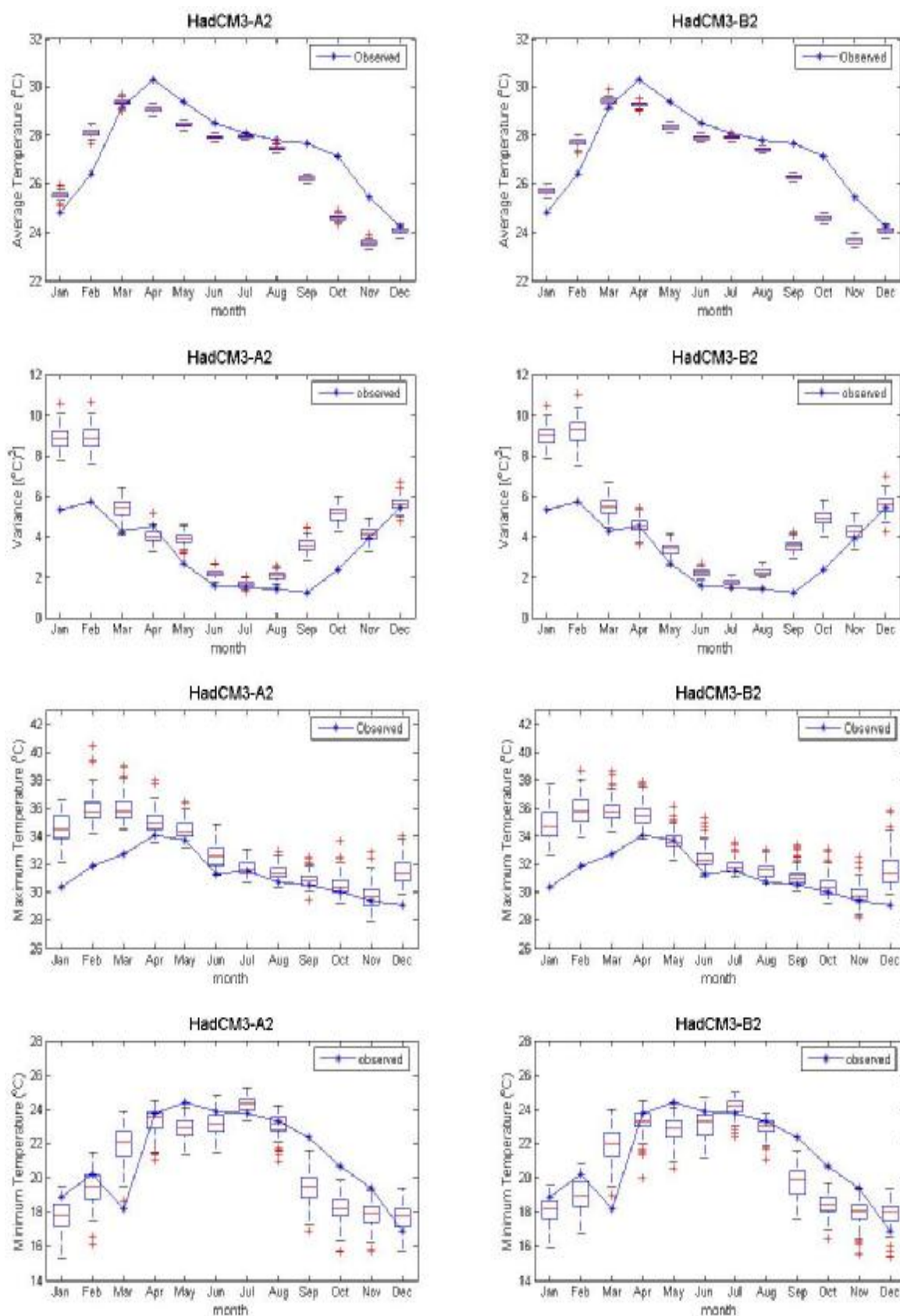
ภาพที่ ค.49 ค่าเฉลี่ย ค่าความแปรปรวน ค่าสูงสุด และค่าต่ำสุดของข้อมูลอุณหภูมิเฉลี่ยรายวันอดีต และของข้อมูลสังเคราะห์จากภาพฉาย HadCM3A2 และ HadCM3B2 สำหรับสถานี 407301 (ปี ค.ศ.1991-2001)
