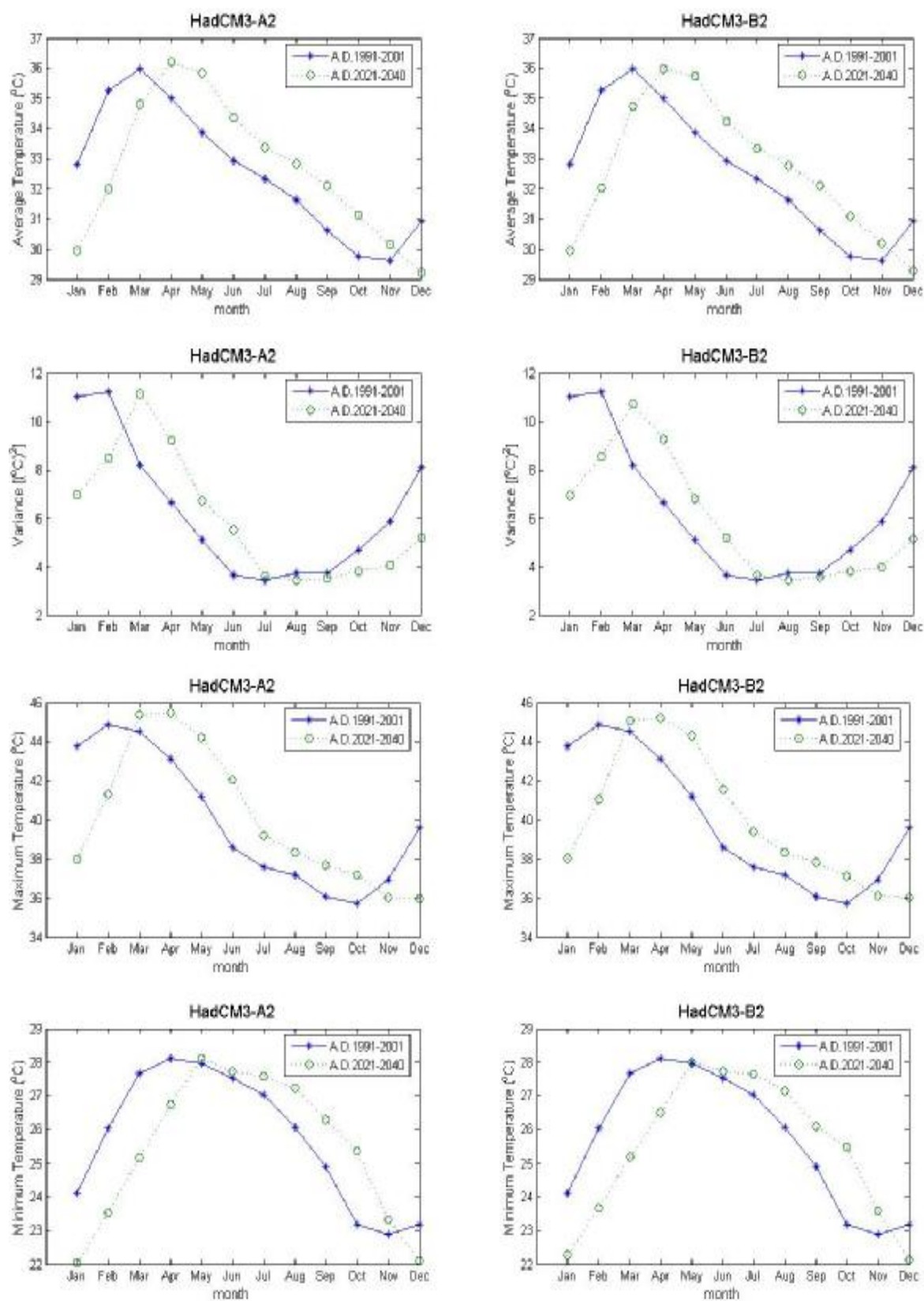
ภาพที่ ค.125 ค่าเฉลี่ย ค่าความแปรปรวน ค่าสูงสุด และค่าต่ำสุดของข้อมูลอุณหภูมิสูงสุดรายวันสังเคราะห์จาก ภาพฉาย HadCM3A2 และ HadCM3B2 สำหรับช่วงปี ค.ศ.1991-2001 และช่วงปี ค.ศ.2021-2040 (สถานี 432401)
