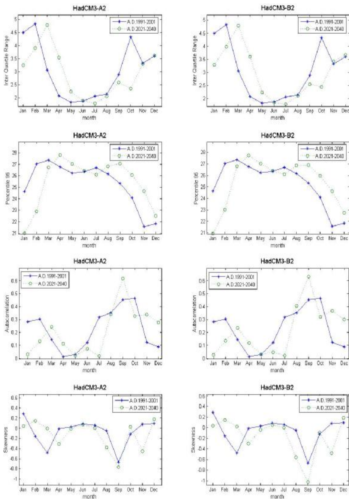
ภาพที่ ค.132 ค่าพิสัยระหว่างควอร์ไทล์ที่ 75 กับควอร์ไทล์ที่ 25 ค่าเปอร์เซ็นต์ไทล์ที่ 95 ค่าสัมประสิทธิ์สหสัมพันธ์ และค่าสัมประสิทธิ์ความเบ้ของข้อมูลอุณหภูมิต่ำสุดรายวันสังเคราะห์จากภาพฉาย HadCM3A2 และ HadCM3B2 สำหรับช่วงปี ค.ศ.1991-2001 และช่วงปี ค.ศ.2021-2040 (สถานี 407501)
