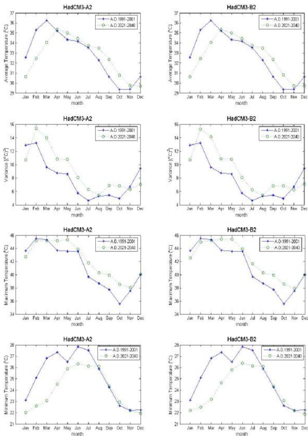
ภาพที่ ค.115 ค่าเฉลี่ย ค่าความแปรปรวน ค่าสูงสุด และค่าต่ำสุดของข้อมูลอุณหภูมิสูงสุดรายวันสังเคราะห์จาก ภาพฉาย HadCM3A2 และ HadCM3B2 สำหรับช่วงปี ค.ศ.1991-2001 และช่วงปี ค.ศ.2021-2040 (สถานี 431201)
