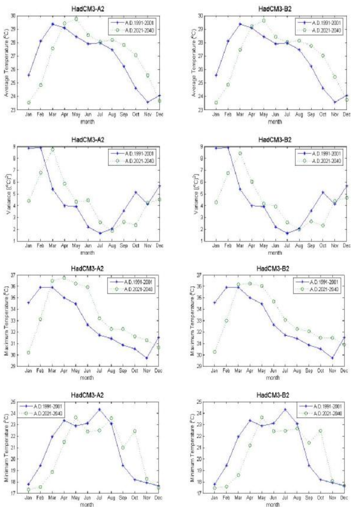
ภาพที่ ค.97 ค่าเฉลี่ย ค่าความแปรปรวน ค่าสูงสุด และค่าต่ำสุดของข้อมูลอุณหภูมิเฉลี่ยรายวันสังเคราะห์จากภาพฉาย HadCM3A2 และ HadCM3B2 สำหรับช่วงปี ค.ศ.1991-2001 และช่วงปี ค.ศ.2021-2040 (สถานี 407301)
