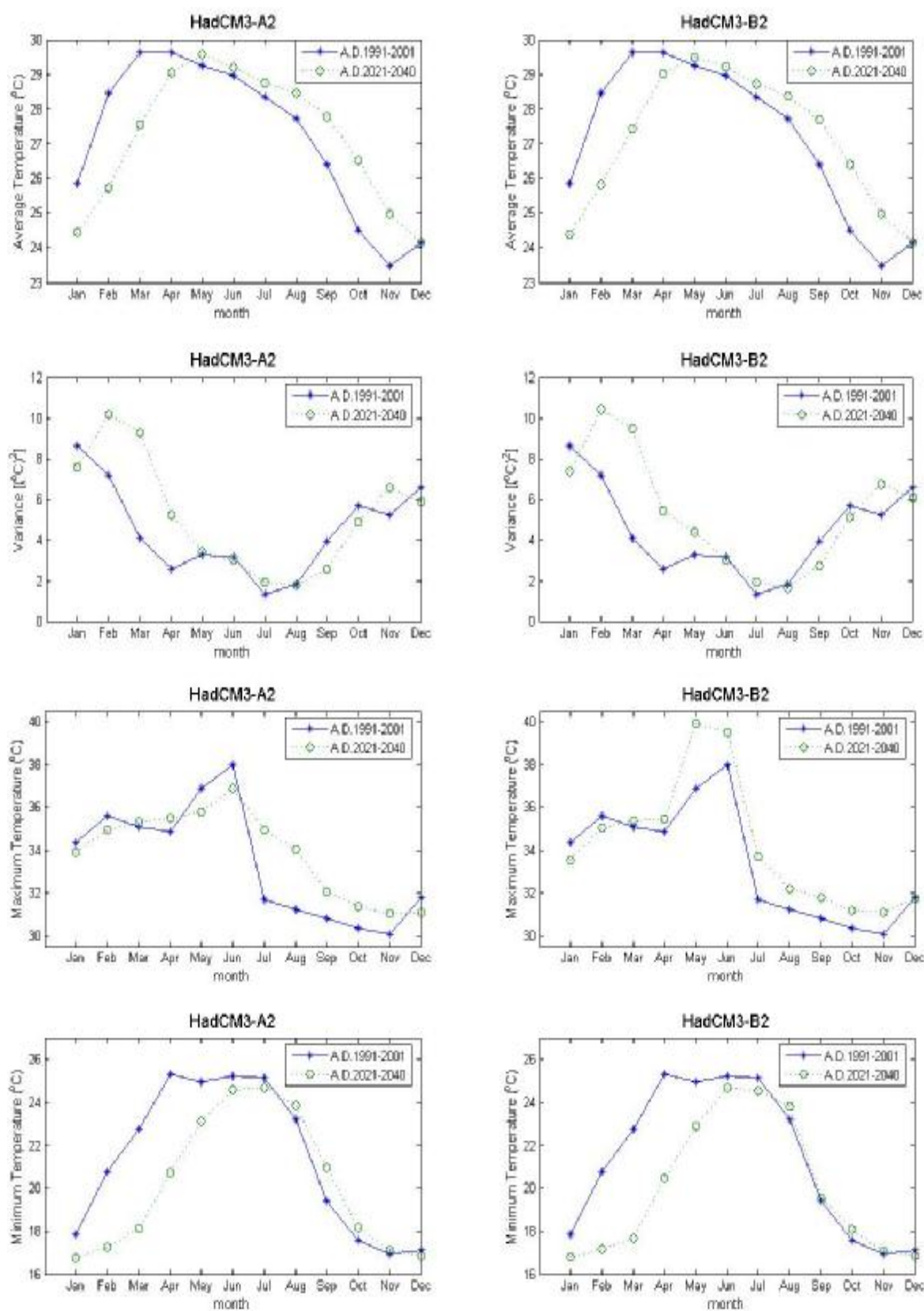
ภาพที่ ค.111 ค่าเฉลี่ย ค่าความแปรปรวน ค่าสูงสุด และค่าต่ำสุดของข้อมูลอุณหภูมิเฉลี่ยรายวันสังเคราะห์จาก ภาพฉาย HadCM3A2 และ HadCM3B2 สำหรับช่วงปี ค.ศ.1991-2001 และช่วงปี ค.ศ.2021-2040 (สถานี 436401)
