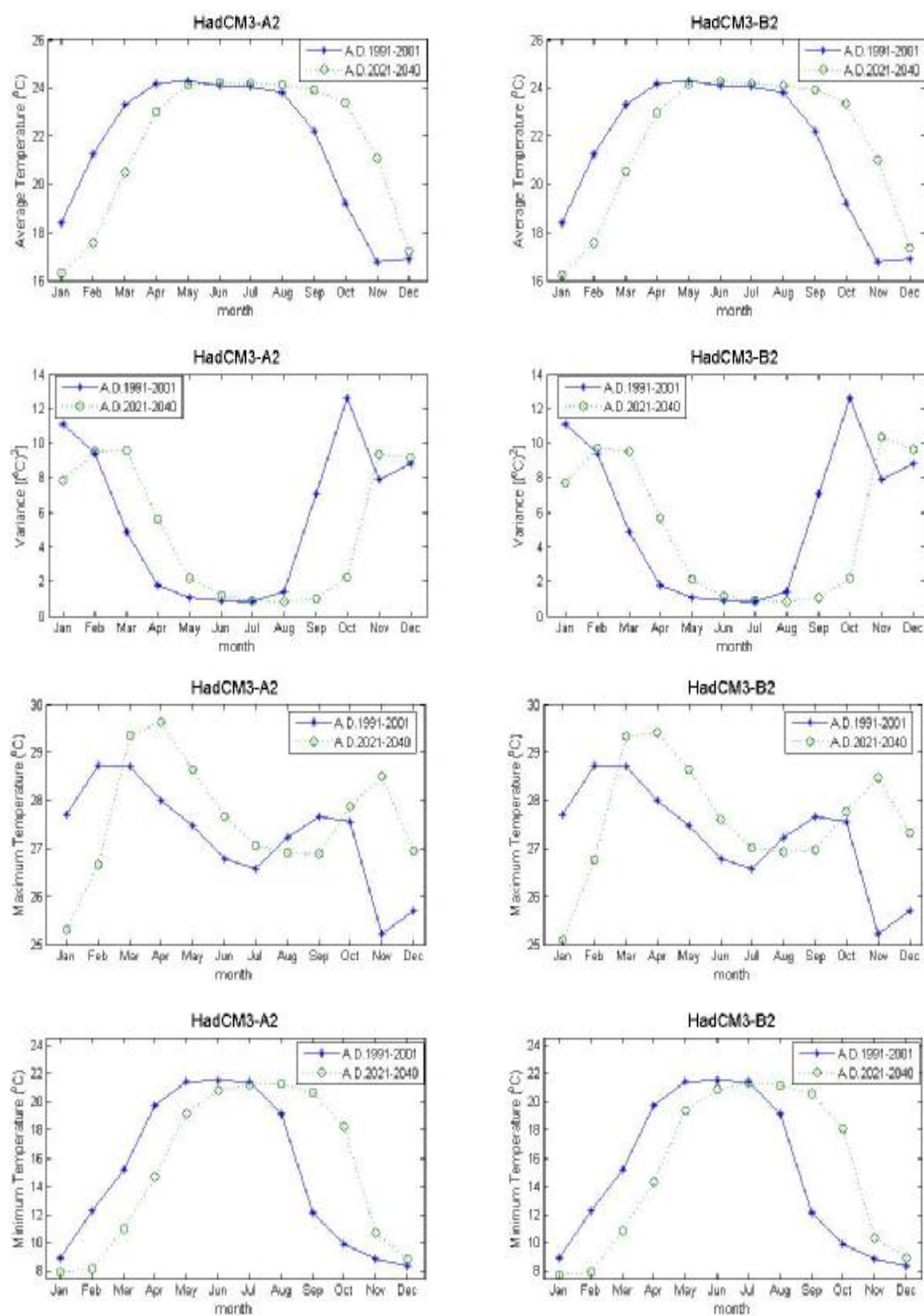
ภาพที่ ค.139 ค่าเฉลี่ย ค่าความแปรปรวน ค่าสูงสุด และค่าต่ำสุดของข้อมูลอุณหภูมิรายวันสังเคราะห์จาก ภาพฉาย HadCM3A2 และ HadCM3B2 สำหรับช่วงปี ค.ศ.1991-2001 และช่วงปี ค.ศ.2021-2040 (สถานี 432301)
