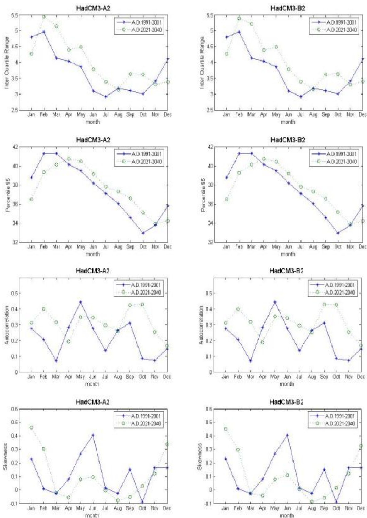
ภาพที่ ค.116 ค่าพิสัยระหว่างควอร์ไทล์ที่ 75 กับควอร์ไทล์ที่ 25 ค่าเปอร์เซ็นต์ไทล์ที่ 95 ค่าสัมประสิทธิ์สหสัมพันธ์ และค่าสัมประสิทธิ์ความเบ้ของข้อมูลอุณหภูมิสูงสุดรายวันสังเคราะห์จากภาพฉาย HadCM3A2 และ HadCM3B2 สำหรับช่วงปี ค.ศ.1991-2001 และช่วงปี ค.ศ.2021-2040 (สถานี 431201)
