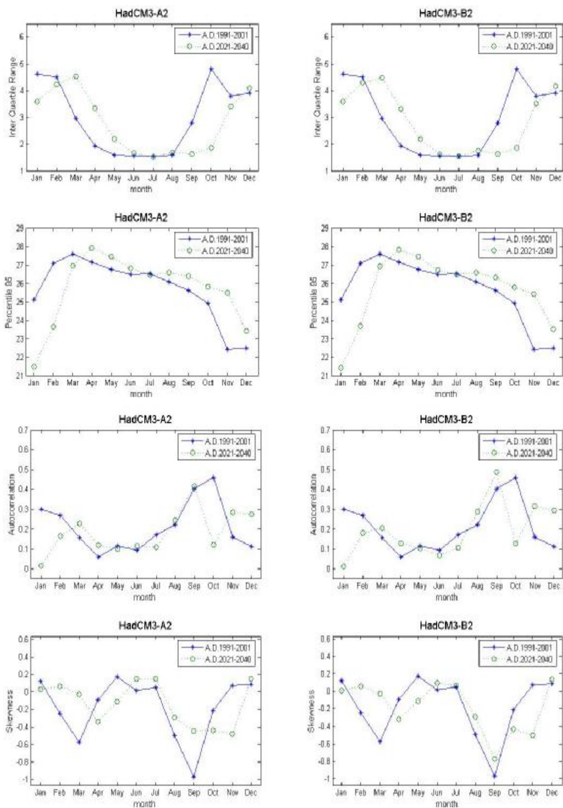
ภาพที่ ค.142 ค่าพิสัยระหว่างควอร์ไทล์ที่ 75 กับควอร์ไทล์ที่ 25 ค่าเปอร์เซ็นต์ไทล์ที่ 95 ค่าสัมประสิทธิ์สหสัมพันธ์ และค่าสัมประสิทธิ์ความเบ้ของข้อมูลอุณหภูมิต่ำสุดรายวันสังเคราะห์จากภาพฉาย HadCM3A2 และ HadCM3B2 สำหรับช่วงปี ค.ศ.1991-2001 และช่วงปี ค.ศ.2021-2040 (สถานี 432401)
