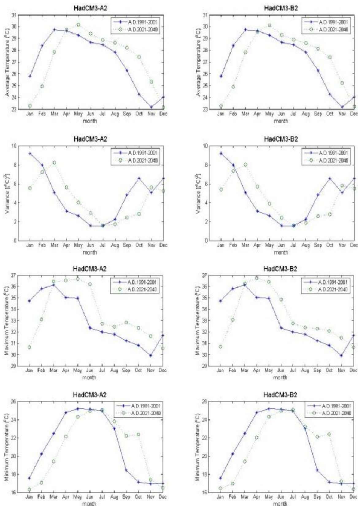
ภาพที่ ค.107 ค่าเฉลี่ย ค่าความแปรปรวน ค่าสูงสุด และค่าต่ำสุดของข้อมูลอุณหภูมิเฉลี่ยรายวันสังเคราะห์จาก ภาพฉาย HadCM3A2 และ HadCM3B2 สำหรับช่วงปี ค.ศ.1991-2001 และช่วงปี ค.ศ.2021-2040 (สถานี 432301)
