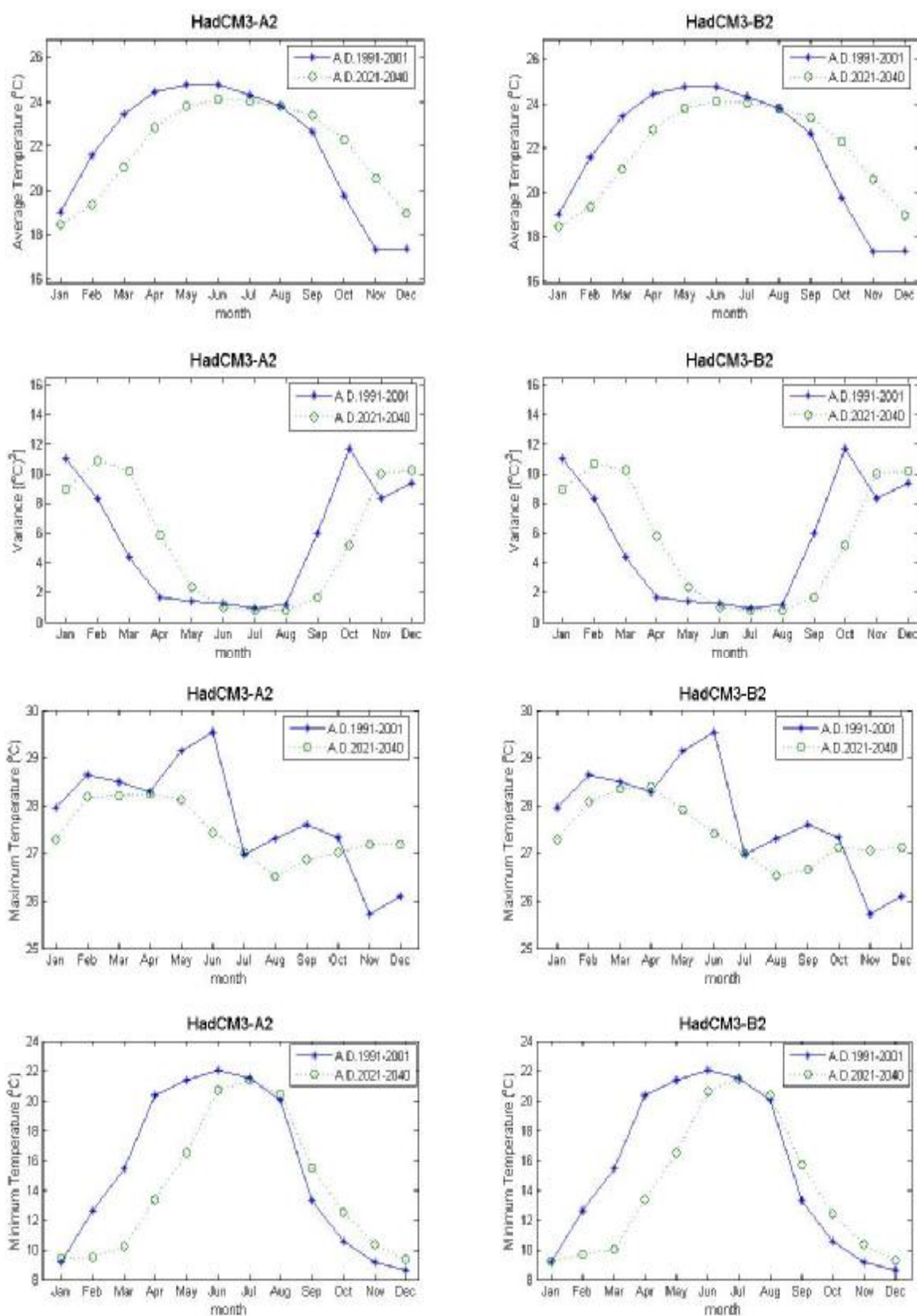
ภาพที่ ค.143 ค่าเฉลี่ย ค่าความแปรปรวน ค่าสูงสุด และค่าต่ำสุดของข้อมูลอุณหภูมิรายวันสังเคราะห์จาก ภาพฉาย HadCM3A2 และ HadCM3B2 สำหรับช่วงปี ค.ศ.1991-2001 และช่วงปี ค.ศ.2021-2040 (สถานี 436401)
