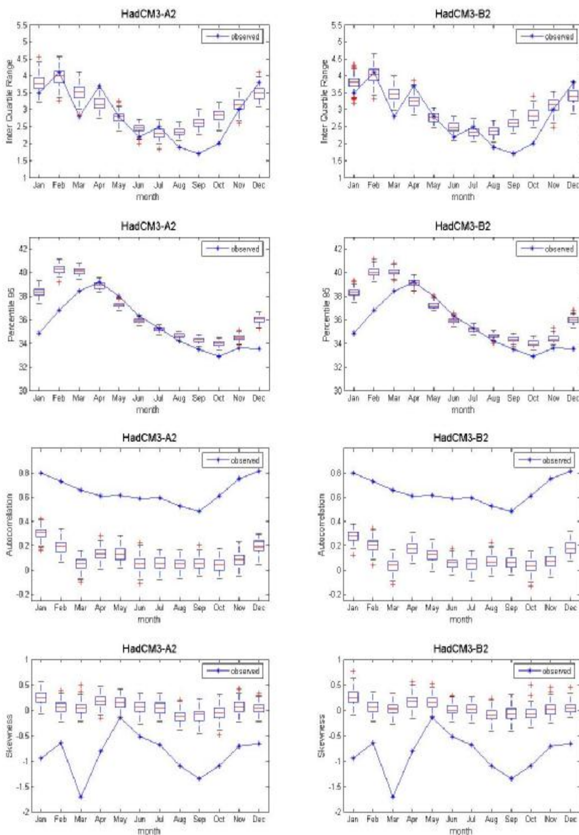
ภาพที่ ค.74 ค่าพิสัยระหว่างควอร์ไทล์ที่ 75 กับควอร์ไทล์ที่ 25 ค่าเปอร์เซ็นต์ไทล์ที่ 95 ค่าสัมประสิทธิ์สหสัมพันธ์ และค่าความเบ้ของข้อมูลอุณหภูมิสูงสุดรายวันอดีต และของข้อมูลสังเคราะห์จากภาพฉาย HadCM3A2 และ HadCM3B2 สำหรับสถานี 432201 (ปี ค.ศ.1991-2001)
