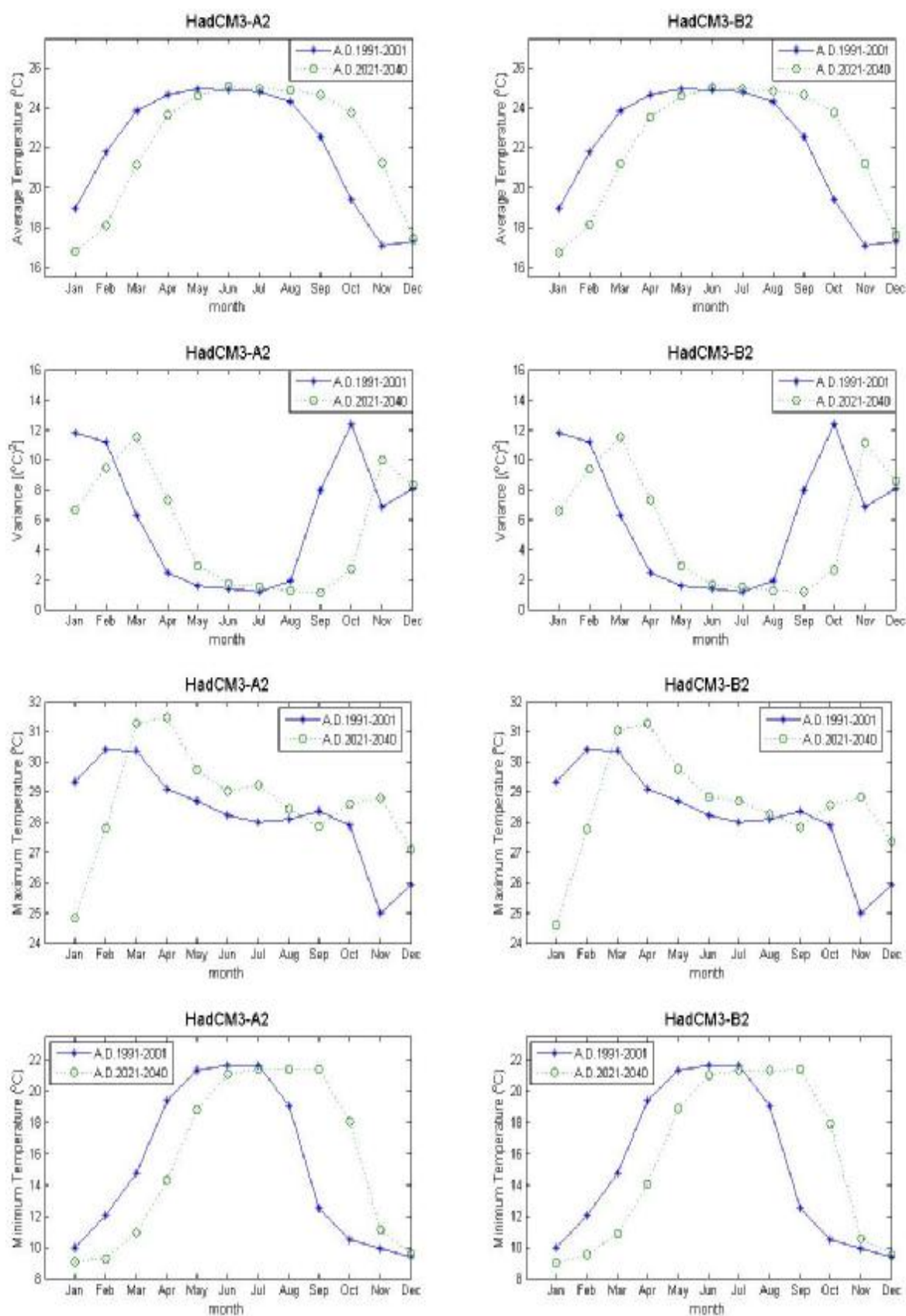
ภาพที่ ค.47 ค่าเฉลี่ย ค่าความแปรปรวน ค่าสูงสุด และค่าต่ำสุดของข้อมูลอุณหภูมิรายวันสังเคราะห์จากภาพฉาย HadCM3A2 และ HadCM3B2 สำหรับช่วงปี ค.ศ.1991-2001 และช่วงปี ค.ศ.2021-2040 (สถานี 405201)
