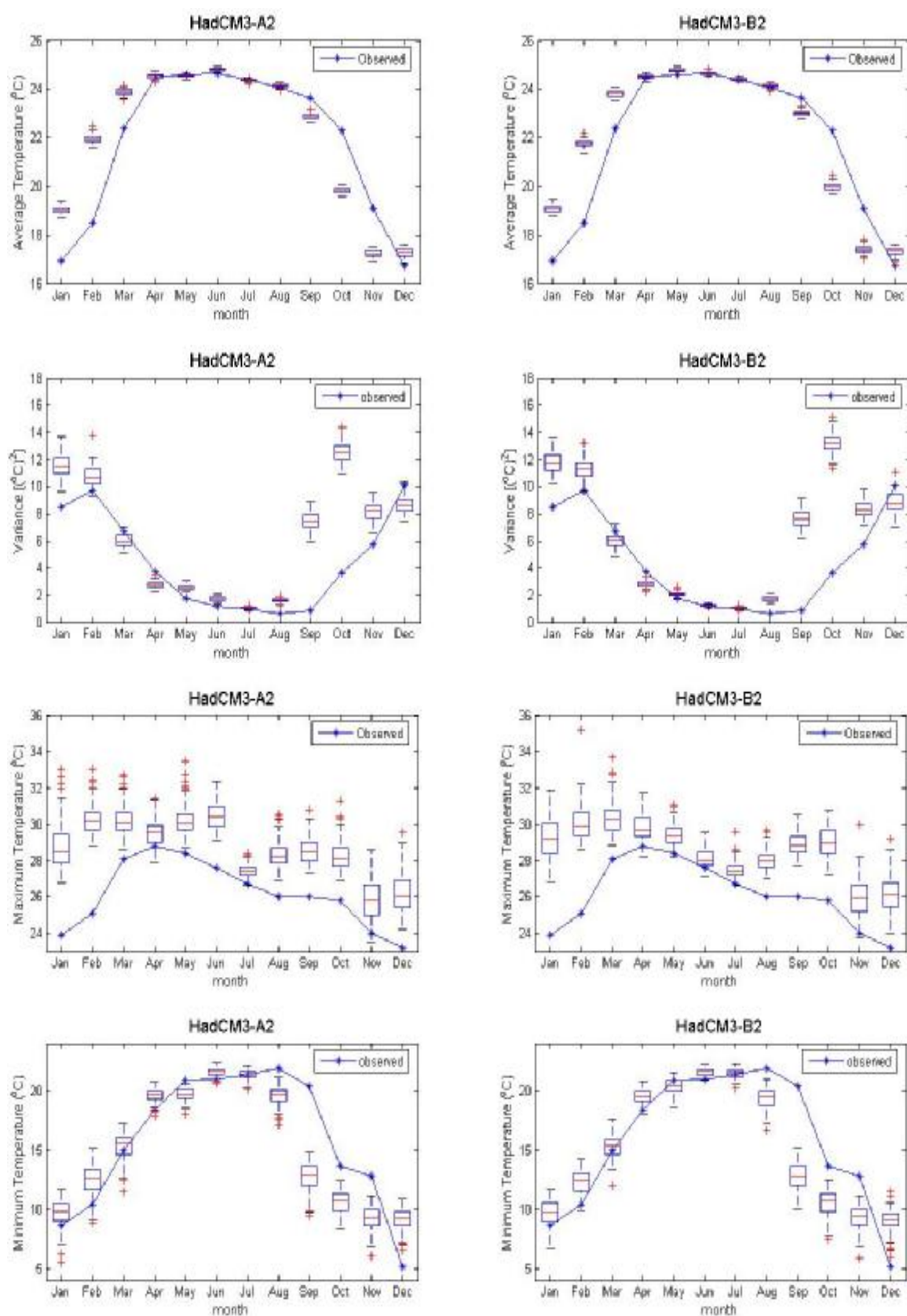
ภาพที่ ค.19 ค่าเฉลี่ย ค่าความแปรปรวน ค่าสูงสุด และค่าต่ำสุดของข้อมูลอุณหภูมิต่ำสุดรายวันอดีต และของข้อมูลสังเคราะห์จากภาพฉาย HadCM3A2 และ HadCM3B2 สำหรับสถานี 381301 (ปี ค.ศ.1991-2001)
