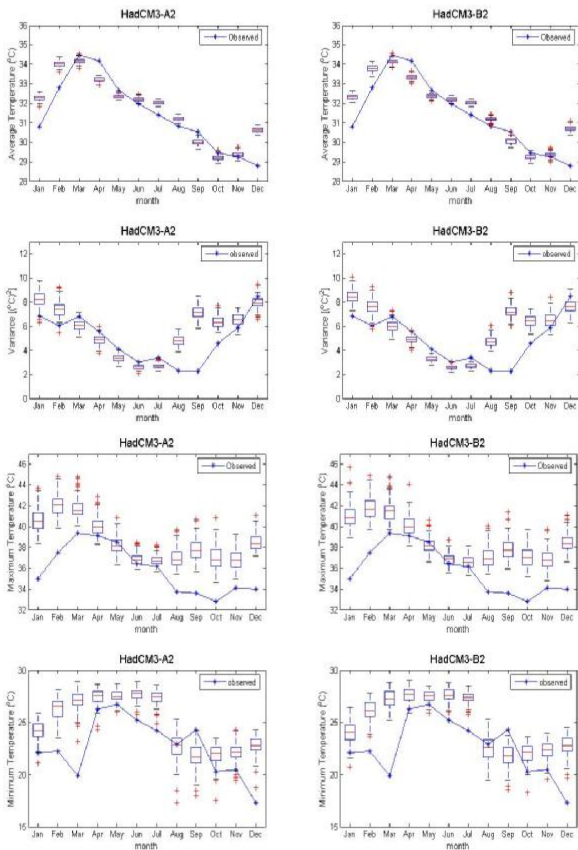
ภาพที่ ค.69 ค่าเฉลี่ย ค่าความแปรปรวน ค่าสูงสุด และค่าต่ำสุดของข้อมูลอุณหภูมิสูงสุดรายวันอดีต และของข้อมูลสังเคราะห์จากภาพฉาย HadCM3A2 และ HadCM3B2 สำหรับสถานี 431301 (ปี ค.ศ.1991-2001)
