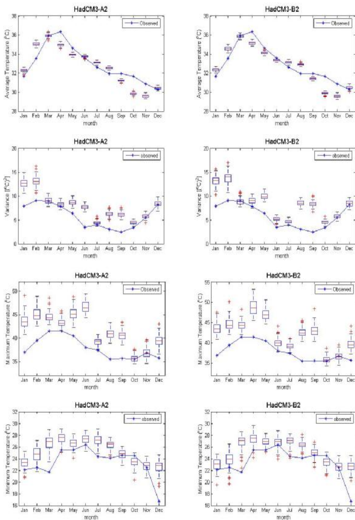
ภาพที่ ค.13 ค่าเฉลี่ย ค่าความแปรปรวน ค่าสูงสุด และค่าต่ำสุดของข้อมูลอุณหภูมิสูงสุดรายวันอดีต และของข้อมูลสังเคราะห์จากภาพฉาย HadCM3A2 และ HadCM3B2 สำหรับสถานี 403201 (ปี ค.ศ.1991-2001)
