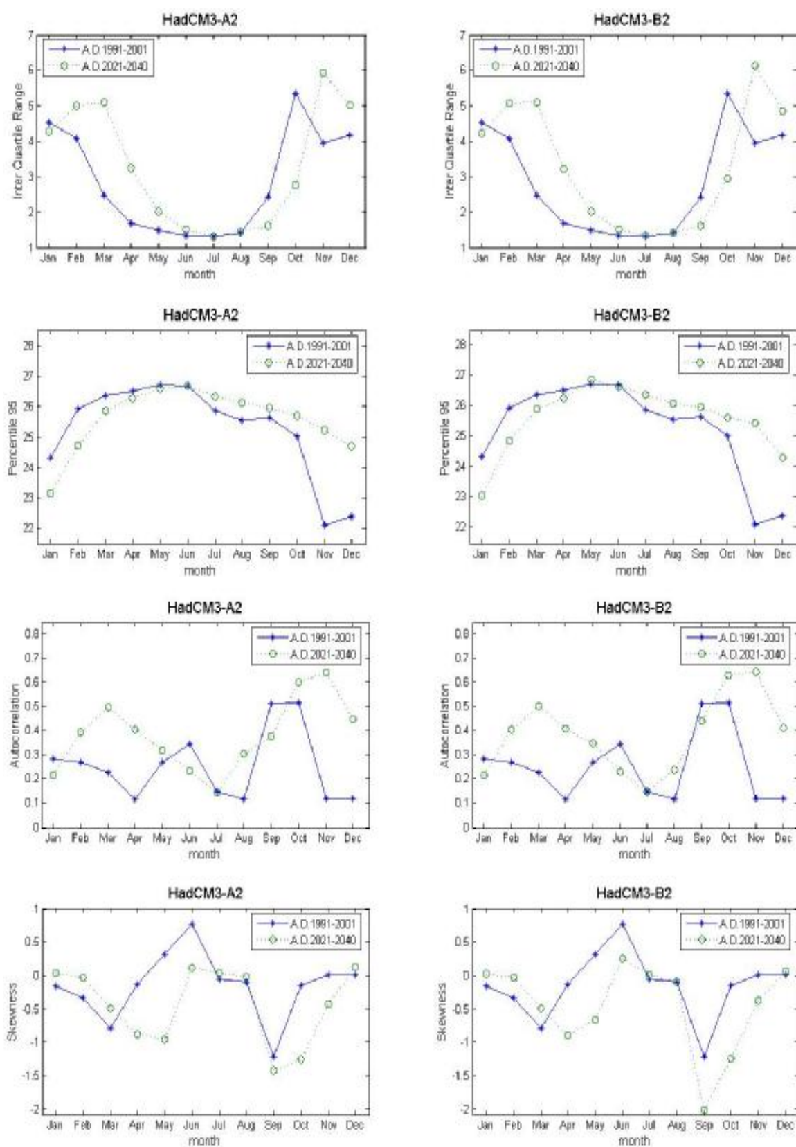
ภาพที่ ค.138 ค่าพิสัยระหว่างควอร์ไทล์ที่ 75 กับควอร์ไทล์ที่ 25 ค่าเปอร์เซ็นต์ไทล์ที่ 95 ค่าสัมประสิทธิ์สหสัมพันธ์ และค่าสัมประสิทธิ์ความเบ้ของข้อมูลอุณหภูมิต่ำสุดรายวันสังเคราะห์จากภาพฉาย HadCM3A2 และ HadCM3B2 สำหรับช่วงปี ค.ศ.1991-2001 และช่วงปี ค.ศ.2021-2040 (สถานี 431401)
