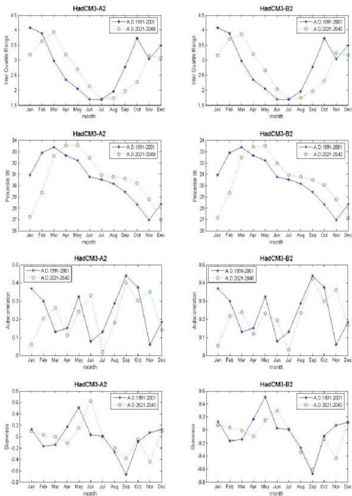
ภาพที่ ค.108 ค่าพิสัยระหว่างควอร์ไทล์ที่ 75 กับควอร์ไทล์ที่ 25 ค่าเปอร์เซ็นต์ไทล์ที่ 95 ค่าสัมประสิทธิ์สหสัมพันธ์ และค่าสัมประสิทธิ์ความเบ้ของข้อมูลอุณหภูมิเฉลี่ยรายวันสังเคราะห์จากภาพฉาย HadCM3A2 และ HadCM3B2 สำหรับช่วงปี ค.ศ.1991-2001 และช่วงปี ค.ศ.2021-2040 (สถานี 432301)
