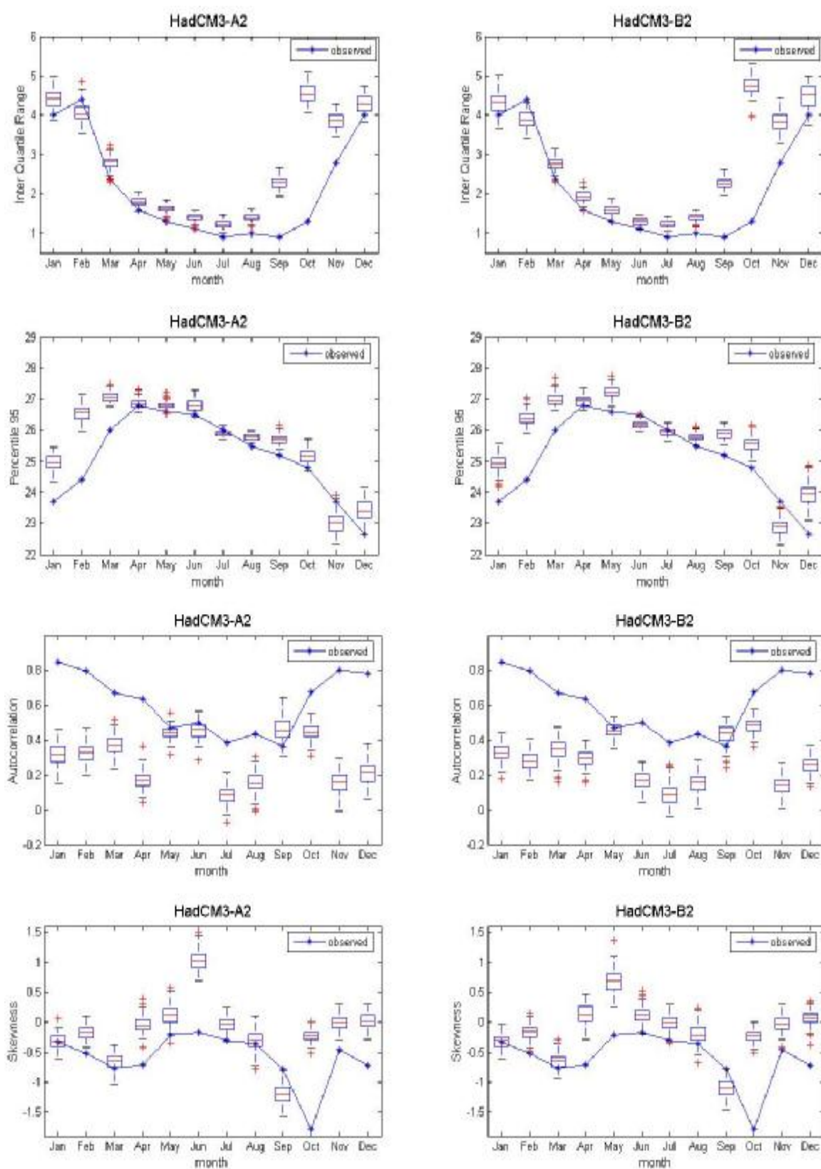
ภาพที่ ค.86 ค่าพิสัยระหว่างควอร์ไทล์ที่ 75 กับควอร์ไทล์ที่ 25 ค่าเปอร์เซ็นต์ไทล์ที่ 95 ค่าสัมประสิทธิ์สหสัมพันธ์ และค่าความเบ้ของข้อมูลอุณหภูมิต่ำสุดรายวันอดีต และของข้อมูลสังเคราะห์จากภาพฉาย HadCM3A2 และ HadCM3B2 สำหรับสถานี 431201 (ปี ค.ศ.1991-2001)
