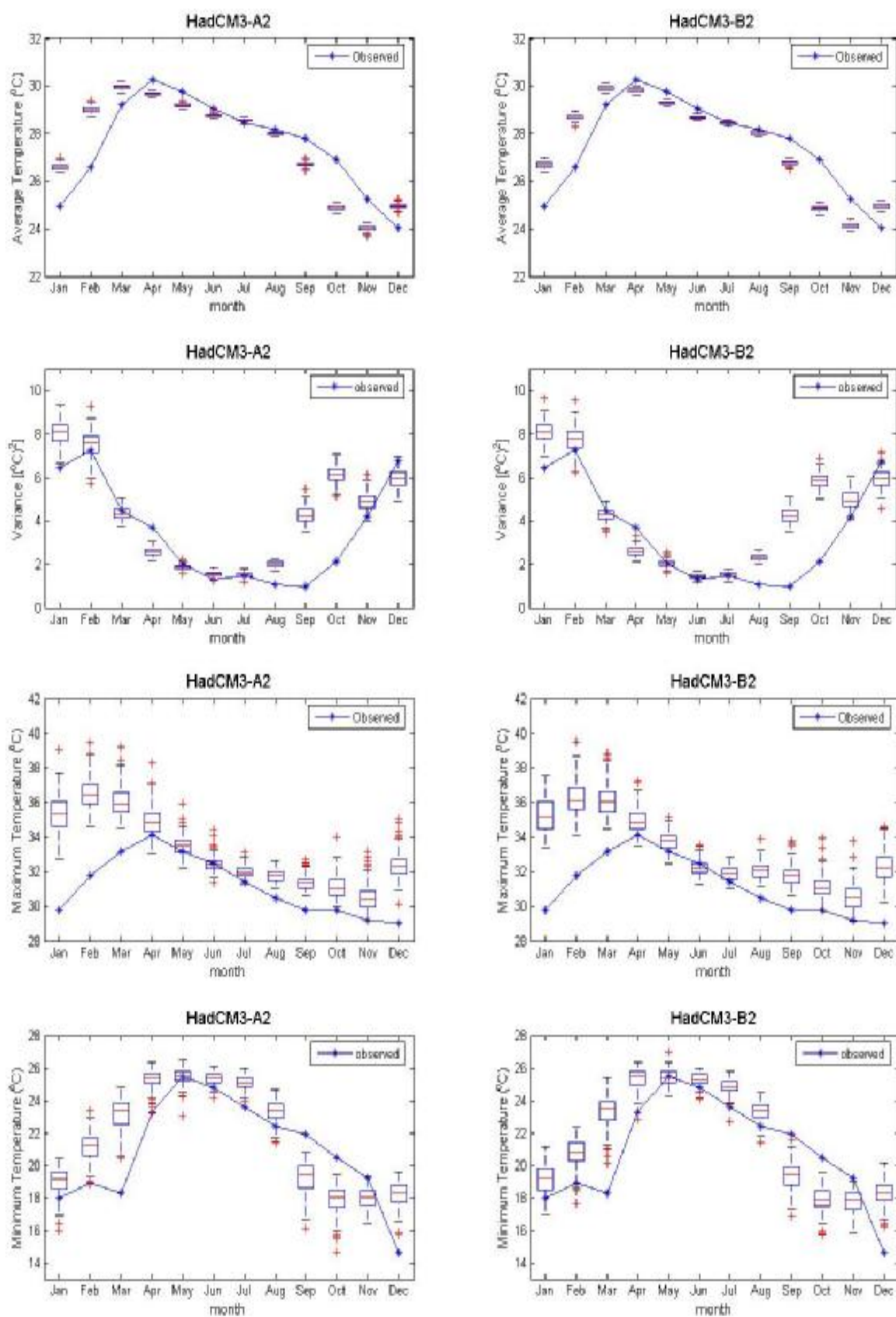
ภาพที่ ค.57 ค่าเฉลี่ย ค่าความแปรปรวน ค่าสูงสุด และค่าต่ำสุดของข้อมูลอุณหภูมิเฉลี่ยรายวันอดีต และของข้อมูลสังเคราะห์จากภาพฉาย HadCM3A2 และ HadCM3B2 สำหรับสถานี 432201 (ปี ค.ศ.1991-2001)
