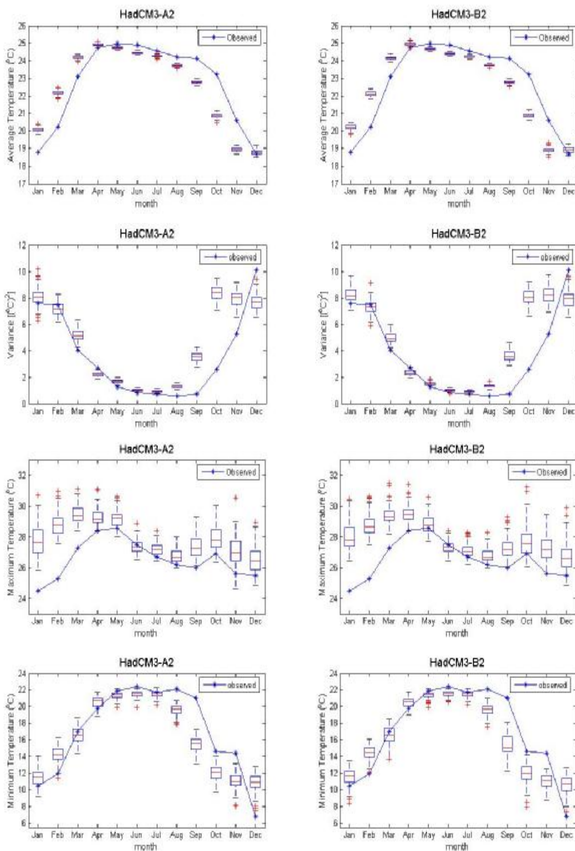
ภาพที่ ค.21 ค่าเฉลี่ย ค่าความแปรปรวน ค่าสูงสุด และค่าต่ำสุดของข้อมูลอุณหภูมิรายวันอดีต และของข้อมูลสังเคราะห์จากภาพฉาย HadCM3A2 และ HadCM3B2 สำหรับสถานี 403201 (ปี ค.ศ.1991-2001)
