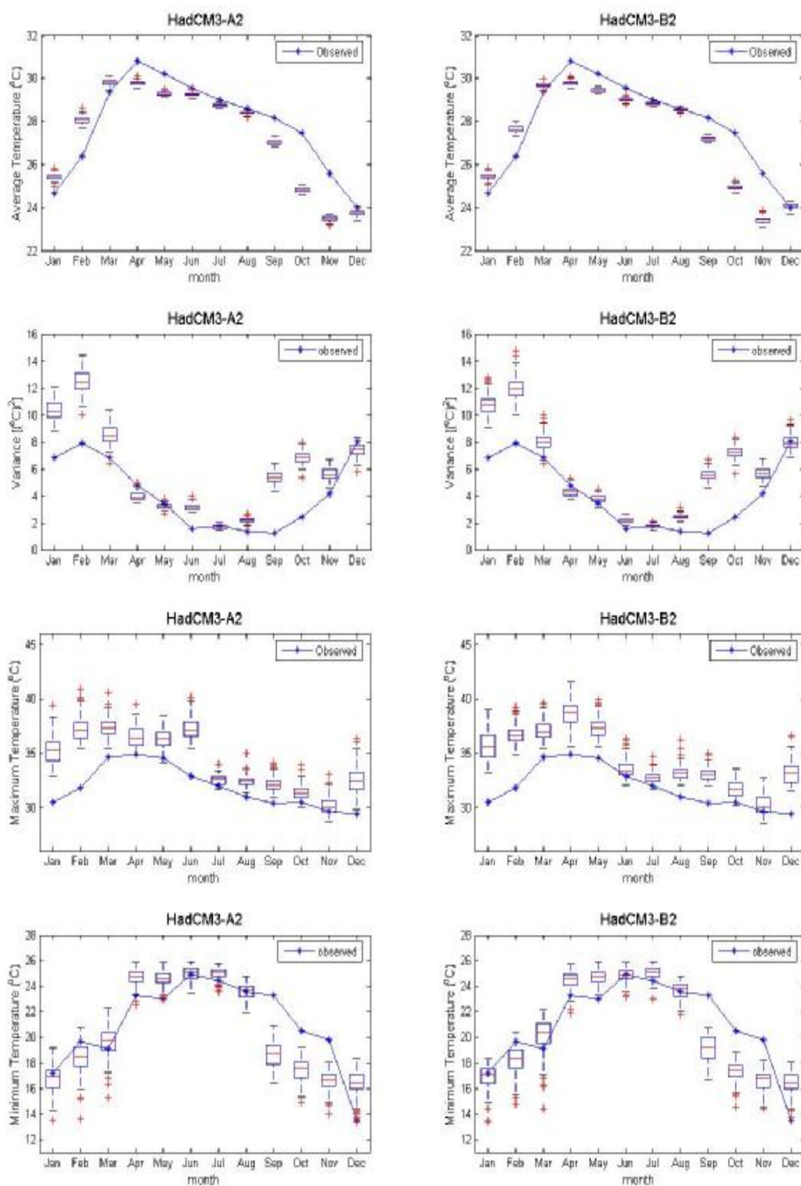
ภาพที่ ค.3 ค่าเฉลี่ย ค่าความแปรปรวน ค่าสูงสุด และค่าต่ำสุดของข้อมูลอุณหภูมิเฉลี่ยรายวันอดีต และของข้อมูลสังเคราะห์จากภาพฉาย HadCM3A2 และ HadCM3B2 สำหรับสถานี 387401 (ปี ค.ศ.1991-2001)
