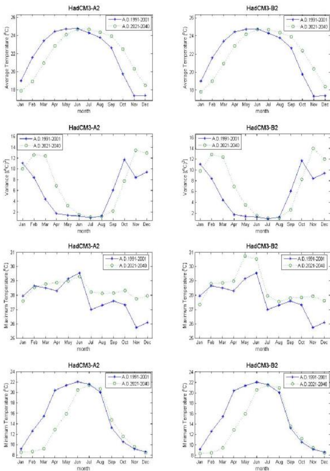
ภาพที่ ค.137 ค่าเฉลี่ย ค่าความแปรปรวน ค่าสูงสุด และค่าต่ำสุดของข้อมูลอุณหภูมิรายวันสังเคราะห์จาก ภาพฉาย HadCM3A2 และ HadCM3B2 สำหรับช่วงปี ค.ศ.1991-2001 และช่วงปี ค.ศ.2021-2040 (สถานี 431401)
