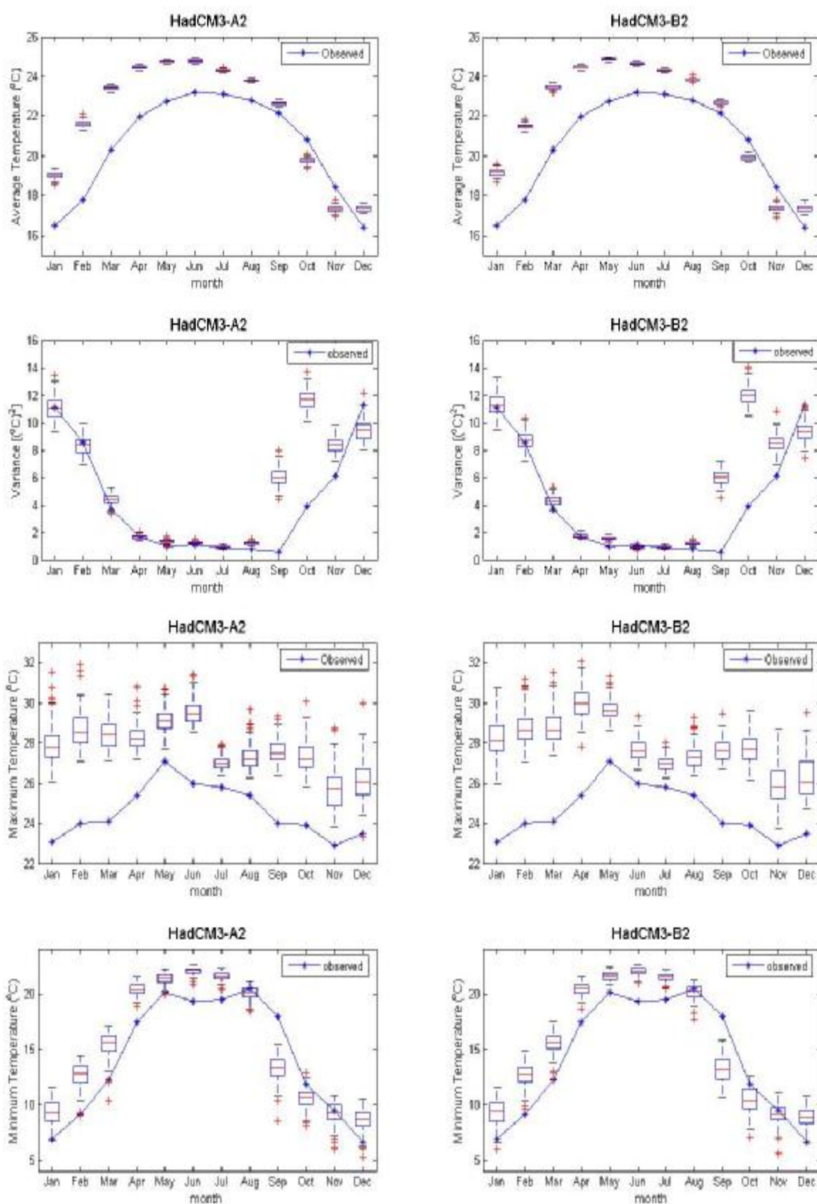
ภาพที่ ค.87 ค่าเฉลี่ย ค่าความแปรปรวน ค่าสูงสุด และค่าต่ำสุดของข้อมูลอุณหภูมิรายวันอดีต และของข้อมูลสังเคราะห์จากภาพฉาย HadCM3A2 และ HadCM3B2 สำหรับสถานี 431301 (ปี ค.ศ.1991-2001)
