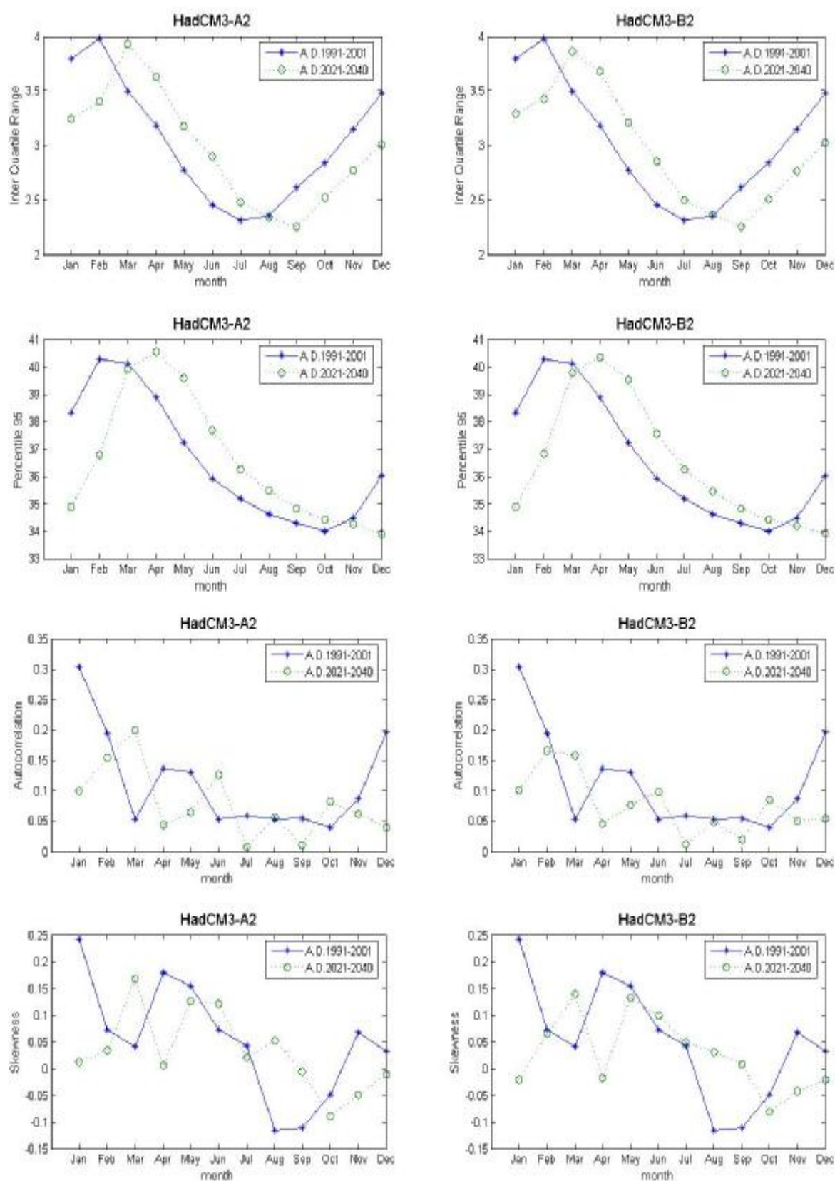
ภาพที่ ค.122 ค่าพิสัยระหว่างควอร์ไทล์ที่ 75 กับควอร์ไทล์ที่ 25 ค่าเปอร์เซ็นต์ไทล์ที่ 95 ค่าสัมประสิทธิ์สหสัมพันธ์ และค่าสัมประสิทธิ์ความเบ้ของข้อมูลอุณหภูมิสูงสุดรายวันสังเคราะห์จากภาพฉาย HadCM3A2 และ HadCM3B2 สำหรับช่วงปี ค.ศ.1991-2001 และช่วงปี ค.ศ.2021-2040 (สถานี 432201)
