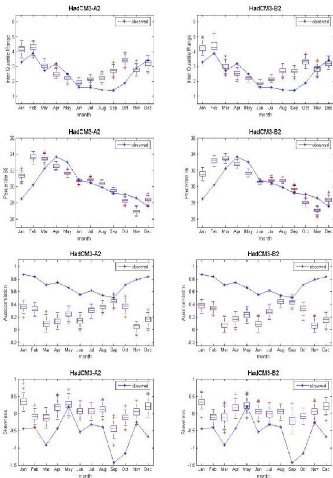
ภาพที่ ค.52 ค่าพิสัยระหว่างควอร์ไทล์ที่ 75 กับควอร์ไทล์ที่ 25 ค่าเปอร์เซ็นต์ไทล์ที่ 95 ค่าสัมประสิทธิ์สหสัมพันธ์ และ ค่าความเบ้ของข้อมูลอุณหภูมิเฉลี่ยรายวันอดีต และของข้อมูลสังเคราะห์จากภาพฉาย HadCM3A2 และ HadCM3B2 สำหรับสถานี 407501 (ปี ค.ศ.1991-2001)
