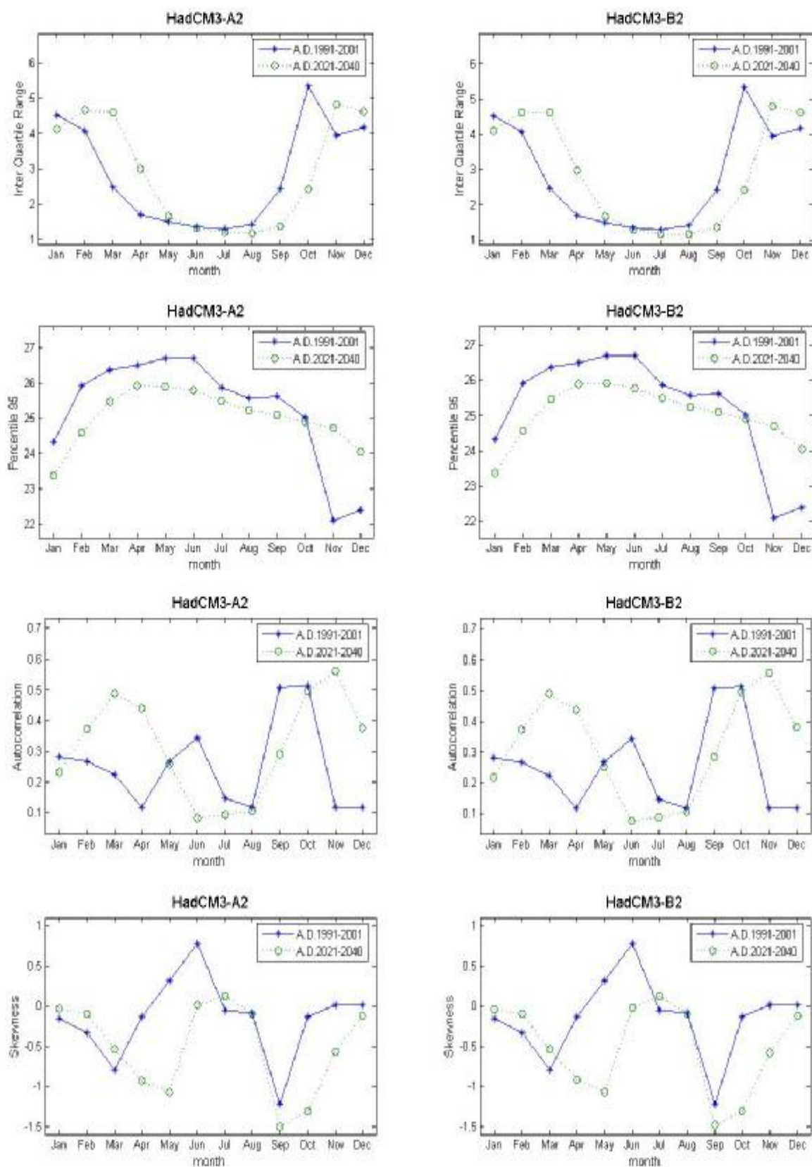
ภาพที่ ค.144 ค่าพิสัยระหว่างควอร์ไทล์ที่ 75 กับควอร์ไทล์ที่ 25 ค่าเปอร์เซ็นต์ไทล์ที่ 95 ค่าสัมประสิทธิ์สหสัมพันธ์ และค่าสัมประสิทธิ์ความเบ้ของข้อมูลอุณหภูมิต่ำสุดรายวันสังเคราะห์จากภาพฉาย HadCM3A2 และ HadCM3B2 สำหรับช่วงปี ค.ศ.1991-2001 และช่วงปี ค.ศ.2021-2040 (สถานี 436401)
