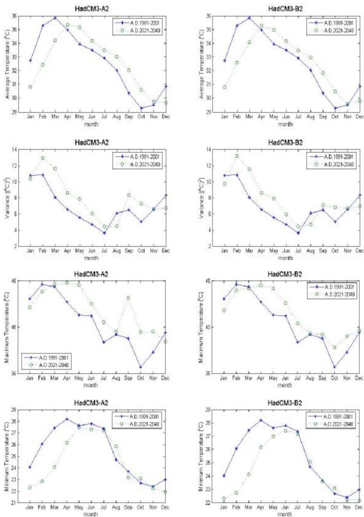
ภาพที่ ค.127 ค่าเฉลี่ย ค่าความแปรปรวน ค่าสูงสุด และค่าต่ำสุดของข้อมูลอุณหภูมิสูงสุดรายวันสังเคราะห์จาก ภาพฉาย HadCM3A2 และ HadCM3B2 สำหรับช่วงปี ค.ศ.1991-2001 และช่วงปี ค.ศ.2021-2040 (สถานี 436401)
