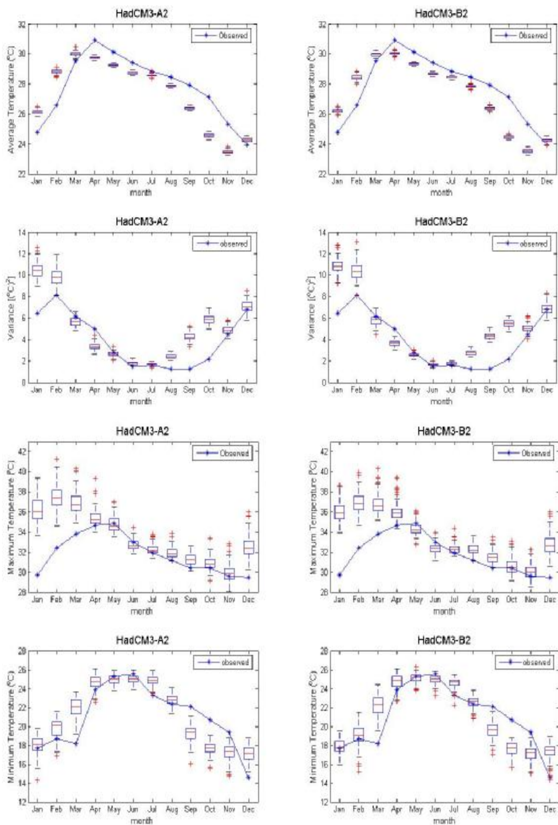
ภาพที่ ค.61 ค่าเฉลี่ย ค่าความแปรปรวน ค่าสูงสุด และค่าต่ำสุดของข้อมูลอุณหภูมิเฉลี่ยรายวันอดีต และของข้อมูลสังเคราะห์จากภาพฉาย HadCM3A2 และ HadCM3B2 สำหรับสถานี 432401 (ปี ค.ศ.1991-2001)
