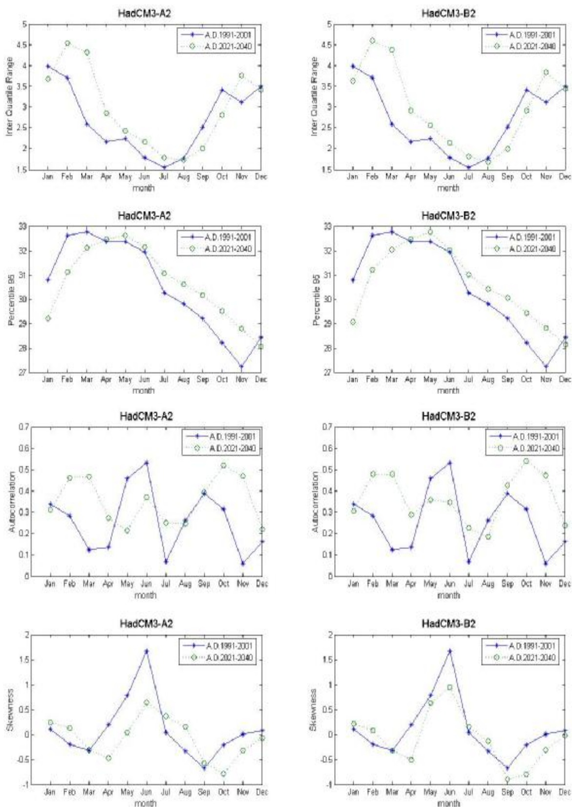
ภาพที่ ค.112 ค่าพิสัยระหว่างควอร์ไทล์ที่ 75 กับควอร์ไทล์ที่ 25 ค่าเปอร์เซ็นต์ไทล์ที่ 95 ค่าสัมประสิทธิ์สหสัมพันธ์ และค่าสัมประสิทธิ์ความเบ้ของข้อมูลอุณหภูมิเฉลี่ยรายวันสังเคราะห์จากภาพฉาย HadCM3A2 และ HadCM3B2 สำหรับช่วงปี ค.ศ.1991-2001 และช่วงปี ค.ศ.2021-2040 (สถานี 436401)
