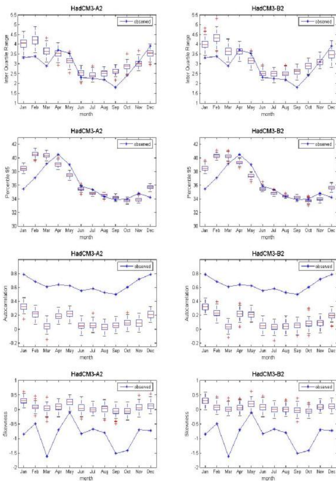
ภาพที่ ค.66 ค่าพิสัยระหว่างควอร์ไทล์ที่ 75 กับควอร์ไทล์ที่ 25 ค่าเปอร์เซ็นต์ไทล์ที่ 95 ค่าสัมประสิทธิ์สหสัมพันธ์ และค่าความเบ้ของข้อมูลอุณหภูมิสูงสุดรายวันอดีต และของข้อมูลสังเคราะห์จากภาพฉาย HadCM3A2 และ HadCM3B2 สำหรับสถานี 407501 (ปี ค.ศ.1991-2001)
