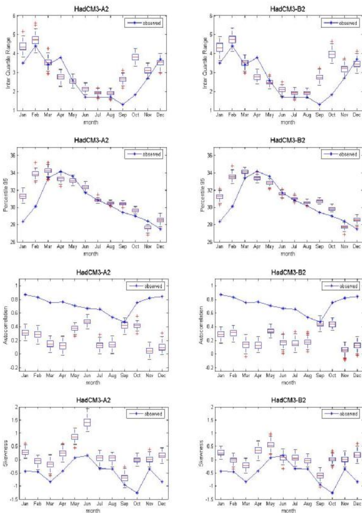
ภาพที่ ค.2 ค่าพิสัยระหว่างควอร์ไทล์ที่ 75 กับควอร์ไทล์ที่ 25 ค่าเปอร์เซ็นต์ไทล์ที่ 95 ค่าสัมประสิทธิ์สหสัมพันธ์ และค่าความเบ้ของข้อมูลอุณหภูมิเฉลี่ยรายวันอดีต และของข้อมูลสังเคราะห์จากภาพฉาย HadCM3A2 และ HadCM3B2 สำหรับสถานี 381201 (ปี ค.ศ.1991-2001)
