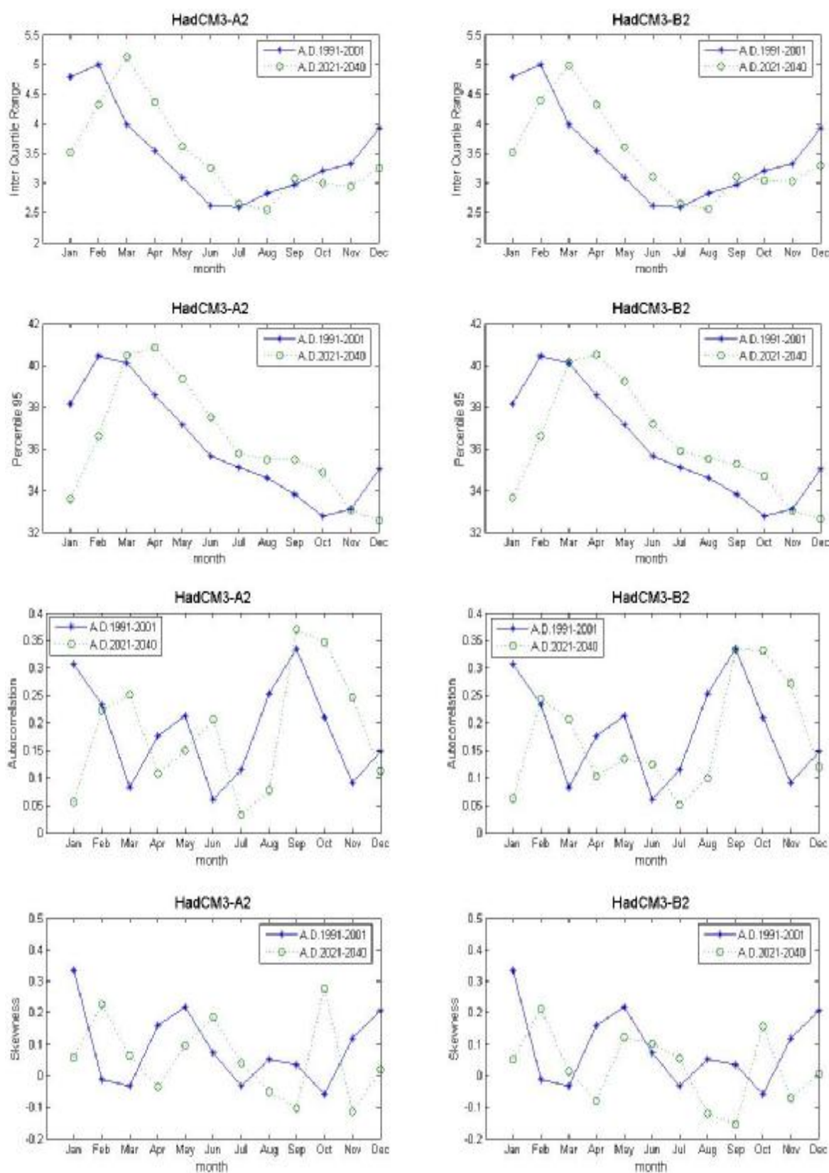
ภาพที่ ค.40 ค่าพิสัยระหว่างควอร์ไทล์ที่ 75 กับควอร์ไทล์ที่ 25 ค่าเปอร์เซ็นต์ไทล์ที่ 95 ค่าสัมประสิทธิ์สหสัมพันธ์ และ ค่าความเบ้ของข้อมูลอุณหภูมิสูงสุดรายวันสังเคราะห์จากภาพฉาย HadCM3A2 และ HadCM3B2 สำหรับช่วงปี ค.ศ.1991-2001 และช่วงปี ค.ศ.2021-2040 (สถานี 405201)
