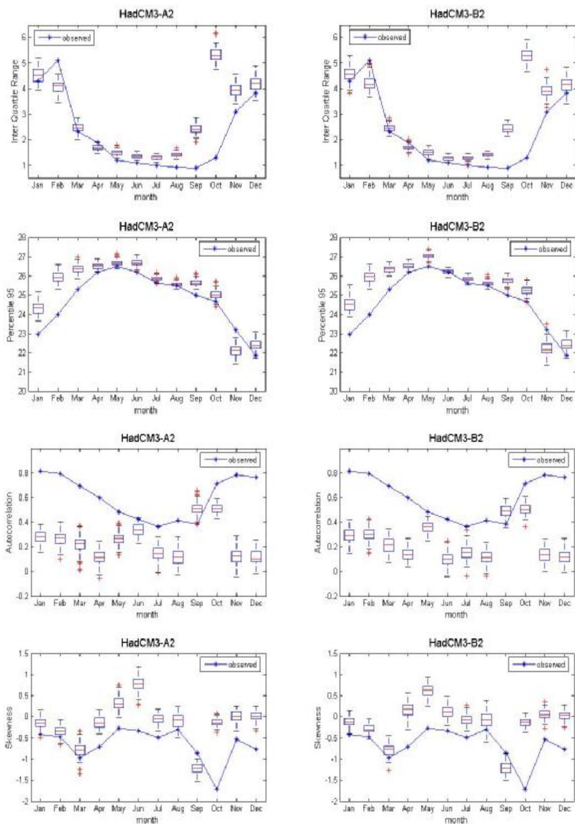
ภาพที่ ค.90 ค่าพิสัยระหว่างควอร์ไทล์ที่ 75 กับควอร์ไทล์ที่ 25 ค่าเปอร์เซ็นต์ไทล์ที่ 95 ค่าสัมประสิทธิ์สหสัมพันธ์ และค่าความเบ้ของข้อมูลอุณหภูมิต่ำสุดรายวันอดีต และของข้อมูลสังเคราะห์จากภาพฉาย HadCM3A2 และ HadCM3B2 สำหรับสถานี 431401 (ปี ค.ศ.1991-2001)
