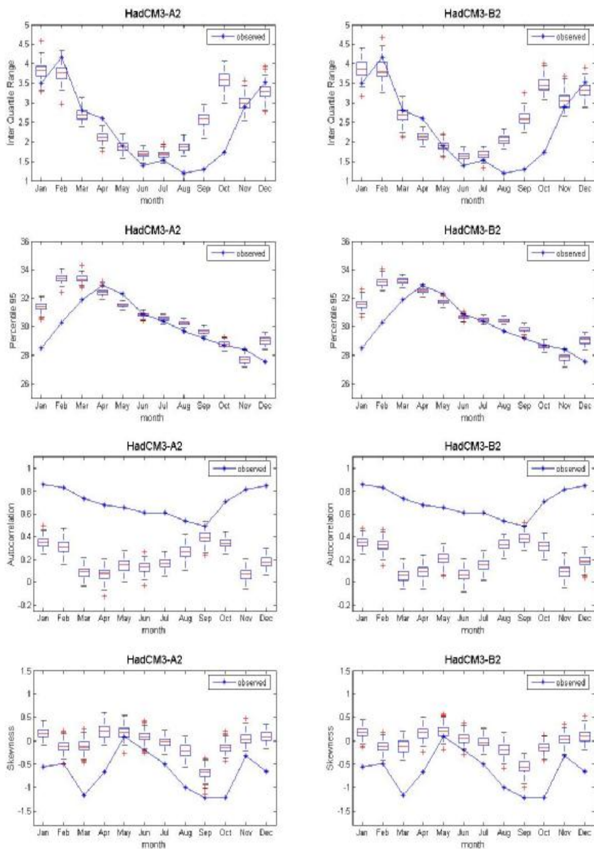
ภาพที่ ค.58 ค่าพิสัยระหว่างควอร์ไทล์ที่ 75 กับควอร์ไทล์ที่ 25 ค่าเปอร์เซ็นต์ไทล์ที่ 95 ค่าสัมประสิทธิ์สหสัมพันธ์ และค่าความเบ้ของข้อมูลอุณหภูมิเฉลี่ยรายวันอดีต และของข้อมูลสังเคราะห์จากภาพฉาย HadCM3A2 และ HadCM3B2 สำหรับสถานี 432201 (ปี ค.ศ.1991-2001)
