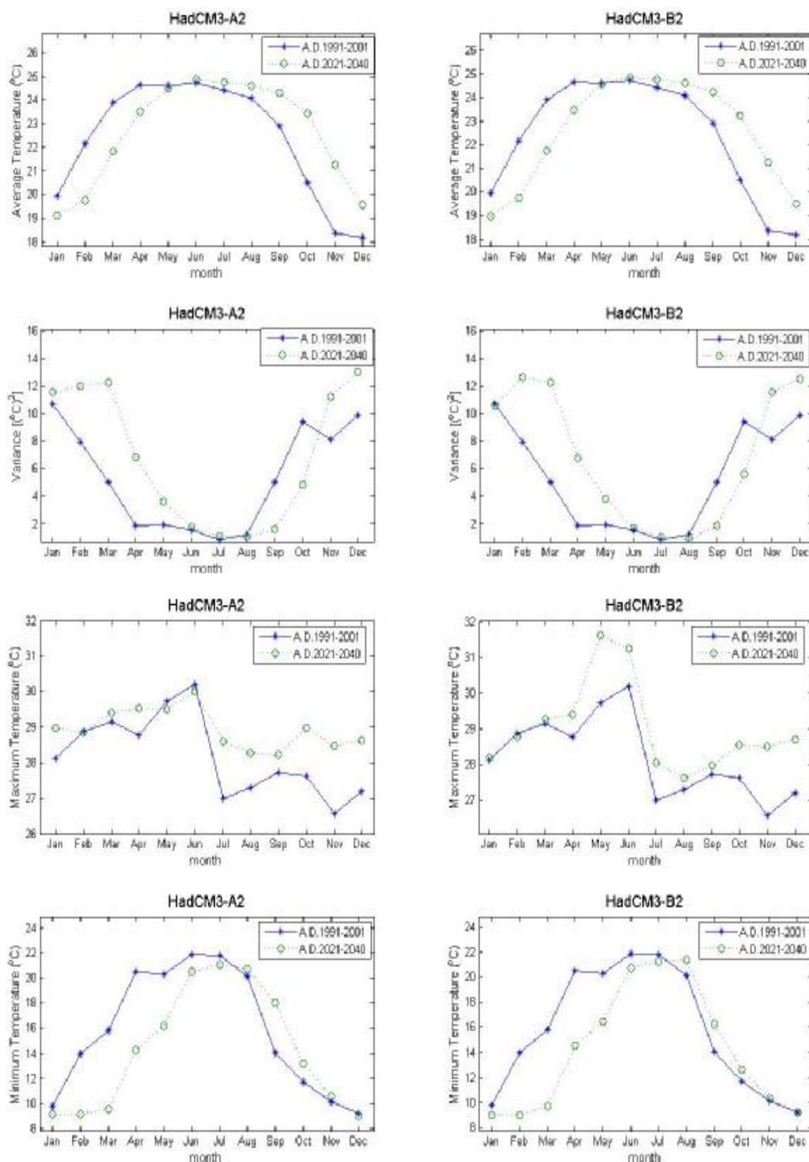
ภาพที่ ค.133 ค่าเฉลี่ย ค่าความแปรปรวน ค่าสูงสุด และค่าต่ำสุดของข้อมูลอุณหภูมิรายวันสังเคราะห์จาก ภาพฉาย HadCM3A2 และ HadCM3B2 สำหรับช่วงปี ค.ศ.1991-2001 และช่วงปี ค.ศ.2021-2040 (สถานี 431201)
