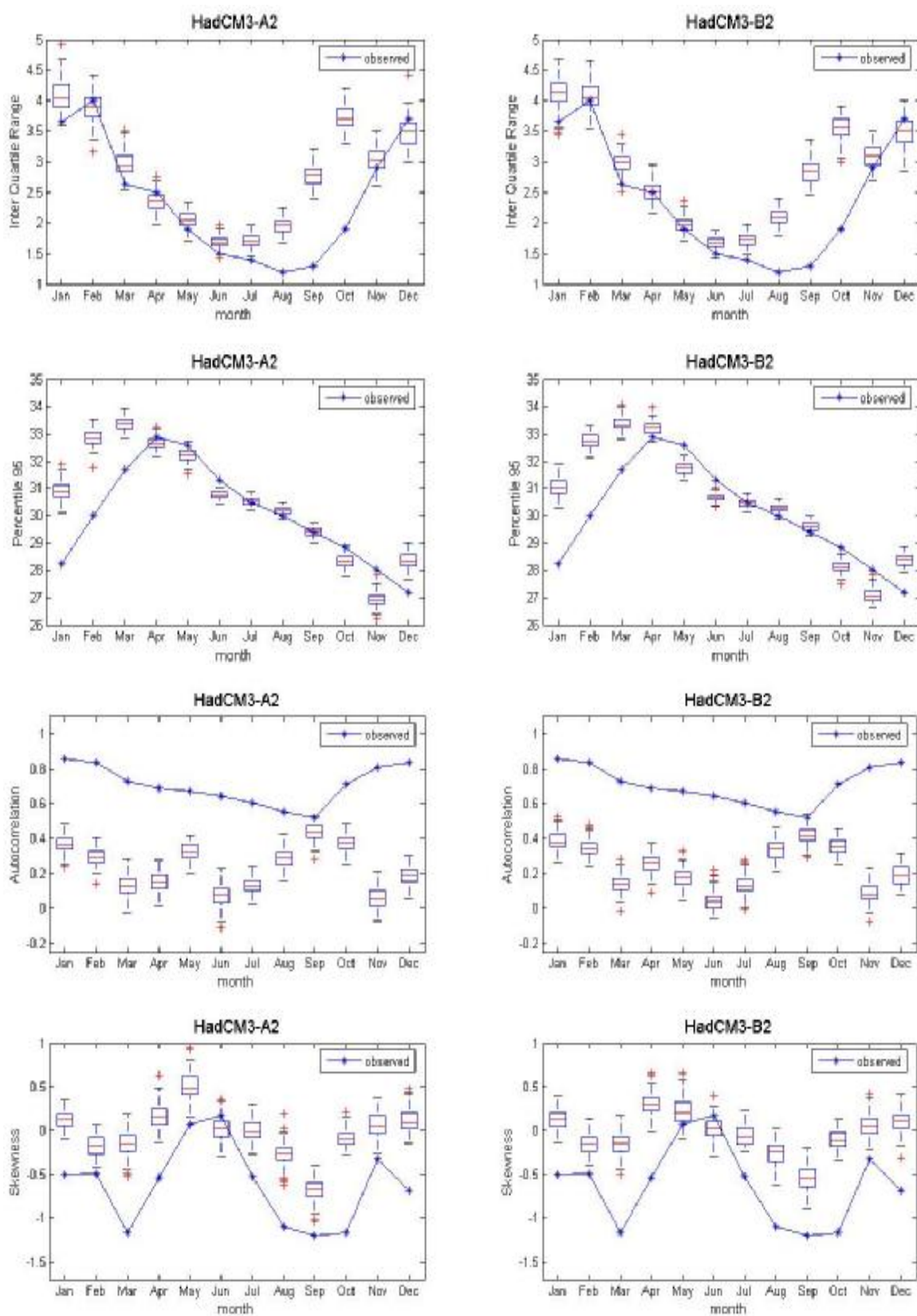
ภาพที่ ค.60 ค่าพิสัยระหว่างควอร์ไทล์ที่ 75 กับควอร์ไทล์ที่ 25 ค่าเปอร์เซ็นต์ไทล์ที่ 95 ค่าสัมประสิทธิ์สหสัมพันธ์ และค่าความเบ้ของข้อมูลอุณหภูมิเฉลี่ยรายวันอดีต และของข้อมูลสังเคราะห์จากภาพฉาย HadCM3A2 และ HadCM3B2 สำหรับสถานี 432301 (ปี ค.ศ.1991-2001)
