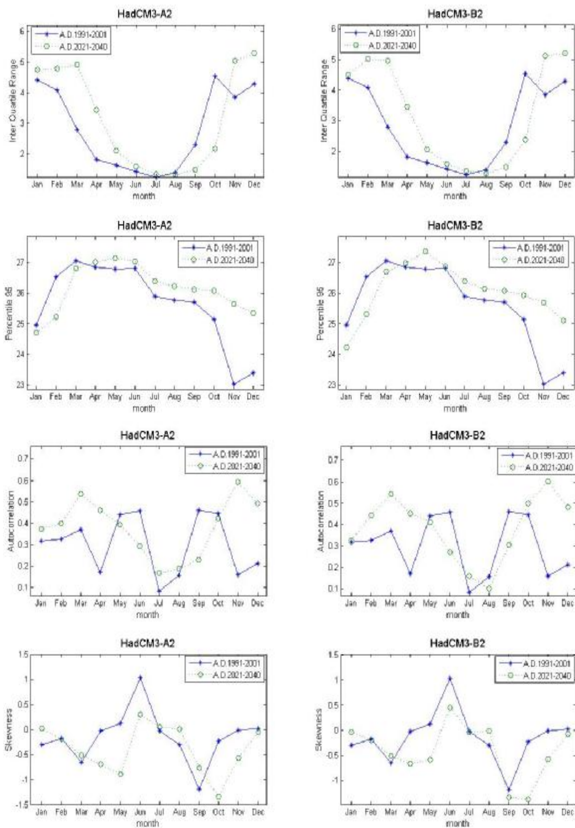
ภาพที่ ค.134 ค่าพิสัยระหว่างควอร์ไทล์ที่ 75 กับควอร์ไทล์ที่ 25 ค่าเปอร์เซ็นต์ไทล์ที่ 95 ค่าสัมประสิทธิ์สหสัมพันธ์ และค่าสัมประสิทธิ์ความเบ้ของข้อมูลอุณหภูมิต่ำสุดรายวันสังเคราะห์จากภาพฉาย HadCM3A2 และ HadCM3B2 สำหรับช่วงปี ค.ศ.1991-2001 และช่วงปี ค.ศ.2021-2040 (สถานี 431201)
