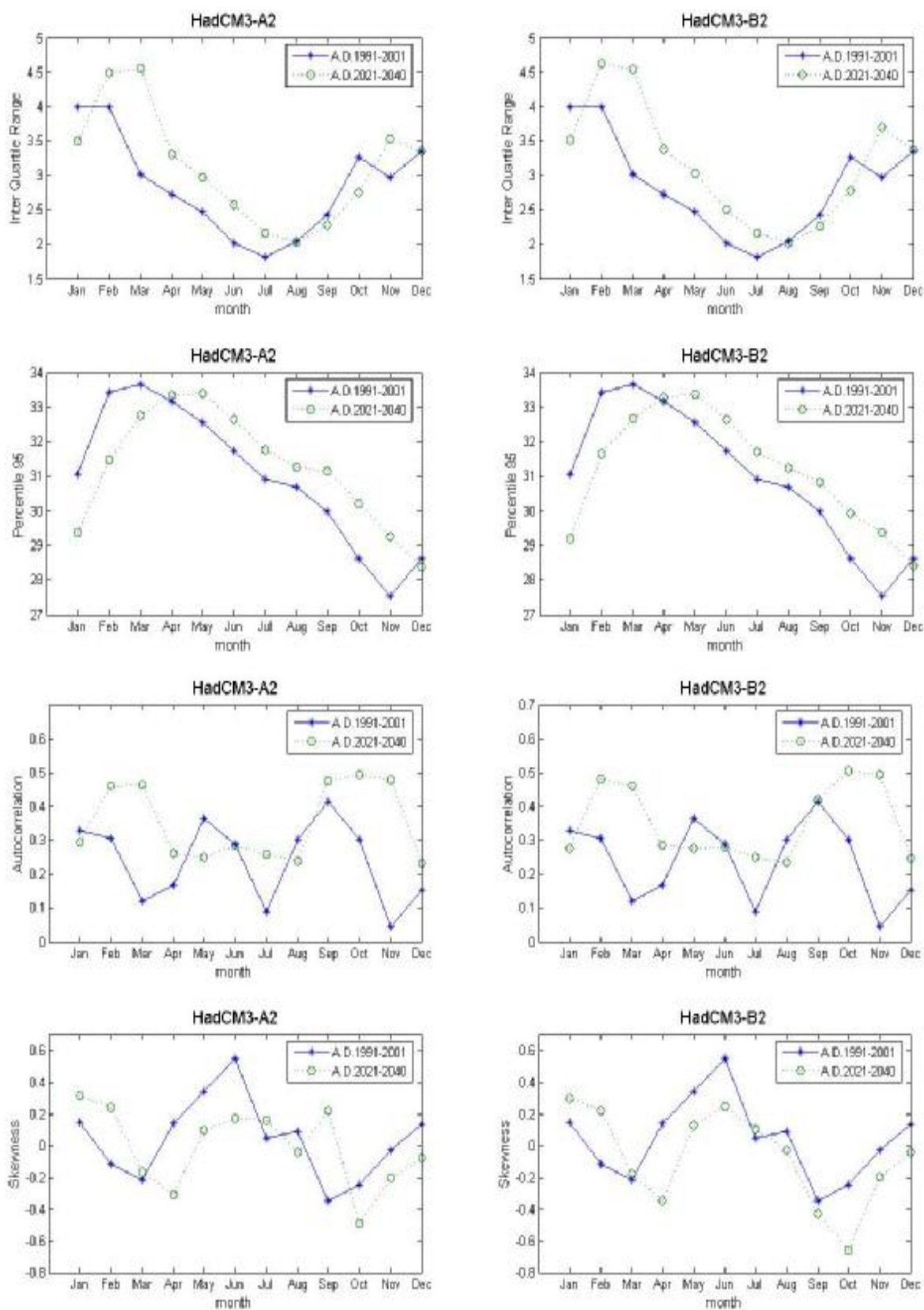
ภาพที่ ค.30 ค่าพิสัยระหว่างควอร์ไทล์ที่ 75 กับควอร์ไทล์ที่ 25 ค่าเปอร์เซ็นต์ไทล์ที่ 95 ค่าสัมประสิทธิ์สหสัมพันธ์ และ ค่าความเบ้ของข้อมูลอุณหภูมิเฉลี่ยรายวันสังเคราะห์จากภาพฉาย HadCM3A2 และ HadCM3B2 สำหรับช่วงปี ค.ศ.1991-2001 และช่วงปี ค.ศ.2021-2040 (สถานี 403201)
