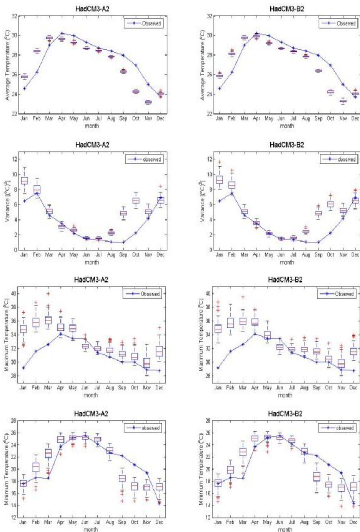
ภาพที่ ค.59 ค่าเฉลี่ย ค่าความแปรปรวน ค่าสูงสุด และค่าต่ำสุดของข้อมูลอุณหภูมิเฉลี่ยรายวันอดีต และของข้อมูลสังเคราะห์จากภาพฉาย HadCM3A2 และ HadCM3B2 สำหรับสถานี 432301 (ปี ค.ศ.1991-2001)
