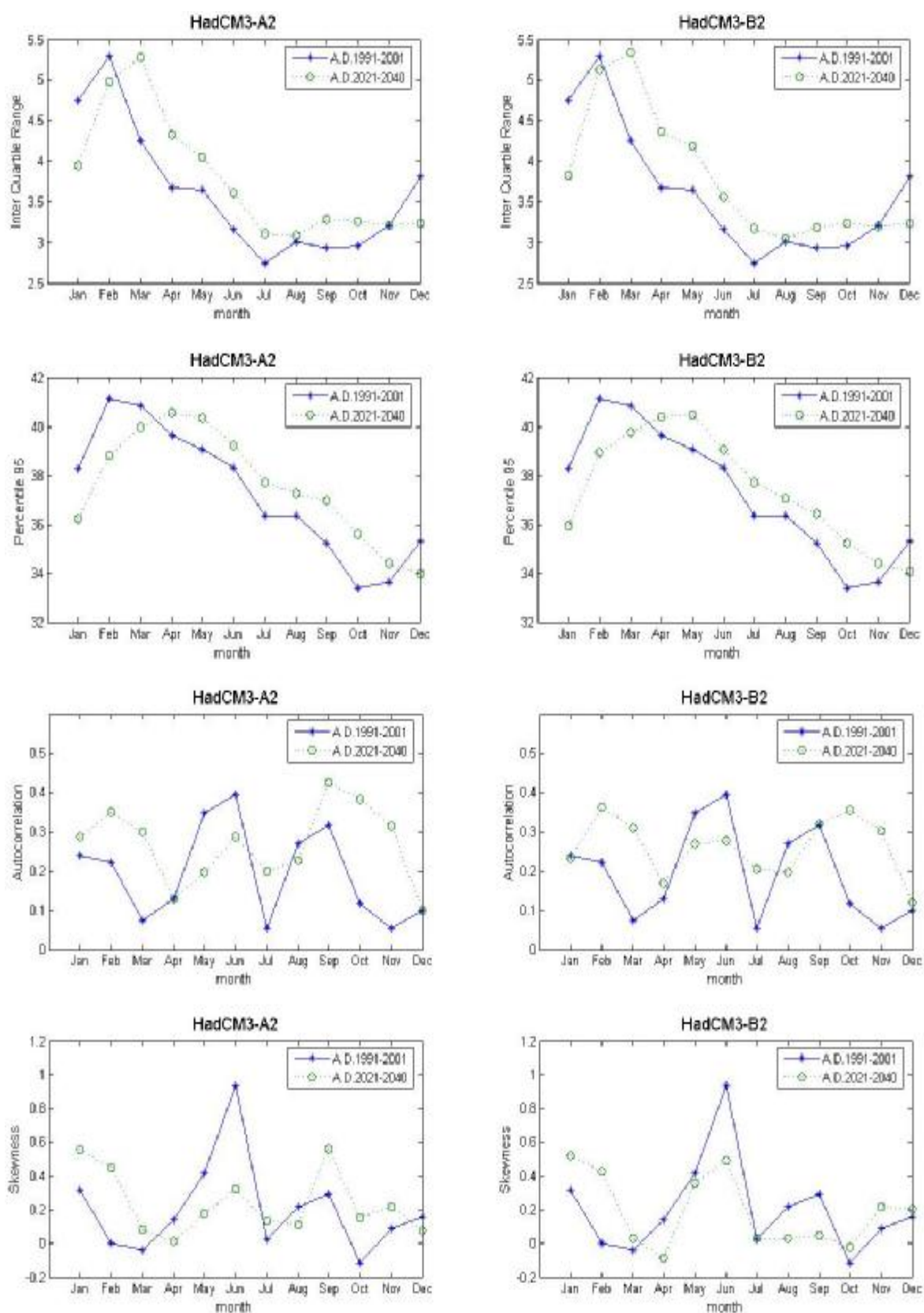
ภาพที่ ค.36 ค่าพิสัยระหว่างควอร์ไทล์ที่ 75 กับควอร์ไทล์ที่ 25 ค่าเปอร์เซ็นต์ไทล์ที่ 95 ค่าสัมประสิทธิ์สหสัมพันธ์ และ ค่าความเบ้ของข้อมูลอุณหภูมิสูงสุดรายวันสังเคราะห์จากภาพฉาย HadCM3A2 และ HadCM3B2 สำหรับช่วงปี ค.ศ.1991-2001 และช่วงปี ค.ศ.2021-2040 (สถานี 387401)
