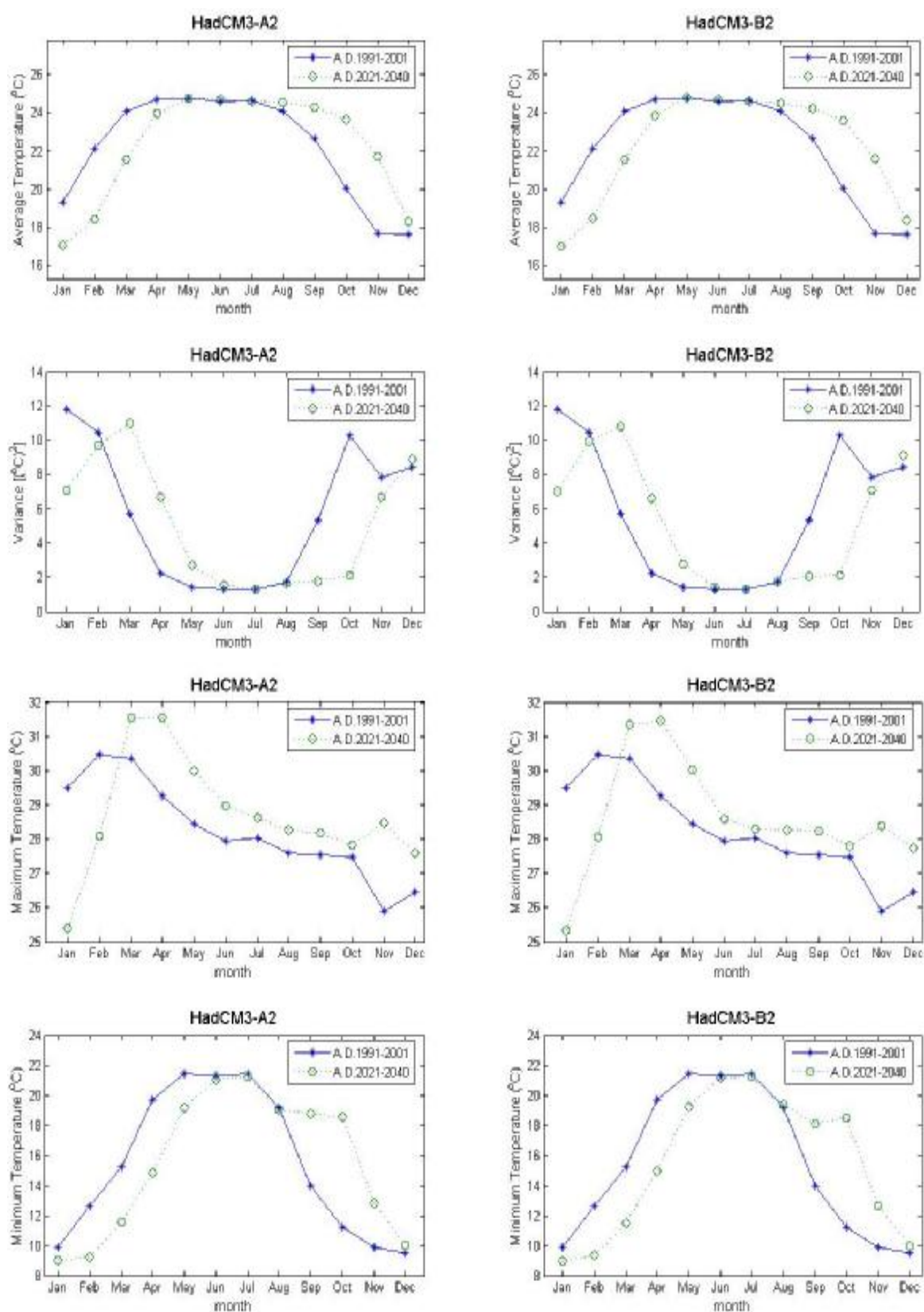
ภาพที่ ค.141 ค่าเฉลี่ย ค่าความแปรปรวน ค่าสูงสุด และค่าต่ำสุดของข้อมูลอุณหภูมิรายวันสังเคราะห์จาก ภาพฉาย HadCM3A2 และ HadCM3B2 สำหรับช่วงปี ค.ศ.1991-2001 และช่วงปี ค.ศ.2021-2040 (สถานี 432401)
