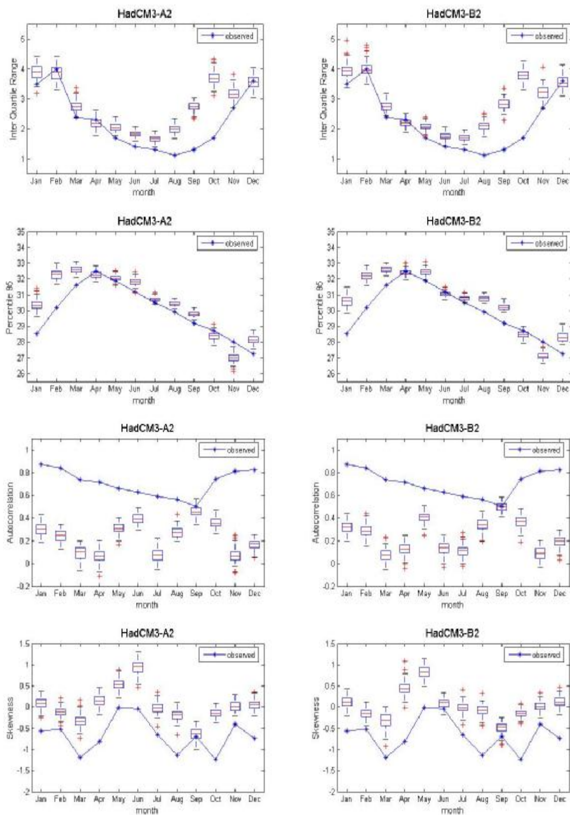
ภาพที่ ค.56 ค่าพิสัยระหว่างควอร์ไทล์ที่ 75 กับควอร์ไทล์ที่ 25 ค่าเปอร์เซ็นต์ไทล์ที่ 95 ค่าสัมประสิทธิ์สหสัมพันธ์ และ ค่าความเบ้ของข้อมูลอุณหภูมิเฉลี่ยรายวันอดีต และของข้อมูลสังเคราะห์จากภาพฉาย HadCM3A2 และ HadCM3B2 สำหรับสถานี 431401 (ปี ค.ศ.1991-2001)
