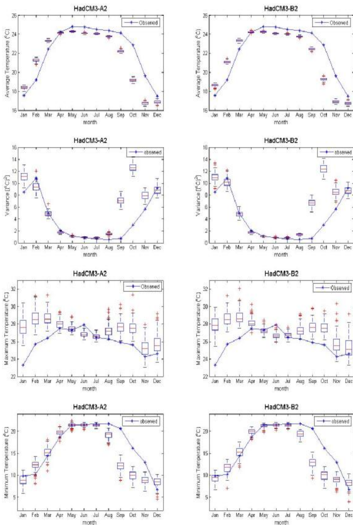
ภาพที่ ค.91 ค่าเฉลี่ย ค่าความแปรปรวน ค่าสูงสุด และค่าต่ำสุดของข้อมูลอุณหภูมิต่ำสุดรายวันอดีต และของข้อมูลสังเคราะห์จากภาพฉาย HadCM3A2 และ HadCM3B2 สำหรับสถานี 432301 (ปี ค.ศ.1991-2001)
