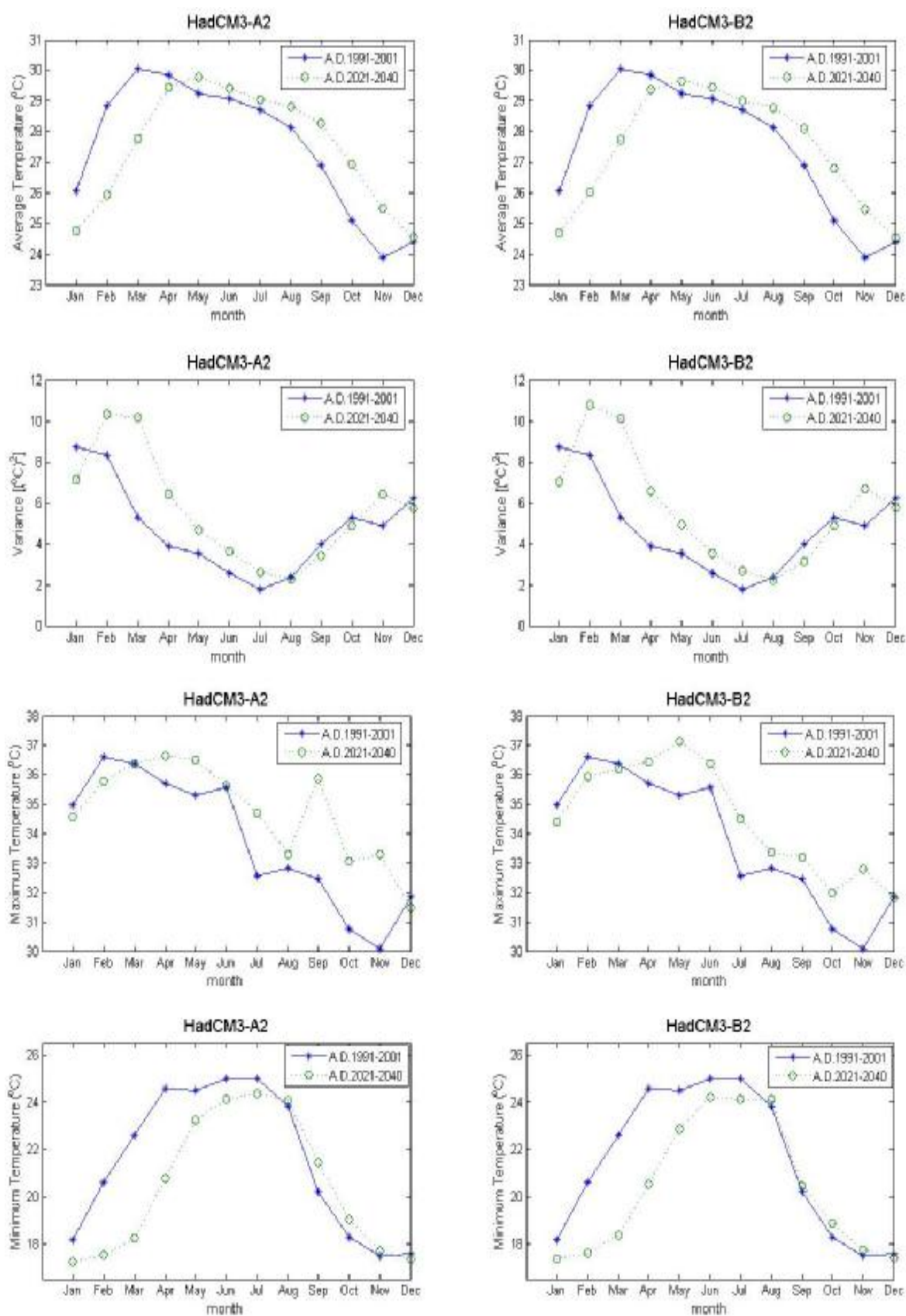
ภาพที่ ค.29 ค่าเฉลี่ย ค่าความแปรปรวน ค่าสูงสุด และค่าต่ำสุดของข้อมูลอุณหภูมิเฉลี่ยรายวันสังเคราะห์จากภาพฉาย HadCM3A2 และ HadCM3B2 สำหรับช่วงปี ค.ศ.1991-2001 และช่วงปี ค.ศ.2021-2040 (สถานี 403201)
