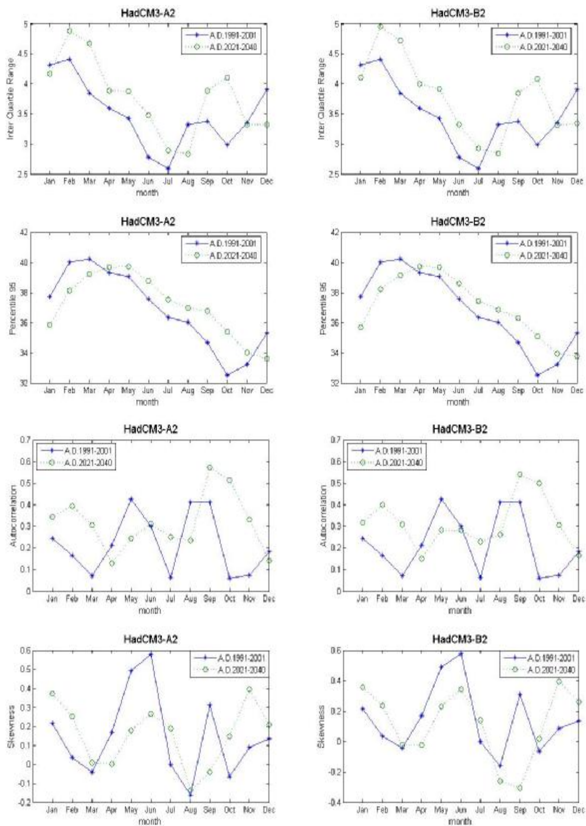
ภาพที่ ค.120 ค่าพิสัยระหว่างควอร์ไทล์ที่ 75 กับควอร์ไทล์ที่ 25 ค่าเปอร์เซ็นต์ไทล์ที่ 95 ค่าสัมประสิทธิ์สหสัมพันธ์ และค่าสัมประสิทธิ์ความเบ้ของข้อมูลอุณหภูมิสูงสุดรายวันสังเคราะห์จากภาพฉาย HadCM3A2 และ HadCM3B2 สำหรับช่วงปี ค.ศ.1991-2001 และช่วงปี ค.ศ.2021-2040 (สถานี 431401)
