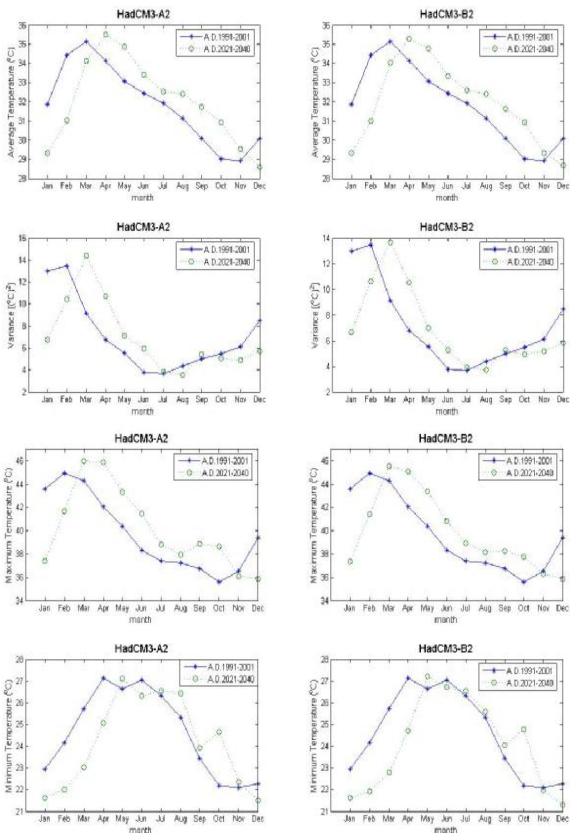
ภาพที่ ค.39 ค่าเฉลี่ย ค่าความแปรปรวน ค่าสูงสุด และค่าต่ำสุดของข้อมูลอุณหภูมิสูงสุดรายวันสังเคราะห์จากภาพฉาย HadCM3A2 และ HadCM3B2 สำหรับช่วงปี ค.ศ.1991-2001 และช่วงปี ค.ศ.2021-2040 (สถานี 405201)
