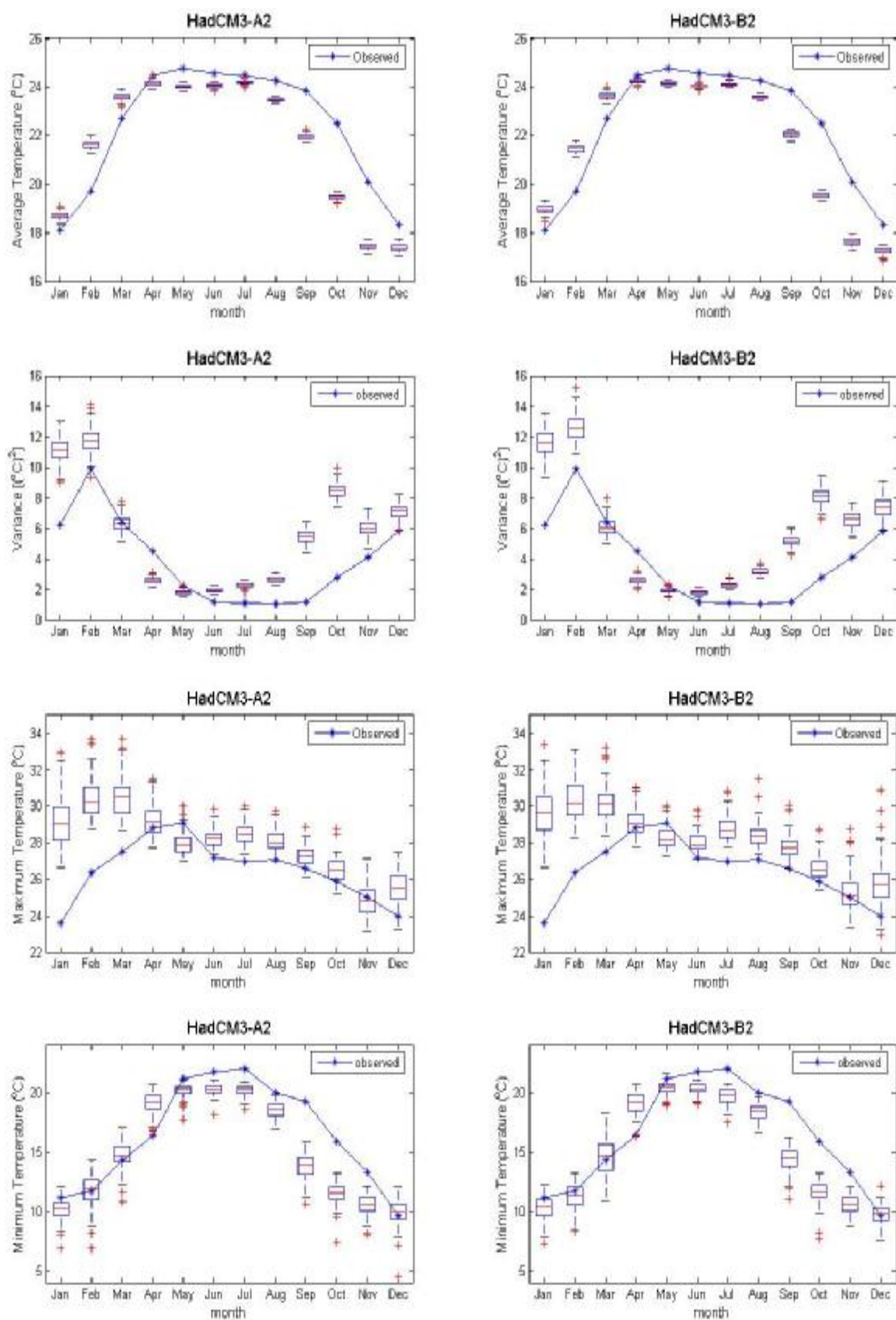
ภาพที่ ค.83 ค่าเฉลี่ย ค่าความแปรปรวน ค่าสูงสุด และค่าต่ำสุดของข้อมูลอุณหภูมิรายวันอดีต และของข้อมูลสังเคราะห์จากภาพฉาย HadCM3A2 และ HadCM3B2 สำหรับสถานี 407501 (ปี ค.ศ.1991-2001)
