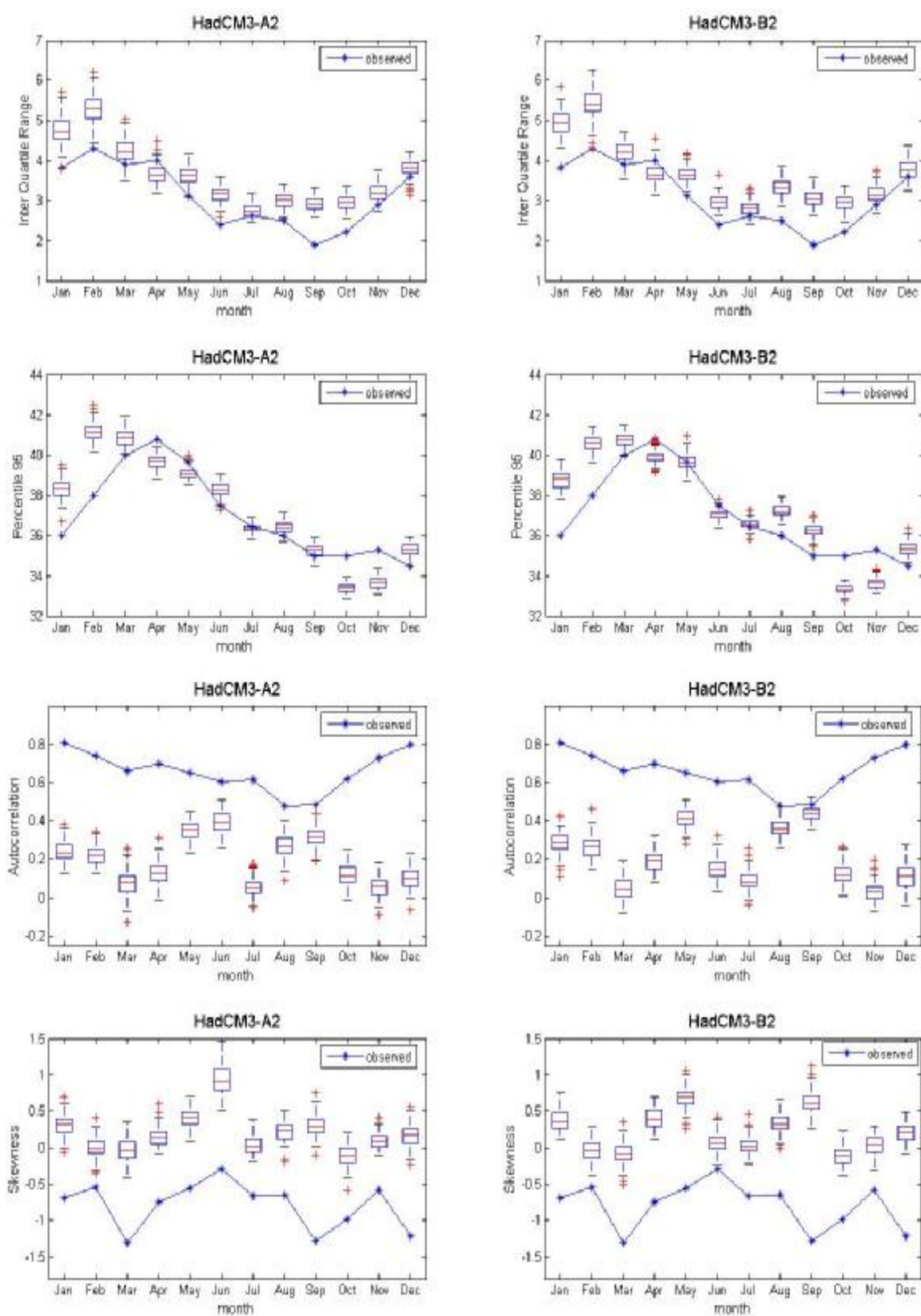
ภาพที่ ค.12 ค่าพิสัยระหว่างควอร์ไทล์ที่ 75 กับควอร์ไทล์ที่ 25 ค่าเปอร์เซ็นต์ไทล์ที่ 95 ค่าสัมประสิทธิ์สหสัมพันธ์ และ ค่าความเบ้ของข้อมูลอุณหภูมิสูงสุดรายวันอดีต และของข้อมูลสังเคราะห์จากภาพฉาย HadCM3A2 และ HadCM3B2 สำหรับสถานี 387401 (ปี ค.ศ.1991-2001)
