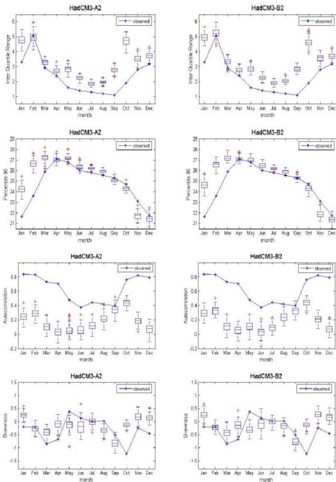
ภาพที่ ค.82 ค่าพิสัยระหว่างควอร์ไทล์ที่ 75 กับควอร์ไทล์ที่ 25 ค่าเปอร์เซ็นต์ไทล์ที่ 95 ค่าสัมประสิทธิ์สหสัมพันธ์ และ ค่าความเบ้ของข้อมูลอุณหภูมิต่ำสุดรายวันอดีต และของข้อมูลสังเคราะห์จากภาพฉาย HadCM3A2 และ HadCM3B2 สำหรับสถานี 407301 (ปี ค.ศ.1991-2001)
