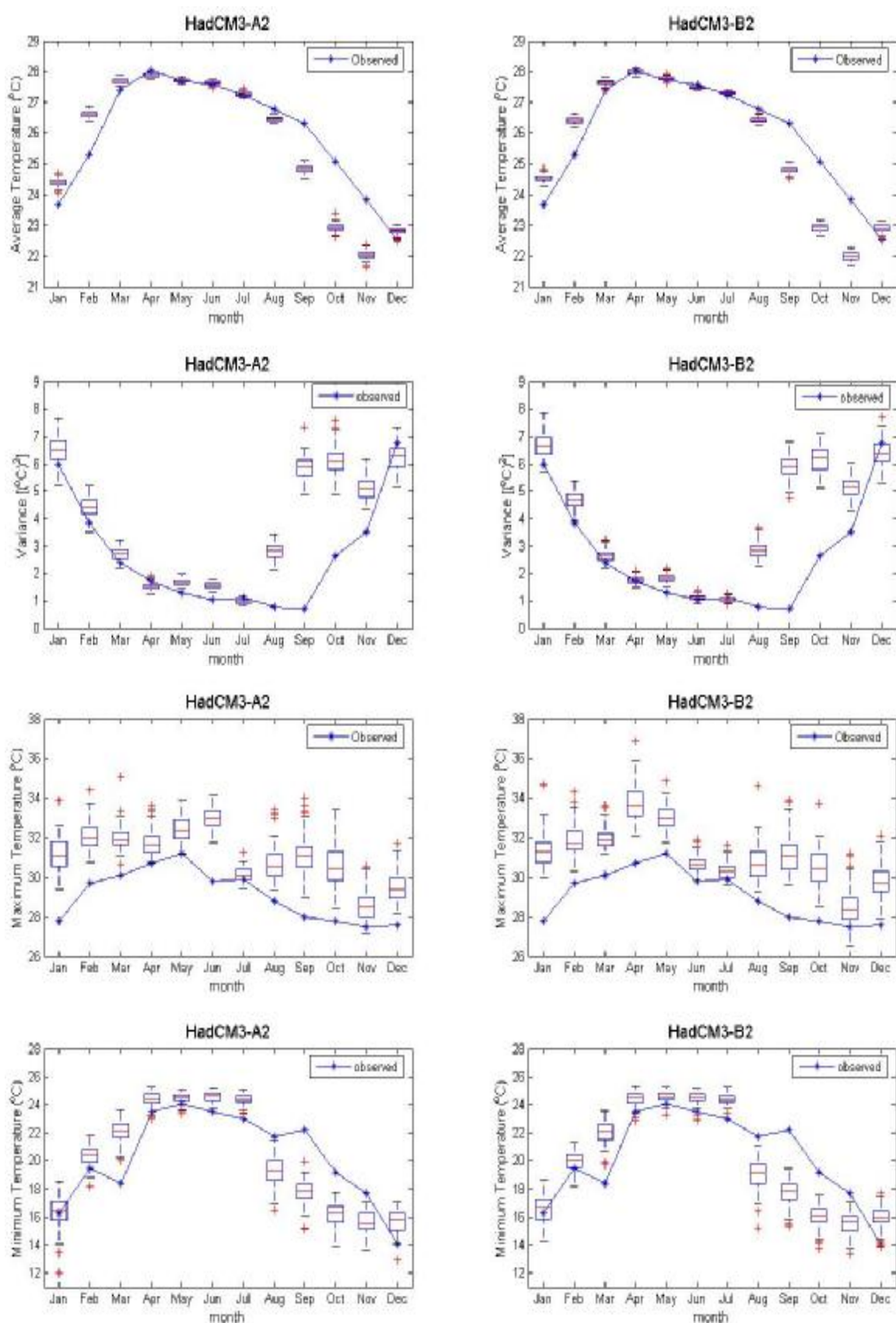
ภาพที่ ค.53 ค่าเฉลี่ย ค่าความแปรปรวน ค่าสูงสุด และค่าต่ำสุดของข้อมูลอุณหภูมิเฉลี่ยรายวันอดีต และของข้อมูลสังเคราะห์จากภาพฉาย HadCM3A2 และ HadCM3B2 สำหรับสถานี 431301 (ปี ค.ศ.1991-2001)
