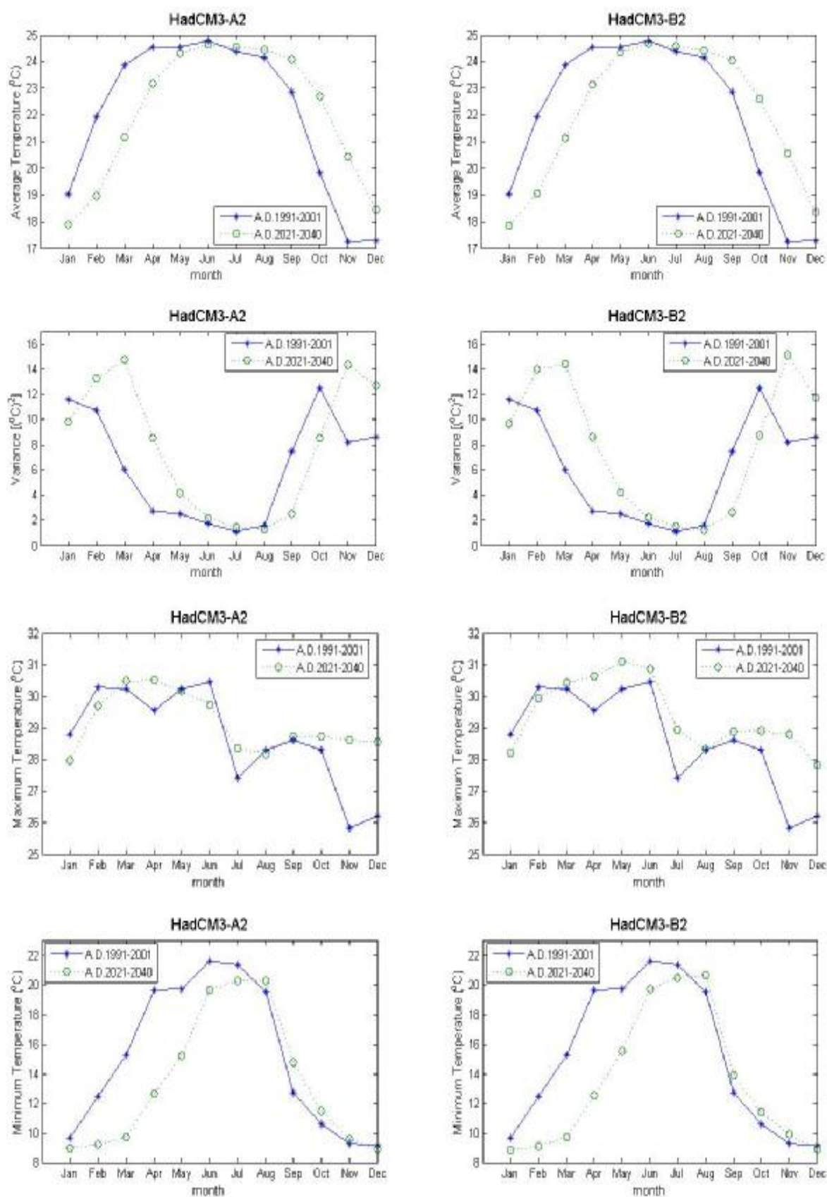
ภาพที่ ค.41 ค่าเฉลี่ย ค่าความแปรปรวน ค่าสูงสุด และค่าต่ำสุดของข้อมูลอุณหภูมิรายวันสังเคราะห์จากภาพฉาย HadCM3A2 และ HadCM3B2 สำหรับช่วงปี ค.ศ.1991-2001 และช่วงปี ค.ศ.2021-2040 (สถานี 381201)
