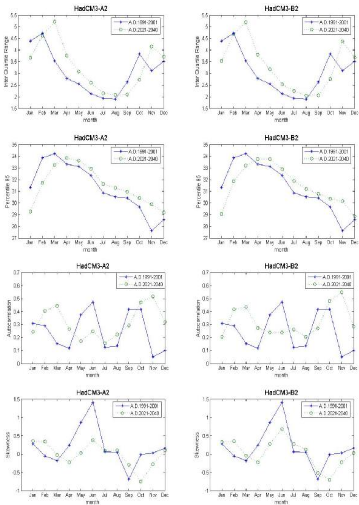
ภาพที่ ค.26 ค่าพิสัยระหว่างควอร์ไทล์ที่ 75 กับควอร์ไทล์ที่ 25 ค่าเปอร์เซ็นต์ไทล์ที่ 95 ค่าสัมประสิทธิ์สหสัมพันธ์ และ ค่าความเบ้ของข้อมูลอุณหภูมิเฉลี่ยรายวันสังเคราะห์จากภาพฉาย HadCM3A2 และ HadCM3B2 สำหรับช่วงปี ค.ศ.1991-2001 และช่วงปี ค.ศ.2021-2040 (สถานี 381201)
