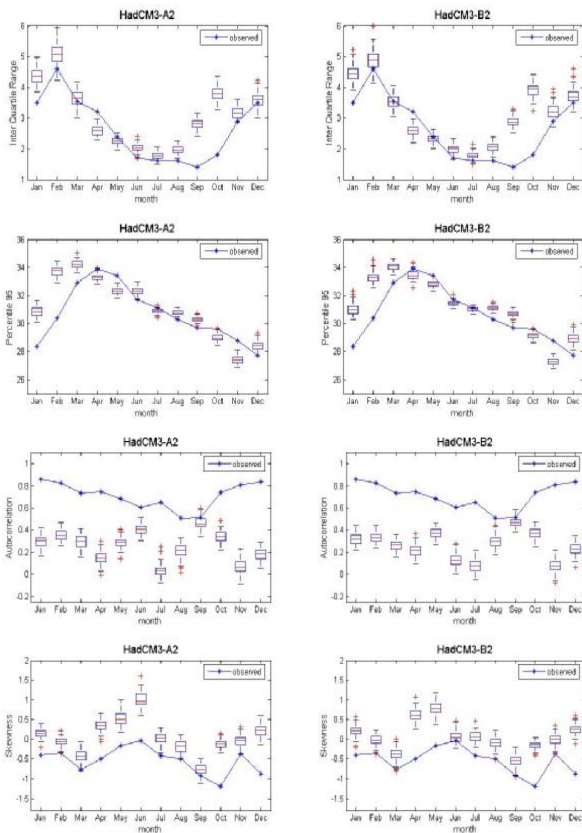
ภาพที่ ค.4 ค่าพิสัยระหว่างควอร์ไทล์ที่ 75 กับควอร์ไทล์ที่ 25 ค่าเปอร์เซ็นต์ไทล์ที่ 95 ค่าสัมประสิทธิ์สหสัมพันธ์ และ ค่าความเบ้ของข้อมูลอุณหภูมิเฉลี่ยรายวันอดีต และของข้อมูลสังเคราะห์จากภาพฉาย HadCM3A2 และ HadCM3B2 สำหรับสถานี 387401 (ปี ค.ศ.1991-2001)
