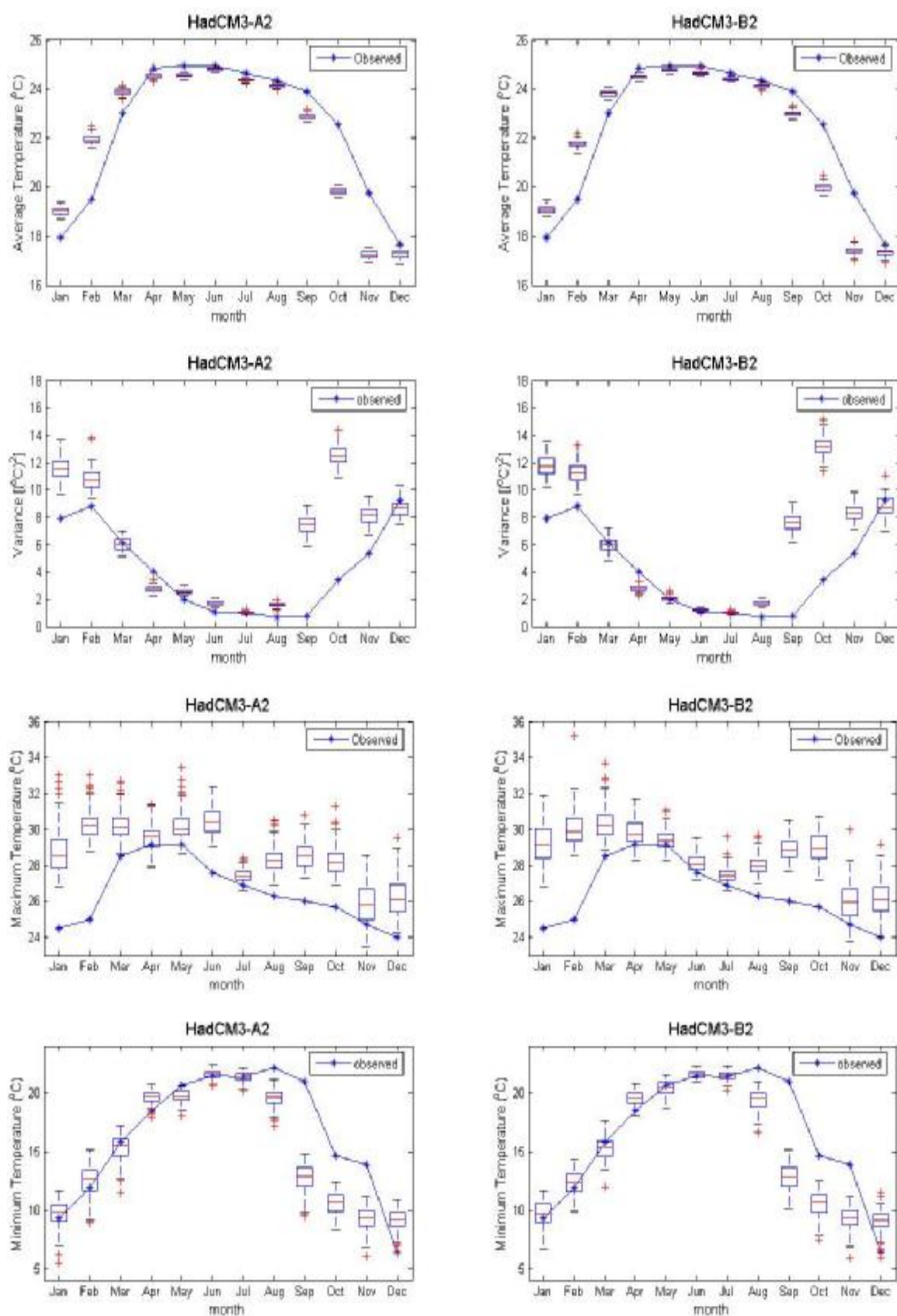
ภาพที่ ค.17 ค่าเฉลี่ย ค่าความแปรปรวน ค่าสูงสุด และค่าต่ำสุดของข้อมูลอุณหภูมิต่ำสุดรายวันอดีต และของข้อมูลสังเคราะห์จากภาพฉาย HadCM3A2 และ HadCM3B2 สำหรับสถานี 381201 (ปี ค.ศ.1991-2001)
