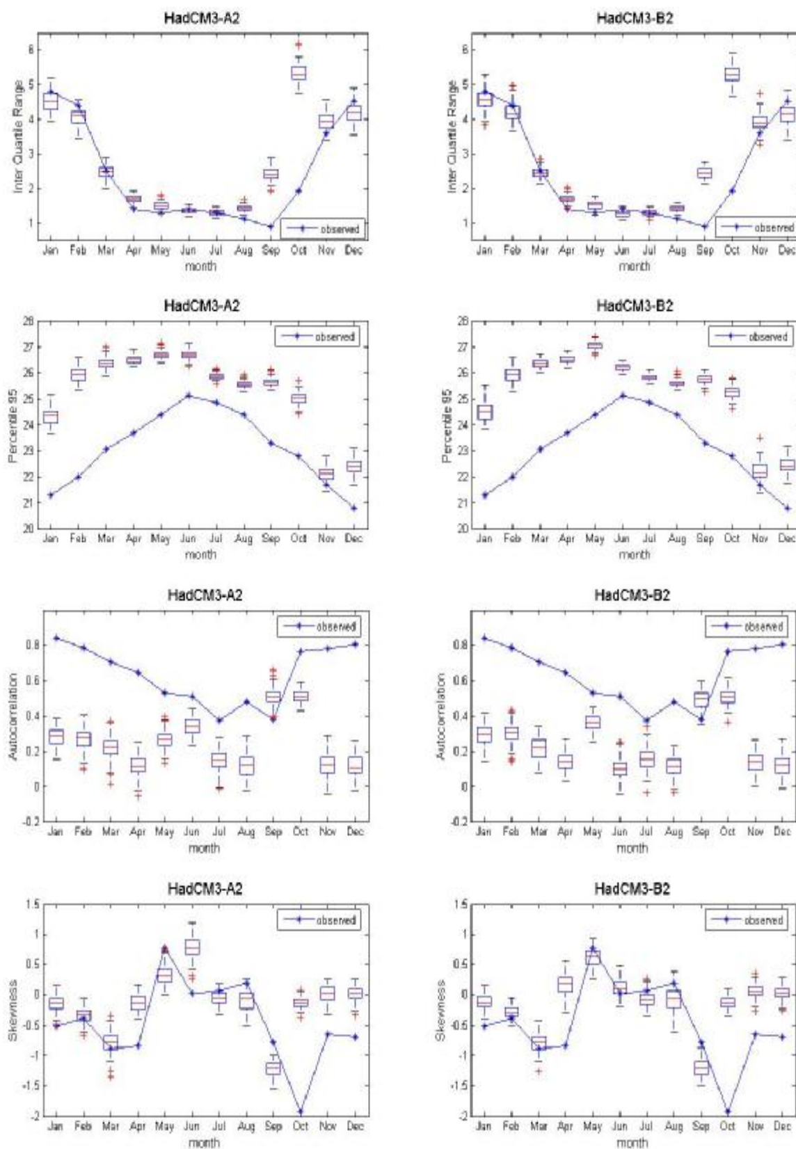
ภาพที่ ค.88 ค่าพิสัยระหว่างควอร์ไทล์ที่ 75 กับควอร์ไทล์ที่ 25 ค่าเปอร์เซ็นต์ไทล์ที่ 95 ค่าสัมประสิทธิ์สหสัมพันธ์ และ ค่าความเบ้ของข้อมูลอุณหภูมิต่ำสุดรายวันอดีต และของข้อมูลสังเคราะห์จากภาพฉาย HadCM3A2 และ HadCM3B2 สำหรับสถานี 431301 (ปี ค.ศ.1991-2001)
