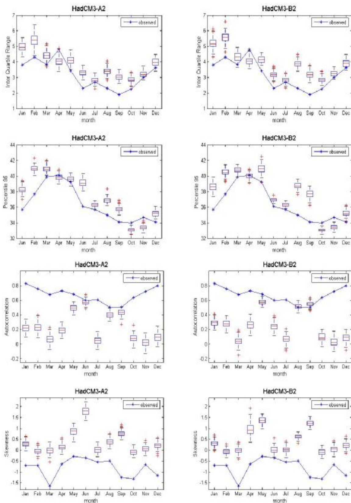
ภาพที่ ค.10 ค่าพิสัยระหว่างควอร์ไทล์ที่ 75 กับควอร์ไทล์ที่ 25 ค่าเปอร์เซ็นต์ไทล์ที่ 95 ค่าสัมประสิทธิ์สหสัมพันธ์ และ ค่าความเบ้ของข้อมูลอุณหภูมิสูงสุดรายวันอดีต และของข้อมูลสังเคราะห์จากภาพฉาย HadCM3A2 และ HadCM3B2 สำหรับสถานี 381301 (ปี ค.ศ.1991-2001)
