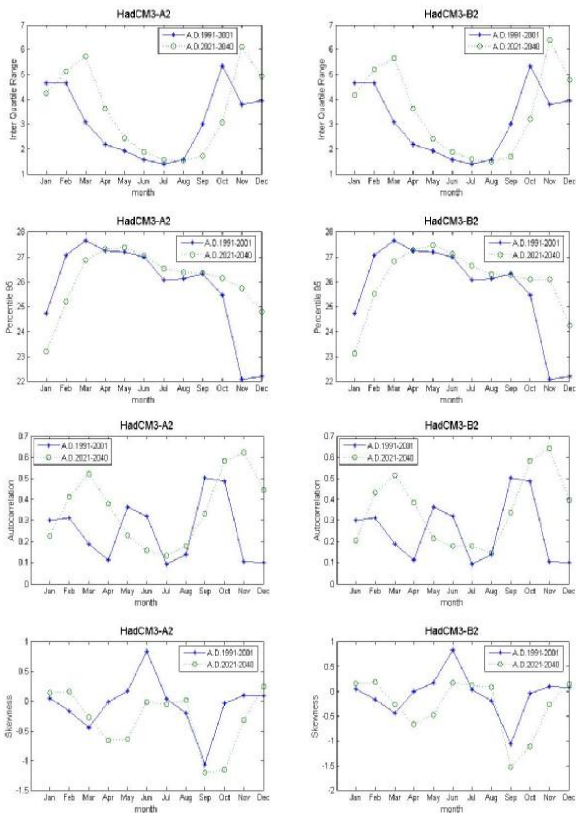
ภาพที่ ค.42 ค่าพิสัยระหว่างควอร์ไทล์ที่ 75 กับควอร์ไทล์ที่ 25 ค่าเปอร์เซ็นต์ไทล์ที่ 95 ค่าสัมประสิทธิ์สหสัมพันธ์ และ ค่าความเบ้ของข้อมูลอุณหภูมิต่ำสุดรายวันสังเคราะห์จากภาพฉาย HadCM3A2 และ HadCM3B2 สำหรับช่วงปี ค.ศ.1991-2001 และช่วงปี ค.ศ.2021-2040 (สถานี 381201)
