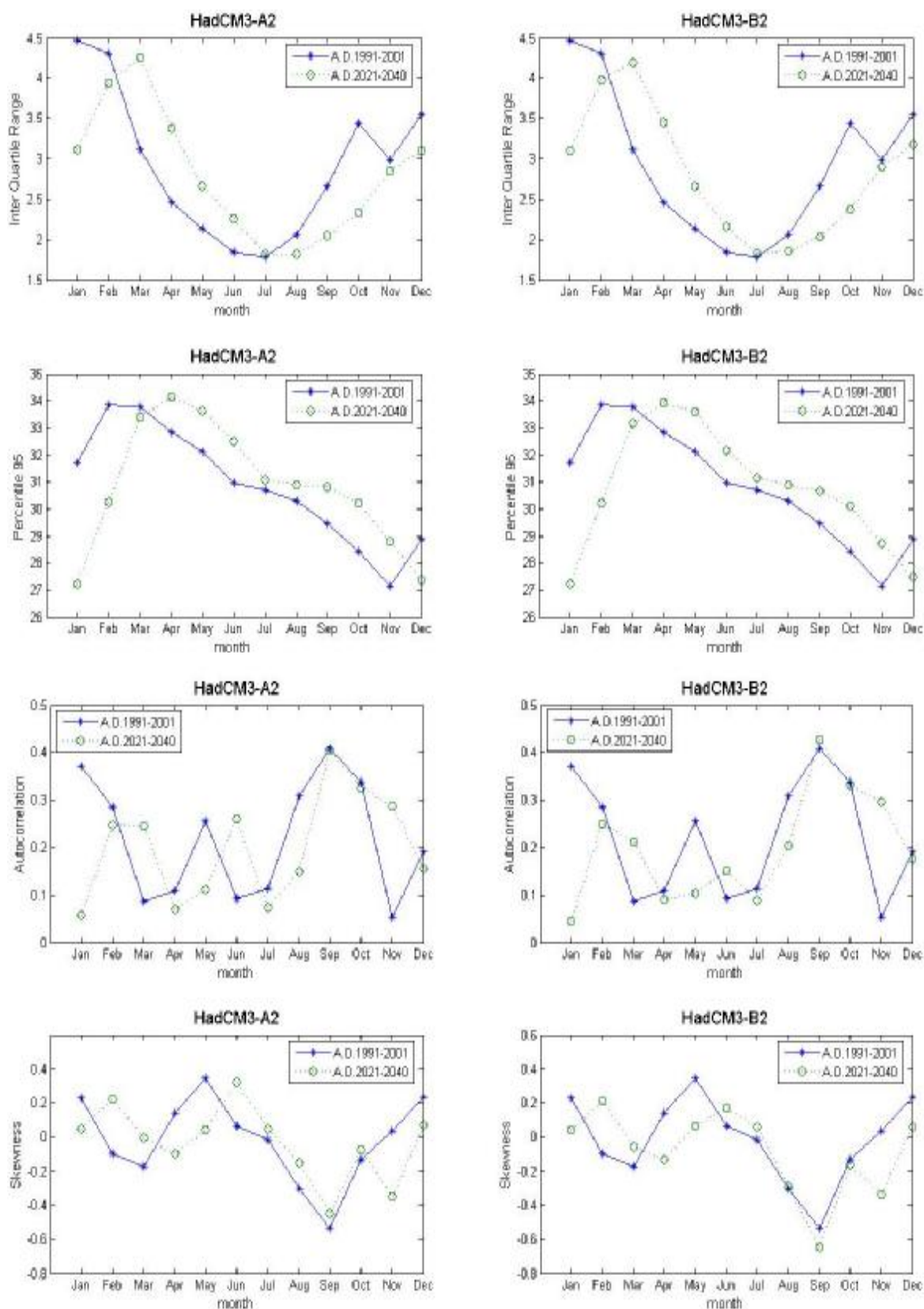
ภาพที่ ค.110 ค่าพิสัยระหว่างควอร์ไทล์ที่ 75 กับควอร์ไทล์ที่ 25 ค่าเปอร์เซ็นต์ไทล์ที่ 95 ค่าสัมประสิทธิ์สหสัมพันธ์ และค่าสัมประสิทธิ์ความเบ้ของข้อมูลอุณหภูมิเฉลี่ยรายวันสังเคราะห์จากภาพฉาย HadCM3A2 และ HadCM3B2 สำหรับช่วงปี ค.ศ.1991-2001 และช่วงปี ค.ศ.2021-2040 (สถานี 432401)
