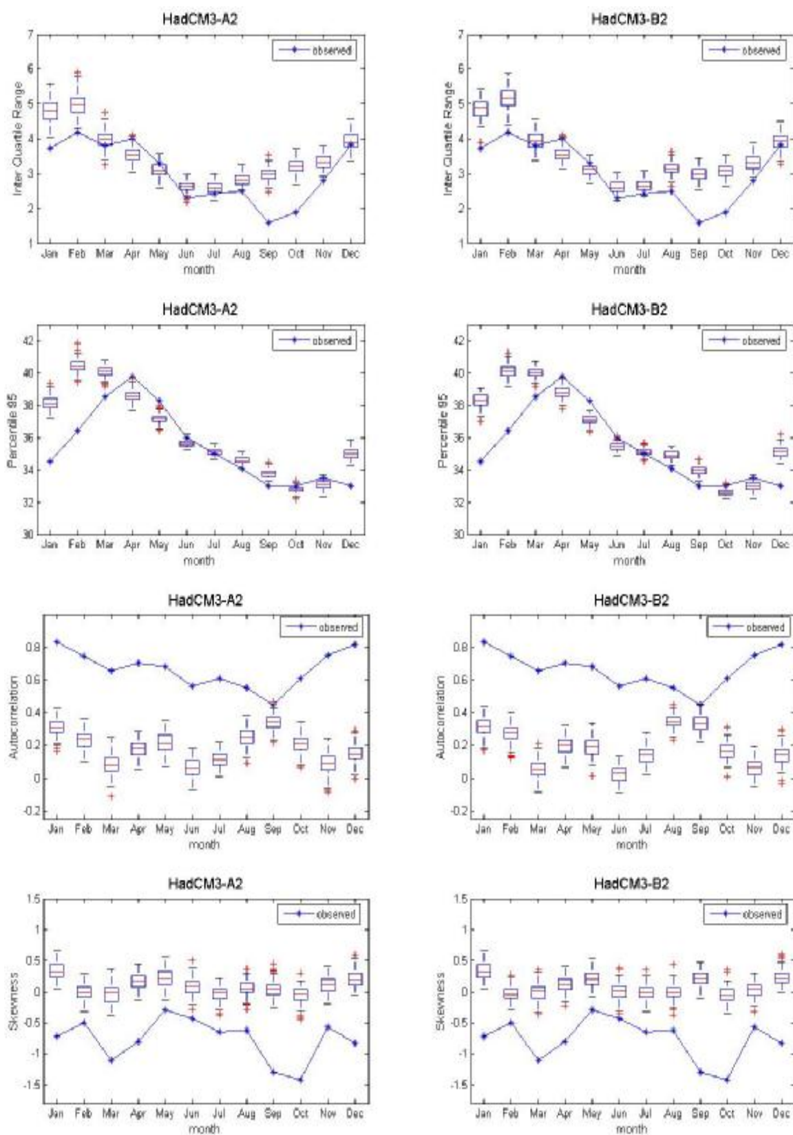
ภาพที่ ค.16 ค่าพิสัยระหว่างควอร์ไทล์ที่ 75 กับควอร์ไทล์ที่ 25 ค่าเปอร์เซ็นต์ไทล์ที่ 95 ค่าสัมประสิทธิ์สหสัมพันธ์ และค่าความเบ้ของข้อมูลอุณหภูมิสูงสุดรายวันอดีต และของข้อมูลสังเคราะห์จากภาพฉาย HadCM3A2 และ HadCM3B2 สำหรับสถานี 405201(ปี ค.ศ.1991-2001)
