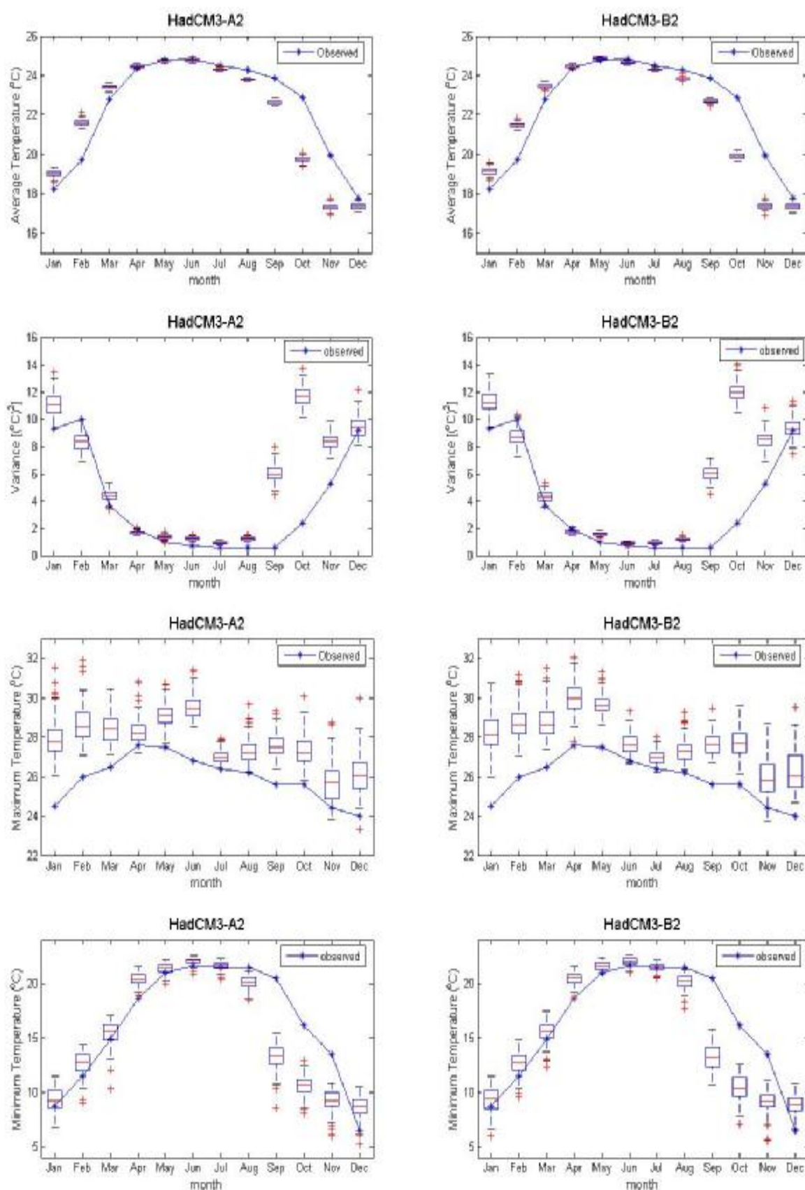
ภาพที่ ค.89 ค่าเฉลี่ย ค่าความแปรปรวน ค่าสูงสุด และค่าต่ำสุดของข้อมูลอุณหภูมิรายวันอดีต และของข้อมูลสังเคราะห์จากภาพฉาย HadCM3A2 และ HadCM3B2 สำหรับสถานี 431401 (ปี ค.ศ.1991-2001)
