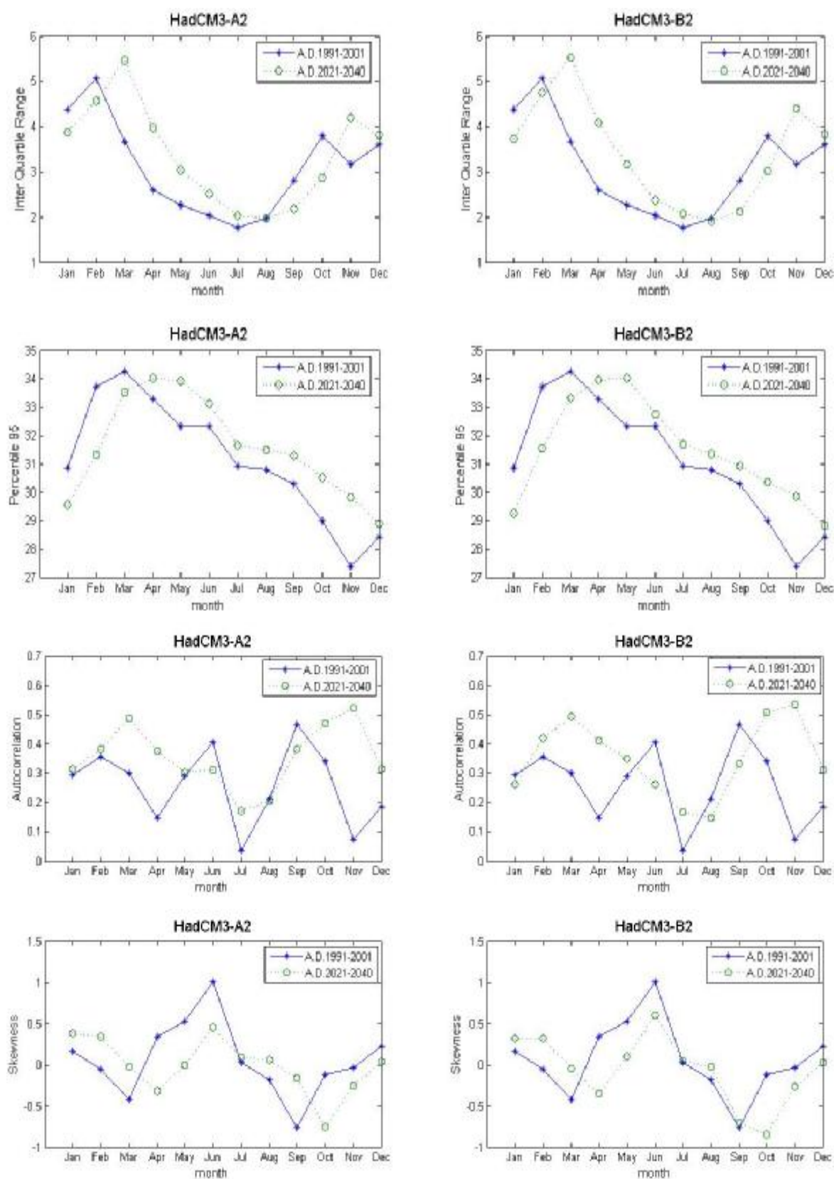
ภาพที่ ค.28 ค่าพิสัยระหว่างควอร์ไทล์ที่ 75 กับควอร์ไทล์ที่ 25 ค่าเปอร์เซ็นต์ไทล์ที่ 95 ค่าสัมประสิทธิ์สหสัมพันธ์ และ ค่าความเบ้ของข้อมูลอุณหภูมิเฉลี่ยรายวันสังเคราะห์จากภาพฉาย HadCM3A2 และ HadCM3B2 สำหรับช่วงปี ค.ศ.1991-2001 และช่วงปี ค.ศ.2021-2040 (สถานี 387401)
