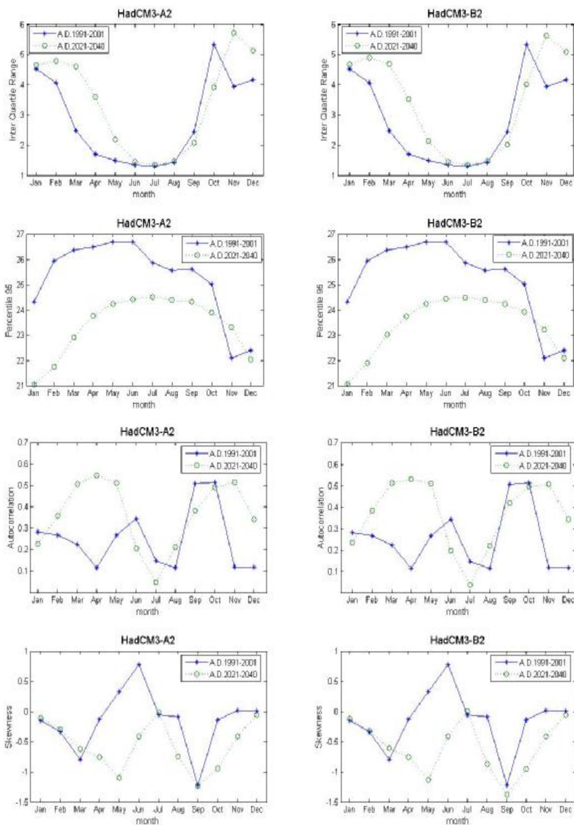
ภาพที่ ค.136 ค่าพิสัยระหว่างควอร์ไทล์ที่ 75 กับควอร์ไทล์ที่ 25 ค่าเปอร์เซ็นต์ไทล์ที่ 95 ค่าสัมประสิทธิ์สหสัมพันธ์ และค่าสัมประสิทธิ์ความเบ้ของข้อมูลอุณหภูมิต่ำสุดรายวันสังเคราะห์จากภาพฉาย HadCM3A2 และ HadCM3B2 สำหรับช่วงปี ค.ศ.1991-2001 และช่วงปี ค.ศ.2021-2040 (สถานี 431301)
