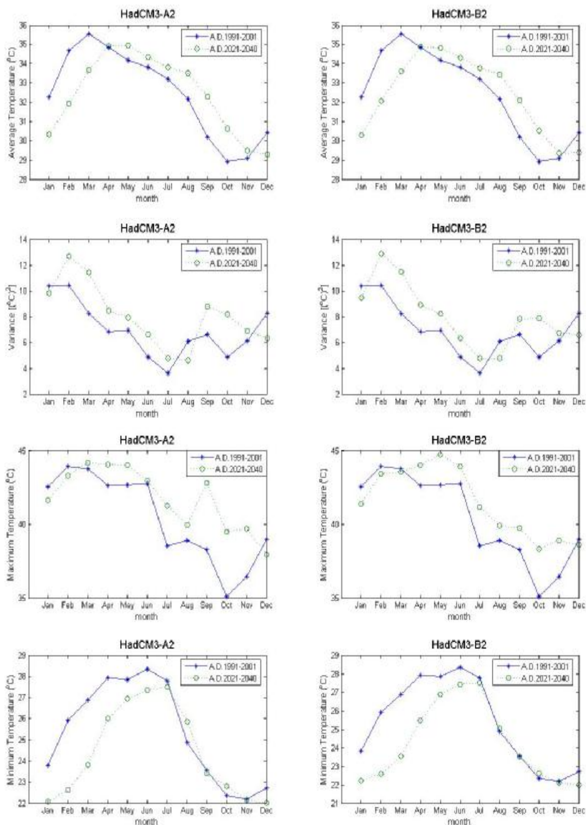
ภาพที่ ค.119 ค่าเฉลี่ย ค่าความแปรปรวน ค่าสูงสุด และค่าต่ำสุดของข้อมูลอุณหภูมิสูงสุดรายวันสังเคราะห์จาก ภาพฉาย HadCM3A2 และ HadCM3B2 สำหรับช่วงปี ค.ศ.1991-2001 และช่วงปี ค.ศ.2021-2040 (สถานี 431401)
