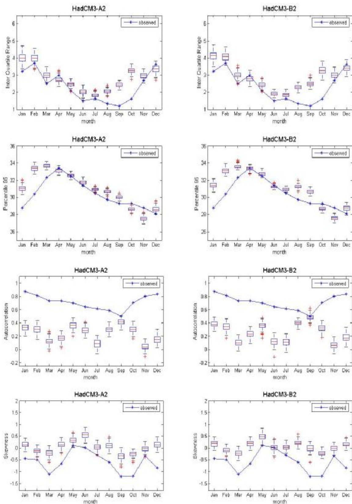
ภาพที่ ค.6 ค่าพิสัยระหว่างควอร์ไทล์ที่ 75 กับควอร์ไทล์ที่ 25 ค่าเปอร์เซ็นต์ไทล์ที่ 95 ค่าสัมประสิทธิ์สหสัมพันธ์ และค่าความเบ้ของข้อมูลอุณหภูมิเฉลี่ยรายวันอดีต และของข้อมูลสังเคราะห์จากภาพฉาย HadCM3A2 และ HadCM3B2 สำหรับสถานี 403201 (ปี ค.ศ.1991-2001)
