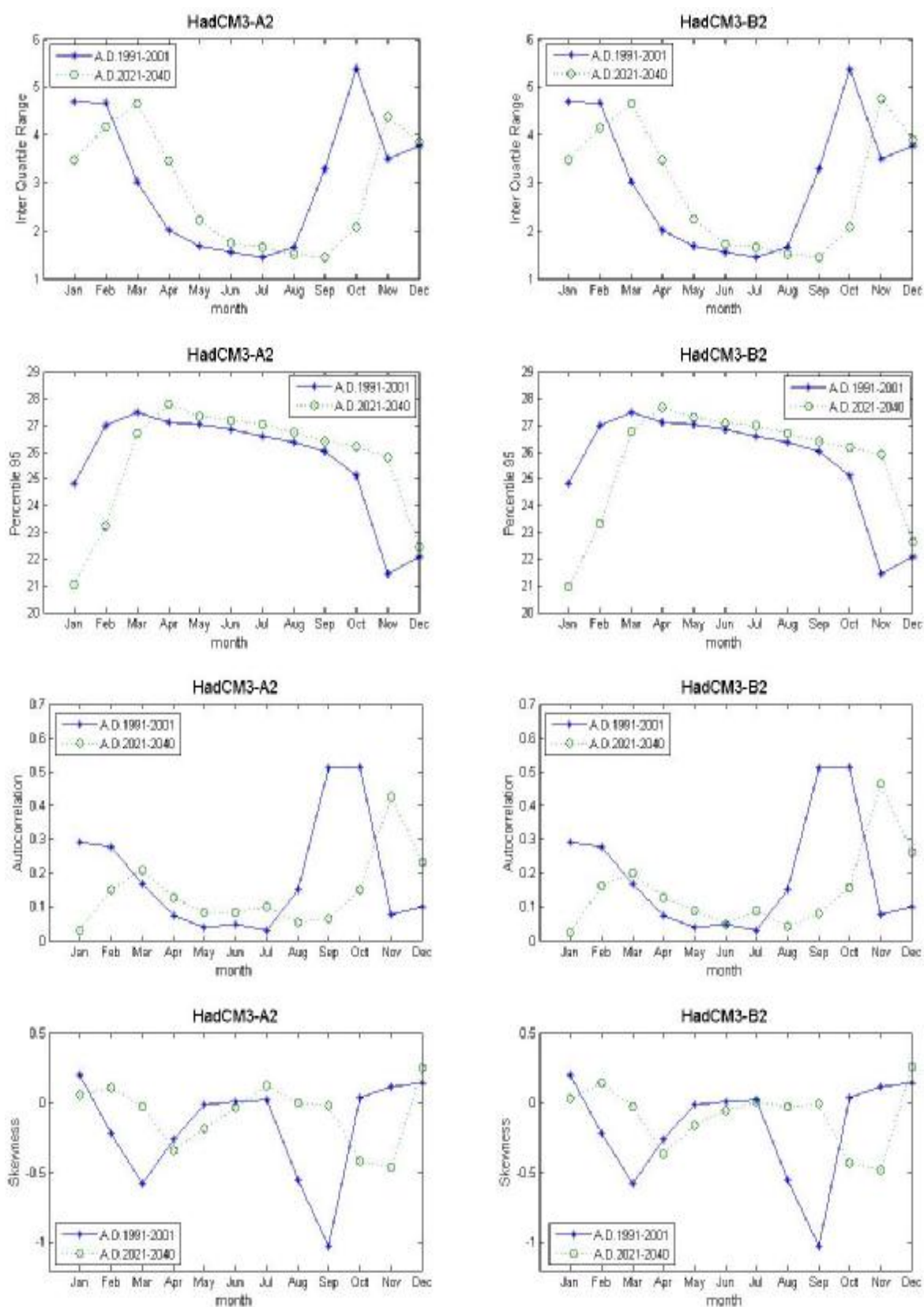
ภาพที่ ค.48 ค่าพิสัยระหว่างควอร์ไทล์ที่ 75 กับควอร์ไทล์ที่ 25 ค่าเปอร์เซ็นต์ไทล์ที่ 95 สัมประสิทธิ์สหสัมพันธ์ และค่าความเบ้ของข้อมูลอุณหภูมิต่ำสุดรายวันสังเคราะห์จากภาพฉาย HadCM3A2 และ HadCM3B2 สำหรับช่วงปี ค.ศ. 1991-2001 และช่วงปี ค.ศ.2021-2040 (สถานี 405201)
