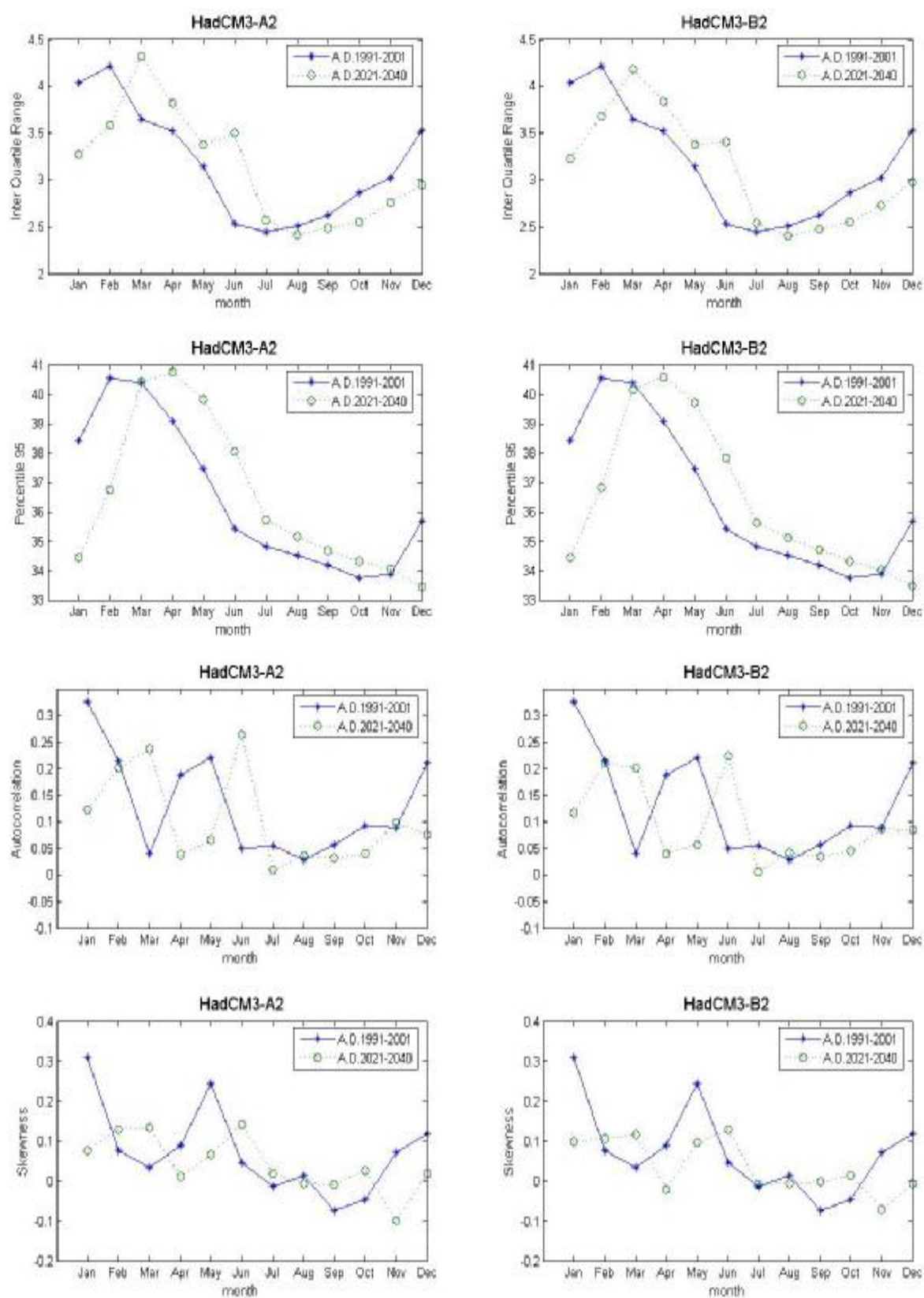
ภาพที่ ค.114 ค่าพิสัยระหว่างควอร์ไทล์ที่ 75 กับควอร์ไทล์ที่ 25 ค่าเปอร์เซ็นต์ไทล์ที่ 95 ค่าสัมประสิทธิ์สหสัมพันธ์ และค่าสัมประสิทธิ์ความเบ้ของข้อมูลอุณหภูมิสูงสุดรายวันสังเคราะห์จากภาพฉาย HadCM3A2 และ HadCM3B2 สำหรับช่วงปี ค.ศ.1991-2001 และช่วงปี ค.ศ.2021-2040 (สถานี 407501)
