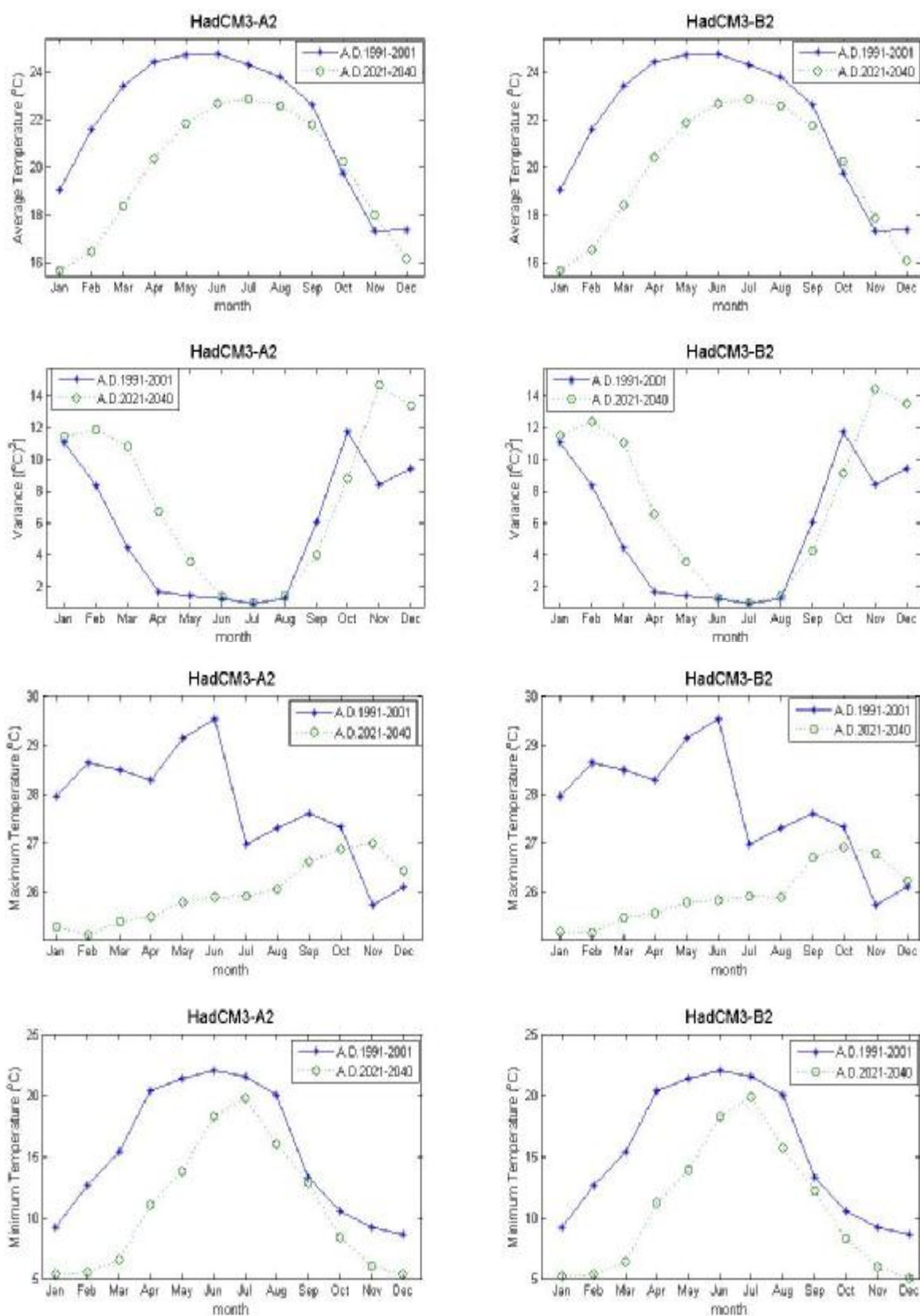
ภาพที่ ค.135 ค่าเฉลี่ย ค่าความแปรปรวน ค่าสูงสุด และค่าต่ำสุดของข้อมูลอุณหภูมิรายวันสังเคราะห์จาก ภาพฉาย HadCM3A2 และ HadCM3B2 สำหรับช่วงปี ค.ศ.1991-2001 และช่วงปี ค.ศ.2021-2040 (สถานี 431301)
