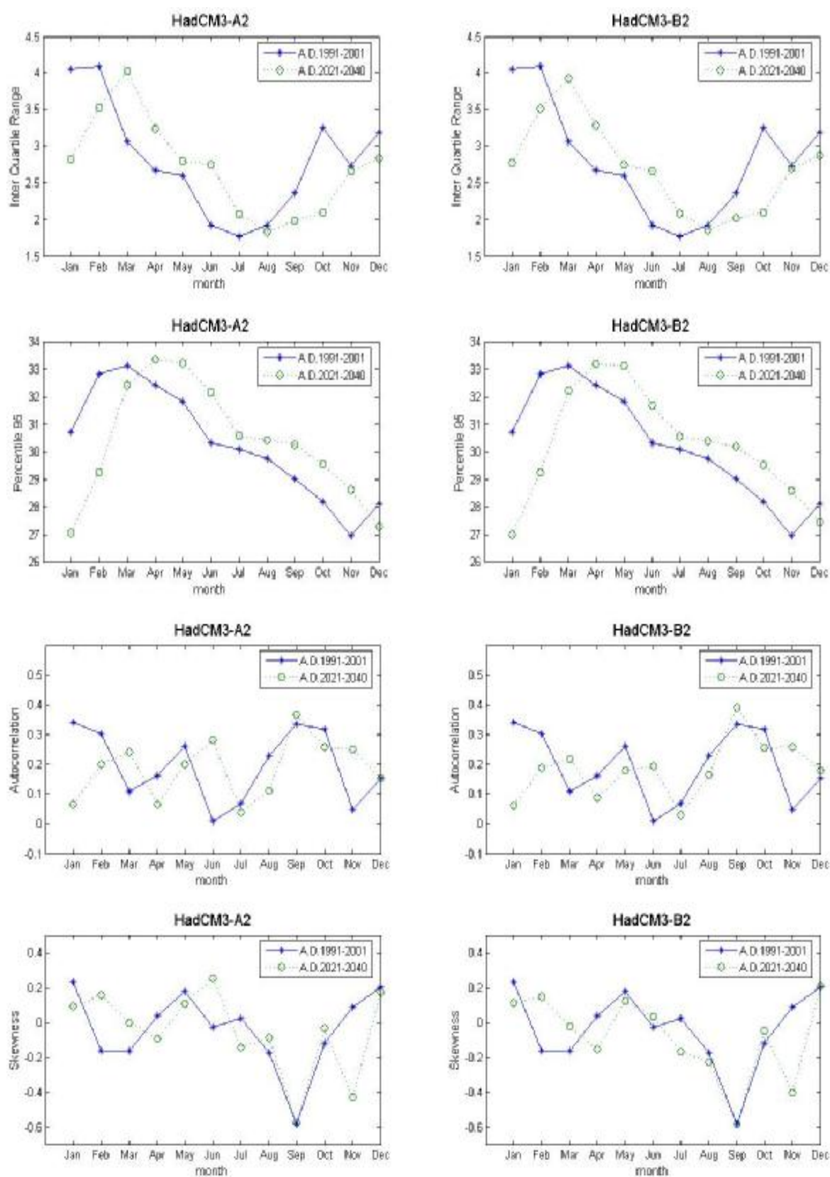
ภาพที่ ค.98 ค่าพิสัยระหว่างควอร์ไทล์ที่ 75 กับควอร์ไทล์ที่ 25 ค่าเปอร์เซ็นต์ไทล์ที่ 95 ค่าสัมประสิทธิ์สหสัมพันธ์ และค่าสัมประสิทธิ์ความเบ้ของข้อมูลอุณหภูมิเฉลี่ยรายวันสังเคราะห์จากภาพฉาย HadCM3A2 และ HadCM3B2 สำหรับช่วงปี ค.ศ.1991-2001 และช่วงปี ค.ศ.2021-2040 (สถานี 407301)
