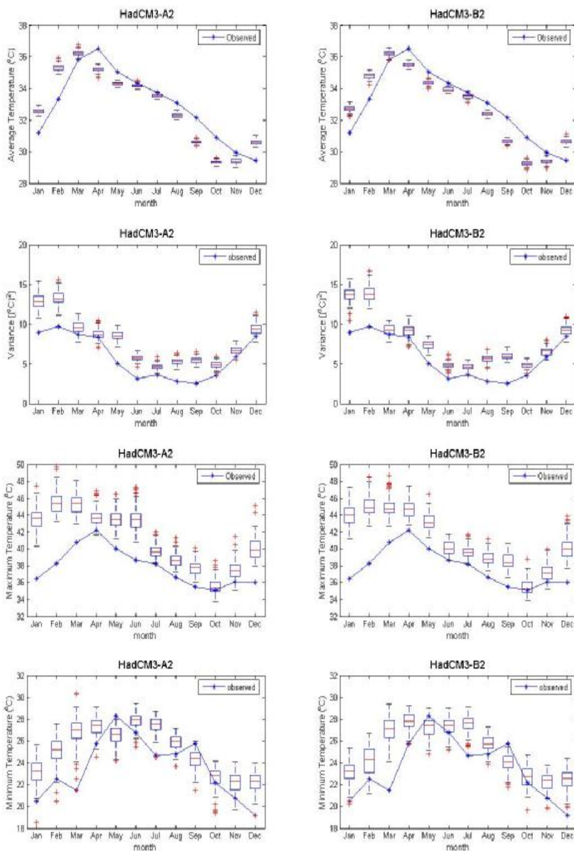
ภาพที่ ค.67 ค่าเฉลี่ย ค่าความแปรปรวน ค่าสูงสุด และค่าต่ำสุดของข้อมูลอุณหภูมิสูงสุดรายวันอดีต และของข้อมูลสังเคราะห์จากภาพฉาย HadCM3A2 และ HadCM3B2 สำหรับสถานี 431201 (ปี ค.ศ.1991-2001)
