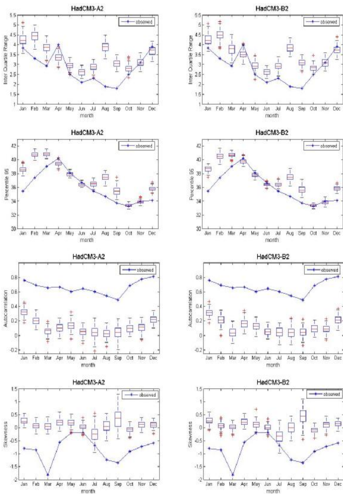
ภาพที่ ค.76 ค่าพิสัยระหว่างควอร์ไทล์ที่ 75 กับควอร์ไทล์ที่ 25 ค่าเปอร์เซ็นต์ไทล์ที่ 95 ค่าสัมประสิทธิ์สหสัมพันธ์ และค่าความเบ้ของข้อมูลอุณหภูมิสูงสุดรายวันอดีต และของข้อมูลสังเคราะห์จากภาพฉาย HadCM3A2 และ HadCM3B2 สำหรับสถานี 432301 (ปี ค.ศ.1991-2001)
