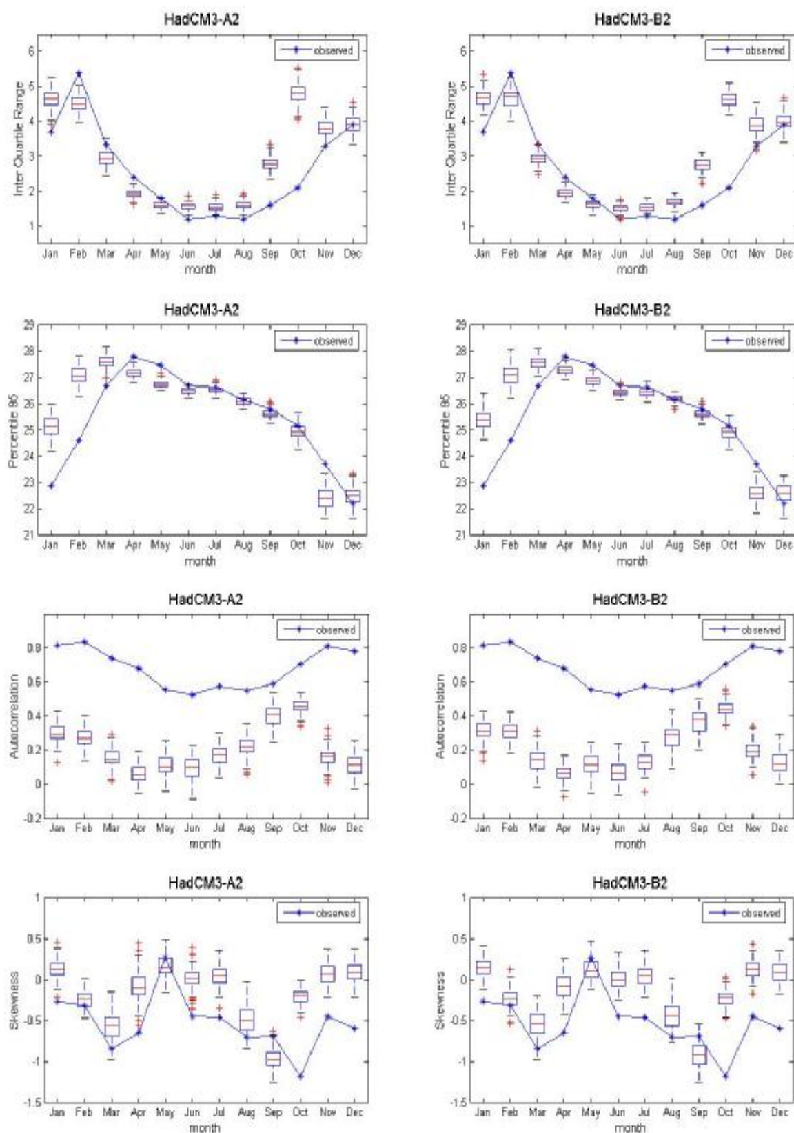
ภาพที่ ค.94 ค่าพิสัยระหว่างควอร์ไทล์ที่ 75 กับควอร์ไทล์ที่ 25 ค่าเปอร์เซ็นต์ไทล์ที่ 95 ค่าสัมประสิทธิ์สหสัมพันธ์ และค่าความเบ้ของข้อมูลอุณหภูมิต่ำสุดรายวันอดีต และของข้อมูลสังเคราะห์จากภาพฉาย HadCM3A2 และ HadCM3B2 สำหรับสถานี 432401 (ปี ค.ศ.1991-2001)
