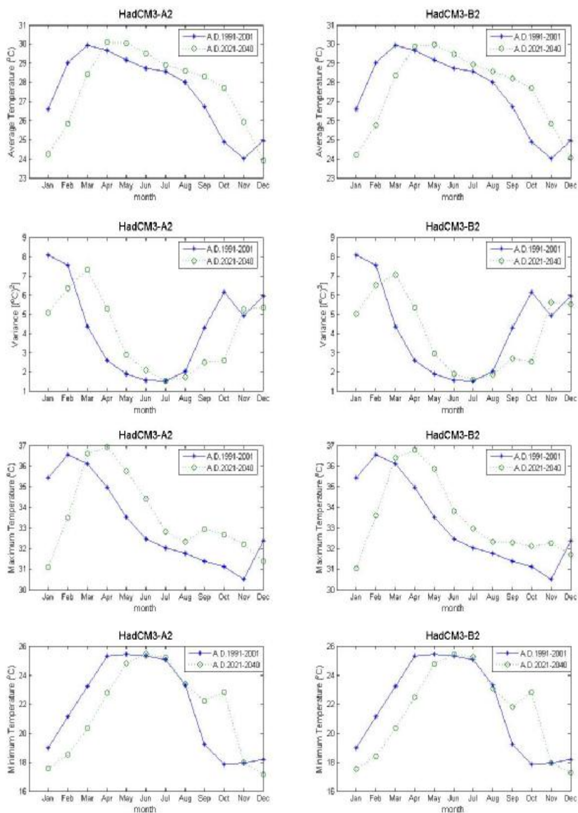
ภาพที่ ค.105 ค่าเฉลี่ย ค่าความแปรปรวน ค่าสูงสุด และค่าต่ำสุดของข้อมูลอุณหภูมิเฉลี่ยรายวันสังเคราะห์จาก ภาพฉาย HadCM3A2 และ HadCM3B2 สำหรับช่วงปี ค.ศ.1991-2001 และช่วงปี ค.ศ.2021-2040 (สถานี 432201)
