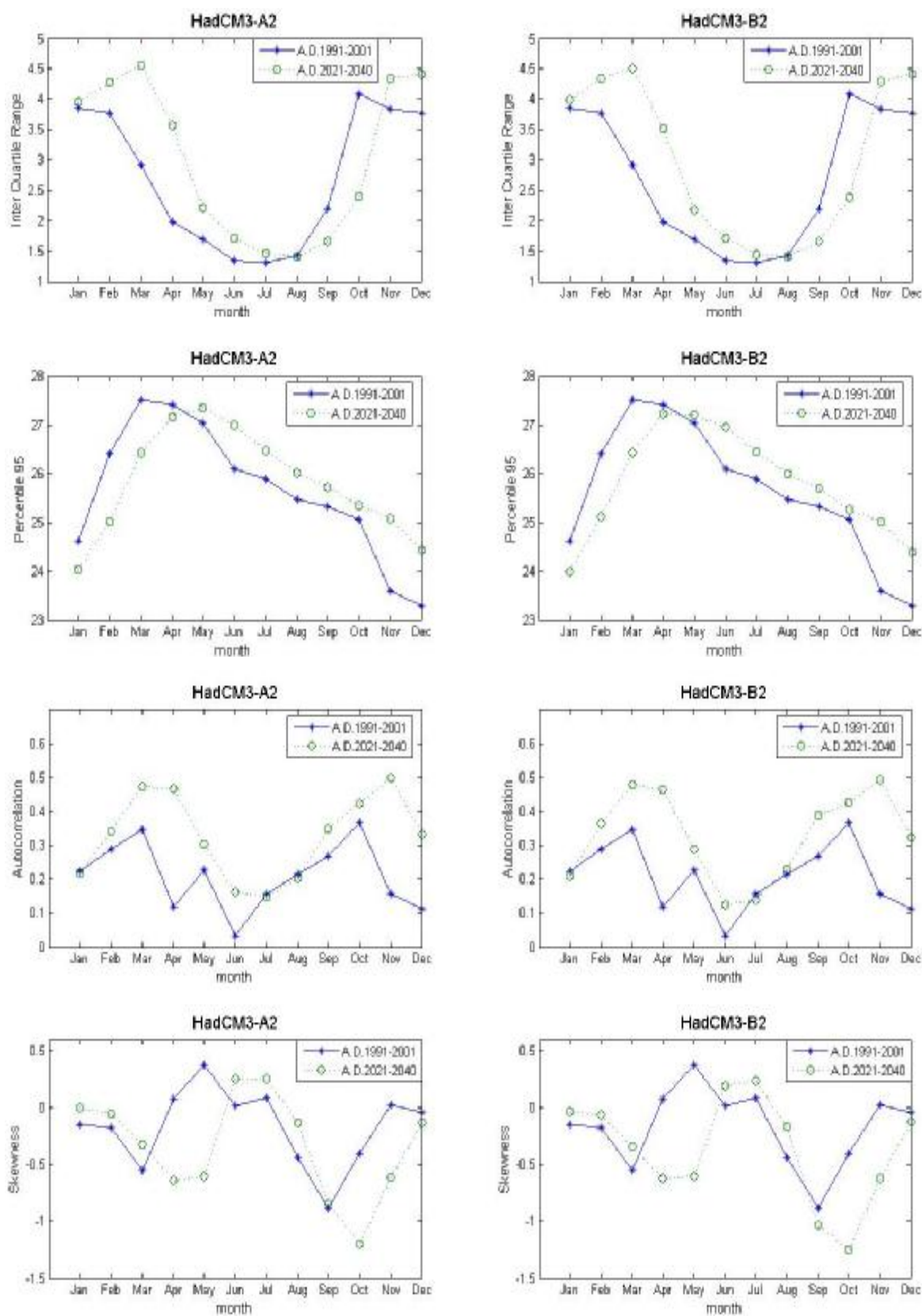
ภาพที่ ค.46 ค่าพิสัยระหว่างควอร์ไทล์ที่ 75 กับควอร์ไทล์ที่ 25 ค่าเปอร์เซ็นต์ไทล์ที่ 95 ค่าสัมประสิทธิ์สหสัมพันธ์ และ ค่าความเบ้ของข้อมูลอุณหภูมิต่ำสุดรายวันสังเคราะห์จากภาพฉาย HadCM3A2 และ HadCM3B2 สำหรับช่วงปี ค.ศ.1991-2001 และช่วงปี ค.ศ.2021-2040 (สถานี 403201)
