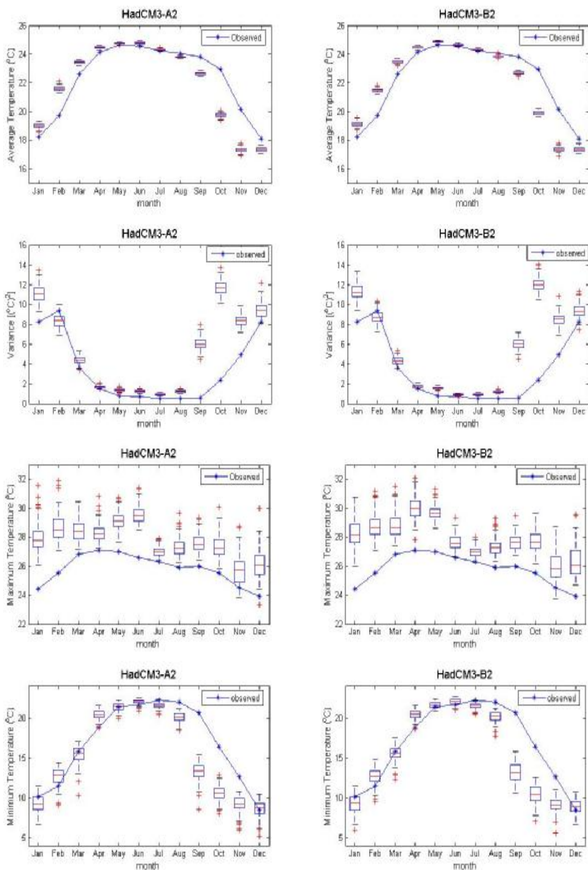
ภาพที่ ค.95 ค่าเฉลี่ย ค่าความแปรปรวน ค่าสูงสุด และค่าต่ำสุดของข้อมูลอุณหภูมิต่ำสุดรายวันอดีต และของข้อมูลสังเคราะห์จากภาพฉาย HadCM3A2 และ HadCM3B2 สำหรับสถานี 436401 (ปี ค.ศ.1991-2001)
