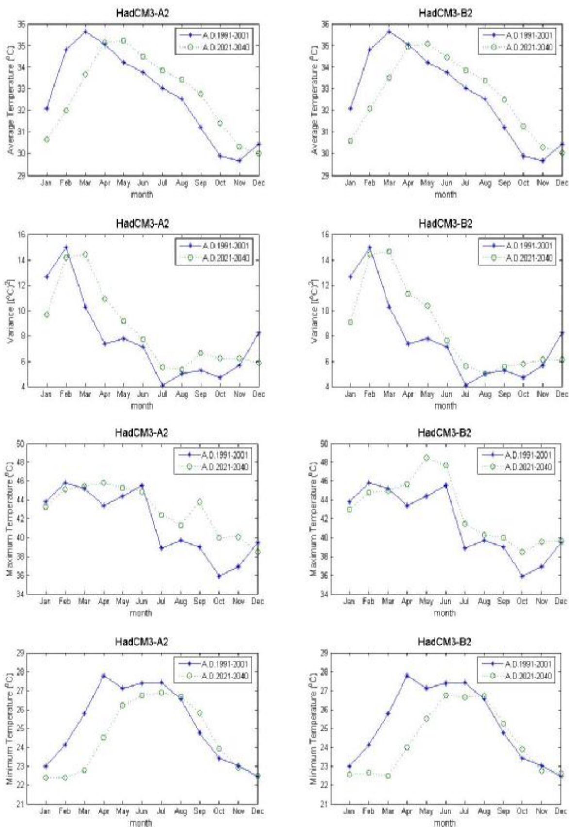
ภาพที่ ค.35 ค่าเฉลี่ย ค่าความแปรปรวน ค่าสูงสุด และค่าต่ำสุดของข้อมูลอุณหภูมิสูงสุดรายวันสังเคราะห์จากภาพฉาย HadCM3A2 และ HadCM3B2 สำหรับช่วงปี ค.ศ.1991-2001 และช่วงปี ค.ศ.2021-2040 (สถานี 387401)
