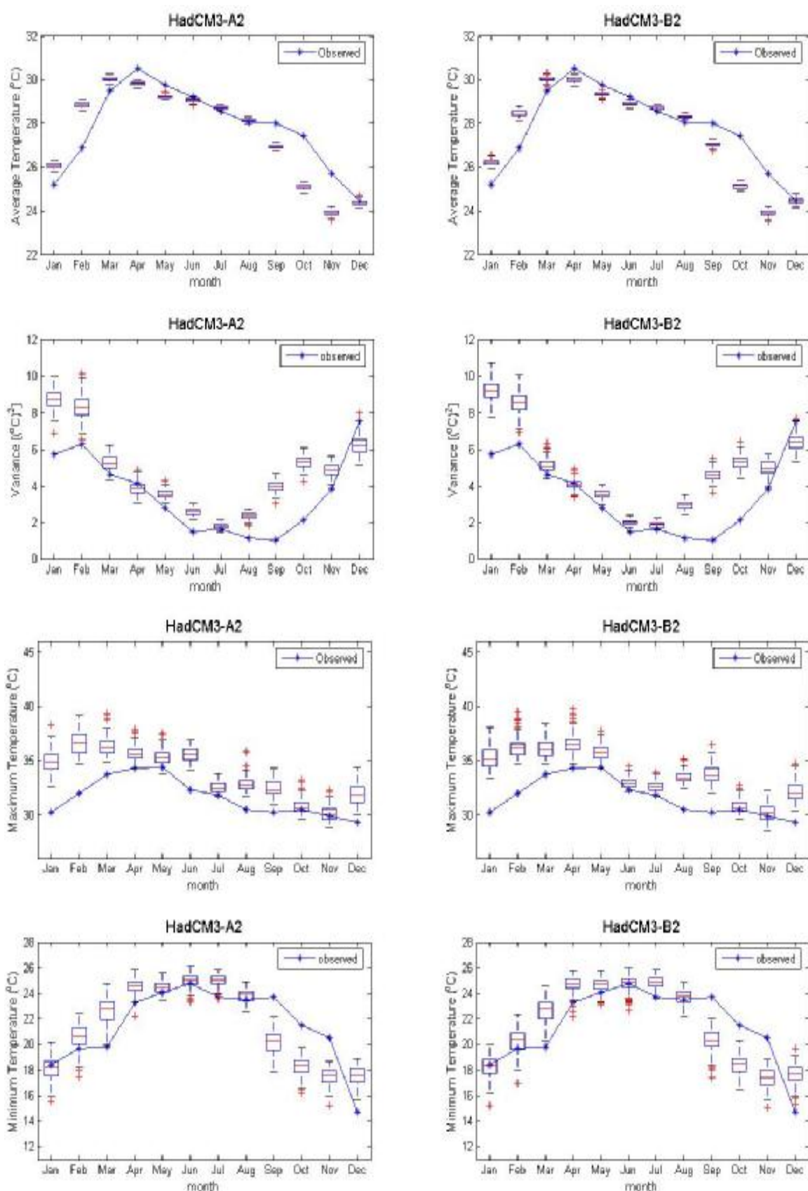
ภาพที่ ค.5 ค่าเฉลี่ย ค่าความแปรปรวน ค่าสูงสุด และค่าต่ำสุดของข้อมูลอุณหภูมิเฉลี่ยรายวันอดีต และของข้อมูลสังเคราะห์จากภาพฉาย HadCM3A2 และ HadCM3B2 สำหรับสถานี 403201 (ปี ค.ศ.1991-2001)
