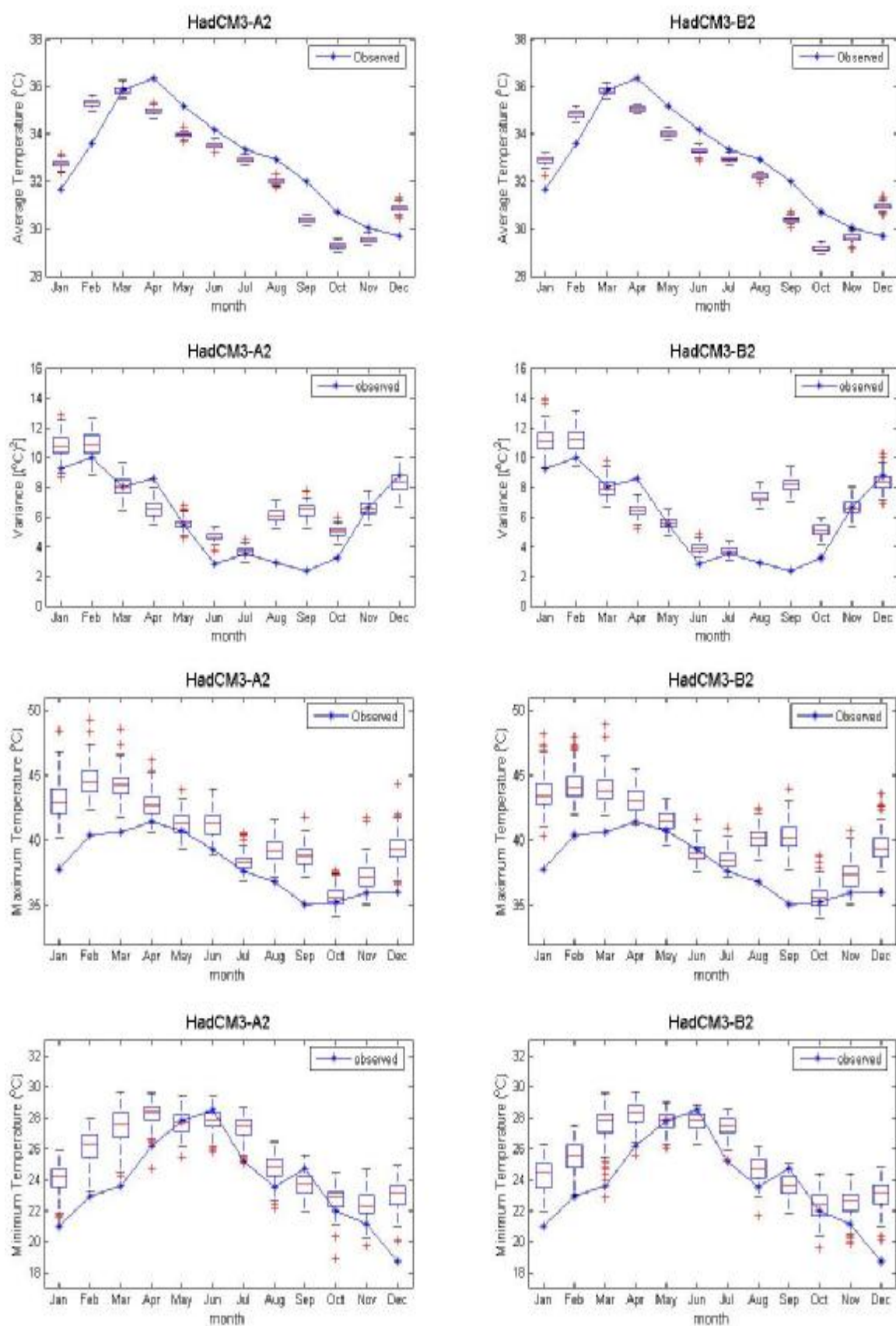
ภาพที่ ค.79 ค่าเฉลี่ย ค่าความแปรปรวน ค่าสูงสุด และค่าต่ำสุดของข้อมูลอุณหภูมิสูงสุดรายวันอดีต และของข้อมูลสังเคราะห์จากภาพฉาย HadCM3A2 และ HadCM3B2 สำหรับสถานี 436401 (ปี ค.ศ.1991-2001)
