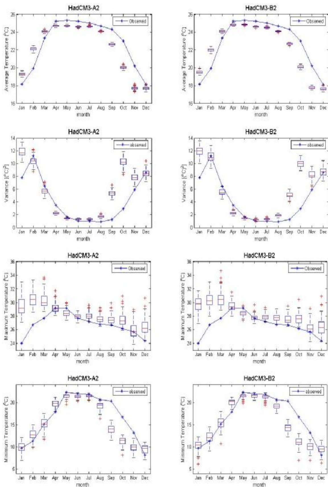
ภาพที่ ค.93 ค่าเฉลี่ย ค่าความแปรปรวน ค่าสูงสุด และค่าต่ำสุดของข้อมูลอุณหภูมิรายวันอดีต และของข้อมูลสังเคราะห์จากภาพฉาย HadCM3A2 และ HadCM3B2 สำหรับสถานี 432401 (ปี ค.ศ.1991-2001)
