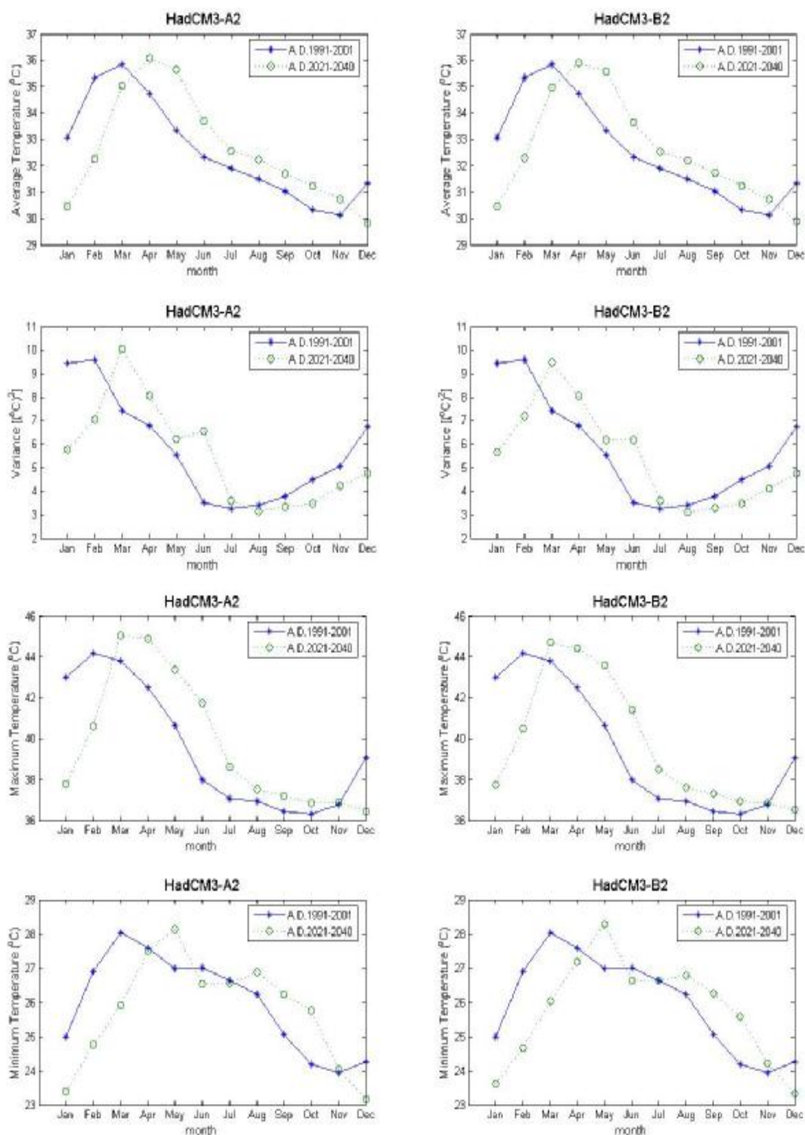
ภาพที่ ค.113 ค่าเฉลี่ย ค่าความแปรปรวน ค่าสูงสุด และค่าต่ำสุดของข้อมูลอุณหภูมิสูงสุดรายวันสังเคราะห์จาก ภาพฉาย HadCM3A2 และ HadCM3B2 สำหรับช่วงปี ค.ศ.1991-2001 และช่วงปี ค.ศ.2021-2040 (สถานี 407501)
