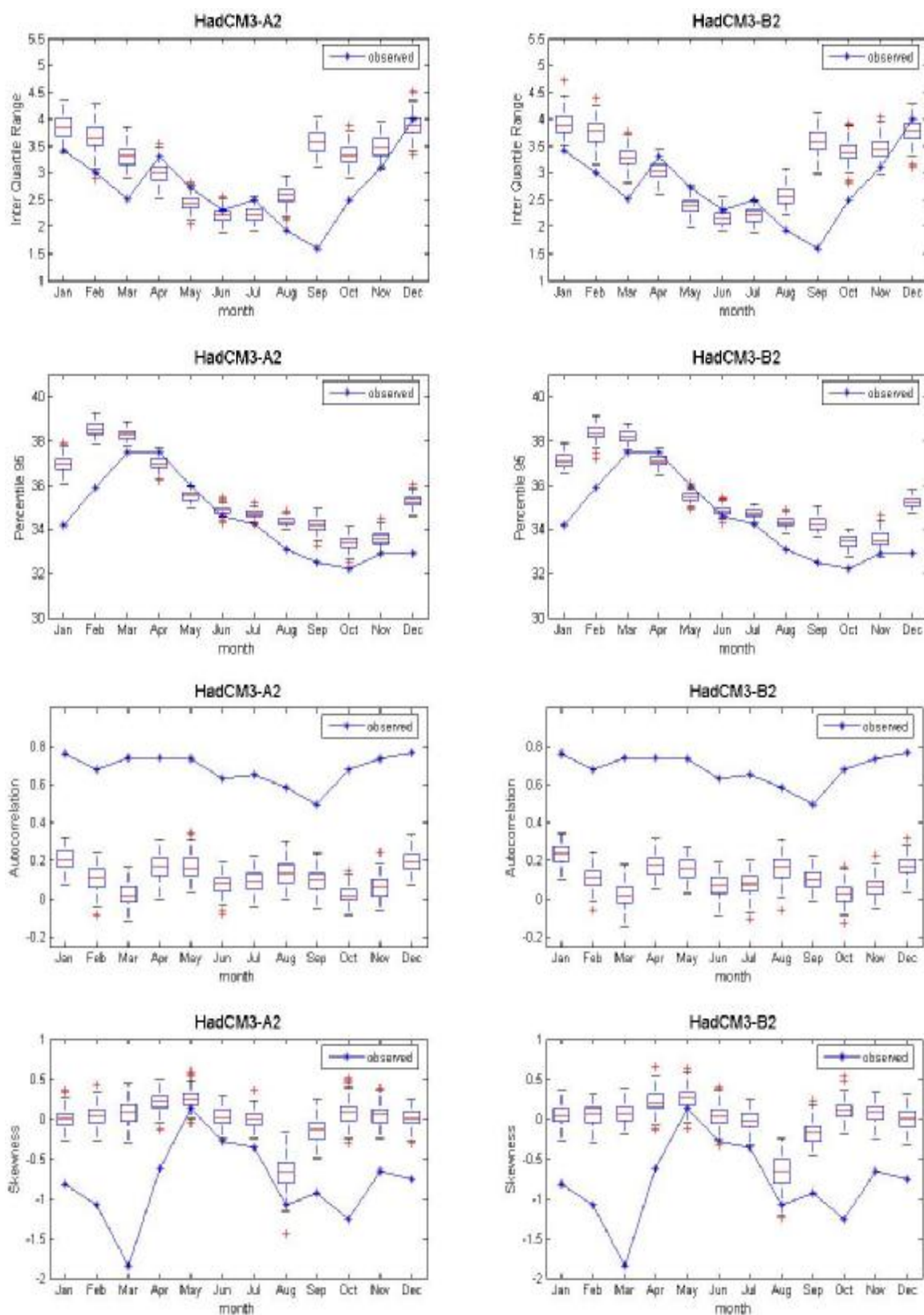
ภาพที่ ค.70 ค่าพิสัยระหว่างควอร์ไทล์ที่ 75 กับควอร์ไทล์ที่ 25 ค่าเปอร์เซ็นต์ไทล์ที่ 95 ค่าสัมประสิทธิ์สหสัมพันธ์ และค่าความเบ้ของข้อมูลอุณหภูมิสูงสุดรายวันอดีต และของข้อมูลสังเคราะห์จากภาพฉาย HadCM3A2 และ HadCM3B2 สำหรับสถานี 431301 (ปี ค.ศ.1991-2001)
