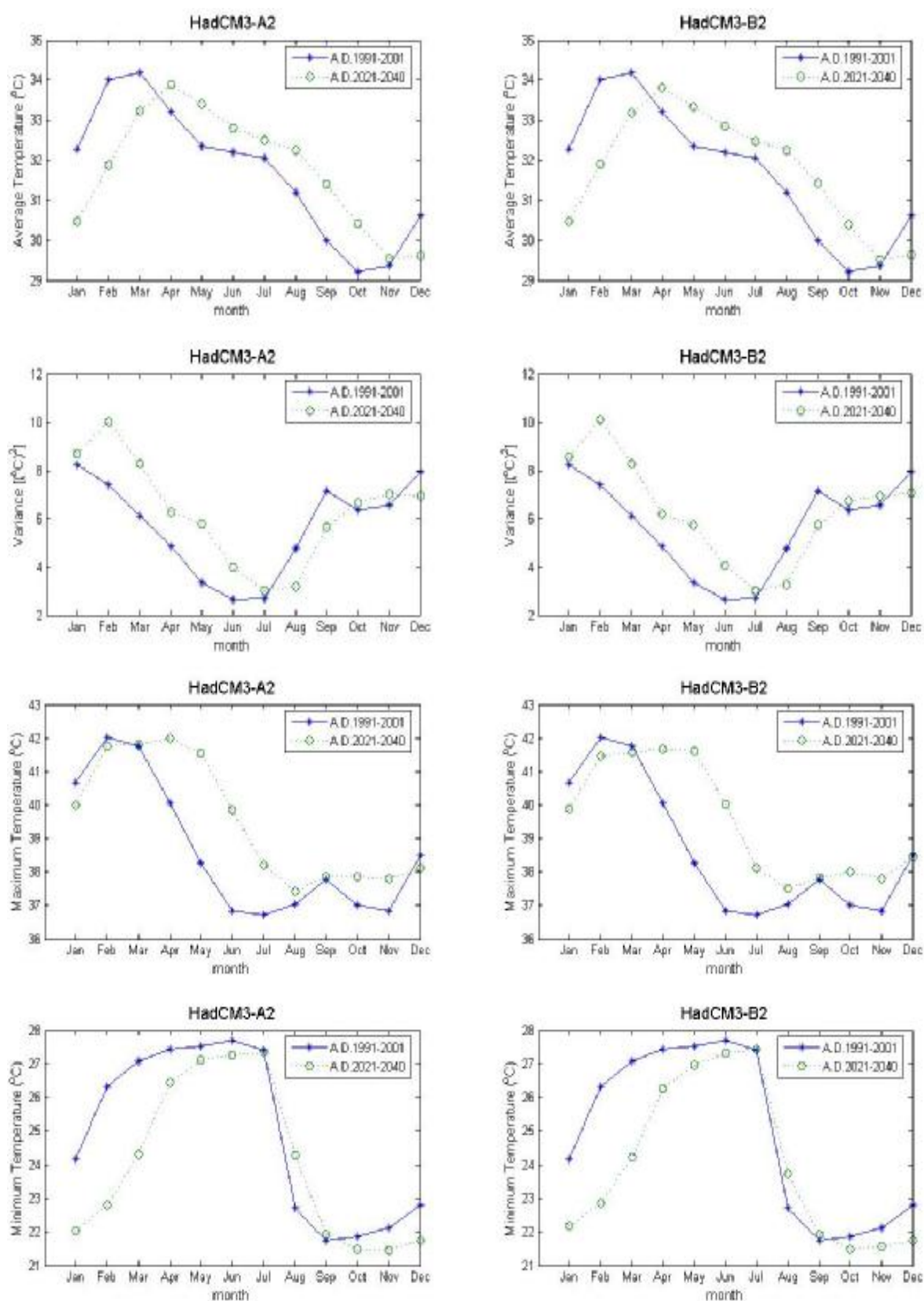
ภาพที่ ค.117 ค่าเฉลี่ย ค่าความแปรปรวน ค่าสูงสุด และค่าต่ำสุดของข้อมูลอุณหภูมิสูงสุดรายวันสังเคราะห์จาก ภาพฉาย HadCM3A2 และ HadCM3B2 สำหรับช่วงปี ค.ศ.1991-2001 และช่วงปี ค.ศ.2021-2040 (สถานี 431301)
