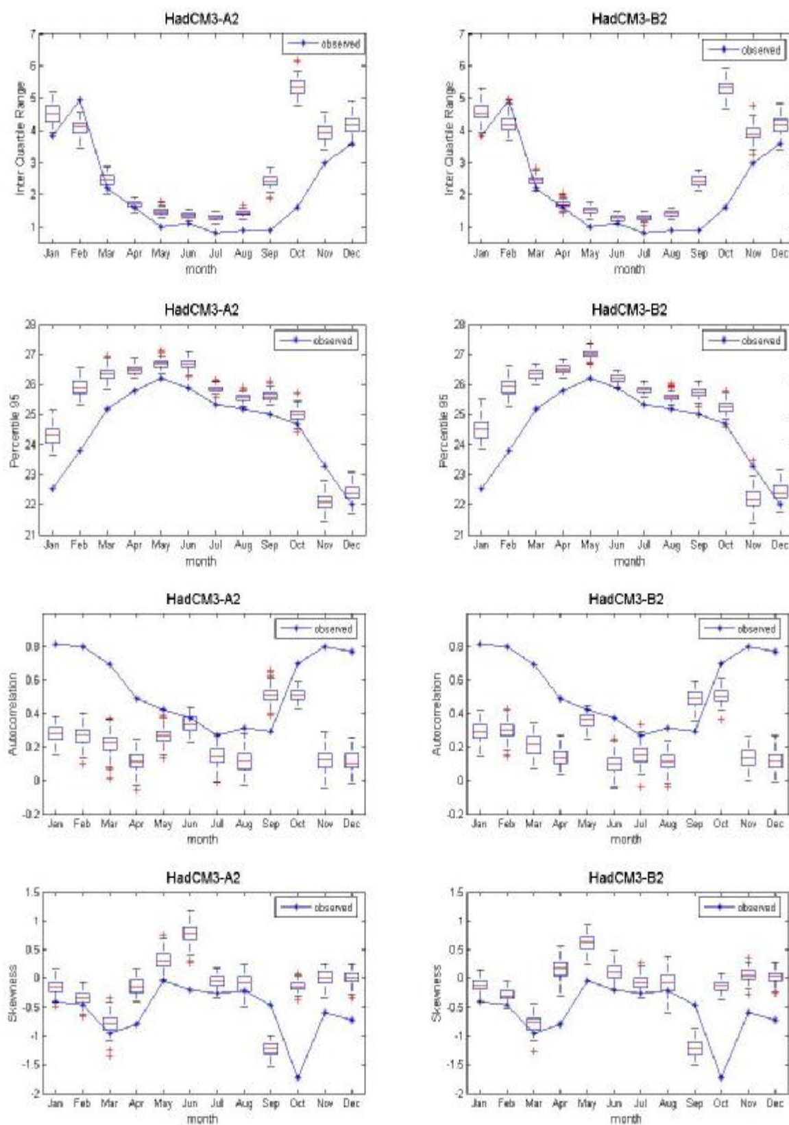
ภาพที่ ค.96 ค่าพิสัยระหว่างควอร์ไทล์ที่ 75 กับควอร์ไทล์ที่ 25 ค่าเปอร์เซ็นต์ไทล์ที่ 95 ค่าสัมประสิทธิ์สหสัมพันธ์ และค่าความเบ้ของข้อมูลอุณหภูมิต่ำสุดรายวันอดีต และของข้อมูลสังเคราะห์จากภาพฉาย HadCM3A2 และ HadCM3B2 สำหรับสถานี 436401 (ปี ค.ศ.1991-2001)
