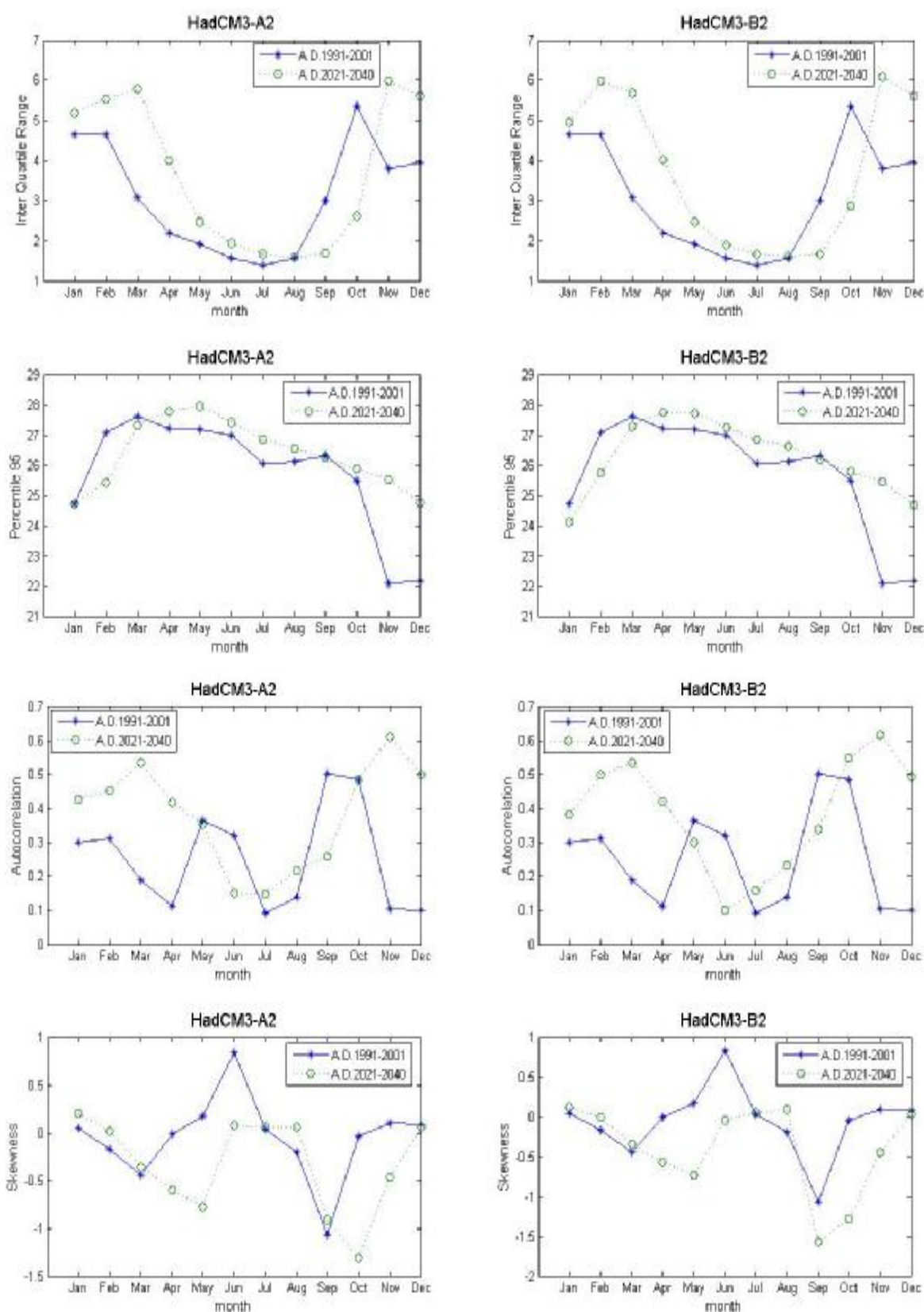
ภาพที่ ค.44 ค่าพิสัยระหว่างควอร์ไทล์ที่ 75 กับควอร์ไทล์ที่ 25 ค่าเปอร์เซ็นต์ไทล์ที่ 95 ค่าสัมประสิทธิ์สหสัมพันธ์ และ ค่าความเบ้ของข้อมูลอุณหภูมิต่ำสุดรายวันสังเคราะห์จากภาพฉาย HadCM3A2 และ HadCM3B2 สำหรับช่วงปี ค.ศ.1991-2001 และช่วงปี ค.ศ.2021-2040 (สถานี 381301)
