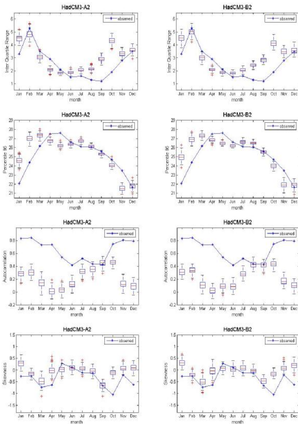
ภาพที่ ค.84 ค่าพิสัยระหว่างควอร์ไทล์ที่ 75 กับควอร์ไทล์ที่ 25 ค่าเปอร์เซ็นต์ไทล์ที่ 95 ค่าสัมประสิทธิ์สหสัมพันธ์ และค่าความเบ้ของข้อมูลอุณหภูมิต่ำสุดรายวันอดีต และของข้อมูลสังเคราะห์จากภาพฉาย HadCM3A2 และ HadCM3B2 สำหรับสถานี 407501 (ปี ค.ศ.1991-2001)
