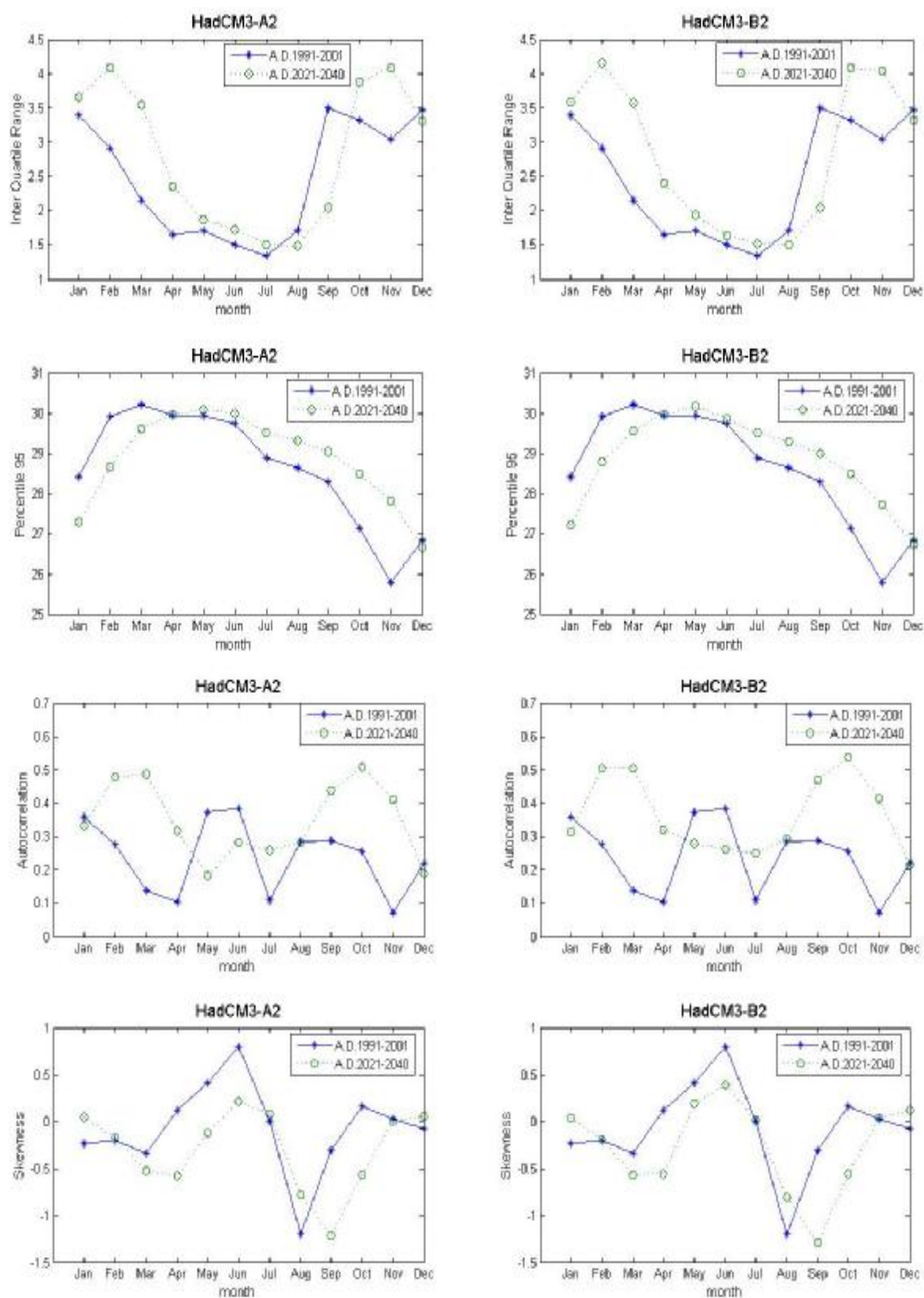
ภาพที่ ค.102 ค่าพิสัยระหว่างควอร์ไทล์ที่ 75 กับควอร์ไทล์ที่ 25 ค่าเปอร์เซ็นต์ไทล์ที่ 95 ค่าสัมประสิทธิ์สหสัมพันธ์ และค่าสัมประสิทธิ์ความเบ้ของข้อมูลอุณหภูมิเฉลี่ยรายวันสังเคราะห์จากภาพฉาย HadCM3A2 และ HadCM3B2 สำหรับช่วงปี ค.ศ.1991-2001 และช่วงปี ค.ศ.2021-2040 (สถานี 431301)
