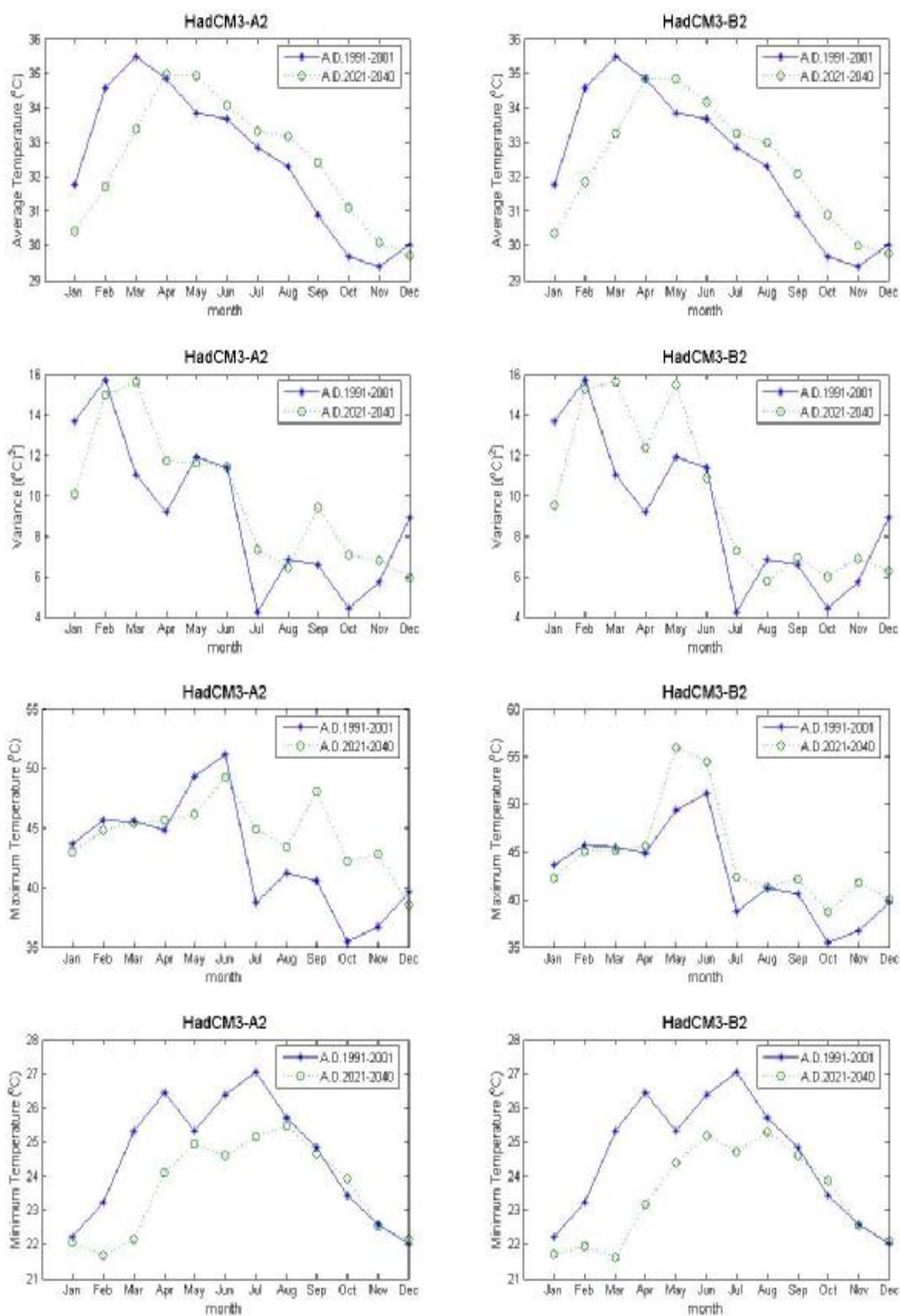
ภาพที่ ค.33 ค่าเฉลี่ย ค่าความแปรปรวน ค่าสูงสุด และค่าต่ำสุดของข้อมูลอุณหภูมิสูงสุดรายวันสังเคราะห์จากภาพฉาย HadCM3A2 และ HadCM3B2 สำหรับช่วงปี ค.ศ.1991-2001 และช่วงปี ค.ศ.2021-2040 (สถานี 381301)
