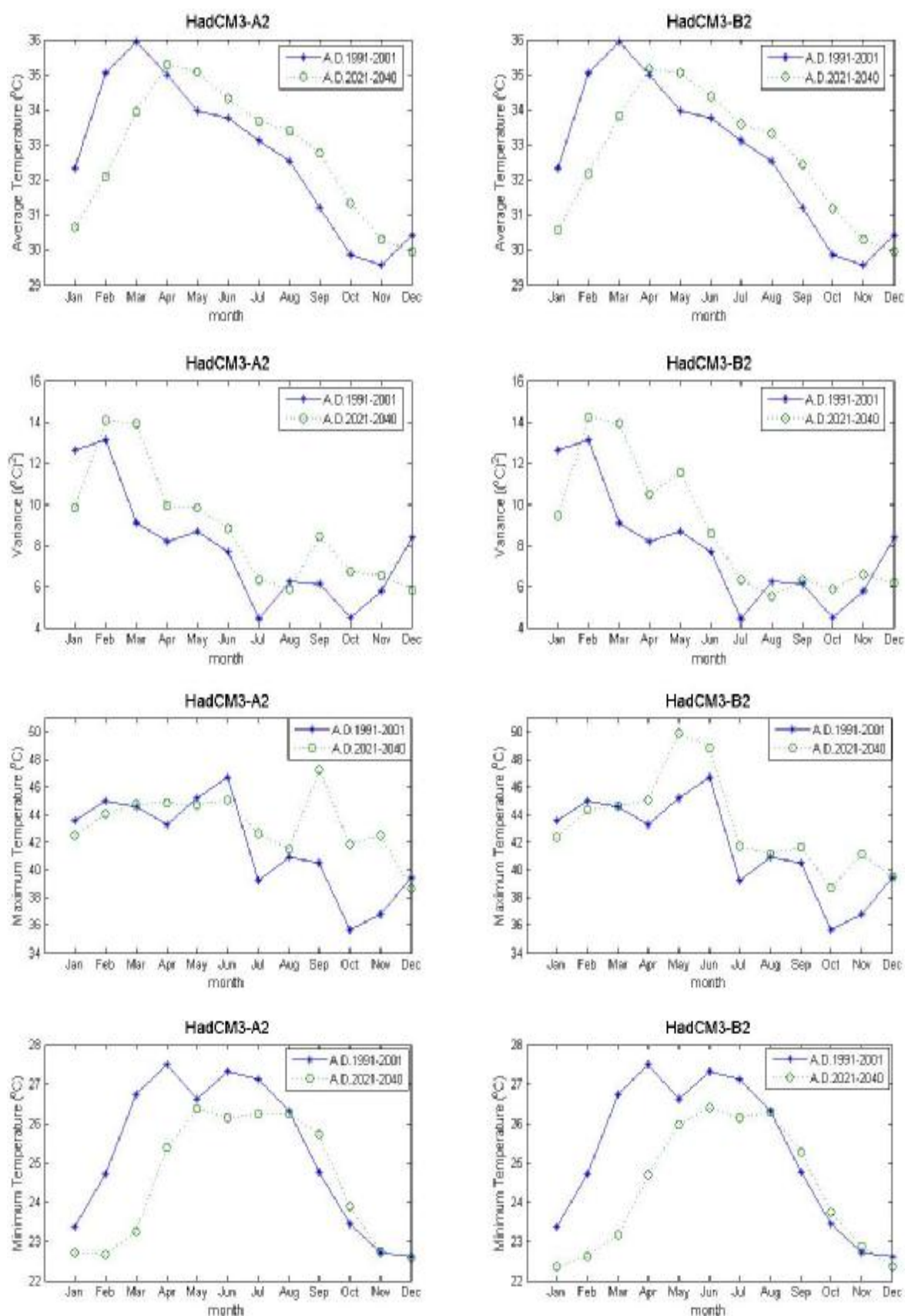
ภาพที่ ค.37 ค่าเฉลี่ย ค่าความแปรปรวน ค่าสูงสุด และค่าต่ำสุดของข้อมูลอุณหภูมิสูงสุดรายวันสังเคราะห์จากภาพฉาย HadCM3A2 และ HadCM3B2 สำหรับช่วงปี ค.ศ.1991-2001 และช่วงปี ค.ศ.2021-2040 (สถานี 403201)
