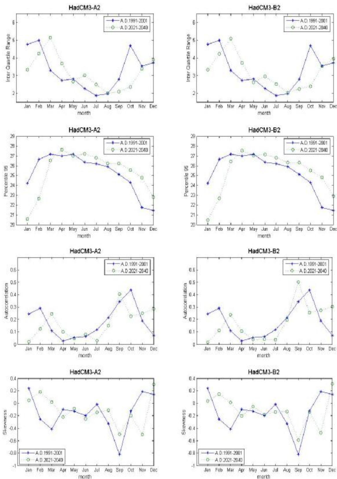
ภาพที่ ค.130 ค่าพิสัยระหว่างควอร์ไทล์ที่ 75 กับควอร์ไทล์ที่ 25 ค่าเปอร์เซ็นต์ไทล์ที่ 95 ค่าสัมประสิทธิ์สหสัมพันธ์ และค่าสัมประสิทธิ์ความเบ้ของข้อมูลอุณหภูมิต่ำสุดรายวันสังเคราะห์จากภาพฉาย HadCM3A2 และ HadCM3B2 สำหรับช่วงปี ค.ศ.1991-2001 และช่วงปี ค.ศ.2021-2040 (สถานี 407301)
