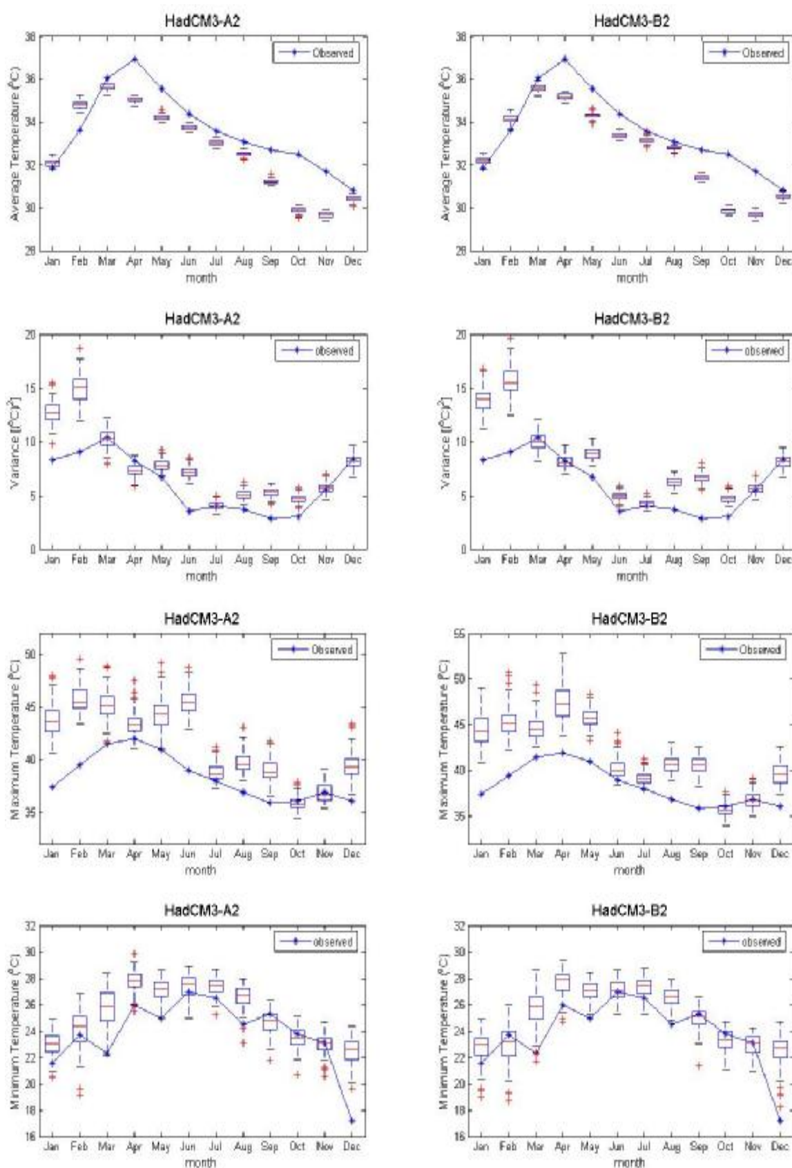
ภาพที่ ค.11 ค่าเฉลี่ย ค่าความแปรปรวน ค่าสูงสุด และค่าต่ำสุดของข้อมูลอุณหภูมิสูงสุดรายวันอดีต และของข้อมูลสังเคราะห์จากภาพฉาย HadCM3A2 และ HadCM3B2 สำหรับสถานี 387401 (ปี ค.ศ.1991-2001)
