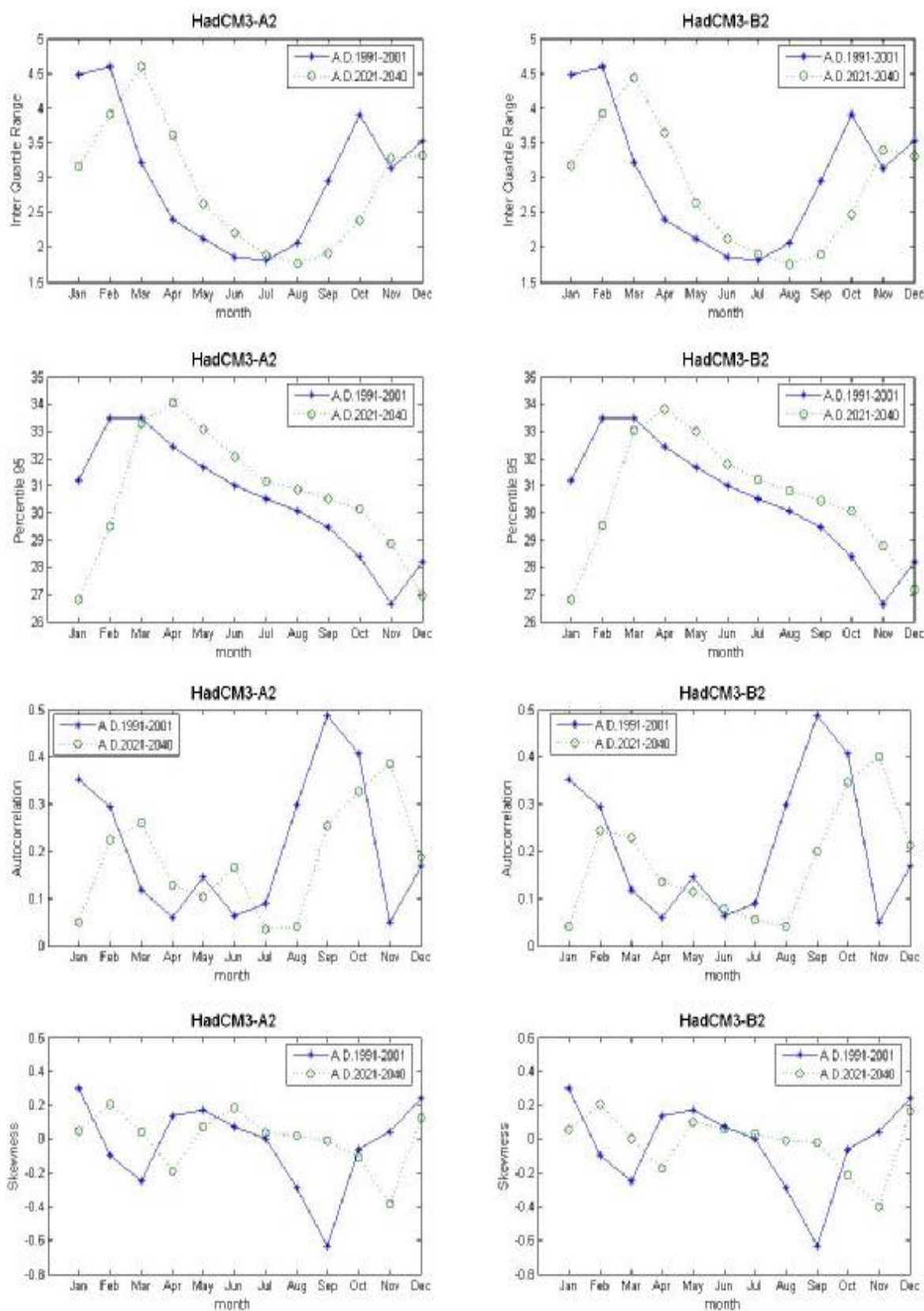
ภาพที่ ค.32 ค่าพิสัยระหว่างควอร์ไทล์ที่ 75 กับควอร์ไทล์ที่ 25 ค่าเปอร์เซ็นต์ไทล์ที่ 95 ค่าสัมประสิทธิ์สหสัมพันธ์ และ ค่าความเบ้ของข้อมูลอุณหภูมิเฉลี่ยรายวันสังเคราะห์จากภาพฉาย HadCM3A2 และ HadCM3B2 สำหรับช่วงปี ค.ศ.1991-2001 และช่วงปี ค.ศ.2021-2040 (สถานี 405201)
