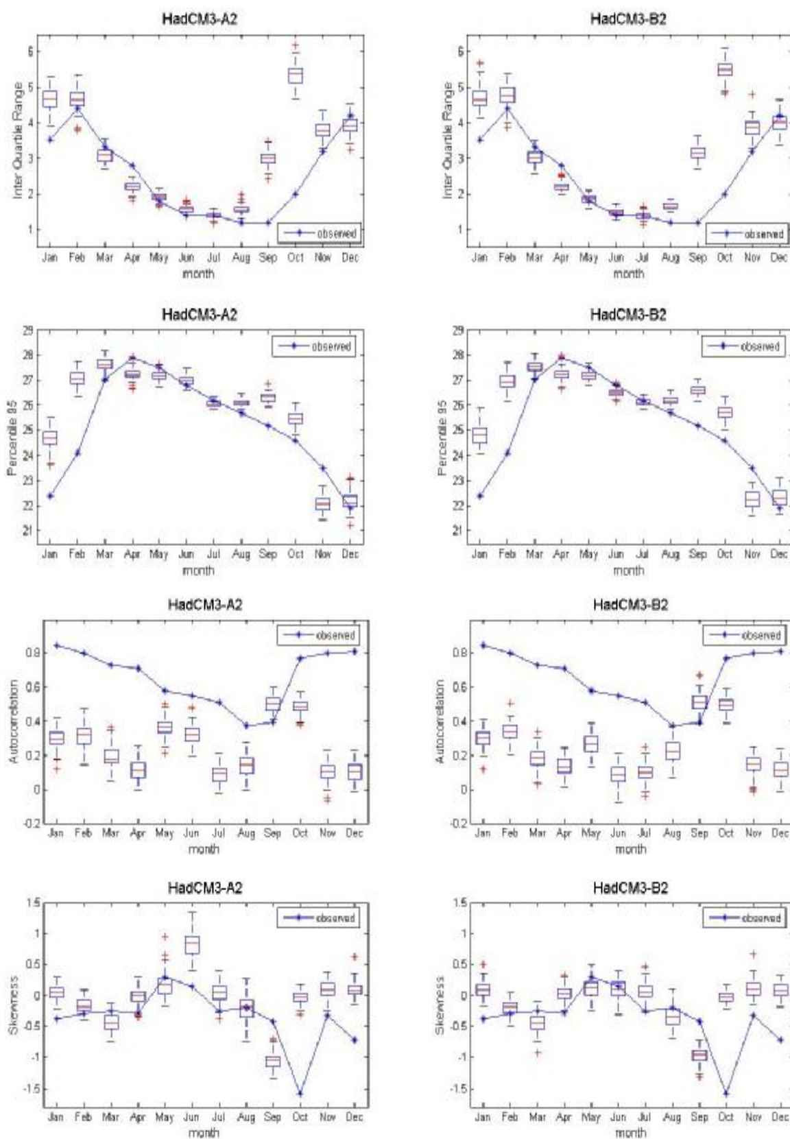
ภาพที่ ค.18 ค่าพิสัยระหว่างควอร์ไทล์ที่ 75 กับควอร์ไทล์ที่ 25 ค่าเปอร์เซ็นต์ไทล์ที่ 95 ค่าสัมประสิทธิ์สหสัมพันธ์ และค่าความเบ้ของข้อมูลอุณหภูมิต่ำสุดรายวันอดีต และของข้อมูลสังเคราะห์จากภาพฉาย HadCM3A2 และ HadCM3B2 สำหรับสถานี 381201 (ปี ค.ศ.1991-2001)
