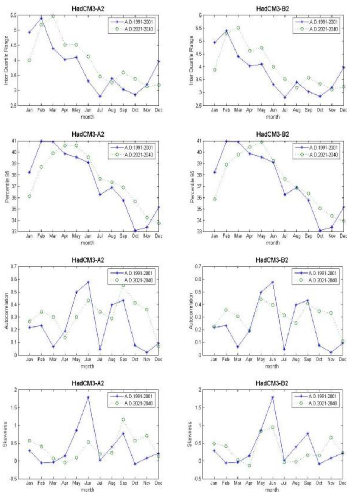
ภาพที่ ค.34 ค่าพิสัยระหว่างควอร์ไทล์ที่ 75 กับควอร์ไทล์ที่ 25 ค่าเปอร์เซ็นต์ไทล์ที่ 95 ค่าสัมประสิทธิ์สหสัมพันธ์ และ ค่าความเบ้ของข้อมูลอุณหภูมิสูงสุดรายวันสังเคราะห์จากภาพฉาย HadCM3A2 และ HadCM3B2 สำหรับช่วงปี ค.ศ.1991-2001 และช่วงปี ค.ศ.2021-2040 (สถานี 381301)
