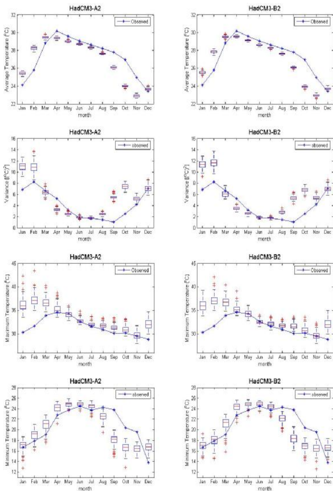
ภาพที่ ค.7 ค่าเฉลี่ย ค่าความแปรปรวน ค่าสูงสุด และค่าต่ำสุดของข้อมูลอุณหภูมิเฉลี่ยรายวันอดีต และของข้อมูลสังเคราะห์จากภาพฉาย HadCM3A2 และ HadCM3B2 สำหรับสถานี 405201 (ปี ค.ศ.1991-2001)
