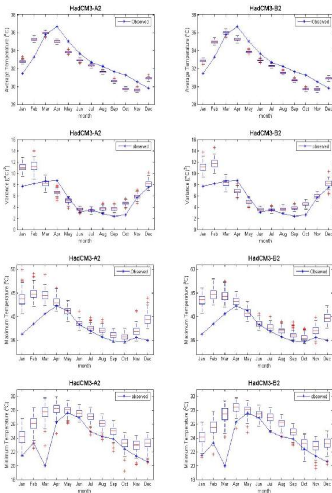
ภาพที่ ค.77 ค่าเฉลี่ย ค่าความแปรปรวน ค่าสูงสุด และค่าต่ำสุดของข้อมูลอุณหภูมิสูงสุดรายวันอดีต และของข้อมูลสังเคราะห์จากภาพฉาย HadCM3A2 และ HadCM3B2 สำหรับสถานี 432401 (ปี ค.ศ.1991-2001)
