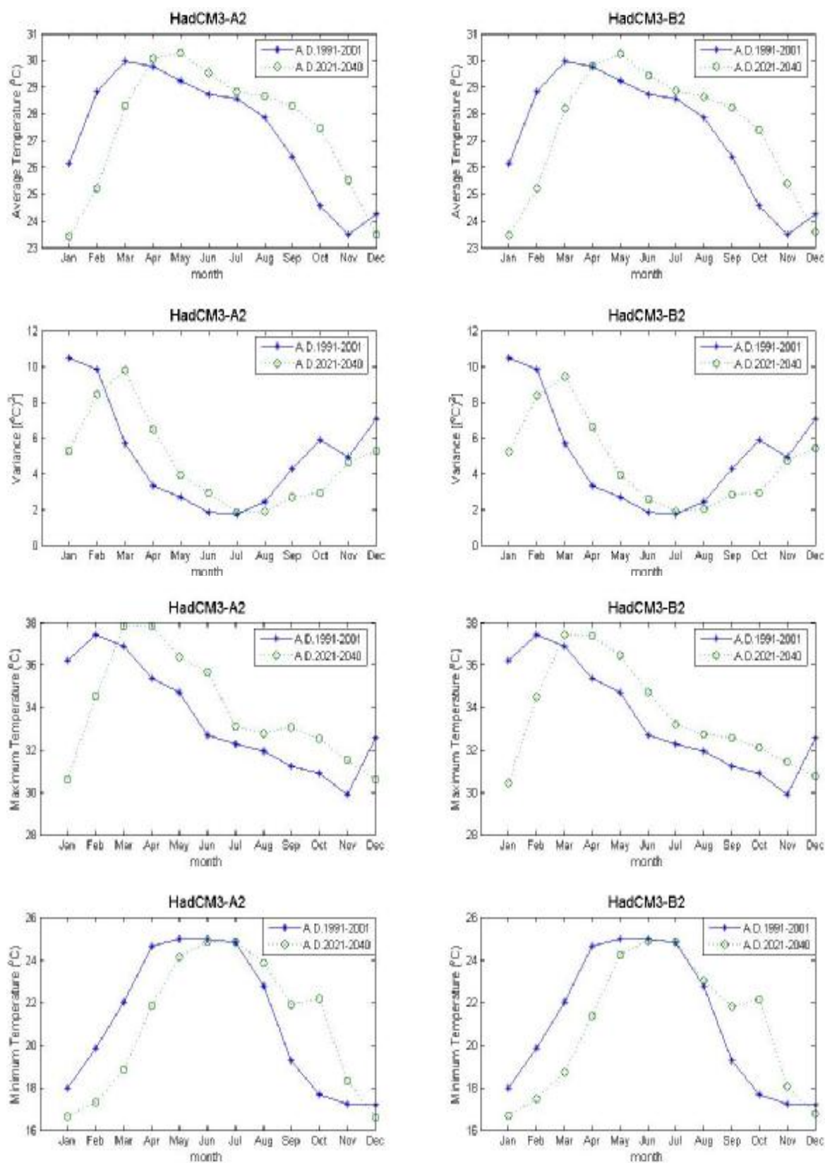
ภาพที่ ค.109 ค่าเฉลี่ย ค่าความแปรปรวน ค่าสูงสุด และค่าต่ำสุดของข้อมูลอุณหภูมิเฉลี่ยรายวันสังเคราะห์จาก ภาพฉาย HadCM3A2 และ HadCM3B2 สำหรับช่วงปี ค.ศ.1991-2001 และช่วงปี ค.ศ.2021-2040 (สถานี 432401)
