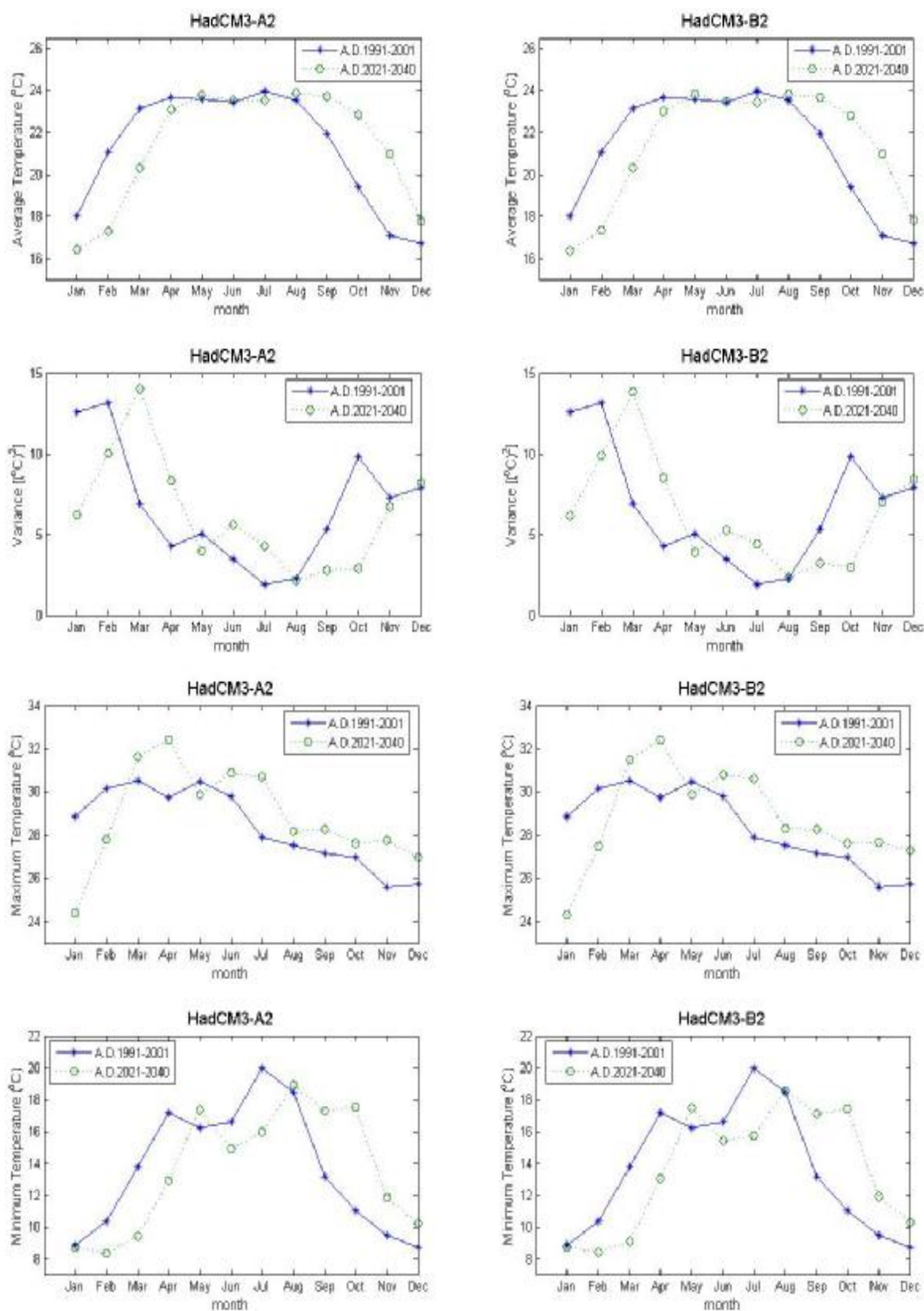
ภาพที่ ค.129 ค่าเฉลี่ย ค่าความแปรปรวน ค่าสูงสุด และค่าต่ำสุดของข้อมูลอุณหภูมิรายวันสังเคราะห์จาก ภาพฉาย HadCM3A2 และ HadCM3B2 สำหรับช่วงปี ค.ศ.1991-2001 และช่วงปี ค.ศ.2021-2040 (สถานี 407301)
