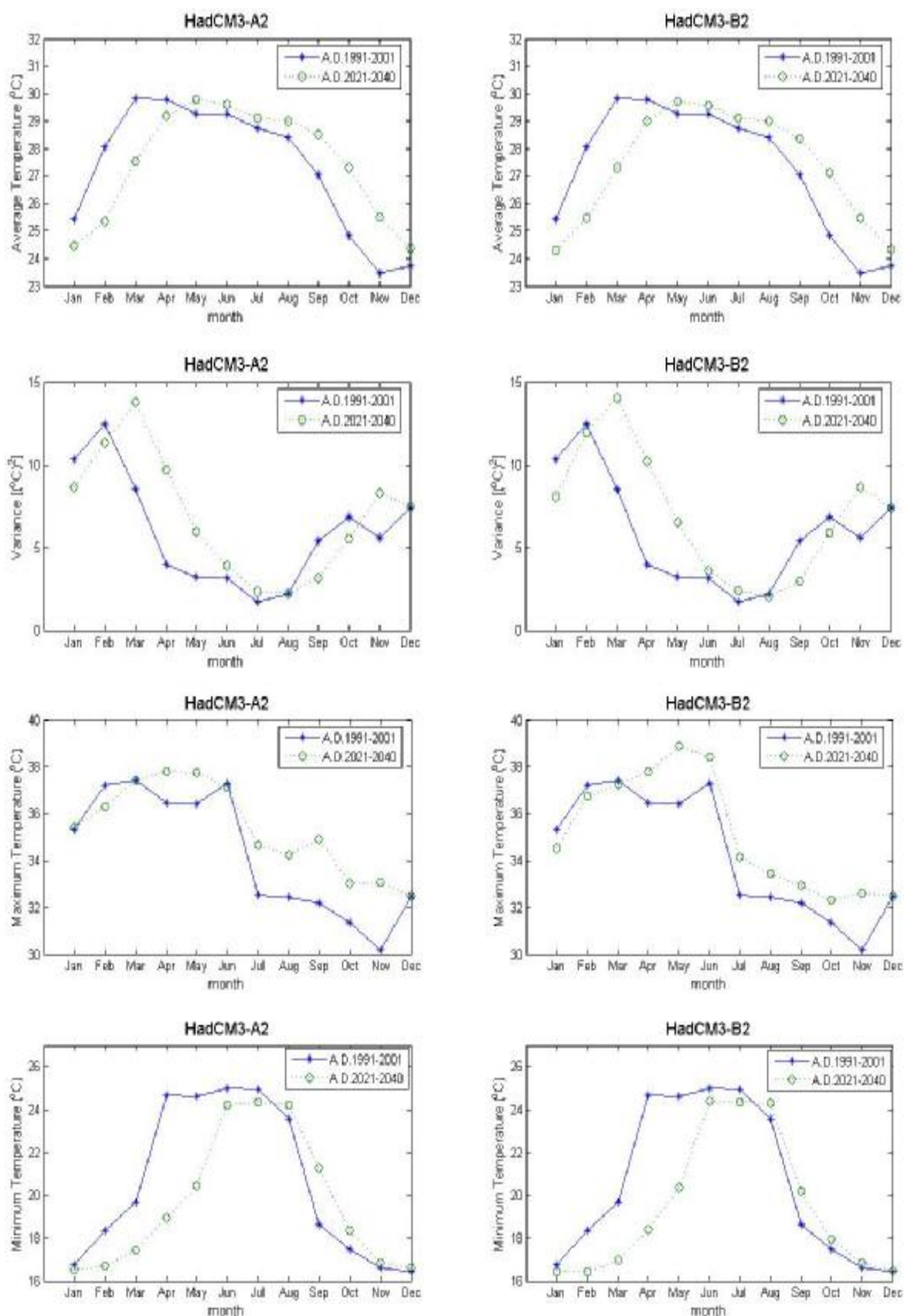
ภาพที่ ค.27 ค่าเฉลี่ย ค่าความแปรปรวน ค่าสูงสุด และค่าต่ำสุดของข้อมูลอุณหภูมิเฉลี่ยรายวันสังเคราะห์จากภาพฉาย HadCM3A2 และ HadCM3B2 สำหรับช่วงปี ค.ศ.1991-2001 และช่วงปี ค.ศ.2021-2040 (สถานี 387401)
