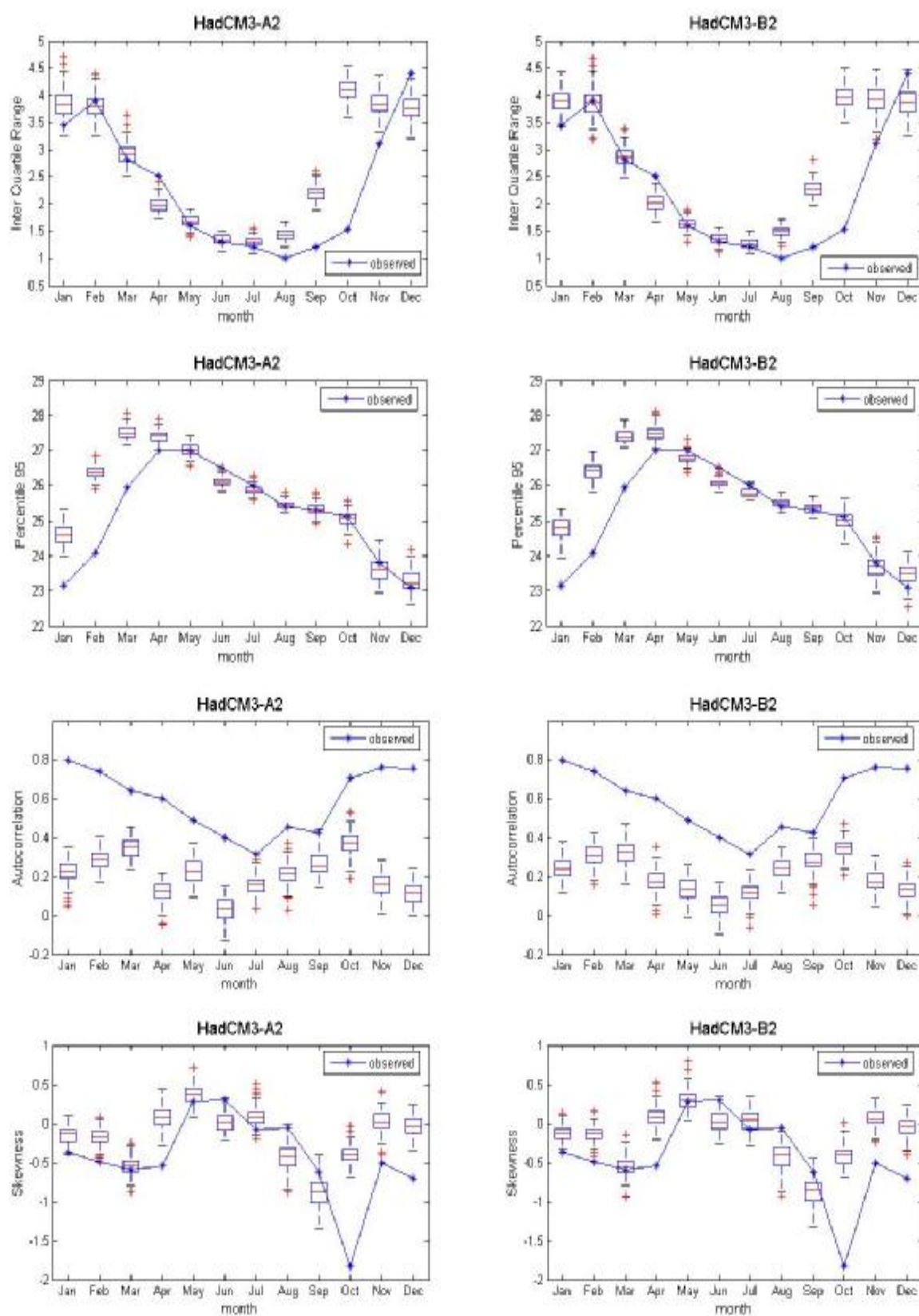
ภาพที่ ค.22 ค่าพิสัยระหว่างควอร์ไทล์ที่ 75 กับควอร์ไทล์ที่ 25 ค่าเปอร์เซ็นต์ไทล์ที่ 95 ค่าสัมประสิทธิ์สหสัมพันธ์ และค่าความเบ้ของข้อมูลอุณหภูมิต่ำสุดรายวันอดีต และของข้อมูลสังเคราะห์จากภาพฉาย HadCM3A2 และ HadCM3B2 สำหรับสถานี 403201 (ปี ค.ศ.1991-2001)
