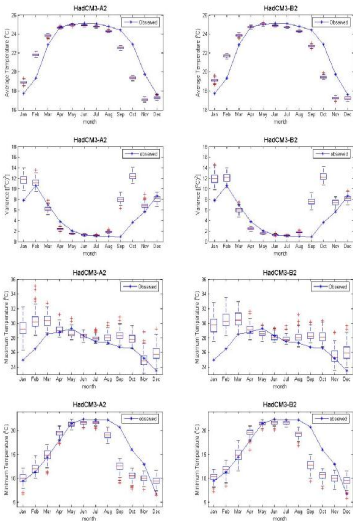
ภาพที่ ค.23 ค่าเฉลี่ย ค่าความแปรปรวน ค่าสูงสุด และค่าต่ำสุดของข้อมูลอุณหภูมิต่ำสุดรายวันอดีต และของข้อมูลสังเคราะห์จากภาพฉาย HadCM3A2 และ HadCM3B2 สำหรับสถานี 405201 (ปี ค.ศ.1991-2001)
