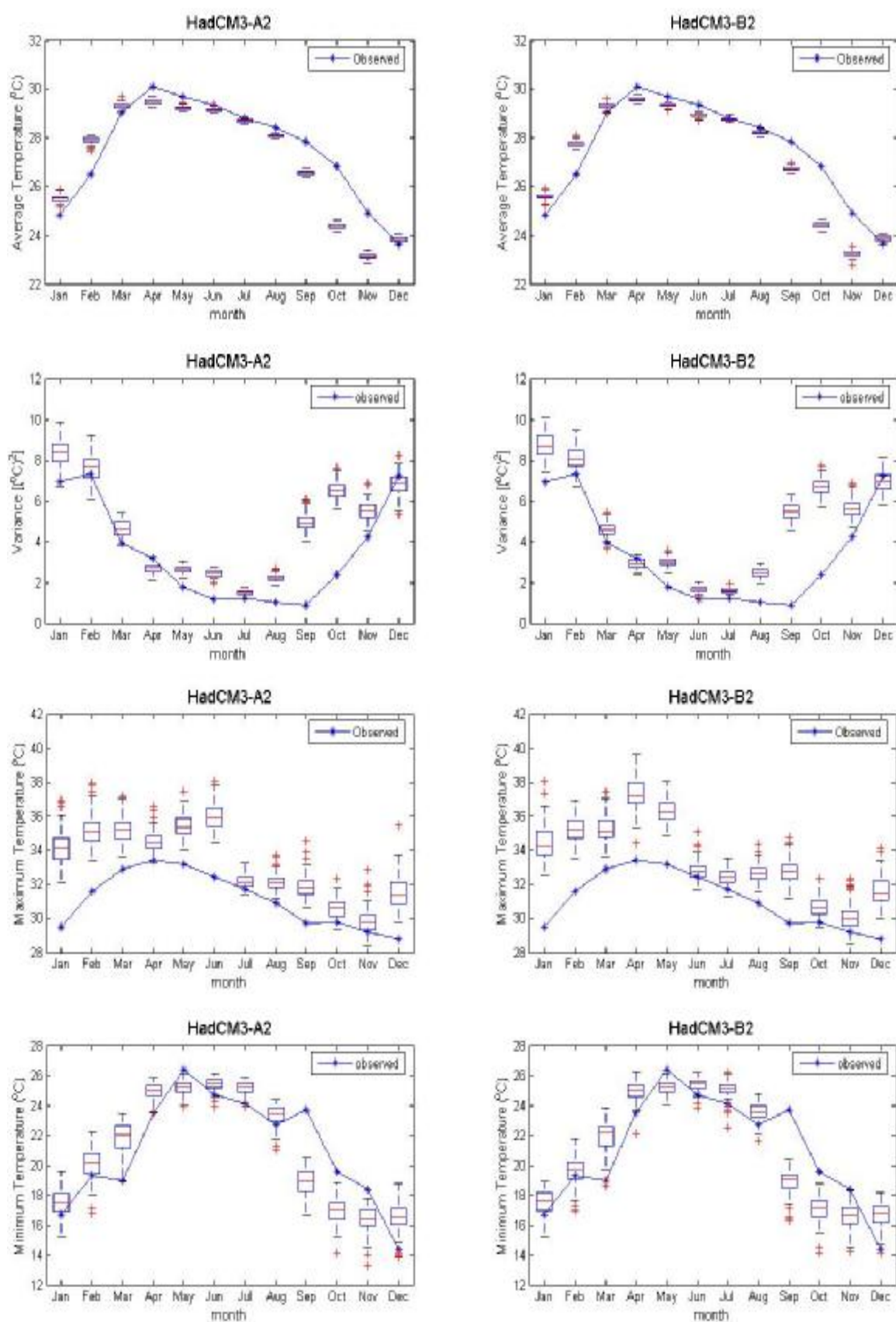
ภาพที่ ค.55 ค่าเฉลี่ย ค่าความแปรปรวน ค่าสูงสุด และค่าต่ำสุดของข้อมูลอุณหภูมิเฉลี่ยรายวันอดีต และของข้อมูลสังเคราะห์จากภาพฉาย HadCM3A2 และ HadCM3B2 สำหรับสถานี 431401 (ปี ค.ศ.1991-2001)
