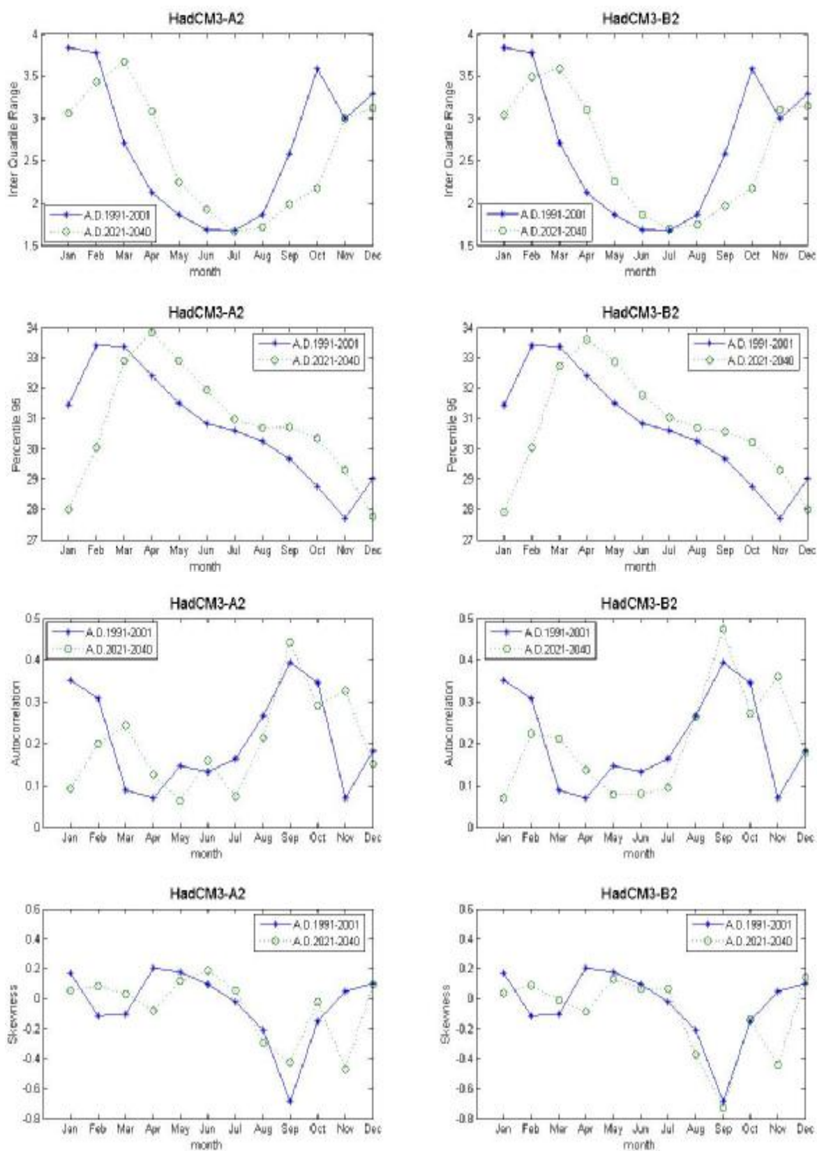
ภาพที่ ค.106 ค่าพิสัยระหว่างควอร์ไทล์ที่ 75 กับควอร์ไทล์ที่ 25 ค่าเปอร์เซ็นต์ไทล์ที่ 95 ค่าสัมประสิทธิ์สหสัมพันธ์ และค่าสัมประสิทธิ์ความเบ้ของข้อมูลอุณหภูมิเฉลี่ยรายวันสังเคราะห์จากภาพฉาย HadCM3A2 และ HadCM3B2 สำหรับช่วงปี ค.ศ.1991-2001 และช่วงปี ค.ศ.2021-2040 (สถานี 432201)
