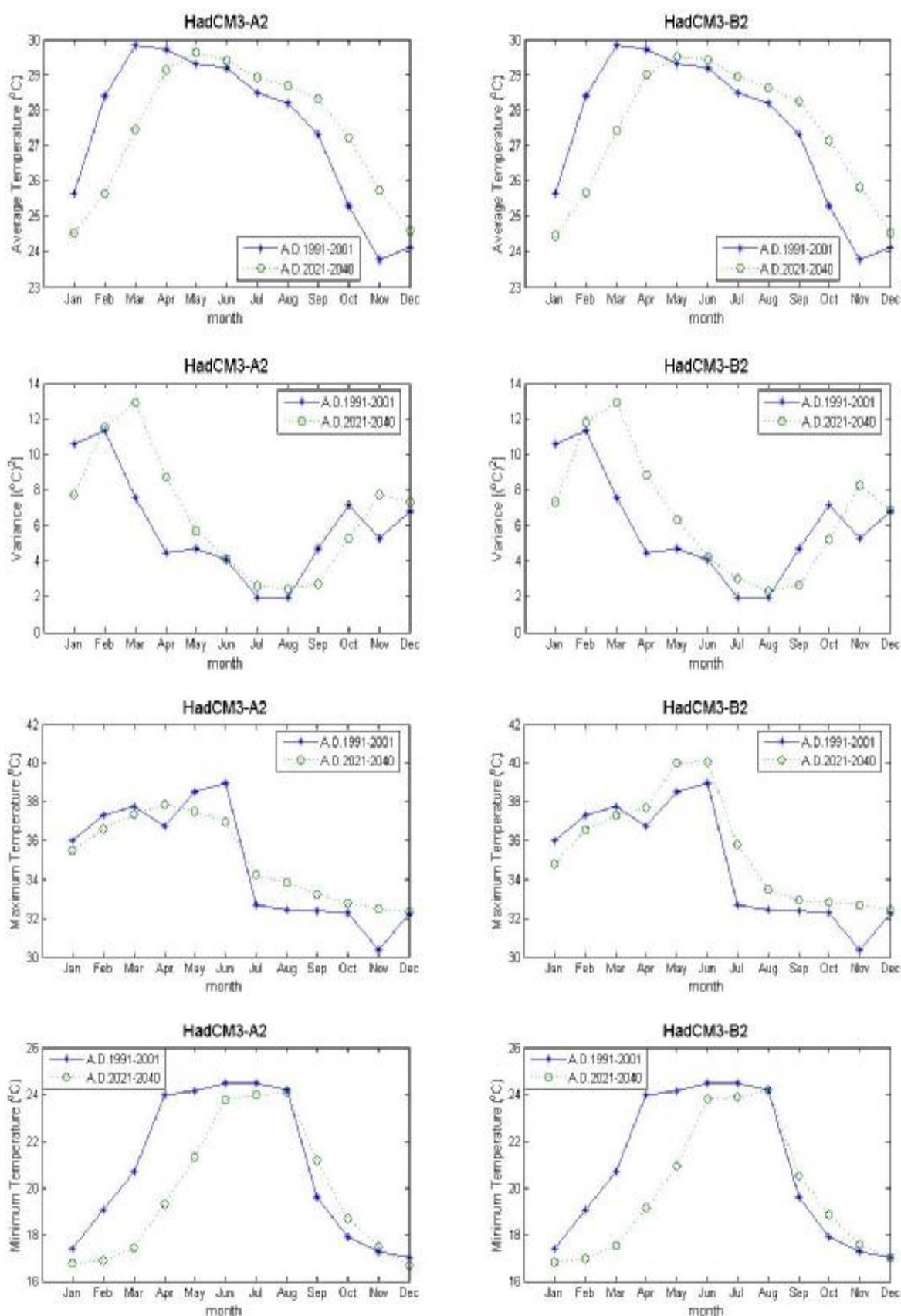
ภาพที่ ค.25 ค่าเฉลี่ย ค่าความแปรปรวน ค่าสูงสุด และค่าต่ำสุดของข้อมูลอุณหภูมิเฉลี่ยรายวันสังเคราะห์จากภาพฉาย HadCM3A2 และ HadCM3B2 สำหรับช่วงปี ค.ศ.1991-2001 และช่วงปี ค.ศ.2021-2040 (สถานี 381201)
