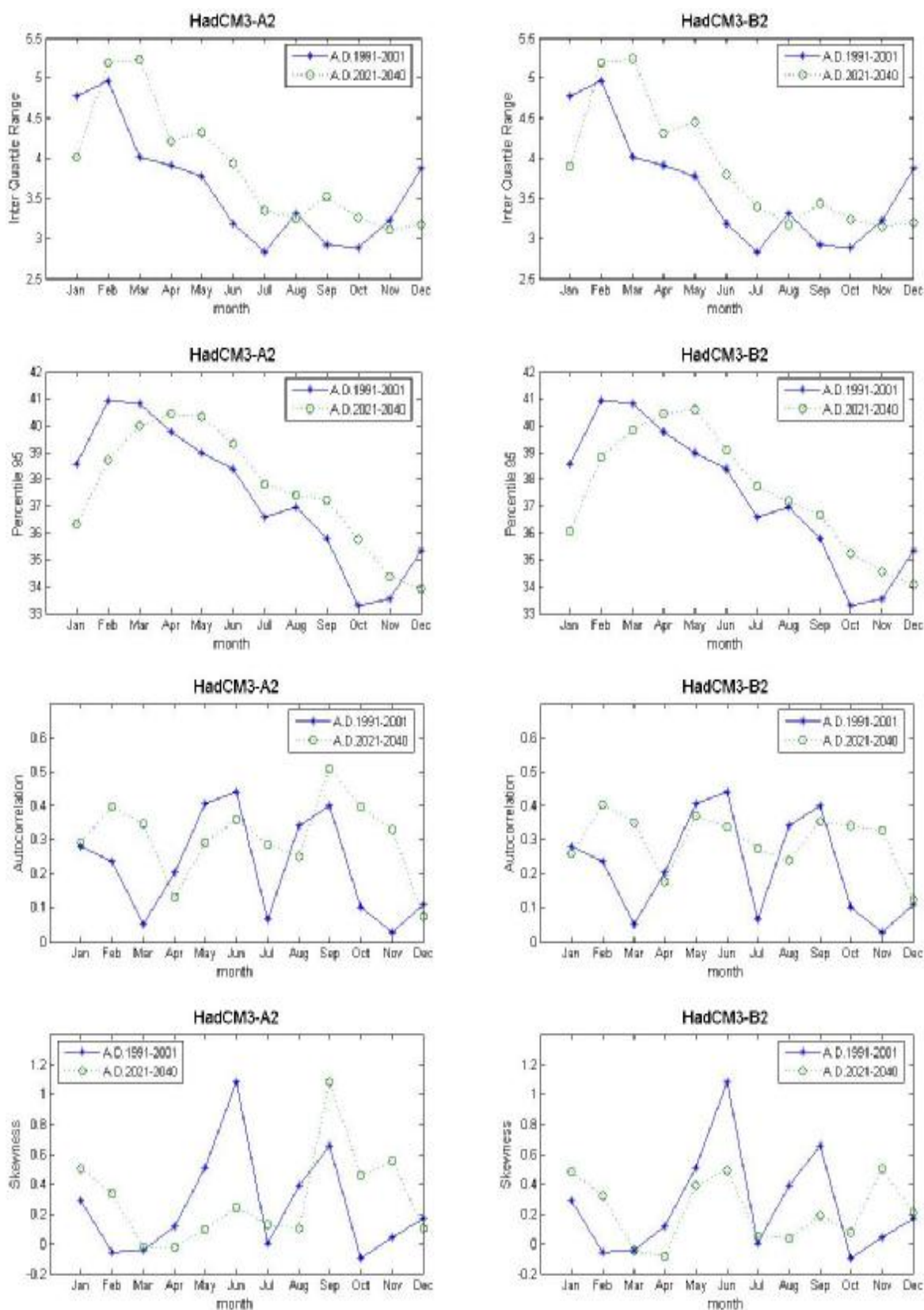
ภาพที่ ค.38 ค่าพิสัยระหว่างควอร์ไทล์ที่ 75 กับควอร์ไทล์ที่ 25 ค่าเปอร์เซ็นต์ไทล์ที่ 95 ค่าสัมประสิทธิ์สหสัมพันธ์ และ ค่าความเบ้ของข้อมูลอุณหภูมิสูงสุดรายวันสังเคราะห์จากภาพฉาย HadCM3A2 และ HadCM3B2 สำหรับช่วงปี ค.ศ.1991-2001 และช่วงปี ค.ศ.2021-2040 (สถานี 403201)
