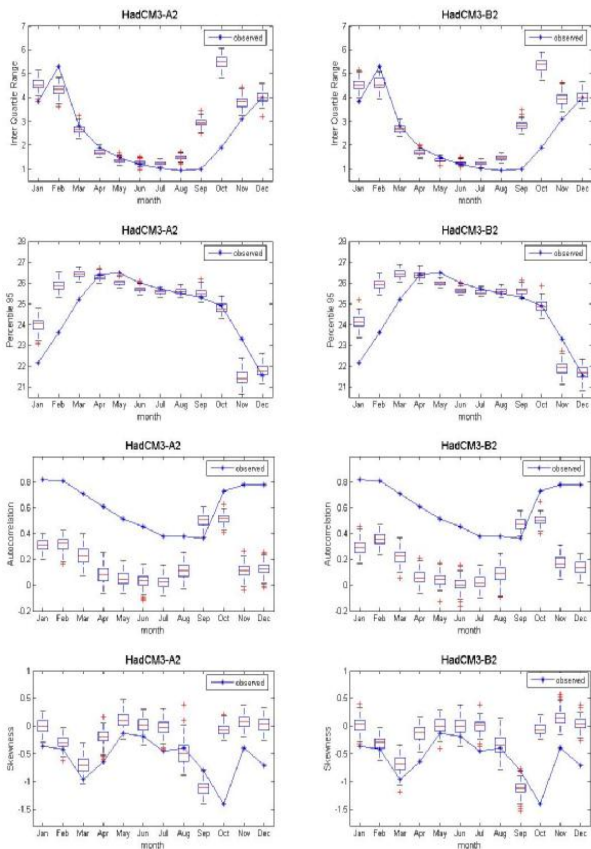
ภาพที่ ค.92 ค่าพิสัยระหว่างควอร์ไทล์ที่ 75 กับควอร์ไทล์ที่ 25 ค่าเปอร์เซ็นต์ไทล์ที่ 95 ค่าสัมประสิทธิ์สหสัมพันธ์ และค่าความเบ้ของข้อมูลอุณหภูมิต่ำสุดรายวันอดีต และของข้อมูลสังเคราะห์จากภาพฉาย HadCM3A2 และ HadCM3B2 สำหรับสถานี 432301 (ปี ค.ศ.1991-2001)
