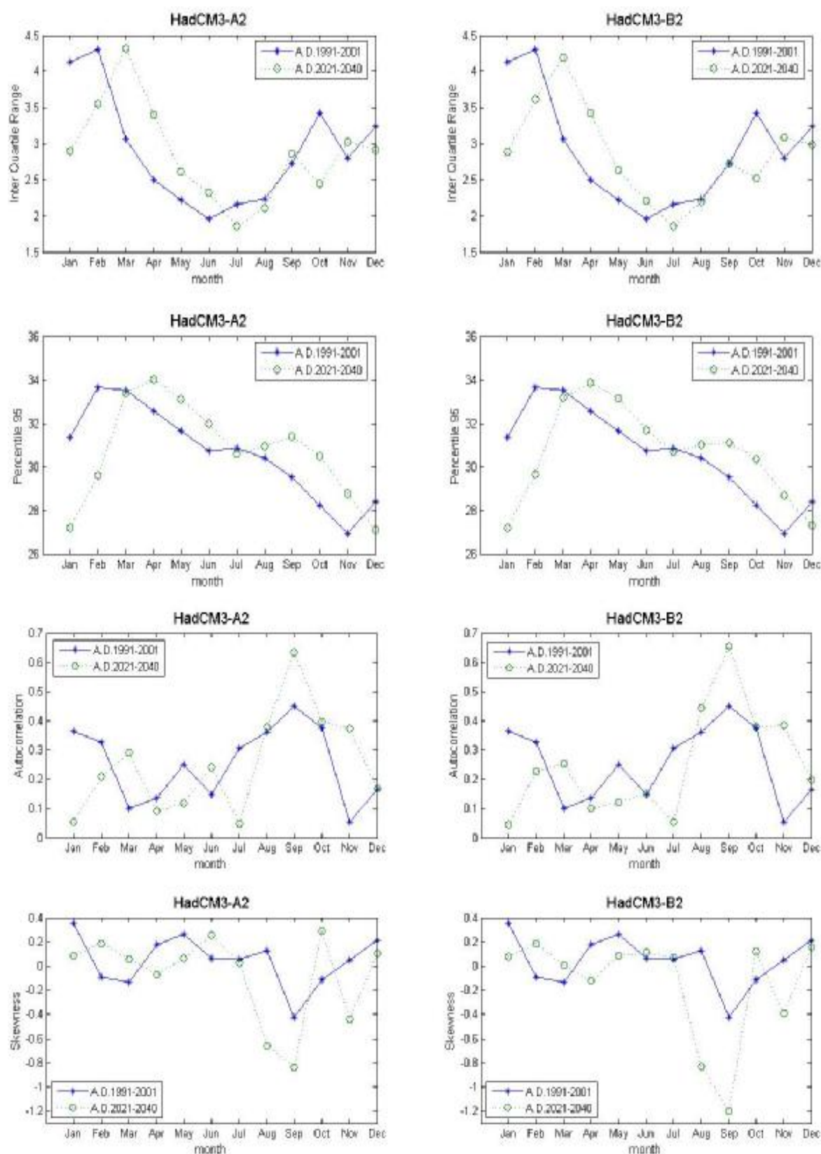
ภาพที่ ค.100 ค่าพิสัยระหว่างควอร์ไทล์ที่ 75 กับควอร์ไทล์ที่ 25 ค่าเปอร์เซ็นต์ไทล์ที่ 95 ค่าสัมประสิทธิ์สหสัมพันธ์ และค่าสัมประสิทธิ์ความเบ้ของข้อมูลอุณหภูมิเฉลี่ยรายวันสังเคราะห์จากภาพฉาย HadCM3A2 และ HadCM3B2 สำหรับช่วงปี ค.ศ.1991-2001 และช่วงปี ค.ศ.2021-2040 (สถานี 407501)
