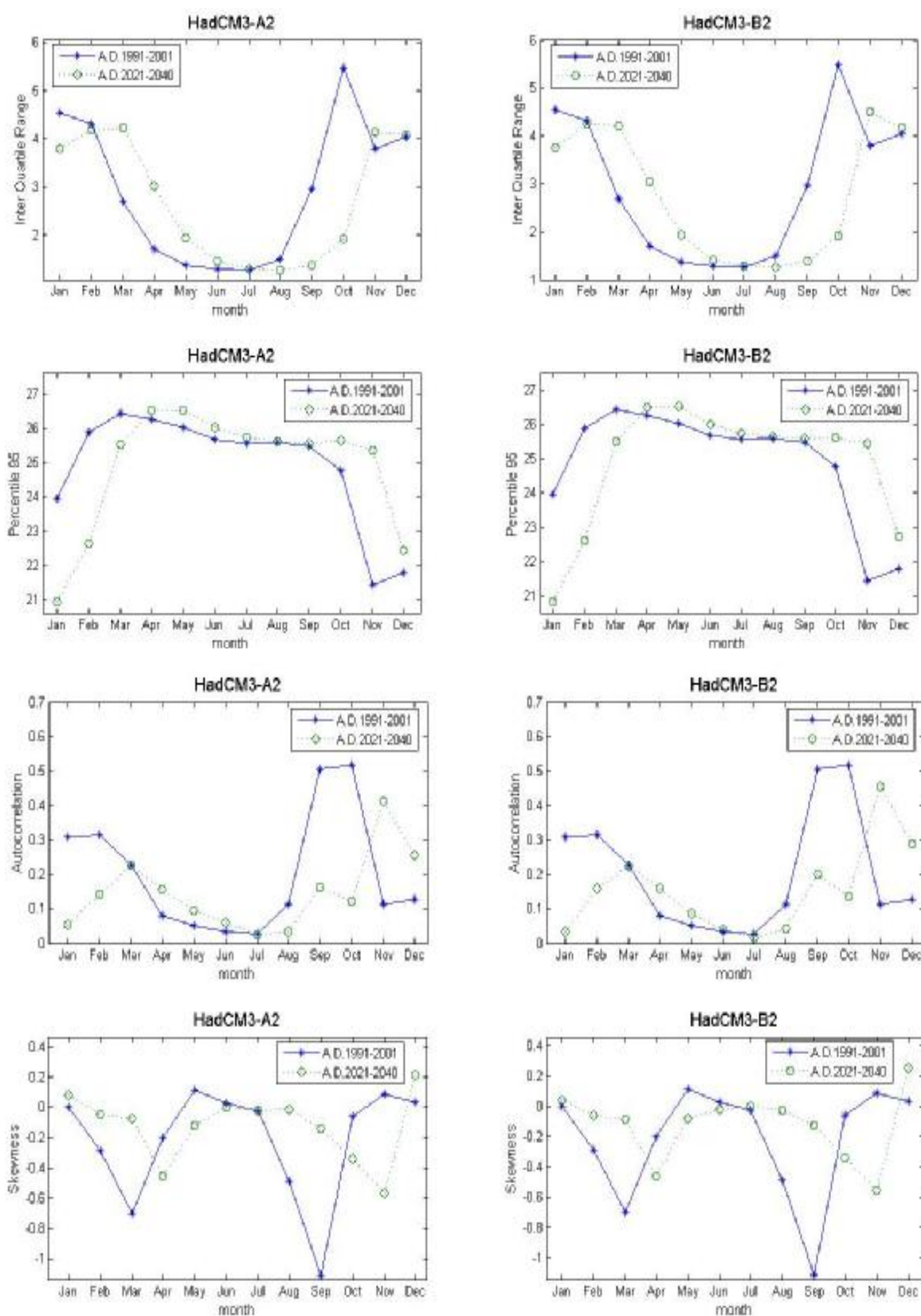
ภาพที่ ค.140 ค่าพิสัยระหว่างควอร์ไทล์ที่ 75 กับควอร์ไทล์ที่ 25 ค่าเปอร์เซ็นต์ไทล์ที่ 95 ค่าสัมประสิทธิ์สหสัมพันธ์ และค่าสัมประสิทธิ์ความเบ้ของข้อมูลอุณหภูมิต่ำสุดรายวันสังเคราะห์จากภาพฉาย HadCM3A2 และ HadCM3B2 สำหรับช่วงปี ค.ศ.1991-2001 และช่วงปี ค.ศ.2021-2040 (สถานี 432301)
