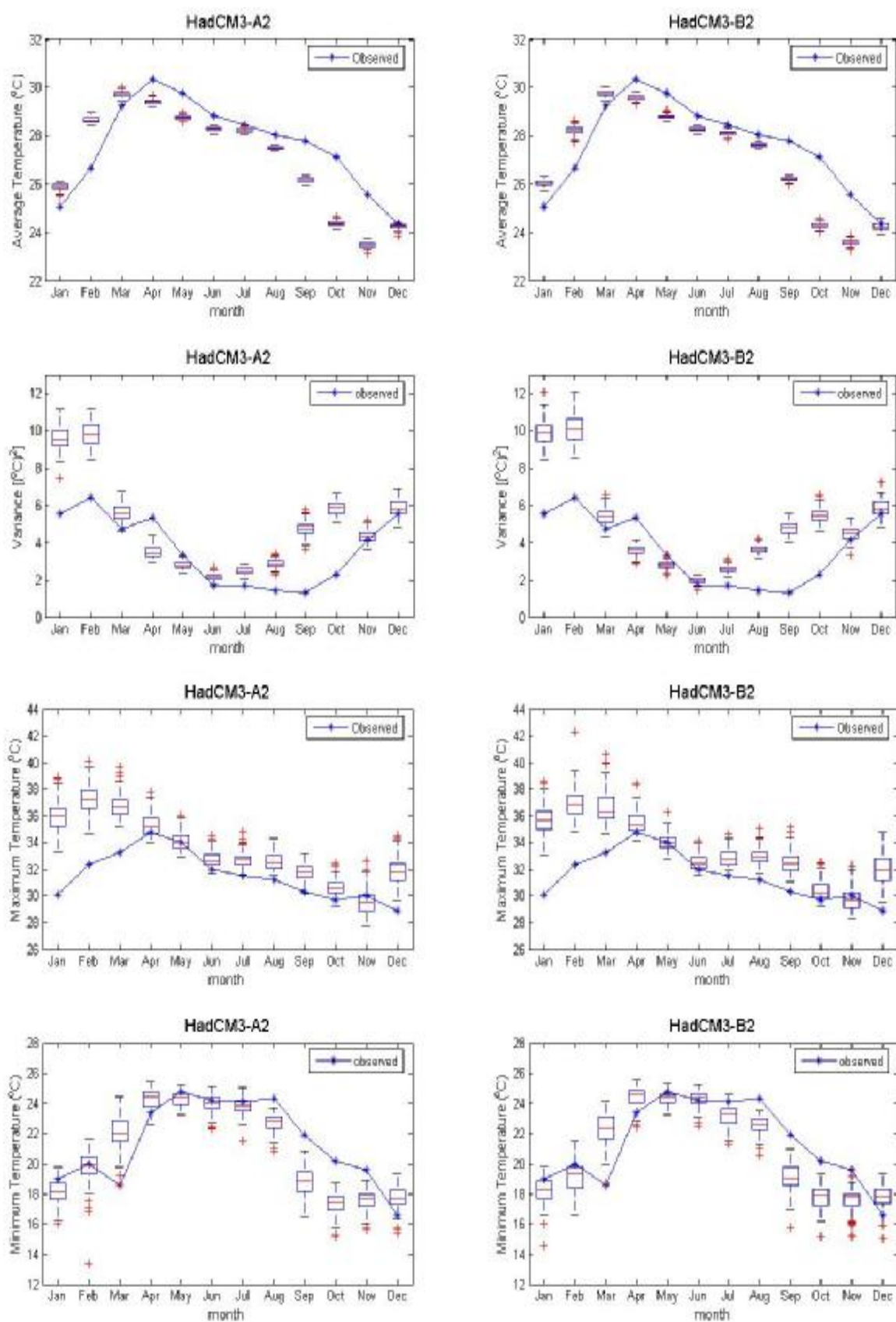
ภาพที่ ค.51 ค่าเฉลี่ย ค่าความแปรปรวน ค่าสูงสุด และค่าต่ำสุดของข้อมูลอุณหภูมิเฉลี่ยรายวันอดีต และของข้อมูลสังเคราะห์จากภาพฉาย HadCM3A2 และ HadCM3B2 สำหรับสถานี 407501 (ปี ค.ศ.1991-2001)
