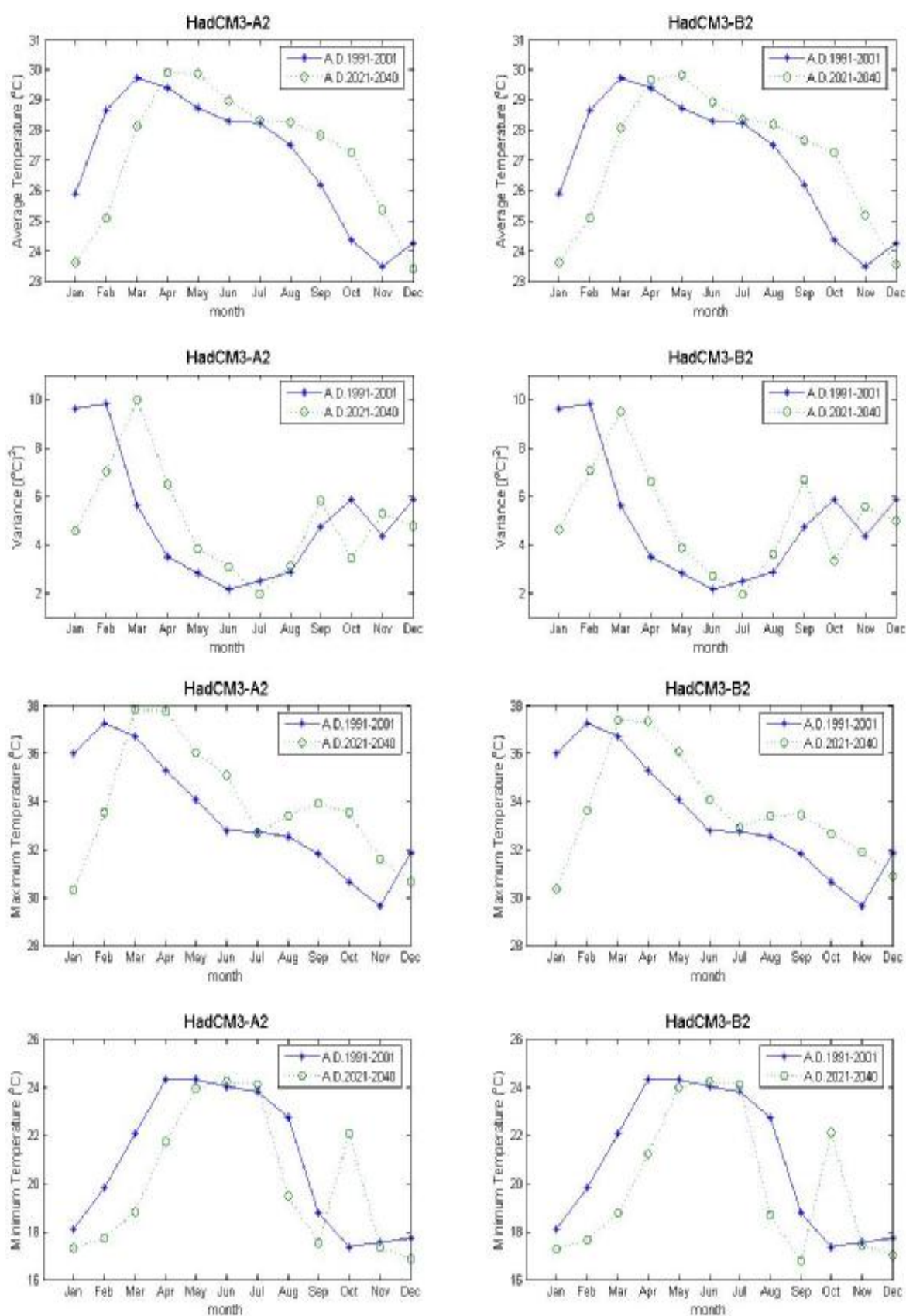
ภาพที่ ค.99 ค่าเฉลี่ย ค่าความแปรปรวน ค่าสูงสุด และค่าต่ำสุดของข้อมูลอุณหภูมิเฉลี่ยรายวันสังเคราะห์จากภาพฉาย HadCM3A2 และ HadCM3B2 สำหรับช่วงปี ค.ศ.1991-2001 และช่วงปี ค.ศ.2021-2040 (สถานี 407501)
