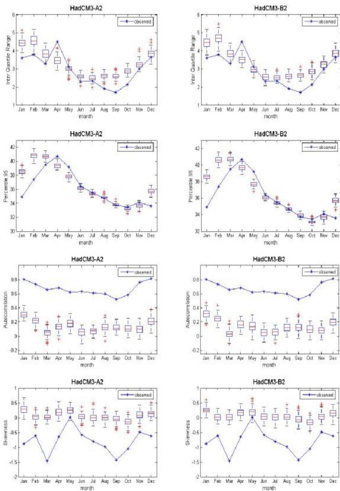
ภาพที่ ค.78 ค่าพิสัยระหว่างควอร์ไทล์ที่ 75 กับควอร์ไทล์ที่ 25 ค่าเปอร์เซ็นต์ไทล์ที่ 95 ค่าสัมประสิทธิ์สหสัมพันธ์ และค่าความเบ้ของข้อมูลอุณหภูมิสูงสุดรายวันอดีต และของข้อมูลสังเคราะห์จากภาพฉาย HadCM3A2 และ HadCM3B2 สำหรับสถานี 432401 (ปี ค.ศ.1991-2001)
