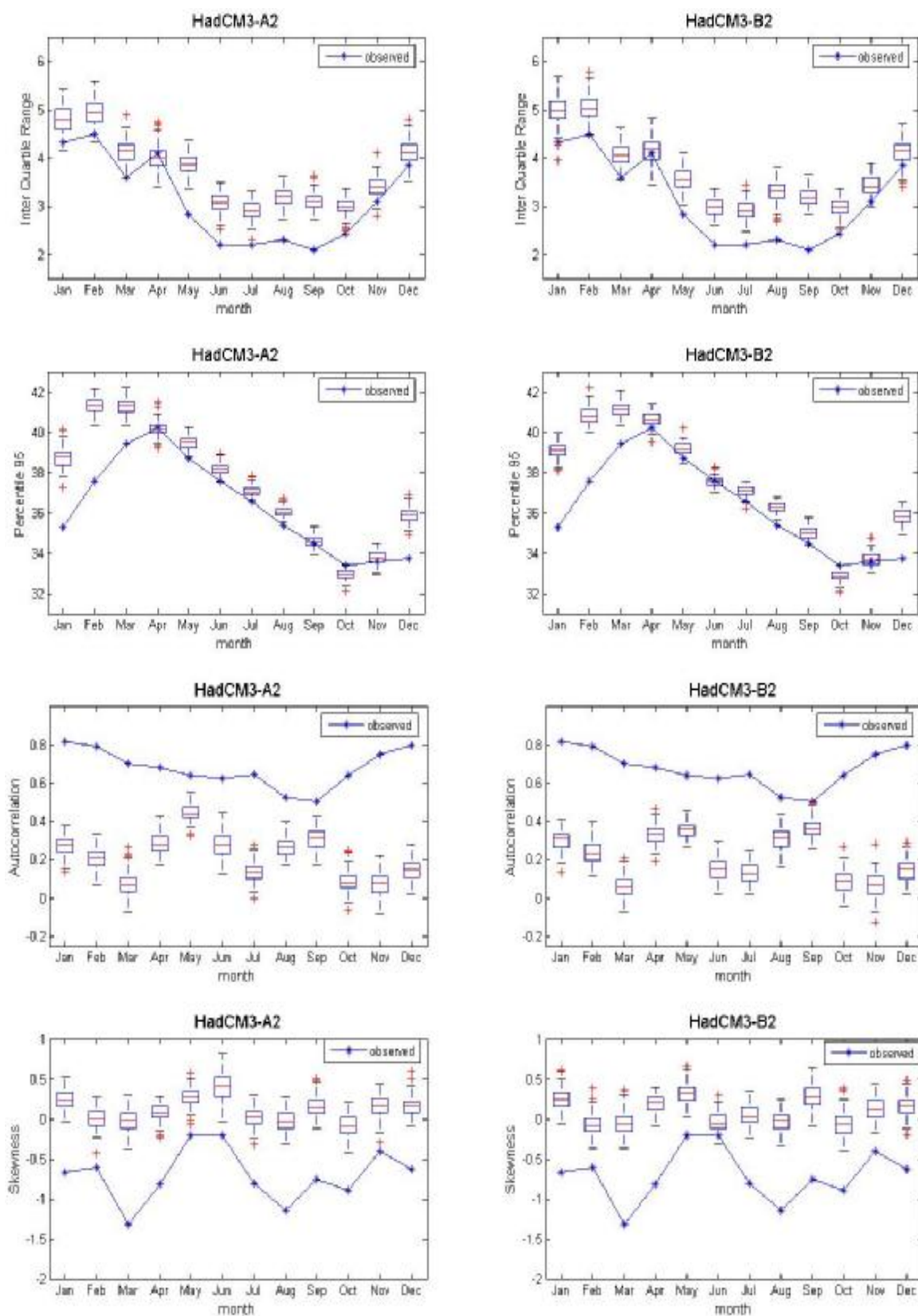
ภาพที่ ค.68 ค่าพิสัยระหว่างควอร์ไทล์ที่ 75 กับควอร์ไทล์ที่ 25 ค่าเปอร์เซ็นต์ไทล์ที่ 95 ค่าสัมประสิทธิ์สหสัมพันธ์ และค่าความเบ้ของข้อมูลอุณหภูมิสูงสุดรายวันอดีต และของข้อมูลสังเคราะห์จากภาพฉาย HadCM3A2 และ HadCM3B2 สำหรับสถานี 431201 (ปี ค.ศ.1991-2001)
