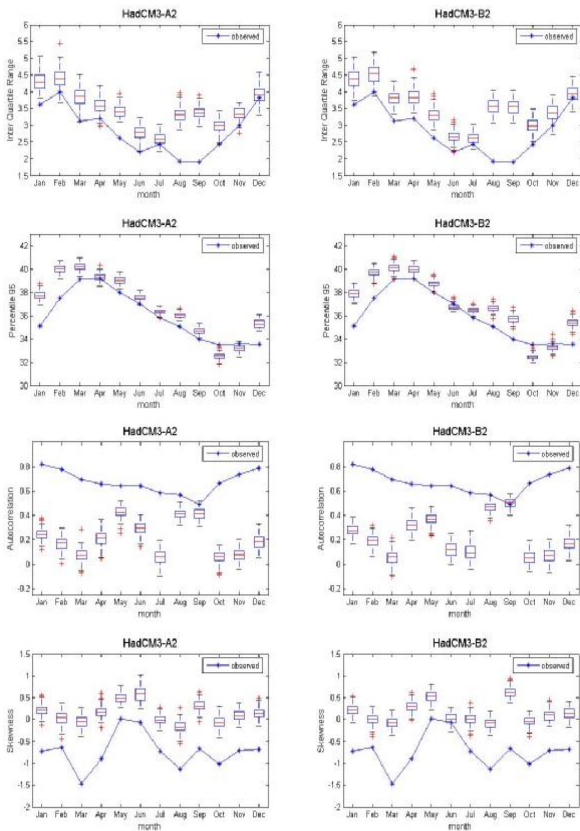
ภาพที่ ค.72 ค่าพิสัยระหว่างควอร์ไทล์ที่ 75 กับควอร์ไทล์ที่ 25 ค่าเปอร์เซ็นต์ไทล์ที่ 95 ค่าสัมประสิทธิ์สหสัมพันธ์ และ ค่าความเบ้ของข้อมูลอุณหภูมิสูงสุดรายวันอดีต และของข้อมูลสังเคราะห์จากภาพฉาย HadCM3A2 และ HadCM3B2 สำหรับสถานี 431401 (ปี ค.ศ.1991-2001)
