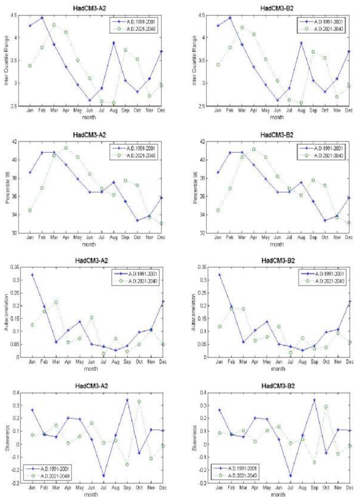
ภาพที่ ค.124 ค่าพิสัยระหว่างควอร์ไทล์ที่ 75 กับควอร์ไทล์ที่ 25 ค่าเปอร์เซ็นต์ไทล์ที่ 95 ค่าสัมประสิทธิ์สหสัมพันธ์ และค่าสัมประสิทธิ์ความเบ้ของข้อมูลอุณหภูมิสูงสุดรายวันสังเคราะห์จากภาพฉาย HadCM3A2 และ HadCM3B2 สำหรับช่วงปี ค.ศ.1991-2001 และช่วงปี ค.ศ.2021-2040 (สถานี 432301)
