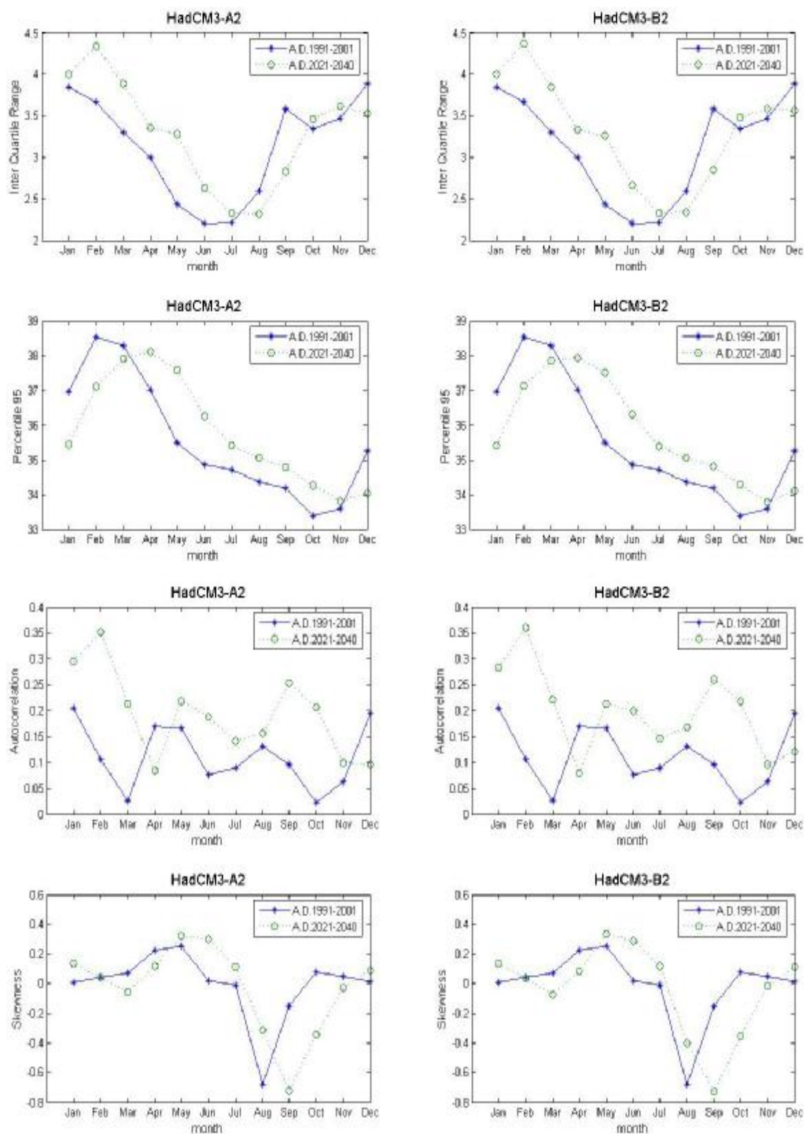
ภาพที่ ค.118 ค่าพิสัยระหว่างควอร์ไทล์ที่ 75 กับควอร์ไทล์ที่ 25 ค่าเปอร์เซ็นต์ไทล์ที่ 95 ค่าสัมประสิทธิ์สหสัมพันธ์ และค่าสัมประสิทธิ์ความเบ้ของข้อมูลอุณหภูมิสูงสุดรายวันสังเคราะห์จากภาพฉาย HadCM3A2 และ HadCM3B2 สำหรับช่วงปี ค.ศ.1991-2001 และช่วงปี ค.ศ.2021-2040 (สถานี 431301)
