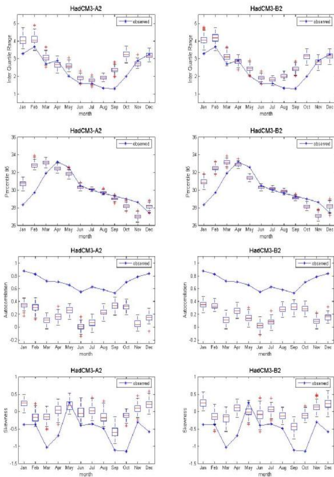
ภาพที่ ค.50 ค่าพิสัยระหว่างควอร์ไทล์ที่ 75 กับควอร์ไทล์ที่ 25 ค่าเปอร์เซ็นต์ไทล์ที่ 95 ค่าสัมประสิทธิ์สหสัมพันธ์ และ ค่าความเบ้ของข้อมูลอุณหภูมิเฉลี่ยรายวันอดีต และของข้อมูลสังเคราะห์จากภาพฉาย HadCM3A2 และ HadCM3B2 สำหรับสถานี 407301 (ปี ค.ศ.1991-2001)
