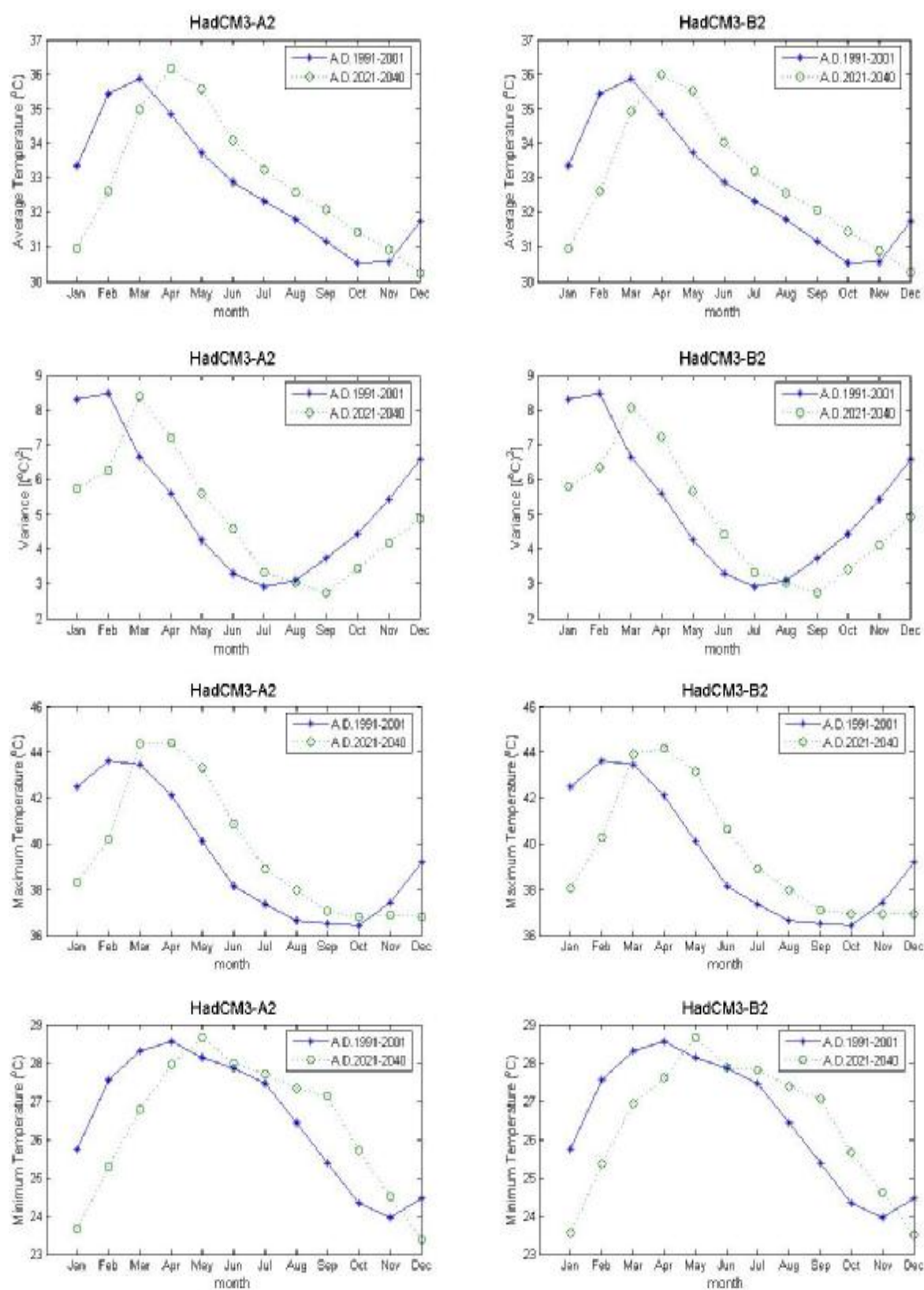
ภาพที่ ค.121 ค่าเฉลี่ย ค่าความแปรปรวน ค่าสูงสุด และค่าต่ำสุดของข้อมูลอุณหภูมิสูงสุดรายวันสังเคราะห์จาก ภาพฉาย HadCM3A2 และ HadCM3B2 สำหรับช่วงปี ค.ศ.1991-2001 และช่วงปี ค.ศ.2021-2040 (สถานี 432201)
