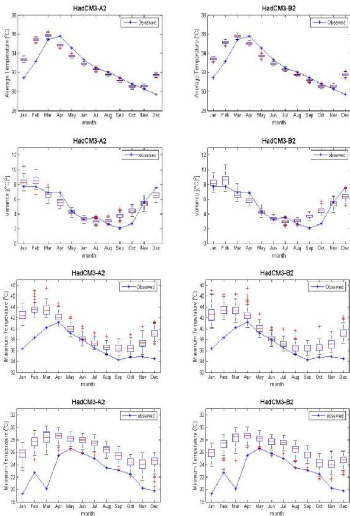
ภาพที่ ค.73 ค่าเฉลี่ย ค่าความแปรปรวน ค่าสูงสุด และค่าต่ำสุดของข้อมูลอุณหภูมิสูงสุดรายวันอดีต และของข้อมูลสังเคราะห์จากภาพฉาย HadCM3A2 และ HadCM3B2 สำหรับสถานี 432201 (ปี ค.ศ.1991-2001)
