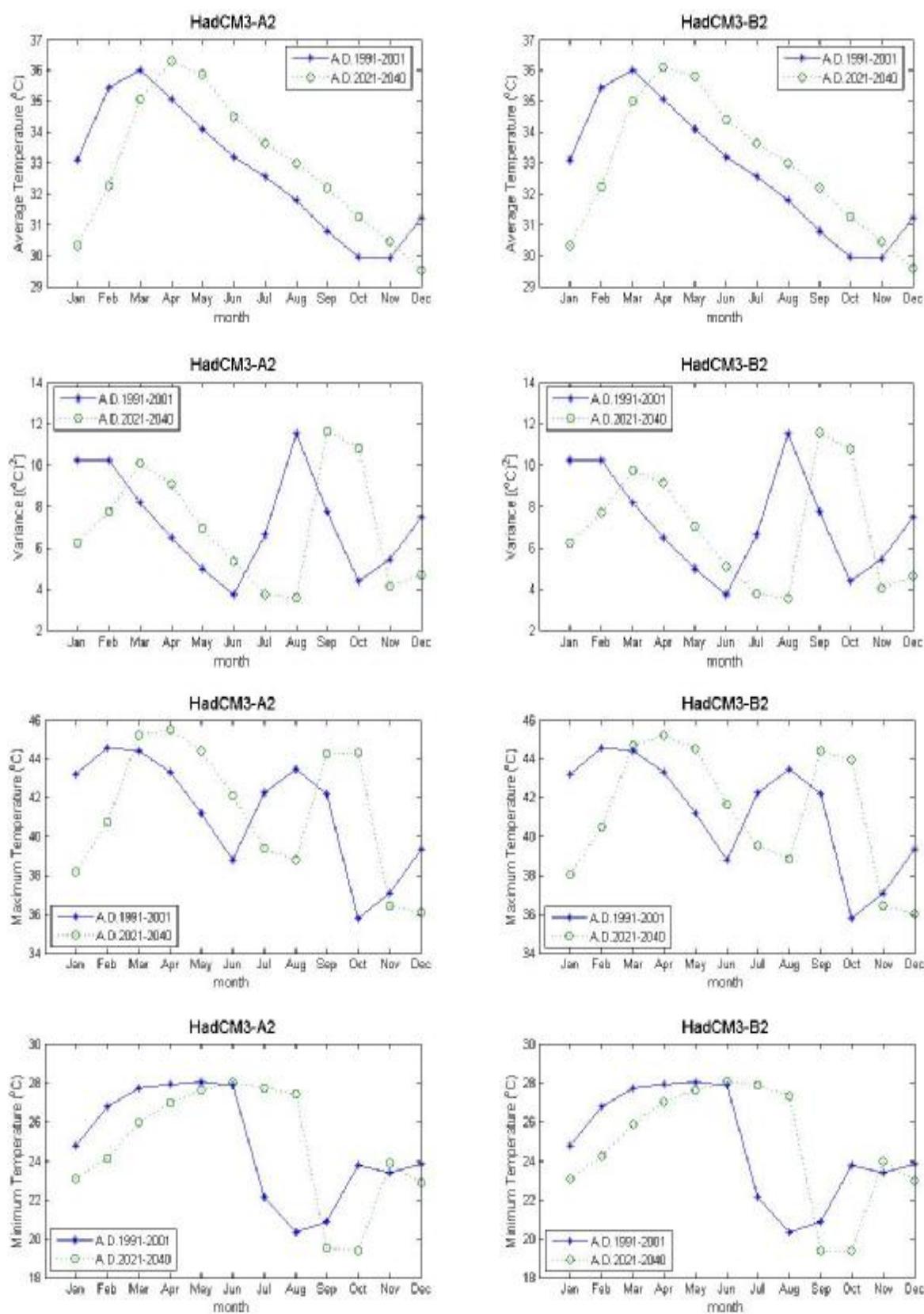
ภาพที่ ค.123 ค่าเฉลี่ย ค่าความแปรปรวน ค่าสูงสุด และค่าต่ำสุดของข้อมูลอุณหภูมิสูงสุดรายวันสังเคราะห์จาก ภาพฉาย HadCM3A2 และ HadCM3B2 สำหรับช่วงปี ค.ศ.1991-2001 และช่วงปี ค.ศ.2021-2040 (สถานี 432301)
