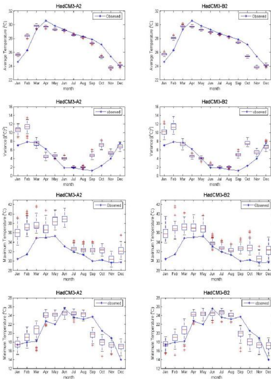
ภาพที่ ค.1 ค่าเฉลี่ย ค่าความแปรปรวน ค่าสูงสุด และค่าต่ำสุดของข้อมูลอุณหภูมิเฉลี่ยรายวันอดีต และของข้อมูลสังเคราะห์จากภาพฉาย HadCM3A2 และ HadCM3B2 สำหรับสถานี 381201 (ปี ค.ศ.1991-2001)
