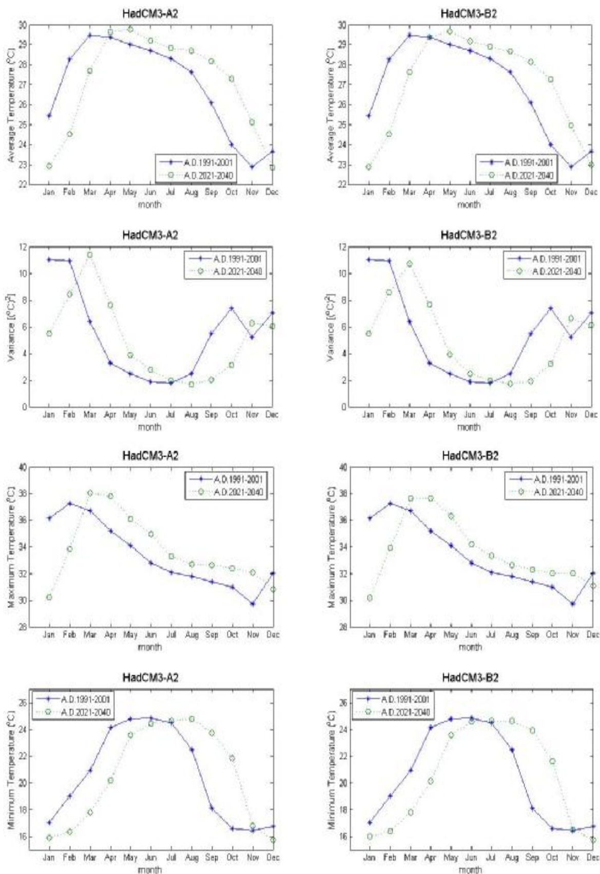
ภาพที่ ค.31 ค่าเฉลี่ย ค่าความแปรปรวน ค่าสูงสุด และค่าต่ำสุดของข้อมูลอุณหภูมิเฉลี่ยรายวันสังเคราะห์จากภาพฉาย HadCM3A2 และ HadCM3B2 สำหรับช่วงปี ค.ศ.1991-2001 และช่วงปี ค.ศ.2021-2040 (สถานี 405201)
