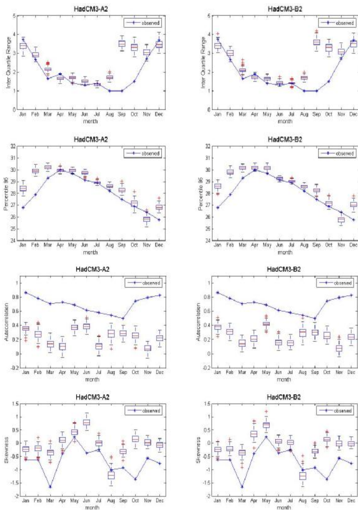
ภาพที่ ค.54 ค่าพิสัยระหว่างควอร์ไทล์ที่ 75 กับควอร์ไทล์ที่ 25 ค่าเปอร์เซ็นไทล์ที่ 95 ค่าสัมประสิทธิ์สหสัมพันธ์ และค่าความเบ้ของข้อมูลอุณหภูมิเฉลี่ยรายวันอดีต และของข้อมูลสังเคราะห์จากภาพฉาย HadCM3A2 และ HadCM3B2 สำหรับสถานี 431301 (ปี ค.ศ.1991-2001)
