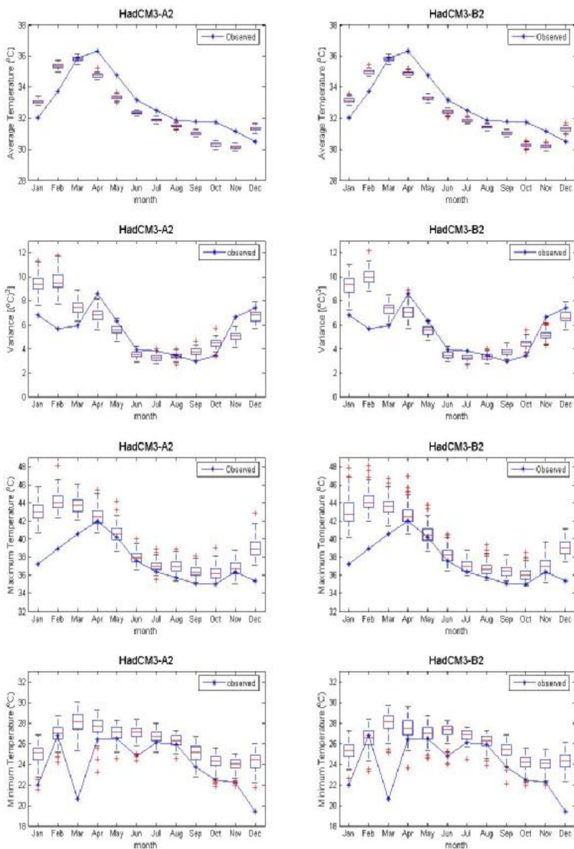
ภาพที่ ค.65 ค่าเฉลี่ย ค่าความแปรปรวน ค่าสูงสุด และค่าต่ำสุดของข้อมูลอุณหภูมิสูงสุดรายวันอดีต และของข้อมูลสังเคราะห์จากภาพฉาย HadCM3A2 และ HadCM3B2 สำหรับสถานี 407501 (ปี ค.ศ.1991-2001)
