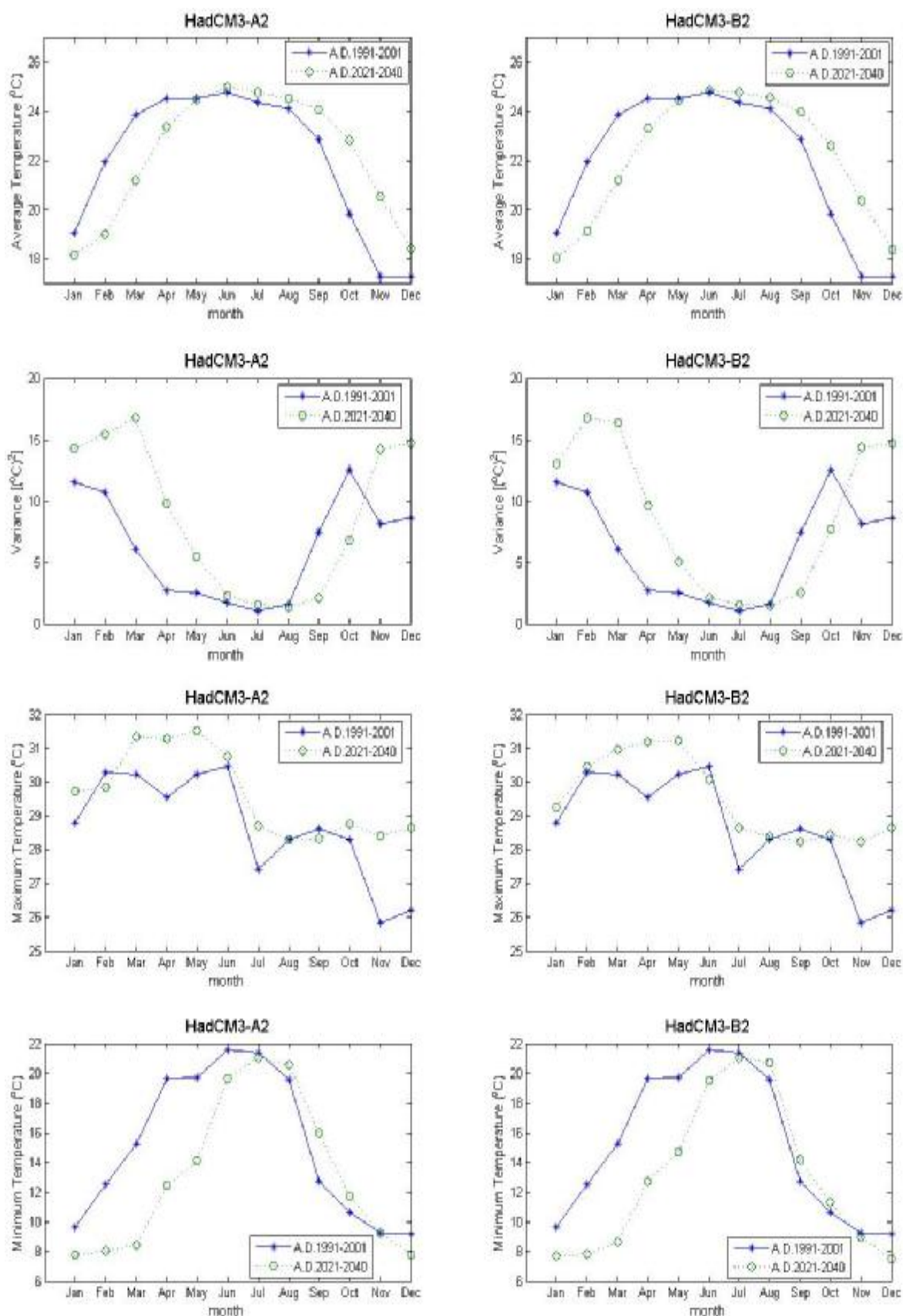
ภาพที่ ค.43 ค่าเฉลี่ย ค่าความแปรปรวน ค่าสูงสุด และค่าต่ำสุดของข้อมูลอุณหภูมิรายวันสังเคราะห์จากภาพฉาย HadCM3A2 และ HadCM3B2 สำหรับช่วงปี ค.ศ.1991-2001 และช่วงปี ค.ศ.2021-2040 (สถานี 381301)
