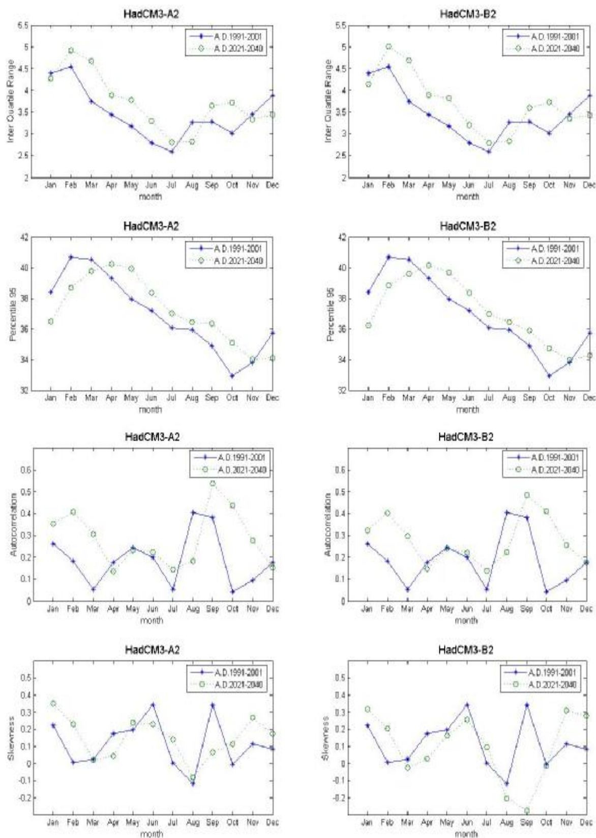
ภาพที่ ค.128 ค่าพิสัยระหว่างควอร์ไทล์ที่ 75 กับควอร์ไทล์ที่ 25 ค่าเปอร์เซ็นต์ไทล์ที่ 95 ค่าสัมประสิทธิ์สหสัมพันธ์ และค่าสัมประสิทธิ์ความเบ้ของข้อมูลอุณหภูมิสูงสุดรายวันสังเคราะห์จากภาพฉาย HadCM3A2 และ HadCM3B2 สำหรับช่วงปี ค.ศ.1991-2001 และช่วงปี ค.ศ.2021-2040 (สถานี 436401)
