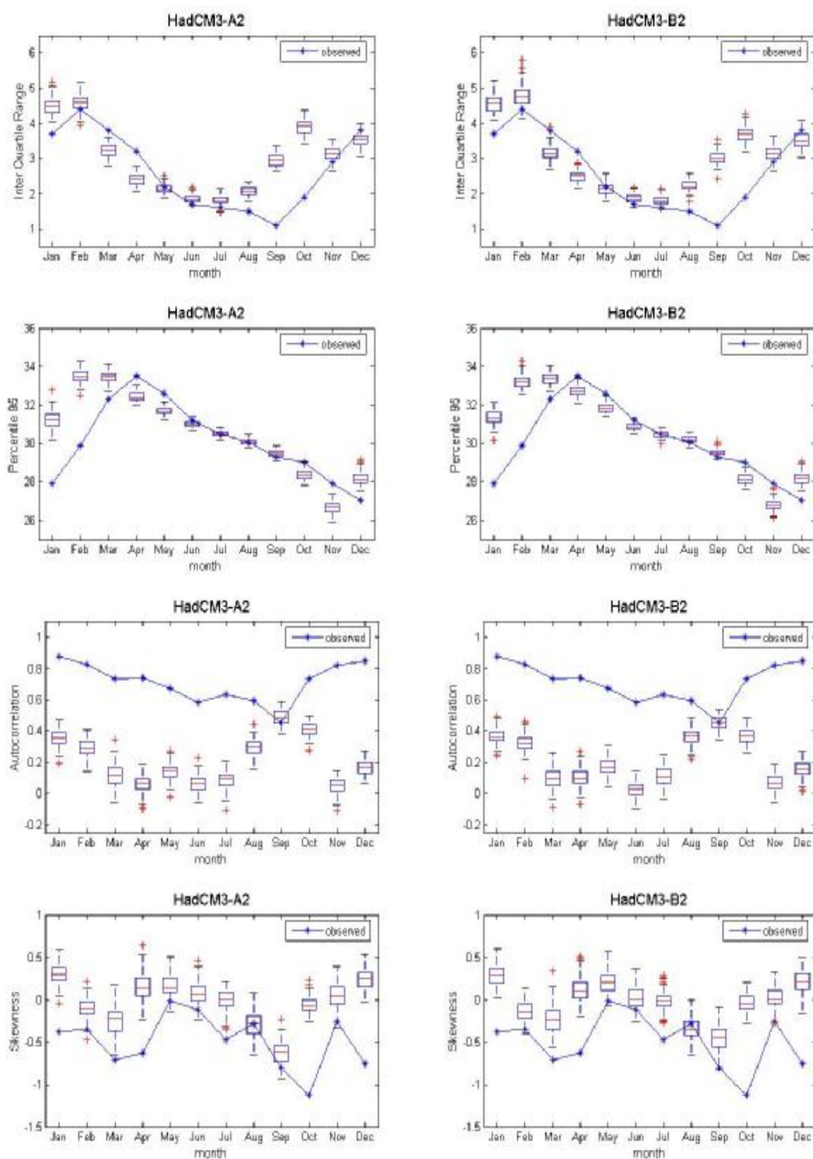
ภาพที่ ค.8 ค่าพิสัยระหว่างควอร์ไทล์ที่ 75 กับควอร์ไทล์ที่ 25 ค่าเปอร์เซ็นต์ไทล์ที่ 95 ค่าสัมประสิทธิ์สหสัมพันธ์ และ ค่าความเบ้ของข้อมูลอุณหภูมิเฉลี่ยรายวันอดีต และของข้อมูลสังเคราะห์จากภาพฉาย HadCM3A2 และ HadCM3B2 สำหรับสถานี 405201 (ปี ค.ศ.1991-2001)
