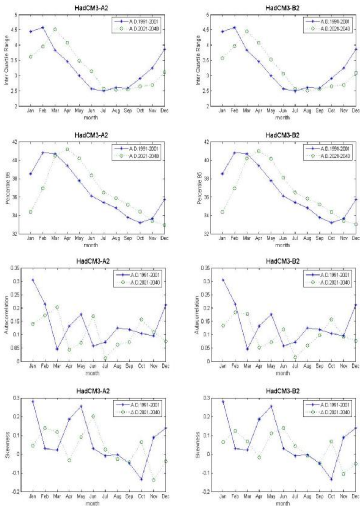
ภาพที่ ค.126 ค่าพิสัยระหว่างควอร์ไทล์ที่ 75 กับควอร์ไทล์ที่ 25 ค่าเปอร์เซ็นต์ไทล์ที่ 95 ค่าสัมประสิทธิ์สหสัมพันธ์ และค่าสัมประสิทธิ์ความเบ้ของข้อมูลอุณหภูมิสูงสุดรายวันสังเคราะห์จากภาพฉาย HadCM3A2 และ HadCM3B2 สำหรับช่วงปี ค.ศ.1991-2001 และช่วงปี ค.ศ.2021-2040 (สถานี 432401)
