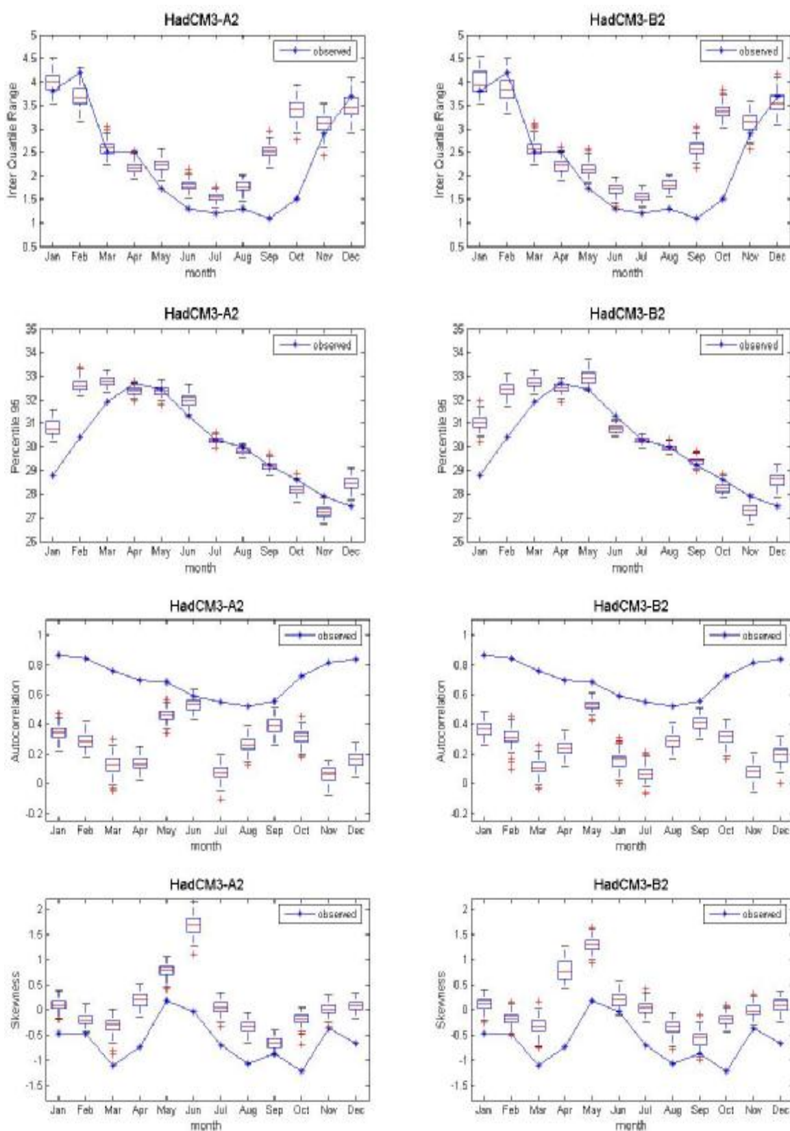
ภาพที่ ค.64 ค่าพิสัยระหว่างควอร์ไทล์ที่ 75 กับควอร์ไทล์ที่ 25 ค่าเปอร์เซ็นต์ไทล์ที่ 95 ค่าสัมประสิทธิ์สหสัมพันธ์ และค่าความเบ้ของข้อมูลอุณหภูมิเฉลี่ยรายวันอดีต และของข้อมูลสังเคราะห์จากภาพฉาย HadCM3A2 และ HadCM3B2 สำหรับสถานี 436401 (ปี ค.ศ.1991-2001)
