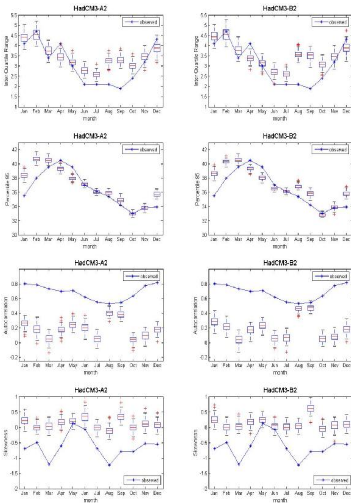
ภาพที่ ค.80 ค่าพิสัยระหว่างควอร์ไทล์ที่ 75 กับควอร์ไทล์ที่ 25 ค่าเปอร์เซ็นต์ไทล์ที่ 95 ค่าสัมประสิทธิ์สหสัมพันธ์ และค่าความเบ้ของข้อมูลอุณหภูมิสูงสุดรายวันอดีต และของข้อมูลสังเคราะห์จากภาพฉาย HadCM3A2 และ HadCM3B2 สำหรับสถานี 436401 (ปี ค.ศ.1991-2001)
