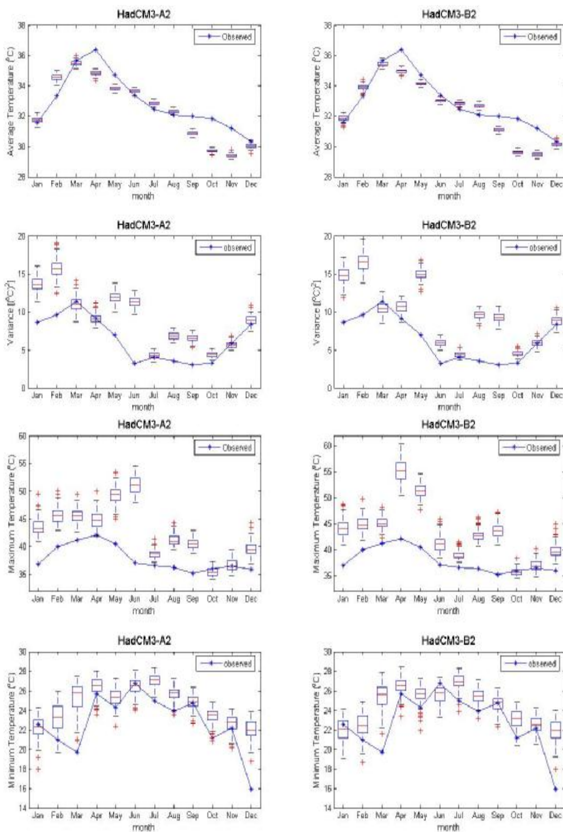
ภาพที่ ค.9 ค่าเฉลี่ย ค่าความแปรปรวน ค่าสูงสุด และค่าต่ำสุดของข้อมูลอุณหภูมิสูงสุดรายวันอดีต และของข้อมูลสังเคราะห์จากภาพฉาย HadCM3A2 และ HadCM3B2 สำหรับสถานี 381301 (ปี ค.ศ.1991-2001)
