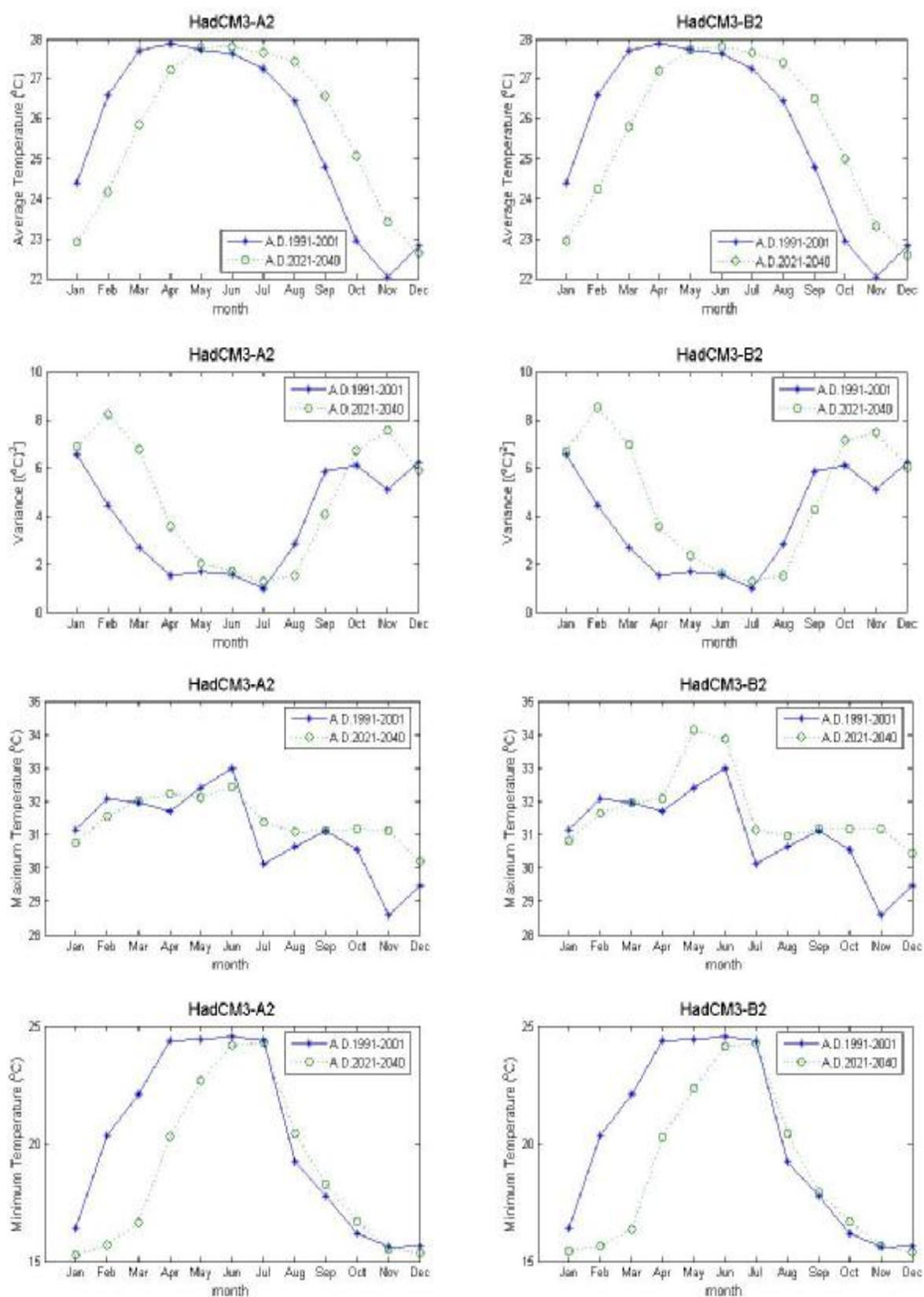
ภาพที่ ค.101 ค่าเฉลี่ย ค่าความแปรปรวน ค่าสูงสุด และค่าต่ำสุดของข้อมูลอุณหภูมิเฉลี่ยรายวันสังเคราะห์จาก ภาพฉาย HadCM3A2 และ HadCM3B2 สำหรับช่วงปี ค.ศ.1991-2001 และช่วงปี ค.ศ.2021-2040 (สถานี 431301)
