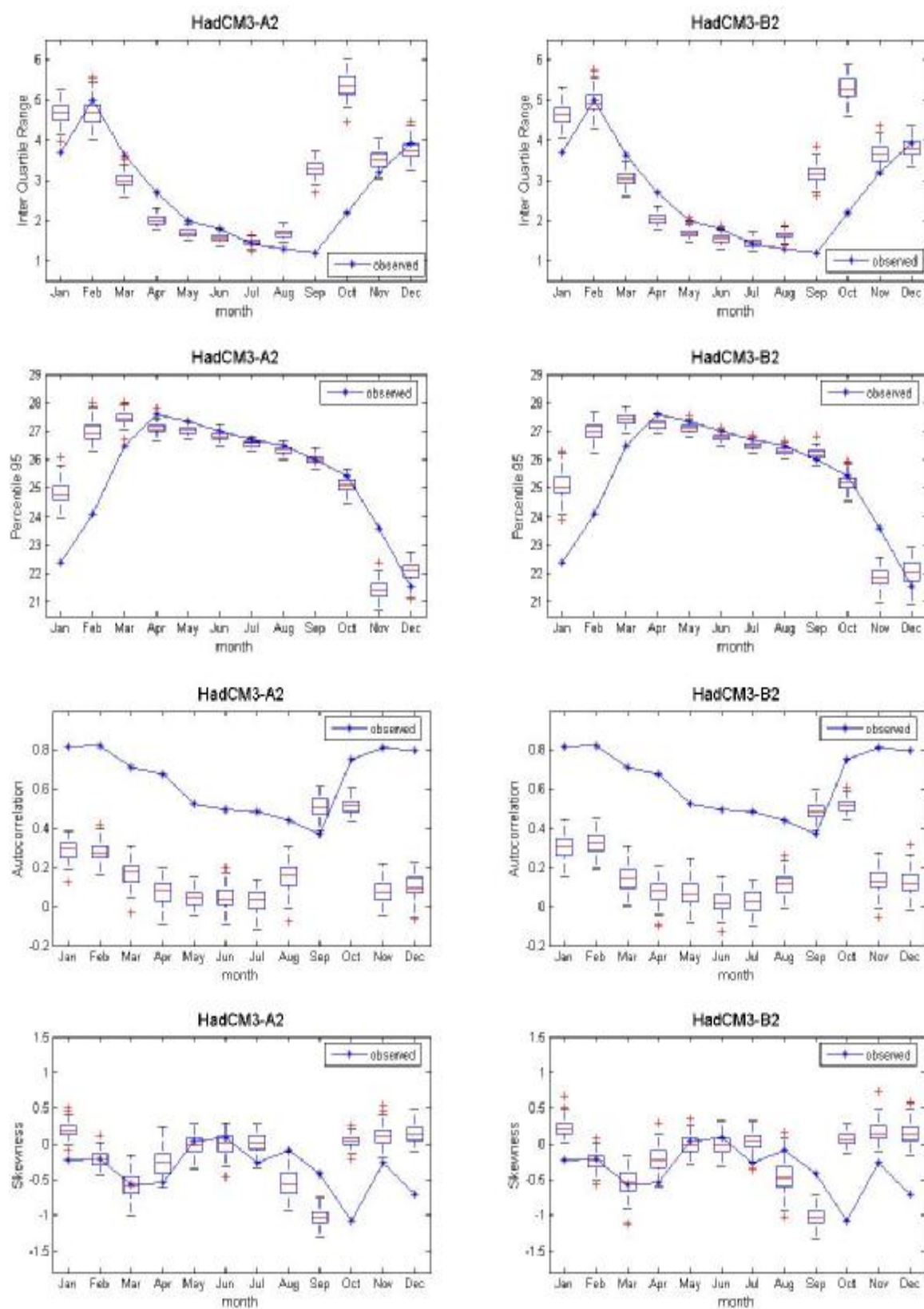
ภาพที่ ค.24 ค่าพิสัยระหว่างควอร์ไทล์ที่ 75 กับควอร์ไทล์ที่ 25 ค่าเปอร์เซ็นต์ไทล์ที่ 95 สัมประสิทธิ์สหสัมพันธ์ และค่าความเบ้ของข้อมูลอุณหภูมิรายวันอดีต และของข้อมูลสังเคราะห์จากภาพฉาย HadCM3A2 และ HadCM3B2 สำหรับสถานี 405201 (ปี ค.ศ.1991-2001)
