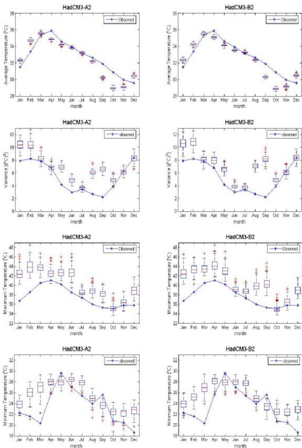
ภาพที่ ค.71 ค่าเฉลี่ย ค่าความแปรปรวน ค่าสูงสุด และค่าต่ำสุดของข้อมูลอุณหภูมิสูงสุดรายวันอดีต และของข้อมูลสังเคราะห์จากภาพฉาย HadCM3A2 และ HadCM3B2 สำหรับสถานี 431401 (ปี ค.ศ.1991-2001)
