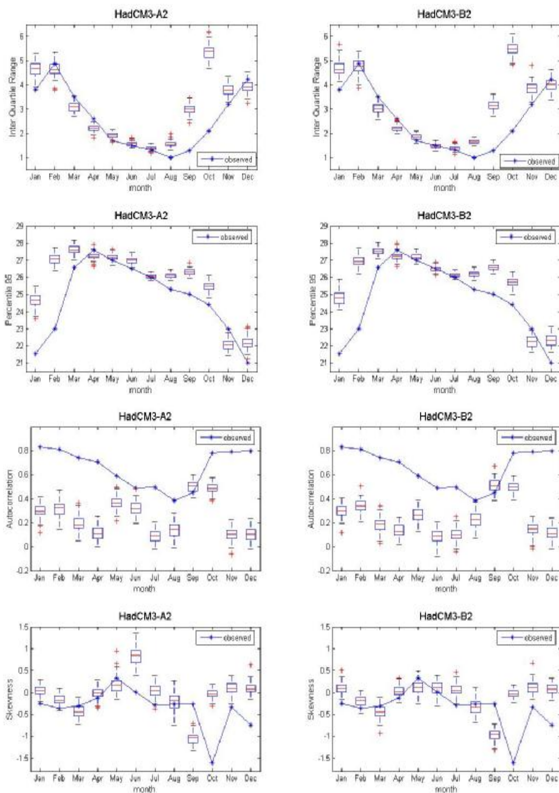
ภาพที่ ค.20 ค่าพิสัยระหว่างควอร์ไทล์ที่ 75 กับควอร์ไทล์ที่ 25 ค่าเปอร์เซ็นต์ไทล์ที่ 95 ค่าสัมประสิทธิ์สหสัมพันธ์ และค่าความเบ้ของข้อมูลอุณหภูมิต่ำสุดรายวันอดีต และของข้อมูลสังเคราะห์จากภาพฉาย HadCM3A2 และ HadCM3B2 สำหรับสถานี 381301 (ปี ค.ศ.1991-2001)
