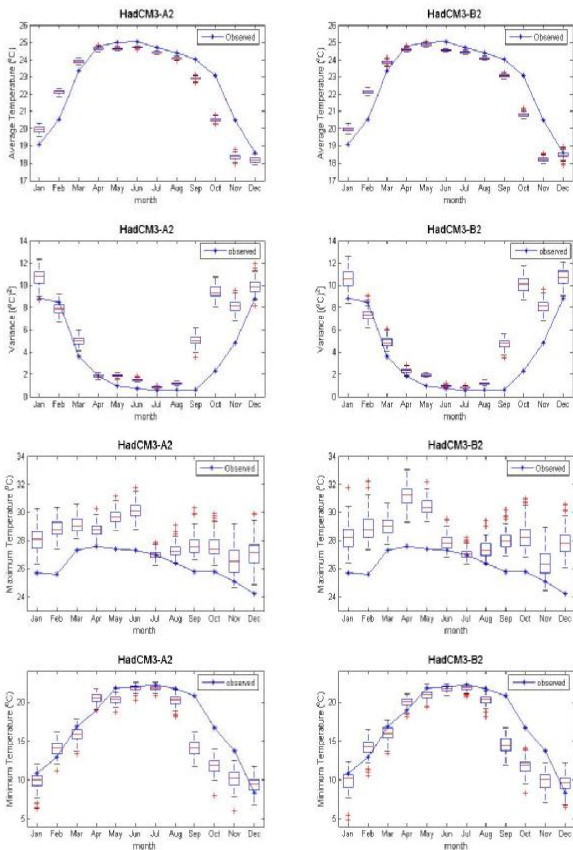
ภาพที่ ค.85 ค่าเฉลี่ย ค่าความแปรปรวน ค่าสูงสุด และค่าต่ำสุดของข้อมูลอุณหภูมิรายวันอดีต และของข้อมูลสังเคราะห์จากภาพฉาย HadCM3A2 และ HadCM3B2 สำหรับสถานี 431201 (ปี ค.ศ.1991-2001)
