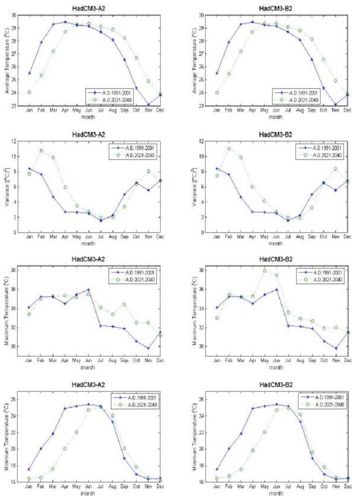
ภาพที่ ค.103 ค่าเฉลี่ย ค่าความแปรปรวน ค่าสูงสุด และค่าต่ำสุดของข้อมูลอุณหภูมิเฉลี่ยรายวันสังเคราะห์จาก ภาพฉาย HadCM3A2 และ HadCM3B2 สำหรับช่วงปี ค.ศ.1991-2001 และช่วงปี ค.ศ.2021-2040 (สถานี 431401)
