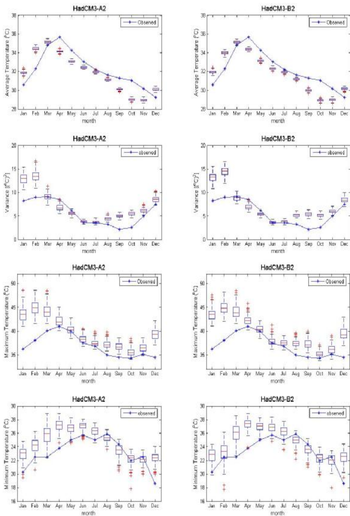
ภาพที่ ค.15 ค่าเฉลี่ย ค่าความแปรปรวน ค่าสูงสุด และค่าต่ำสุดของข้อมูลอุณหภูมิสูงสุดรายวันอดีต และของข้อมูลสังเคราะห์จากภาพฉาย HadCM3A2 และ HadCM3B2 สำหรับสถานี 405201 (ปี ค.ศ.1991-2001)
