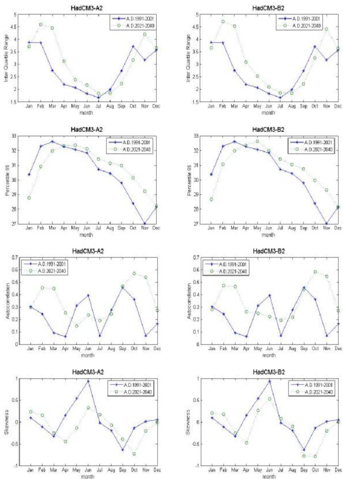
ภาพที่ ค.104 ค่าพิสัยระหว่างควอร์ไทล์ที่ 75 กับควอร์ไทล์ที่ 25 ค่าเปอร์เซ็นต์ไทล์ที่ 95 ค่าสัมประสิทธิ์สหสัมพันธ์ และค่าสัมประสิทธิ์ความเบ้ของข้อมูลอุณหภูมิเฉลี่ยรายวันสังเคราะห์จากภาพฉาย HadCM3A2 และ HadCM3B2 สำหรับช่วงปี ค.ศ.1991-2001 และช่วงปี ค.ศ.2021-2040 (สถานี 431401)
