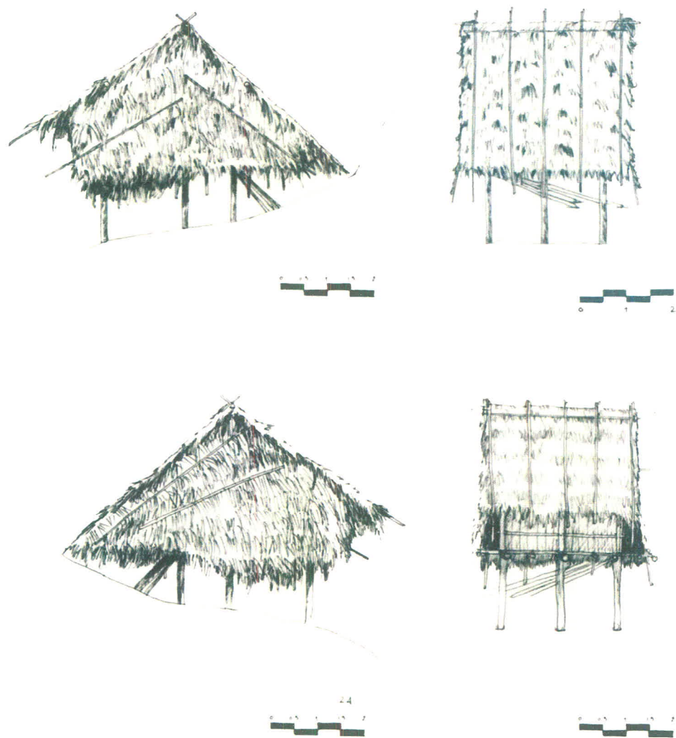
ภาพที่ 3.58 ลักษณะโครงสร้างและรูปทรงของรานชา นายหมอก ใจปึง
