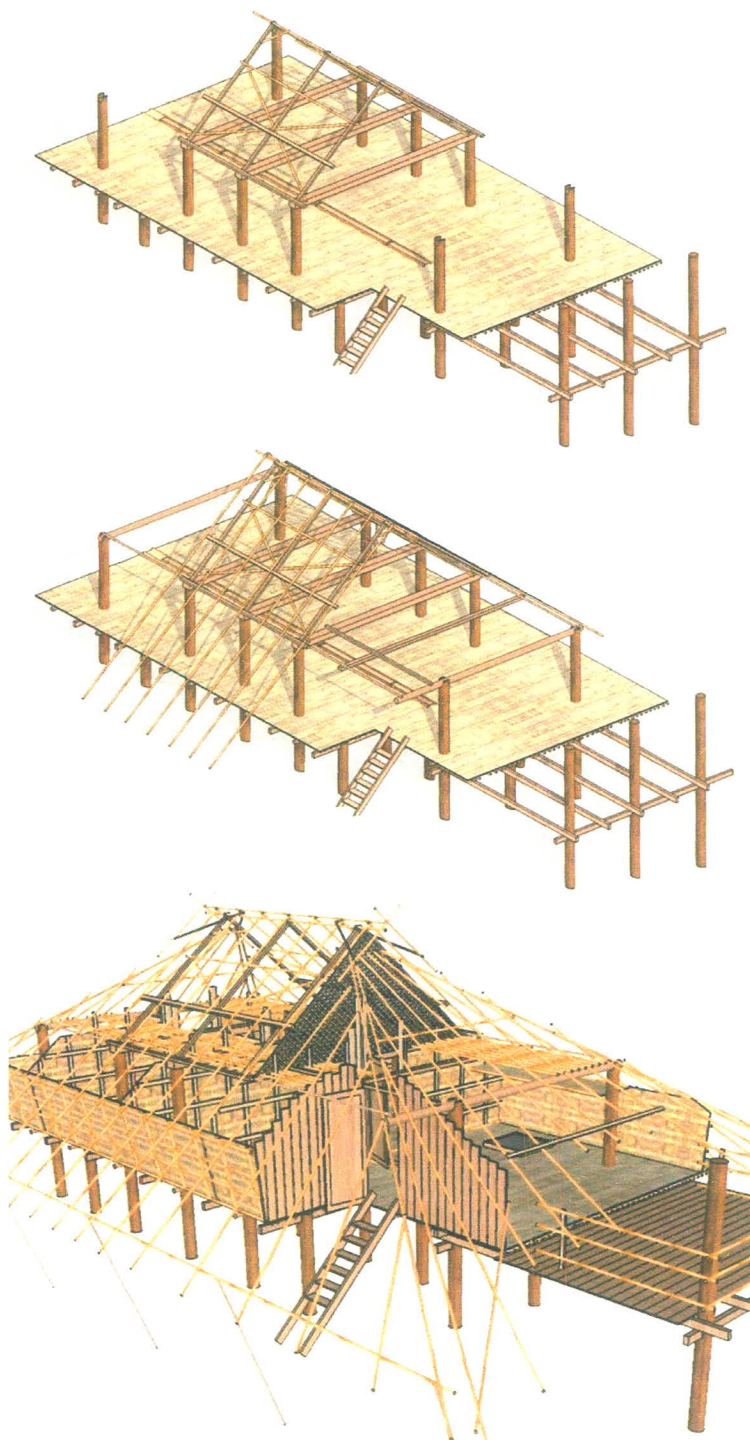
ภาพที่ 3.95 แสดงลักษณะโครงสร้างช่วงกลางของเรือน
