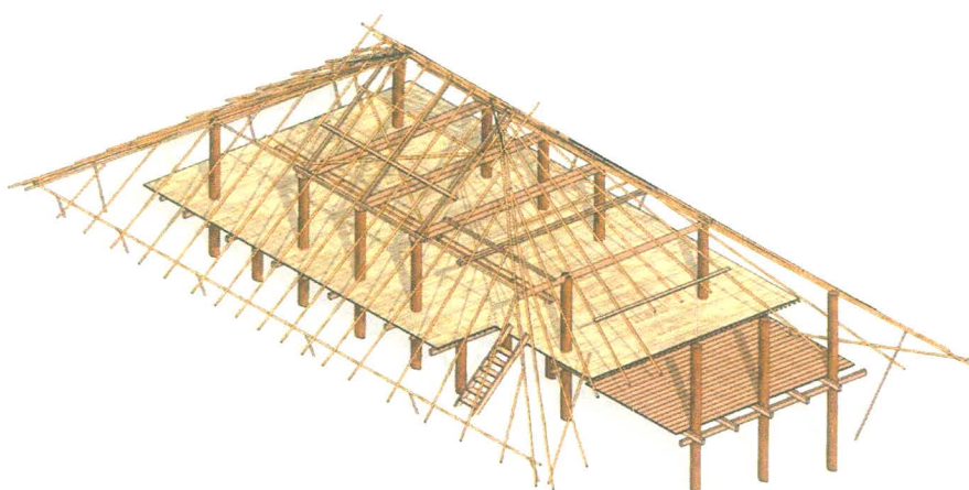
14. ปูพื้นชานแดด
