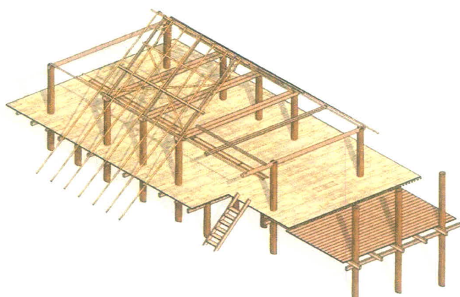
14. ปูพื้นชานแดด
