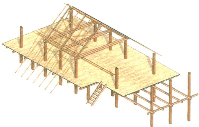
12. พาดโครงหลังคาด้านหลัง
