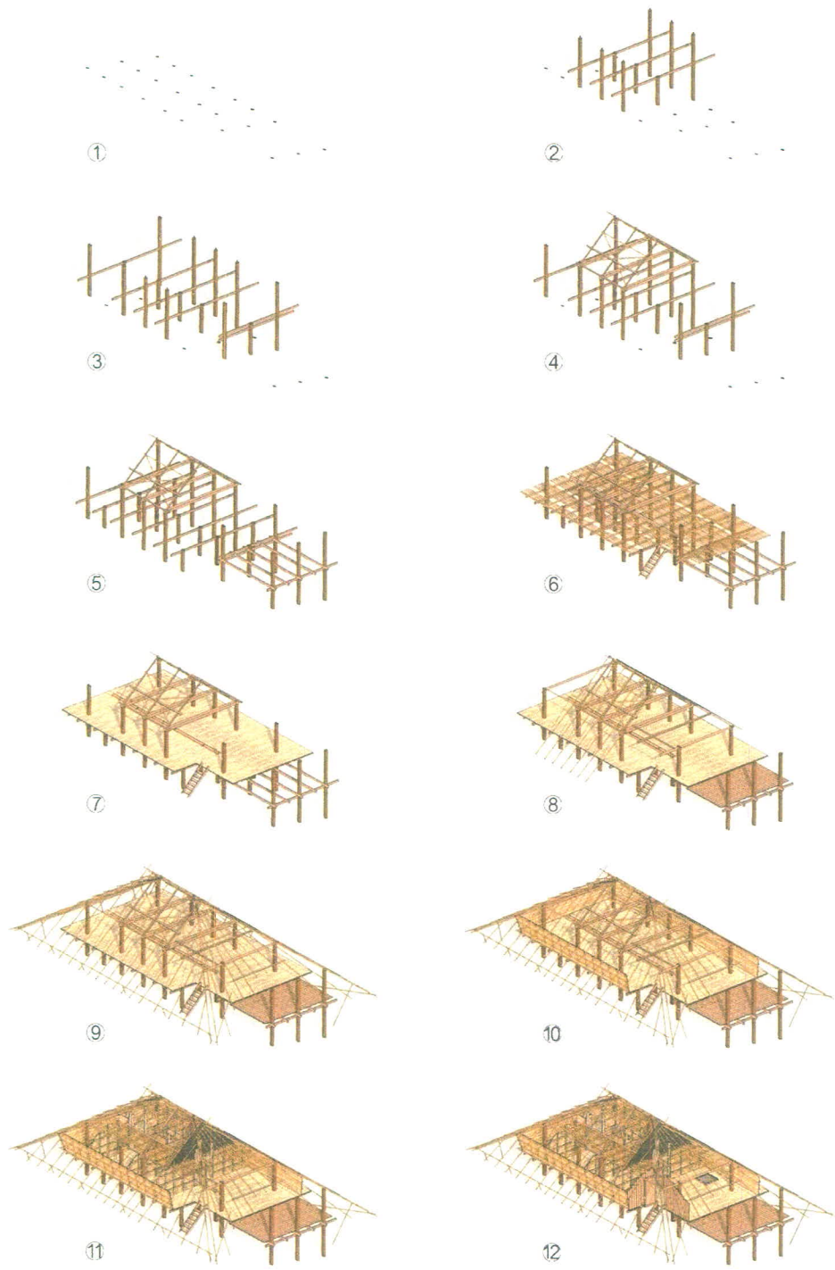
ภาพที่ 3.36 แสดงขั้นตอนสร้างเรือนนายใจ ใจปึง ภาพจำลอง 3 มิติ โดย นายศิริพงษ์ งามโขนนง
