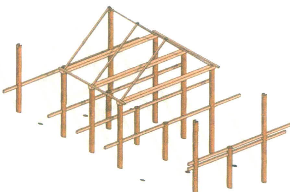
5. วางแปหัวเสาด้านข้างเสา 3 คู่ กลางเรือน
