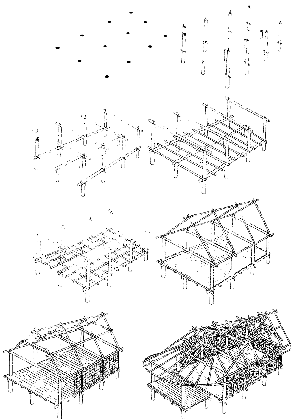
ภาพที่ 3.88 แสดงขั้นตอนการปลูกเรือน ดัดแปลงจากโครงการวิเคราะห์ทางสถาปัตตะยะกำ เฮือนชนเผ่าปรัย เมืองไชยะบุรี โดย สัญชัย สุทธิพัฒน์มงคล
