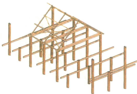
7. วางไม้ขวางยึดจันทันและวางไถ่ยั้งลมกากบาท ทะแยงมุมยึดจันทัน
