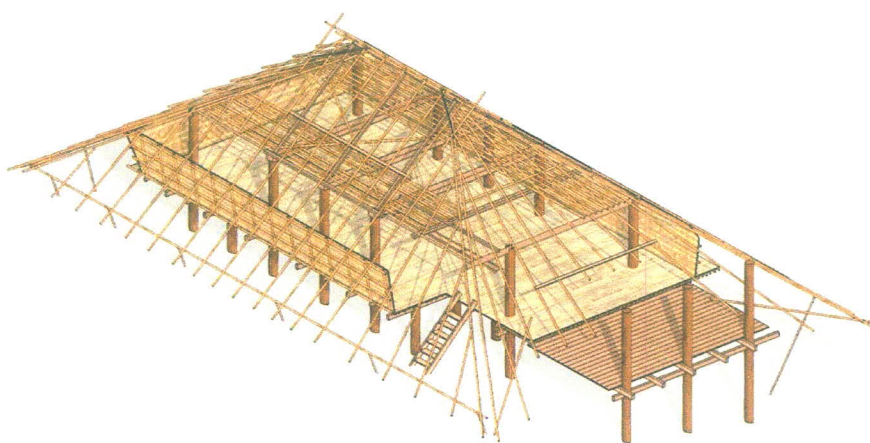
17. พาดท่อนไม้เหนือช่อกลางเรือน
