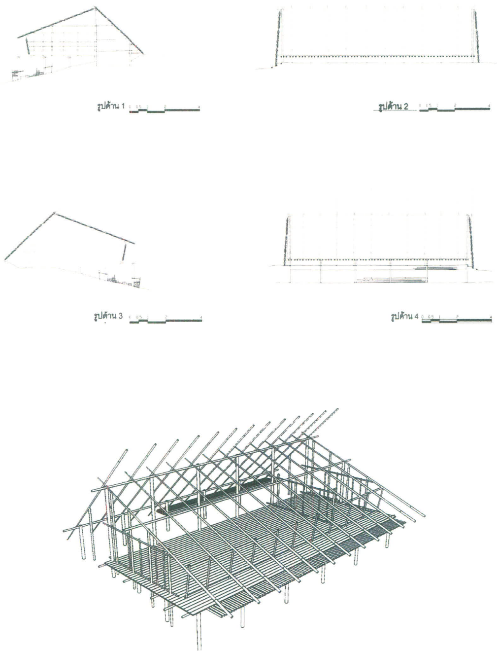
ภาพที่ 3.45 ลักษณะรายละเอียดของเรือนชั่วคราว นายเป็ก ใจปึง (ที่มา : จากการสำรวจภาคสนาม)
