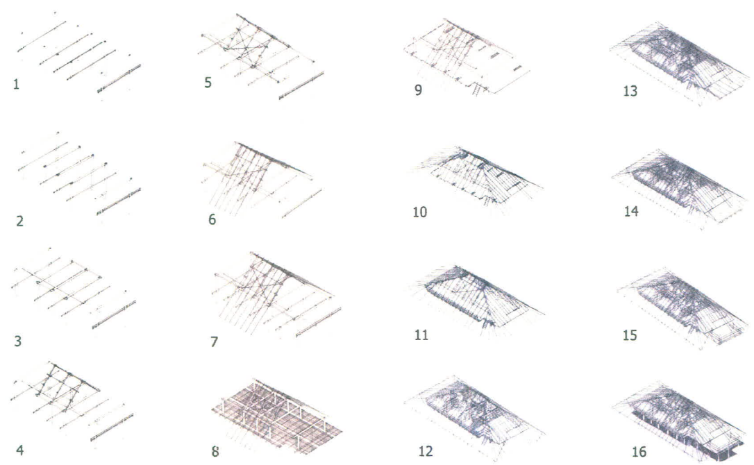
ภาพที่ 3.29 แสดงขั้นตอนสร้างเรือนนายมูล ใจปิง ที่มา : จากการสำรวจภาคสนามโดย สัณชัย สุทธิพัฒน์มงคล
