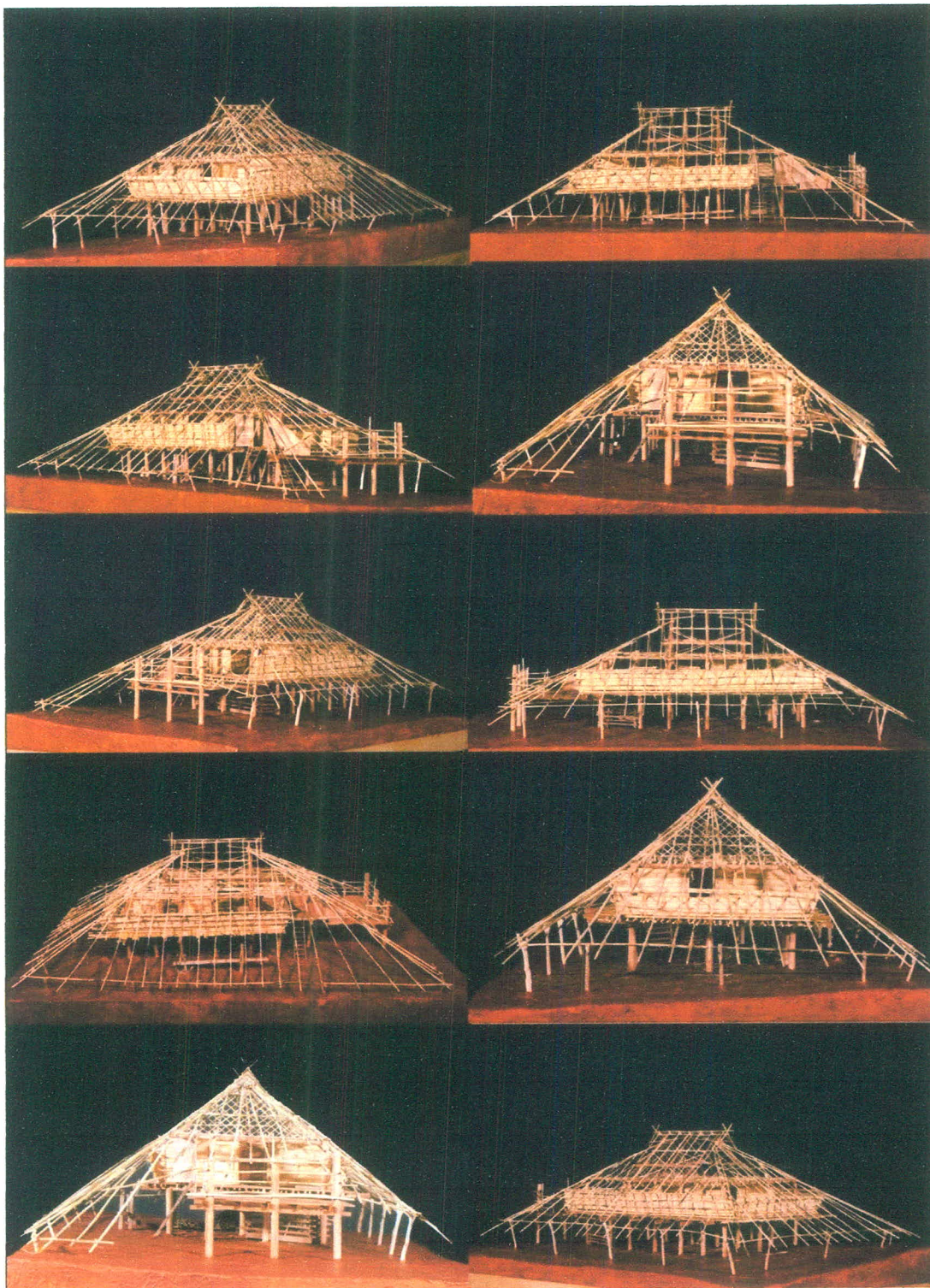
ภาพที่ 3.106 แสดงหุ่นจำลองศึกษาโครงสร้างเรือนปรียบ้านปากำ จัดทำโดย : นายวิชณวัตร ซอแก้ว และนาย ศิริพงษ์ งามขโนง
