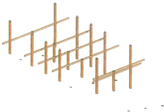
2. ตั้งเสาหลัก 3 คู่ กลางเรือน สอดคานรับพื้นวางเสารับคาน
