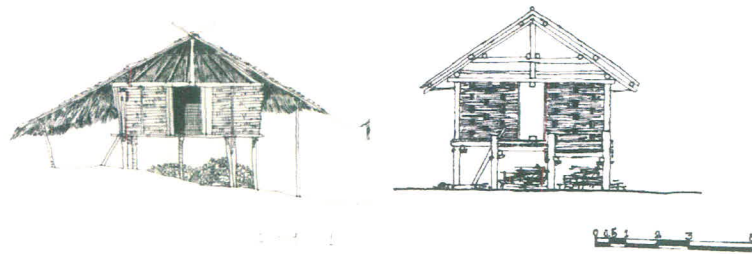
ภาพแสดง รูปตัดเรือนปรัย บ้านน้ำแพะ
