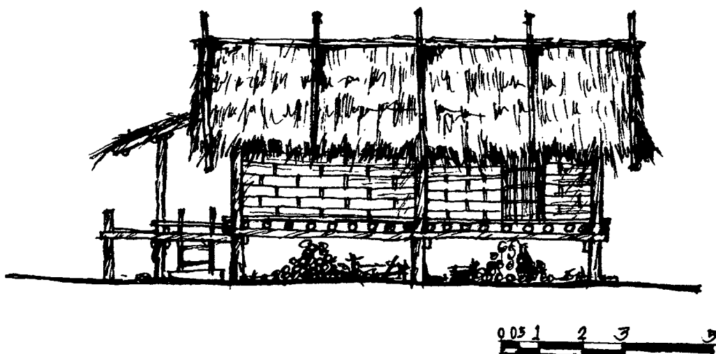
ภาพที่ 3.84 รูปด้านข้างเรือนปรียบ้านสันแต เมืองไชยะบุรี สปป.ลาว วาดจากโครงการวิเคราะห์ทางสถาปัตยกรรมเก่าเรือนชนเผ่าปรียบ เมืองไชยะบุรี โดย สักชัย สุพิพัฒน์มงคล
