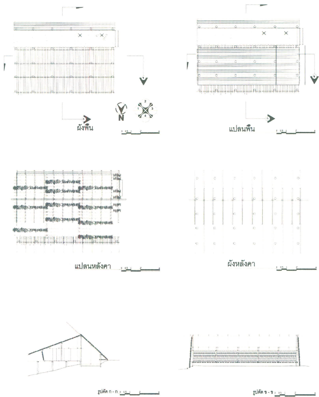
ภาพที่ 3.44 ลักษณะรายละเอียดของเรือนชั่วคราว นายเป็ก ใจปิง (ที่มา : จากการสำรวจภาคสนาม)
