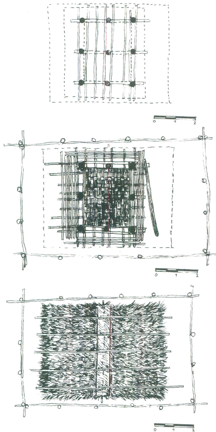
ภาพที่ 3.59 ลักษณะรายละเอียดของรานชา นายมูล ใจปึง
