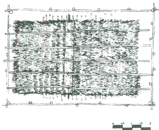
ภาพที่ 3.55 ลักษณะรายละเอียดของรานชา นายบัน ใจปิง
