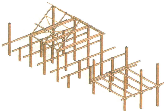
8. วางคานรับพื้นเพิ่มระหว่างเสาคันทันและหลัง
