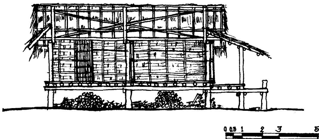
ภาพที่ 3.85 รูปตัดเรือนปรียบ้านสันแต เมืองไชยะบุรี สปป.ลาว วาดจากโครงการวิเคราะห์ทางสถาปัตยกรรมเก่า เรือนชนเผ่าปรียบ เมืองไชยะบุรี โดย สักชัย สุพิพัฒน์มงคล
