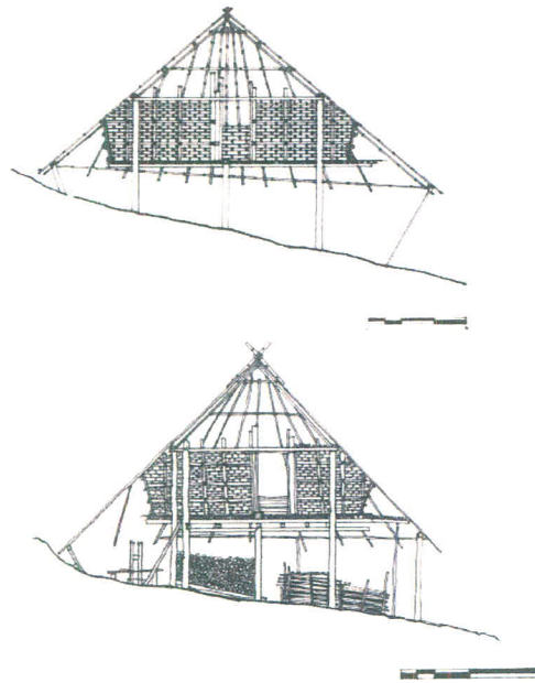
ภาพแสดง รูปตัดเรือนปรัย บ้านปากำ
