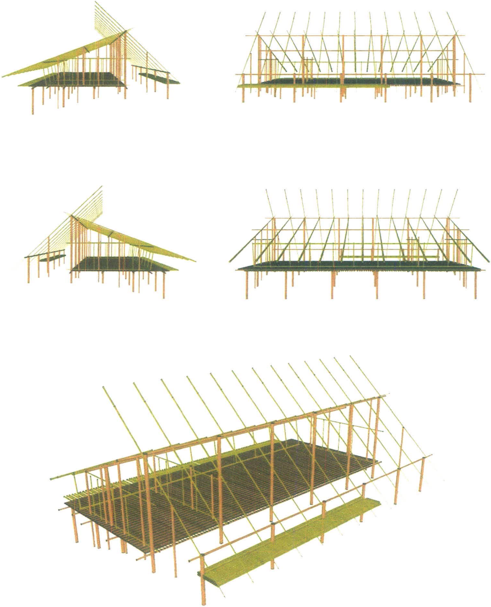
ภาพที่ 3.46 ลักษณะโครงสร้างของเรือนชั่วคราว นายเป็ก ใจปึง ภาพจำลอง 3 มิติ โดย นายศิริพงษ์ งามโชนง
