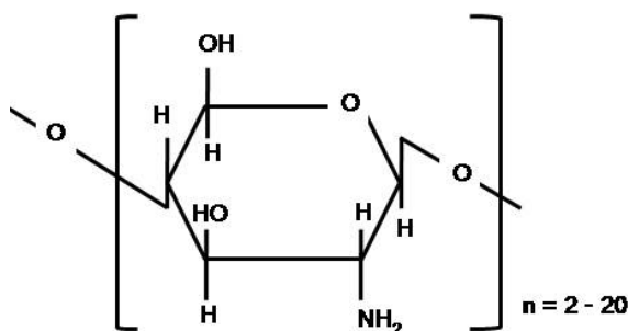
รูปที่ 2.5 โครงสร้างโมเลกุลของไคโตโอลิโกแซคคาไรด์
