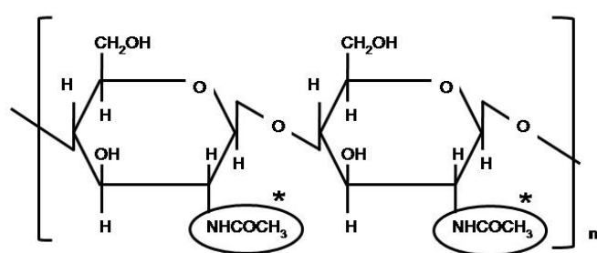
ไคติน (chitin)
