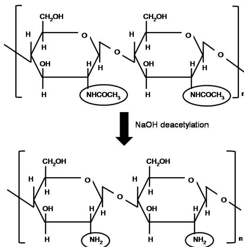
รูปที่ 2.3 การเปลี่ยนหมู่อะซิทิลของไคตินมาเป็นหมู่อะมิโนของไคโตซาน
