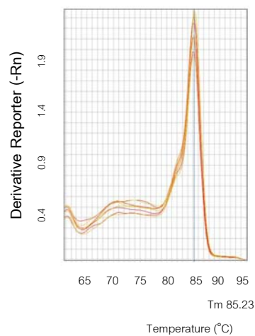
รูปที่ 4.3 แสดงผล Amplification curve (ด้านซ้ายมือ) และแสดงผล dissociation curves (ด้านขวามือ) ของยีน 18S rRNA (ก) และ PepT1 (ข)
