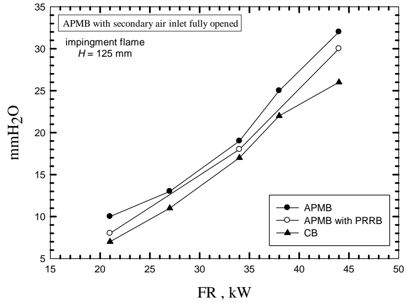
รูปที่ ๕.๕ กราฟเปรียบเทียบ pressure drop ของเตา APMB
