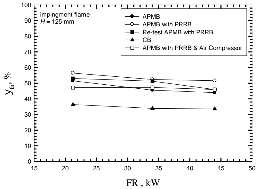
รูปที่ ๕.๖ กราฟเปรียบเทียบประสิทธิภาพเชิงความร้อนระหว่างการทดลองครั้งที่ 1 และครั้งที่ 2
