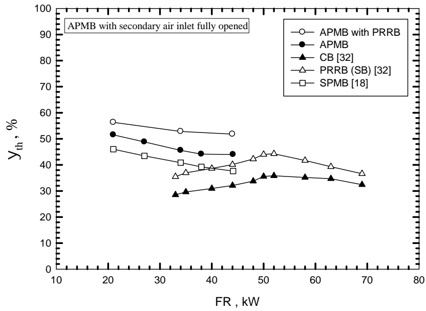
รูปที่ ข.9 กราฟเปรียบเทียบประสิทธิภาพเชิงความร้อนกับงานวิจัยที่ผ่านมา
