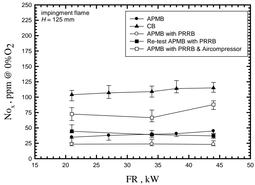
รูปที่ ๑.๒ กราฟแสดงปริมาณการปลดปล่อยมลพิษในการทดลองครั้งที่ ๒ ในส่วนของ NOx
