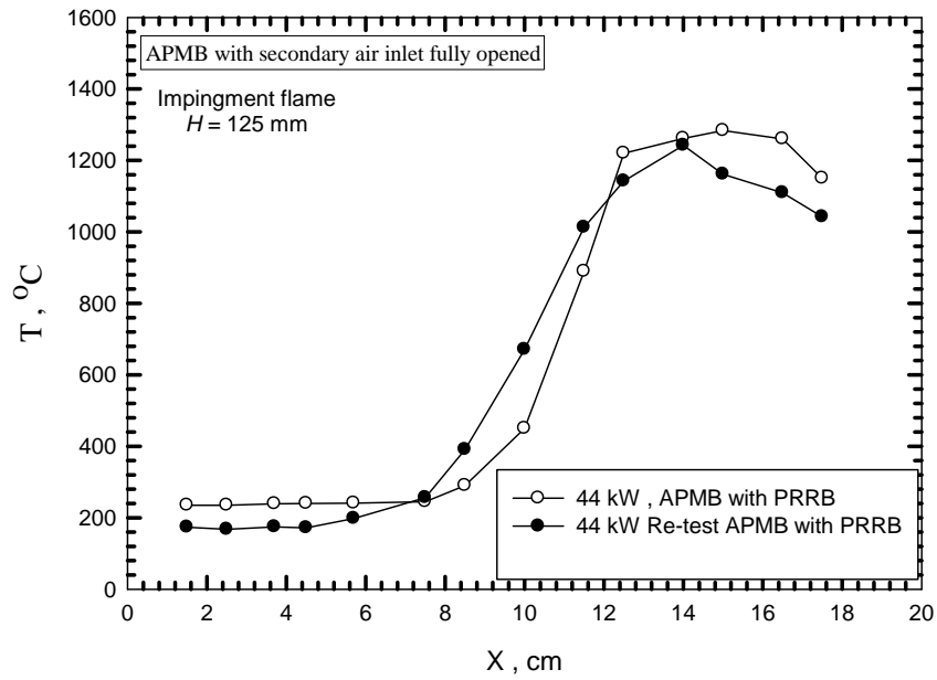
รูปที่ ๗.8 กราฟเปรียบเทียบ Temperature profile ระหว่างการทดลองครั้งที่ 1 และครั้งที่ 2
