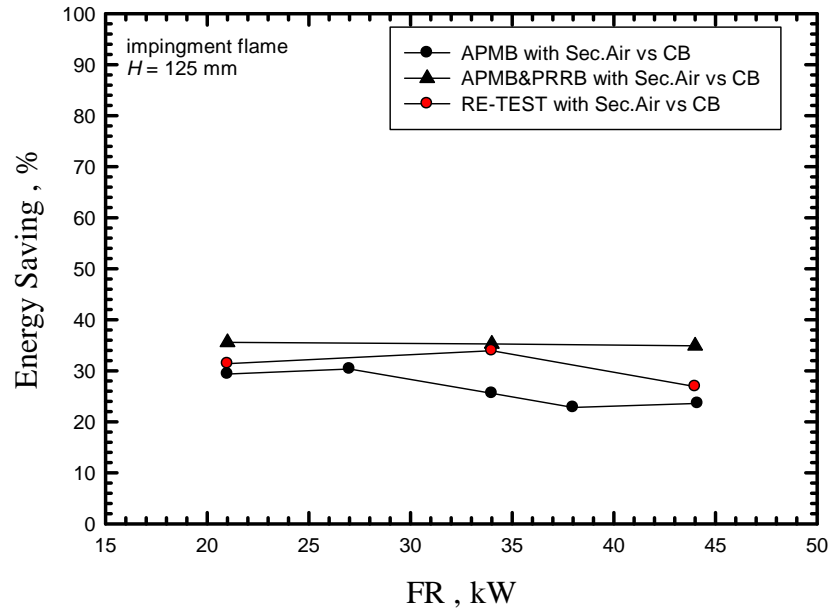
รูปที่ ๗.7 กราฟเปรียบเทียบการประหยัดพลังงานระหว่างการทดลองครั้งที่ 1 และครั้งที่ 2
