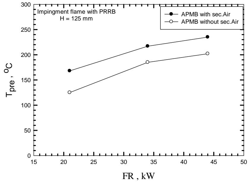
รูปที่ 3.4 กราฟเปรียบเทียบอุณหภูมิ preheated ของเตา APMB with PRRB
