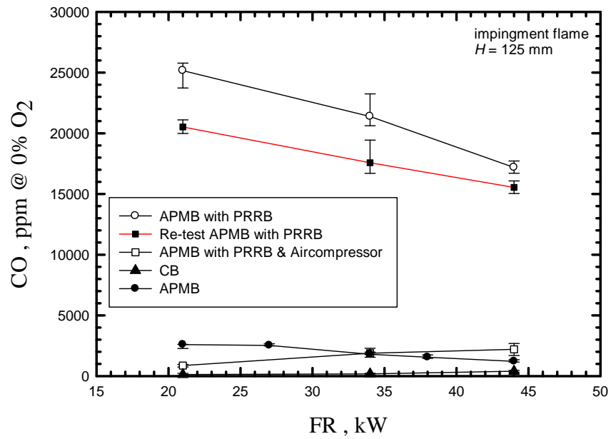
รูปที่ ๑.๑ กราฟแสดงปริมาณการปลดปล่อยมลพิษในการทดลองครั้งที่ ๒ ในส่วนของ CO
