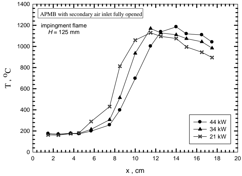
รูปที่ 3.3 กราฟ Temperature profile ของการทดลองครั้งที่ 2
