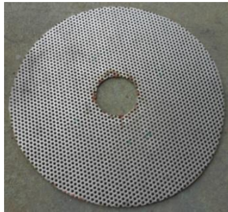
รูปที่ ก.9 แผ่นกั้น Flashback
