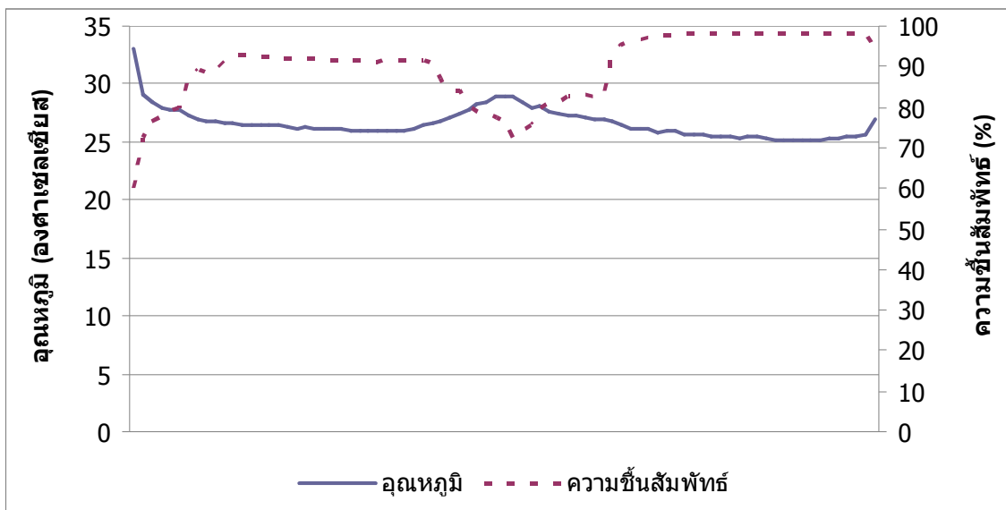
ภาพที่ 10 กราฟของอุณหภูมิและความชื้นด้านนอกถ้าเทพนิมิตร
