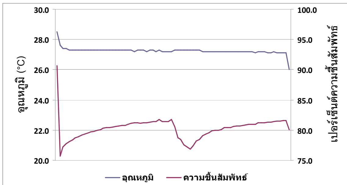
ภาพที่ 13 กราฟของอุณหภูมิและความชื้นด้านในถ้ำพระ
