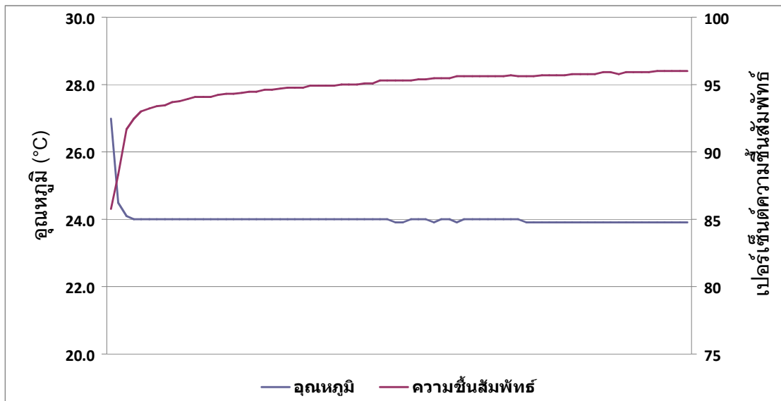
ภาพที่ 11 กราฟของอุณหภูมิและความชื้นด้านในถ้าเทพนิมิตร
