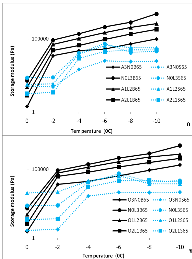
รูปที่ 4.12 ค่ามอดุลัสสะสมของตัวอย่างส่วนผสมแป้งอะซิทิเลต (ก) หรือแป้งโซเดียมออกเทนิลซัค-ซิเนต (ข) กับโพลีสปินกัมที่มีสัดส่วนต่างๆ ที่มีร้อยละ strain เท่ากับ 1 และความถี่ 2 Hz ที่อุณหภูมิ 0 ถึง -10 องศาเซลเซียส และมีค่าความเป็นกรด-ด่าง 6.5 ในสภาวะที่เติมและไม่เติมน้ำตาลซูโครสร้อยละ
