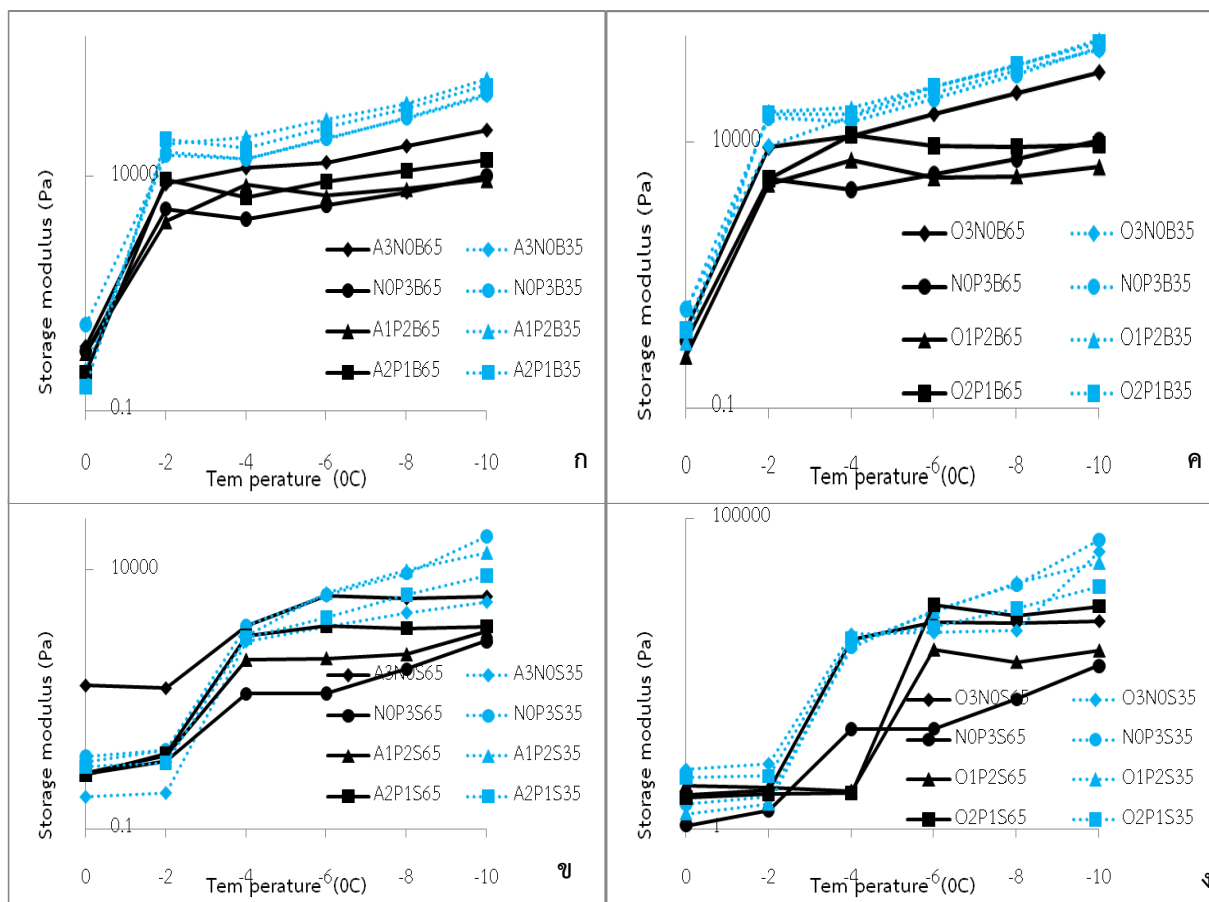
รูปที่ 4.25 ค่ามอดุลัสสะสมของสารผสมระหว่างพอลิเมอร์กับตัวอย่างแบ่งอะซิทีลเตทในระบบที่ไม่เติมน้ำตาลซูโครส (ก) หรือเติมน้ำตาลซูโครส (ข) หรือแบ่งโซเดียมออกซิเจนคลอไรด์ที่ไม่เติมน้ำตาลซูโครส (ค) หรือเติมน้ำตาลซูโครส (ง) ที่มี strain ร้อยละ 1 และความถี่ 2 Hz ที่อุณหภูมิ 0 ถึง -10 องศาเซลเซียส ที่มีค่าความเป็นกรด-ด่าง 3.5 หรือ 6.5
