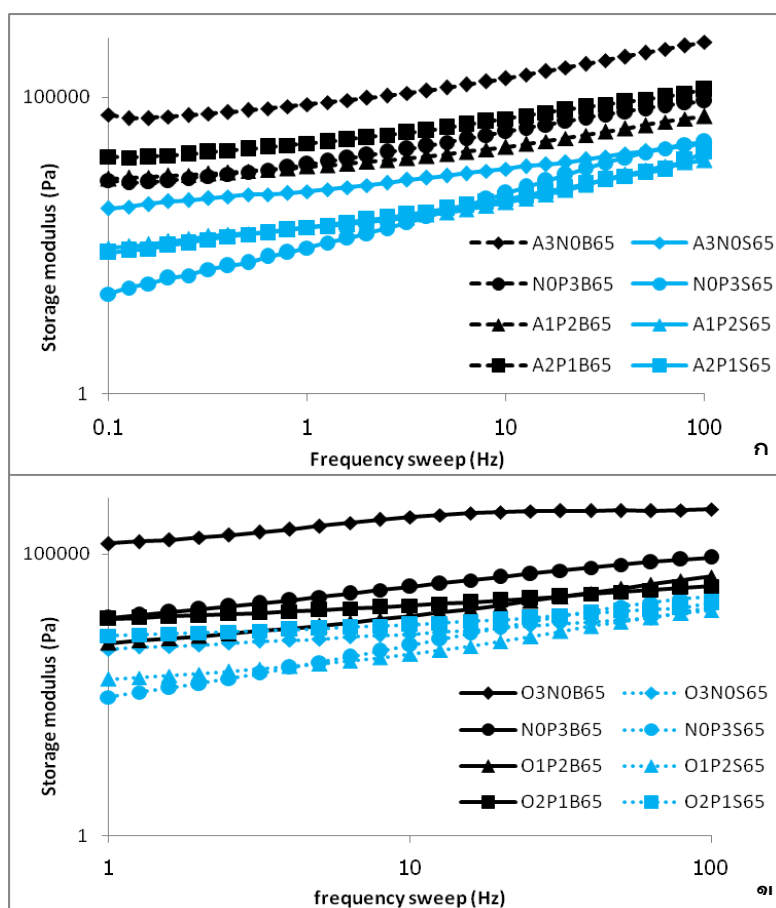
รูปที่ 4.15 มอดุลัสสะสมของตัวอย่างส่วนผสมแป้งอะซิทีเลเตท (ก) หรือแป้งโซเดียมออกเตนิลซัค-ซิเนต (ข) กับ เพคตินที่มีร้อยละ strain เท่ากับ 1 และความถี่ 0.1-100 Hz ที่อุณหภูมิ -10 องศาเซลเซียส และมีค่าความเป็นกรดต่าง 6.5 ในสภาวะที่เติมและไม่เติมน้ำตาลซูโครสร้อยละ 16
