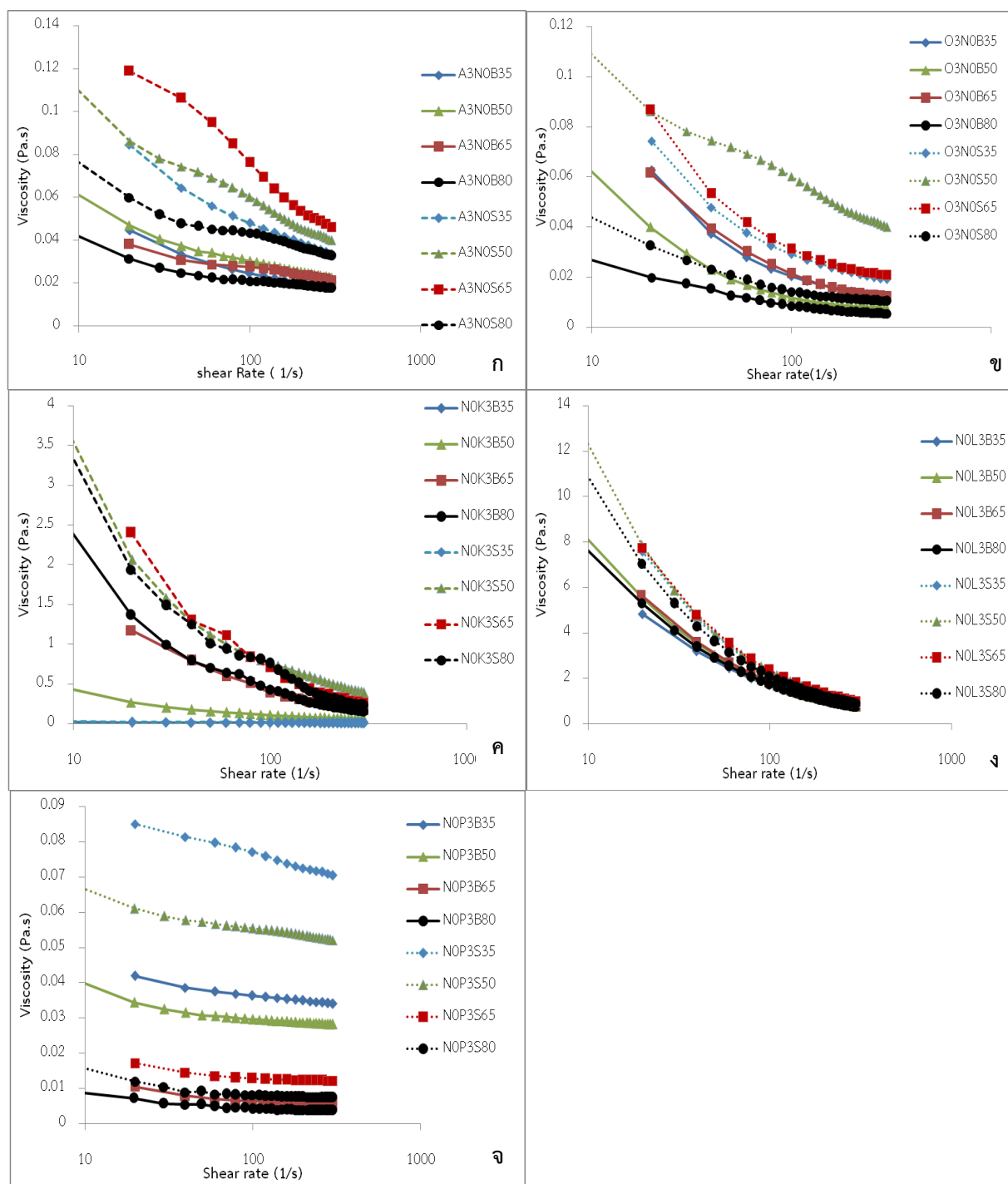
รูปที่ 4.18 ความหนืดของตัวอย่างแป้งดัดแปรอะซิทีเลต (ก) แป้งโซเดียมออกเทนิลซัคซินेट (ข) แคปปา-คาราจีแนน (ค) โคล์สปีนัม (ง) และ เพคติน (จ) ในระบบที่มีและไม่มีน้ำตาลซูโครสที่มีค่าความเป็นกรด-ด่างแตกต่างกัน ที่อุณหภูมิ 25 องศาเซลเซียส ที่มีอัตราเฉือน 0- 300 1/s
