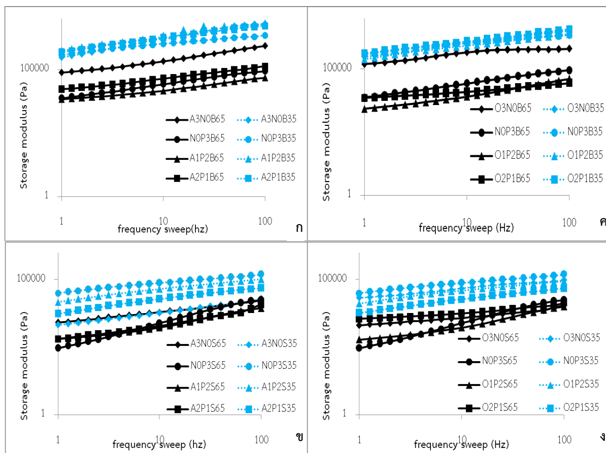
รูปที่ 4.26 โมดูลัสสะสมของสารผสมระหว่างเพคตินกับตัวอย่างแป้งอะซีทิลเลตในแบบที่ไม่เติมน้ำตาลซูโครส (ก) หรือเติมน้ำตาลซูโครส (ข) หรือแป้งโซเดียมออกเทนิลซัคซิเนตที่ไม่เติมน้ำตาลซูโครส (ค) หรือเติมน้ำตาลซูโครส (ง) ที่มี strain ร้อยละ 1 และความถี่ของการสั่น 0.1-100 Hz อุณหภูมิ -10 องศาเซลเซียส ที่มีค่าความเป็นกรดต่าง 3.5 หรือ 6.5
