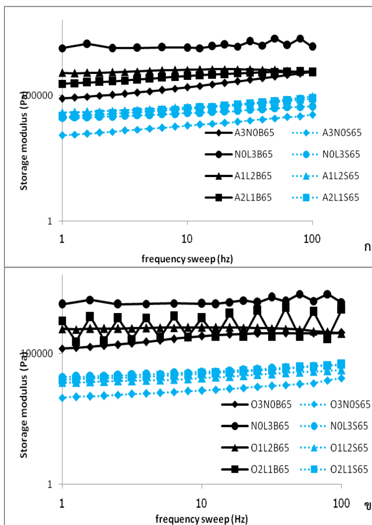
รูปที่ 4.13 มอดุลัสสะสมของตัวอย่างส่วนผสมแป้งอะซิทิเลเตด (ก) หรือแป้งโซเดียมออกเทนิลซัคซิเนต (ข) กับโพลีสปีนัมที่มีร้อยละ strain เท่ากับ 1 และความถี่ 0.1-100 Hz ที่อุณหภูมิ -10 องศาเซลเซียส และมีค่าความเป็นกรด-ด่าง 6.5 ในสถานะที่เต็มและไม่เติมน้ำตาลซูโครสร้อยละ 16
