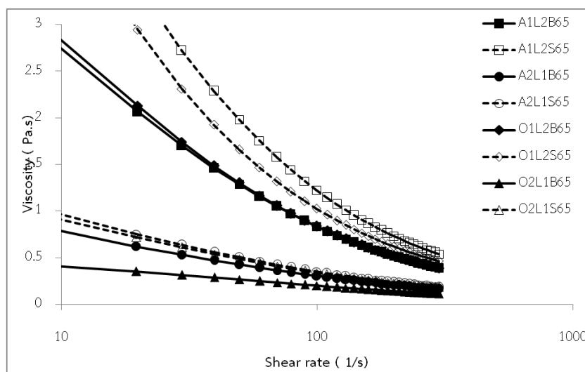
รูปที่ 4.3 คุณสมบัติด้านความหนืดของตัวอย่างส่วนผสมระหว่างแป้งมันสำปะหลังดัดแปรอะซิทิเลเตด หรือ โซเดียมออกเทนิลซัคซิเนต กับโลคัสปินกัมที่มีสัดส่วนแตกต่างกัน โดยวัดที่อุณหภูมิ 25 องศาเซลเซียส และมีค่าความเป็นกรด-ด่าง 6.5 ในสถานะที่เต็มและไม่เติมน้ำตาลทรายร้อยละ 16
