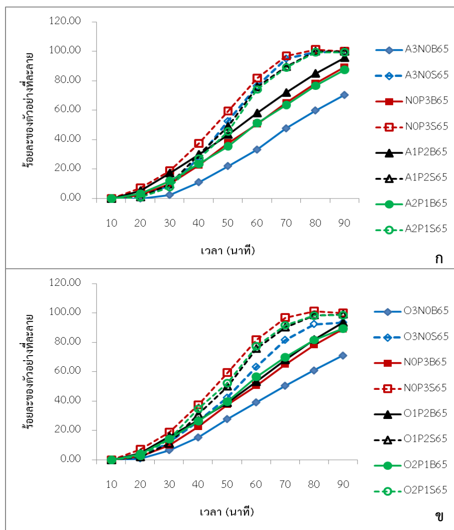
รูปที่ 4.7 อัตราการละลายของตัวอย่างส่วนผสมระหว่างแป้งมันสำปะหลังดัดแปรอะซิทีเลเตด (ก) หรือ โซเดียมออกเทนนิลซัคซิเนต (ข) กับเพคตินที่มีสัดส่วนแตกต่างกัน โดยวัดที่อุณหภูมิ 25 องศาเซลเซียส และมีค่าความเป็นกรด ต่าง 6.5 ในสถานะที่เต็มและไม่เติมน้ำตาลทรายร้อยละ 16
