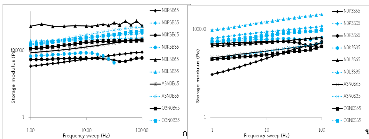
รูปที่ 4.17 มอดุลัสสะสมของตัวอย่างแป้งตัดแปรรหรือไฮโดรคอลลอยด์ในระบบที่ไม่มีน้ำตาลซูโครส (ก) หรือระบบที่มีน้ำตาลซูโครส (ข) ที่มีร้อยละ strain เท่ากับ 1 และความถี่ระหว่าง 0.1-100 Hz ที่อุณหภูมิ -10 องศาเซลเซียส ที่มีค่าความเป็นกรด-ด่าง 3.5 หรือ 6.5
