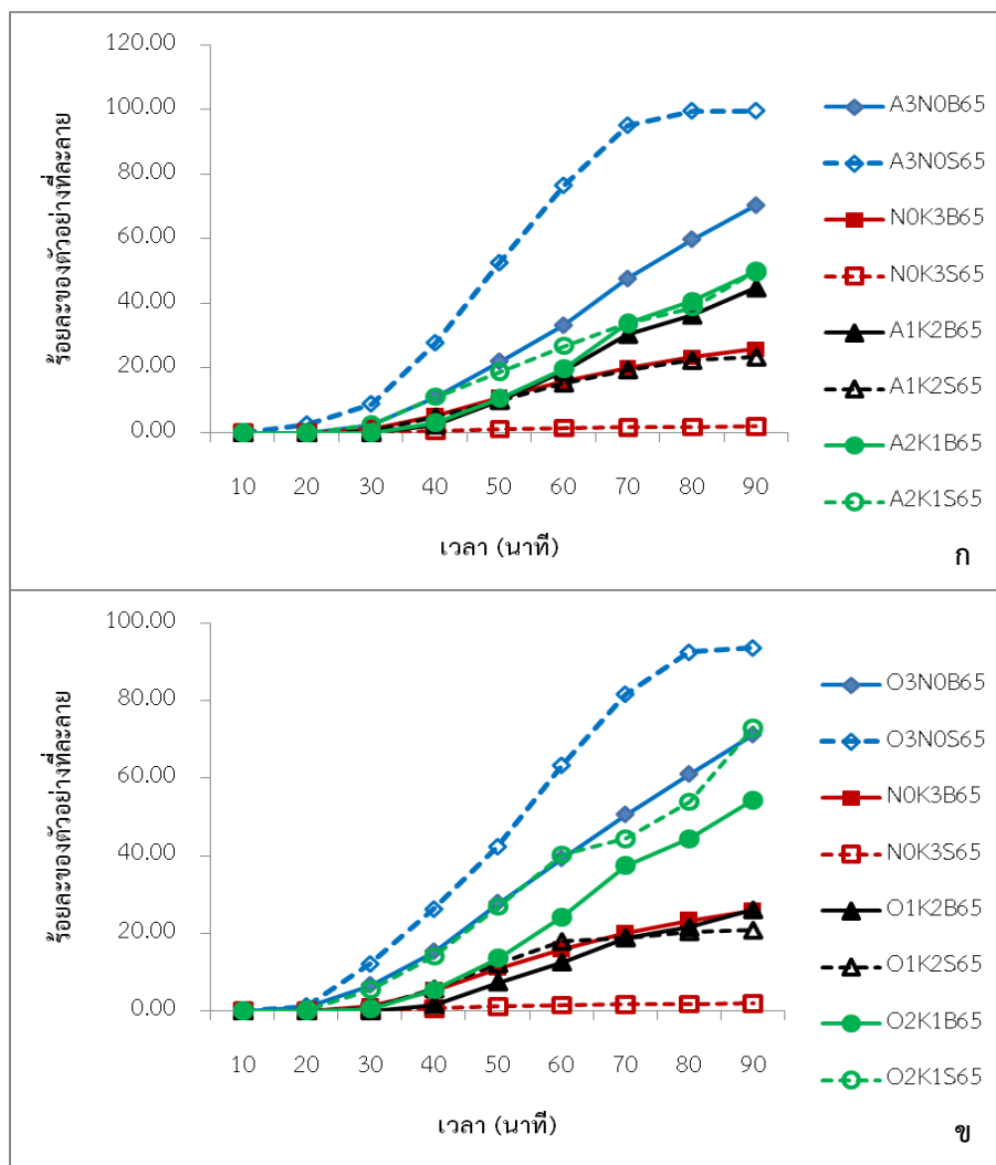
รูปที่ 4.5 อัตราการละลายของตัวอย่างส่วนผสมระหว่างแป้งมันสำปะหลังดัดแปรอะซิทีเลต (ก) หรือ โซเดียมออกเทนิลซัคซิเนต (ข) กับแคปทา-คาร์ราจีแนนที่มีสัดส่วนแตกต่างกัน โดยวัดที่อุณหภูมิ 25 องศาเซลเซียส และมีค่าความเป็นกรด ต่าง 6.5 ในสถานะที่เต็มและไม่เติมน้ำตาลทรายร้อยละ 16
