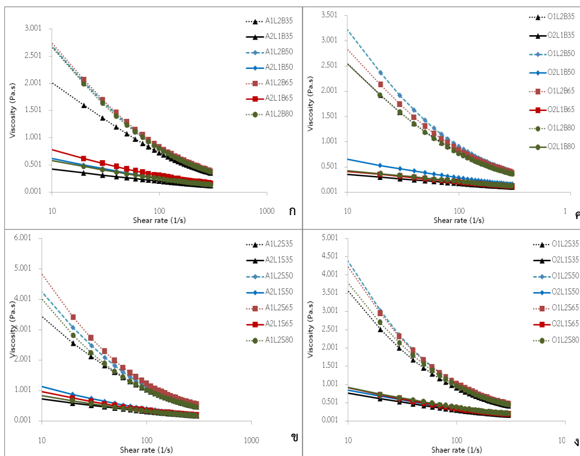
รูปที่ 4.24 ความหนืดของสารผสมระหว่างโลคัสป็นกับกับตัวอย่างแป้งอะซิทิเลเตทในระบบที่ไม่เติมน้ำตาลซูโครส (ก) หรือเติมน้ำตาลซูโครส (ข) หรือแป้งโซเดียมออกเทนิลซัคซินเนตที่ไม่เติมน้ำตาลซูโครส (ค) หรือเติมน้ำตาลซูโครส (ง) ที่มีอัตราเฉือน 1-300 1/s ที่อุณหภูมิ 25 องศาเซลเซียส ที่มีค่าความเป็นกรด-ด่าง 3.5, 5.0, 6.5 หรือ 8.0
