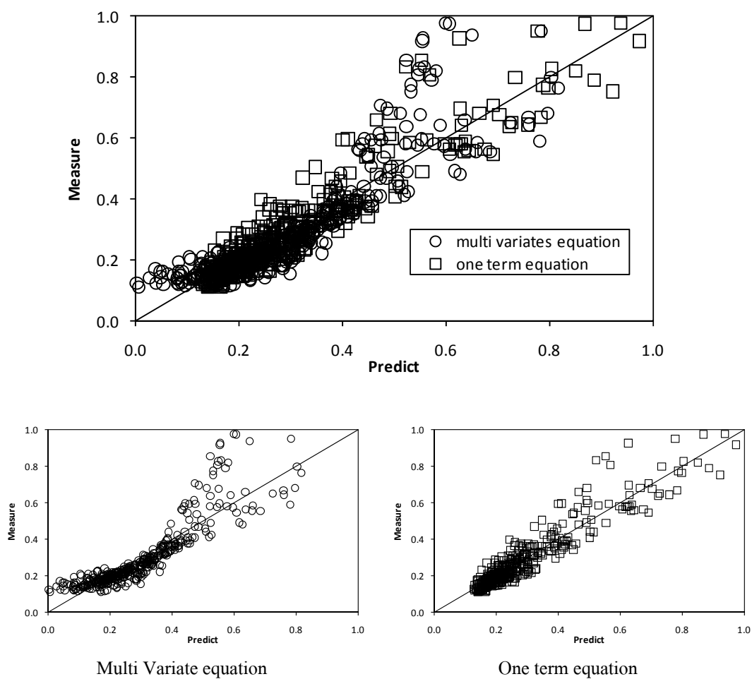
รูปที่ 5.27 การเปรียบเทียบค่าทำนายกับค่าที่ตรวจวัดกรณีแผงกรองคลื่นทำงาน 3 แผง คลื่นเอียงทำมุม 45 - 90 องศา กับแนวแผงกรองคลื่น
