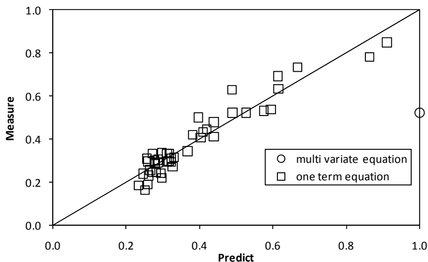
รูปที่ 5.25 การเปรียบเทียบค่าทำนายกับค่าที่ตรวจวัดกรณีแผงกรองคลื่นทำงาน 2 แผง คลื่นเฉียงทำมุม 45 - 90 องศา กับแนวแผงกรองคลื่น
