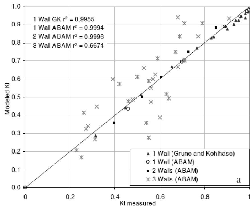
รูปที่ 3.11 การเปรียบเทียบผลวิเคราะห์จากแบบจำลองคณิตศาสตร์กับผลทดลองของ Grune and Kohlhasse (1974) และ ABAM (1993) กรณีค่าสัมประสิทธิ์การส่งผ่านคลื่น
