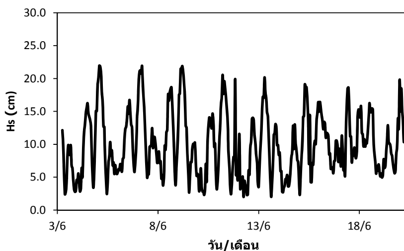
รูปที่ 5.6 ความสูงคลื่นนัยสำคัญด้านหลังแพงกรองคลื่น
