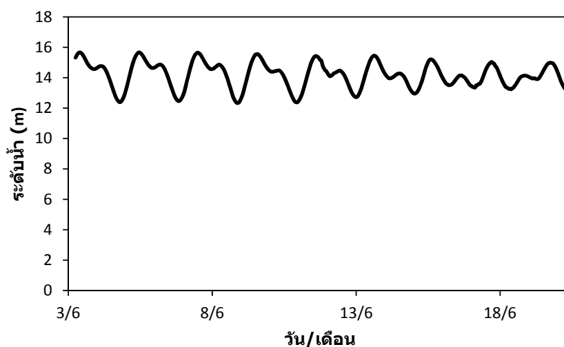
รูปที่ 5.5 ความลึกน้ำด้านหลังแพงกรองคลื่นตรวจวัดโดยอุปกรณ์เอดับบลิวเอช-ยูเอสบี
