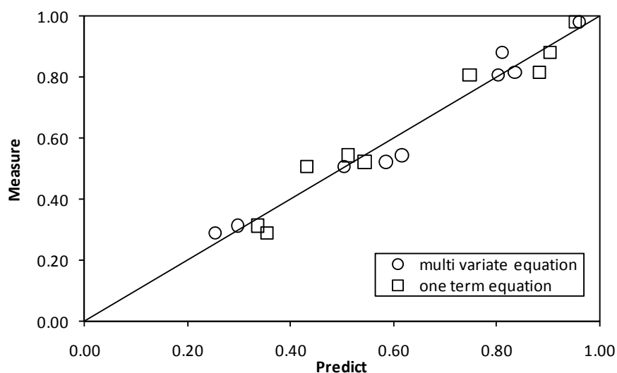
รูปที่ 5.24 การเปรียบเทียบค่าทำนายกับค่าที่ตรวจวัดกรณีแพ่งกรองคลื่นทำงาน 2 แผง คลื่นเฉียงทำมุม 0 – 45 องศา กับแนวแพ่งกรองคลื่น
