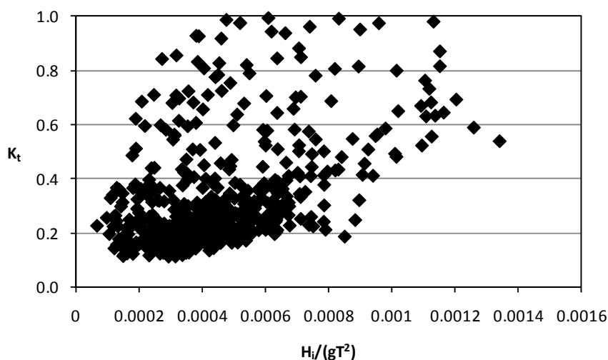
รูปที่ 5.19 ความสัมพันธ์ระหว่าง H_t/(gT^2) กับ K_t
