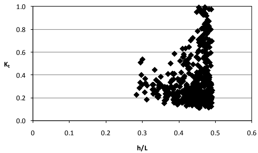
รูปที่ 5.21 ความสัมพันธ์ระหว่าง h/L กับ K_t
