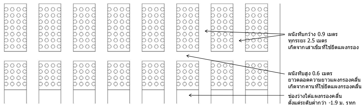
(ก) รูปด้านแผงกรองคสล.แผงนอก
