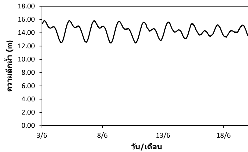
รูปที่ 5.4 ความลึกน้ำด้านหน้าแพงกรองคลื่นตรวจวัดโดยอุปกรณ์ไทรตัน เอดีวี
