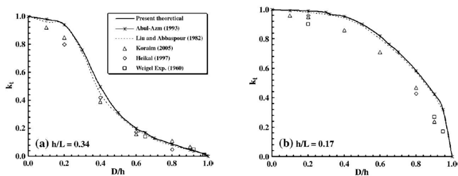
รูปที่ 3.18 การศึกษาความสัมพันธ์ระหว่างค่าสัมประสิทธิ์การส่งผ่านคลื่นกับอัตราส่วนระยะกินน้ำลึกต่อความลึกน้ำ ( D/h ) และอัตราส่วนความลึกน้ำต่อความยาวคลื่น ( h/L ) ของ Rageh and Koriem (2010)
