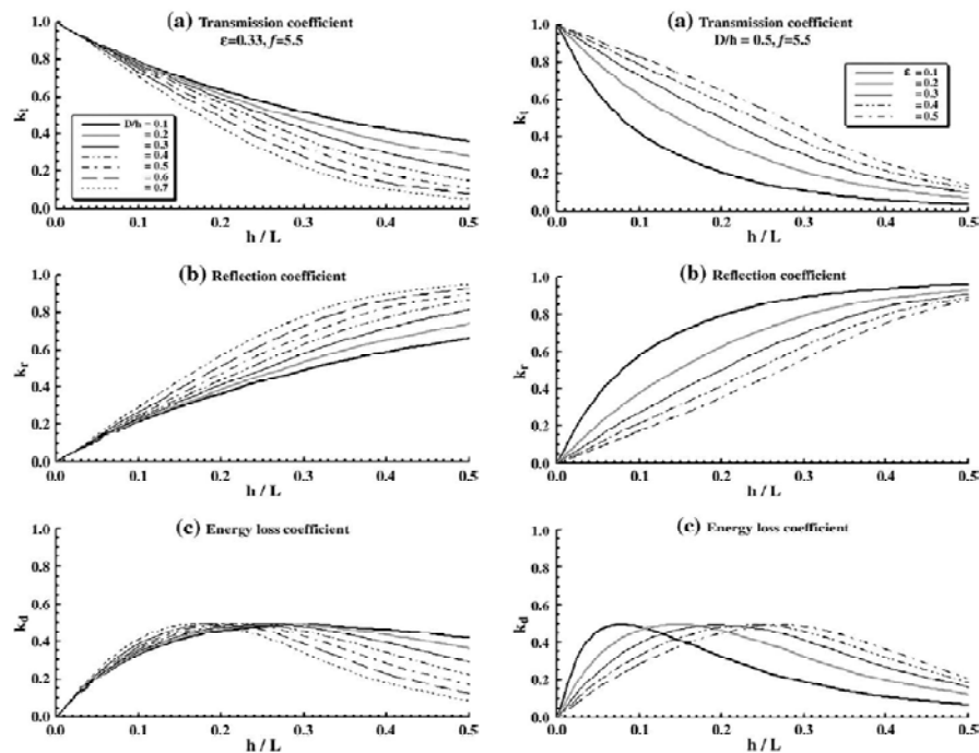
รูปที่ 3.20 การศึกษาความสัมพันธ์ระหว่างค่าสัมประสิทธิ์การส่งผ่านคลื่น การสะท้อนกลับ และการสูญเสียพลังงาน กับอัตราส่วนความลึกน้ำต่อความยาวคลื่น ( h/L ) และความพรุนของ Rageh and Koriem (2010)
