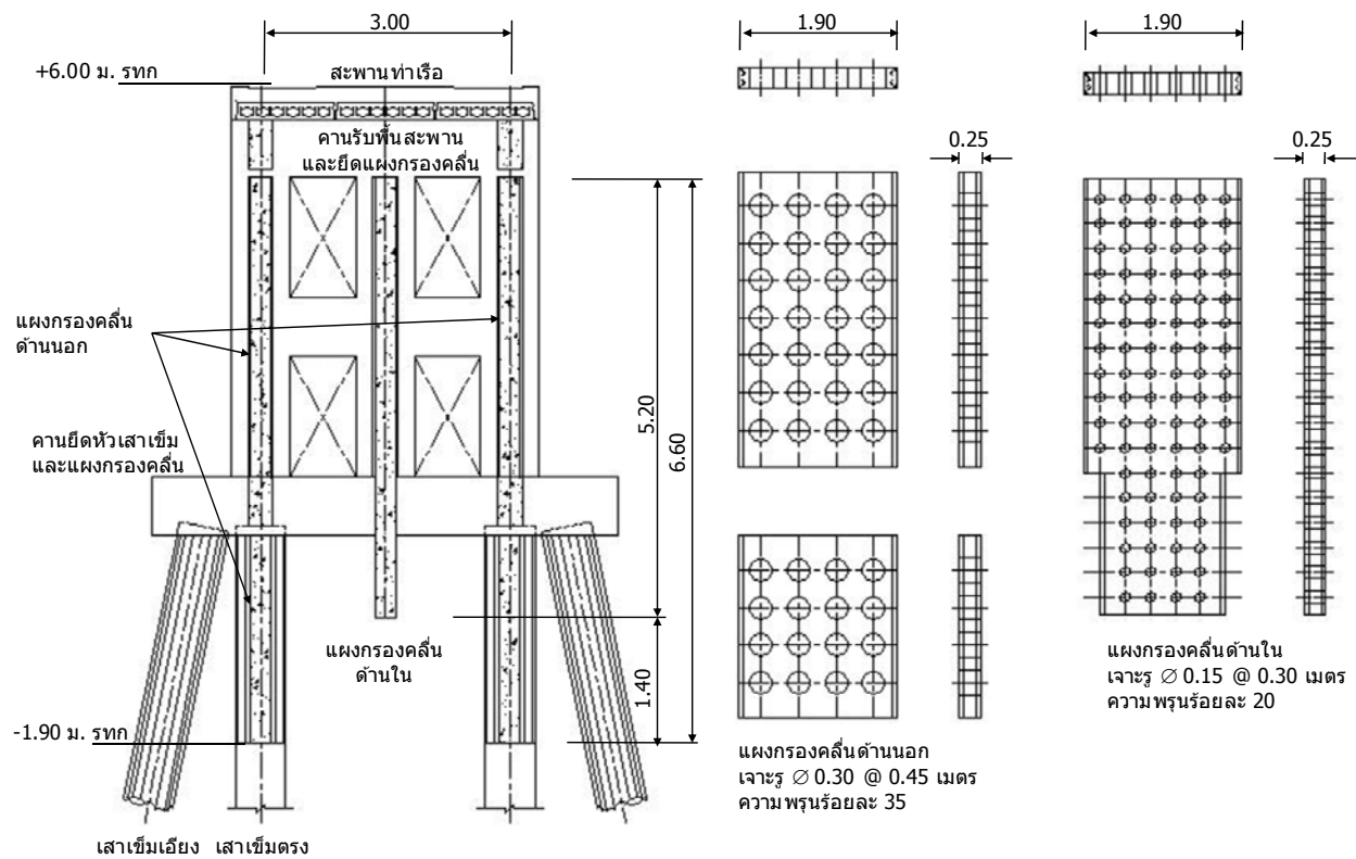
รูปที่ 2.3 รูปตัดสะพานทำเรือและรายละเอียดแฉงกรองคลื่น
