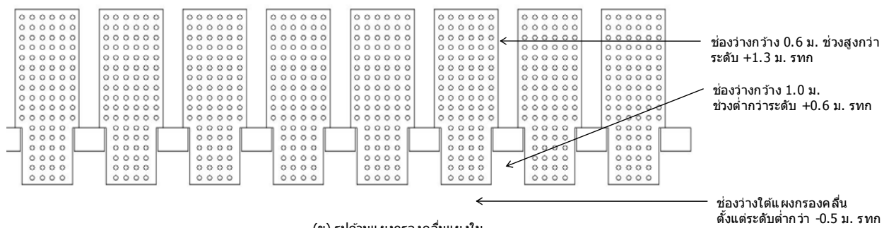
(ข) รูปด้านแผงกรองคสล.แผงใน
