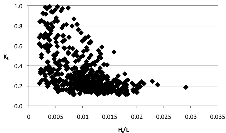
รูปที่ 5.18 ความสัมพันธ์ระหว่าง H_t/L กับ K_t
