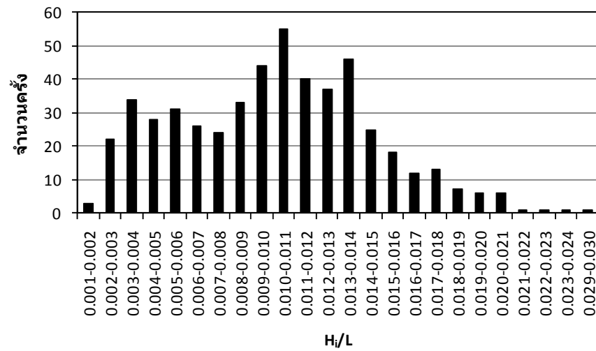
รูปที่ 5.11 ลักษณะการกระจายตัวของความชันคลื่น ( H_i/L )
