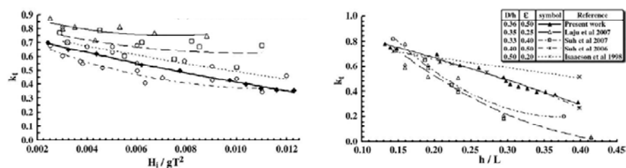
รูปที่ 3.19 การศึกษาความสัมพันธ์ระหว่างค่าสัมประสิทธิ์การส่งผ่านคลื่นกับคุณสมบัติคลื่น ( H_1/gT^2 ) และอัตราส่วนความลึกน้ำต่อความยาวคลื่น ( h/L ) ของ Rageh and Koriem (2010)
