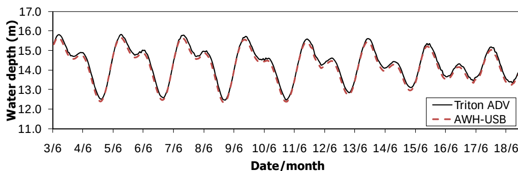
รูปที่ 5.7 การเปรียบเทียบความลึกน้ำตรวจวัดโดยไตรตัน เอดีวี กับเอดับบลิวเอช-ยูเอสบี
