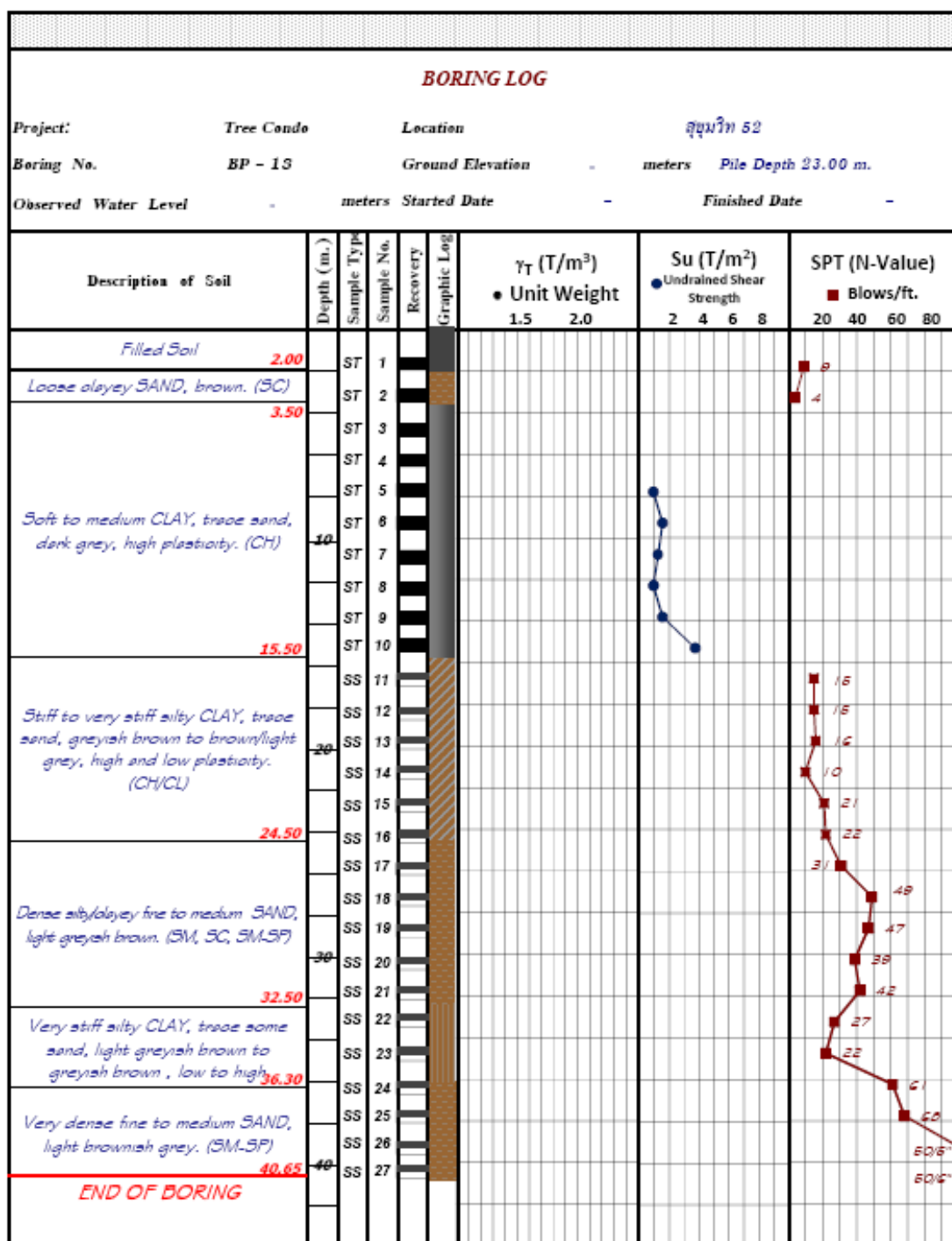
รูปที่ ค.13 ข้อมูลเจาะสำรวจชั้นดินของ โครงการ Tree Condo สุขุมวิท 52 (P - 13)
