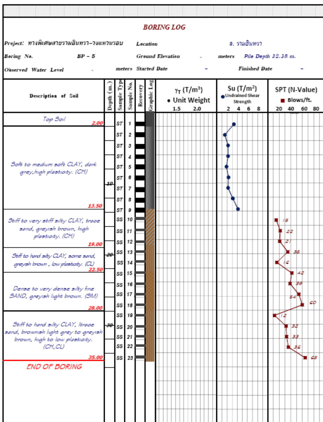
รูปที่ ก.5 ข้อมูลเจาะสำรวจชั้นดินของ โครงการทางพิเศษสายรามอินทรา - วงแหวนรอบนอก อ.รามอินทรา (P - 5)
