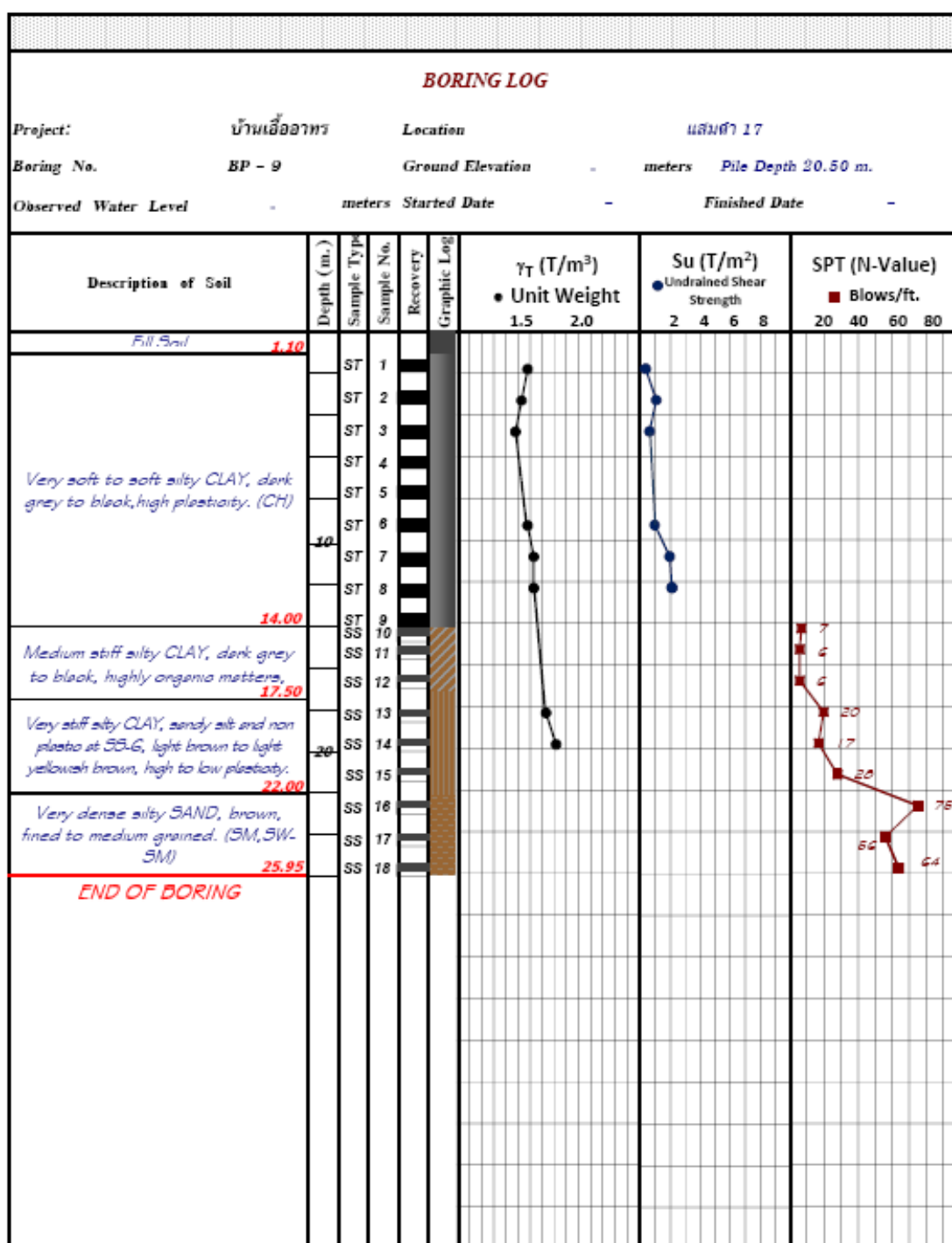
รูปที่ ก.9 ข้อมูลเจาะสำรวจชั้นดินของ โครงการบ้านเอื้ออาทร แสมดำ 17 (P - 9)
