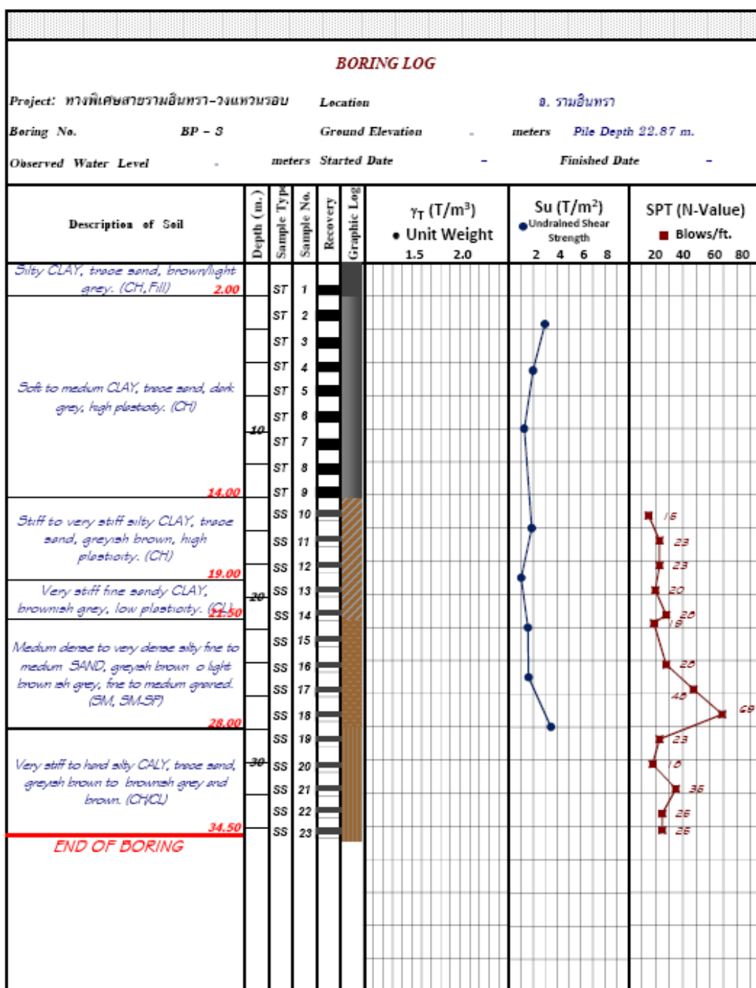
รูปที่ ก.3 ข้อมูลเจาะสำรวจชั้นดินของ โครงการทางพิเศษสายรามอินทรา - วงแหวนรอบนอก อ.รามอินทรา (P - 3)
