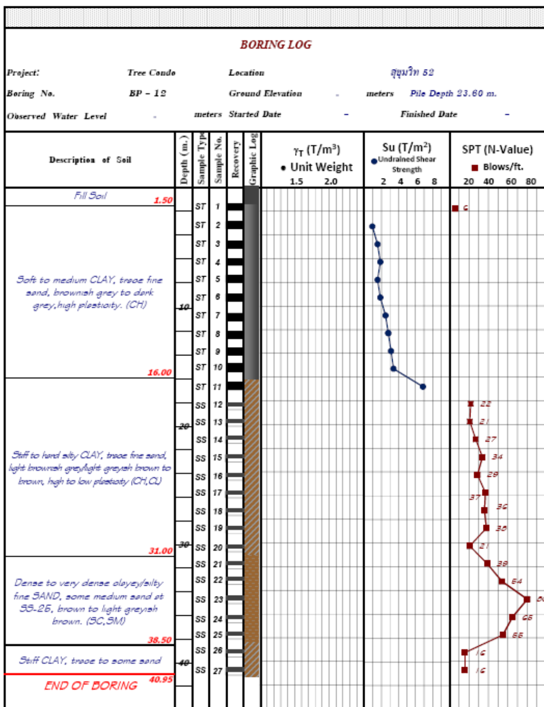
รูปที่ ค.12 ข้อมูลเจาะสำรวจชั้นดินของ โครงการ Tree Condo สุขุมวิท 52 (P - 12)
