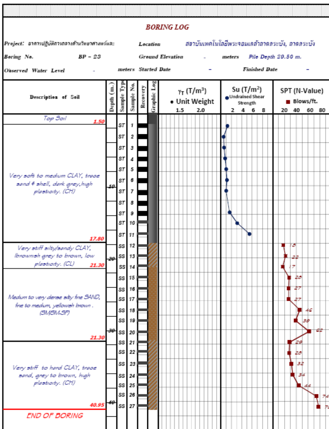
รูปที่ ค.18 ข้อมูลเจาะสำรวจชั้นดินของ โครงการอาคารปฏิบัติการกลางด้านวิทยาศาสตร์และ เทคโนโลยี สจล. ลาดกระบัง (P - 23)
