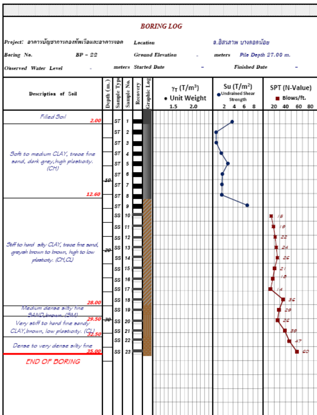
รูปที่ ค.17 ข้อมูลเจาะสำรวจชั้นดินของ โครงการอาคารบัญชาการกองทัพอากาศและอาคารจอด อ.อิสรภาพ บางกอกน้อย (P - 22)
