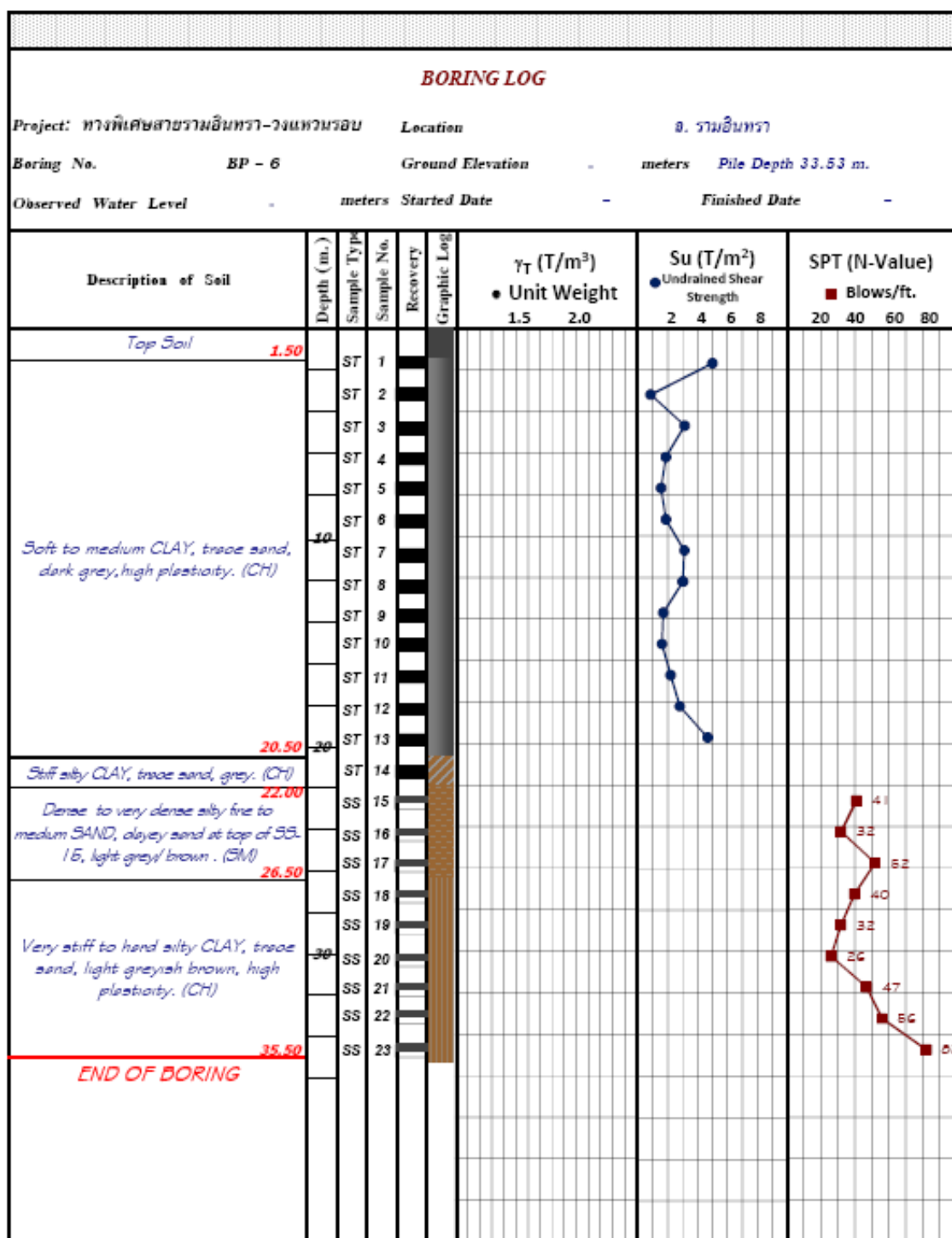
รูปที่ ก.6 ข้อมูลเจาะสำรวจชั้นดินของ โครงการทางพิเศษสายรามอินทรา - วงแหวนรอบนอก อ.รามอินทรา (P - 6)
