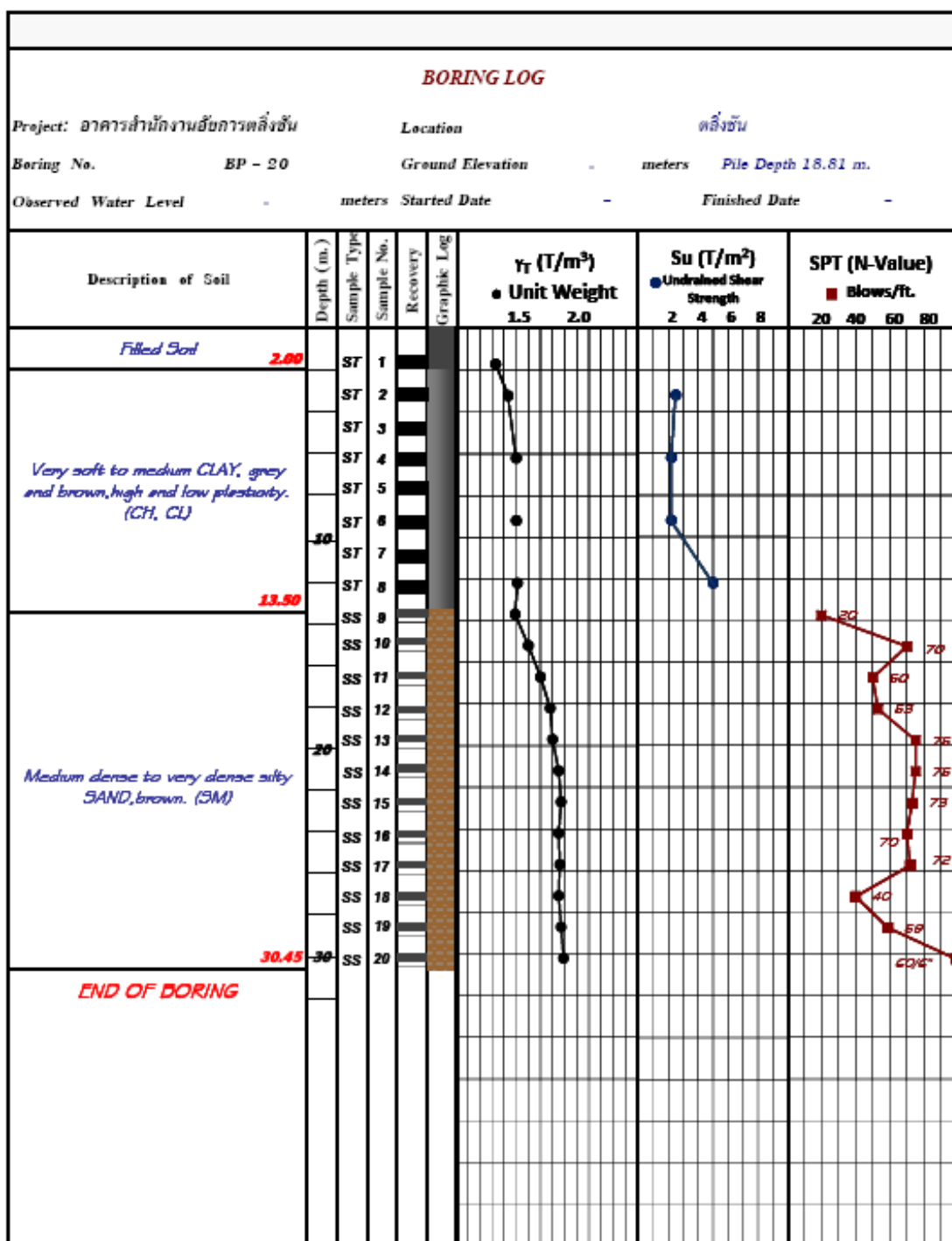
รูปที่ ก.15 ข้อมูลเจาะสำรวจชั้นดินของ โครงการอาคารสำนักงานตลิ่งชัน (P - 20)
