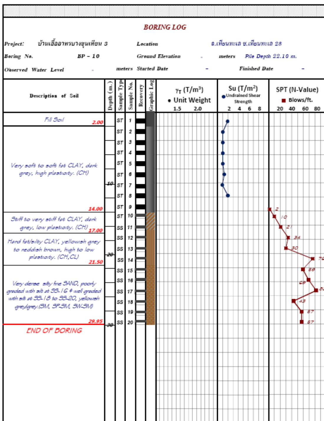
รูปที่ ค.10 ข้อมูลเจาะสำรวจชั้นดินของ โครงการบ้านเอื้ออาทร บางขุนเทียน 3 ช.เทียนทะเล 28
