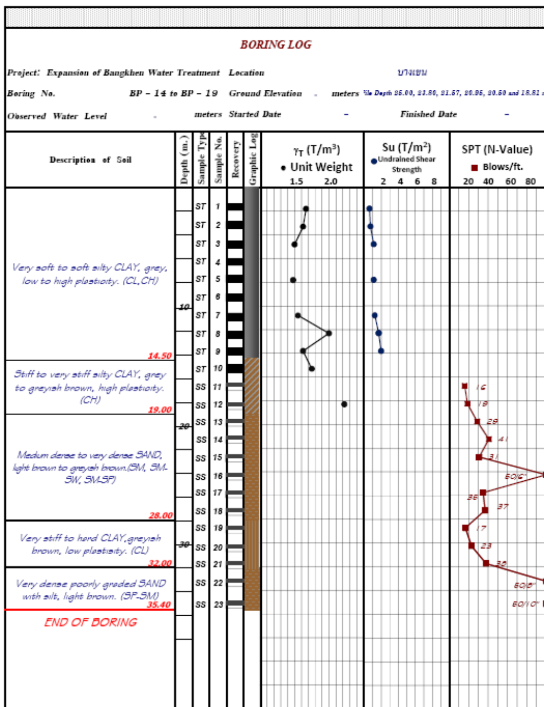
รูปที่ ค.14 ข้อมูลเจาะสำรวจชั้นดินของ โครงการ Expansion of Bangkhen Water Treatment บางเขน (P - 14 ถึง P-19)
