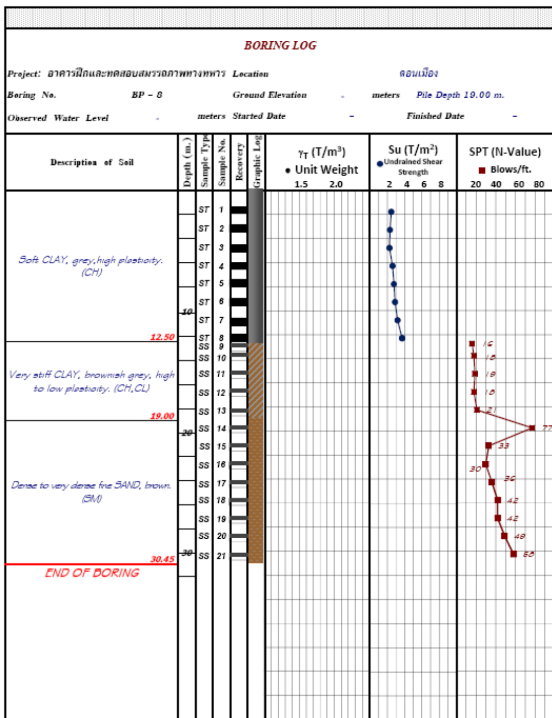
รูปที่ ค.8 ข้อมูลเจาะสำรวจชั้นดินของ โครงการอาคารฝึกและทดสอบสมรรถภาพทางทหาร ดอนเมือง (P - 8)
