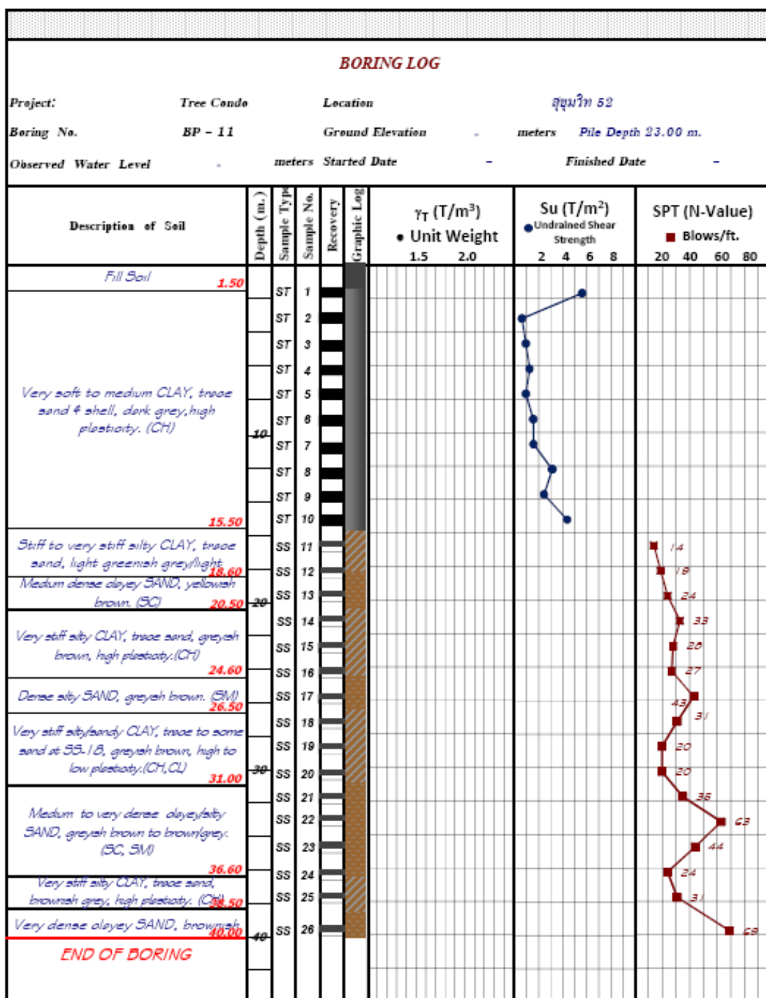
รูปที่ ค.11 ข้อมูลเจาะสำรวจชั้นดินของ โครงการ Tree Condo สุขุมวิท 52 (P - 11)
