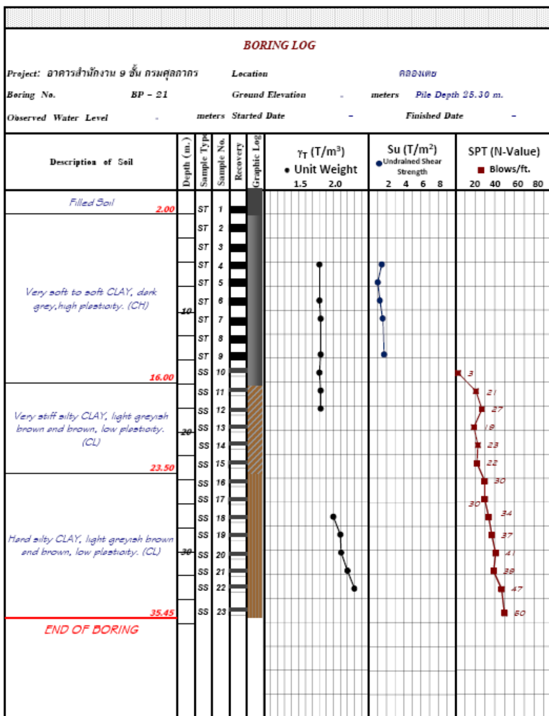
รูปที่ ค.16 ข้อมูลเจาะสำรวจชั้นดินของ โครงการอาคารสำนักงาน 9 ชั้น กรมศุลกากร คลองเตย
