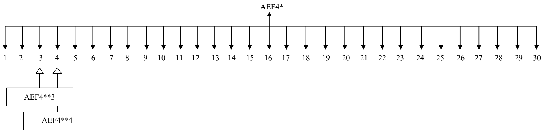
แผนภาพที่ ค.2 การแยกสารสกัดจากผักกูดด้วยวิธีคอลัมน์โครมาโทกราฟีของเฟรคชั่น AEF4*
