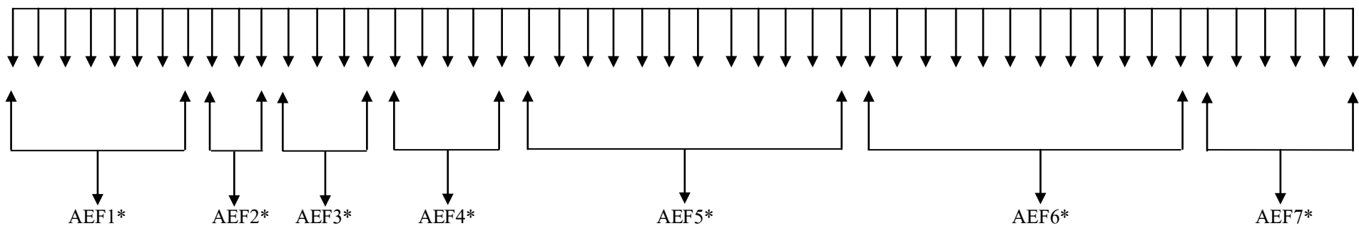
แผนภาพที่ ค.1 การแยกสารสกัดจากผักกูดด้วยวิธีคอลัมน์โครมาโทกราฟี และแผ่นโครมาโทกราฟี
