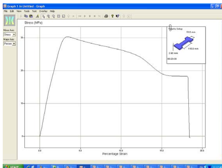
รูปที่ ก.3 ค่าความทนทานต่อแรงดึงของ PLA/PBSA ที่อัตราส่วน 80/20 ที่ปริมาณ PBAT 30 %โดยน้ำหนัก
