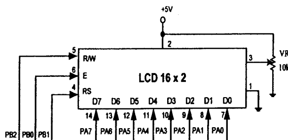
รูปที่ 3 วงจรการเชื่อมต่อแอลซีดี
