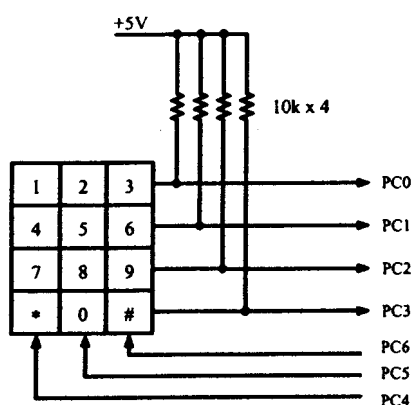
รูปที่ 2 วงจรอินพุตที่เป็นสวิตช์ต่อแบบเมตริกซ์
