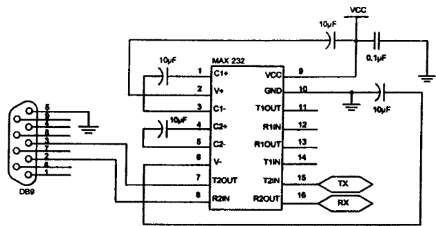
รูปที่ 5 วงจรการเชื่อมต่อพอร์ทอนุกรมมาตรฐาน RS-232
