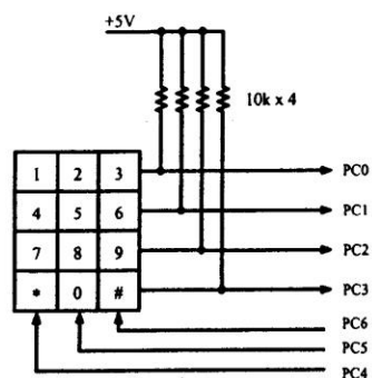
รูปที่ 2 วงจรอินพุตที่เป็นสวิตช์ต่อแบบเมตริกซ์ ตารางที่ 1 การกดคีย์
