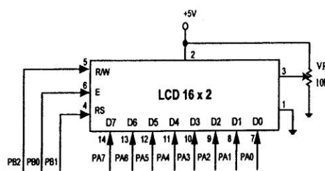
รูปที่ 3 วงจรการเชื่อมต่อแอลซีดี
