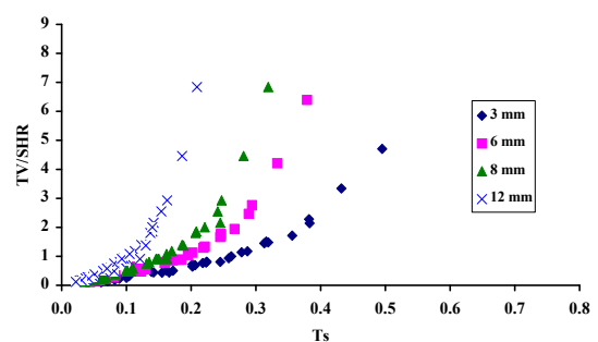
รูปที่ 5 ความสัมพันธ์ของค่าพารามิเตอร์ ( Tv/SHR ) กับค่าการส่งผ่านรังสีในช่วงรังสีแสงอาทิตย์ ( T_s ) ของกระจกสีเขียวติดฟิล์มทุกชนิดที่มีความหนา 3 6 8 และ 12 มม
