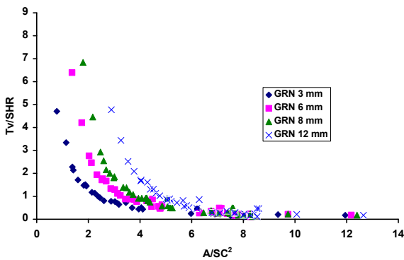
รูปที่ 8 ความสัมพันธ์ของค่าพารามิเตอร์ ( T_v/SHR ) กับอัตราส่วนค่าการดูดกลืนรังสีต่อค่าสัมประสิทธิ์บังเงากำลังสอง ( A/SC^2 ) ของกระจกสีเขียวติดฟิล์มทุกชนิดที่ความหนา 3 6 8 และ 12 มม
