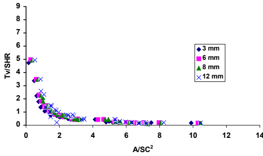
รูปที่ 6 ความสัมพันธ์ของค่าพารามิเตอร์ ( T_v/SHR ) กับอัตราส่วนค่าการดูดกลืนรังสีต่อค่าสัมประสิทธิ์บังเงากำลังสอง ( A/SC^2 ) ของกระจกใสติดฟิล์มทุกชนิดที่ความหนา 3 6 8 และ 12 มม
