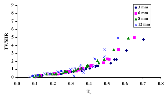
รูปที่ 3 ความสัมพันธ์ของค่าพารามิเตอร์ ( Tv/SHR ) กับค่าการส่งผ่านรังสีในช่วงรังสีแสงอาทิตย์ ( T_s ) ของกระจกใสติดฟิล์มทุกชนิดที่มีความหนา 3 6 8 และ 12 มม
