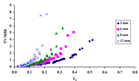
รูปที่ 4 ความสัมพันธ์ของค่าพารามิเตอร์ ( Tv/SHR ) กับค่าการส่งผ่านรังสีในช่วงรังสีแสงอาทิตย์ ( T_s ) ของกระจกสปีรอนซ์และสีเทาดิตฟิล์มทุกชนิดที่มีความหนา 3 6 8 และ 12 มม
