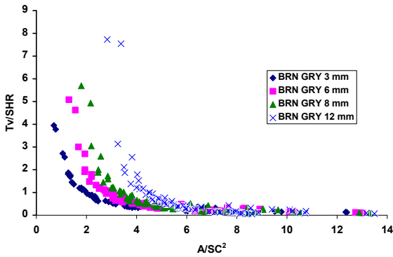
รูปที่ 7 ความสัมพันธ์ของค่าพารามิเตอร์ ( T_v/SHR ) กับอัตราส่วนค่าการดูดกลืนรังสีต่อค่าสัมประสิทธิ์บังเงากำลังสอง ( A/SC^2 ) ของกระจกสีบรอนซ์และสีเทาติดฟิล์มทุกชนิดที่ความหนา 3 6 8 และ 12 มม
