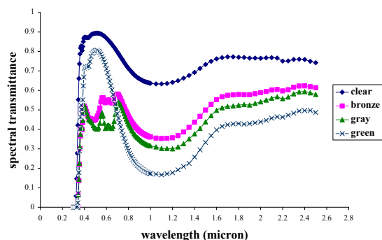
รูปที่ 1 ตัวอย่างของค่าการส่งผ่านรังสี ( T ) ที่แปรตามความยาวคลื่นของกระจกสีต่าง ๆ กันที่ความหนา 6 มม.
