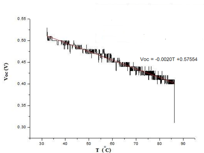
รูปที่4.6 กราฟแสดงความสัมพันธ์ระหว่างค่าแรงดันไฟฟ้าวงจรเปิด(V)กับอุณหภูมิของเซลล์แสงอาทิตย์( °C)
