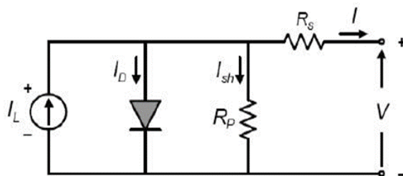
รูปที่2.5 การต่อวงจรสมมูลของเซลล์แสงอาทิตย์
