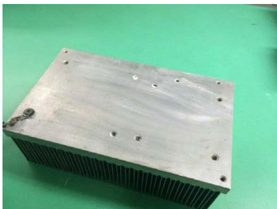
รูปที่ 3.3ข ฮีทซิงค์ขนาด 12 cm. x 19.5 cm. จำนวน 48 ครีบ แต่ละครีบมีความยาว 5.3 cm
