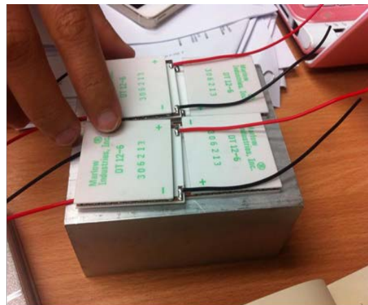
รูปที่3.16 การติดตั้งเทอร์โมอิเล็กทริกโมดูลบนฮีทซิงค์
