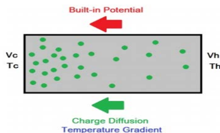
รูปที่ 2.8 ภาพการเคลื่อนที่ของพาหะข้างมากในสารกึ่งตัวนำที่มีอุณหภูมิสองด้านไม่เท่ากัน
