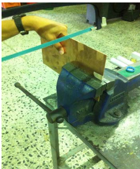
รูปที่3.14 การตัดแผ่นทองแดงด้วยเลื่อยตัดเหล็ก
