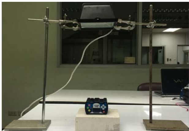
รูปที่ 4.1 อุปกรณ์การทดลองการหาค่าความเข้มแสงและสเปกตรัมของแหล่งกำเนิดแสง (ก) หลอดไฟ IP 65 E 40 ขนาด 400 W (ข) หลอดไฟ BEC Halogen Floodlight CQ 500D ขนาด 500 W
