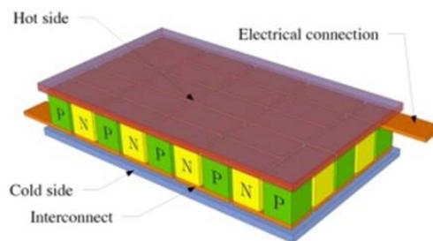
รูปที่ 2.9 โครงสร้างภายในของเทอร์โมอิเล็กทริกโมดูล
