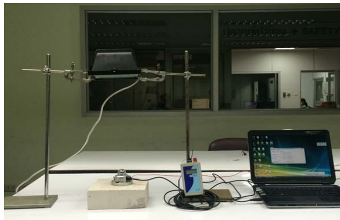
รูปที่ 4.3 อุปกรณ์การทดลองในการกำหนดระยะห่างของหลอดไฟ BEC Halogen Floodlight CQ 500D ขนาด 500 W กับเซลล์แสงอาทิตย์
