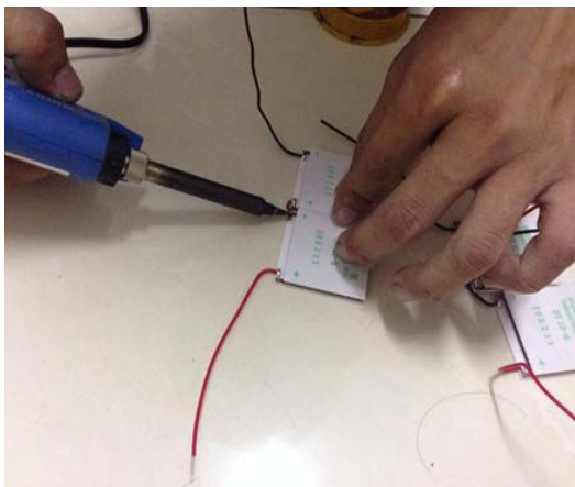
รูปที่3.16 การติดตั้งเทอร์โมอิเล็กทริกโมดูลบนฮีทซิงค์
