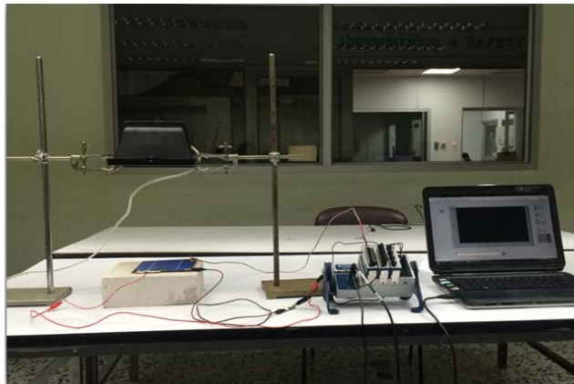
รูปที่ 4.5 อุปกรณ์การทดลองในการบันทึกค่าแรงดันไฟฟ้าวงจรเปิด (V) และอุณหภูมิ ( ^{\circ}\text{C} ) ของเซลล์แสงอาทิตย์
