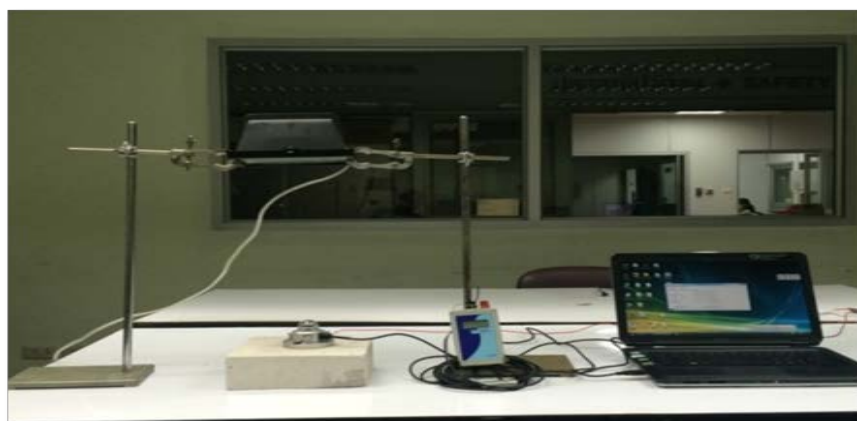
รูปที่ 3.20 อุปกรณ์การทดลองการกำหนดระยะห่างของหลอดไฟ BEC Halogen Floodlight CQ500D ขนาด 500 W กับ แผงเซลล์แสงอาทิตย์
