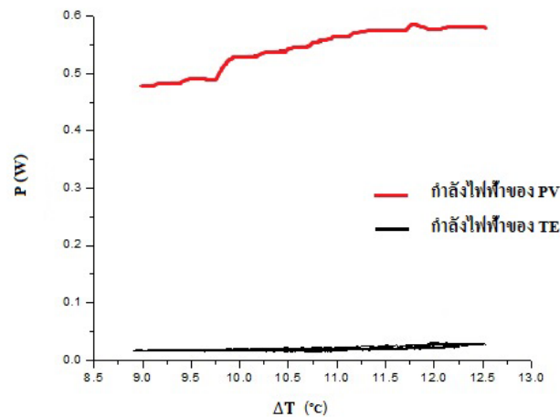
รูปที่4.11 กราฟแสดงความสัมพันธ์ระหว่าง \Delta T ( °C)กับค่ากำลังไฟฟ้าที่ได้ (W) เมื่อเปลี่ยนขนาดของฮีทซิงค์
