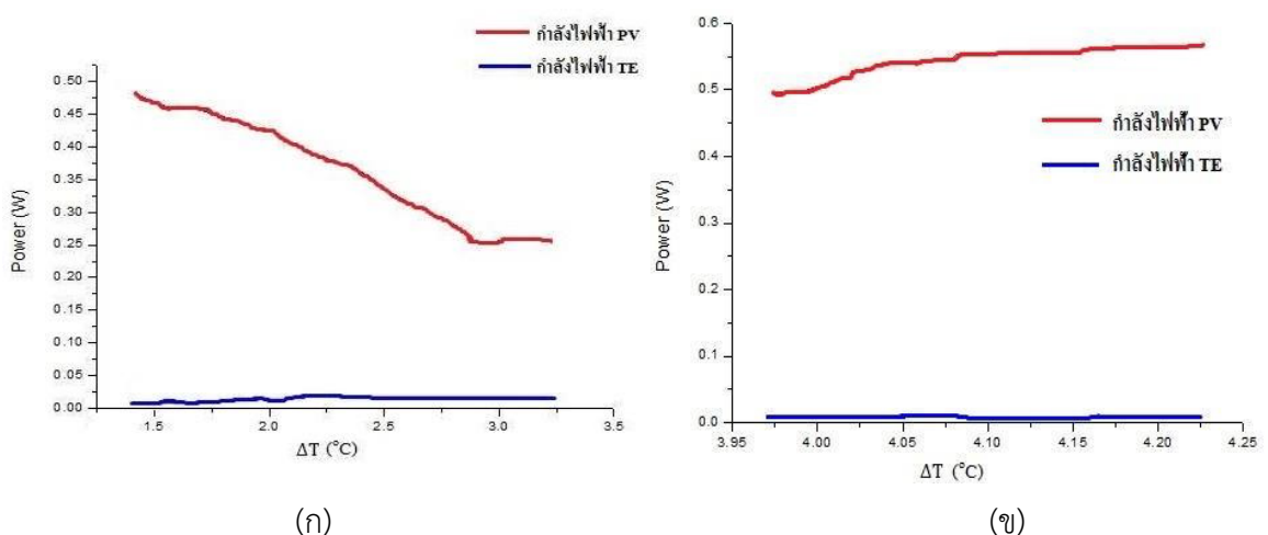
รูปที่4.10 กราฟแสดงความสัมพันธ์ระหว่าง \Delta T กับค่ากำลังไฟฟ้าที่ได้ (W) (ก) กำลังไฟฟ้าที่ได้จากระบบรวมแบบไม่มีพัลลภระบายความร้อน (ข) กำลังไฟฟ้าที่ได้จากระบบรวมแบบมีพัลลภระบายความร้อน
