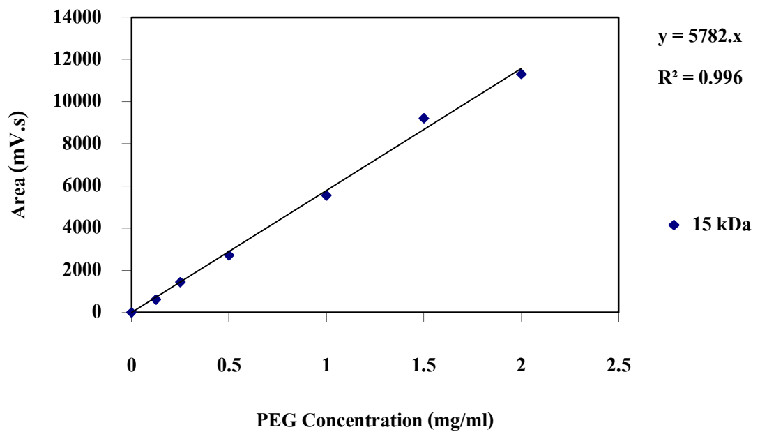
รูปที่ ข.2 กราฟเปรียบเทียบระหว่างความเข้มข้น PEG 15 kDa กับพื้นที่ใต้กราฟ (mV.s)
