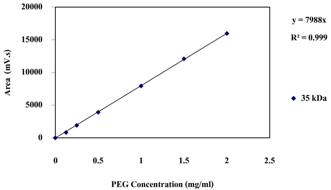
รูปที่ ข.3 กราฟเปรียบเทียบระหว่างความเข้มข้น PEG 35 kDa กับพื้นที่ใต้กราฟ (mV.s)
