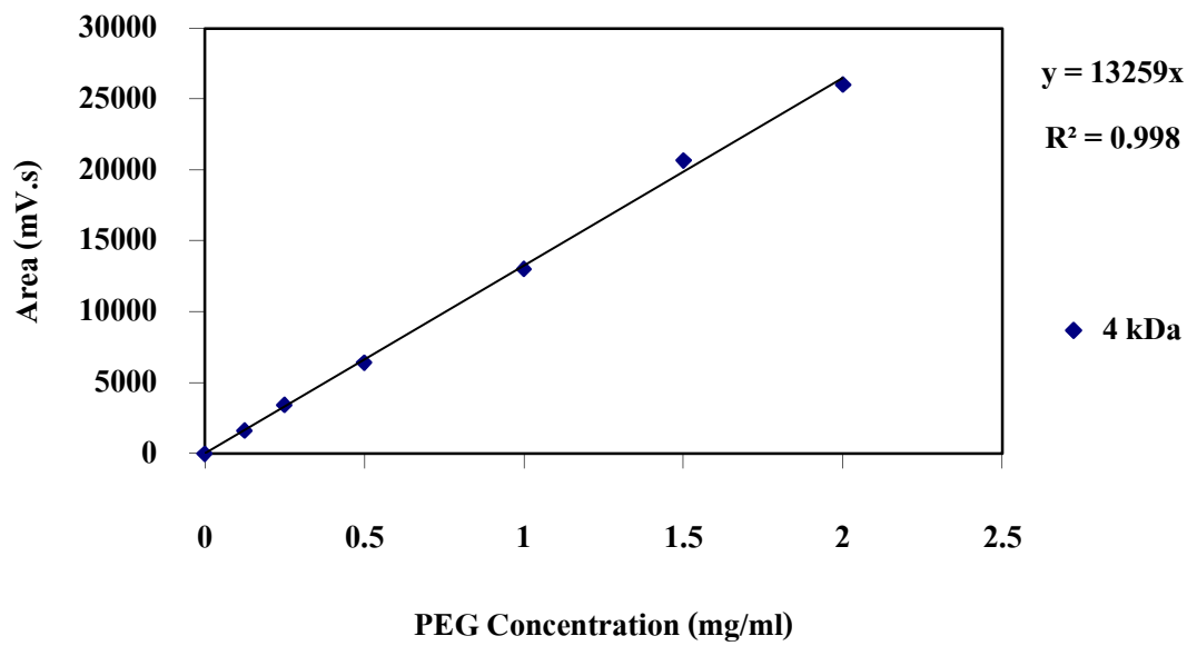
รูปที่ ข.1 กราฟเปรียบเทียบระหว่างความเข้มข้น PEG 4 kDa กับพื้นที่ใต้กราฟ (mV.s)
