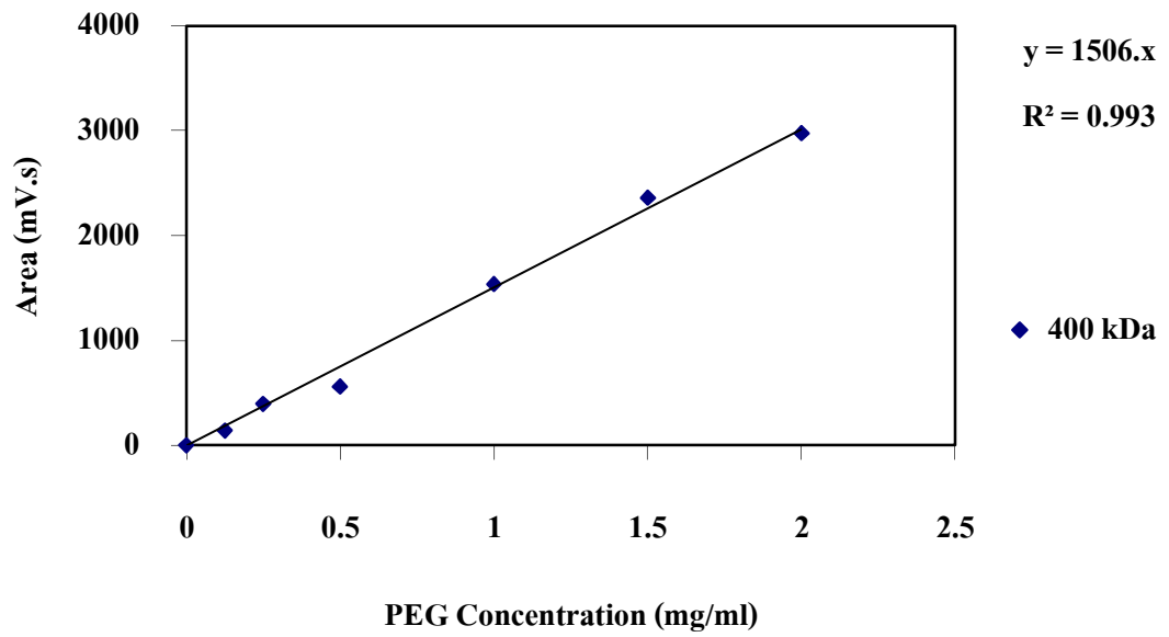
รูปที่ ข.5 กราฟเปรียบเทียบระหว่างความเข้มข้น PEG 400 kDa กับพื้นที่ใต้กราฟ (mV.s)
