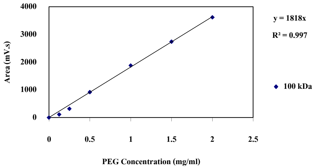
รูปที่ ข.4 กราฟเปรียบเทียบระหว่างความเข้มข้น PEG 100 kDa กับพื้นที่ใต้กราฟ (mV.s)
