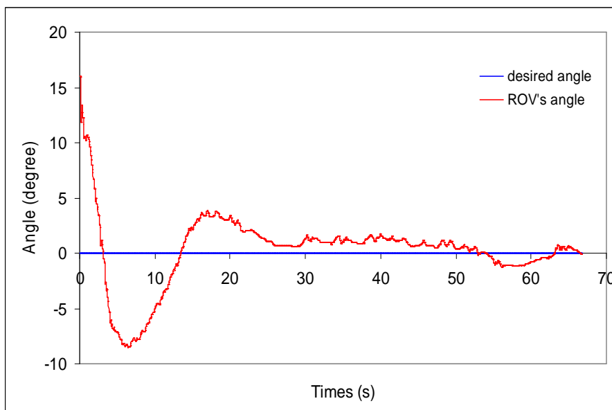
รูปที่ จ.2 การติดตามการควบคุมแบบพีไอดีที่ 0 องศา
