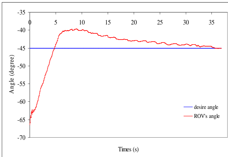
รูปที่ จ.3 การติดตามการควบคุมแบบพีไอดีที่ -45 องศา
