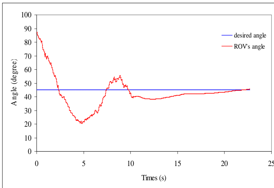
รูปที่ จ.1 การติดตามการควบคุมแบบพีไอดีที่ 45 องศา
