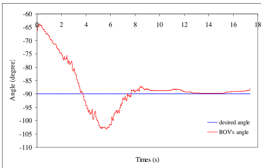
รูปที่ จ.4 การติดตามการควบคุมแบบพีไอดีที่ -90 องศา
