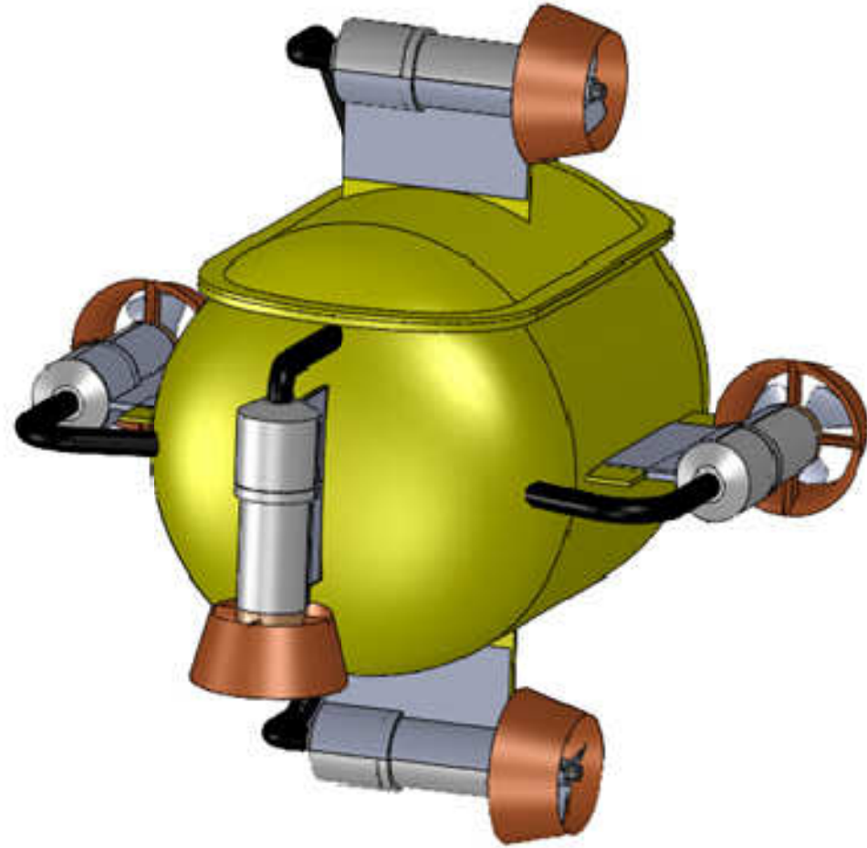
รูปที่ ข.1 รายละเอียดของยานใต้น้ำขนาดเล็ก
