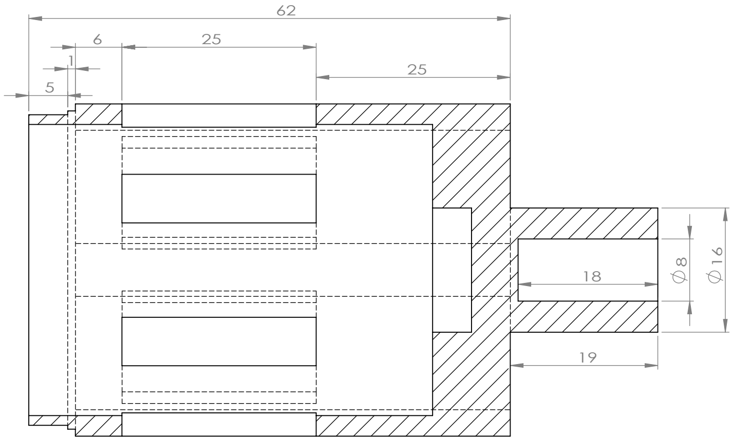
SECTION I-I SCALE 2 : 1
