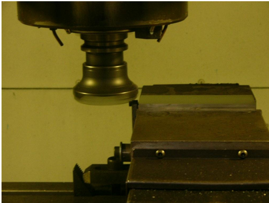
รูปที่ ค.6 การจับยึดชิ้นงาน เข้ากับเครื่องกัดซีเอ็นซี
