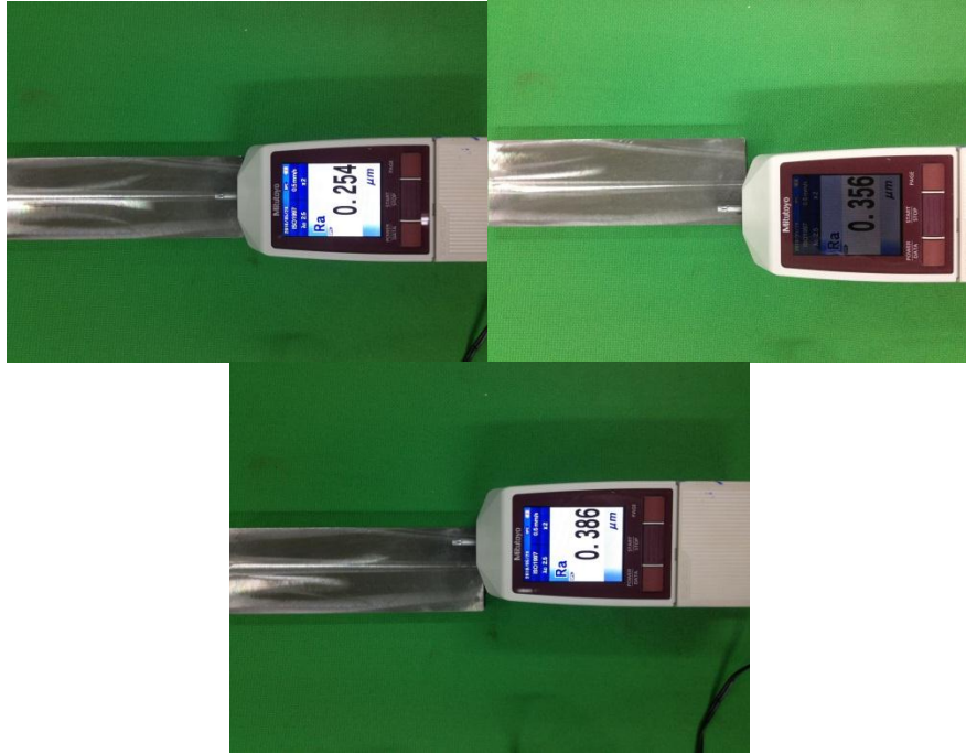
รูปที่ ค.9 การวัดค่าความเรียบผิวงานตำแหน่งที่ 1
