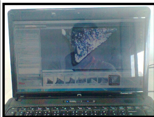
รูปที่ ๓.๔ แสดงการใช้กล้องจุลทรรศน์ถ่ายภาพการสีกหรือของพื้นผิว
