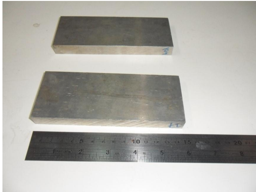
รูปที่ ค.5 แท่งอะลูมิเนียมผสมที่ผ่านการบ่มแข็ง
