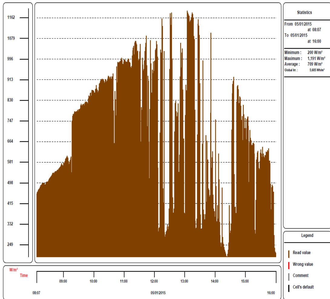
รูปที่ ก.3.1 พลังงานแสงอาทิตย์ที่วัดได้ วันที่ 5 มกราคม 2558
