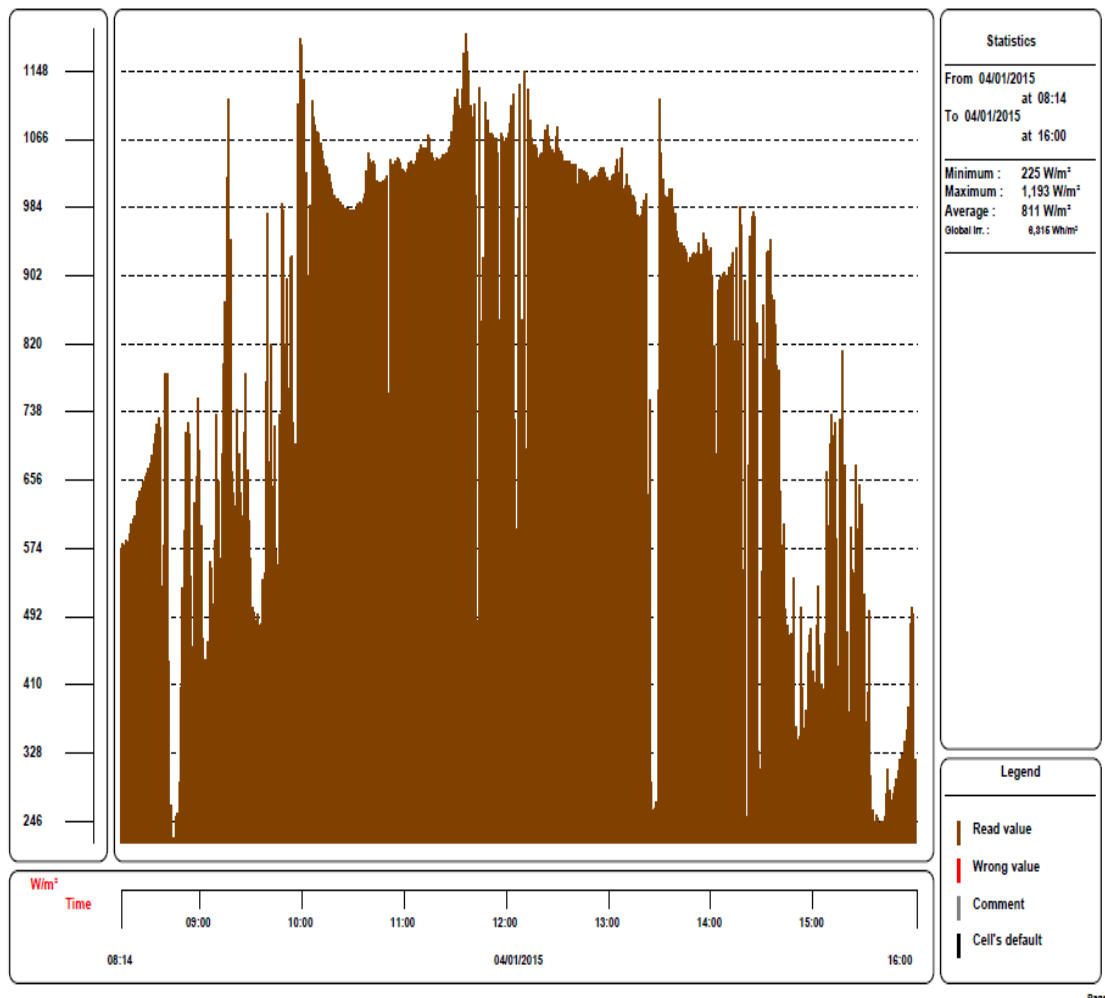
รูปที่ ก.2.1 พลังงานแสงอาทิตย์ที่วัดได้ วันที่ 4 มกราคม 2558
