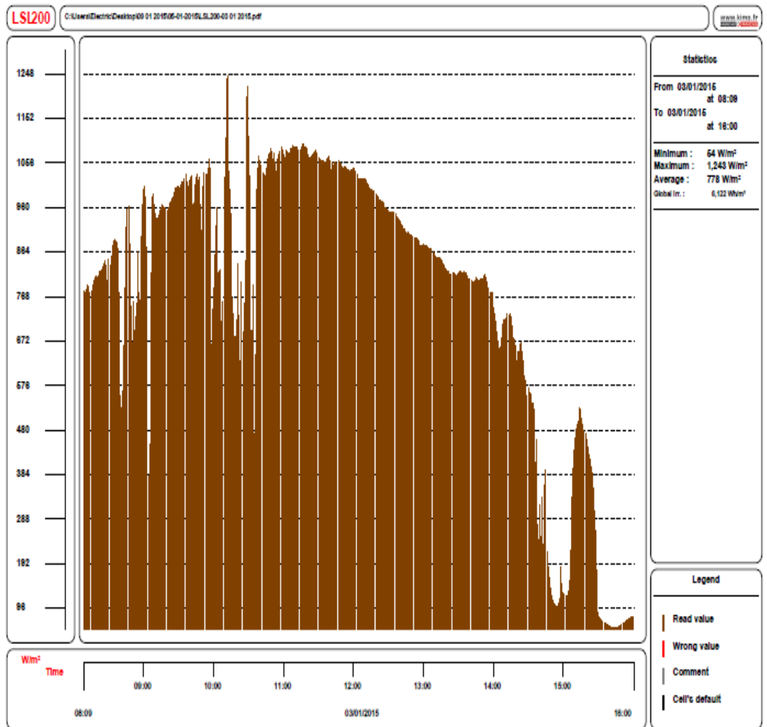
รูปที่ ก.1.2 พลังงานแสงอาทิตย์ที่วัดได้ วันที่ 3 มกราคม 2558
