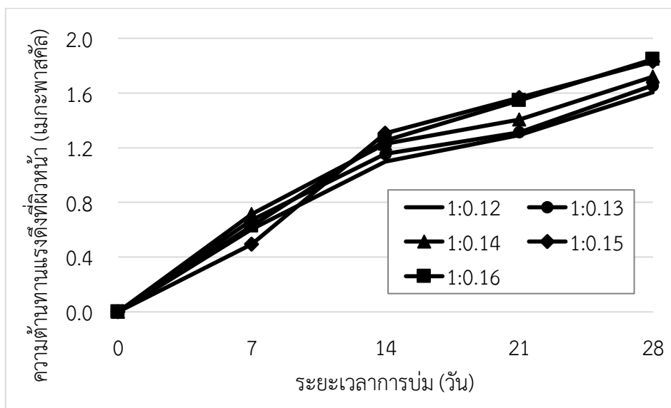
รูปที่ 4.12 ความต้านทานแรงดึงตั้งฉากกับผิวหน้าของแผ่นซีเมนต์บอร์ดจากเถ้ากะลามะพร้าว ที่อายุการบ่ม 28 วัน
