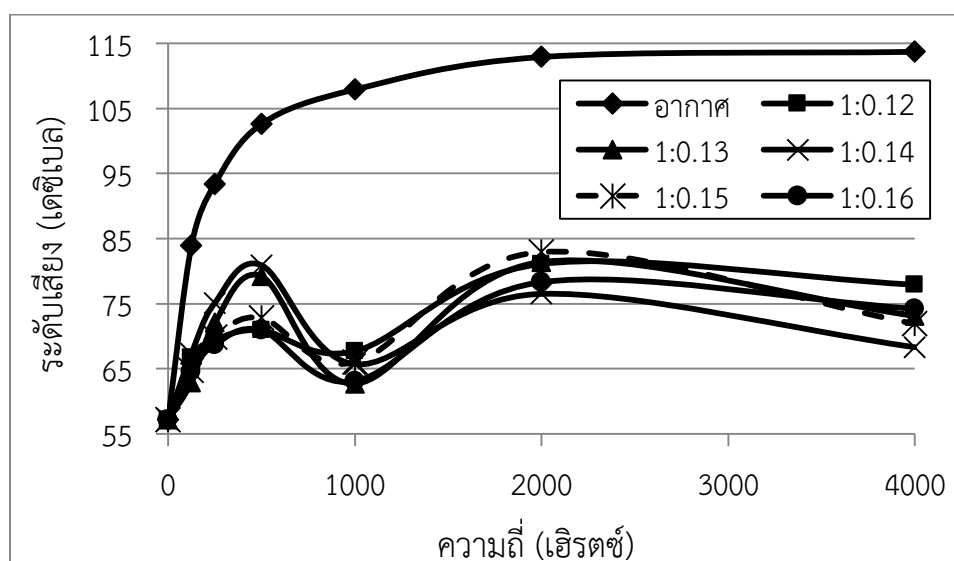
รูปที่ 4.14 ระดับเสียงที่ผ่านแผ่นซีเมนต์บอร์ดจากเถ้ากะลามะพร้าวออกจากห้องจำลอง ที่อายุการบ่ม 28 วัน
