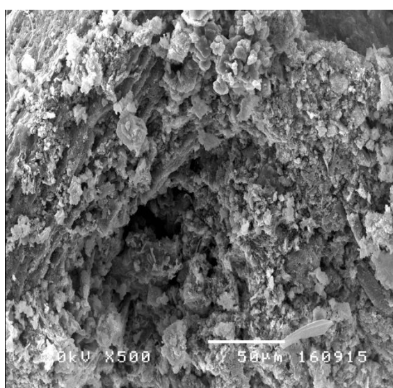
รูปที่ 4.6 ภาพขยายของแผ่นซีเมนต์บอร์ดจากเก้าอี้กาะมะพร้าวด้วยกล้องจุลทรรศน์อิเล็กตรอนแบบส่องกราด (SEM) ที่กำลังขยาย 500 เท่า
