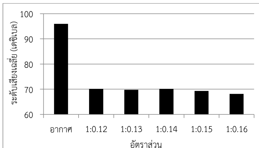
รูปที่ 4.15 ระดับเสียงเฉลี่ยที่ผ่านแผ่นซีเมนต์บอร์ดจากเก้าะลามาพร้าวออกจากห้องจำลอง ที่อายุการบ่ม 28 วัน
