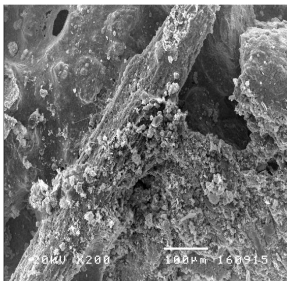
รูปที่ 4.5 ภาพขยายของแผ่นซีเมนต์บอร์ดจากเก้าอี้กาะมะพร้าวด้วยกล้องจุลทรรศน์อิเล็กตรอนแบบส่องกราด (SEM) ที่กำลังขยาย 200 เท่า
