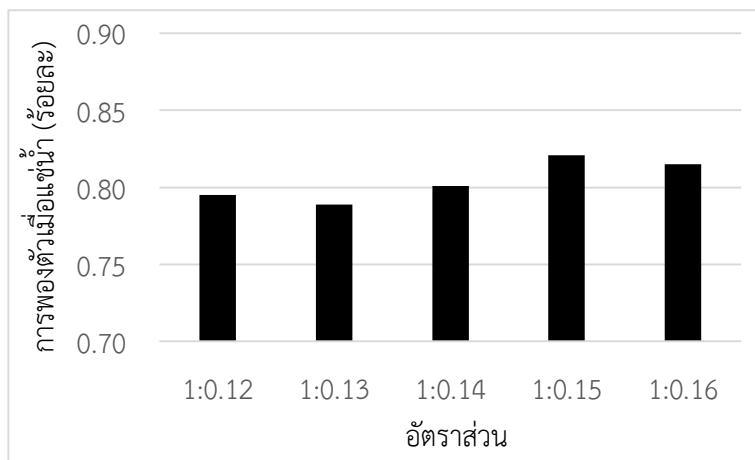
รูปที่ 8 การพองตัวเมื่อแช่น้ำของแผ่นซีเมนต์บอร์ดจากเถ้ากะลามะพร้าว ที่อายุการบ่ม 28 วัน
