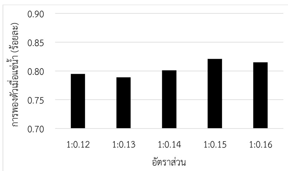
รูปที่ 4.9 การพองตัวเมื่อแช่น้ำของแผ่นซีเมนต์บอร์ดจากเถ้ากะลามาพร้าว ที่อายุการบ่ม 28 วัน
