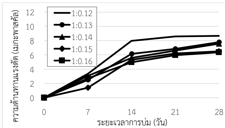
รูปที่ 11 ความต้านทานแรงดัดของแผ่นซีเมนต์บอร์ดจากเถ้ากะลามะพร้าว ที่อายุการบ่ม 28 วัน
