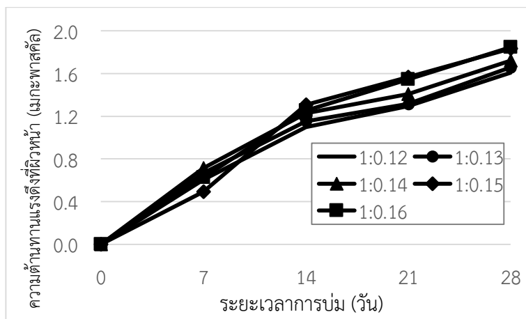
รูปที่ 13 ความต้านทานแรงดึงตั้งฉากกับผิวหน้าของแผ่นซีเมนต์บอร์ดจากเถ้ากละมะพร้าว ที่อายุการบ่ม 28 วัน
