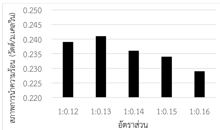
รูปที่ 10 สภาพการนำความร้อนของแผ่นซีเมนต์บอร์ดจากเถ้ากะลามะพร้าว ที่อายุการบ่ม 28 วัน
