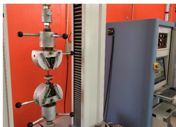
รูปที่ 3.31 การติดตั้งชิ้นส่วนแผ่นซีเมนต์บอร์ดจากเถ้ากะลามะพร้าวสำหรับทดสอบ ความต้านทานแรงดึงตั้งฉากที่ผิวหน้าด้วยเครื่องทดสอบอเนกประสงค์
