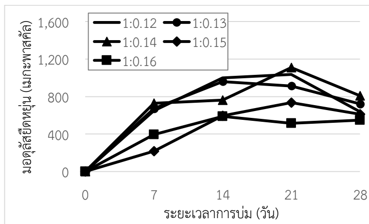
รูปที่ 12 มอดุลัสยืดหยุ่นของแผ่นซีเมนต์บอร์ดจากเถ้ากะลามะพร้าว ที่อายุการบ่ม 28 วัน
