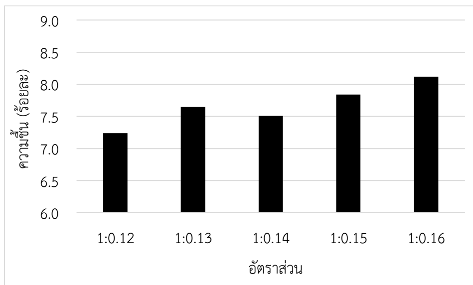
รูปที่ 4.8 ความชื้นของแผ่นซีเมนต์บอร์ดจากเถ้ากะลามาพร้าว ที่อายุการบ่ม 28 วัน
