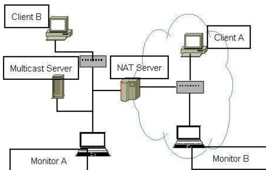
ภาพที่ 3.1 แสดงเครือข่ายจำลองที่ใช้ในการทดสอบ
