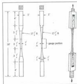
ภาพภาพที่ 2.6 แสดงการทดสอบความเค้นดึงขนานเส้นใย
