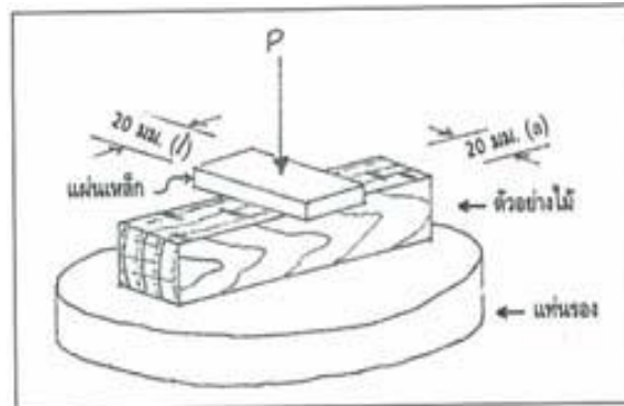
ภาพที่ 2.5 แสดงการทดสอบความเค้นอัดตั้งฉากเส้นใย
