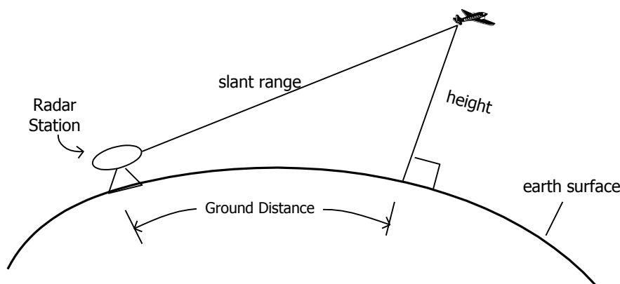
รูปที่ 2.2 การตรวจจับเป้าวัตถุของระบบเรดาร์
