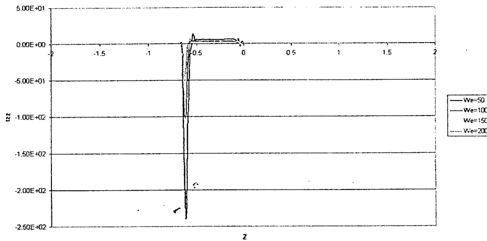
(d) Normal stress T_{zz} at top surface
