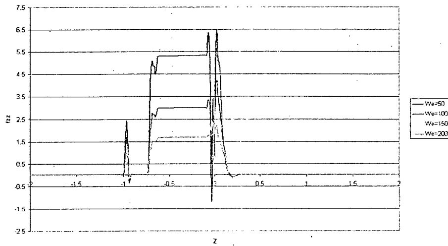
(d) Normal stress T_{zz} at bottom surface
