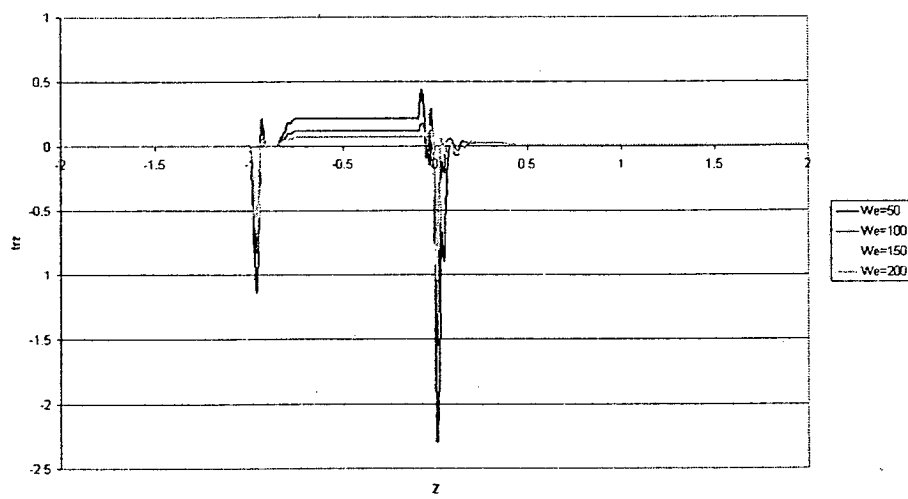
(c) Shear stress Trz at bottom surface
