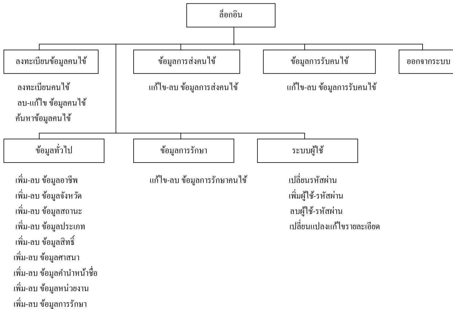
รูป 3.7 เมนูและรายการคำสั่งในส่วนผู้ควบคุมระบบ
