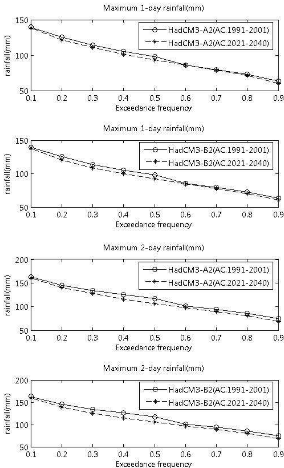
ภาพที่ ข.77 ปริมาณฝนสูงสุด 1 วัน และ 2 วัน ที่สังเคราะห์ได้จากภาพฉาย HadCM3-A2 และ HadCM3-B2 สำหรับสถานี 436005 (ปี ค.ศ. 1991-2001 และ ปี ค.ศ. 2021-2040)
