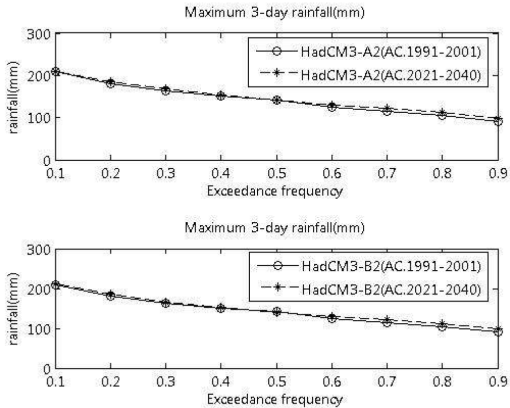
ภาพที่ ข.30 ปริมาณฝนสูงสุด 3 วัน ที่สังเคราะห์ได้จากภาพฉาย HadCM3-A2 และ HadCM3-B2 สำหรับสถานี 21190 (ปี ค.ศ. 1991-2001 และ ปี ค.ศ. 2021-2040)
