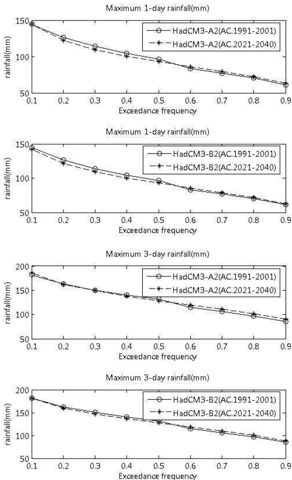
ภาพที่ ข.63 ปริมาณฝนสูงสุด 1 วัน และ 2 วัน ที่สังเคราะห์ได้จากภาพฉาย HadCM3-A2 และ HadCM3-B2 สำหรับสถานี 407015 (ปี ค.ศ. 1991-2001 และ ปี ค.ศ. 2021-2040)
