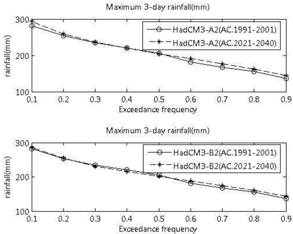
ภาพที่ ข.56 ปริมาณฝนสูงสุด 3 วัน ที่สังเคราะห์ได้จากภาพฉาย HadCM3-A2 และ HadCM3-B2 สำหรับสถานี 406005 (ปี ค.ศ. 1991-2001 และ ปี ค.ศ. 2021-2040)
