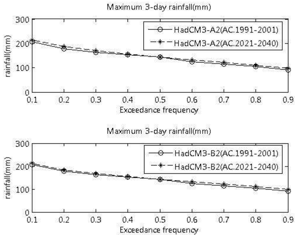
ภาพที่ ข.18 ปริมาณฝนสูงสุด 3 วัน ที่สังเคราะห์ได้จากภาพฉาย HadCM3-A2 และ HadCM3-B2 สำหรับสถานี 11210 (ปี ค.ศ. 1991-2001 และ ปี ค.ศ. 2021-2040)
