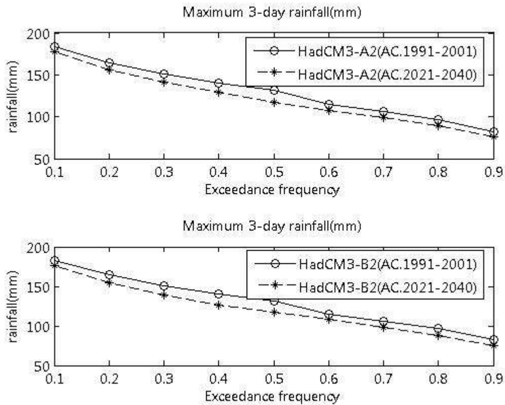
ภาพที่ ข.78 ปริมาณฝนสูงสุด 3 วัน ที่สังเคราะห์ได้จากภาพฉาย HadCM3-A2 และ HadCM3-B2 สำหรับสถานี 436005 (ปี ค.ศ. 1991-2001 และ ปี ค.ศ. 2021-2040)
