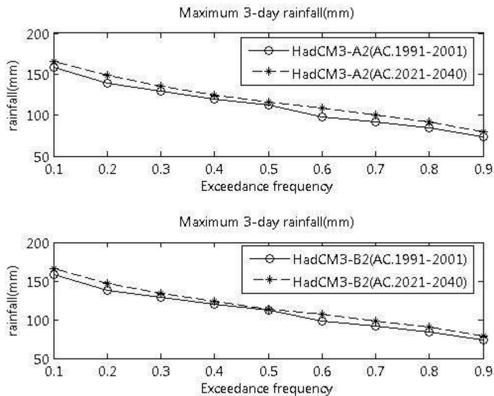
ภาพที่ ข.58 ปริมาณฝนสูงสุด 3 วัน ที่สังเคราะห์ได้จากภาพฉาย HadCM3-A2 และ HadCM3-B2 สำหรับสถานี 407002 (ปี ค.ศ. 1991-2001 และ ปี ค.ศ. 2021-2040)
