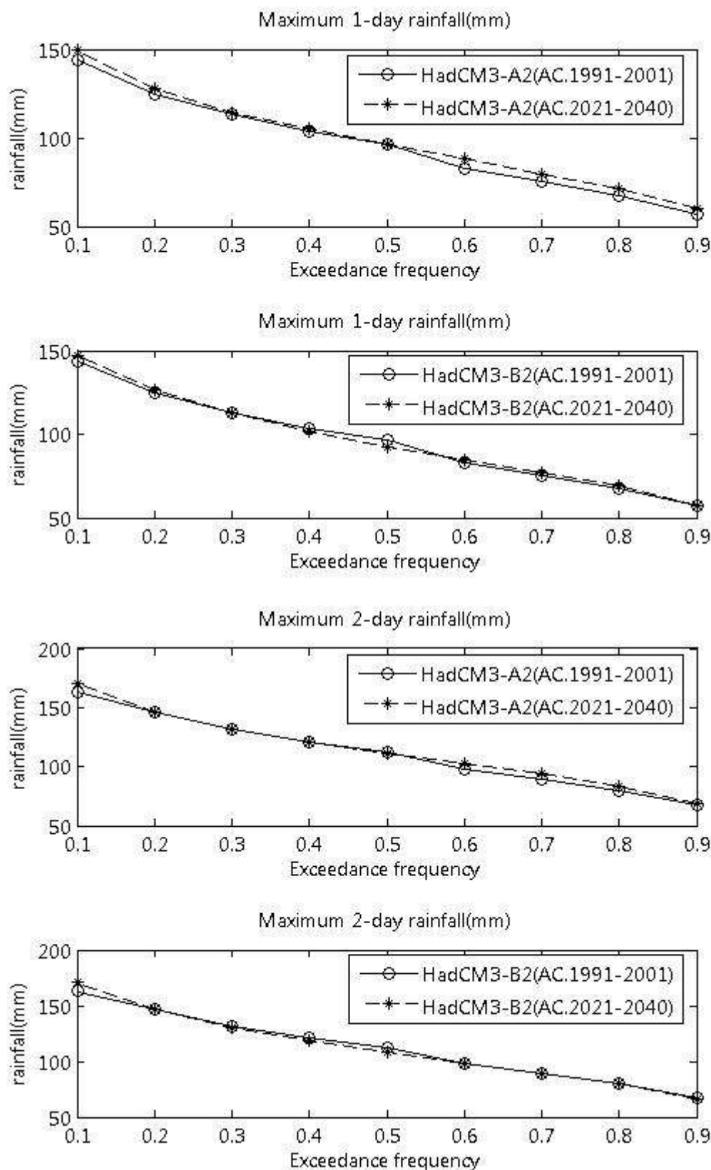
ภาพที่ ข.37 ปริมาณฝนสูงสุด 1 วัน และ 2 วัน ที่สังเคราะห์ได้จากภาพฉาย HadCM3-A2 และ HadCM3-B2 สำหรับสถานี 68150 (ปี ค.ศ. 1991-2001 และ ปี ค.ศ. 2021-2040)
