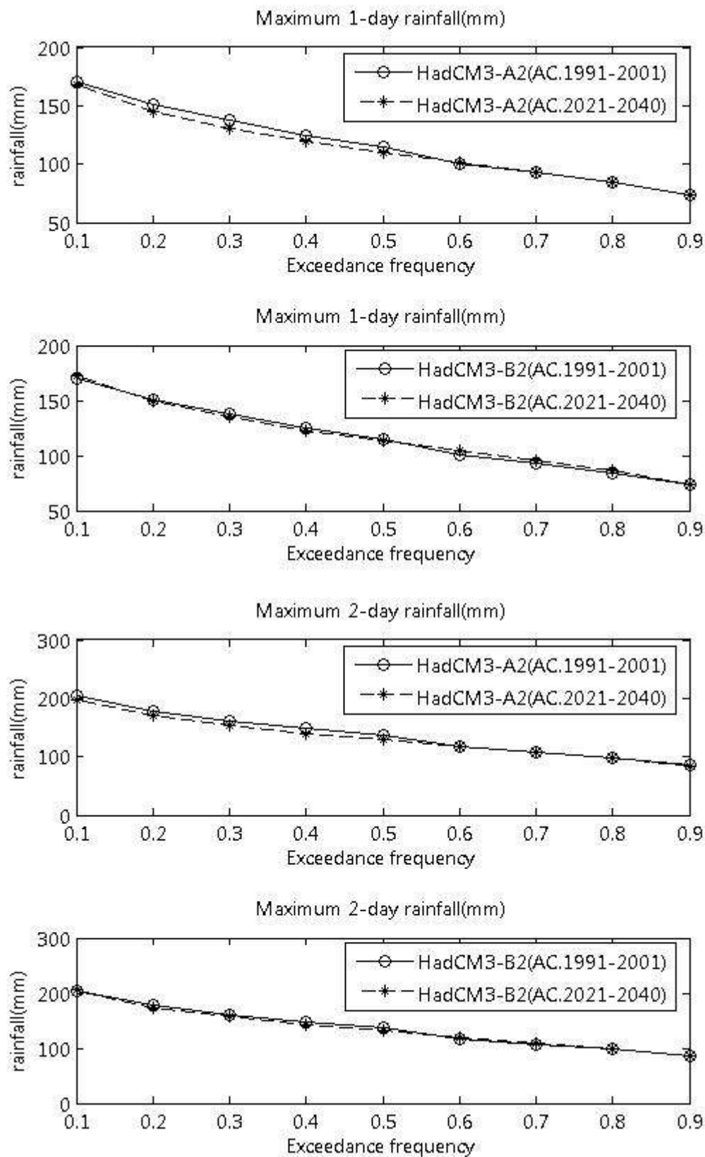
ภาพที่ ข.33 ปริมาณฝนสูงสุด 1 วัน และ 2 วัน ที่สังเคราะห์ได้จากภาพฉาย HadCM3-A2 และ HadCM3-B2 สำหรับสถานี 49062 (ปี ค.ศ. 1991-2001 และ ปี ค.ศ. 2021-2040)
