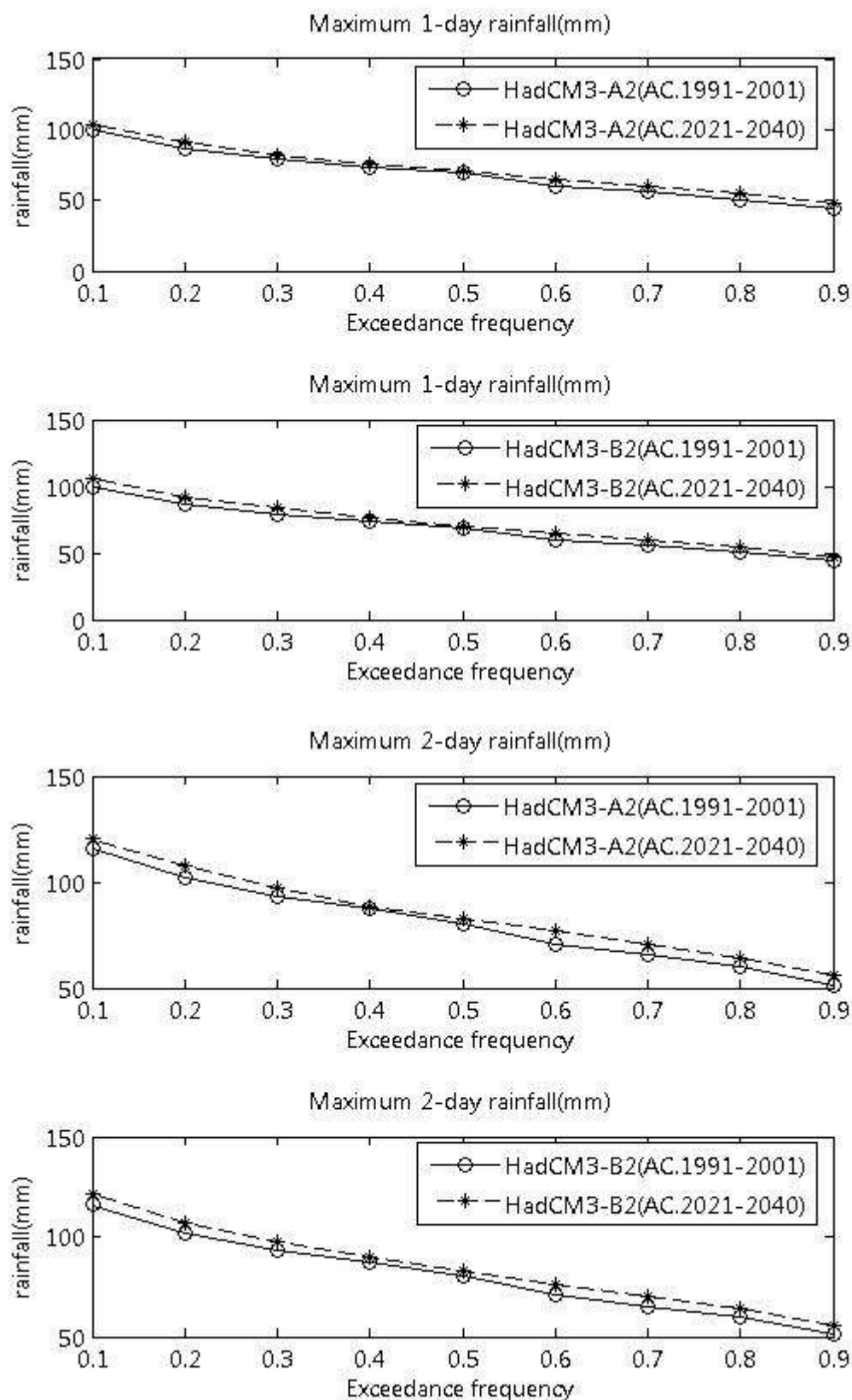
ภาพที่ ข.19 ปริมาณฝนสูงสุด 1 วัน และ 2 วัน ที่สังเคราะห์ได้จากภาพฉาย HadCM3-A2 และ HadCM3-B2 สำหรับสถานี 14052 (ปี ค.ศ. 1991-2001 และ ปี ค.ศ. 2021-2040)
