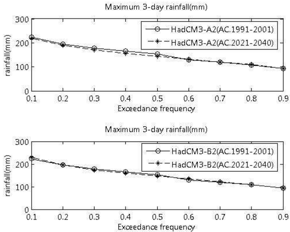
ภาพที่ ข.34 ปริมาณฝนสูงสุด 3 วัน ที่สังเคราะห์ได้จากภาพฉาย HadCM3-A2 และ HadCM3-B2 สำหรับสถานี 49062 (ปี ค.ศ. 1991-2001 และ ปี ค.ศ. 2021-2040)
