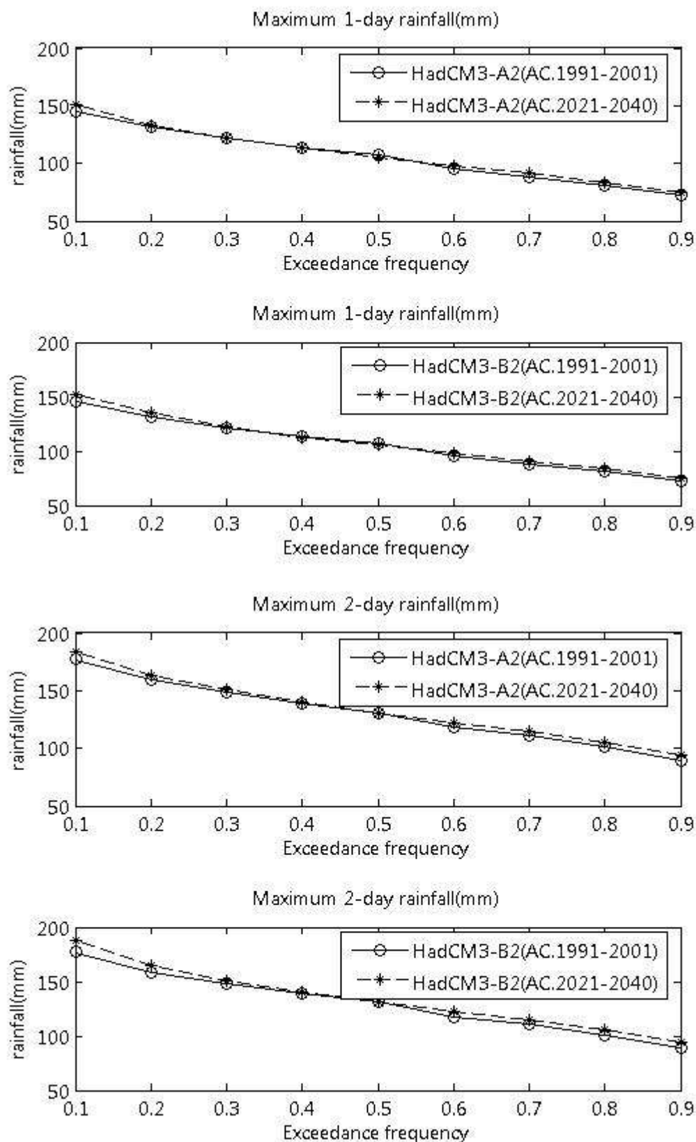
ภาพที่ ข.61 ปริมาณฝนสูงสุด 1 วัน และ 2 วัน ที่สังเคราะห์ได้จากภาพฉาย HadCM3-A2 และ HadCM3-B2 สำหรับสถานี 407009 (ปี ค.ศ. 1991-2001 และ ปี ค.ศ. 2021-2040)
