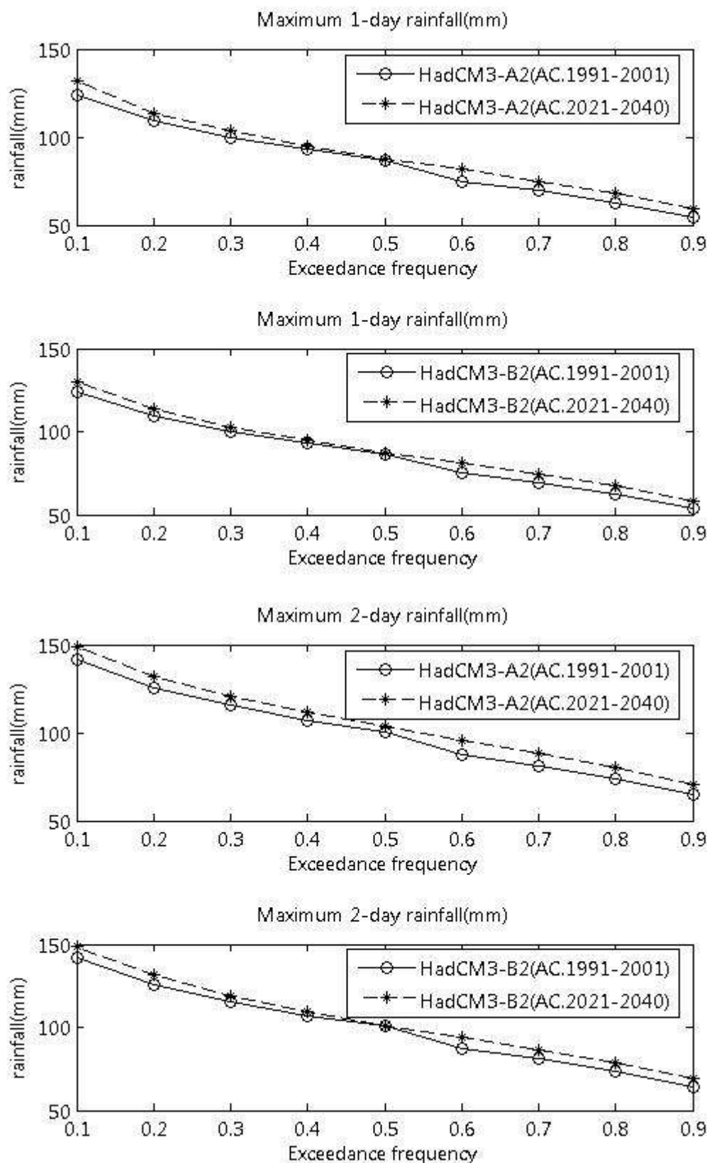
ภาพที่ ข.57 ปริมาณฝนสูงสุด 1 วัน และ 2 วัน ที่สังเคราะห์ได้จากภาพฉาย HadCM3-A2 และ HadCM3-B2 สำหรับสถานี 407002 (ปี ค.ศ. 1991-2001 และ ปี ค.ศ. 2021-2040)
