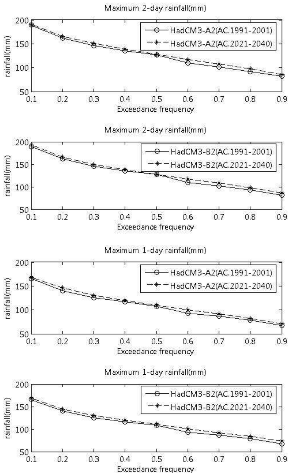
ภาพที่ ข.17 ปริมาณฝนสูงสุด 1 วัน และ 2 วัน ที่สังเคราะห์ได้จากภาพฉาย HadCM3-A2 และ HadCM3-B2 สำหรับสถานี 11210 (ปี ค.ศ. 1991-2001 และ ปี ค.ศ. 2021-2040)
