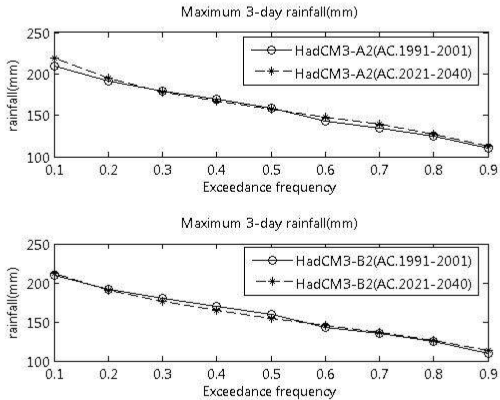
ภาพที่ ข.54 ปริมาณฝนสูงสุด 3 วัน ที่สังเคราะห์ได้จากภาพฉาย HadCM3-A2 และ HadCM3-B2 สำหรับสถานี 406004 (ปี ค.ศ. 1991-2001 และ ปี ค.ศ. 2021-2040)
