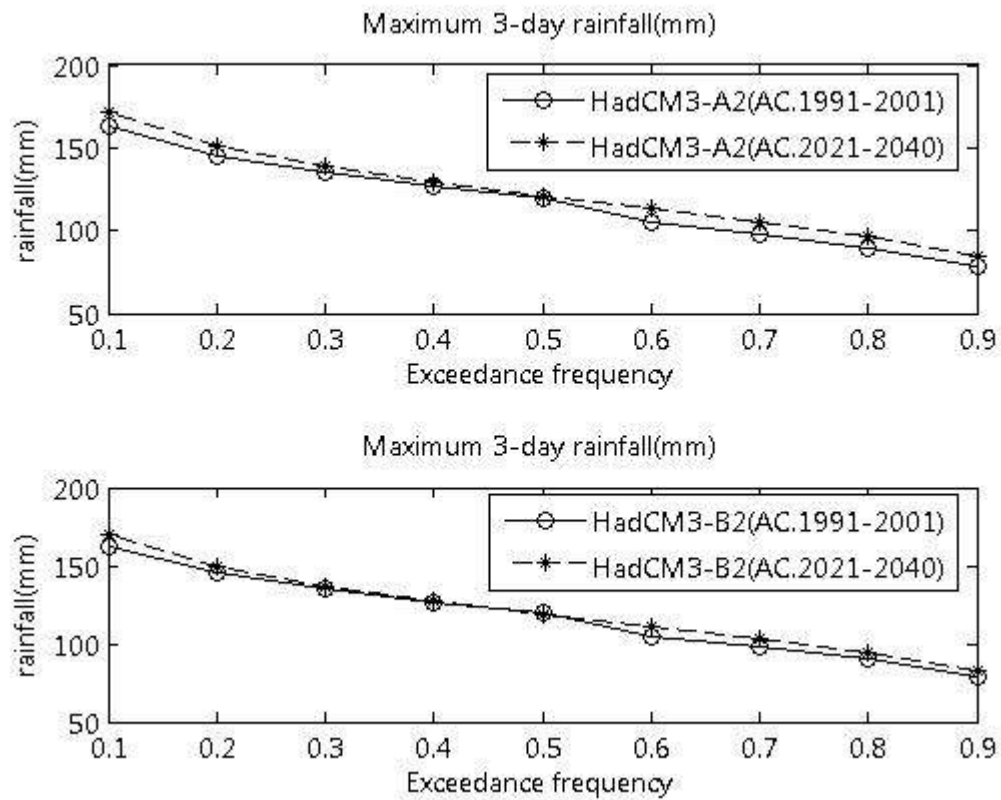
ภาพที่ ข.70 ปริมาณฝนสูงสุด 3 วัน ที่สังเคราะห์ได้จากภาพฉาย HadCM3-A2 และ HadCM3-B2 สำหรับสถานี 432004 (ปี ค.ศ. 1991-2001 และ ปี ค.ศ. 2021-2040)
