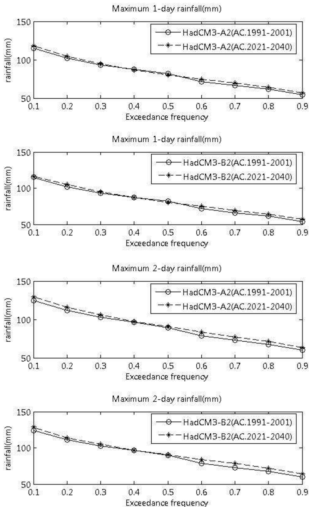
ภาพที่ ข.5 ปริมาณฝนสูงสุด 1 วัน และ 2 วัน ที่สังเคราะห์ได้จากภาพฉาย HadCM3-A2 และ HadCM3-B2 สำหรับสถานี 05032 (ปี ค.ศ. 1991-2001 และ ปี ค.ศ. 2021-2040)
