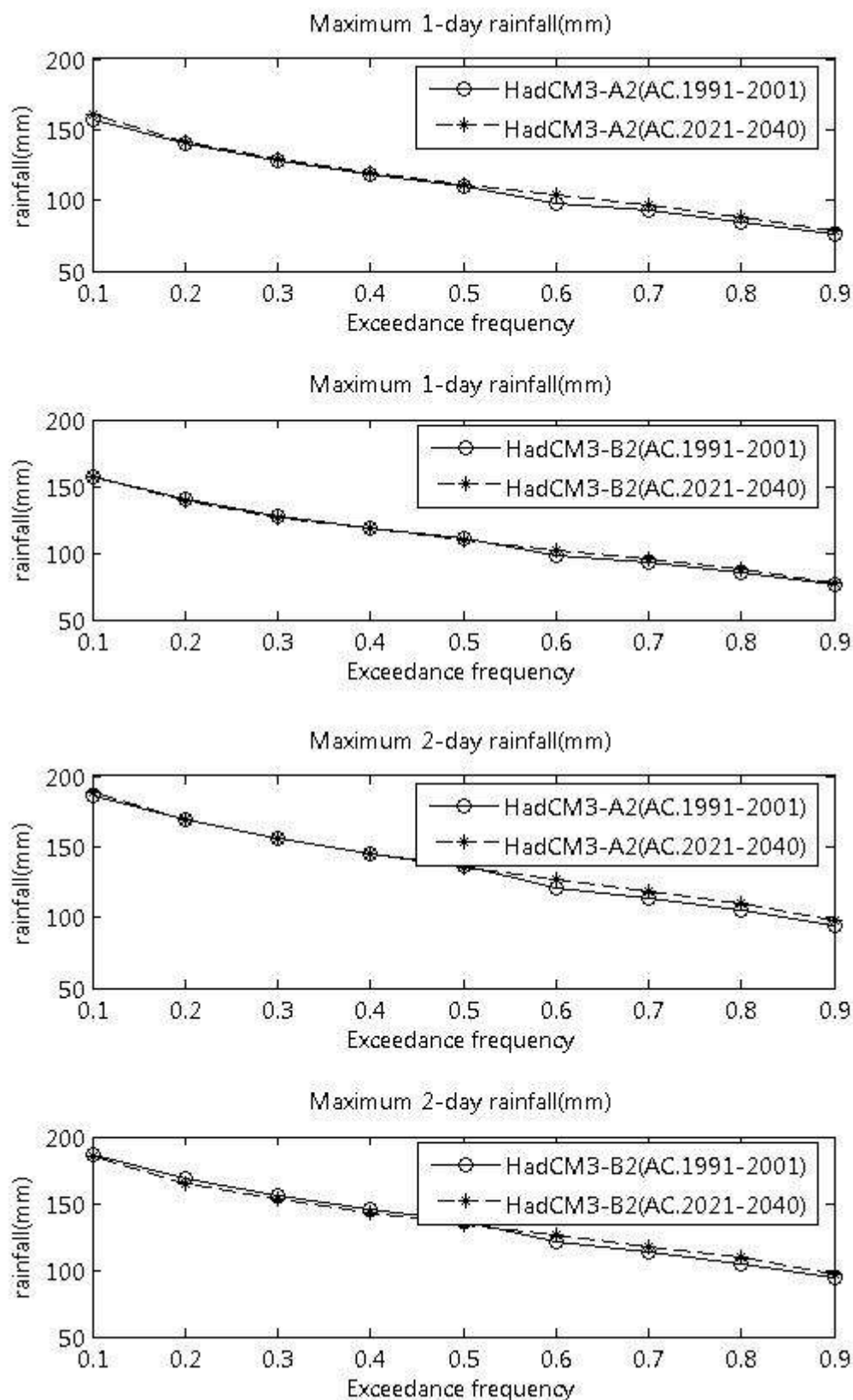
ภาพที่ ข.53 ปริมาณฝนสูงสุด 1 วัน และ 2 วัน ที่สังเคราะห์ได้จากภาพฉาย HadCM3-A2 และ HadCM3-B2 สำหรับสถานี 406004 (ปี ค.ศ. 1991-2001 และ ปี ค.ศ. 2021-2040)
