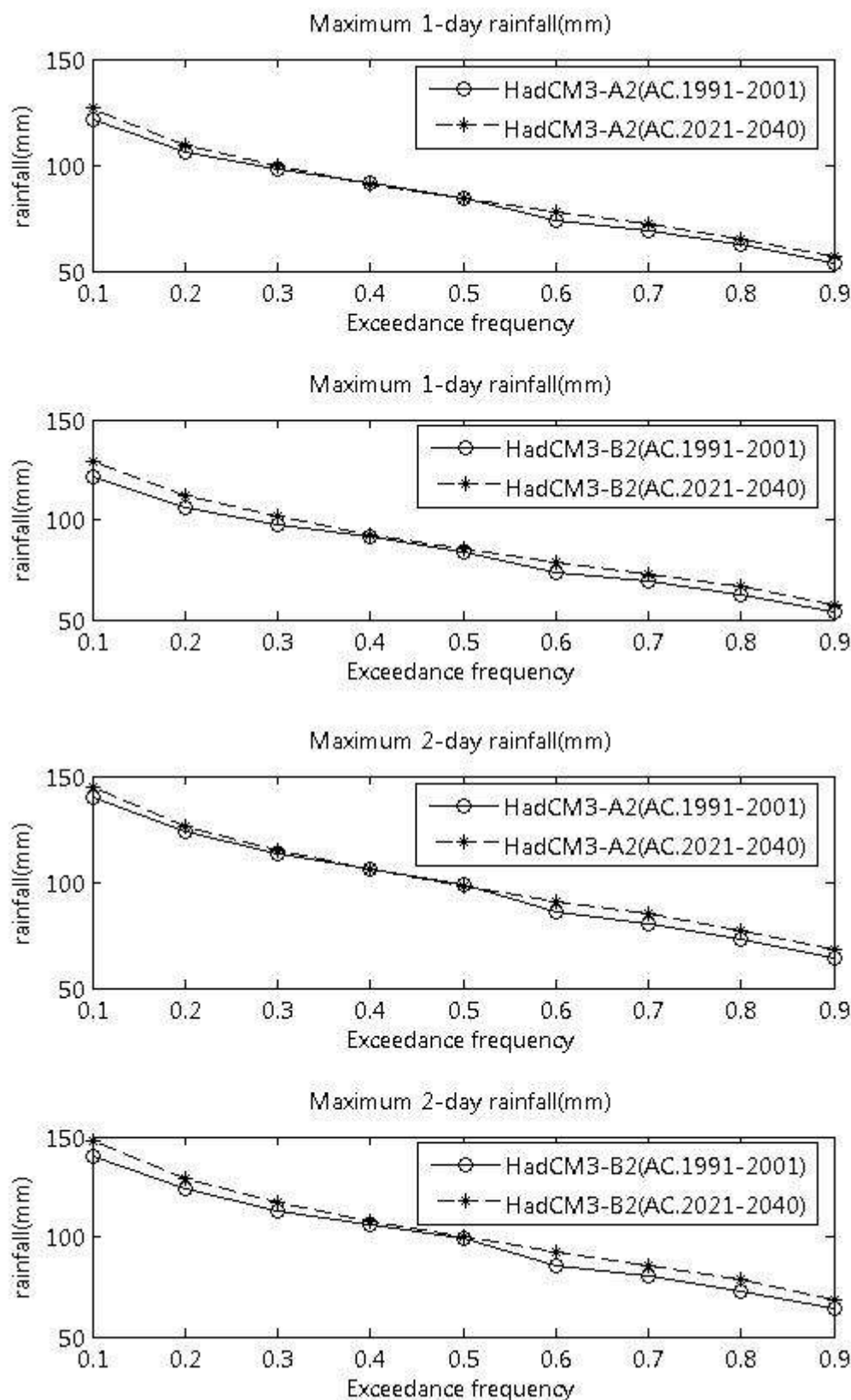
ภาพที่ ข.67 ปริมาณฝนสูงสุด 1 วัน และ 2 วัน ที่สังเคราะห์ได้จากภาพฉาย HadCM3-A2 และ HadCM3-B2 สำหรับสถานี 432001 (ปี ค.ศ. 1991-2001 และ ปี ค.ศ. 2021-2040)
