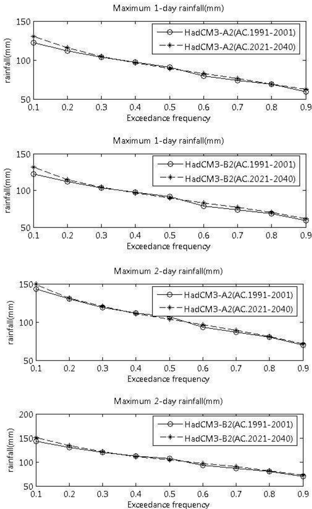
ภาพที่ ข.83 ปริมาณฝนสูงสุด 1 วัน และ 2 วัน ที่สังเคราะห์ได้จากภาพฉาย HadCM3-A2 และ HadCM3-B2 สำหรับสถานี 436013 (ปี ค.ศ. 1991-2001 และ ปี ค.ศ. 2021-2040)
