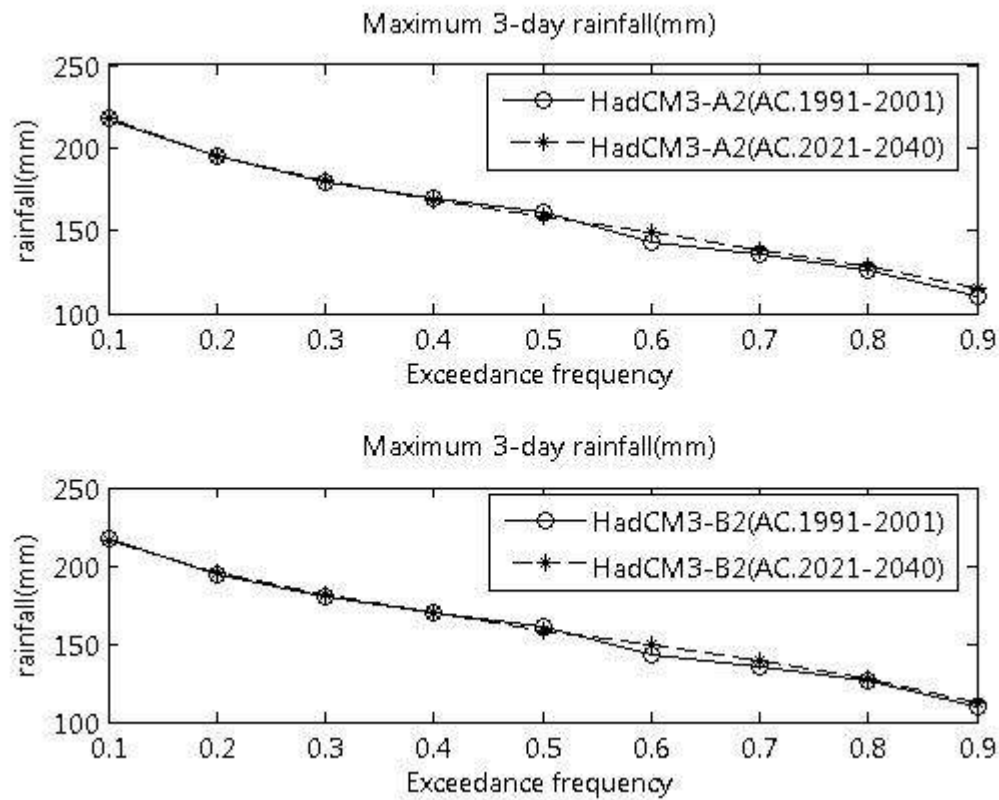
ภาพที่ ข.60 ปริมาณฝนสูงสุด 3 วัน ที่สังเคราะห์ได้จากภาพฉาย HadCM3-A2 และ HadCM3-B2 สำหรับสถานี 407006 (ปี ค.ศ. 1991-2001 และ ปี ค.ศ. 2021-2040)
