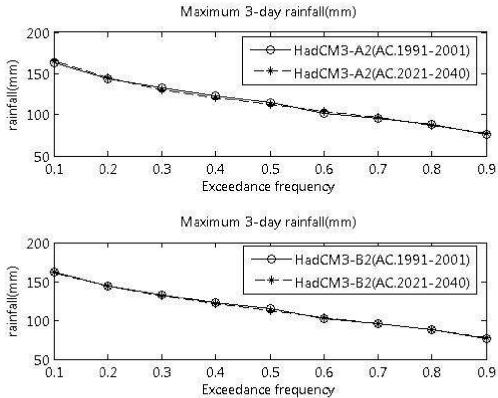
ภาพที่ ข.32 ปริมาณฝนสูงสุด 3 วัน ที่สังเคราะห์ได้จากภาพฉาย HadCM3-A2 และ HadCM3-B2 สำหรับสถานี 49013 (ปี ค.ศ. 1991-2001 และ ปี ค.ศ. 2021-2040)
