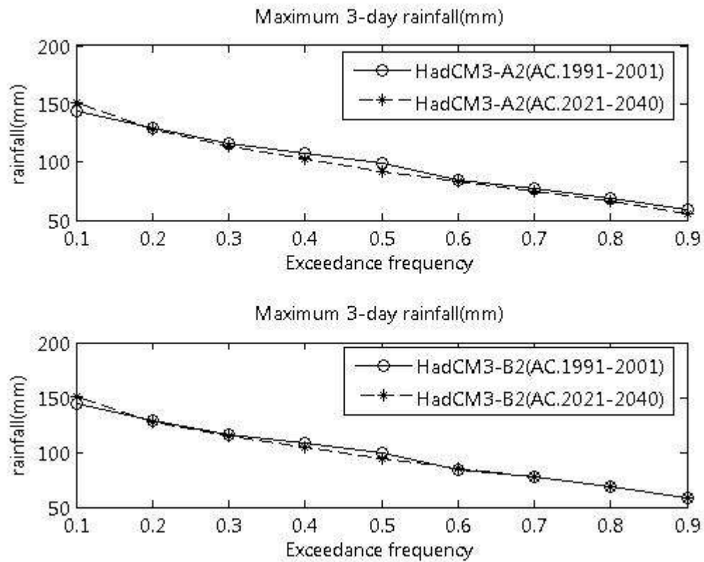
ภาพที่ ข.44 ปริมาณฝนสูงสุด 3 วัน ที่สังเคราะห์ได้จากภาพฉาย HadCM3-A2 และ HadCM3-B2 สำหรับสถานี 75052 (ปี ค.ศ. 1991-2001 และ ปี ค.ศ. 2021-2040)
