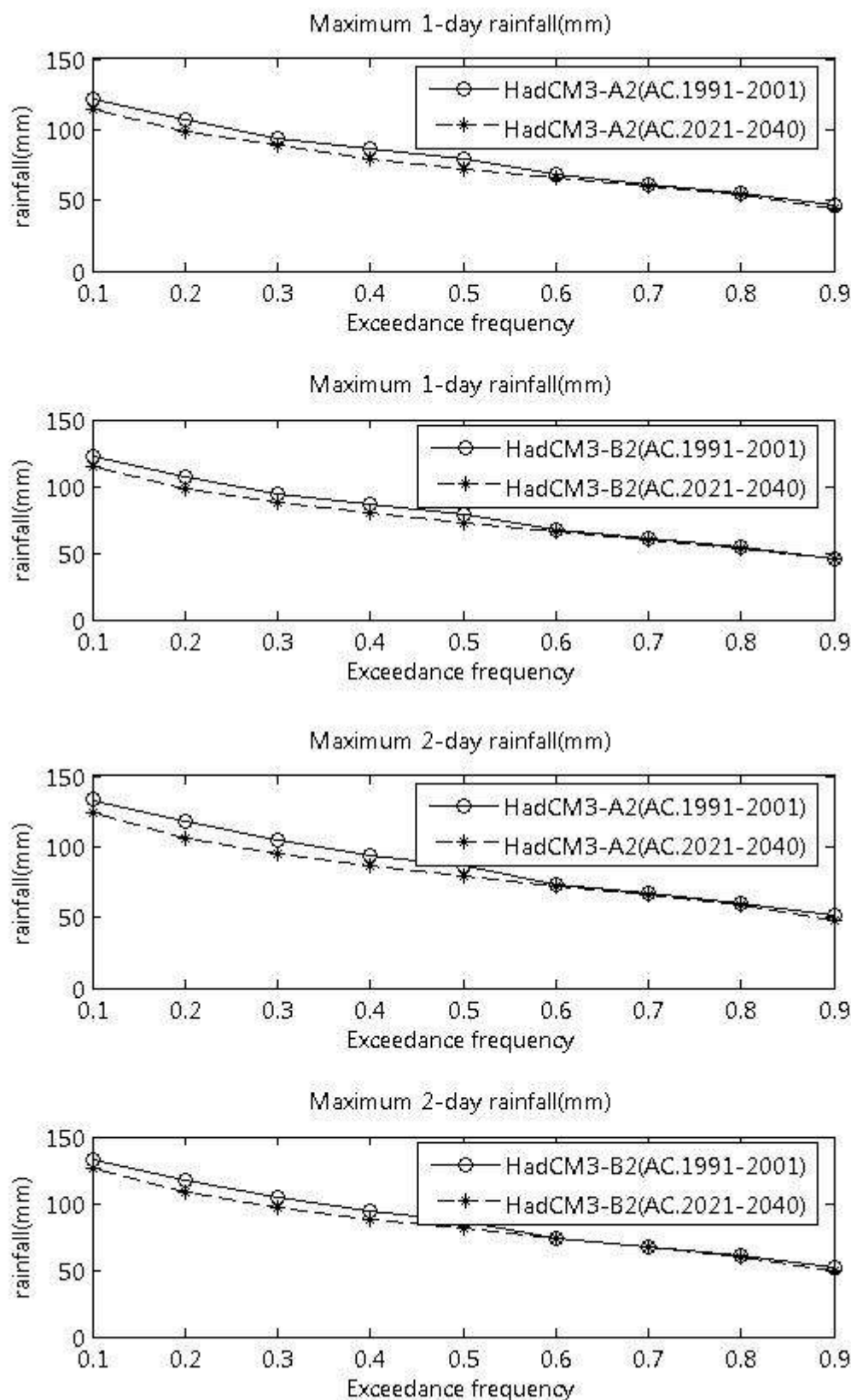
ภาพที่ ข.7 ปริมาณฝนสูงสุด 1 วัน และ 2 วัน ที่สังเคราะห์ได้จากภาพฉาย HadCM3-A2 และ HadCM3-B2 สำหรับ 05092 (ปี ค.ศ. 1991-2001 และ ปี ค.ศ. 2021-2040)
