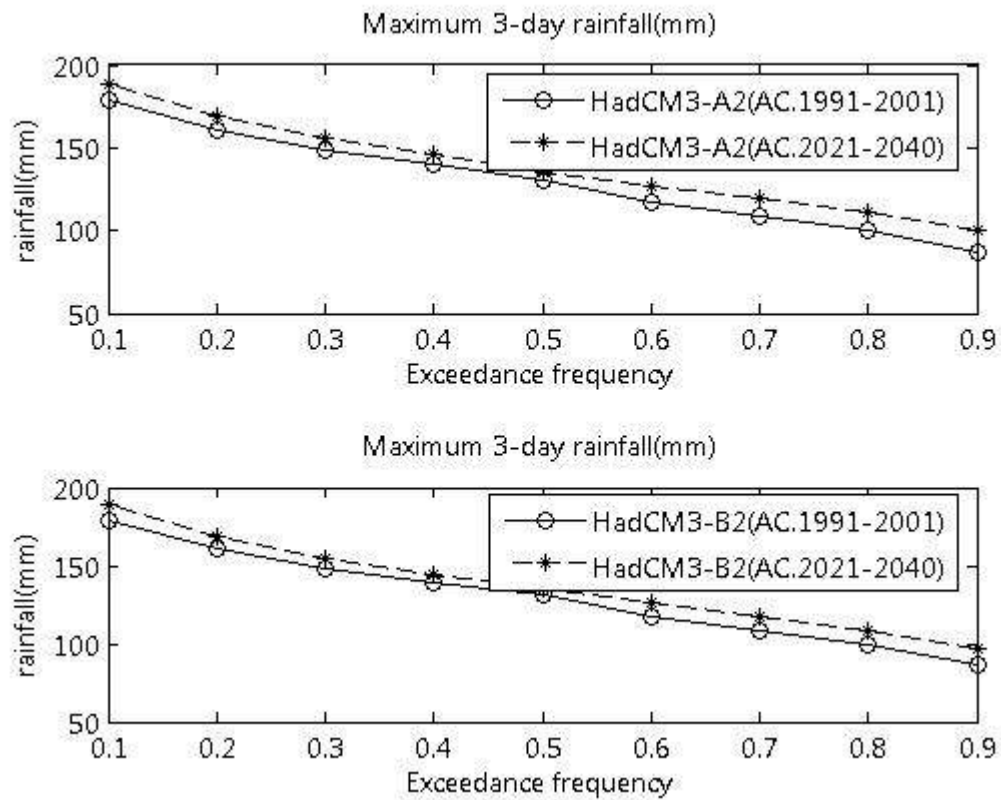
ภาพที่ ข.42 ปริมาณฝนสูงสุด 3 วัน ที่สังเคราะห์ได้จากภาพฉาย HadCM3-A2 และ HadCM3-B2 สถานี 75032 (ปี ค.ศ. 1991-2001 และ ปี ค.ศ. 2021-2040)
