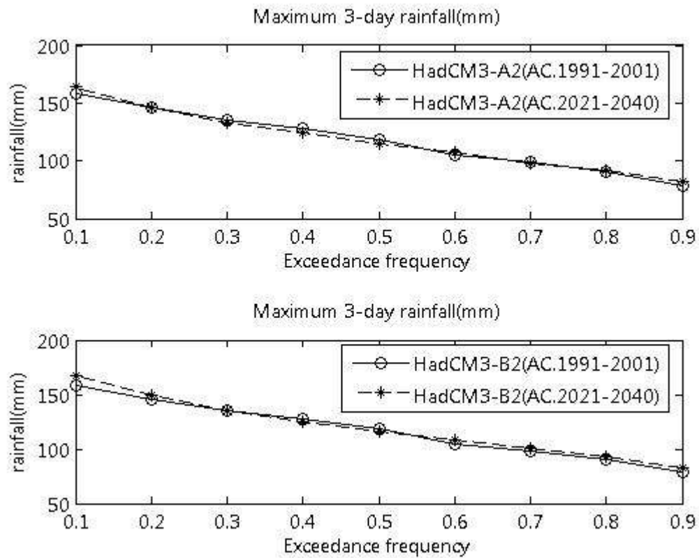
ภาพที่ ข.76 ปริมาณฝนสูงสุด 3 วัน ที่สังเคราะห์ได้จากภาพฉาย HadCM3-A2 และ HadCM3-B2 สำหรับสถานี 436004 (ปี ค.ศ. 1991-2001 และ ปี ค.ศ. 2021-2040)
