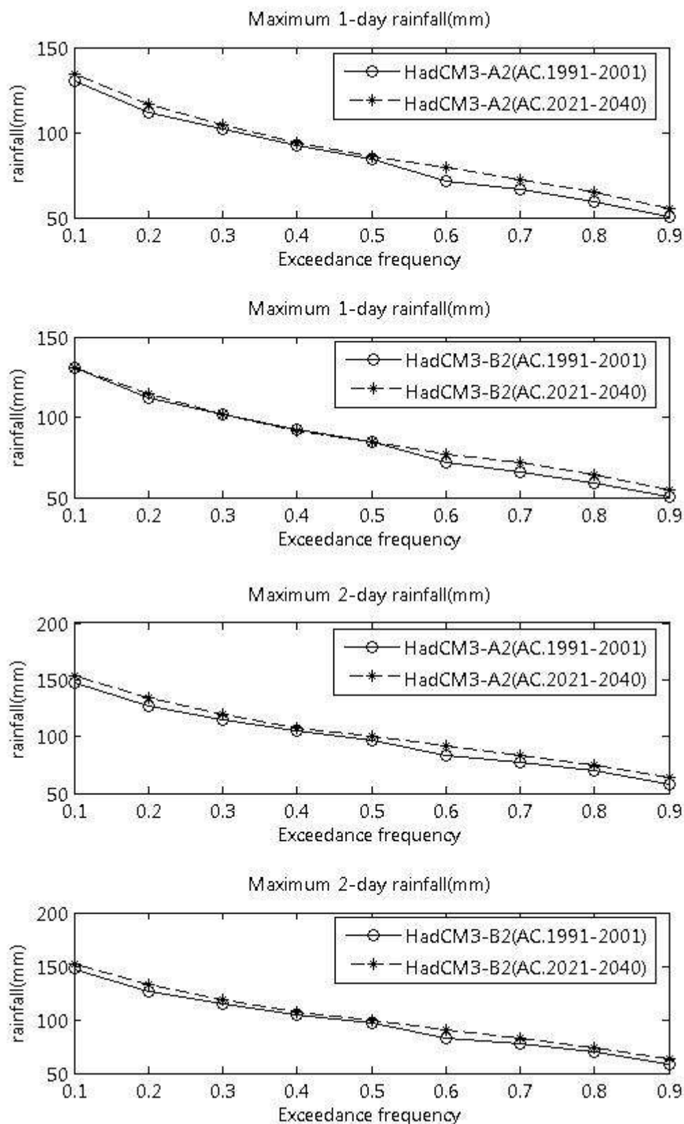
ภาพที่ ข.23 ปริมาณฝนสูงสุด 1 วัน และ 2 วัน ที่สังเคราะห์ได้จากภาพฉาย HadCM3-A2 และ HadCM3-B2 สำหรับสถานี 14112 (ปี ค.ศ. 1991-2001 และ ปี ค.ศ. 2021-2040)
