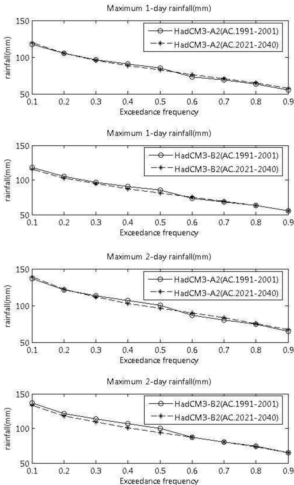
ภาพที่ ข.65 ปริมาณฝนสูงสุด 1 วัน และ 2 วัน ที่สังเคราะห์ได้จากภาพฉาย HadCM3-A2 และ HadCM3-B2 สำหรับสถานี 409004 (ปี ค.ศ. 1991-2001 และ ปี ค.ศ. 2021-2040)
