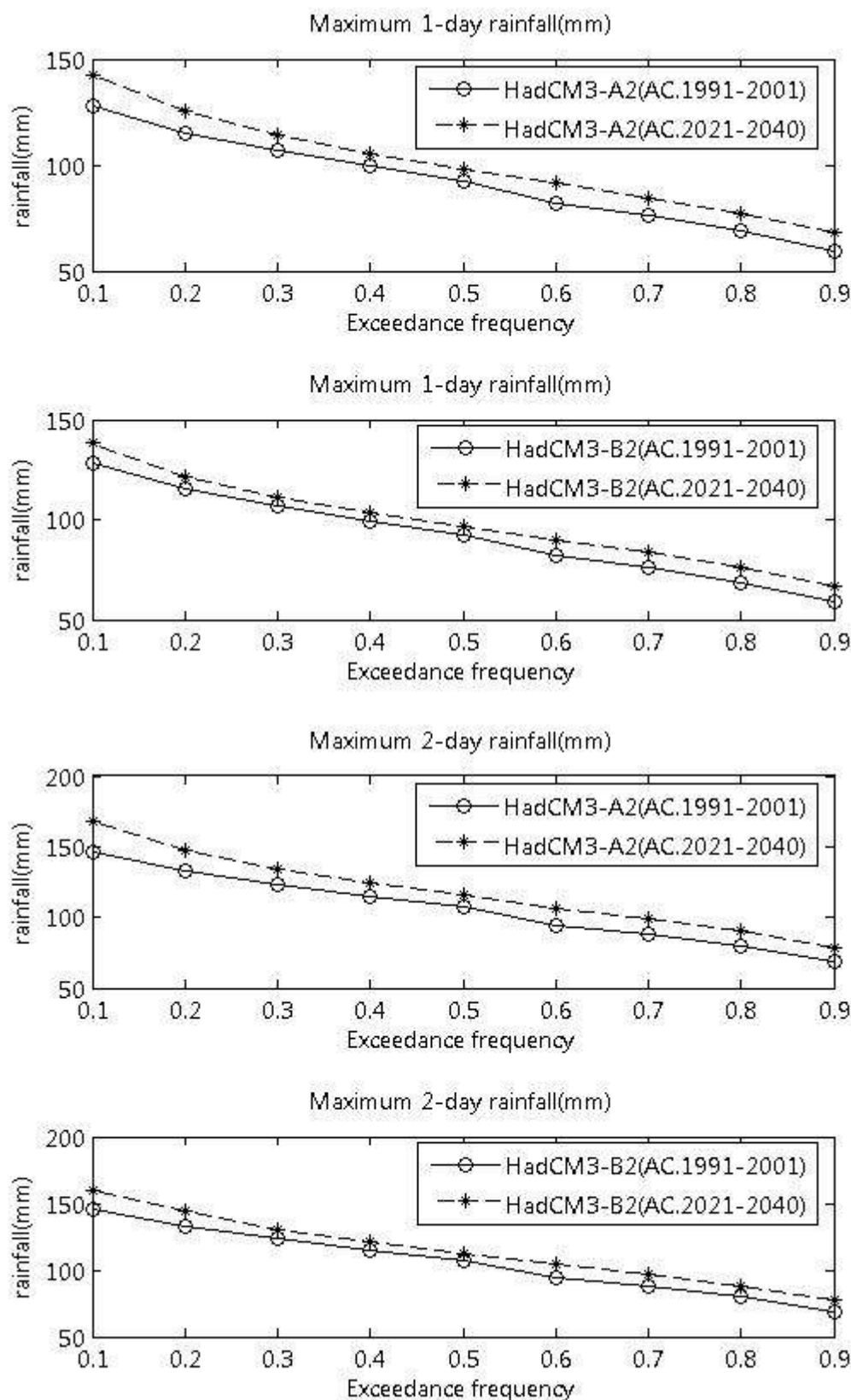
ภาพที่ ข.15 ปริมาณฝนสูงสุด 1 วัน และ 2 วัน ที่สังเคราะห์ได้จากภาพฉาย HadCM3-A2 และ HadCM3-B2 สำหรับสถานี 11202 (ปี ค.ศ. 1991-2001 และ ปี ค.ศ. 2021-2040)
