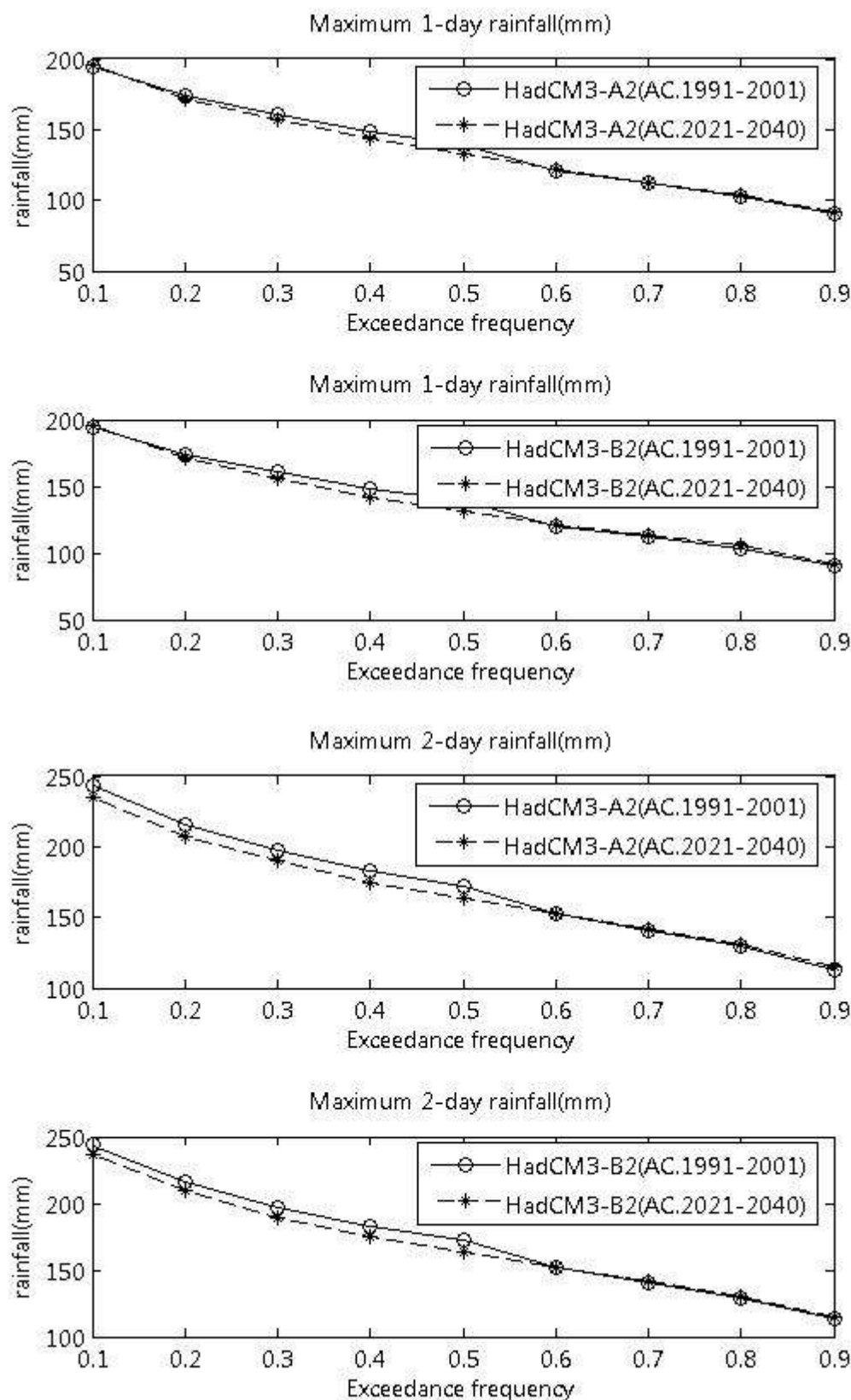
ภาพที่ ข.47 ปริมาณฝนสูงสุด 1 วัน และ 2 วัน ที่สังเคราะห์ได้จากภาพฉาย HadCM3-A2 และ HadCM3-B2 สำหรับสถานี 405002 (ปี ค.ศ. 1991-2001 และ ปี ค.ศ. 2021-2040)
