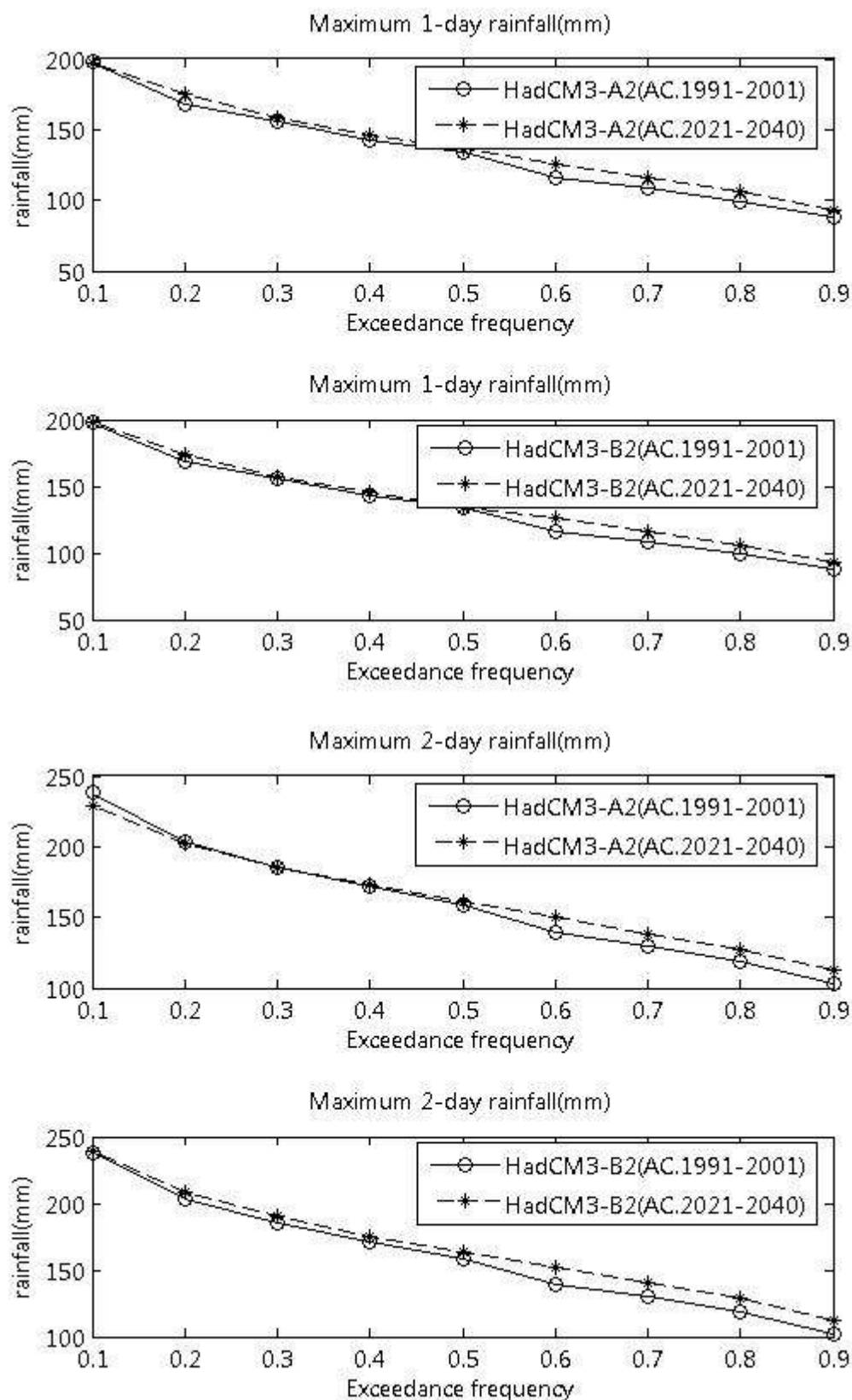
ภาพที่ ข.73 ปริมาณฝนสูงสุด 1 วัน และ 2 วัน ที่สังเคราะห์ได้จากภาพฉาย HadCM3-A2 และ HadCM3-B2 สำหรับสถานี 432006 (ปี ค.ศ. 1991-2001 และ ปี ค.ศ. 2021-2040)
