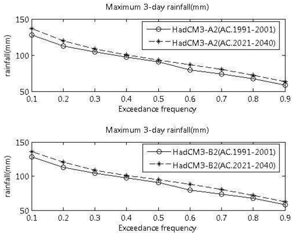
ภาพที่ ข.20 ปริมาณฝนสูงสุด 3 วัน ที่สังเคราะห์ได้จากภาพฉาย HadCM3-A2 และ HadCM3-B2 สำหรับสถานี 14052 (ปี ค.ศ. 1991-2001 และ ปี ค.ศ. 2021-2040)
