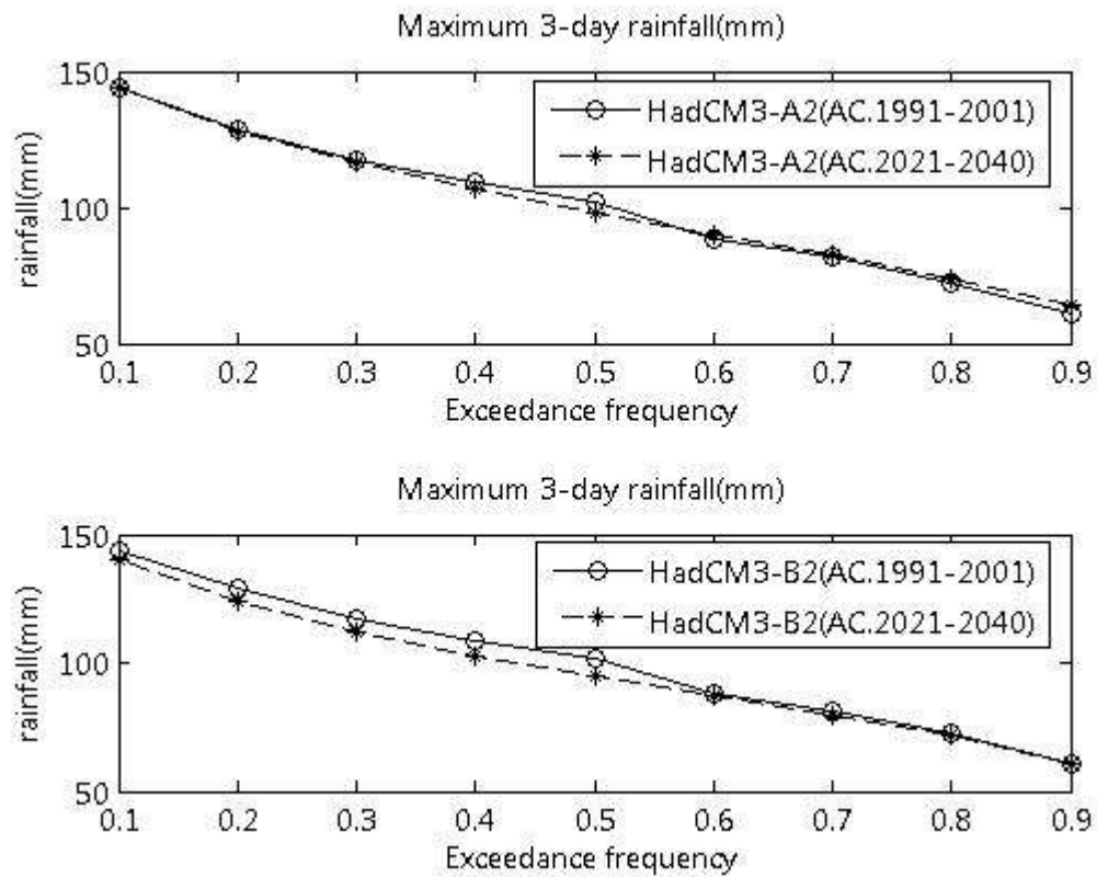
ภาพที่ ข.28 ปริมาณฝนสูงสุด 3 วัน ที่สังเคราะห์ได้จากภาพฉาย HadCM3-A2 และ HadCM3-B2 สถานี 21043 (ปี ค.ศ. 1991-2001 และ ปี ค.ศ. 2021-2040)
