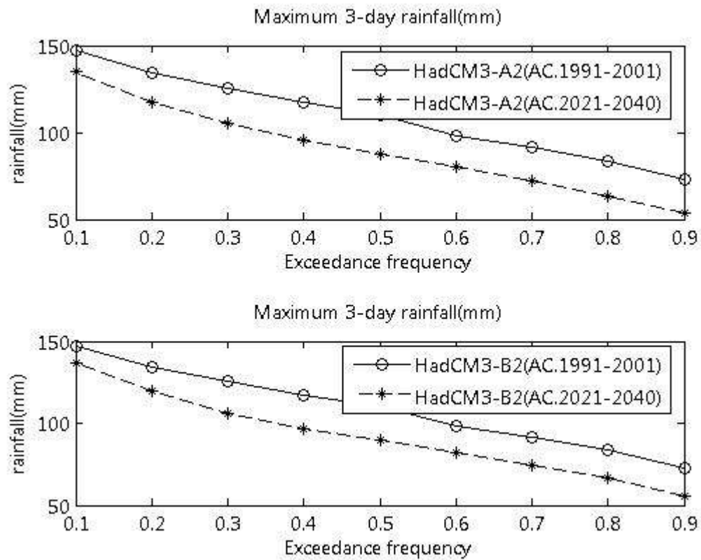
ภาพที่ ข.80 ปริมาณฝนสูงสุด 3 วัน ที่สังเคราะห์ได้จากภาพฉาย HadCM3-A2 และ HadCM3-B2 สำหรับสถานี 436006 (ปี ค.ศ. 1991-2001 และ ปี ค.ศ. 2021-2040)
