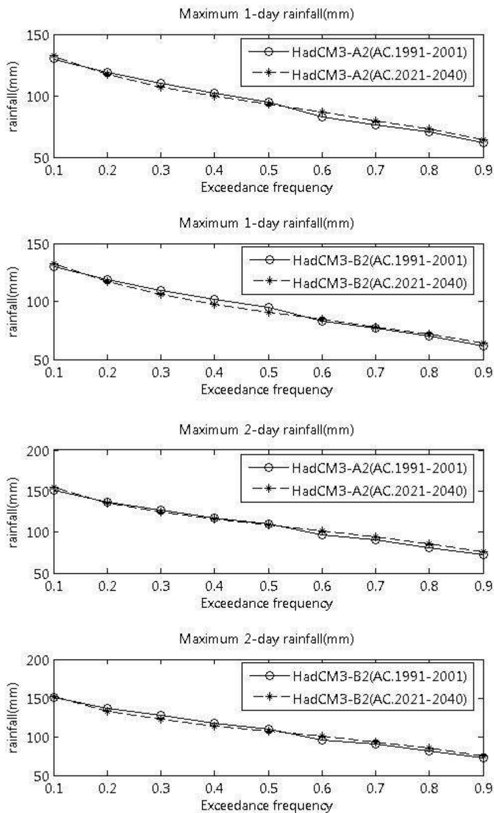
ภาพที่ ข.35 ปริมาณฝนสูงสุด 1 วัน และ 2 วัน ที่สังเคราะห์ได้จากภาพฉาย HadCM3-A2 และ HadCM3-B2 สำหรับสถานี 49301 (ปี ค.ศ. 1991-2001 และ ปี ค.ศ. 2021-2040)
