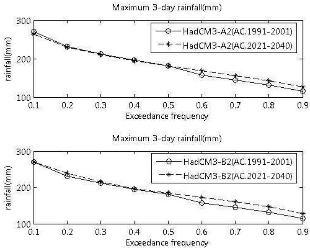
ภาพที่ ข.74 ปริมาณฝนสูงสุด 3 วัน ที่สังเคราะห์ได้จากภาพฉาย HadCM3-A2 และ HadCM3-B2 สำหรับสถานี 432006 (ปี ค.ศ. 1991-2001 และ ปี ค.ศ. 2021-2040)
