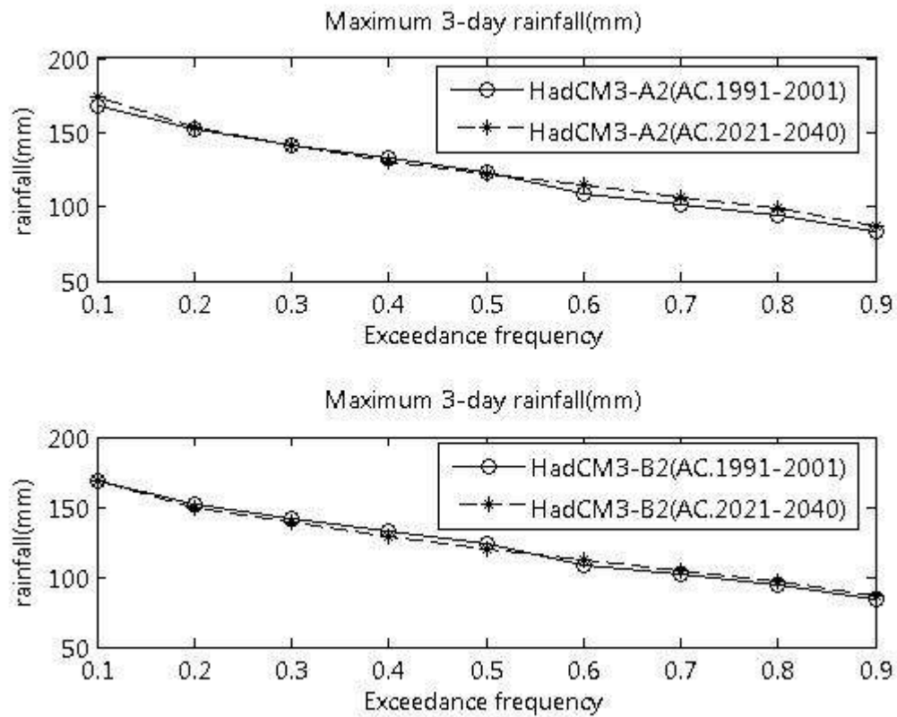
ภาพที่ ข.36 ปริมาณฝนสูงสุด 3 วัน ที่สังเคราะห์ได้จากภาพฉาย HadCM3-A2 และ HadCM3-B2 สำหรับสถานี 49301 (ปี ค.ศ. 1991-2001 และ ปี ค.ศ. 2021-2040)
