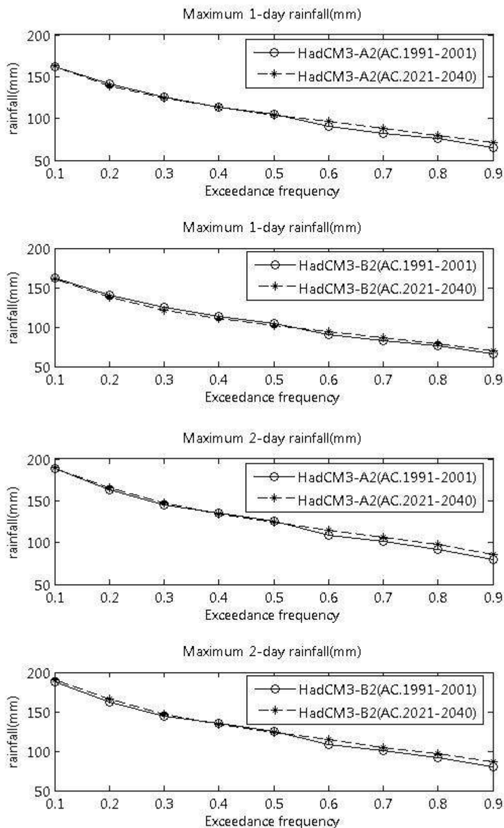
ภาพที่ ข.29 ปริมาณฝนสูงสุด 1 วัน และ 2 วัน ที่สังเคราะห์ได้จากภาพฉาย HadCM3-A2 และ HadCM3-B2 สำหรับสถานี 21190 (ปี ค.ศ. 1991-2001 และ ปี ค.ศ. 2021-2040)
