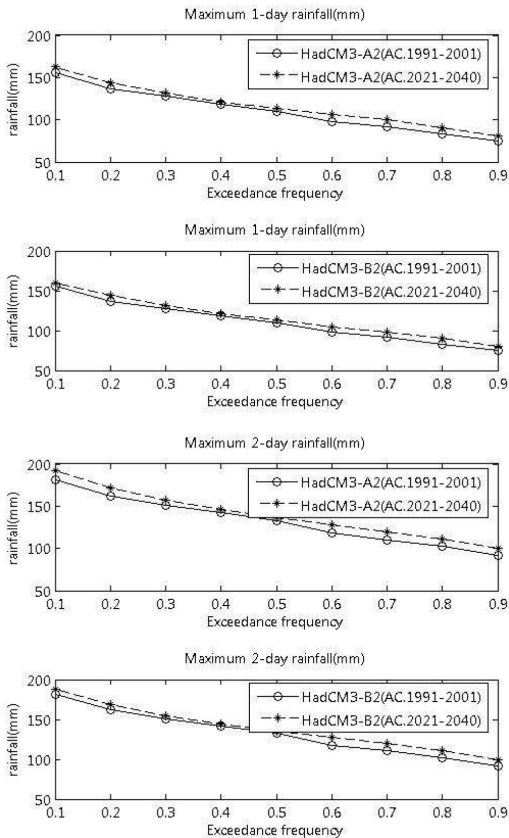
ภาพที่ ข.51 ปริมาณฝนสูงสุด 1 วัน และ 2 วัน ที่สังเคราะห์ได้จากภาพฉาย HadCM3-A2 และ HadCM3-B2 สำหรับสถานี 406002 (ปี ค.ศ. 1991-2001 และ ปี ค.ศ. 2021-2040)
