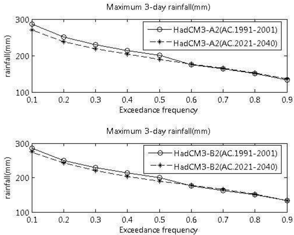
ภาพที่ ข.48 ปริมาณฝนสูงสุด 3 วัน ที่สังเคราะห์ได้จากภาพฉาย HadCM3-A2 และ HadCM3-B2 สำหรับสถานี 405002 (ปี ค.ศ. 1991-2001 และ ปี ค.ศ. 2021-2040)
