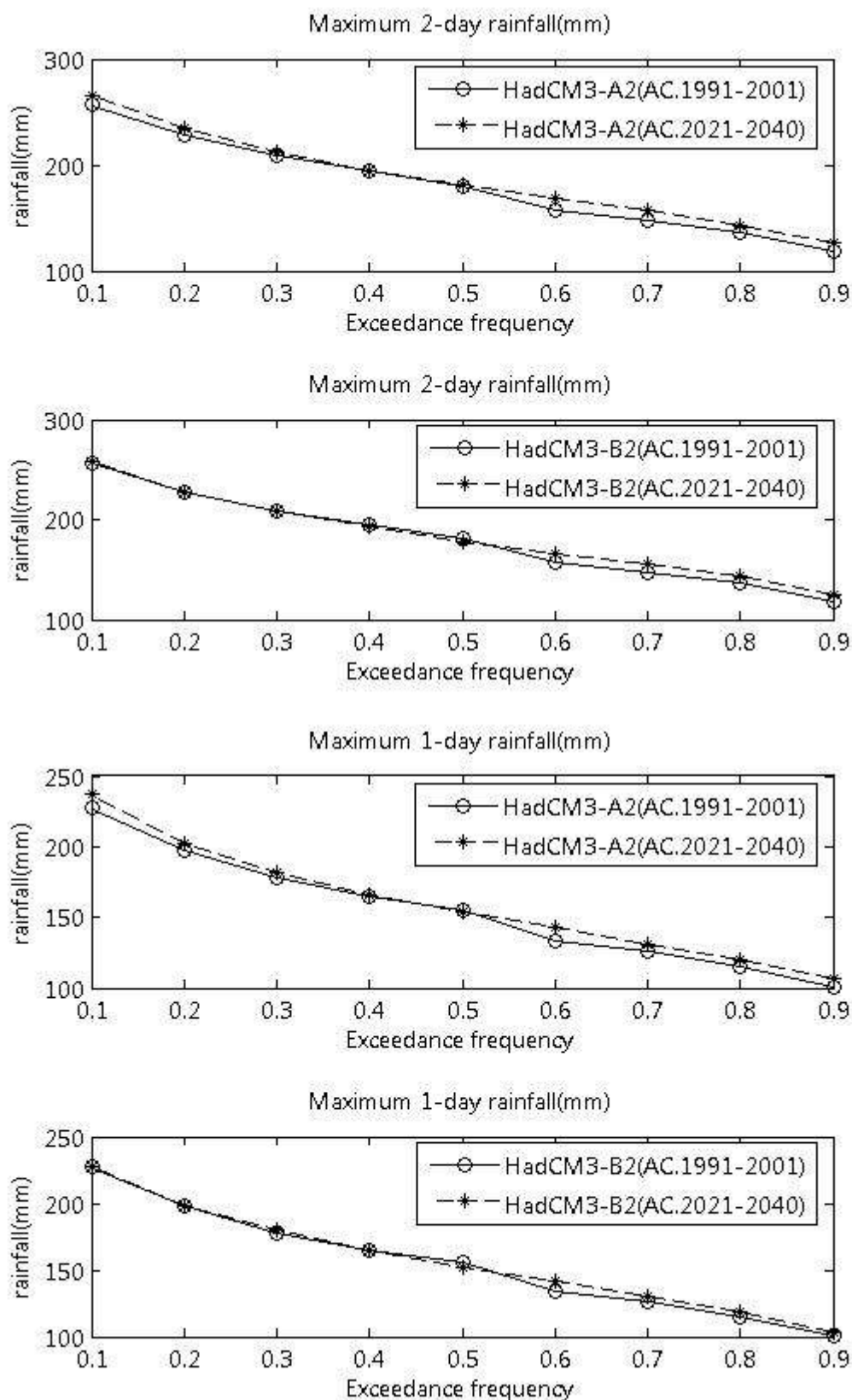
ภาพที่ ข.55 ปริมาณฝนสูงสุด 1 วัน และ 2 วัน ที่สังเคราะห์ได้จากภาพฉาย HadCM3-A2 และ HadCM3-B2 ปี ค.ศ. 1991-2001 สำหรับสถานี 406005 (ปี ค.ศ. 1991-2001 และ ปี ค.ศ. 2021-2040)
