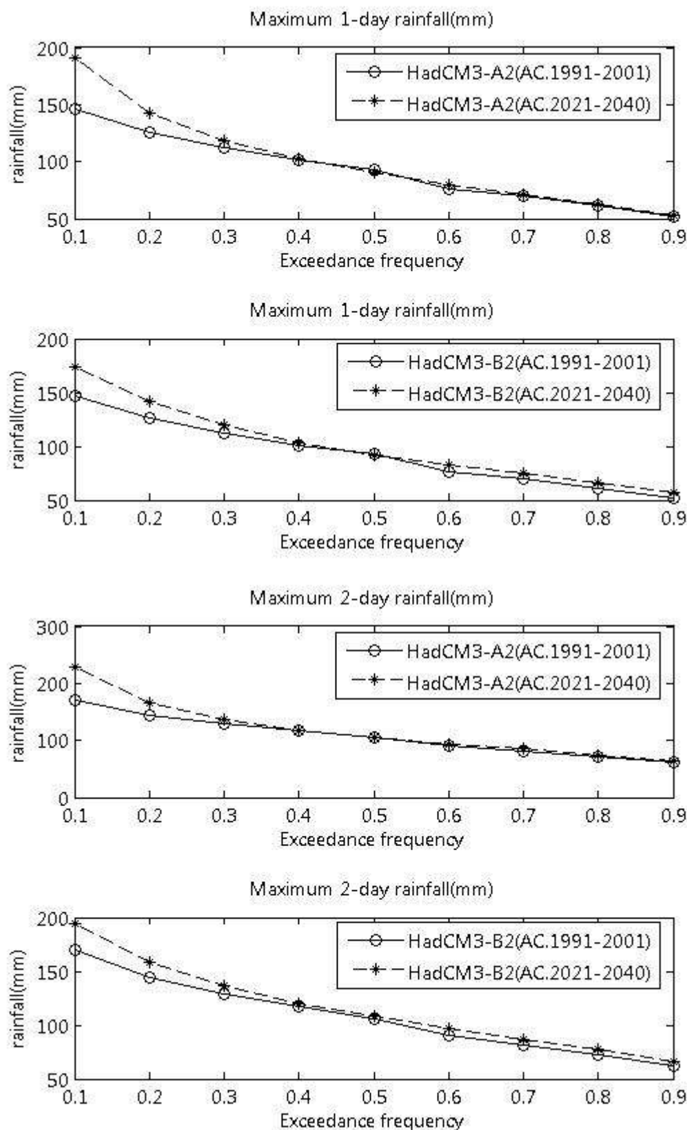
ภาพที่ ข.9 ปริมาณฝนสูงสุด 1 วัน และ 2 วัน ที่สังเคราะห์ได้จากภาพฉาย HadCM3-A2 และ HadCM3-B2 สำหรับสถานี 05171 (ปี ค.ศ. 1991-2001 และ ปี ค.ศ. 2021-2040)
