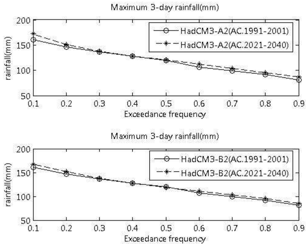
ภาพที่ ข.14 ปริมาณฝนสูงสุด 3 วัน ที่สังเคราะห์ได้จากภาพฉาย HadCM3-A2 และ HadCM3-B2 สำหรับสถานี 11170 (ปี ค.ศ. 1991-2001 และ ปี ค.ศ. 2021-2040)
