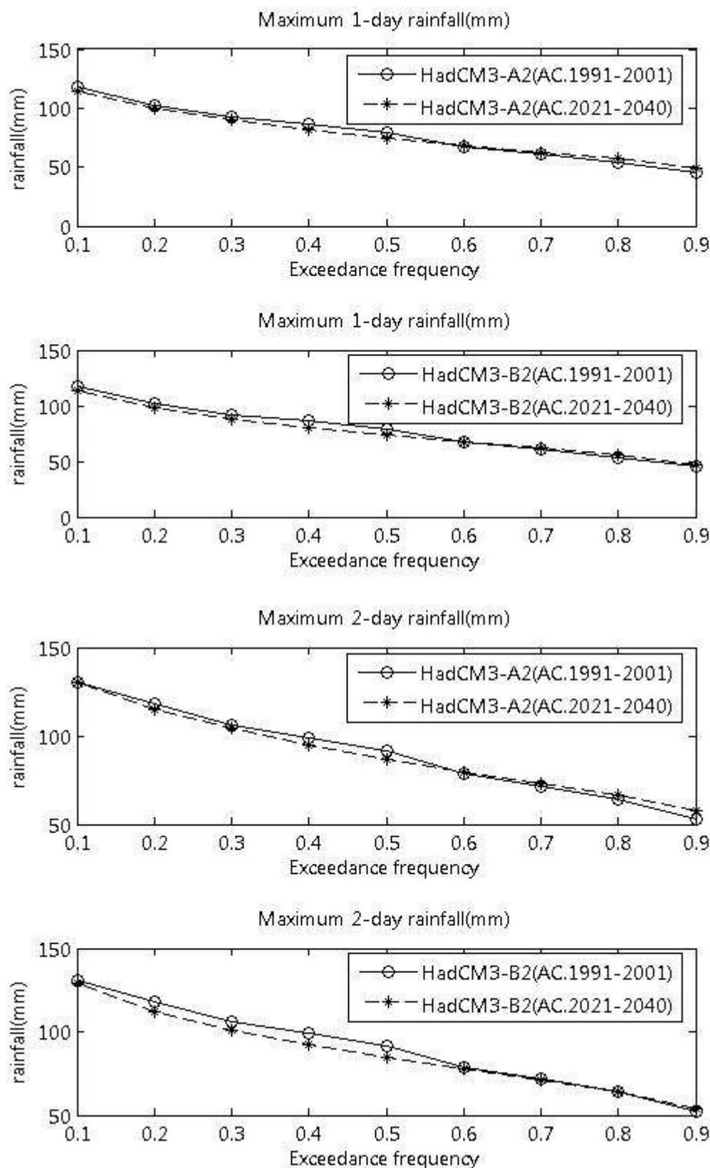
ภาพที่ ข.27 ปริมาณฝนสูงสุด 1 วัน และ 2 วัน ที่สังเคราะห์ได้จากภาพฉาย HadCM3-A2 และ HadCM3-B2 สถานี 21043 (ปี ค.ศ. 1991-2001 และ ปี ค.ศ. 2021-2040)
