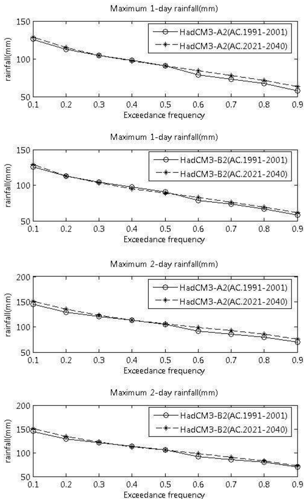
ภาพที่ ข.69 ปริมาณฝนสูงสุด 1 วัน และ 2 วัน ที่สังเคราะห์ได้จากภาพฉาย HadCM3-A2 และ HadCM3-B2 สำหรับสถานี 432004 (ปี ค.ศ. 1991-2001 และ ปี ค.ศ. 2021-2040)
