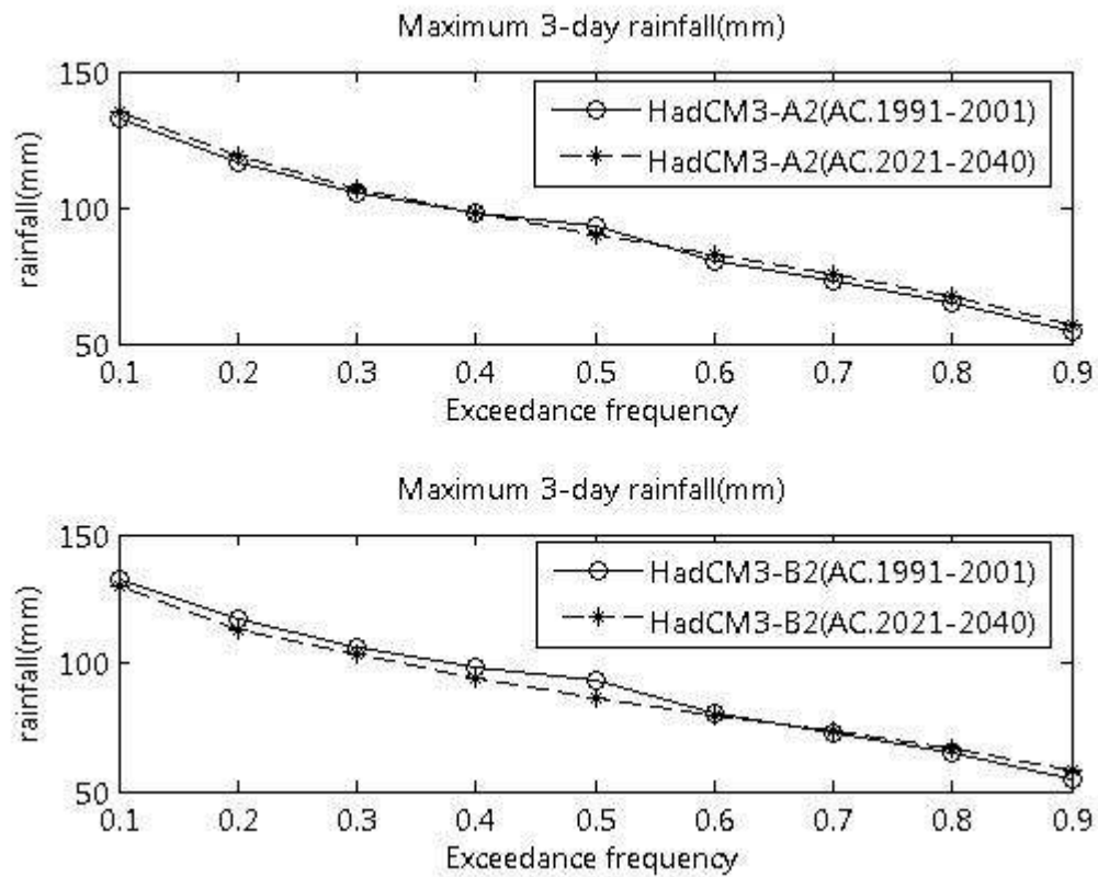
ภาพที่ ข.22 ปริมาณฝนสูงสุด 3 วัน ที่สังเคราะห์ได้จากภาพฉาย HadCM3-A2 และ HadCM3-B2 สำหรับสถานี 14062 (ปี ค.ศ. 1991-2001 และ ปี ค.ศ. 2021-2040)
