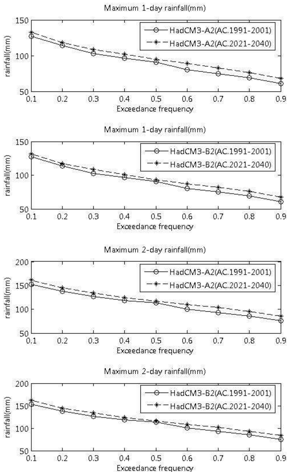
ภาพที่ ข.41 ปริมาณฝนสูงสุด 1 วัน และ 2 วัน ที่สังเคราะห์ได้จากภาพฉาย HadCM3-A2 และ HadCM3-B2 สถานี 75032 (ปี ค.ศ. 1991-2001 และ ปี ค.ศ. 2021-2040)
