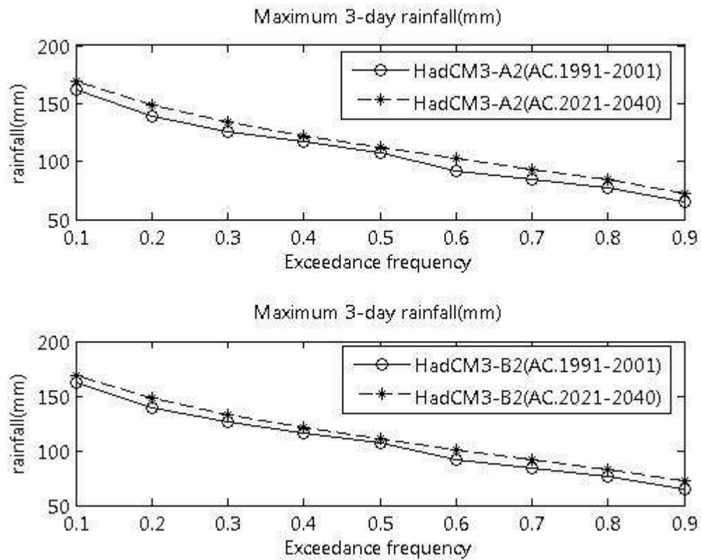
ภาพที่ ข.24 ปริมาณฝนสูงสุด 3 วัน ที่สังเคราะห์ได้จากภาพฉาย HadCM3-A2 และ HadCM3-B2 สำหรับสถานี 14112 (ปี ค.ศ. 1991-2001 และ ปี ค.ศ. 2021-2040)
