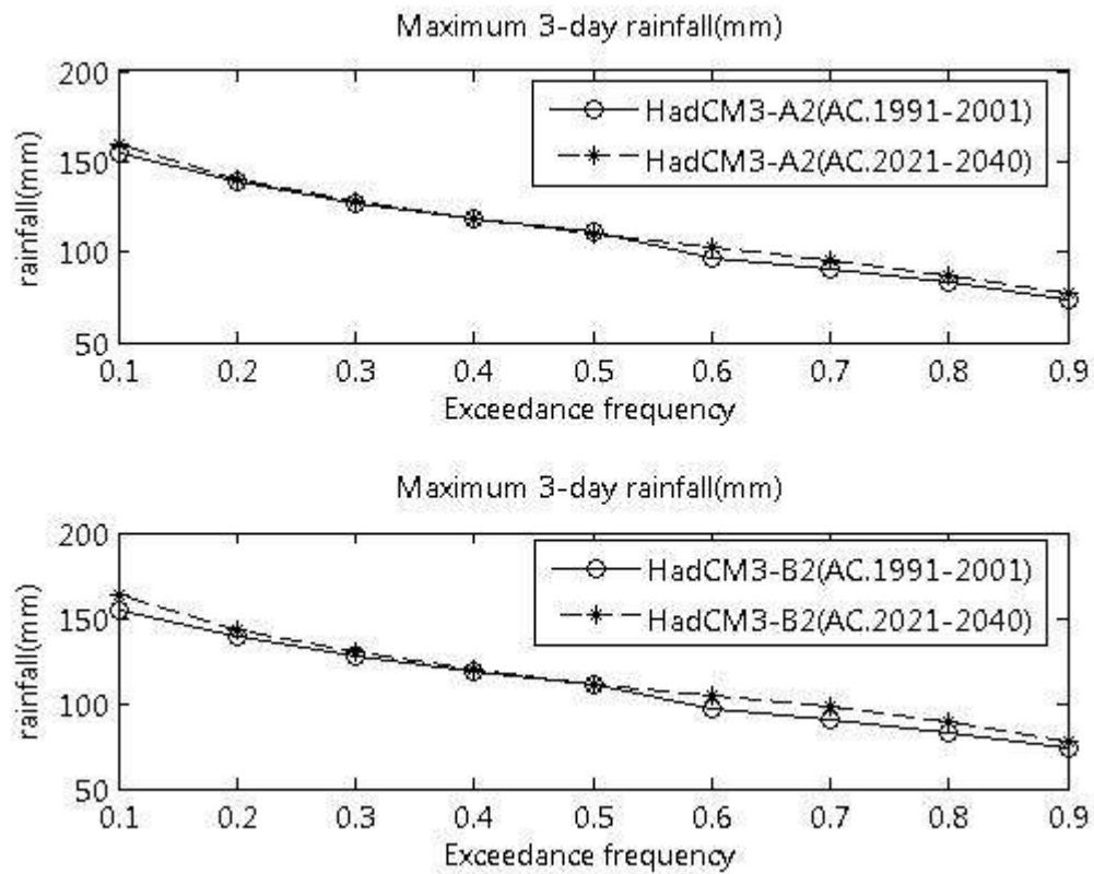
ภาพที่ ข.68 ปริมาณฝนสูงสุด 3 วัน ที่สังเคราะห์ได้จากภาพฉาย HadCM3-A2 และ HadCM3-B2 สำหรับสถานี 432001 (ปี ค.ศ. 1991-2001 และ ปี ค.ศ. 2021-2040)
