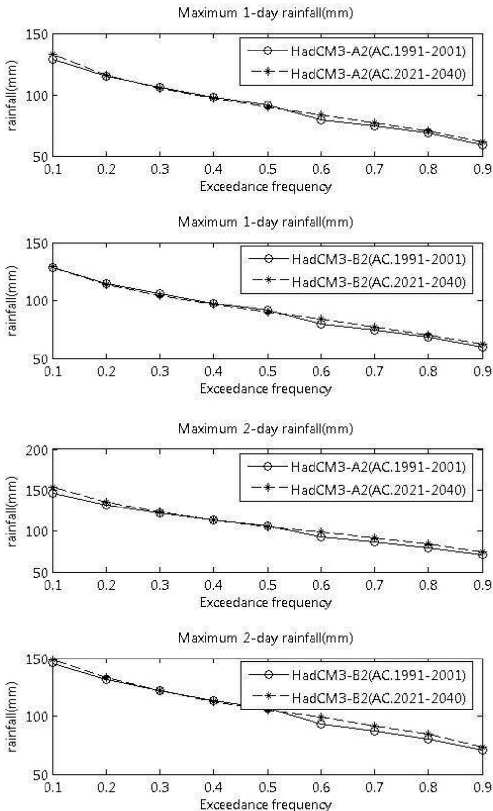
ภาพที่ ข.13 ปริมาณฝนสูงสุด 1 วัน และ 2 วัน ที่สังเคราะห์ได้จากภาพฉาย HadCM3-A2 และ HadCM3-B2 สำหรับสถานี 11170 (ปี ค.ศ. 1991-2001 และ ปี ค.ศ. 2021-2040)
