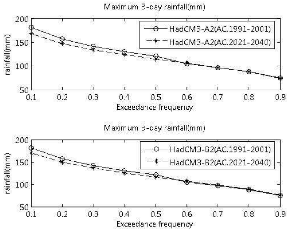
ภาพที่ ข.4 ปริมาณฝนสูงสุด 3 วัน ที่สังเคราะห์ได้จากภาพฉาย HadCM3-A2 และ HadCM3-B2 สำหรับสถานี 05023 (ปี ค.ศ. 1991-2001 และ ปี ค.ศ. 2021-2040)
