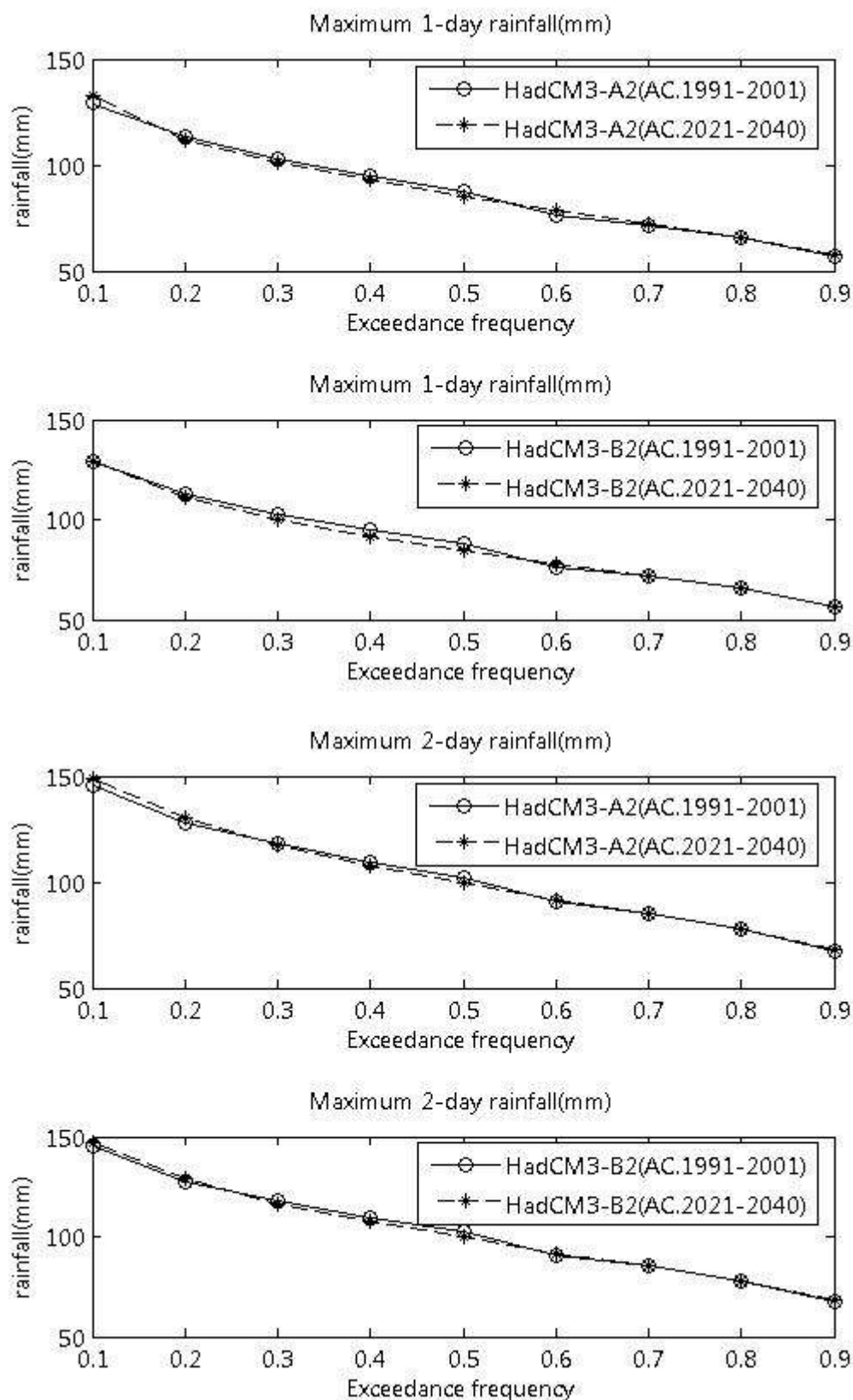
ภาพที่ ข.31 ปริมาณฝนสูงสุด 1 วัน และ 2 วัน ที่สังเคราะห์ได้จากภาพฉาย HadCM3-A2 และ HadCM3-B2 สำหรับสถานี 49013 (ปี ค.ศ. 1991-2001 และ ปี ค.ศ. 2021-2040)
