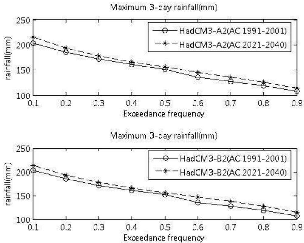
ภาพที่ ข.52 ปริมาณฝนสูงสุด 3 วัน ที่สังเคราะห์ได้จากภาพฉาย HadCM3-A2 และ HadCM3-B2 สำหรับสถานี 406002 (ปี ค.ศ. 1991-2001 และ ปี ค.ศ. 2021-2040)
