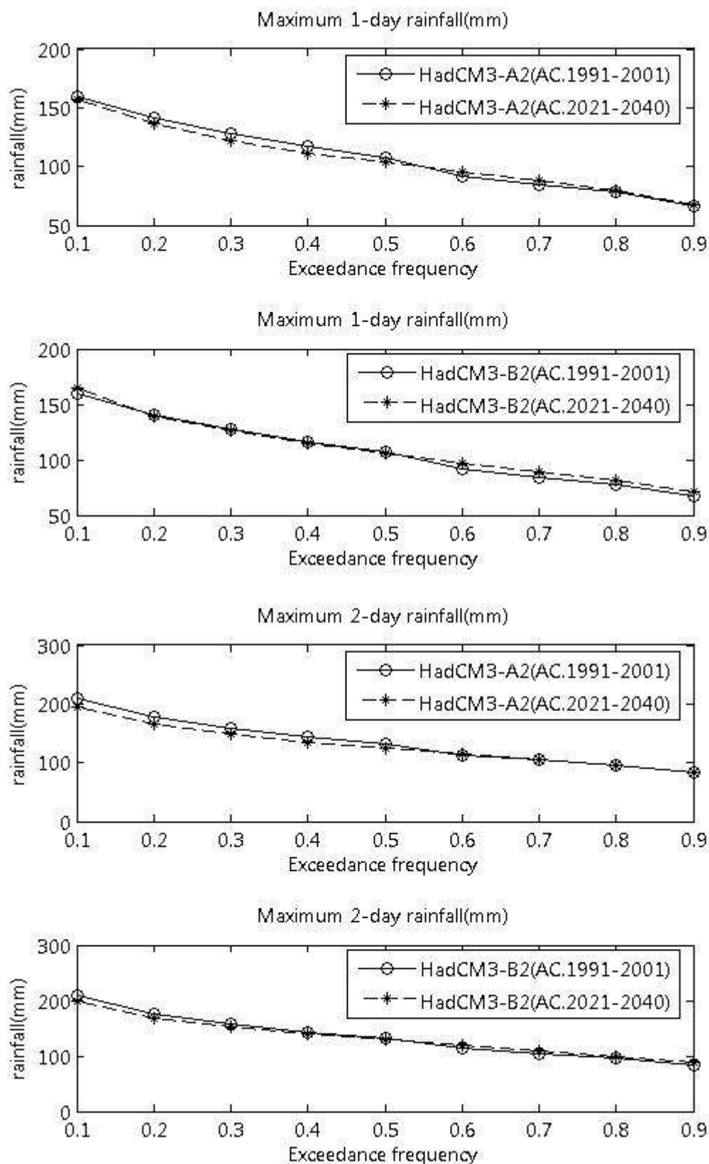
ภาพที่ ข.81 ปริมาณฝนสูงสุด 1 วัน และ 2 วัน ที่สังเคราะห์ได้จากภาพฉาย HadCM3-A2 และ HadCM3-B2 สำหรับสถานี 436007 (ปี ค.ศ. 1991-2001 และ ปี ค.ศ. 2021-2040)
