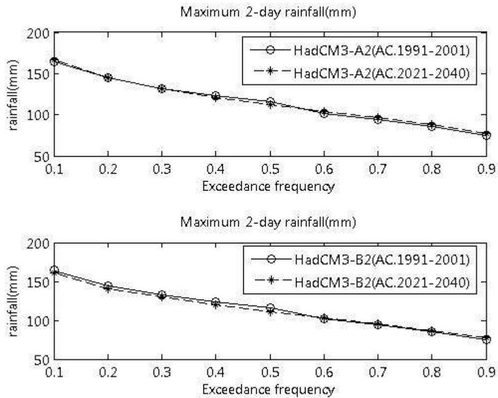
ภาพที่ ข.64 ปริมาณฝนสูงสุด 3 วัน ที่สังเคราะห์ได้จากภาพฉาย HadCM3-A2 และ HadCM3-B2 สำหรับสถานี 407015 (ปี ค.ศ. 1991-2001 และ ปี ค.ศ. 2021-2040)
