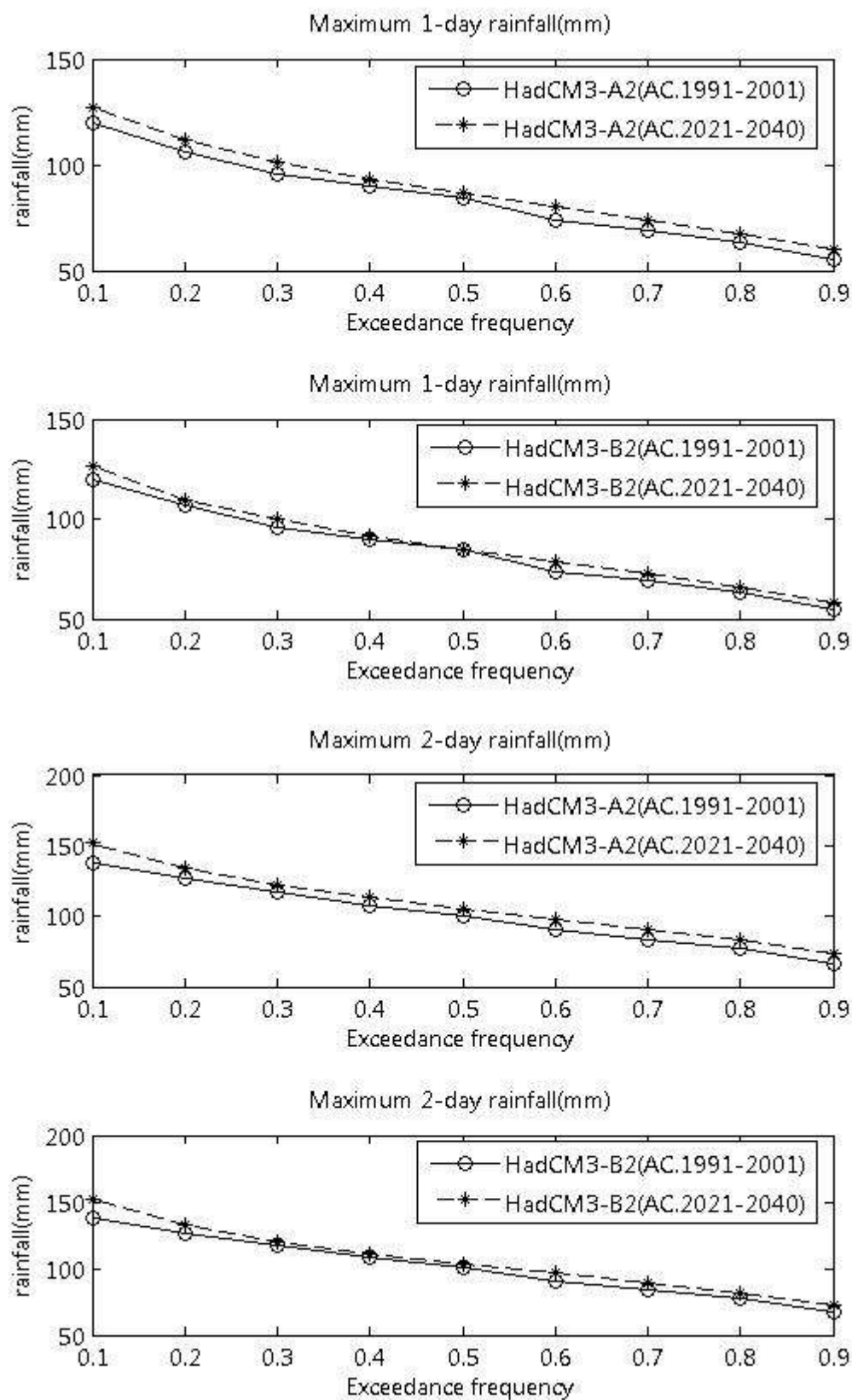
ภาพที่ ข.25 ปริมาณฝนสูงสุด 1 วัน และ 2 วัน ที่สังเคราะห์ได้จากภาพฉาย HadCM3-A2 และ HadCM3-B2 สถานี 18073 (ปี ค.ศ. 1991-2001 และ ปี ค.ศ. 2021-2040)
