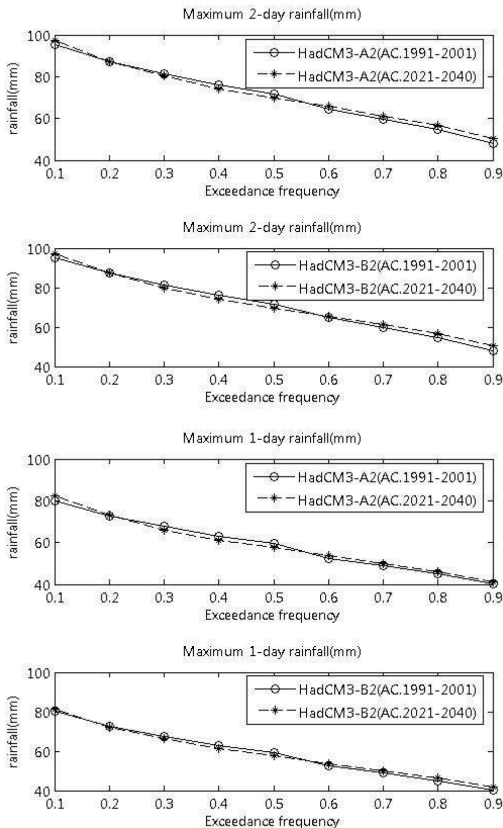
ภาพที่ ข.71 ปริมาณฝนสูงสุด 1 วัน และ 2 วัน ที่สังเคราะห์ได้จากภาพฉาย HadCM3-A2 และ HadCM3-B2 สำหรับสถานี 432005 (ปี ค.ศ. 1991-2001 และ ปี ค.ศ. 2021-2040)
