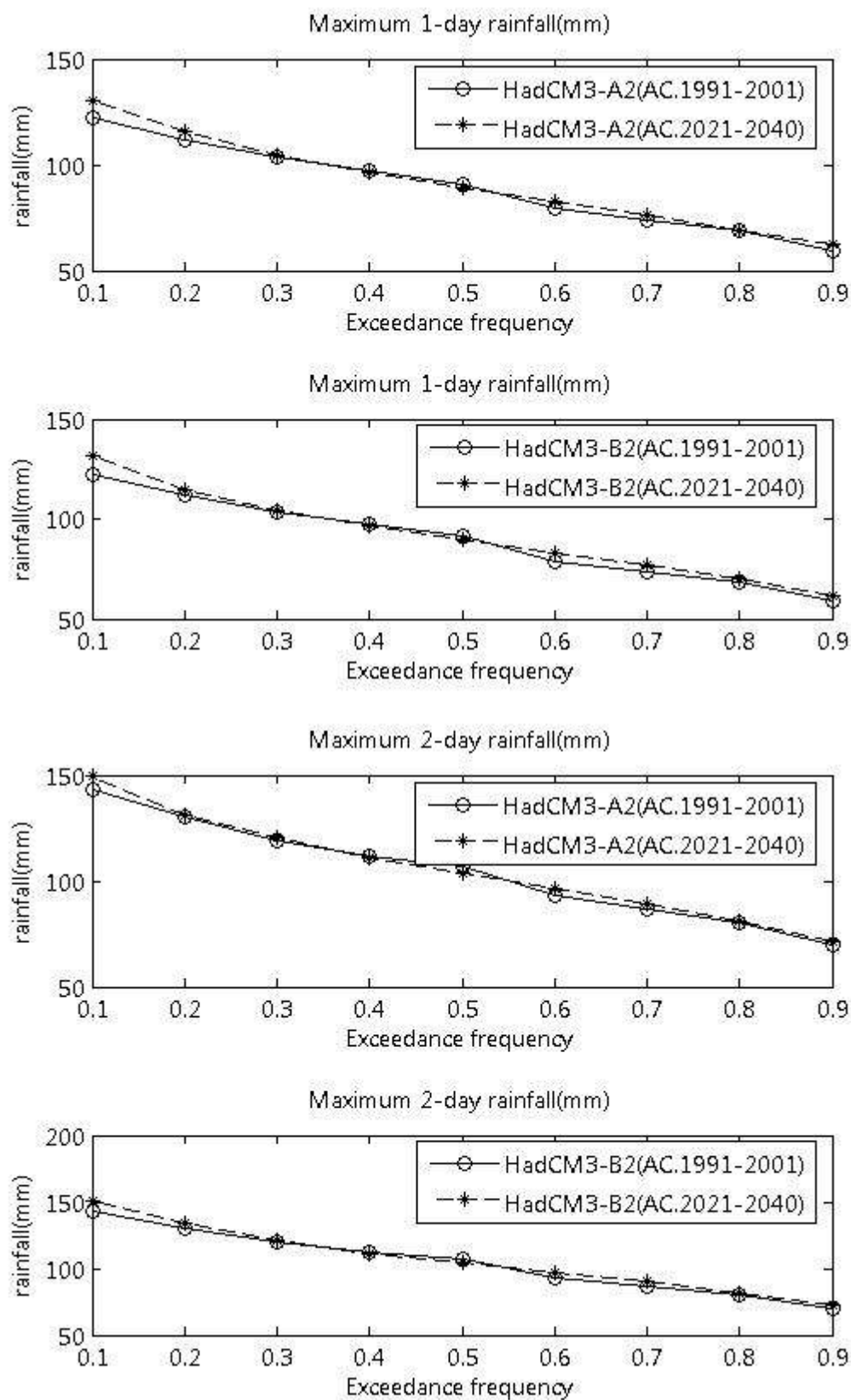
ภาพที่ ข.75 ปริมาณฝนสูงสุด 1 วัน และ 2 วัน ที่สังเคราะห์ได้จากภาพฉาย HadCM3-A2 และ HadCM3-B2 สำหรับสถานี 436004 (ปี ค.ศ. 1991-2001 และ ปี ค.ศ. 2021-2040)
