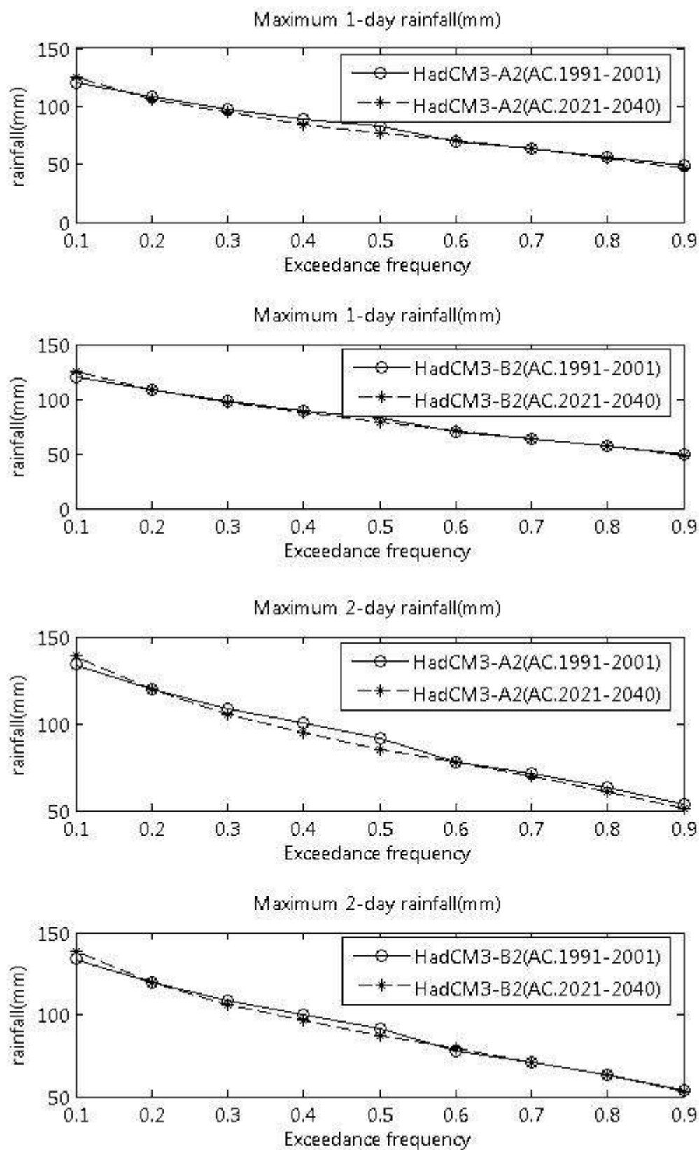
ภาพที่ ข.43 ปริมาณฝนสูงสุด 1 วัน และ 2 วัน ที่สังเคราะห์ได้จากภาพฉาย HadCM3-A2 และ HadCM3-B2 สำหรับสถานี 75052 (ปี ค.ศ. 1991-2001 และ ปี ค.ศ. 2021-2040)
