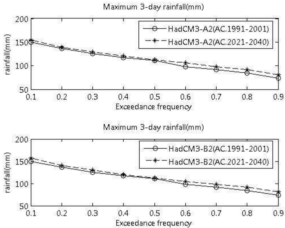
ภาพที่ ข.46 ปริมาณฝนสูงสุด 3 วัน ที่สังเคราะห์ได้จากภาพฉาย HadCM3-A2 และ HadCM3-B2 สำหรับสถานี 404003 (ปี ค.ศ. 1991-2001 และ ปี ค.ศ. 2021-2040)
