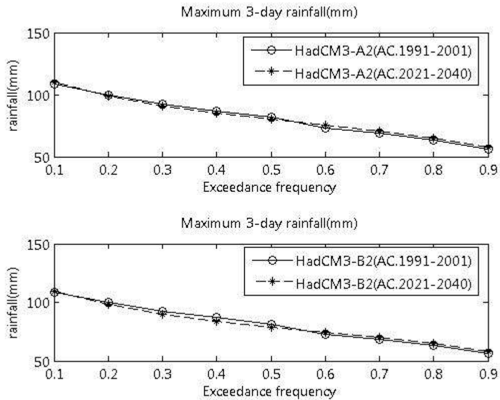
ภาพที่ ข.72 ปริมาณฝนสูงสุด 3 วัน ที่สังเคราะห์ได้จากภาพฉาย HadCM3-A2 และ HadCM3-B2 สำหรับสถานี 432005 (ปี ค.ศ. 1991-2001 และ ปี ค.ศ. 2021-2040)
