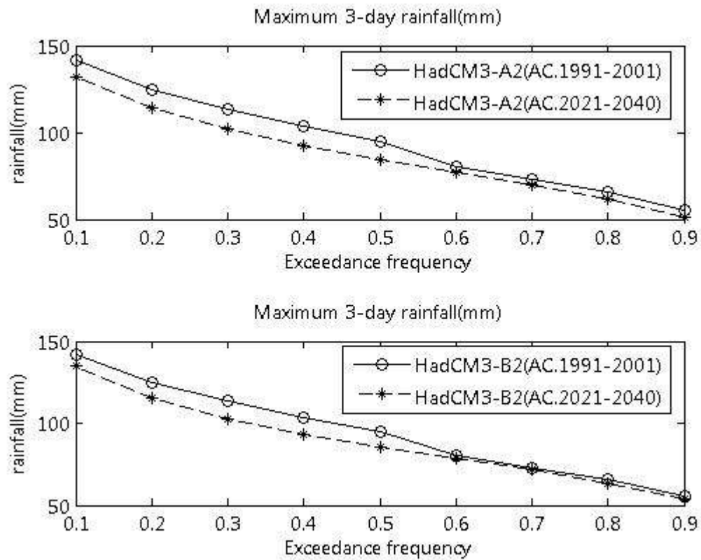
ภาพที่ ข.8 ปริมาณฝนสูงสุด 3 วัน ที่สังเคราะห์ได้จากภาพฉาย HadCM3-A2 และ HadCM3-B2 สำหรับ 05092 (ปี ค.ศ. 1991-2001 และ ปี ค.ศ. 2021-2040)
