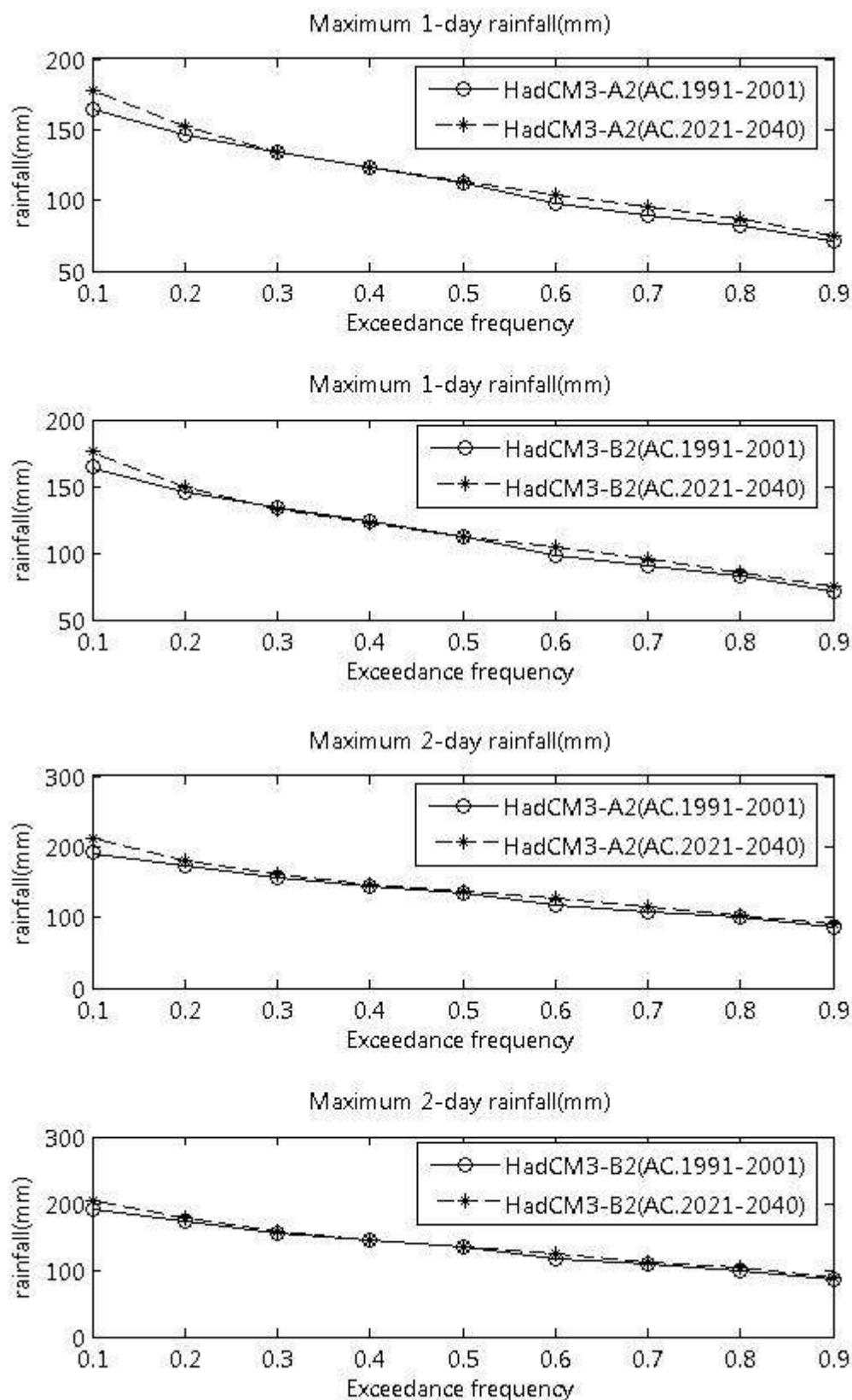
ภาพที่ ข.39 ปริมาณฝนสูงสุด 1 วัน และ 2 วัน ที่สังเคราะห์ได้จากภาพฉาย HadCM3-A2 และ HadCM3-B2 สำหรับสถานี 72022 (ปี ค.ศ. 1991-2001 และ ปี ค.ศ. 2021-2040)
