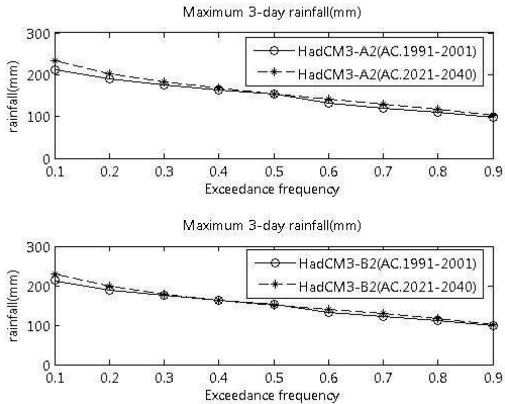
ภาพที่ ข.40 ปริมาณฝนสูงสุด 3 วัน ที่สังเคราะห์ได้จากภาพฉาย HadCM3-A2 และ HadCM3-B2 สำหรับสถานี 72022 (ปี ค.ศ. 1991-2001 และ ปี ค.ศ. 2021-2040)
