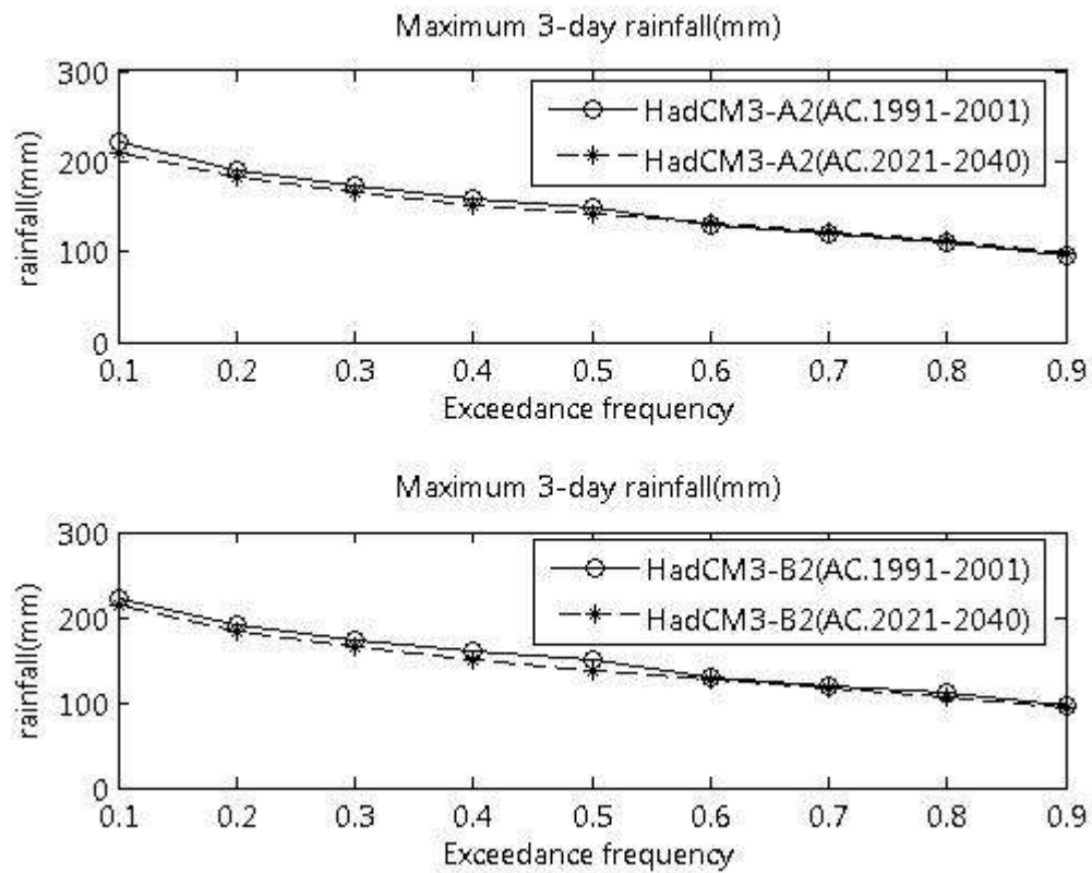
ภาพที่ ข.12 ปริมาณฝนสูงสุด 3 วัน ที่สังเคราะห์ได้จากภาพฉาย HadCM3-A2 และ HadCM3-B2 สำหรับสถานี สถานี 11022 (ปี ค.ศ. 1991-2001 และ ปี ค.ศ. 2021-2040)
