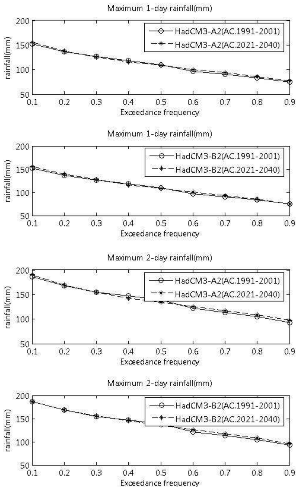
ภาพที่ ข.59 ปริมาณฝนสูงสุด 1 วัน และ 2 วัน ที่สังเคราะห์ได้จากภาพฉาย HadCM3-A2 และ HadCM3-B2 สำหรับสถานี 407006 (ปี ค.ศ. 1991-2001 และ ปี ค.ศ. 2021-2040)
