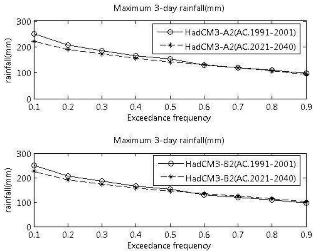
ภาพที่ ข.82 ปริมาณฝนสูงสุด 3 วัน ที่สังเคราะห์ได้จากภาพฉาย HadCM3-A2 และ HadCM3-B2 สำหรับสถานี 436007 (ปี ค.ศ. 1991-2001 และ ปี ค.ศ. 2021-2040)
