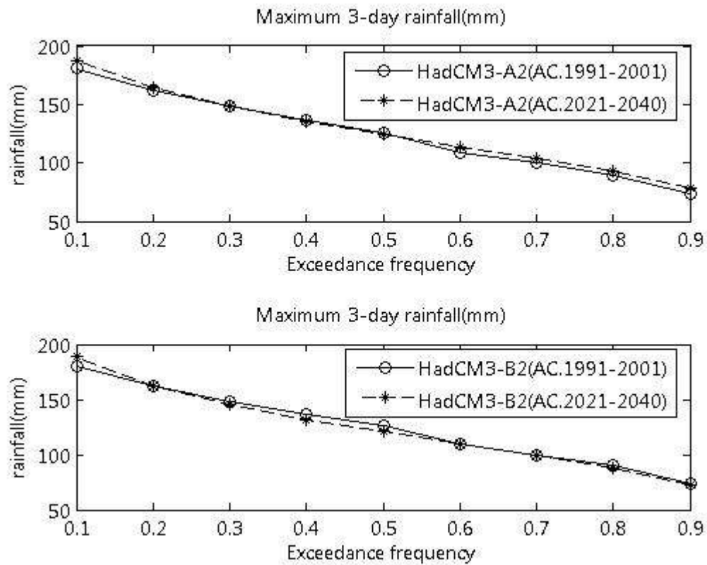
ภาพที่ ข.38 ปริมาณฝนสูงสุด 3 วัน ที่สังเคราะห์ได้จากภาพฉาย HadCM3-A2 และ HadCM3-B2 สำหรับสถานี 68150 (ปี ค.ศ. 1991-2001 และ ปี ค.ศ. 2021-2040)
