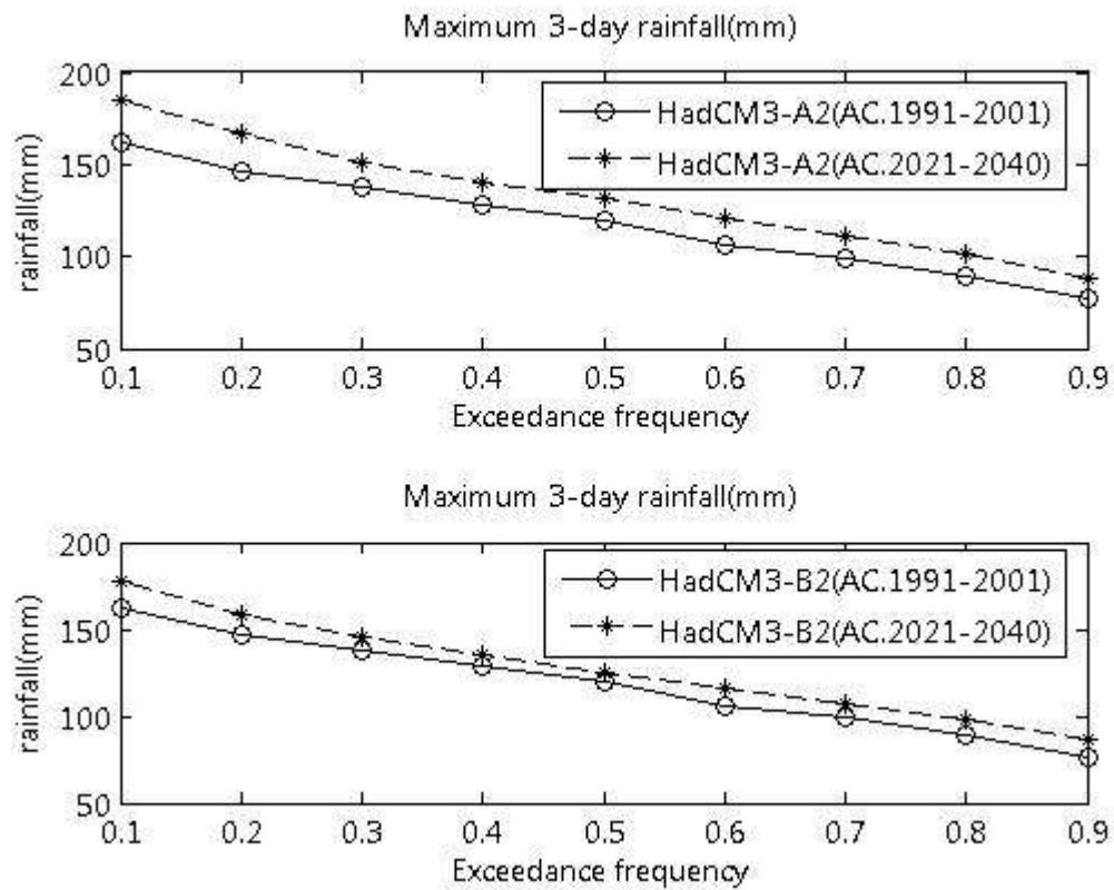
ภาพที่ ข.16 ปริมาณฝนสูงสุด 3 วัน ที่สังเคราะห์ได้จากภาพฉาย HadCM3-A2 และ HadCM3-B2 สำหรับสถานี 11202 (ปี ค.ศ. 1991-2001 และ ปี ค.ศ. 2021-2040)
