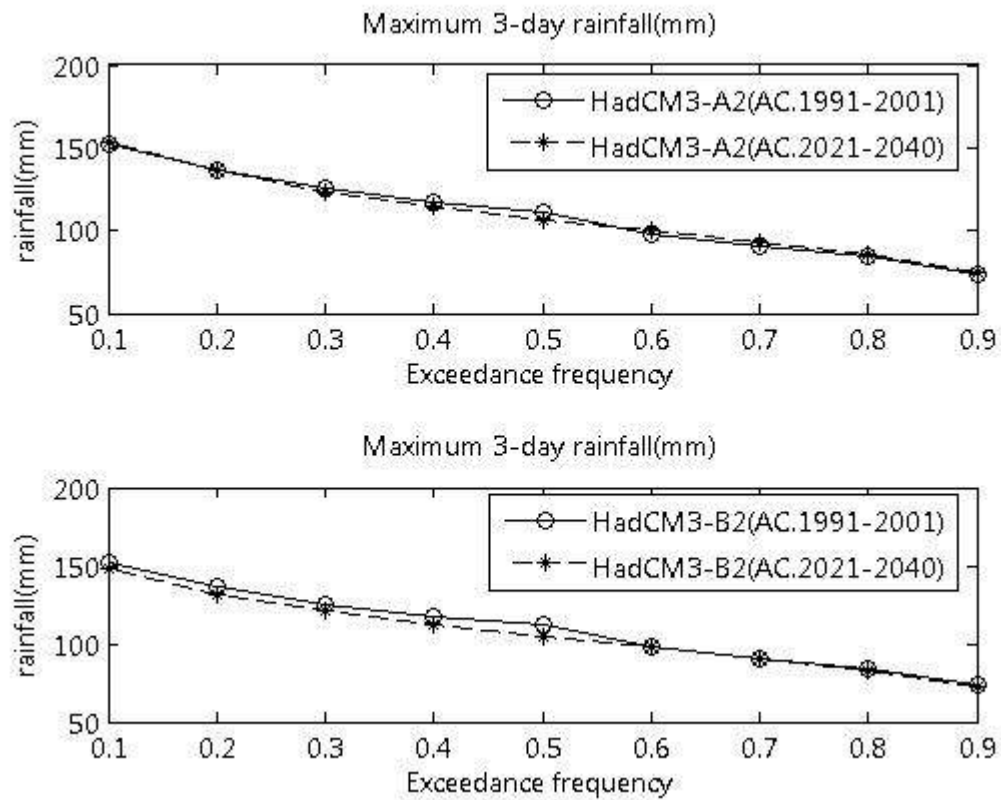
ภาพที่ ข.66 ปริมาณฝนสูงสุด 3 วัน ที่สังเคราะห์ได้จากภาพฉาย HadCM3-A2 และ HadCM3-B2 สำหรับสถานี 409004 (ปี ค.ศ. 1991-2001 และ ปี ค.ศ. 2021-2040)
