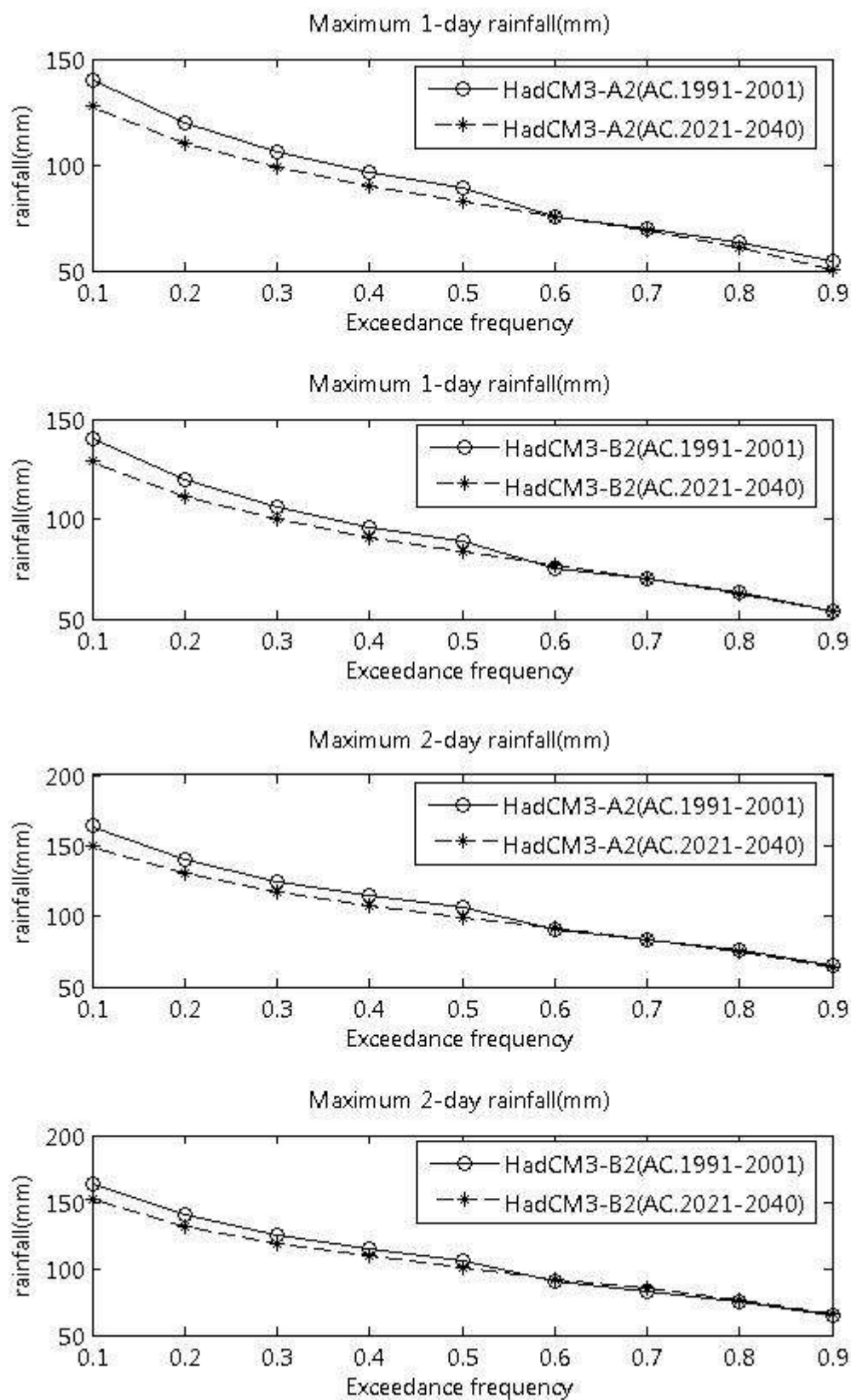
ภาพที่ ข.3 ปริมาณฝนสูงสุด 1 วัน และ 2 วัน ที่สังเคราะห์ได้จากภาพฉาย HadCM3-A2 และ HadCM3-B2 สำหรับสถานี 05023 (ปี ค.ศ. 1991-2001 และ ปี ค.ศ. 2021-2040)
