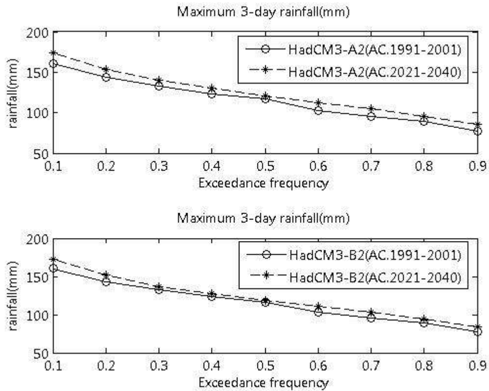
ภาพที่ ข.26 ปริมาณฝนสูงสุด 3 วัน ที่สังเคราะห์ได้จากภาพฉาย HadCM3-A2 และ HadCM3-B2 สถานี 18073 (ปี ค.ศ. 1991-2001 และ ปี ค.ศ. 2021-2040)
