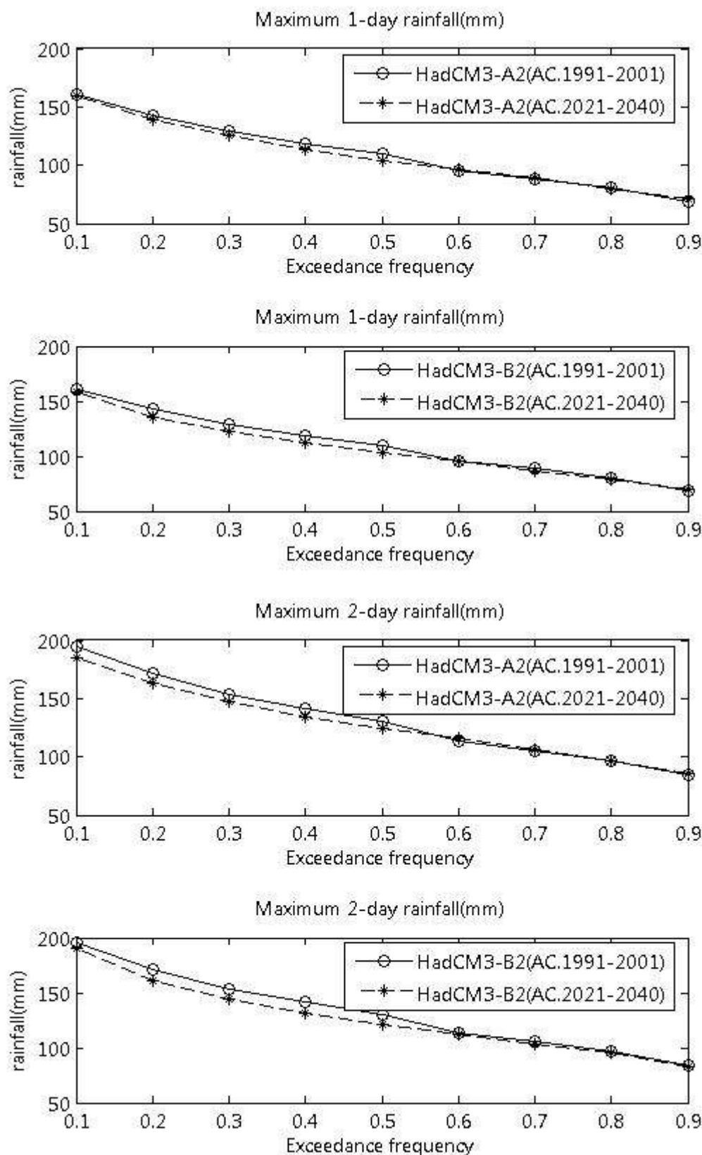
ภาพที่ ข.11 ปริมาณฝนสูงสุด 1 วัน และ 2 วัน ที่สังเคราะห์ได้จากภาพฉาย HadCM3-A2 และ HadCM3-B2 สำหรับสถานี สถานี 11022 (ปี ค.ศ. 1991-2001 และ ปี ค.ศ. 2021-2040)
