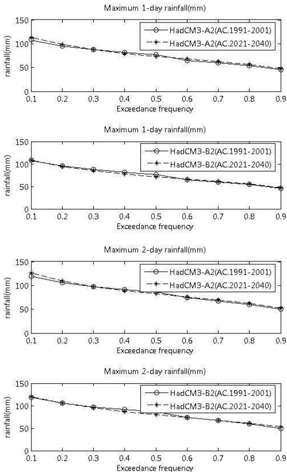
ภาพที่ ข.21 ปริมาณฝนสูงสุด 1 วัน และ 2 วัน ที่สังเคราะห์ได้จากภาพฉาย HadCM3-A2 และ HadCM3-B2 สำหรับสถานี 14062 (ปี ค.ศ. 1991-2001 และ ปี ค.ศ. 2021-2040)
