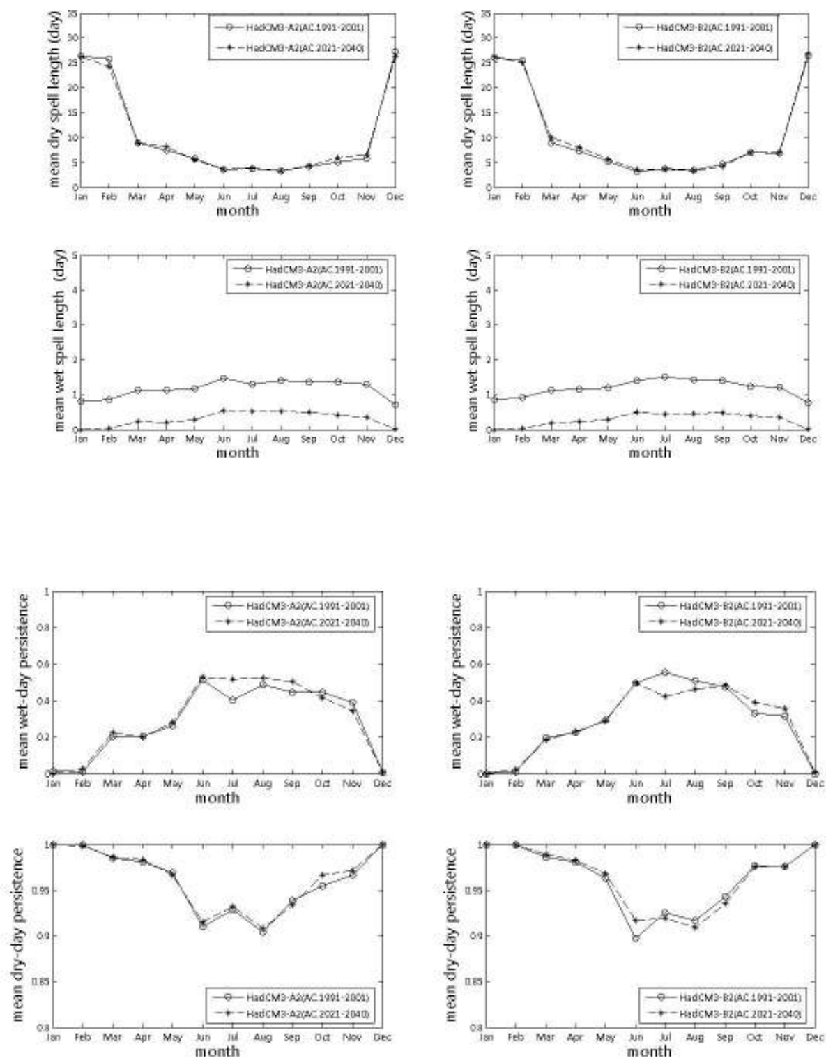
ภาพที่ ข.34 ช่วงเวลาที่ฝนไม่ตก ช่วงเวลาที่ฝนตก จำนวนครั้งสัมพัทธ์ที่ฝนตก จำนวนครั้งสัมพัทธ์ที่ฝนไม่ตกจากภาพฉาย HadCM3-A2 และ HadCM3-B2 สำหรับสถานี 49062 (ปี ค.ศ.1991-2001 และ ปี ค.ศ.2020-2040)
