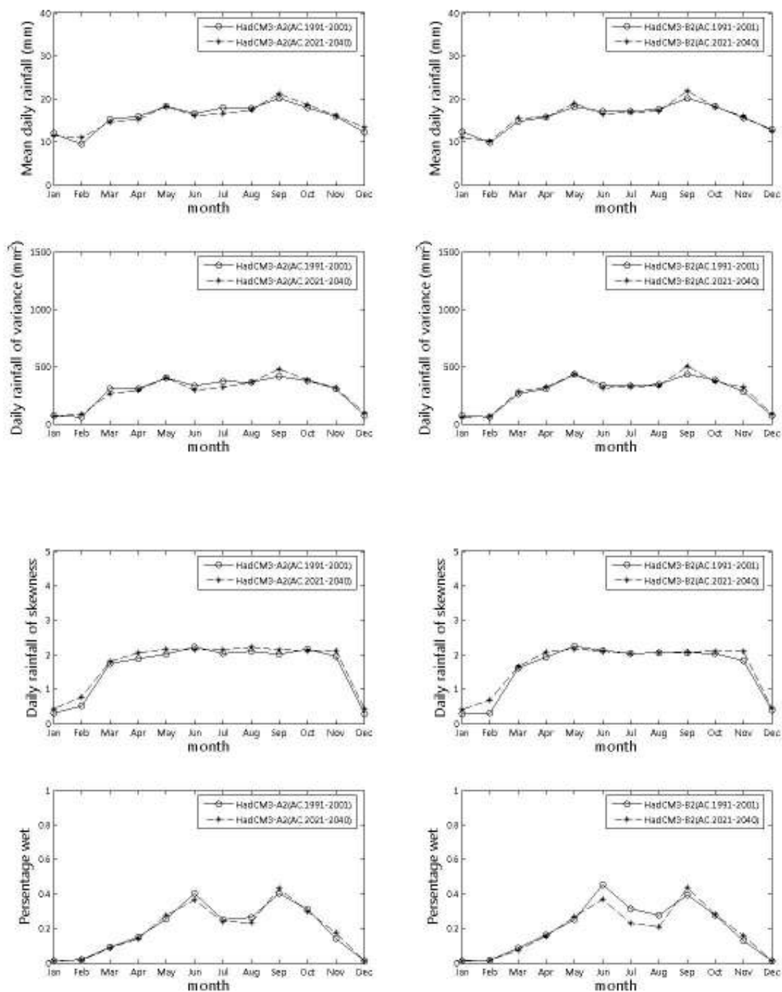
ภาพที่ ๑.13 ค่าเฉลี่ย ค่าความแปรปรวน ค่าสัมประสิทธิ์ความเบ้ และเปอร์เซ็นต์ฝนตก ที่ได้จากภาพฉาย HadCM3-A2 และ HadCM3-B2 สำหรับสถานี 11170 (ปี ค.ศ.1991-2001 และ ปี ค.ศ.2020-2040)
