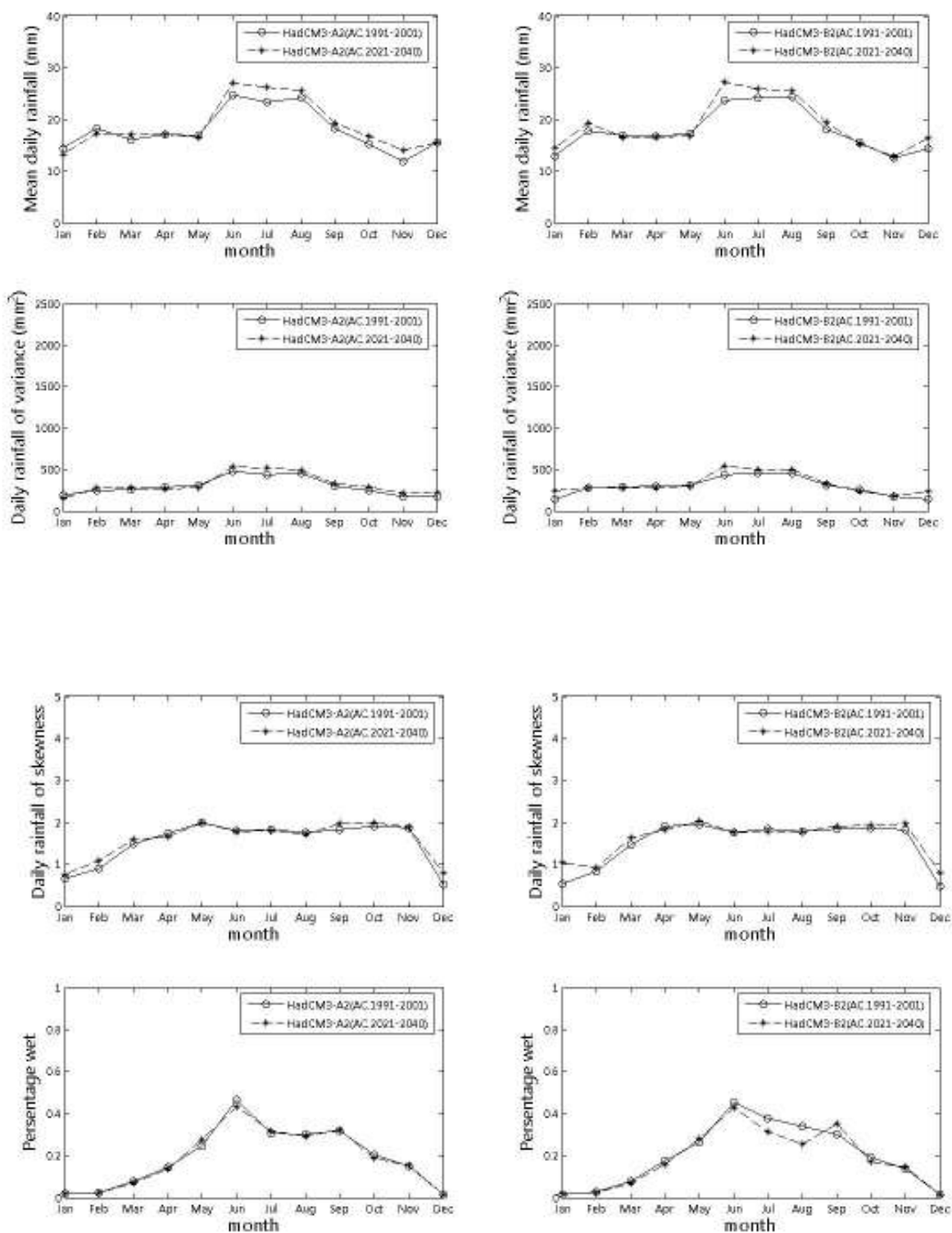
ภาพที่ ข.41 ค่าเฉลี่ย ความแปรปรวน สัมประสิทธิ์ความเบ้ และเปอร์เซ็นต์ฝนตก ที่ได้จากภาพฉาย HadCM3-A2 และ HadCM3-B2 สำหรับสถานี 75032 (ปี ค.ศ.1991-2001 และ ปี ค.ศ.2020-2040)
