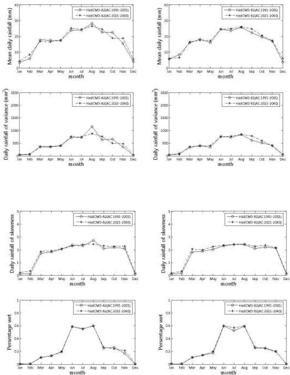
ภาพที่ ๑.๔๗ ค่าเฉลี่ย ค่าความแปรปรวน ค่าสัมประสิทธิ์ความเบ้ และเปอร์เซ็นต์ฝนตก ที่ได้จากภาพฉาย HadCM3-A2 และ HadCM3-B2 สำหรับสถานี 405002 (ปี ค.ศ.1991-2001 และ ปี ค.ศ. 2020-2040)
