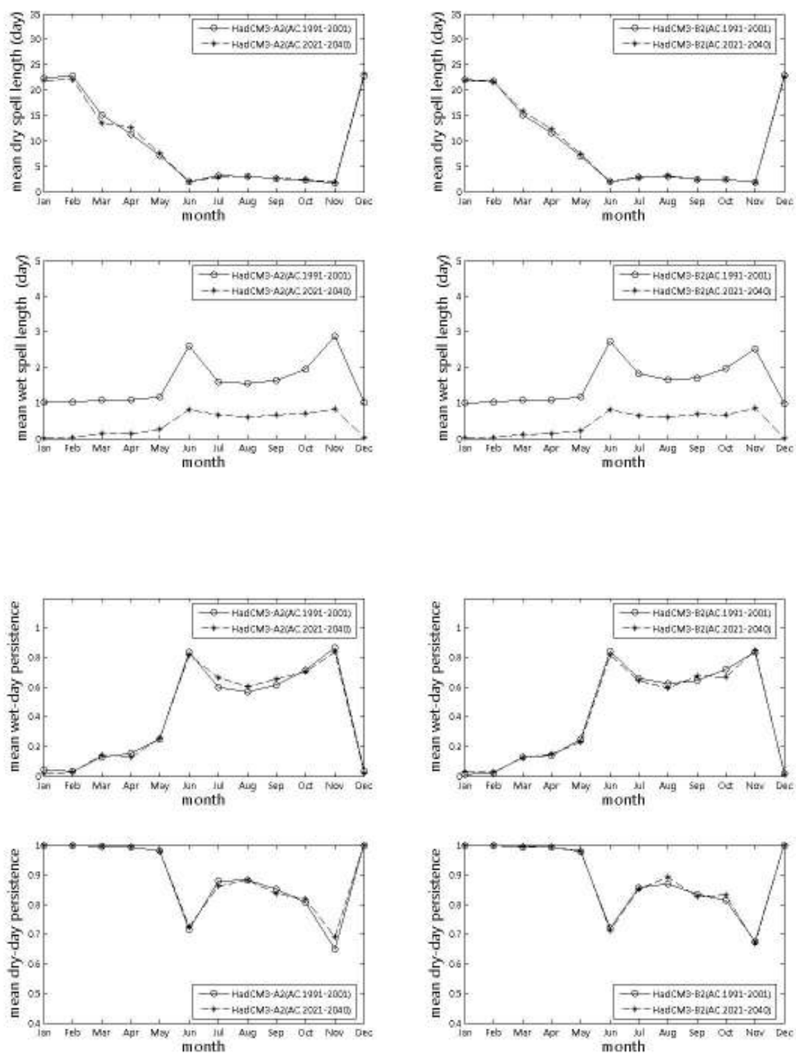
ภาพที่ ข.68 ช่วงเวลาที่ฝนไม่ตก ช่วงเวลาที่ฝนตก จำนวนครั้งสัมพัทธ์ที่ฝนตก จำนวนครั้งสัมพัทธ์ที่ฝนไม่ตกจากภาพฉาย HadCM3-A2 และ HadCM3-B2 สำหรับสถานี 432001 (ปี ค.ศ.1991-2001 และ ปี ค.ศ.2020-2040)
