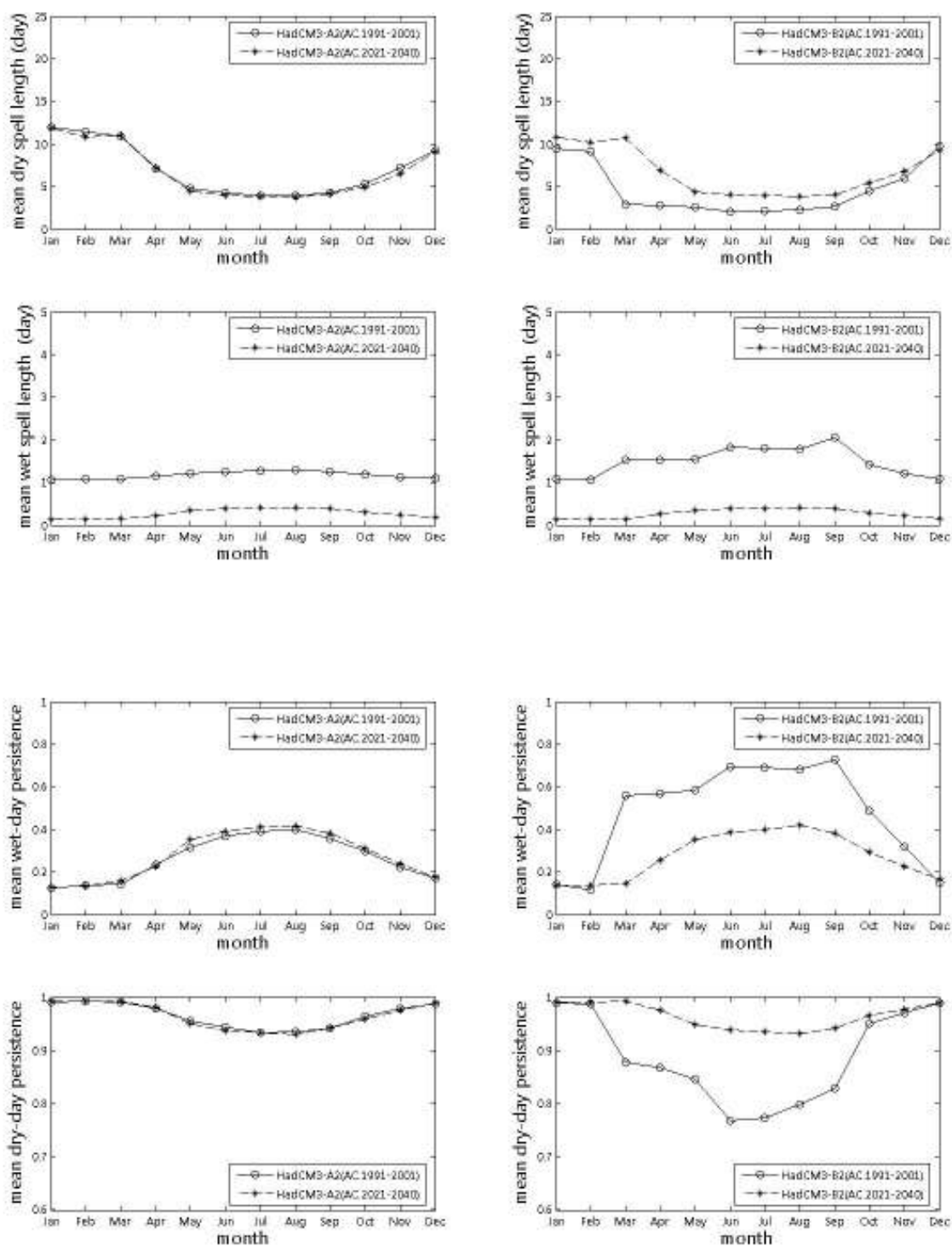
ภาพที่ ๑.6 ช่วงเวลาที่ฝนไม่ตก ช่วงเวลาที่ฝนตก จำนวนครั้งสัมพัทธ์ที่ฝนตก จำนวนครั้งสัมพัทธ์ที่ฝนไม่ตกจากภาพฉาย HadCM3-A2 และ HadCM3-B2 สำหรับสถานี 05032 (ปี ค.ศ.1991-2001 และ ปี ค.ศ.2020-2040)
