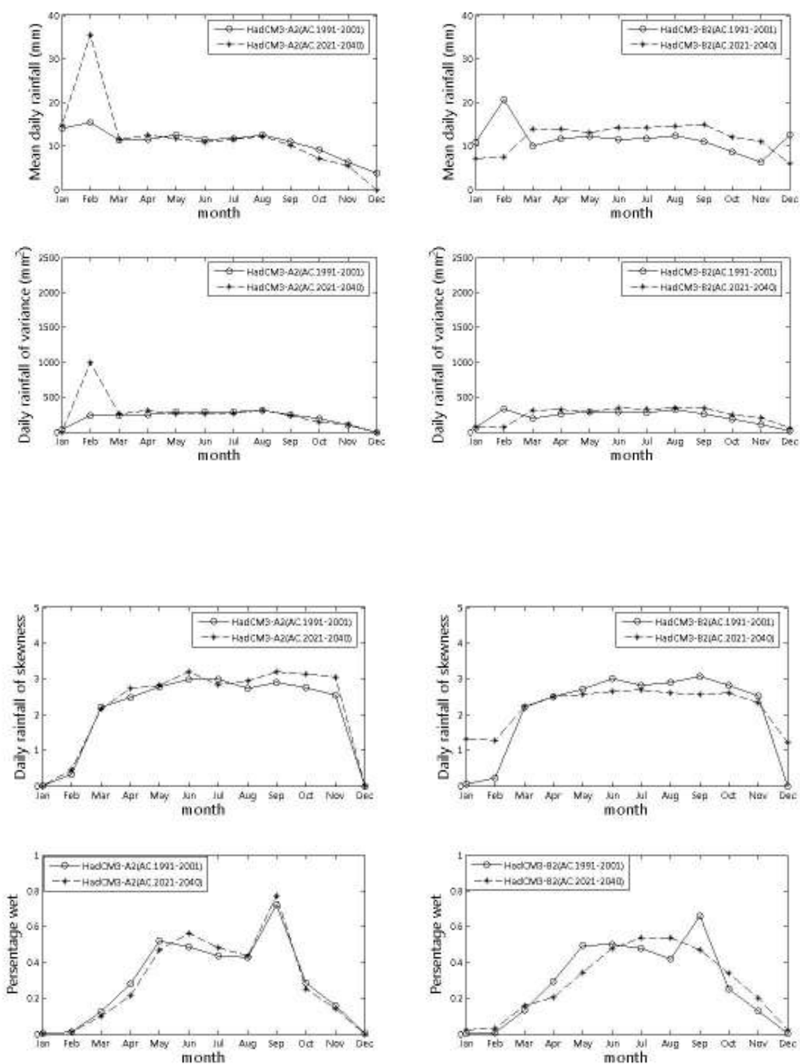
ภาพที่ ข.31 ค่าเฉลี่ย ค่าความแปรปรวน ค่าสัมประสิทธิ์ความเบ้ และเปอร์เซ็นต์ฝนตก ที่ได้จากภาพฉาย HadCM3-A2 และ HadCM3-B2 สำหรับสถานี 49013 (ปี ค.ศ.1991-2001 และ ปี ค.ศ.2020-2040)
