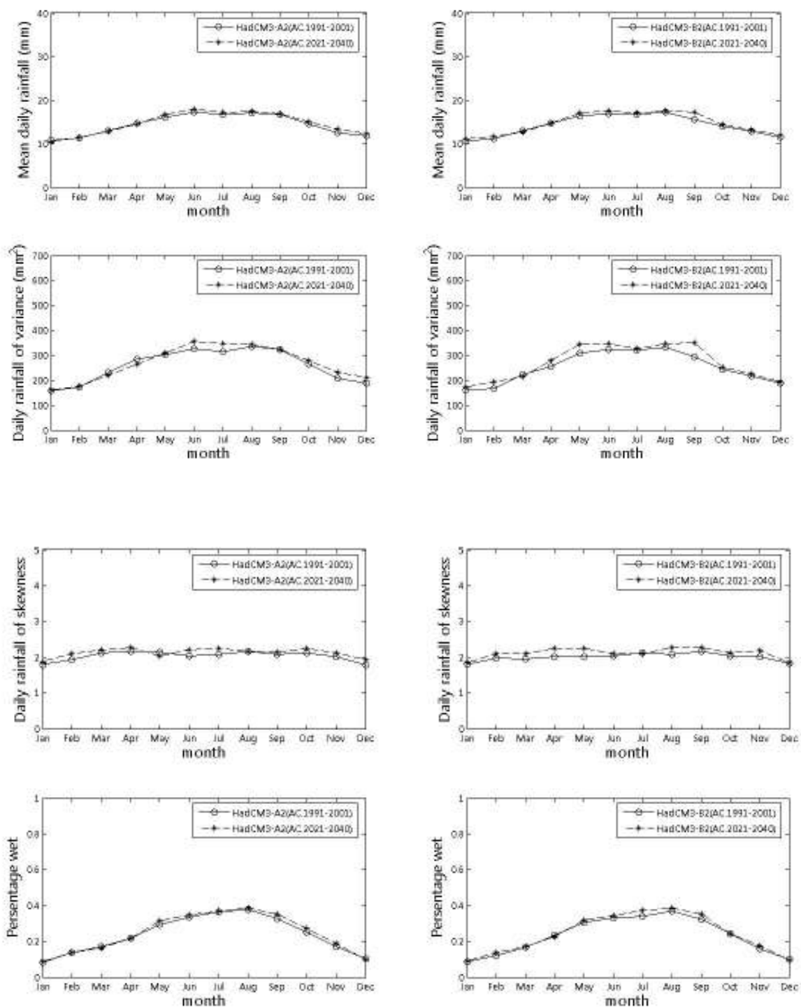
ภาพที่ ๑.๒๗ ค่าเฉลี่ย ค่าความแปรปรวน ค่าสัมประสิทธิ์ความเบ้ และเปอร์เซ็นต์ฝนตก ที่ได้จากภาพฉาย HadCM3-A2 และ HadCM3-B2 สถานี 21043 (ปี ค.ศ.1991-2001 และ ปี ค.ศ.2020-2040)
