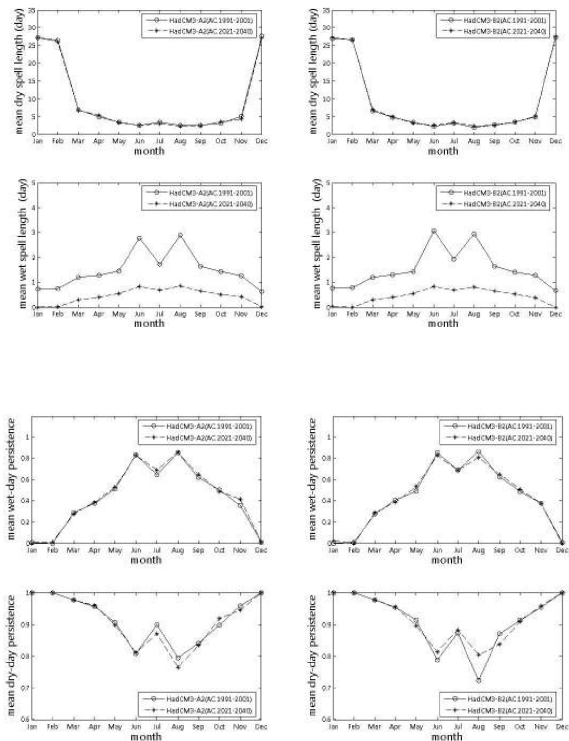
ภาพที่ ข.60 ช่วงเวลาที่ฝนไม่ตก ช่วงเวลาที่ฝนตก จำนวนครั้งสัมพัทธ์ที่ฝนตก จำนวนครั้งสัมพัทธ์ที่ฝนไม่ตกจากภาพฉาย HadCM3-A2 และ HadCM3-B2 สำหรับสถานี 407006 (ปี ค.ศ.1991-2001 และ ปี ค.ศ.2020-2040)
