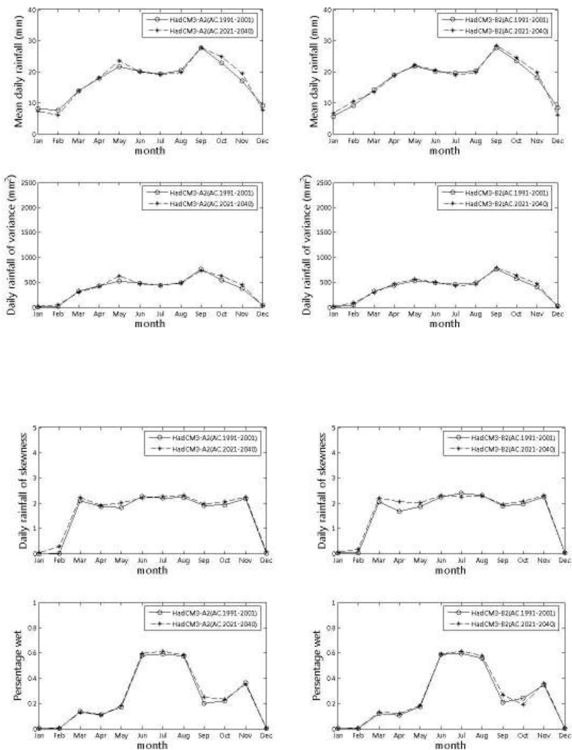
ภาพที่ ข.51 ค่าเฉลี่ย ค่าความแปรปรวน ค่าสัมประสิทธิ์ความเบ้ และเปอร์เซ็นต์ฝนตก ที่ได้จากภาพฉาย HadCM3-A2 และ HadCM3-B2 สำหรับสถานี 406002 (ปี ค.ศ.1991-2001 และ ปี ค.ศ. 2020-2040)
