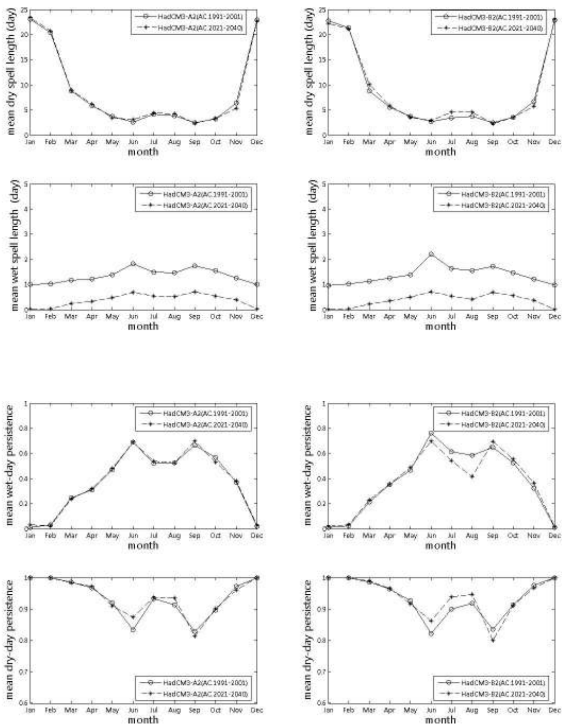
ภาพที่ ๑.14 ช่วงเวลาที่ฝนไม่ตก ช่วงเวลาที่ฝนตก จำนวนครั้งสัมพัทธ์ที่ฝนตก จำนวนครั้งสัมพัทธ์ที่ฝนไม่ตกจากภาพฉาย HadCM3-A2 และ HadCM3-B2 สำหรับสถานี 11170 (ปี ค.ศ.1991-2001 และ ปี ค.ศ.2020-2040)
