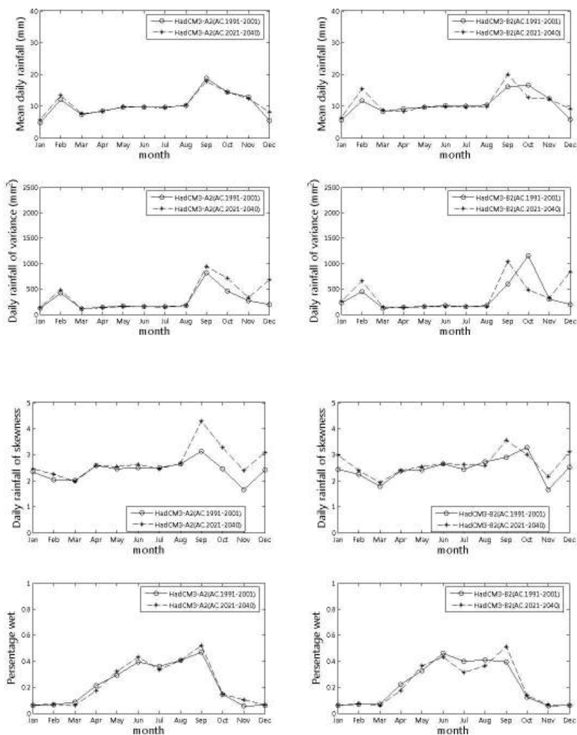
ภาพที่ ๑.๙ ค่าเฉลี่ย ค่าความแปรปรวน ค่าสัมประสิทธิ์ความเบ้ และเปอร์เซ็นต์ฝนตก ที่ได้จากภาพฉาย HadCM3-A2 และ HadCM3-B2 สำหรับสถานี 05171 (ปี ค.ศ.1991-2001 และ ปี ค.ศ.2020-2040)
