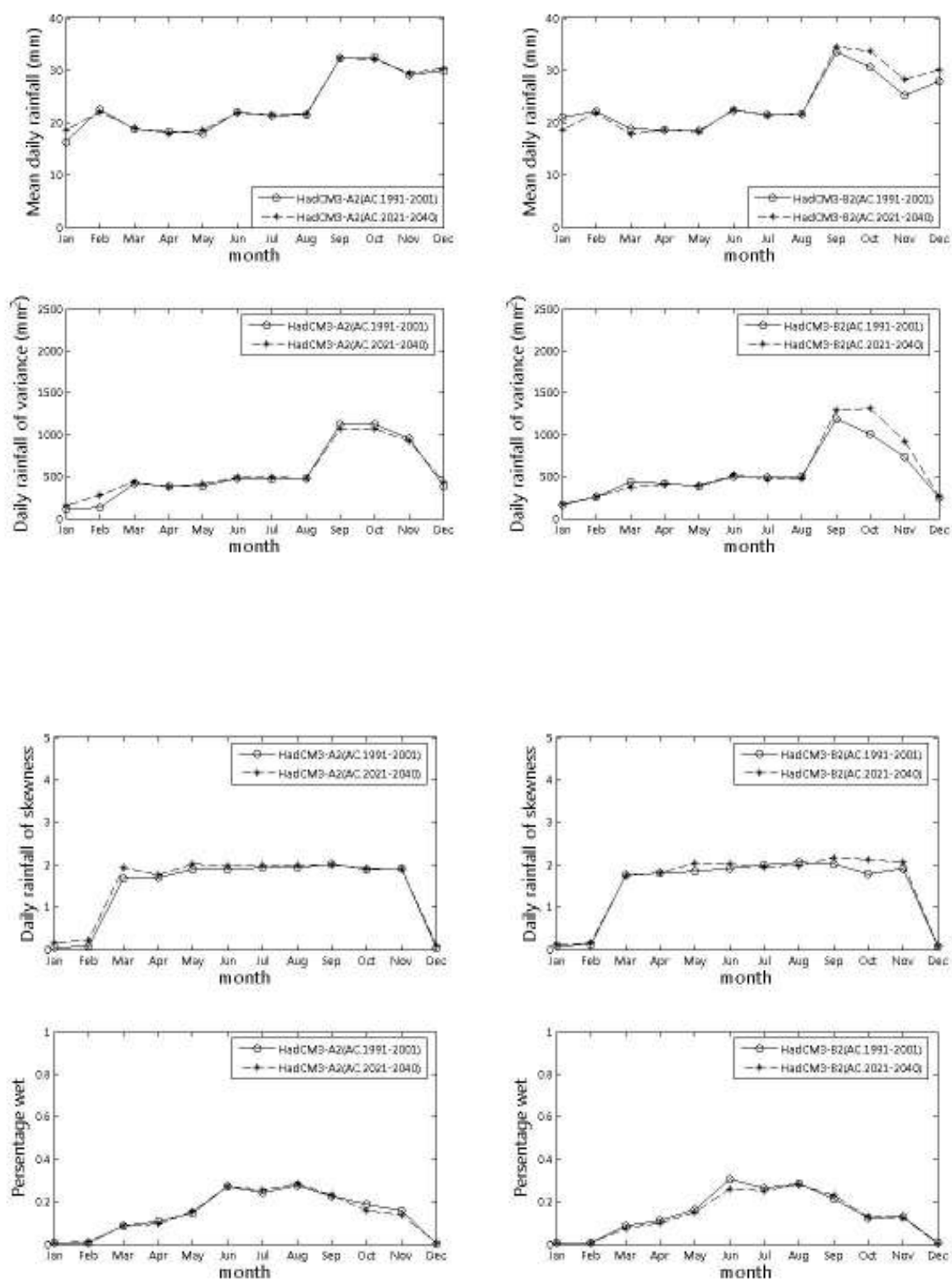
ภาพที่ ข.33 ค่าเฉลี่ย ค่าความแปรปรวน ค่าสัมประสิทธิ์ความเบ้ และเปอร์เซ็นต์ฝนตก ที่ได้จากภาพฉาย HadCM3-A2 และ HadCM3-B2 สำหรับสถานี 49062 (ปี ค.ศ.1991-2001 และ ปี ค.ศ.2020-2040)
