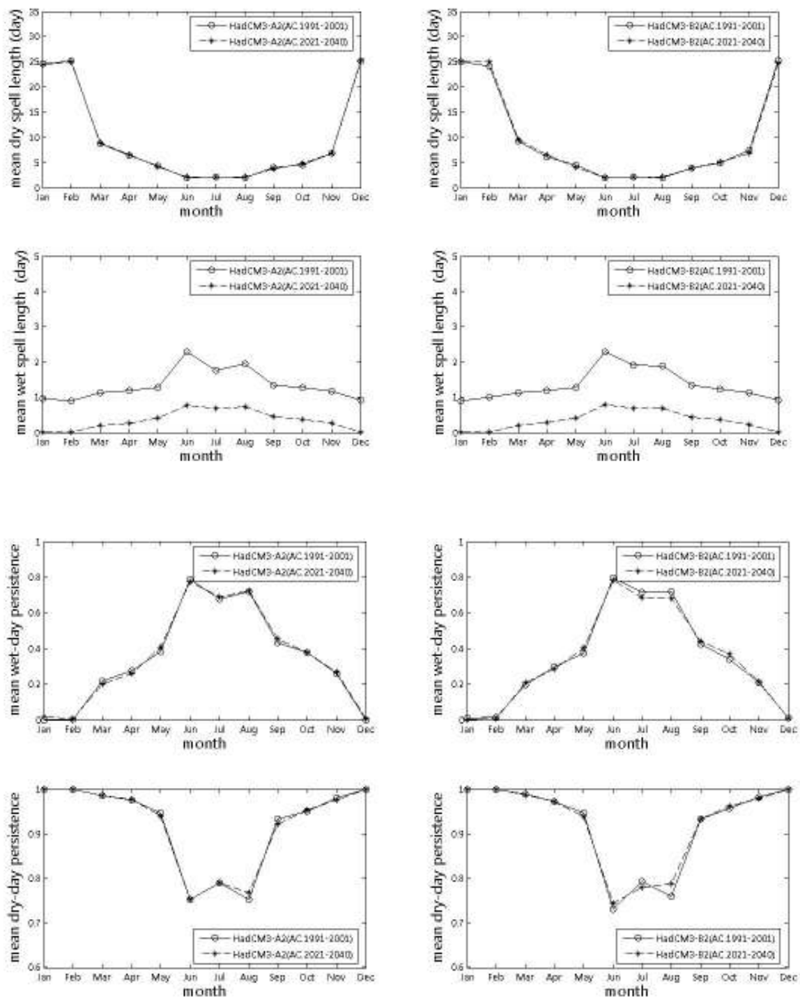
ภาพที่ ข.56 ช่วงเวลาที่ฝนไม่ตก ช่วงเวลาที่ฝนตก จำนวนครั้งสัมพัทธ์ที่ฝนตก จำนวนครั้งสัมพัทธ์ที่ฝนไม่ตกจากภาพฉาย HadCM3-A2 และ HadCM3-B2 สำหรับสถานี 406005 (ปี ค.ศ.1991-2001 และ ปี ค.ศ.2020-2040)
