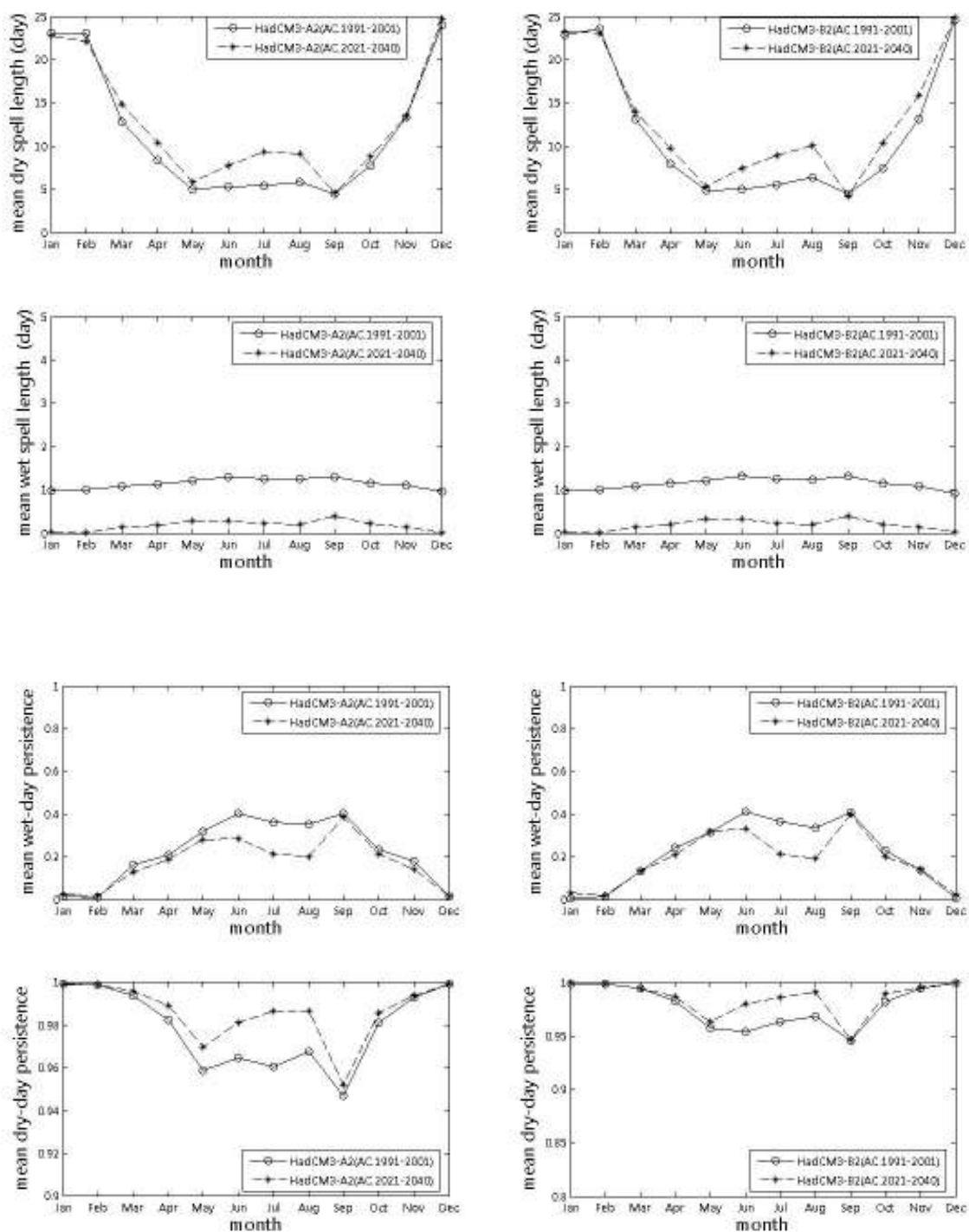
ภาพที่ ๘.8 ช่วงเวลาที่ฝนไม่ตก ช่วงเวลาที่ฝนตก จำนวนครั้งสัมพัทธ์ที่ฝนตก จำนวนครั้งสัมพัทธ์ที่ฝนไม่ตกจากภาพฉาย HadCM3-A2 และ HadCM3-B2 สำหรับสถานี 05092 (ปี ค.ศ.1991-2001 และ ปี ค.ศ.2020-2040)
