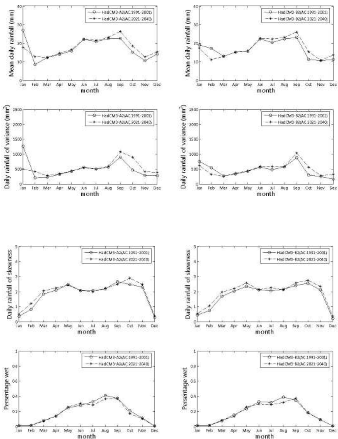
ภาพที่ ข.39 ค่าเฉลี่ย ค่าความแปรปรวน ค่าสัมประสิทธิ์ความเบ้ และเปอร์เซ็นต์ฝนตก ที่ได้จากภาพฉาย HadCM3-A2 และ HadCM3-B2 สำหรับสถานี 7202 (ปี ค.ศ.1991-2001 และ ปี ค.ศ.2020-2040)
