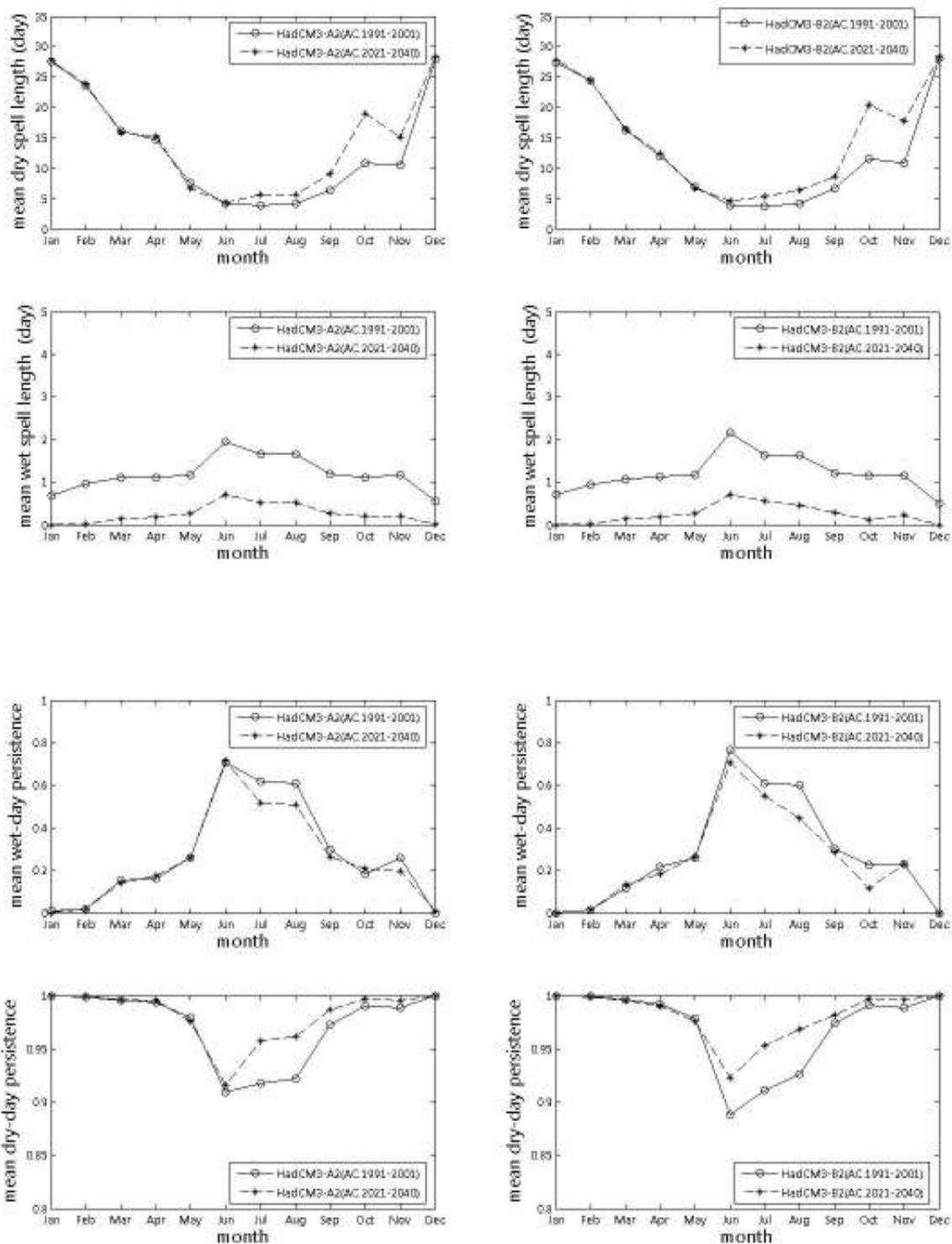
ภาพที่ ข.38 ช่วงเวลาที่ฝนไม่ตก ช่วงเวลาที่ฝนตก จำนวนครั้งสัมพัทธ์ที่ฝนตก จำนวนครั้งสัมพัทธ์ที่ฝนไม่ตกจากภาพฉาย HadCM3-A2 และ HadCM3-B2 สำหรับสถานี 68150 (ปี ค.ศ.1991-2001 และ ปี ค.ศ.2020-2040)
