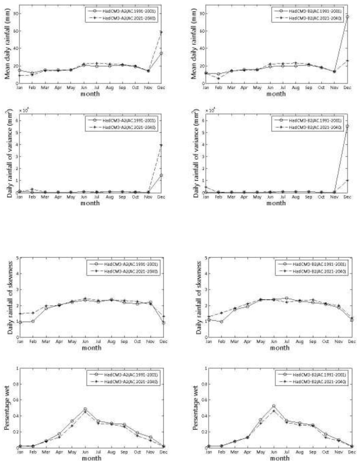
ภาพที่ ๑.17 ค่าเฉลี่ย ค่าความแปรปรวน ค่าสัมประสิทธิ์ความเบ้ และเปอร์เซ็นต์ฝนตก ที่ได้จากภาพฉาย HadCM3-A2 และ HadCM3-B2 สำหรับสถานี 11210 (ปี ค.ศ.1991-2001 และ ปี ค.ศ.2020-2040)
