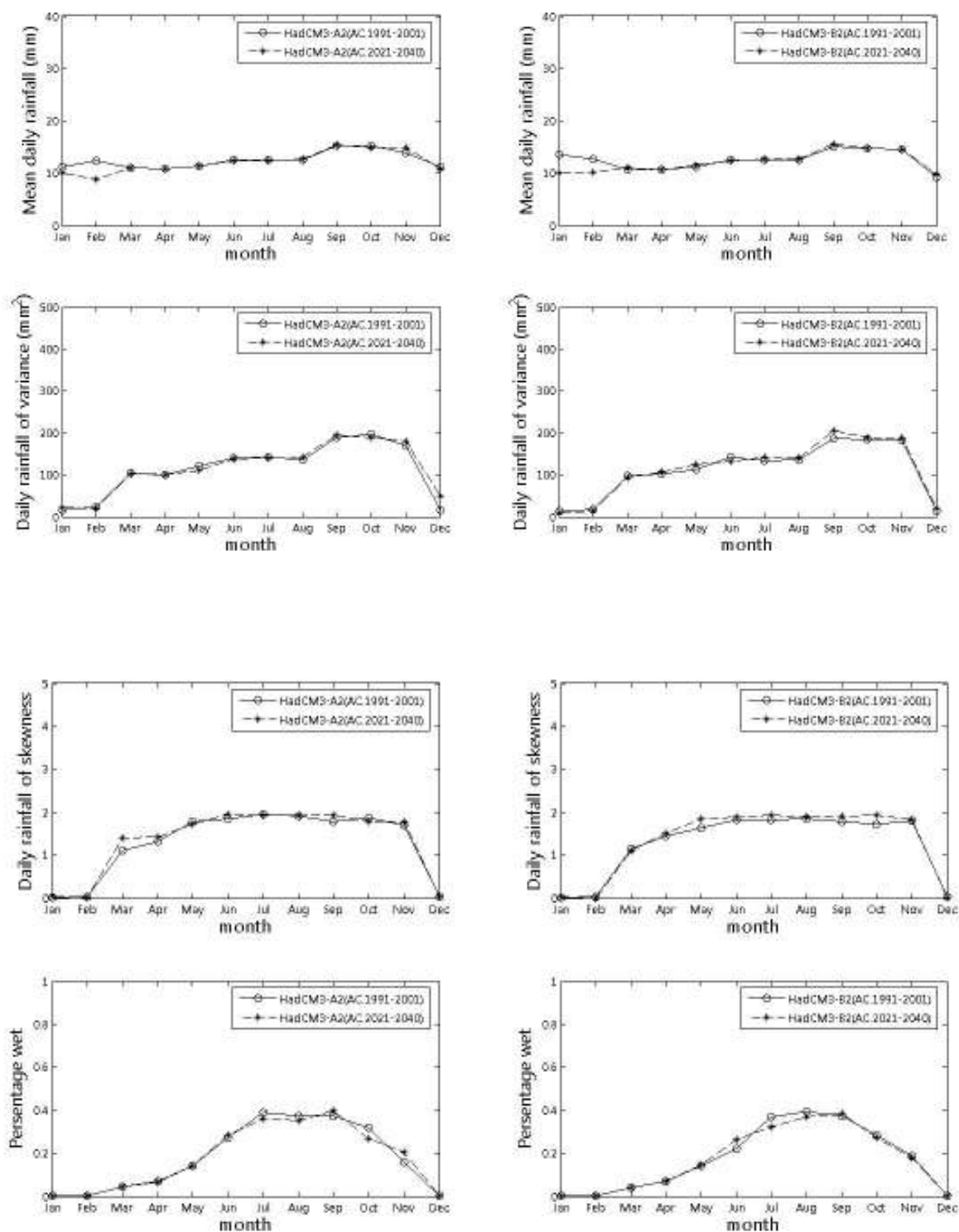
ภาพที่ จ.71 ค่าเฉลี่ย ค่าความแปรปรวน ค่าสัมประสิทธิ์ความเบ้ และเปอร์เซ็นต์ฝนตก ที่ได้จากภาพฉาย HadCM3-A2 และ HadCM3-B2 สำหรับสถานี 432005 (ปี ค.ศ.1991-2001 และ ปี ค.ศ. 2020-2040)
