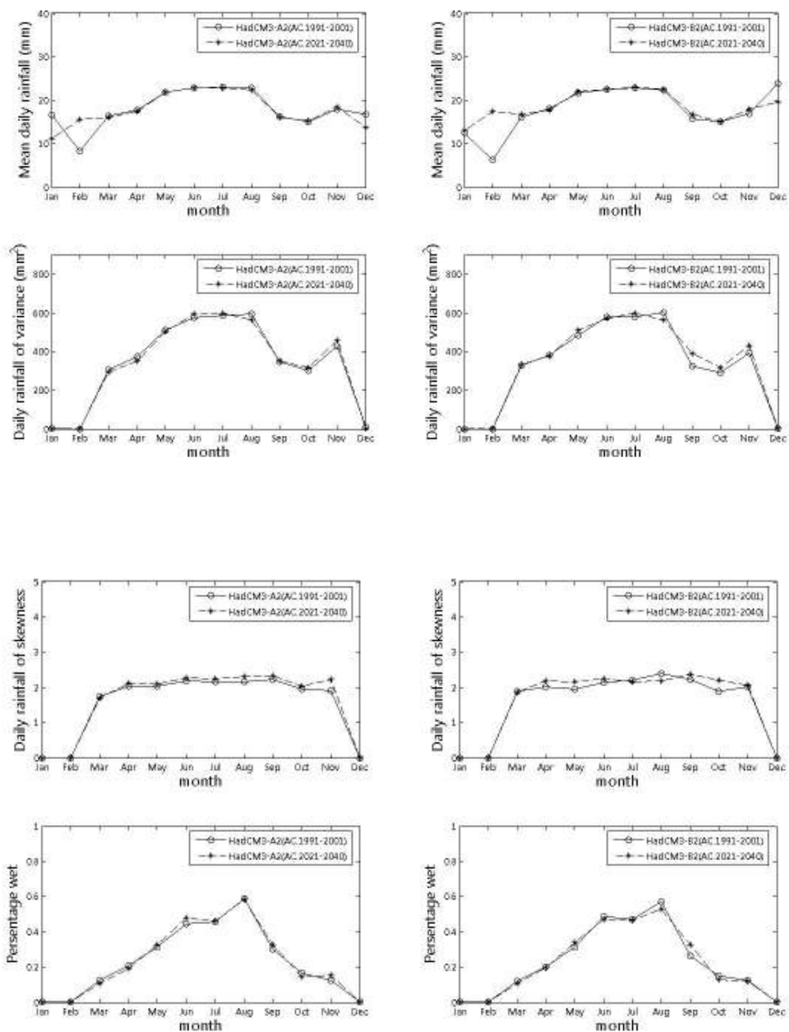
ภาพที่ ข.53 ค่าเฉลี่ย ค่าความแปรปรวน ค่าสัมประสิทธิ์ความเบ้ และเปอร์เซ็นต์ฝนตก ที่ได้จากภาพฉาย HadCM3-A2 และ HadCM3-B2 สำหรับสถานี 406004 (ปี ค.ศ.1991-2001 และ ปี ค.ศ. 2020-2040)
