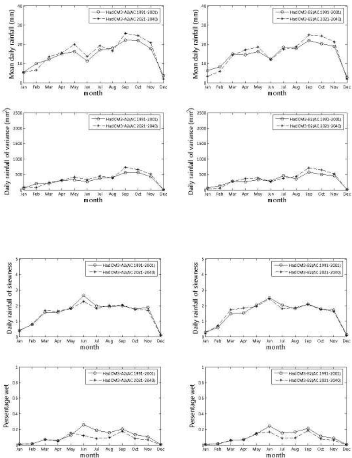
ภาพที่ ๔.๔๓ ค่าเฉลี่ย ค่าความแปรปรวน ค่าสัมประสิทธิ์ความเบ้ และเปอร์เซ็นต์ฝนตก ที่ได้จากภาพฉาย HadCM3-A2 และ HadCM3-B2 สำหรับสถานี 75052 (ปี ค.ศ.1991-2001 และ ปี ค.ศ.2020-2040)
