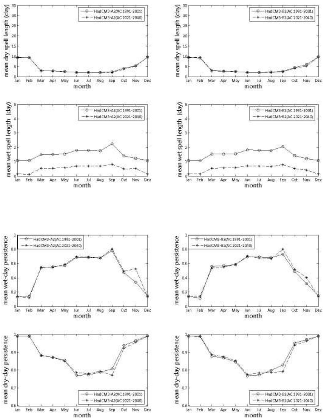
ภาพที่ ๑.๒ ช่วงเวลาที่ฝนไม่ตก ช่วงเวลาที่ฝนตก จำนวนครั้งสัมพัทธ์ที่ฝนตก จำนวนครั้งสัมพัทธ์ที่ฝนไม่ตกจากภาพฉาย HadCM3-A2 และ HadCM3-B2 สำหรับสถานี 05013 (ปี ค.ศ.1991-2001 และ ปี ค.ศ.2020-2040)
