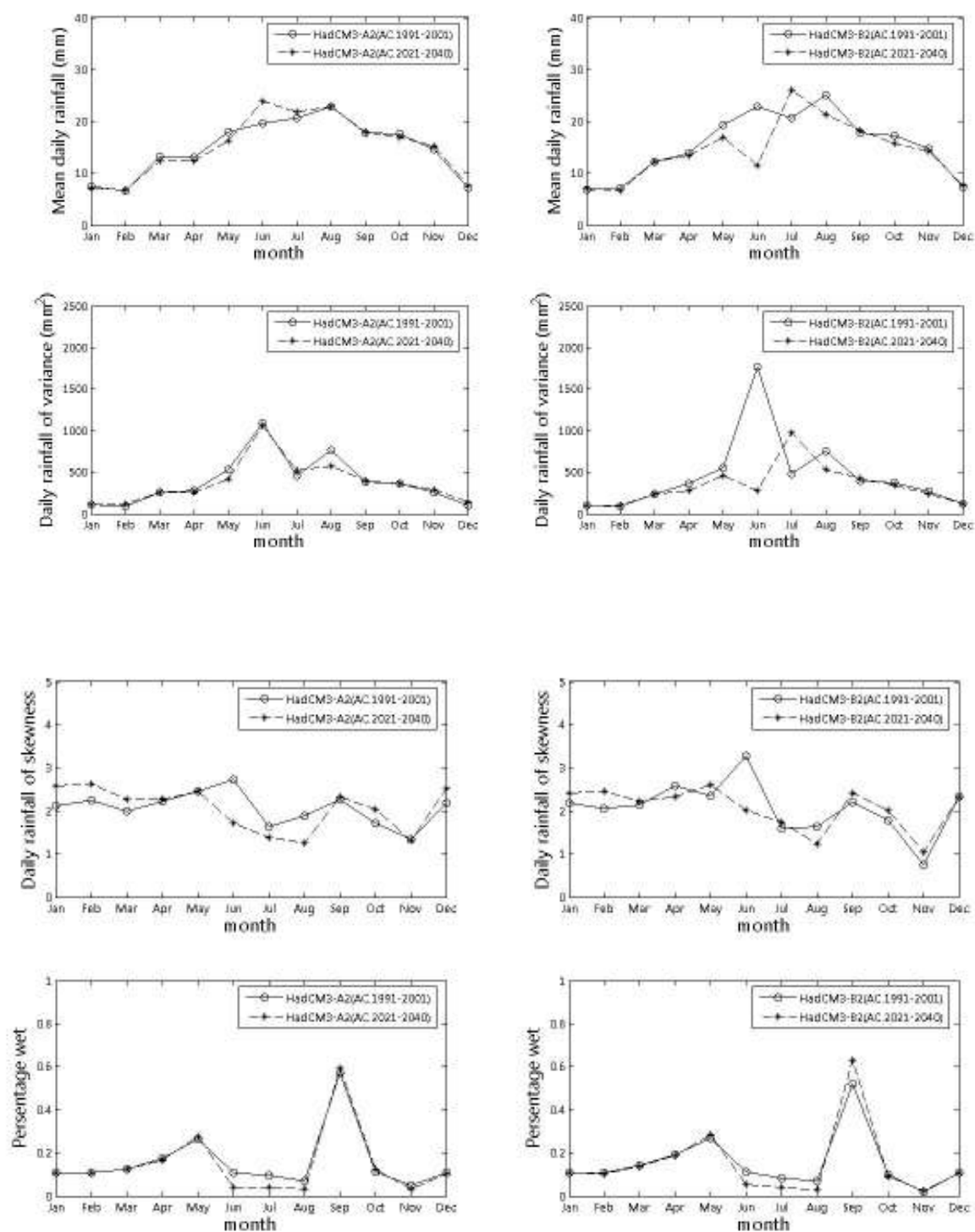
ภาพที่ ๓.3 ค่าเฉลี่ย ค่าความแปรปรวน ค่าสัมประสิทธิ์ความเบ้ และเปอร์เซ็นต์ฝนตก ที่ได้จากภาพฉาย HadCM3-A2 และ HadCM3-B2 สำหรับสถานี 05023 (ปี ค.ศ.1991-2001 และ ปี ค.ศ.2020-2040)
