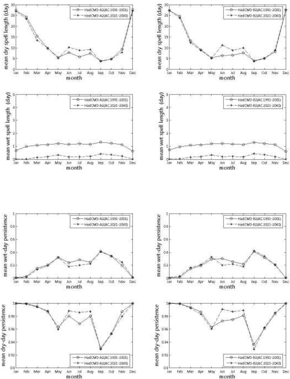
ภาพที่ ข.22 ช่วงเวลาที่ฝนไม่ตก ช่วงเวลาที่ฝนตก จำนวนครั้งสัมพัทธ์ที่ฝนตก จำนวนครั้งสัมพัทธ์ที่ฝนไม่ตกจากภาพฉาย HadCM3-A2 และ HadCM3-B2 สำหรับสถานี 14062 (ปี ค.ศ.1991-2001 และ ปี ค.ศ.2020-2040)
