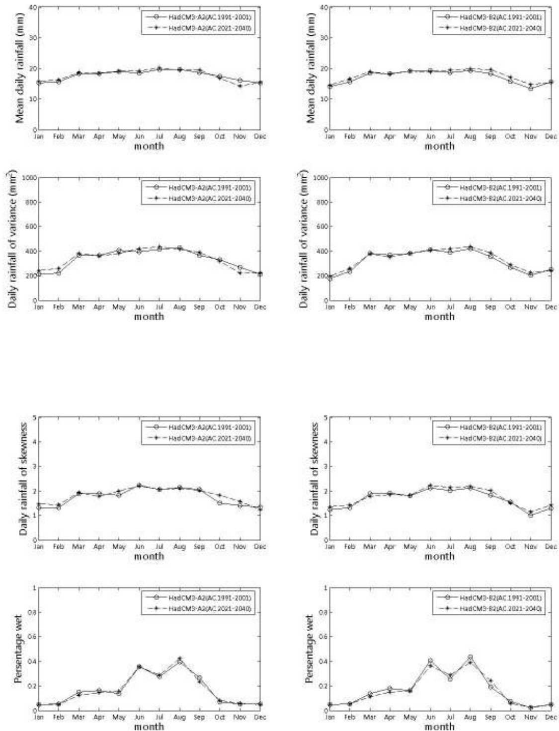
ภาพที่ ข. 69 ค่าเฉลี่ย ค่าความแปรปรวน ค่าสัมประสิทธิ์ความเบ้ และเปอร์เซ็นต์ฝนตก ที่ได้จาก ภาพฉาย HadCM3-A2 และ HadCM3-B2 สำหรับสถานี 432004 (ปี ค.ศ.1991-2001 และ ปี ค.ศ. 2020-2040)
