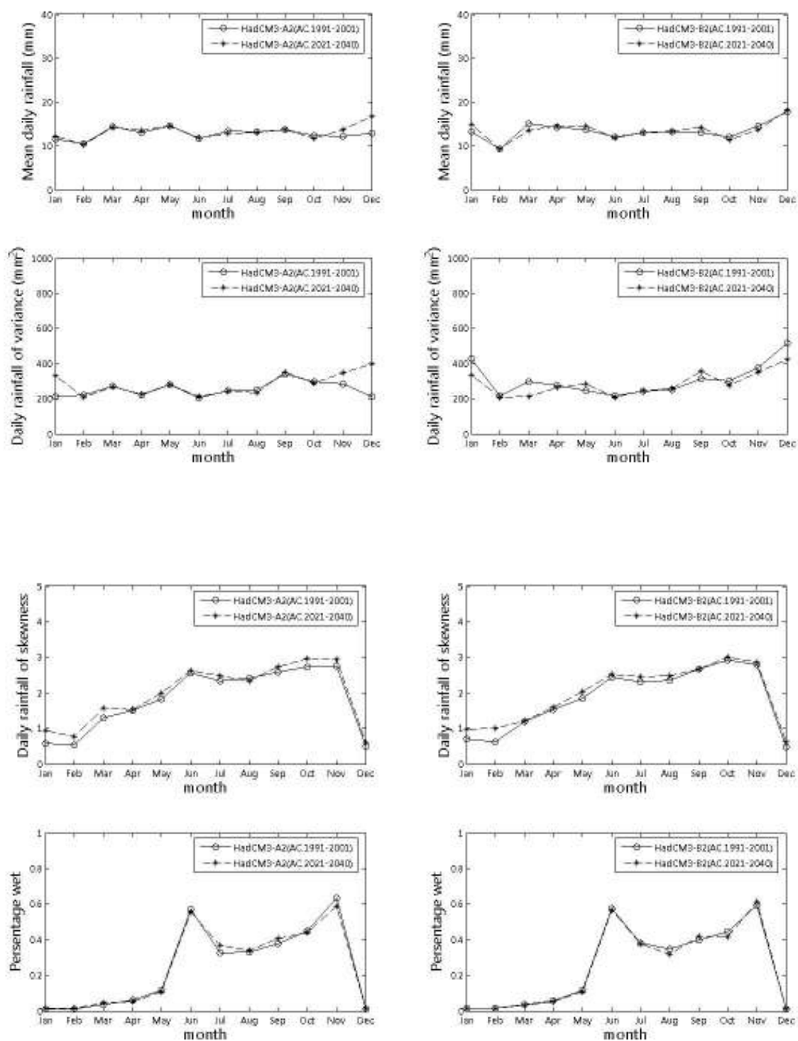
ภาพที่ ข.67 ค่าเฉลี่ย ค่าความแปรปรวน ค่าสัมประสิทธิ์ความเบ้ และเปอร์เซ็นต์ฝนตก ที่ได้จากภาพฉาย HadCM3-A2 และ HadCM3-B2 สำหรับสถานี 432001 (ปี ค.ศ.1991-2001 และ ปี ค.ศ. 2020-2040)
